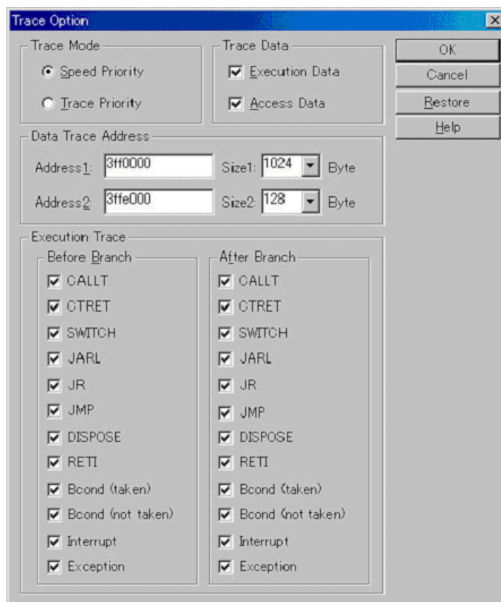
図5 - 18 トレース・データの設定
