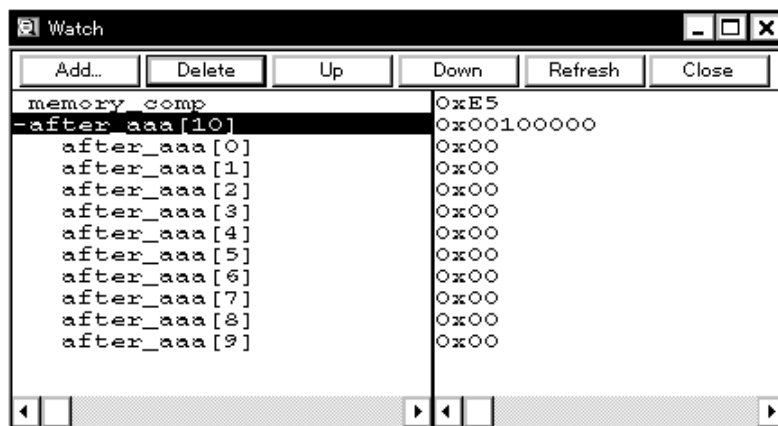
図6 - 23 ウォッチ・ウィンドウ
