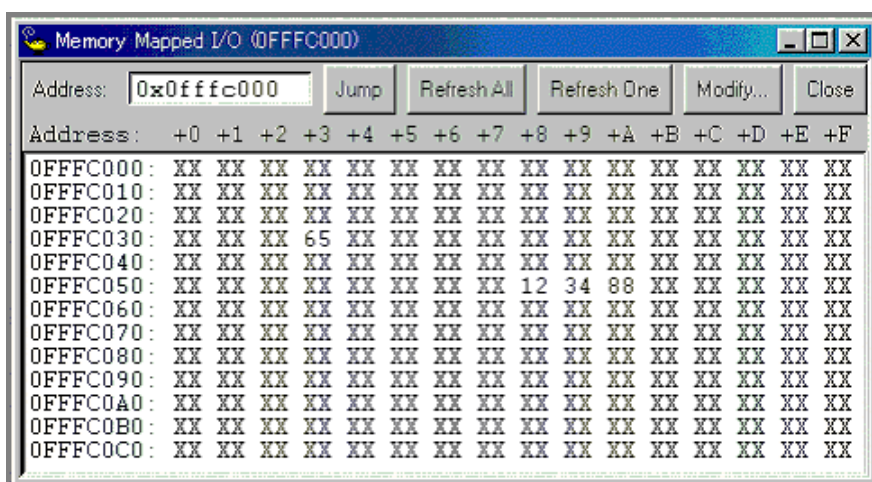
図 A - 5 Memory Mapped I/O ウィンドウ
