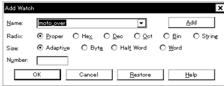
図6 - 25 ウォッチ登録ダイアログ
