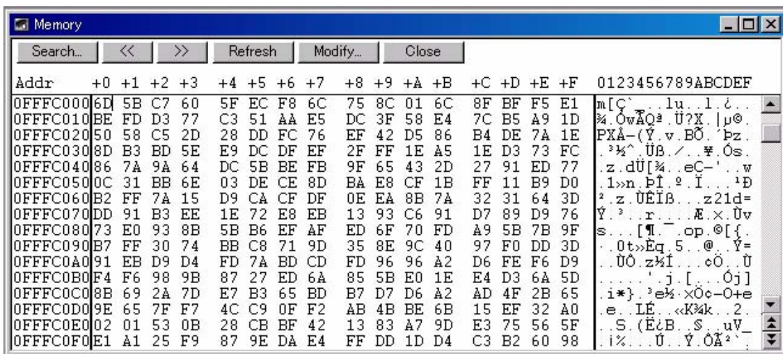
図 5 - 13 メモリ内容の表示，変更
