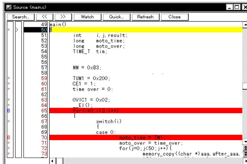
図 6 - 16 ソース・テキスト・ウィンドウ
