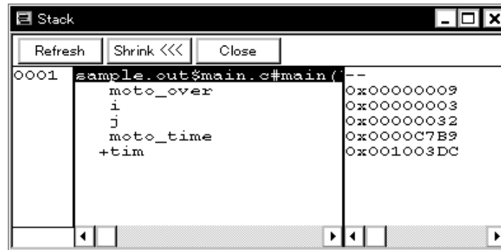
図 6 - 28 スタック・トレース・ウィンドウ
