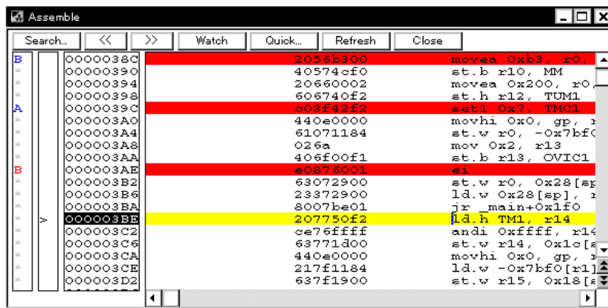
図6 - 19 逆アセンブル・ウィンドウ
