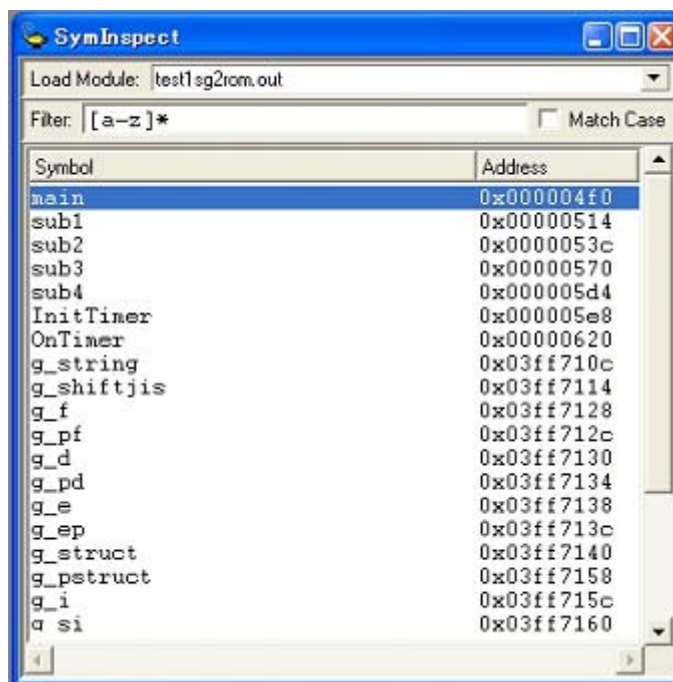
図 A - 7 Sym Inspect ウィンドウ
