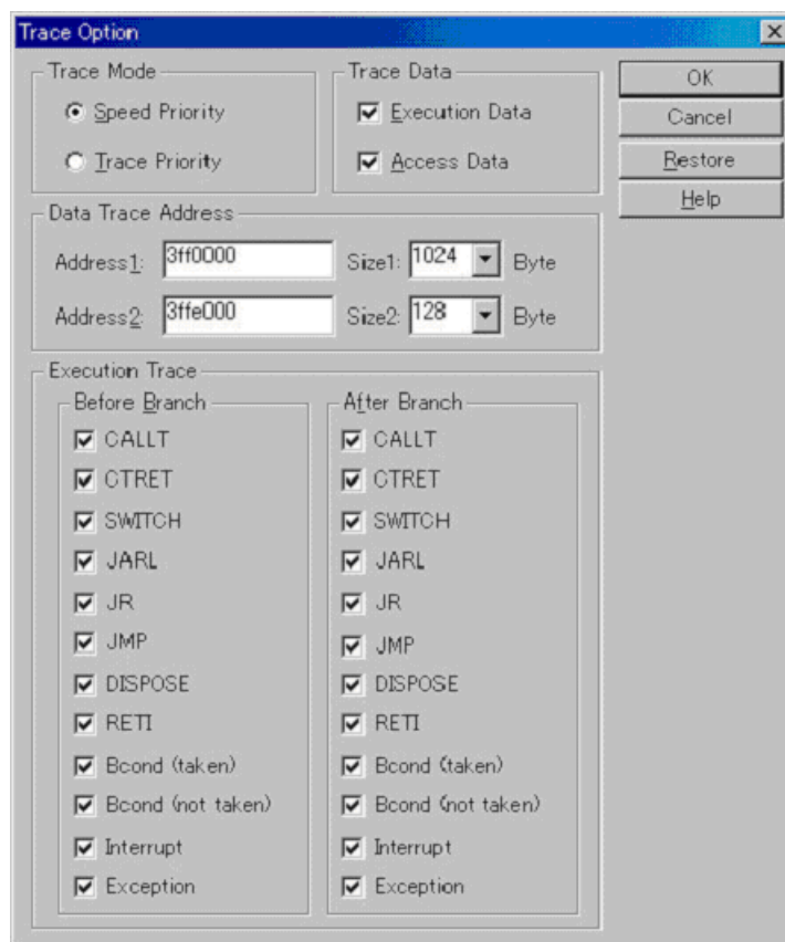
図 6 - 7 トレース・オプション設定ダイアログ
