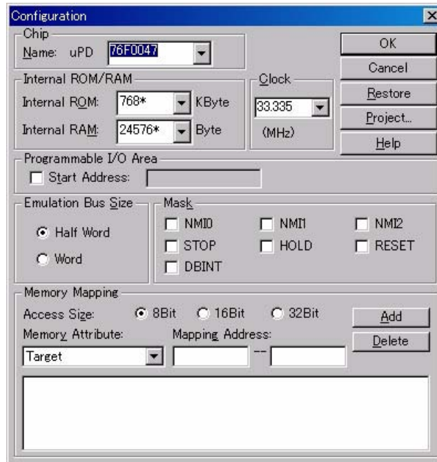
図 3 - 3 コンフィグレーション・ダイアログ
