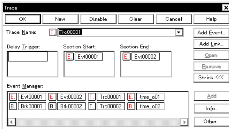
図 6 - 43 トレース・ダイアログ
