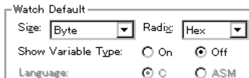
図 5 - 8 ウォッチ表示形式の指定 (ディバッガ・オプション設定ダイアログ)
