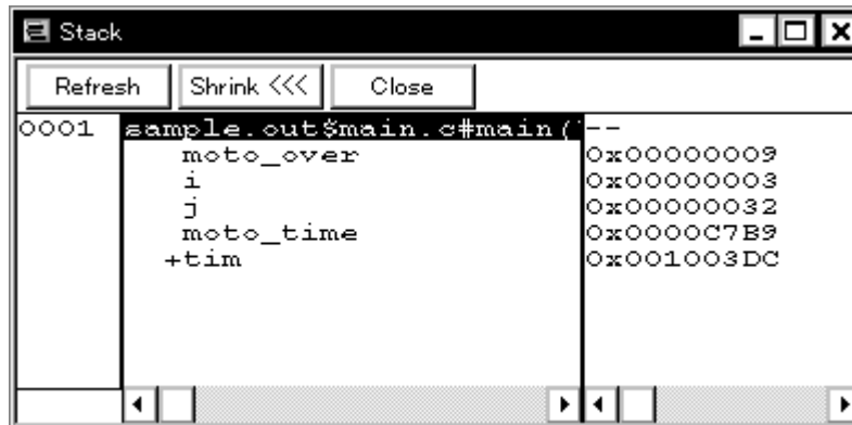
図5 - 12 スタック・トレース・ウィンドウ
