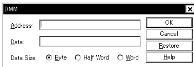
図 5 - 14 メモリ内容の書き換え (DMM ダイアログ)
