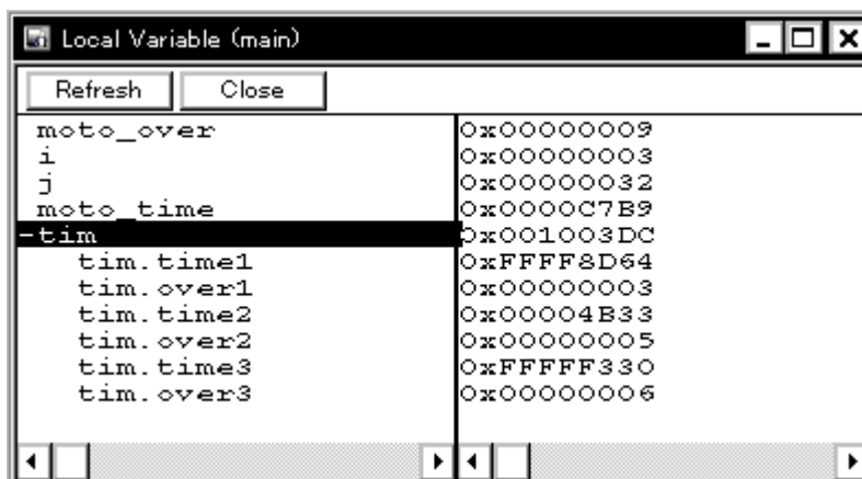
図 5 - 9 ローカル変数ウィンドウ
