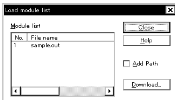
図6 - 15 ロード・モジュール一覧ダイアログ
