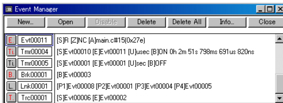
図6 - 47 イベント・マネージャ（詳細表示時）
