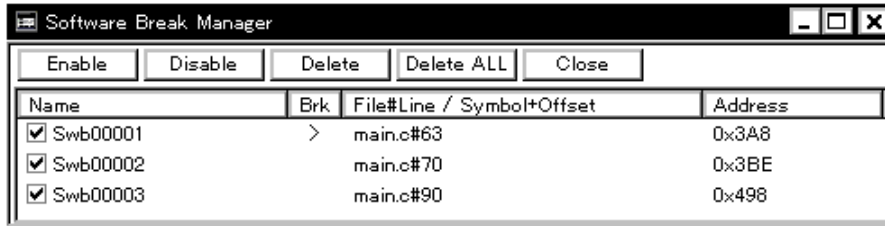
図 6 - 46 ソフトウェア・ブレーク・マネージャ
