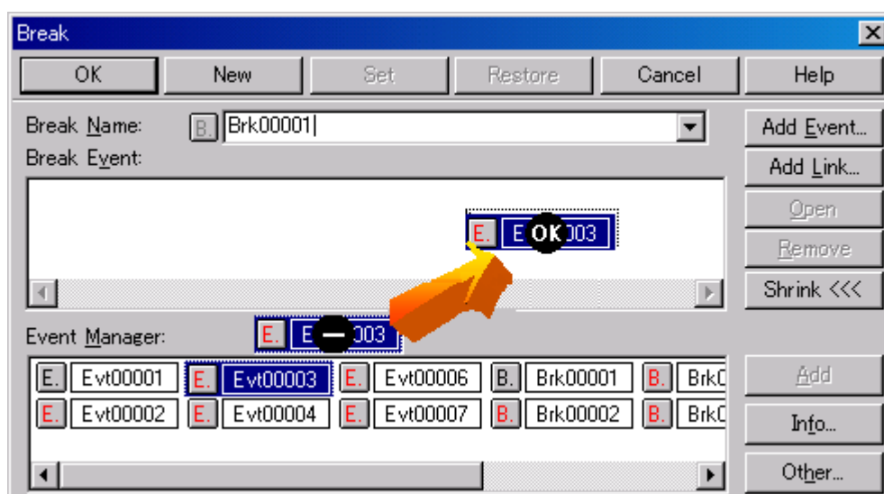
図 5 - 20 各種イベント条件の設定方法
