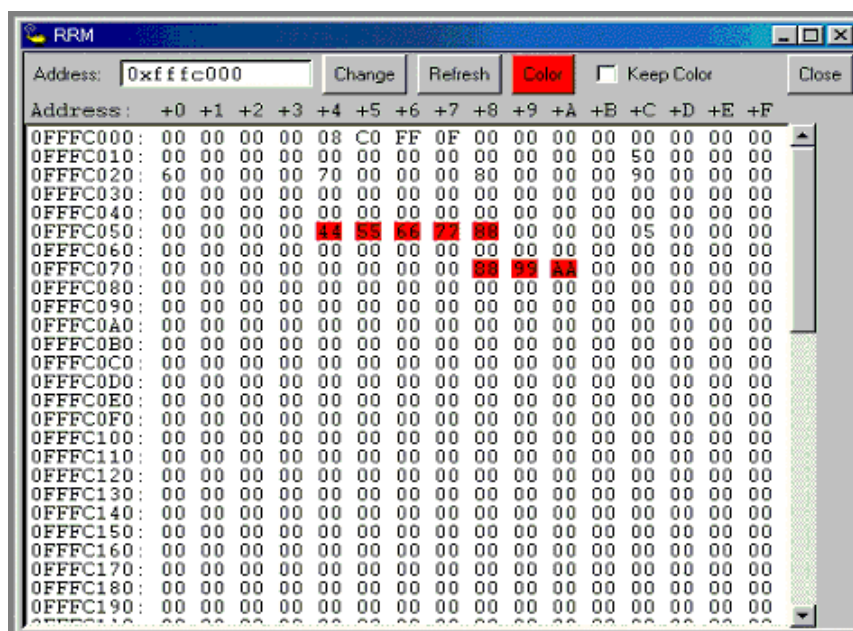
図 A - 3 RRM ウィンドウ
