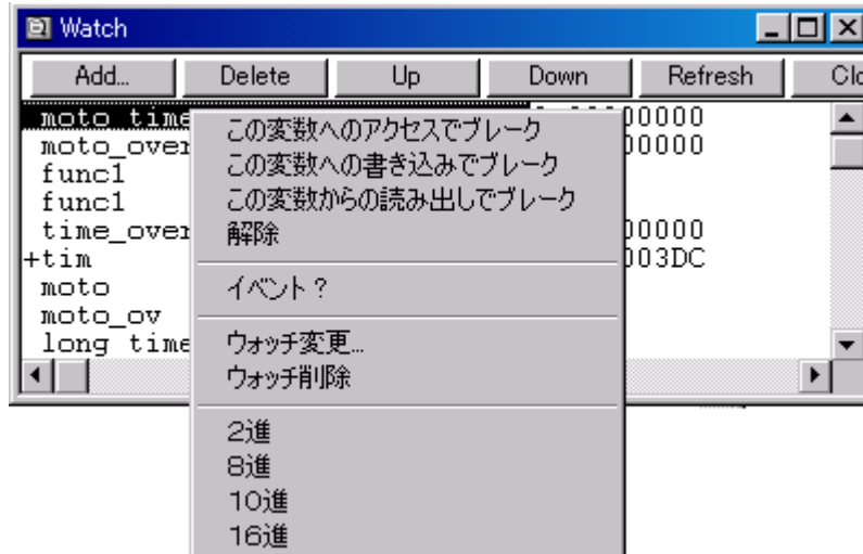
図5 - 3 変数へのブレーク設定
