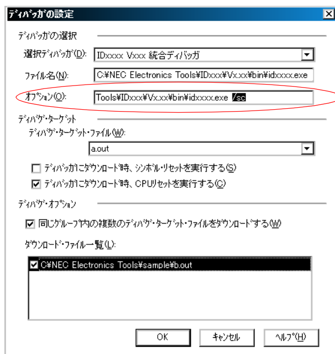
図3 - 1 [ディバッガの設定] ダイアログ (PM+)
