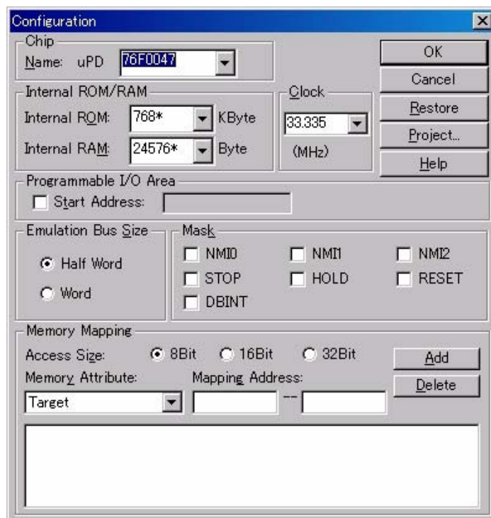
図 6 - 5 コンフィグレーション・ダイアログ
