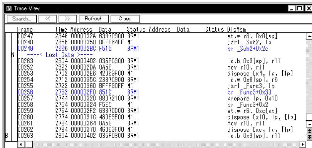
図 6 - 41 トレース・ウィンドウ
