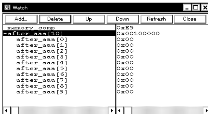
図 5 - 7 ウォッチ・ウィンドウ
