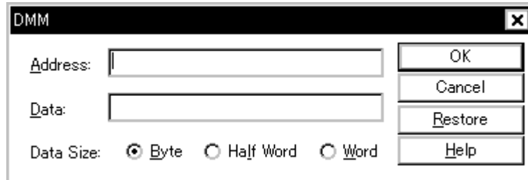
図 6 - 35 DMM ダイアログ
