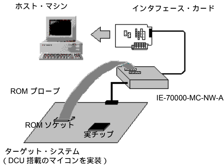
図 1 - 1 システム構成例
