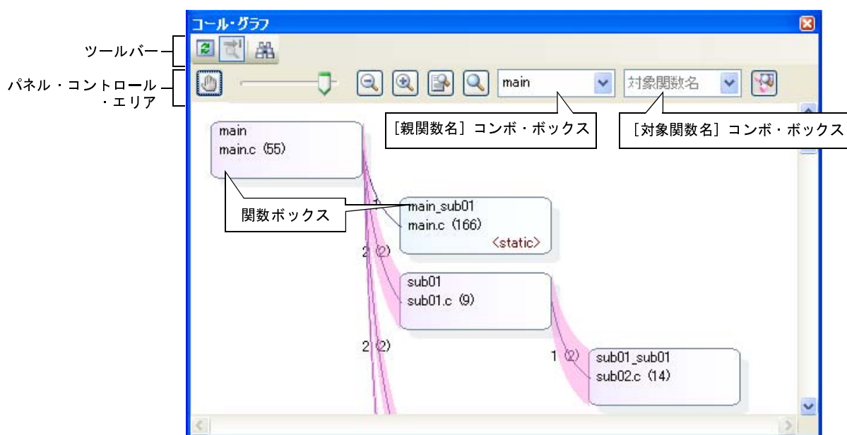
図 2—3 関数間の呼び出し関係の表示（コール・グラフパネル：全体表示）
