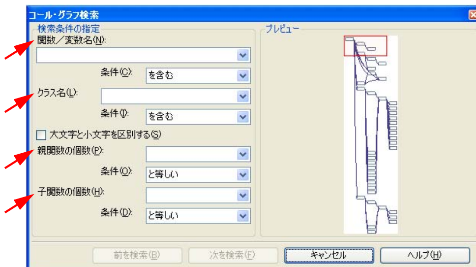
図 2—6 関数の検索（コール・グラフ検索 ダイアログ）
