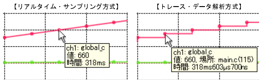
図 2—33 遷移箇所のポップアップ表示例
