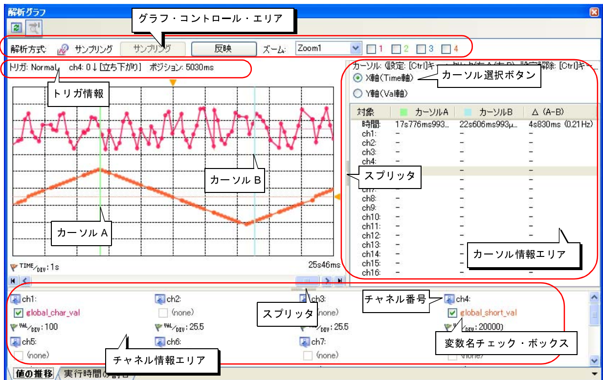
図 2-26 変数値の推移のグラフ化
