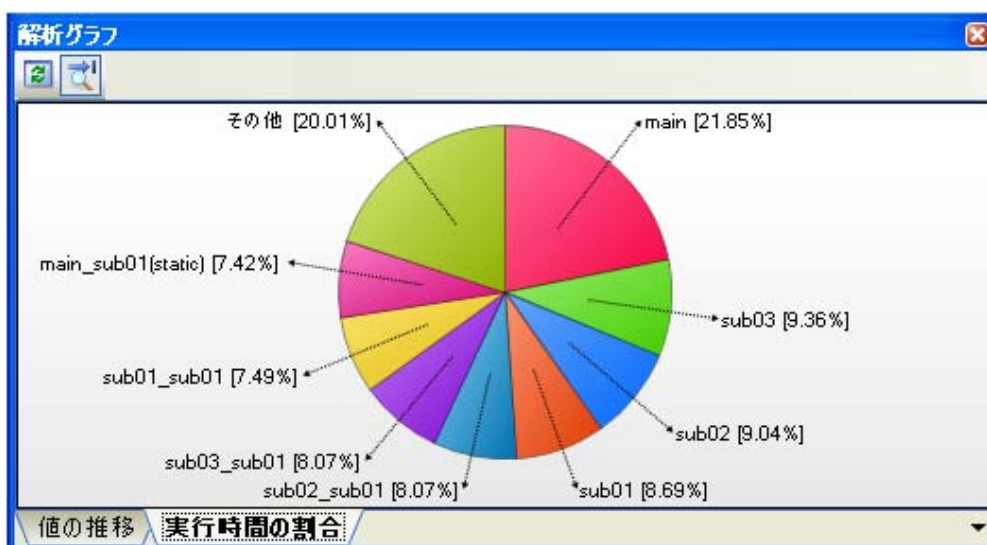
図 2—37 関数の実行時間率のグラフ化
