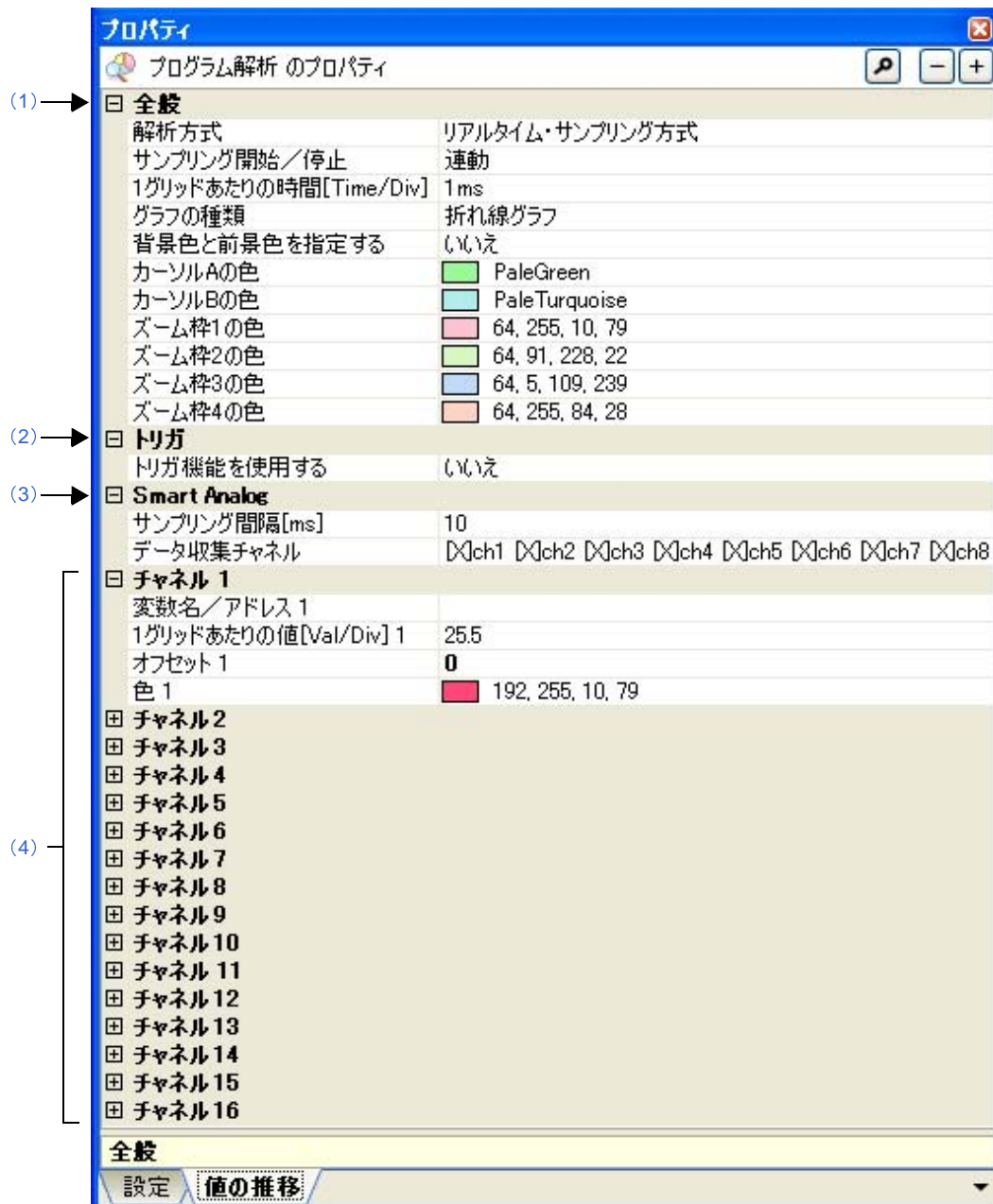
図 A—5 プロパティ パネル：[値の推移] タブ（【E1 【RL78】】の例）
