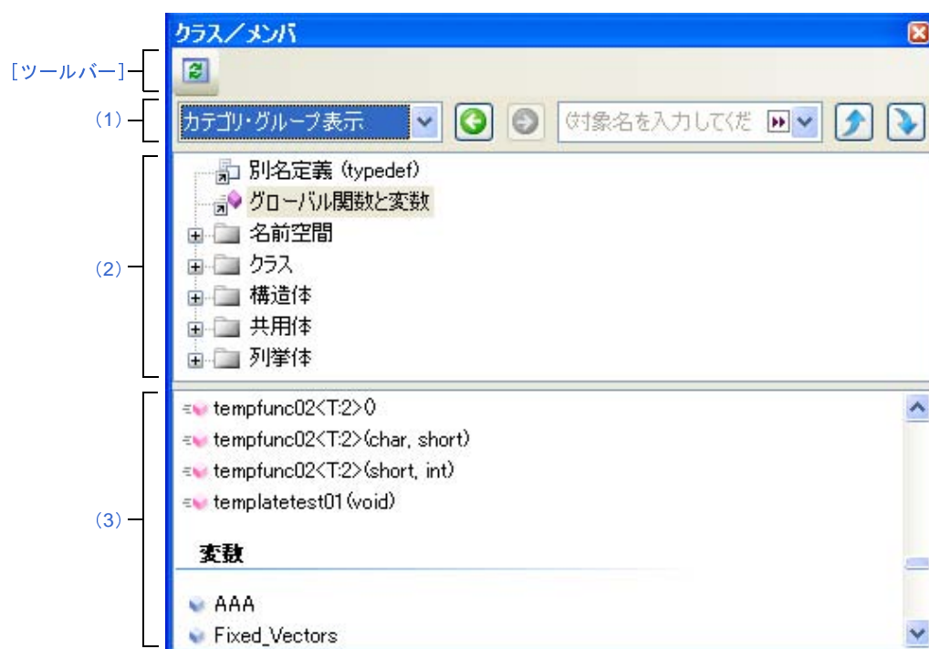
図 A—24 クラス／メンバパネル
