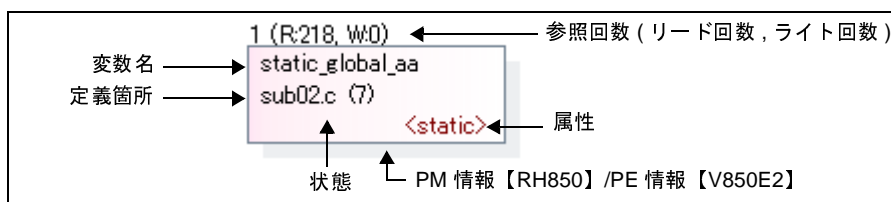
図 A—22 変数ボックスの情報
