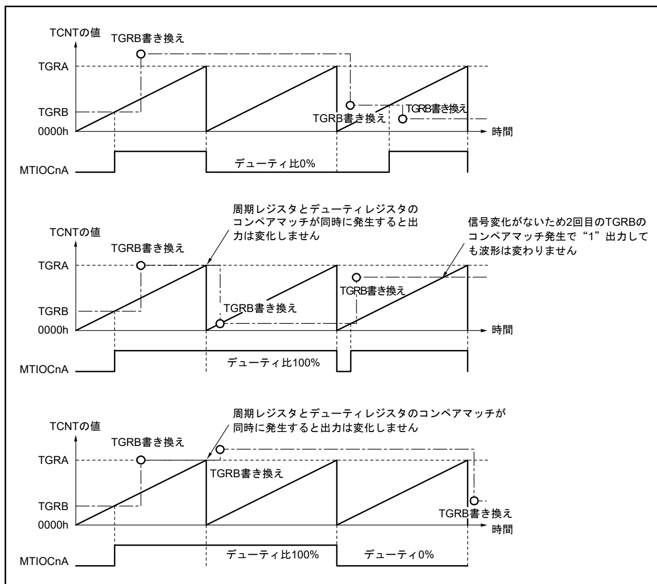
図 20.29 PWM モード動作例（デューティ0%、デューティ100%のPWM波形を出力する例） (n = 0 ~ 4, 6, 7, 9)
