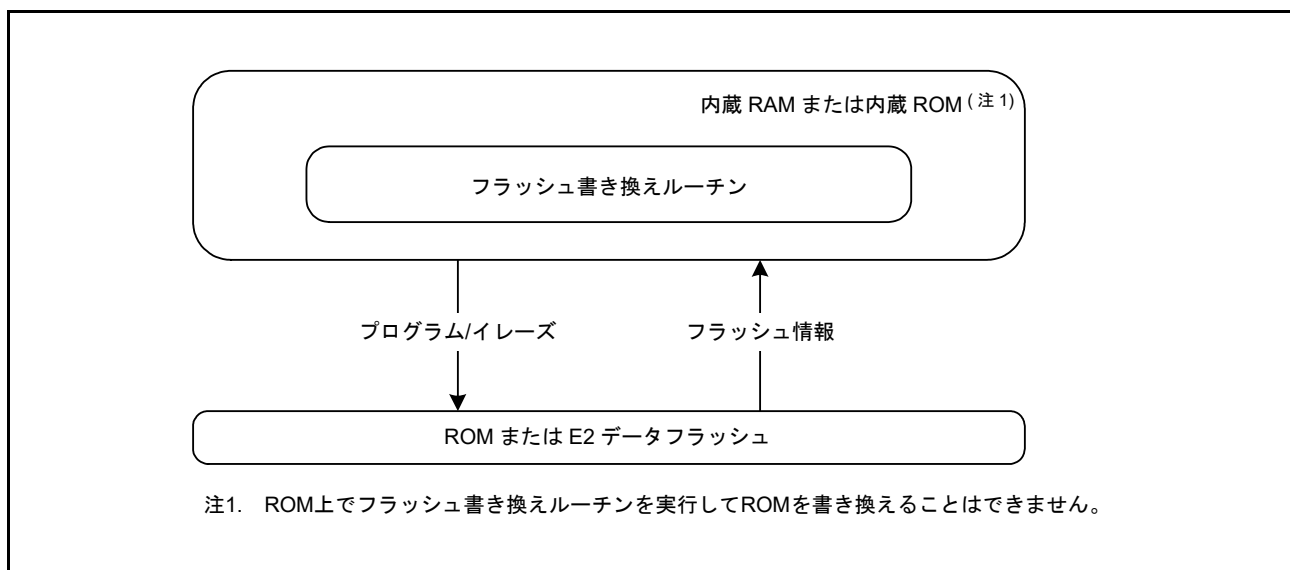
図 36.41 セルフプログラミングの概念
