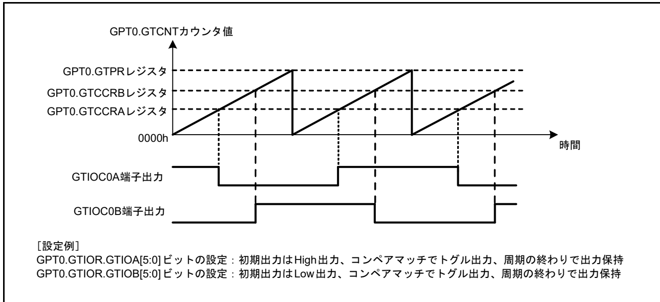
図 22.9 トグル出力動作例 (1)
