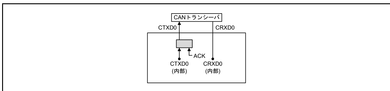
図 28.11 セルフテストモード0 選択時の接続
