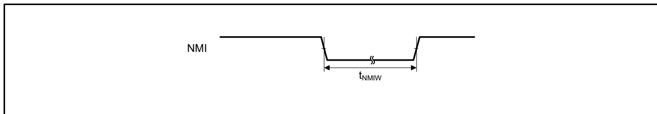
図 37.32 NMI 割り込み入カタイミング
