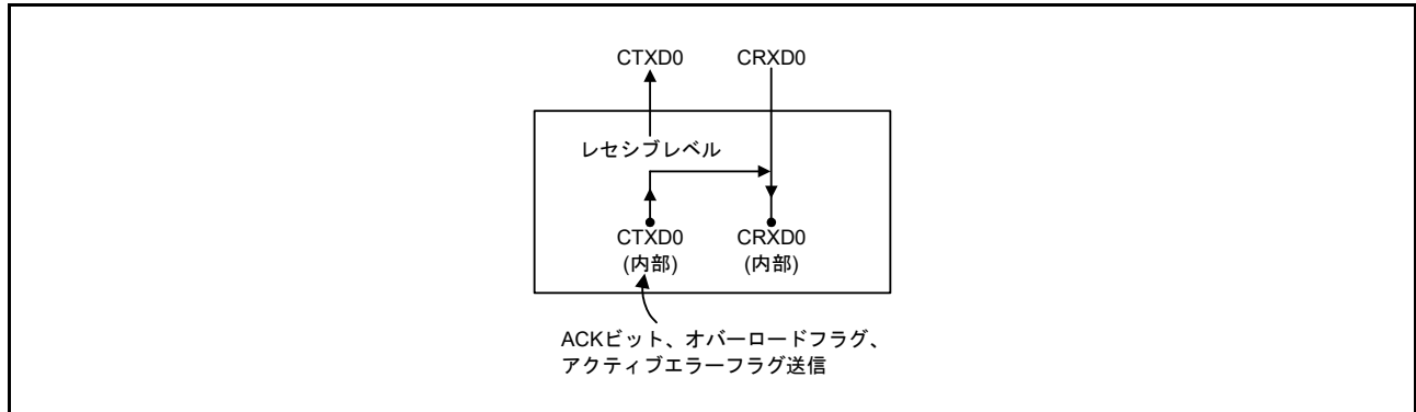
図 28.10 リッスンオンリモード選択時の接続
