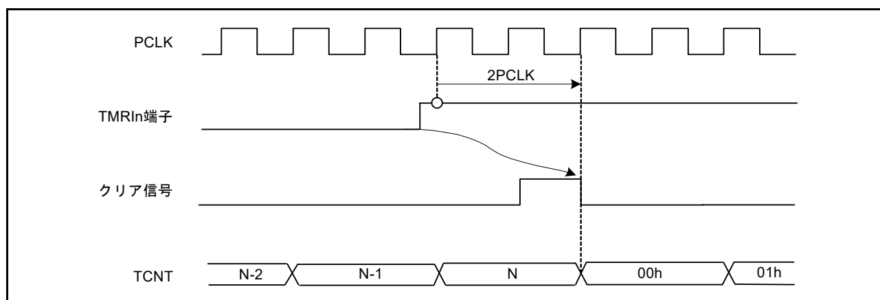
図 23.12 外部カウンタリセット信号によるクリアタイミング (立ち上がりエッジ)
