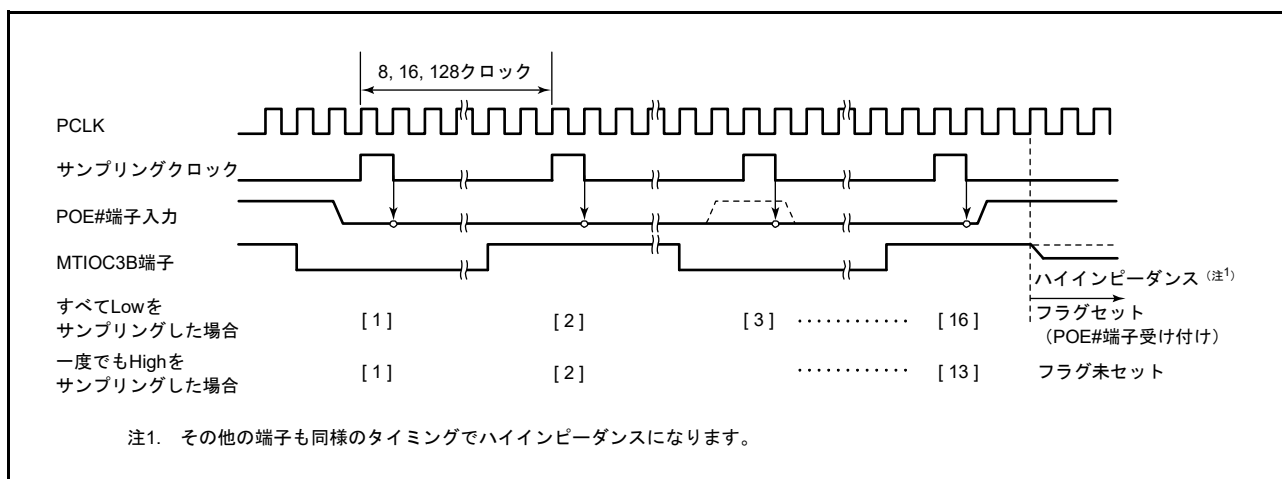
図 21.8 Low 検出、ハイインピーダンスを選択した場合の動作
