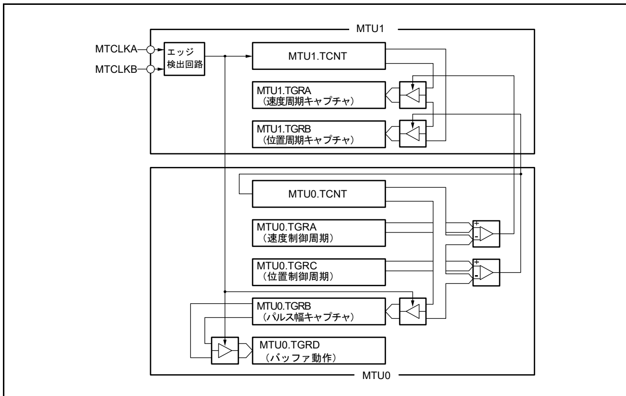
図 20.41 16ビット位相計数モードの応用例
