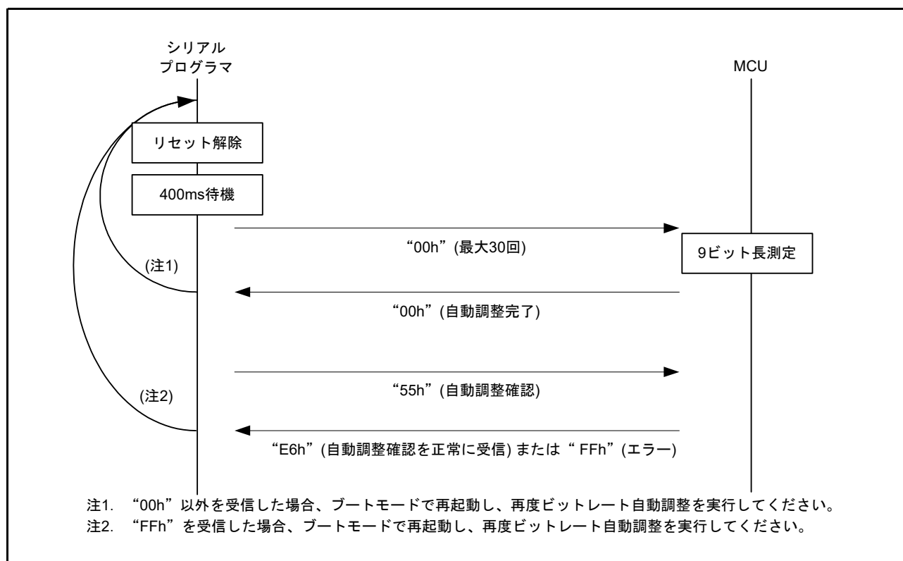
図 36.31 ビットレート自動調整の手順
