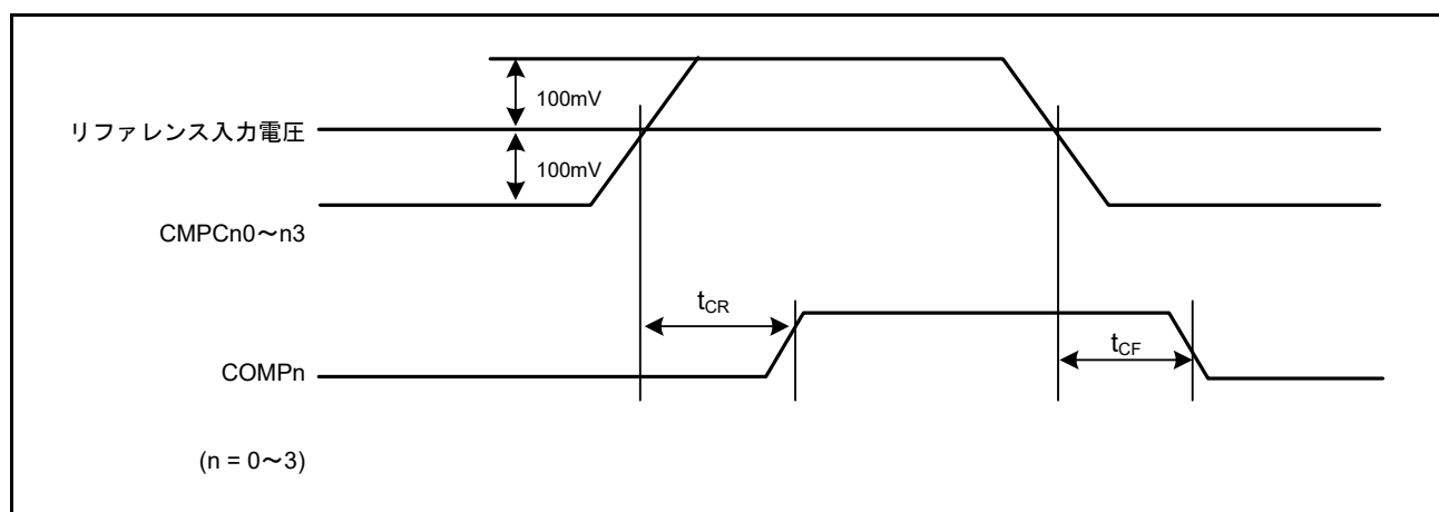
図 37.52 コンパレータ応答時間
