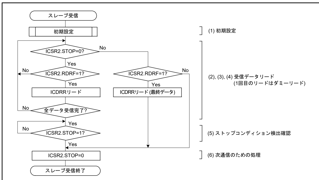
図 27.18 スレーブ受信のフローチャート例
