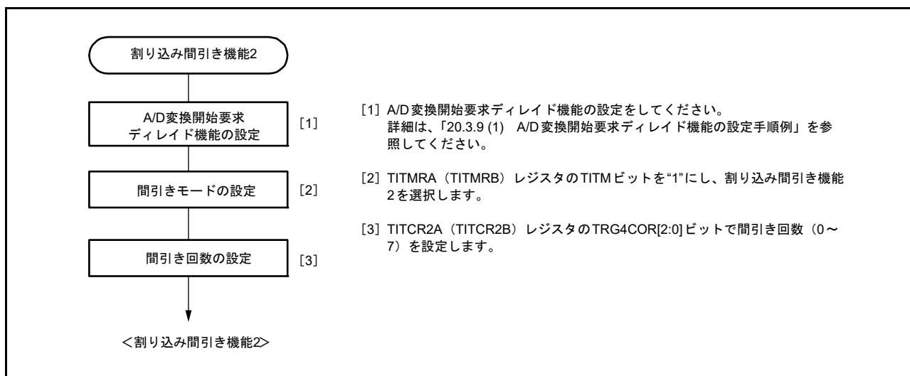
図 20.96 割り込み間引き機能2の設定手順例
