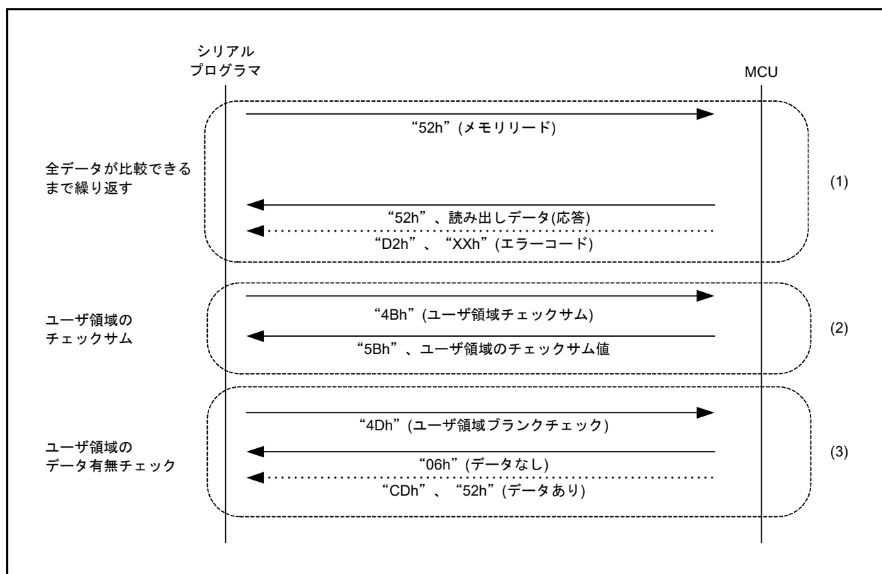
図 36.38 ユーザ領域のデータ確認手順
