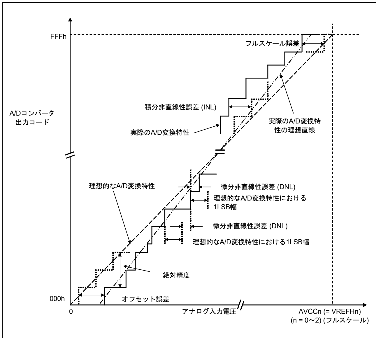
図 37.51 A/D コンバータ特性用語説明図
