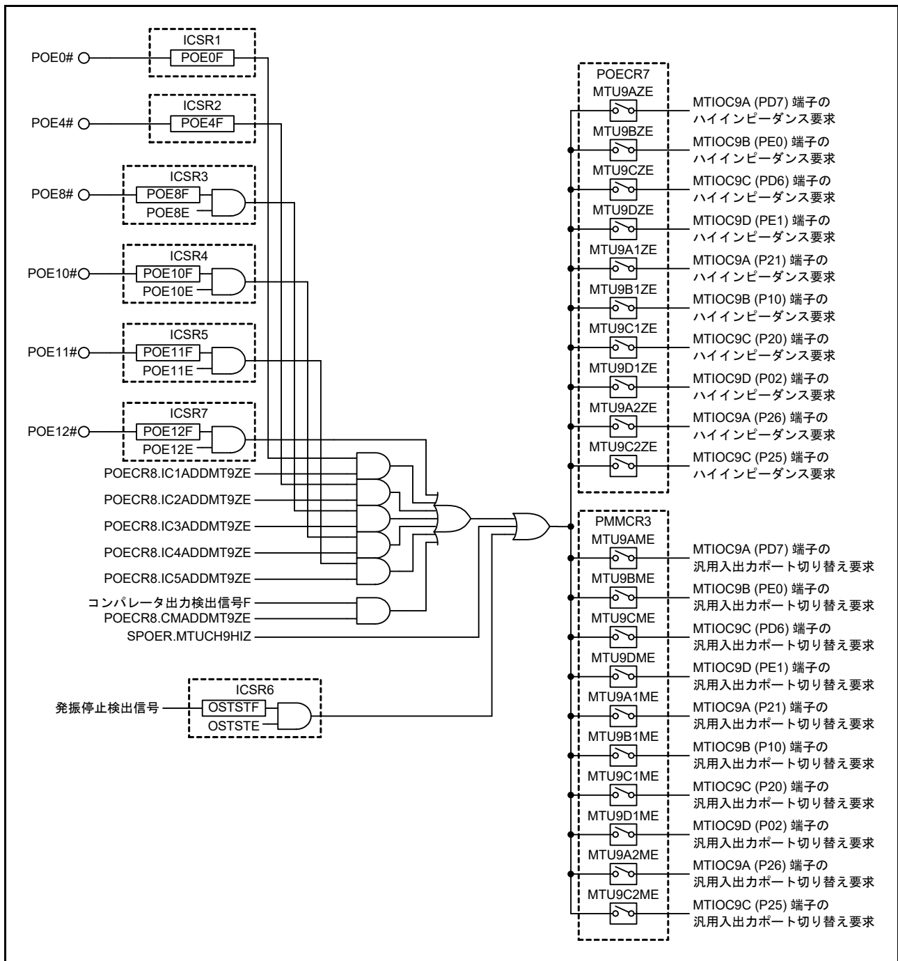
図 21.5 ハイインピーダンス制御の対象と条件 (4)
