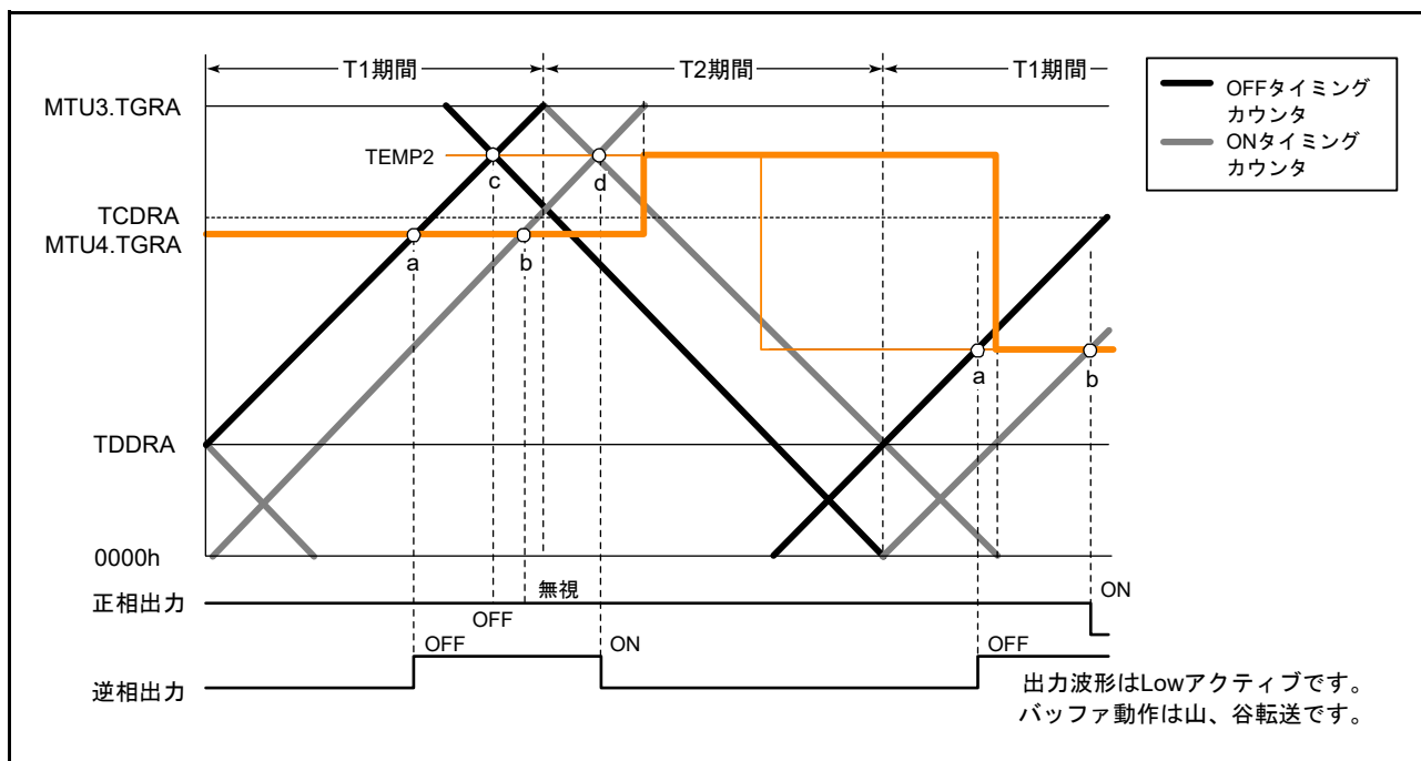
図 20.56 相補 PWM モード波形出力例 (MTU3, MTU4) (2)
