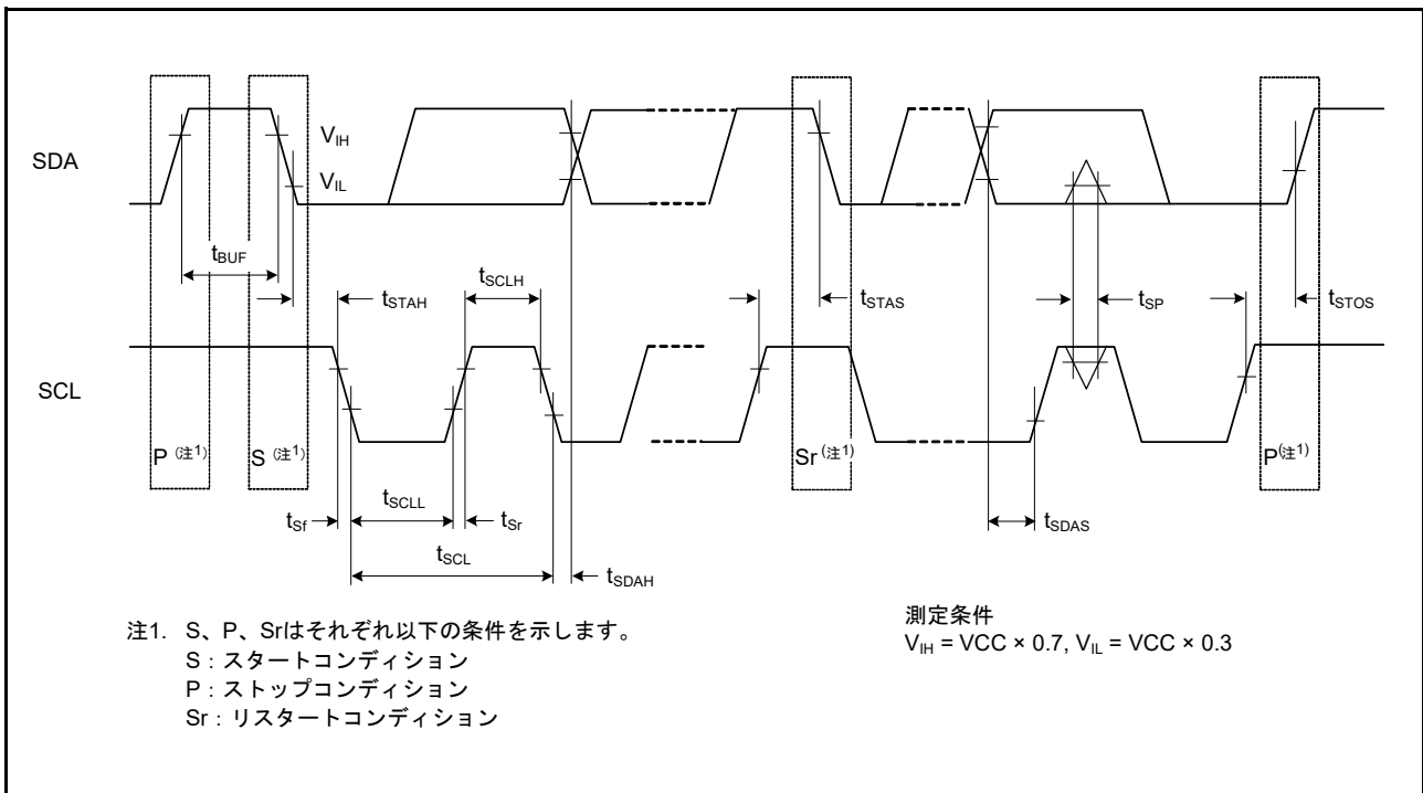
図 37.50 I 2 C バスインタフェース入出力タイミング / 簡易 I 2 C バスインタフェース入出力タイミング
