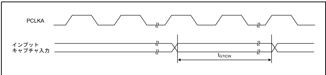
図 37.38 GPT インプットキャプチャ入力タイミング
