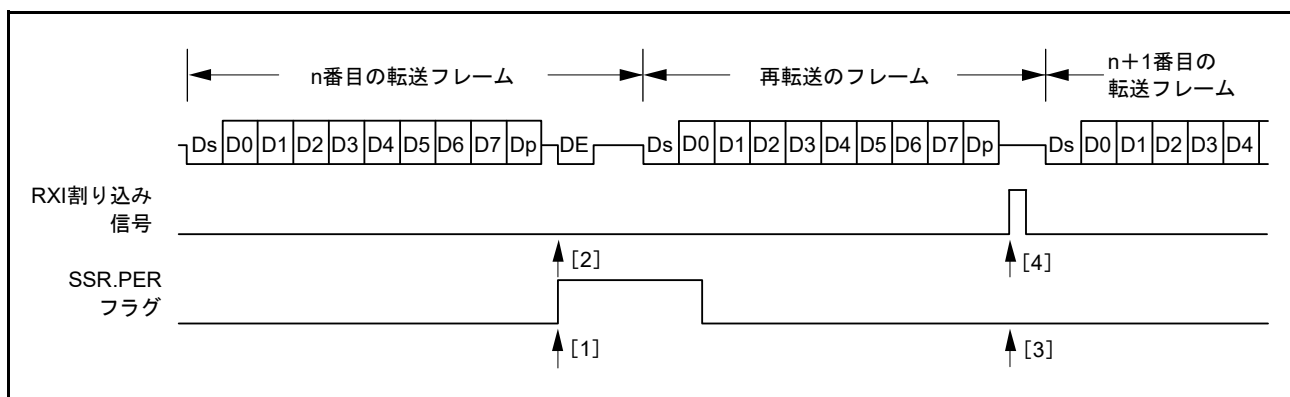
図 26.40 SCI 受信モードの場合の再転送動作（受信時の再転送動作）
