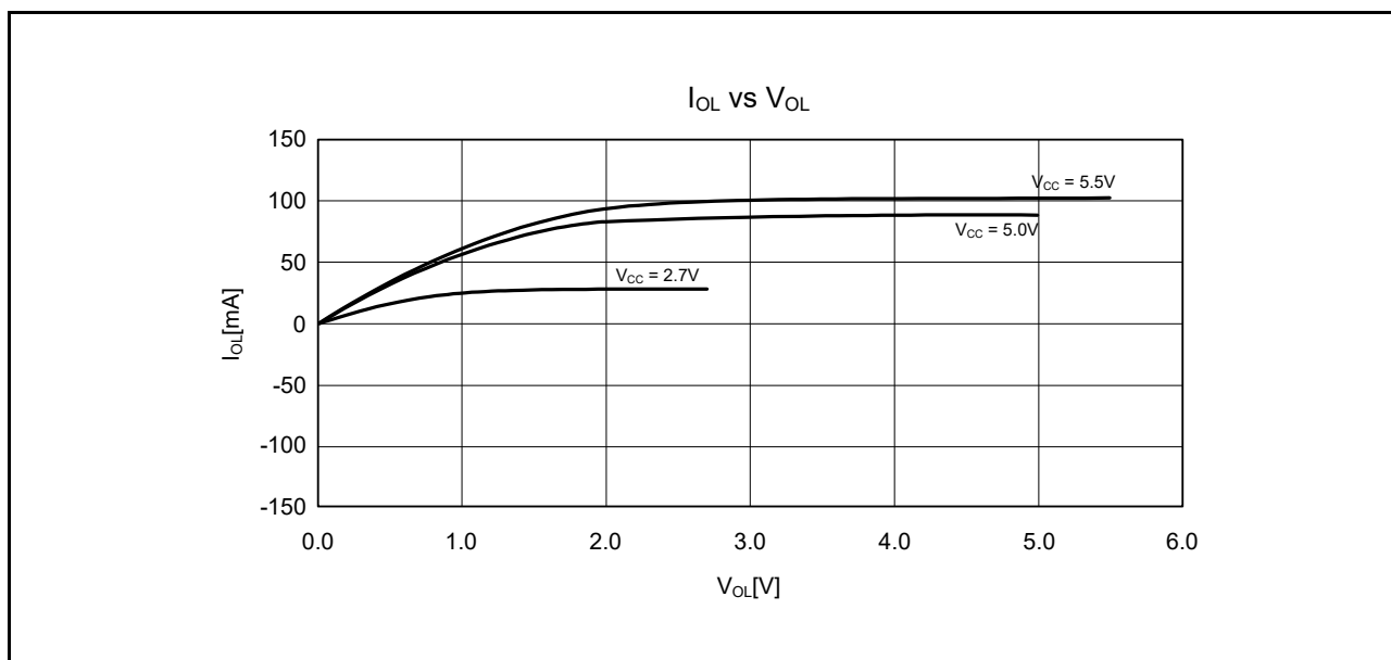
図 37.16 RIIC 出力端子の V_{OL} 、 I_{OL} 電圧特性 T_a = 25^\circ\text{C} (参考データ)
