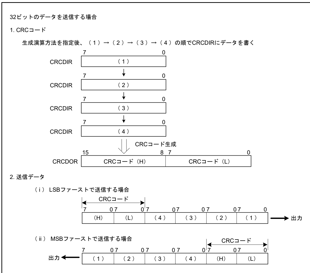
図 30.6 LSBファーストとMSBファーストの送信データ
