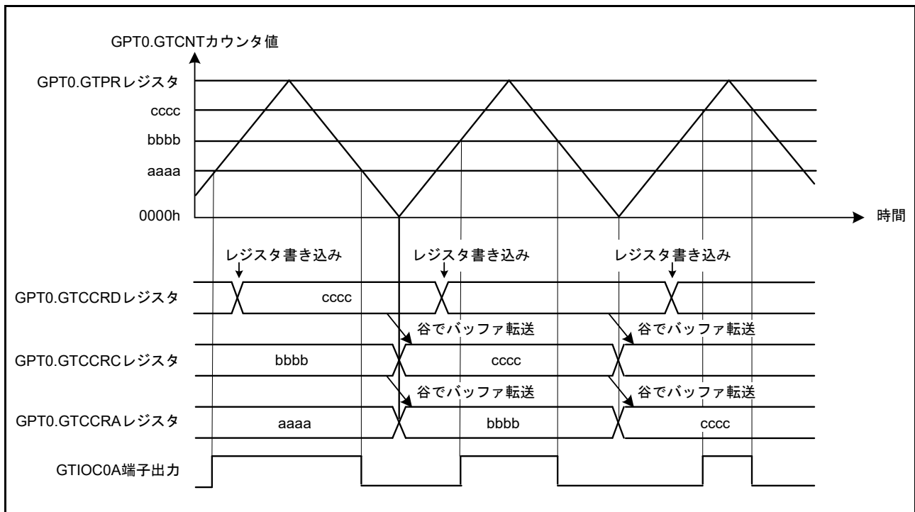
図 22.19 GTCCRA, GTCCRB レジスタのダブルバッファ動作例 (アウトプットコンペア、三角波、谷でバッファ転送、GTCCRA コンペアマッチでトグル出力、 周期の終わりで出力保持の場合)
