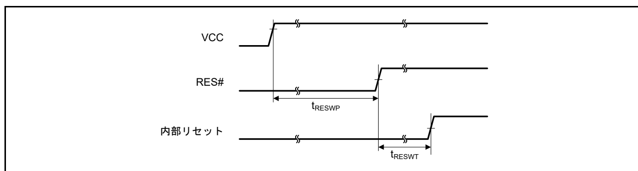
図 37.27 電源投入時リセット入力タイミング
