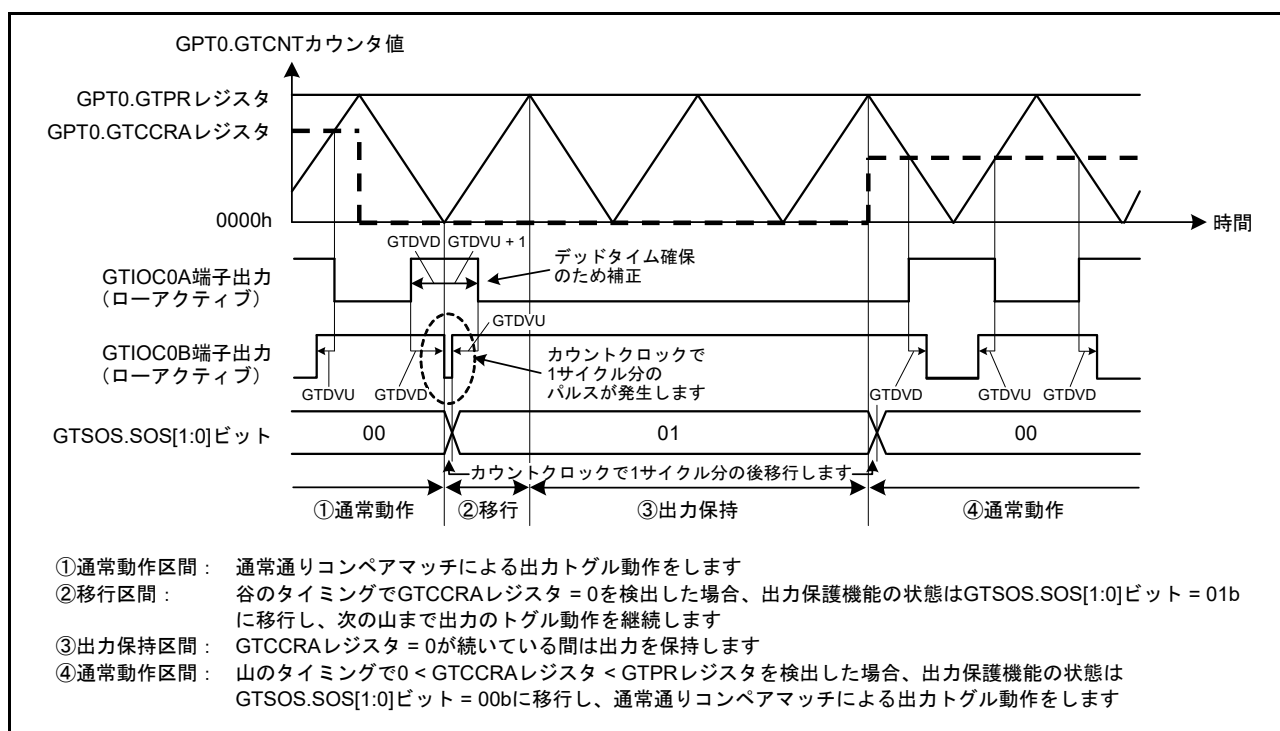
図 22.87 山のバッファ転送で GTCRA レジスタが“0000h”である場合の出力保護機能の動作例 (山のバッファ転送で 0 < \text{GTCRA レジスタ} < \text{GTPR レジスタ} に復帰、アクティブレベルは Low の場合)
