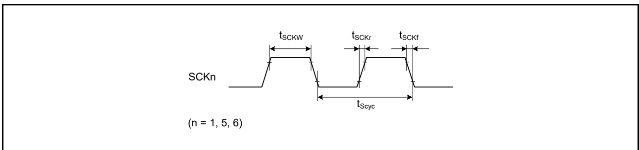
図 37.42 SCK クロック入力タイミング
