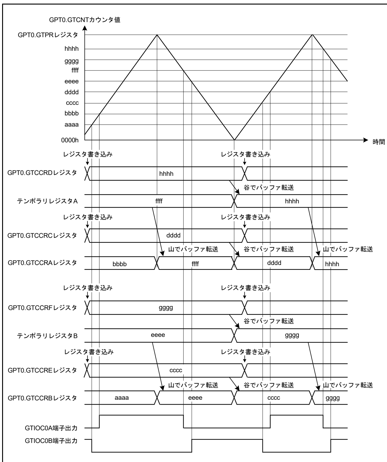
図 22.37 三角波 PWM モード 3 動作例 (初期出力で GTIOC0A 端子 = Low 出力 /GTIOC0B 端子 = High 出力、GTCCRA/GTCCRB レジスタのコンペアマッチでトグル出力、周期の終わりで出力保持の場合)
