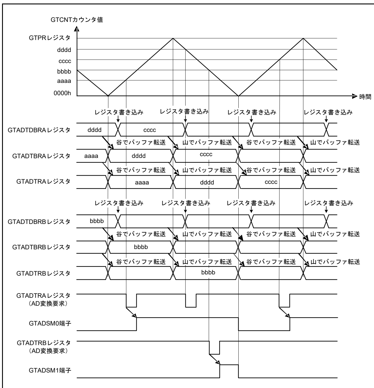
図 22.79 A/D 変換開始要求の動作例 (三角波、ダブルバッファ動作、谷 / 山両方でバッファ転送、GTADTRA0 レジスタはアップカウンタ / ダウンカウンタ両方で A/D 変換開始要求、GTADTRB0 レジスタはダウンカウンタで A/D 変換開始要求を発生の場合)
