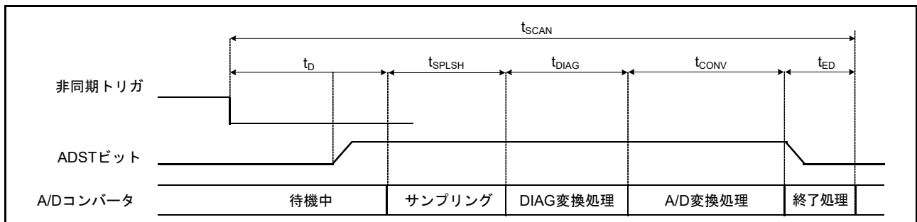
図 31.30 スキャン変換のタイミング (非同期トリガ起動の場合)
