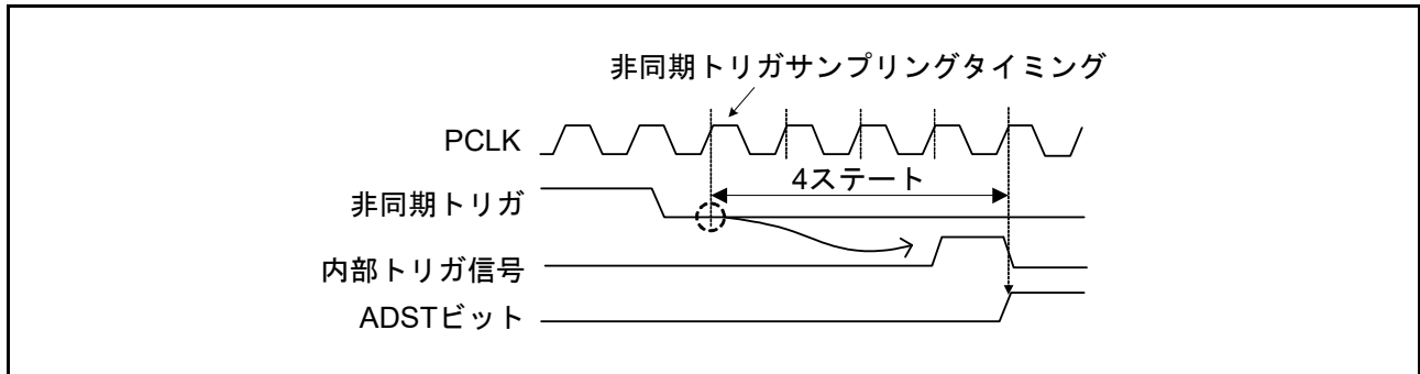
図 31.34 非同期トリガ入力タイミング
