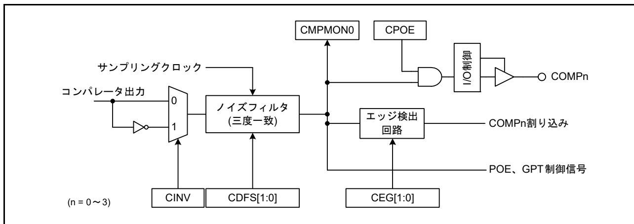
図 33.3 ノイズフィルタとエッジ検出回路の構成
