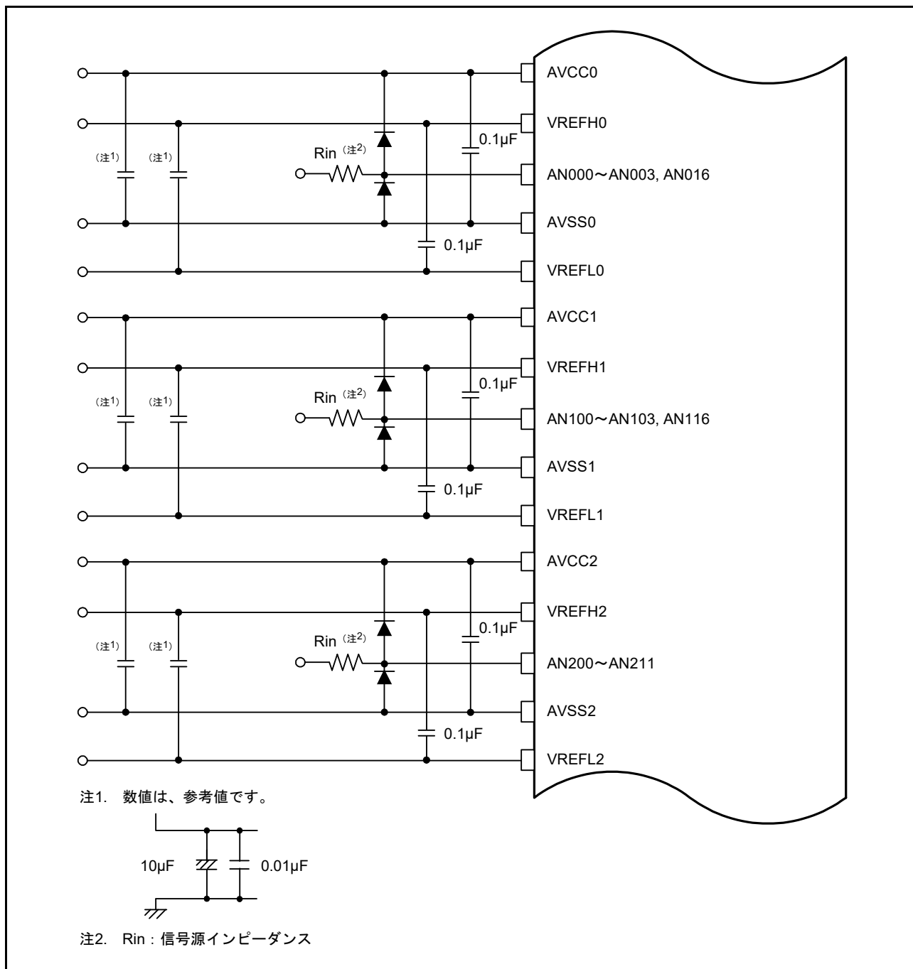
図 31.38 アナログ入力保護回路の例
