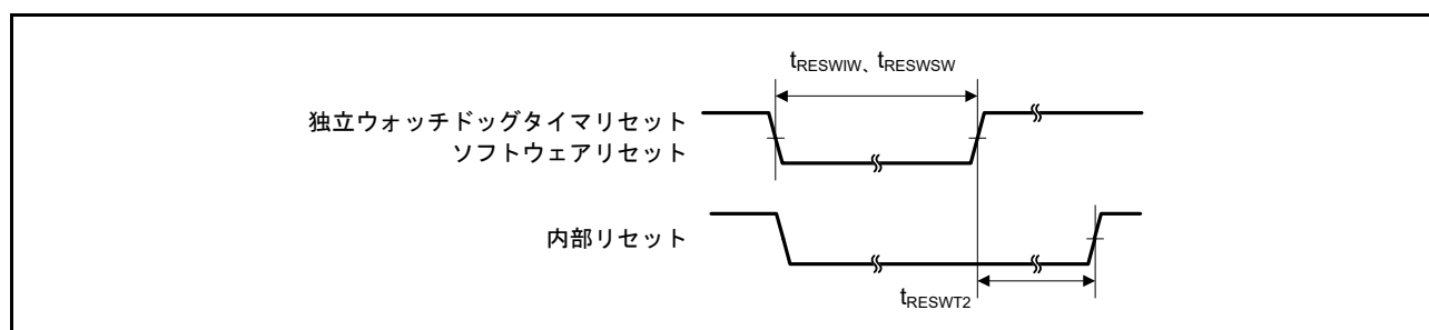
図 37.29 リセット入力タイミング (2)
