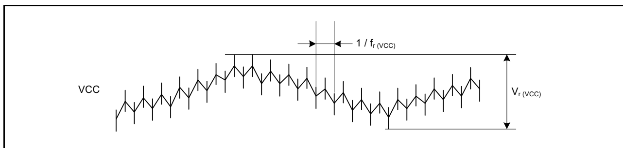
図 37.3 電源リップル波形
