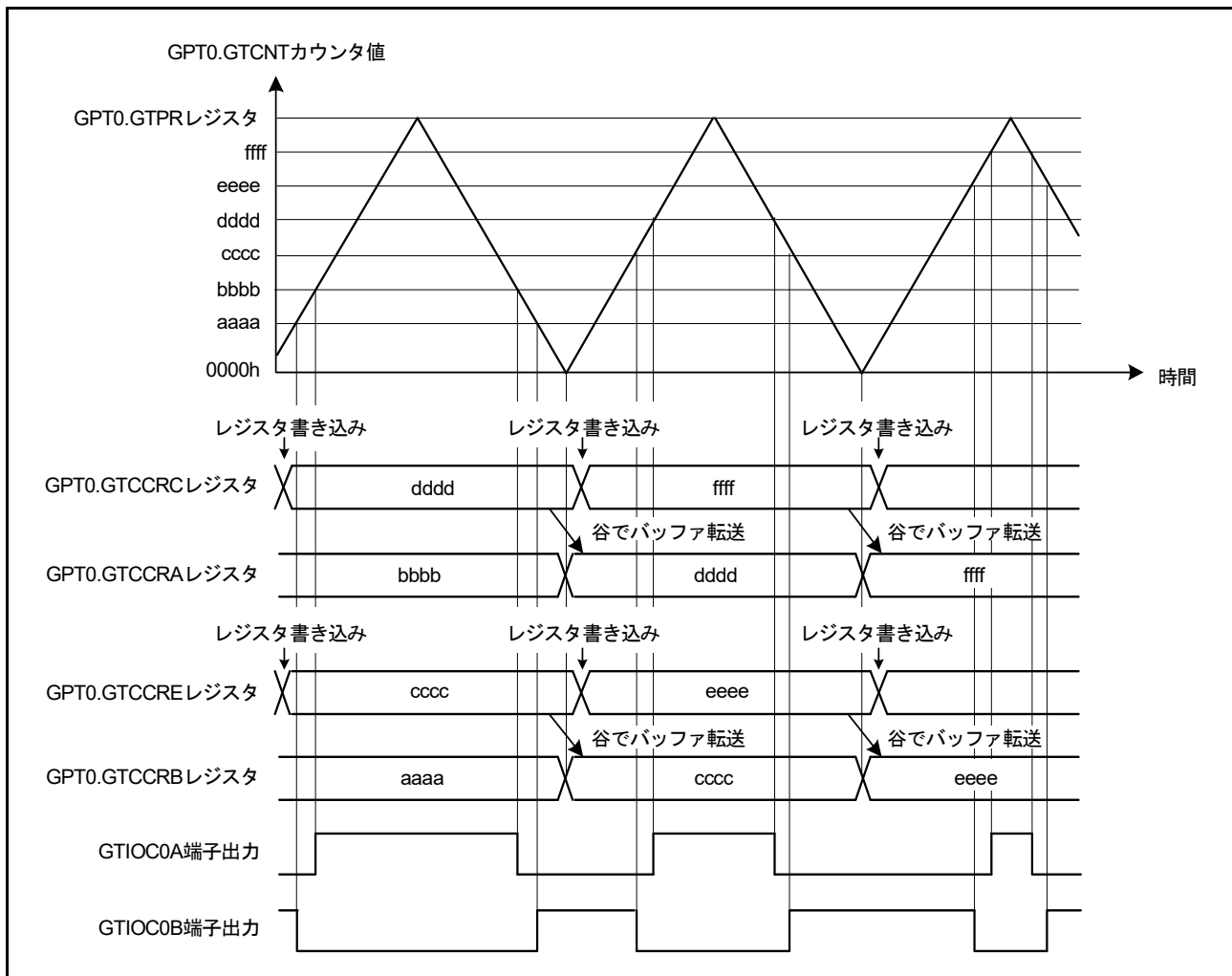
図 22.33 三角波 PWM モード 1 動作例
