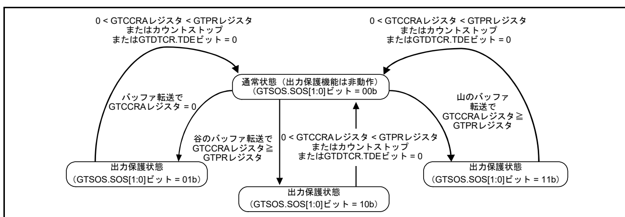
図 22.83 出力保護機能
