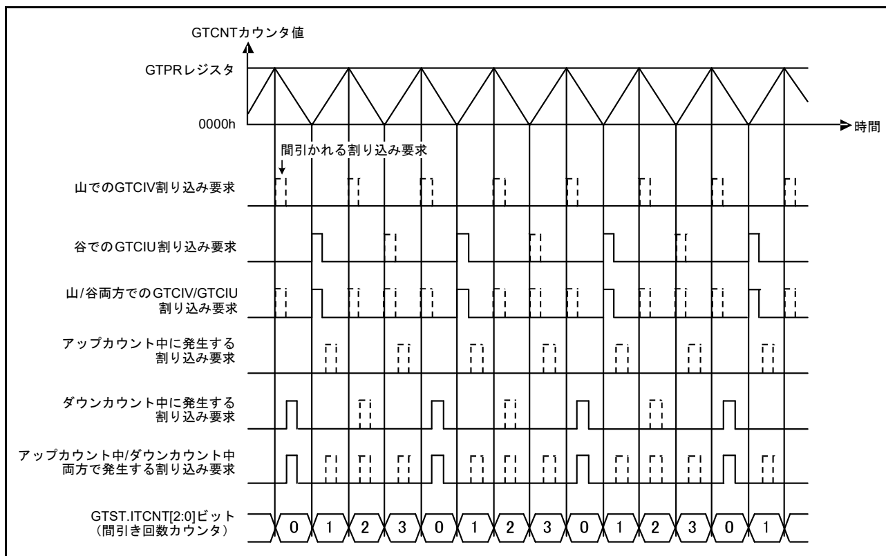
図 22.76 割り込み間引き機能の動作例 (三角波、谷 / 山両方をカウントして間引き、間引き回数 3、アップカウントで間引き開始の場合)
