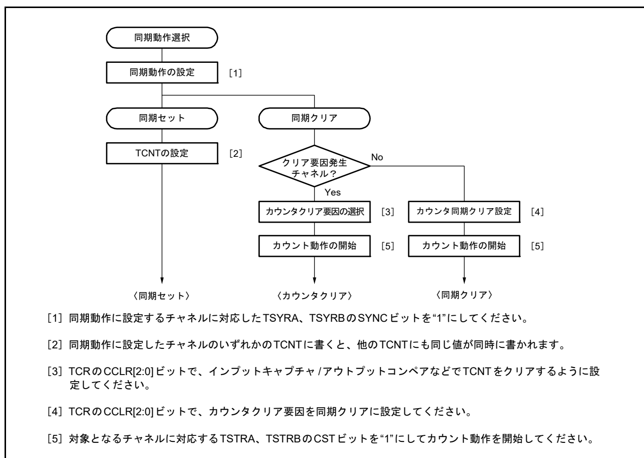
図 20.13 同期動作の設定手順例
