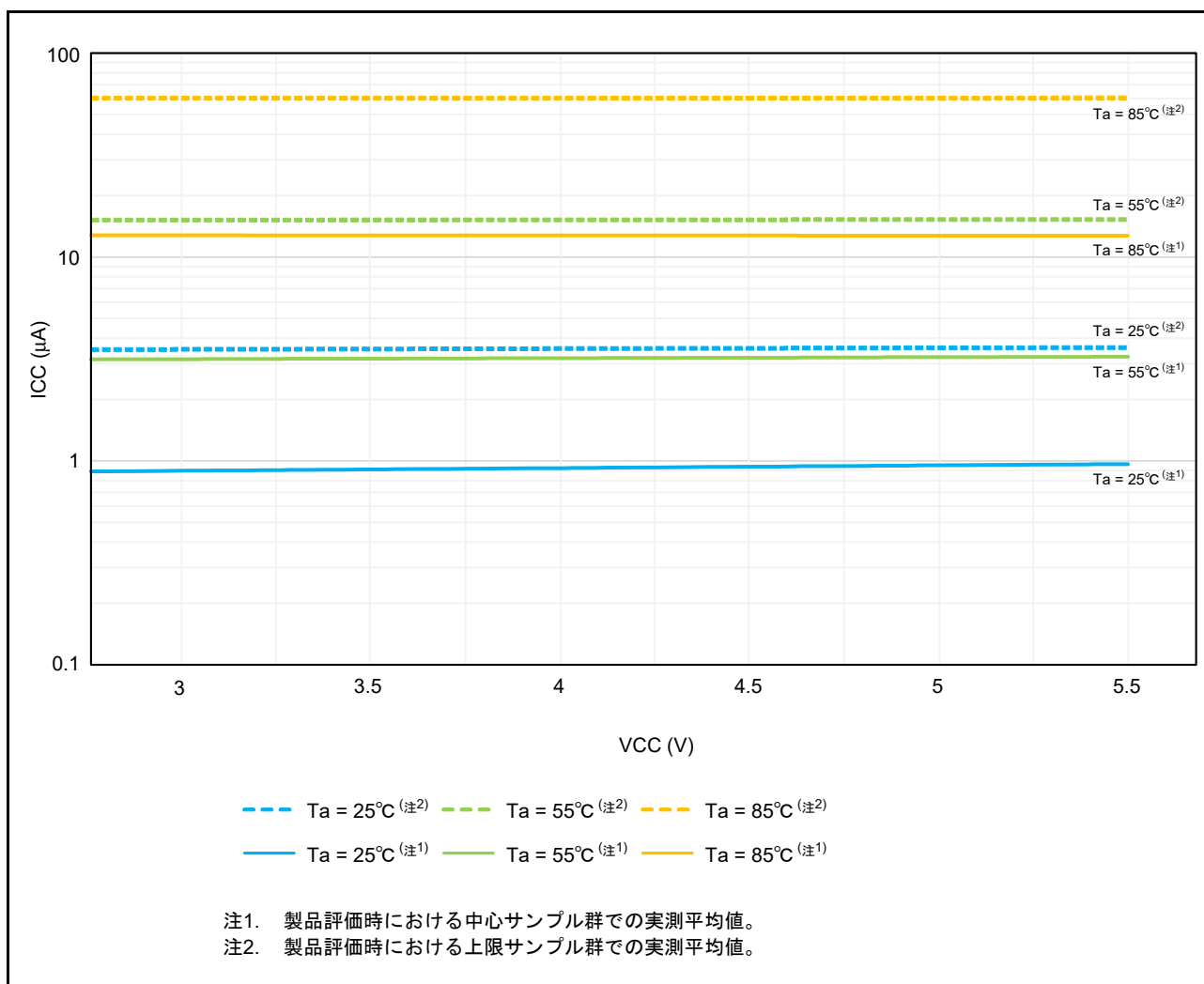
図 37.1 ソフトウェアスタンバイモード時の電圧依存性 (参考データ)
