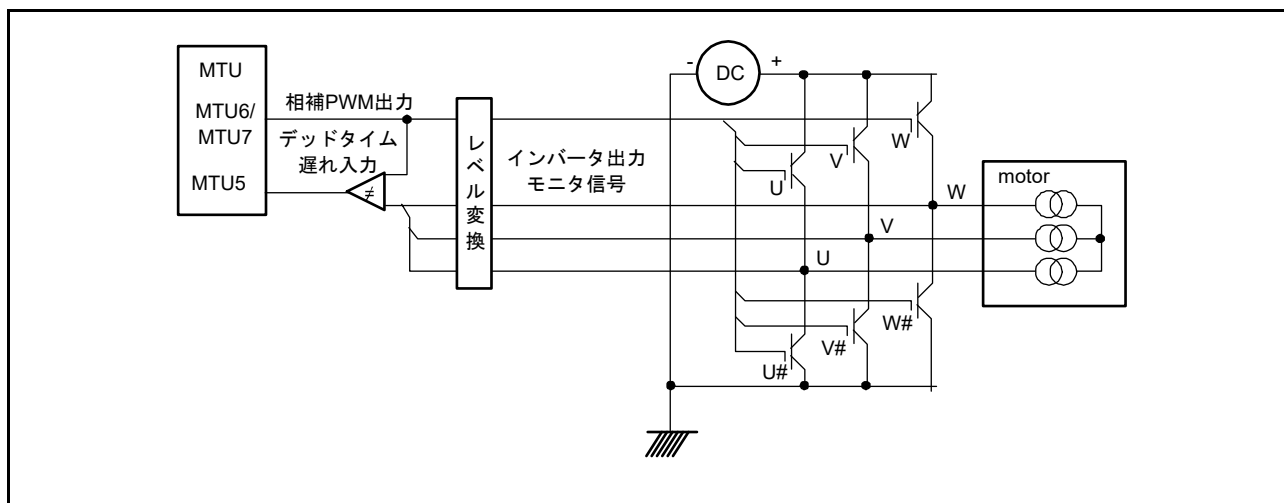
図 20.105 モータ制御回路例
