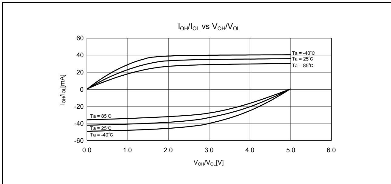
図 37.6 通常出力を選択したときの V_{OH}/V_{OL} 、 I_{OH}/I_{OL} 温度特性 VCC = 5.0V (参考データ)
