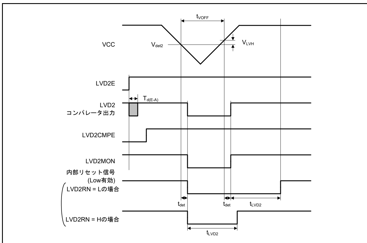
図 37.57 電圧検出回路タイミング (V det2 )
