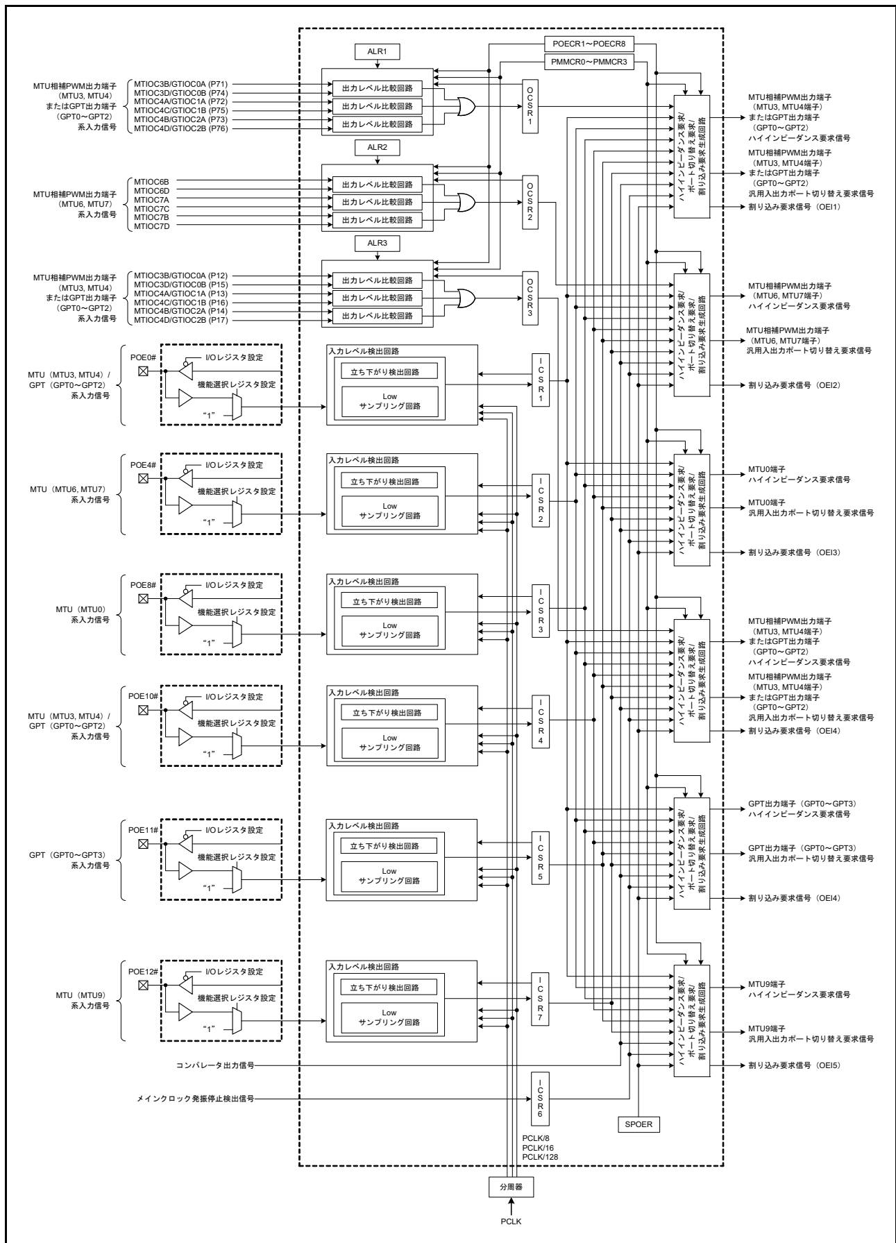
図 21.1 POEのブロック図
