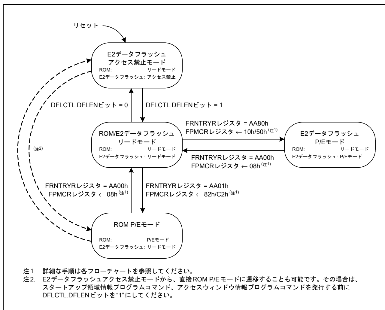
図 36.6 フラッシュメモリのモード遷移図
