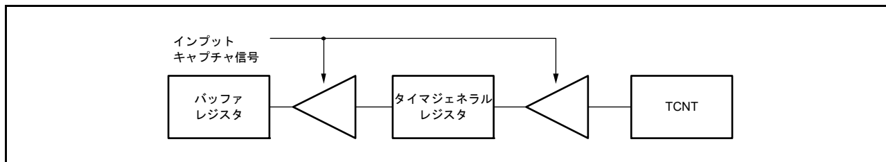
図 20.16 インพุットキャプチャバッファ動作
