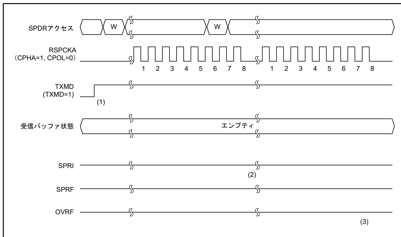
図 29.25 SPCR.TXMD = 1 の動作例
