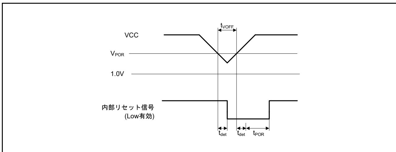
図 37.53 電圧検出リセットタイミング
