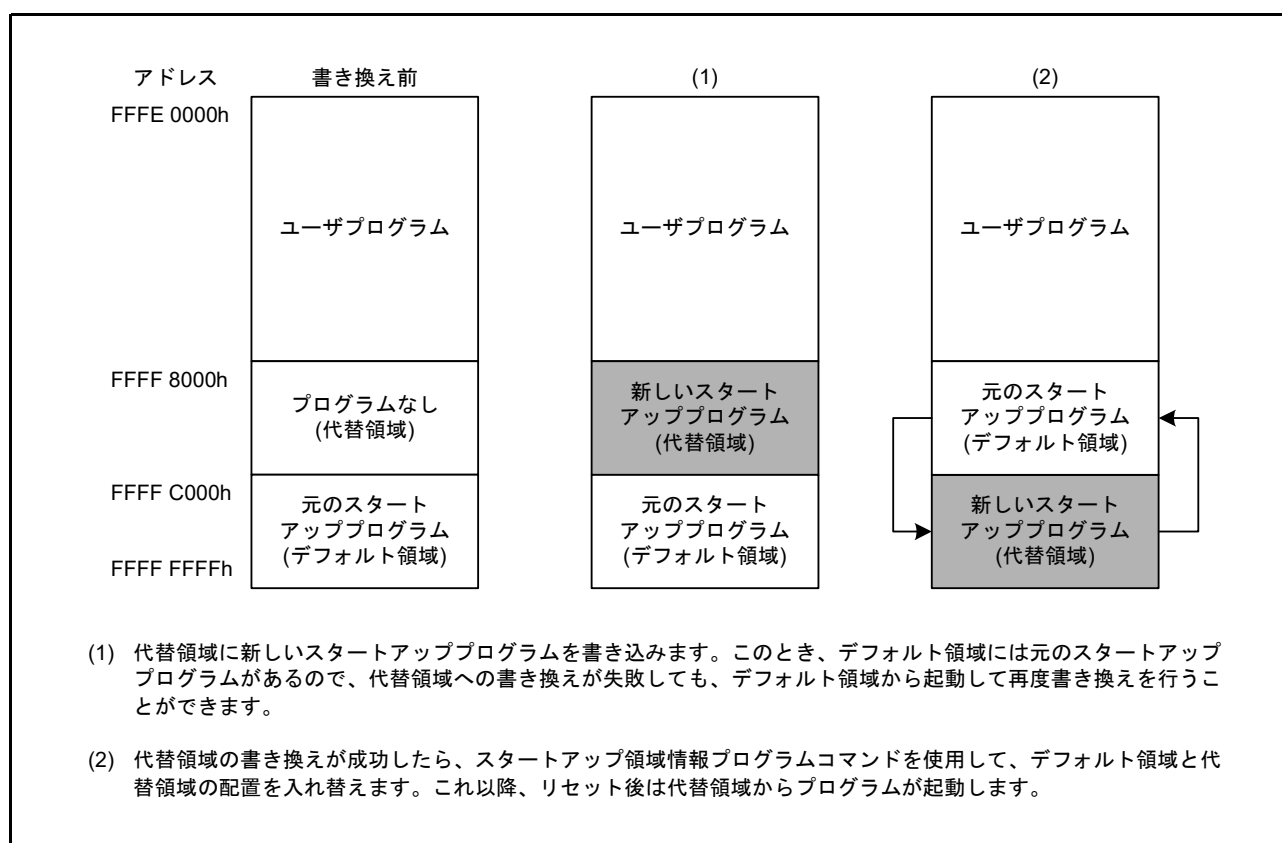
図 36.4 スタートアッププログラム保護機能の概念
