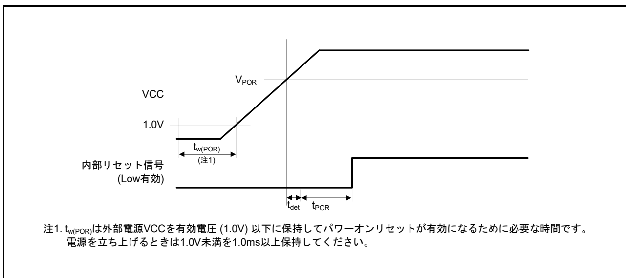
図 37.54 パワーオンリセットタイミング
