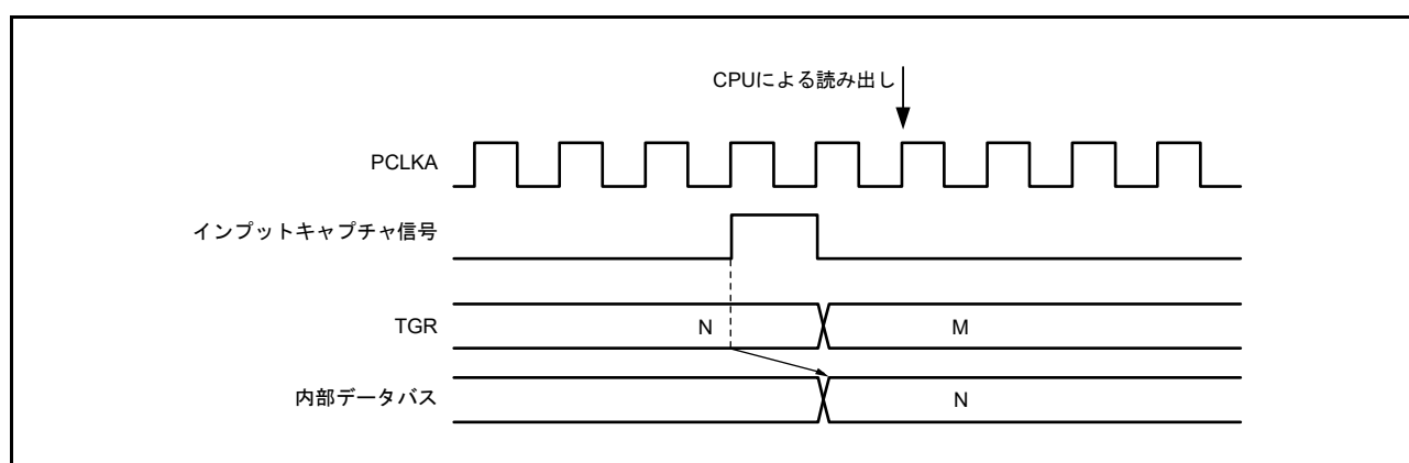
図 20.139 TGR レジスタの読み出しとインプットキャプチャの競合 (MTU0 ~ MTU7, MTU9)
