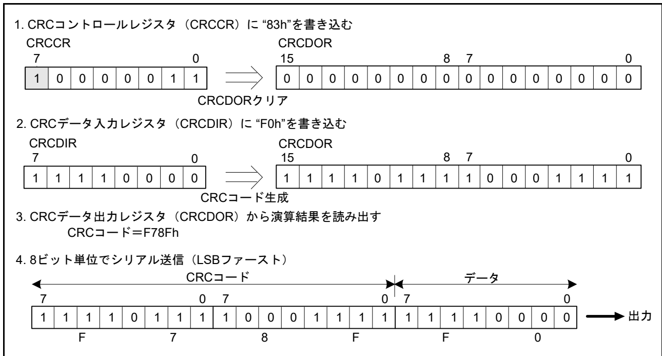
図 30.2 LSB ファーストでのデータ送信
