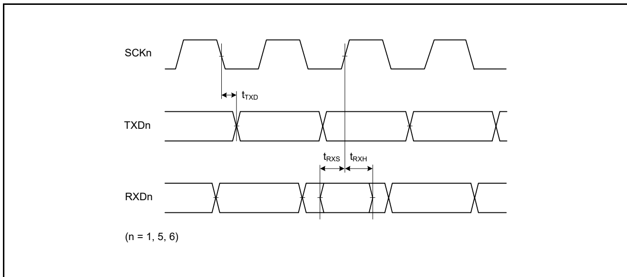
図 37.43 SCI 入出力タイミング/クロック同期式モード
