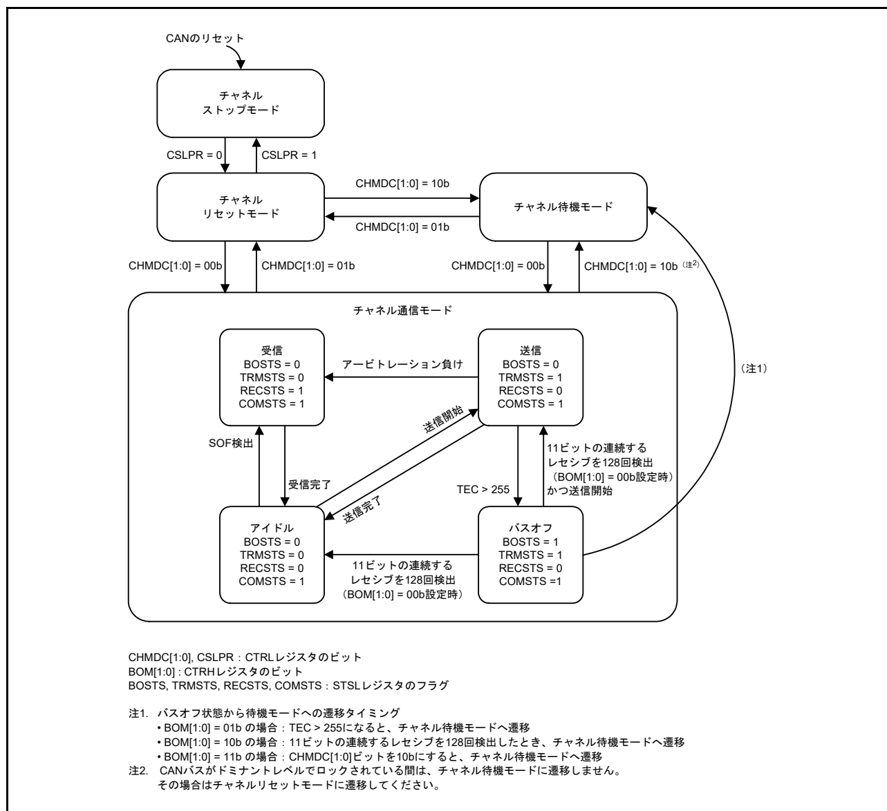
図 28.3 チャネルモードの状態遷移図
