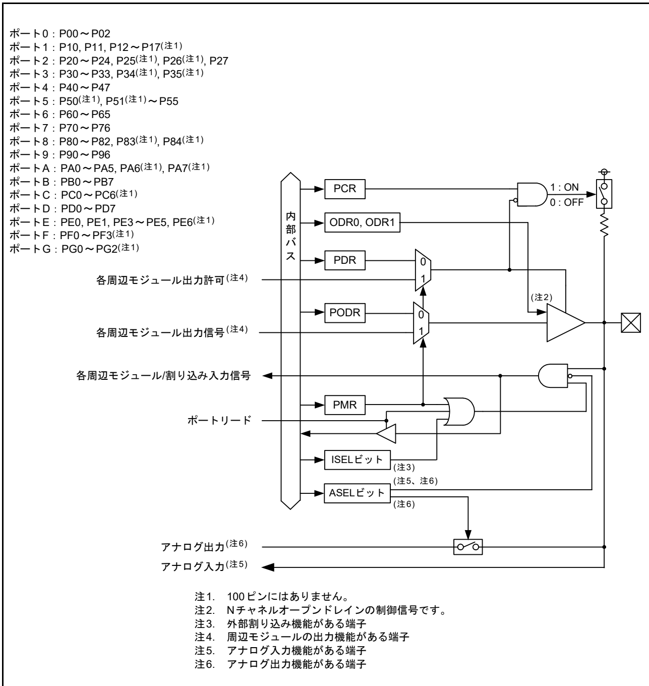
図 18.1 入出力ポートの構成 (1)
