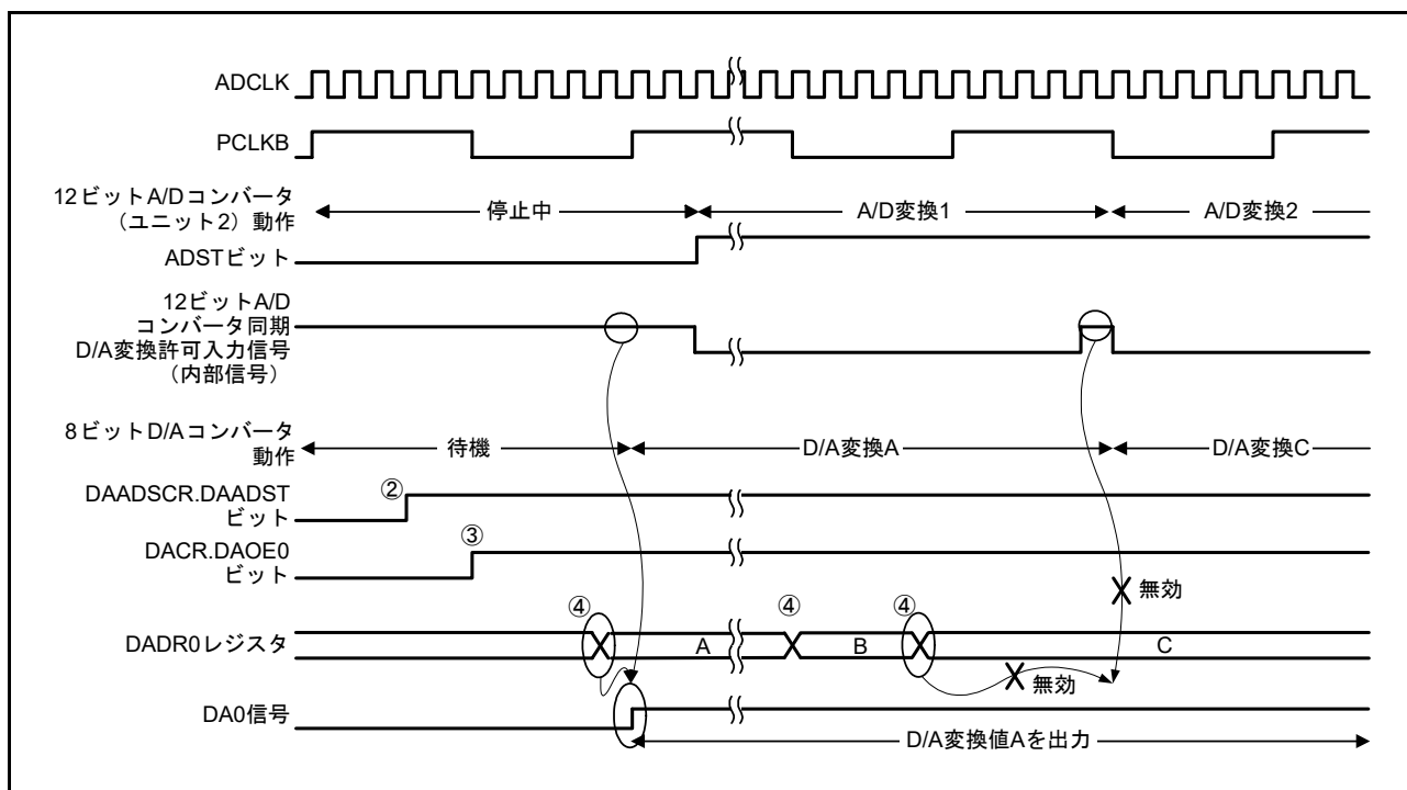
図 32.4 8ビットD/Aコンバータが12ビットA/Dコンバータ同期D/A変換許可入力信号を取り込めない例
