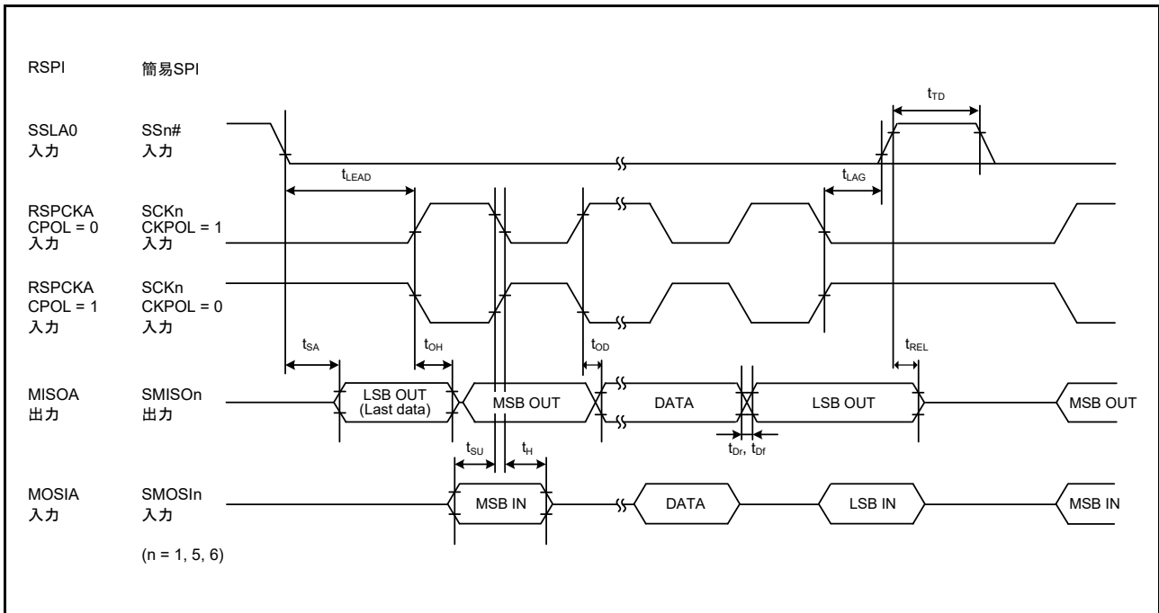
図 37.49 RSPI タイミング (スレーブ、CPHA = 1)/ 簡易 SPI タイミング (スレーブ、CKPH = 0)
