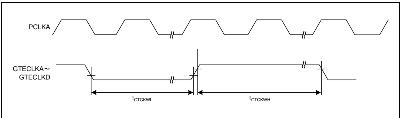
図 37.40 GPT クロック入力タイミング
