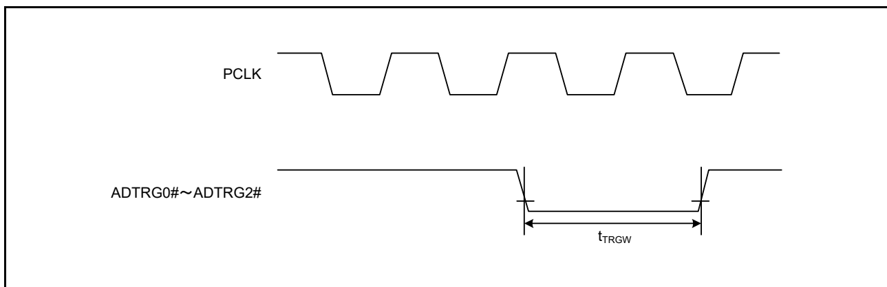
図 37.44 A/D コンバータ外部トリガ入力タイミング
