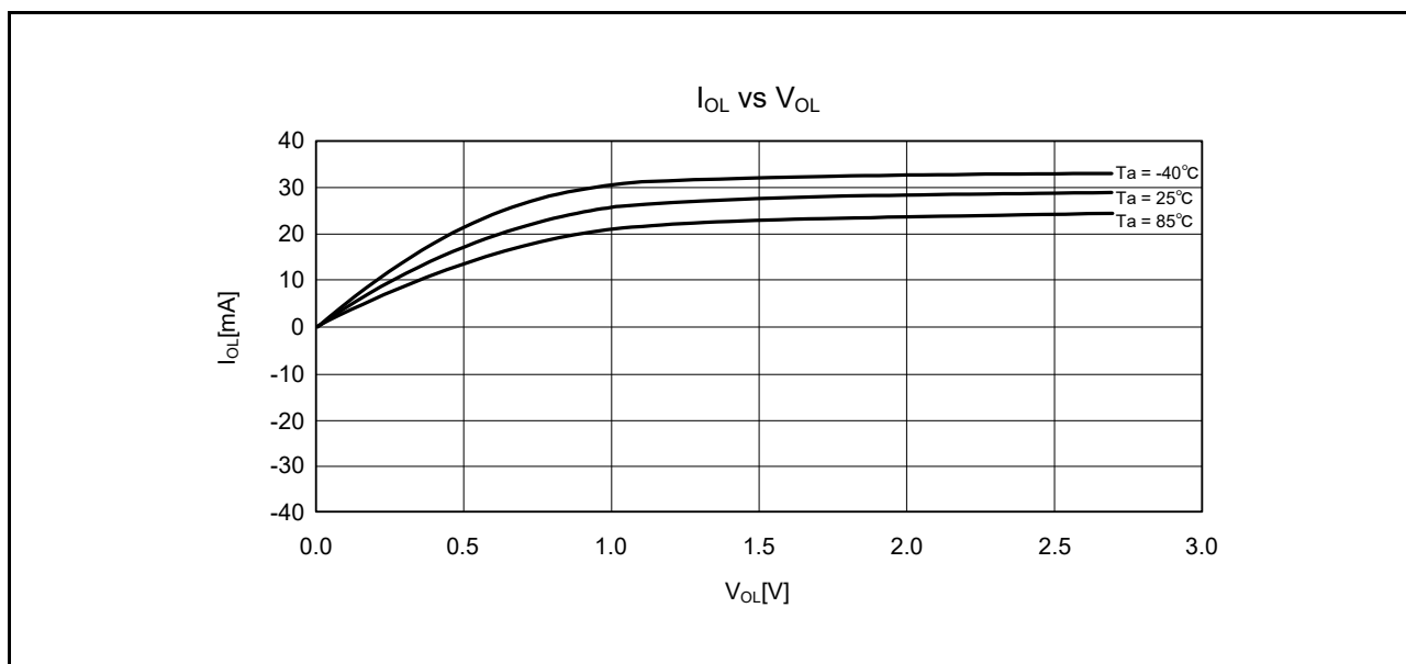
図 37.17 RIIC 出力端子の V_{OL} 、 I_{OL} 温度特性 V_{CC} = 2.7V (参考データ)
