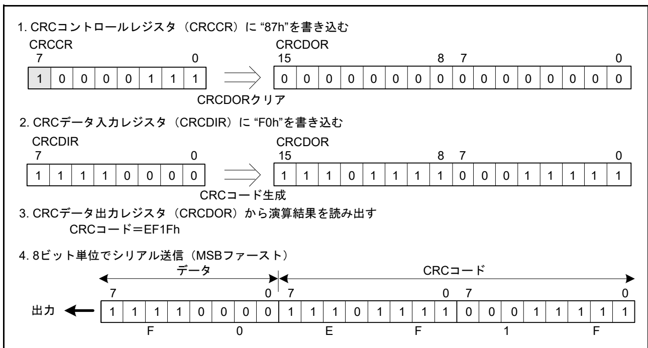
図 30.3 MSB ファーストでのデータ送信
