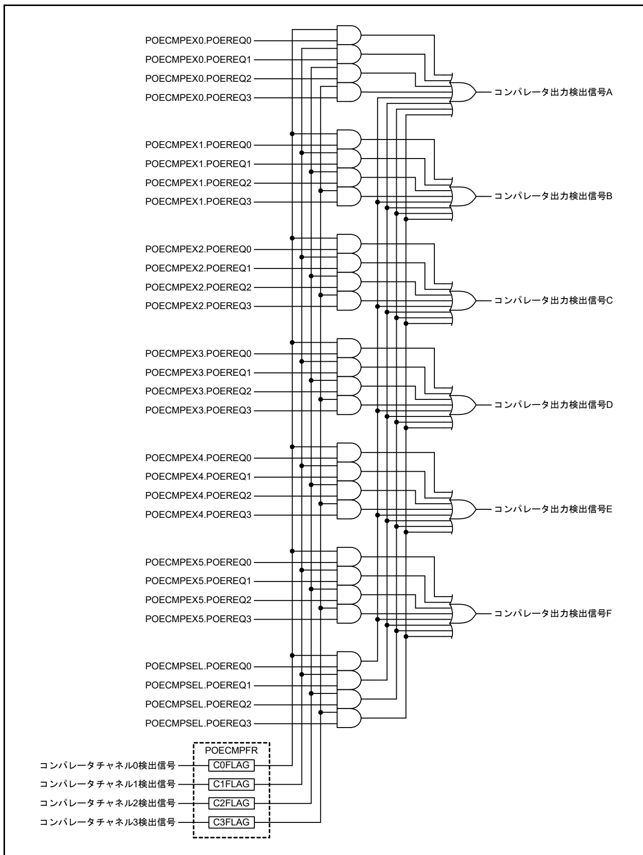
図 21.6 コンパレータ出力検出信号生成ブロック
