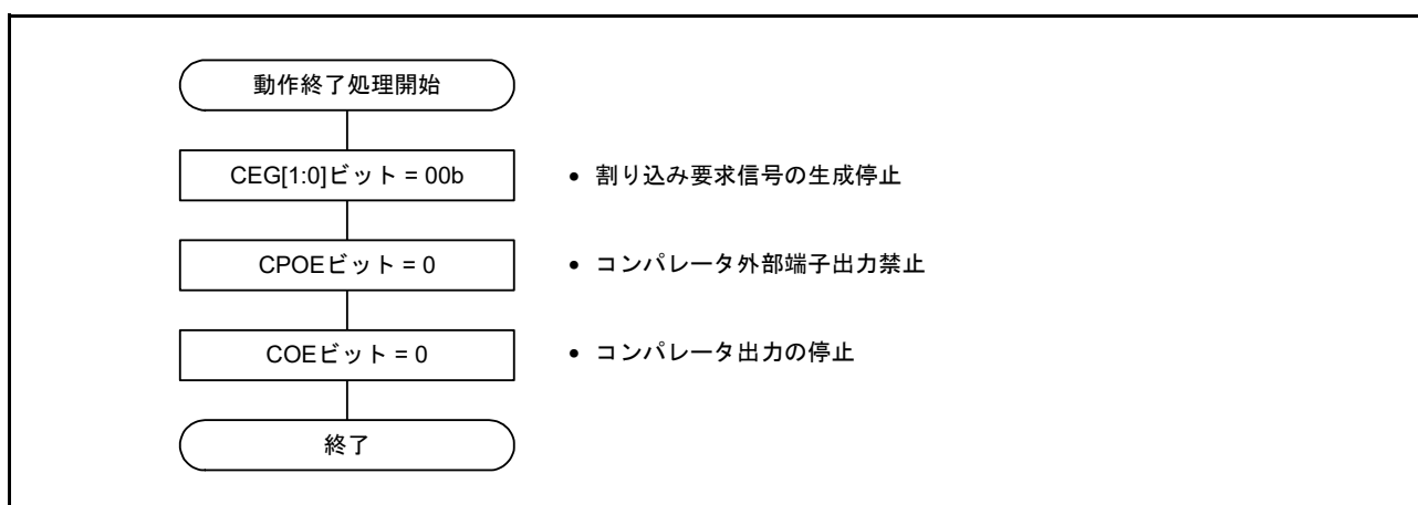
図 33.6 コンパレータ動作終了フローチャート
