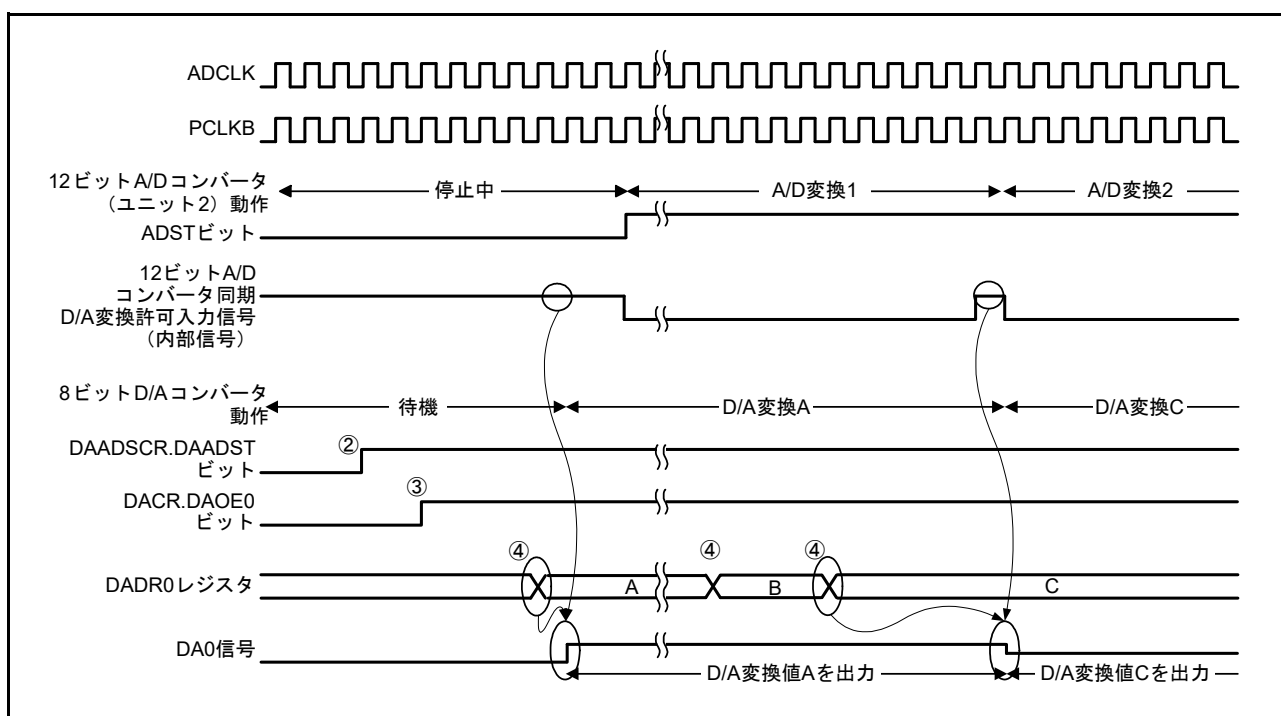
図 32.3 8ビットD/Aコンバータを12ビットA/Dコンバータ(ユニット2)に同期して変換する例
