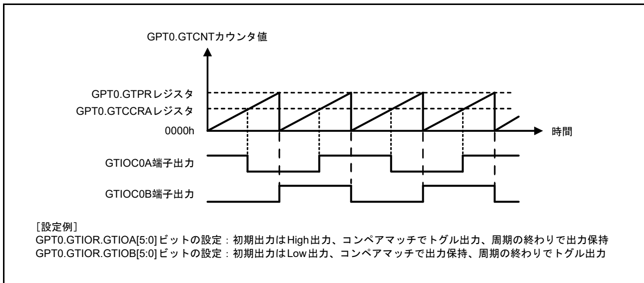
図 22.10 トグル出力動作例 (2)
