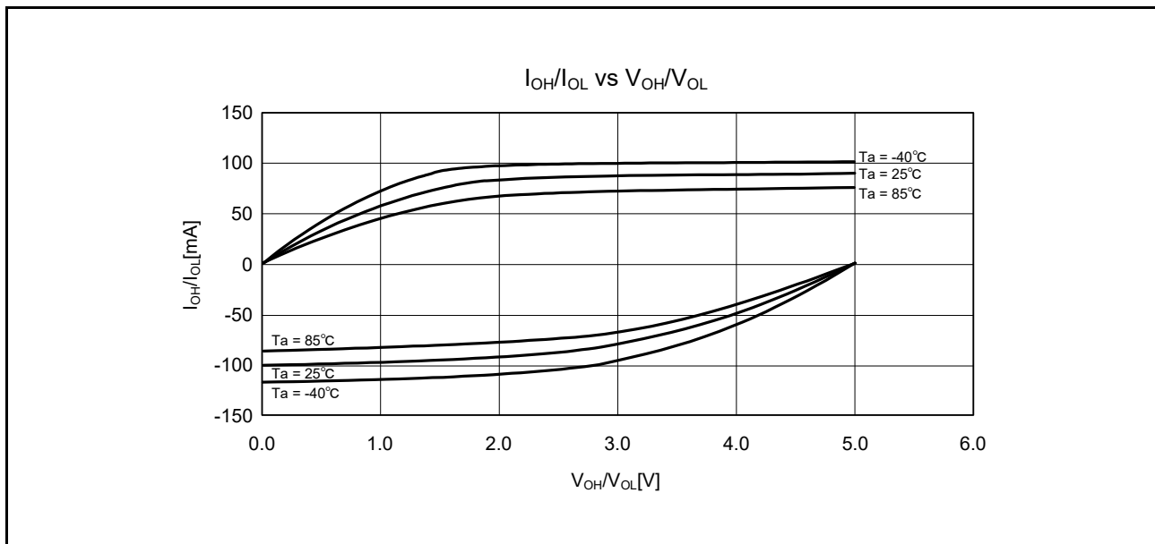
図 37.10 通常出力を選択したときの V_{OH}/V_{OL} 、 I_{OH}/I_{OL} 温度特性 V_{CC} = 5.0V (参考データ)
