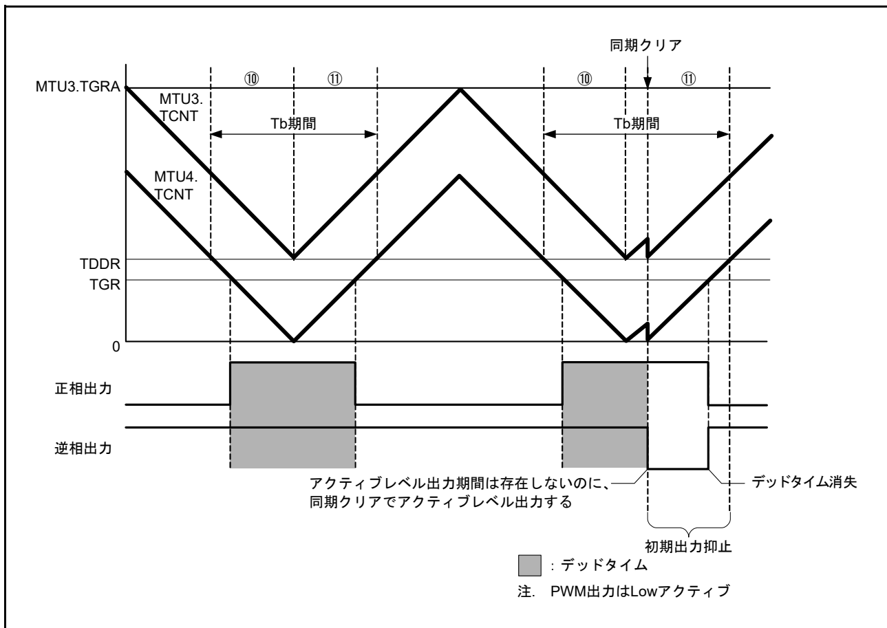
図 20.150 同期クリア例 (条件 2 の場合)
