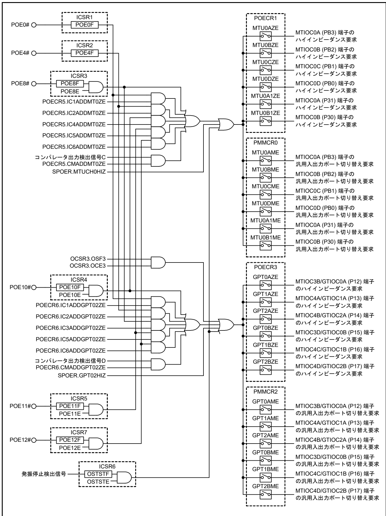
図 21.3 ハイインピーダンス制御の対象と条件 (2)
