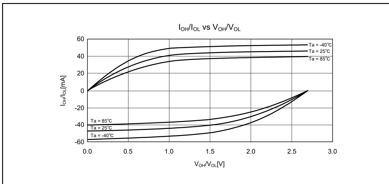
図 37.13 大電流端子の V_{OH}/V_{OL} 、 I_{OH}/I_{OL} 温度特性 V_{CC} = 2.7\text{V} (参考データ)
