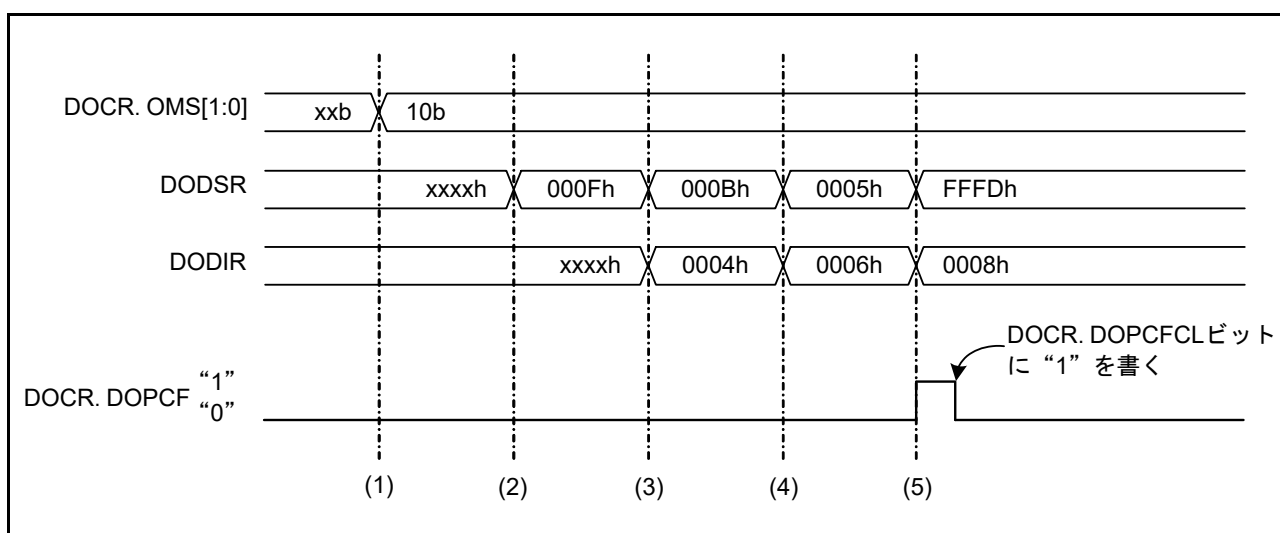
図 34.4 データ減算モードの動作例
