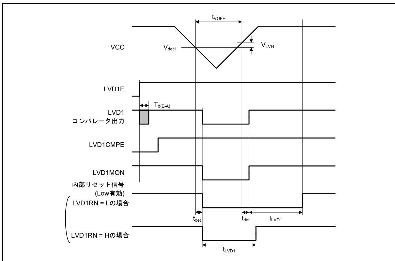
図 37.56 電圧検出回路タイミング (V det1 )
