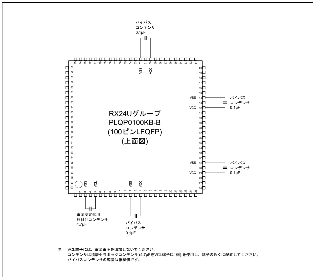
図 37.60 コンデンサ接続方法 (100ピン)
