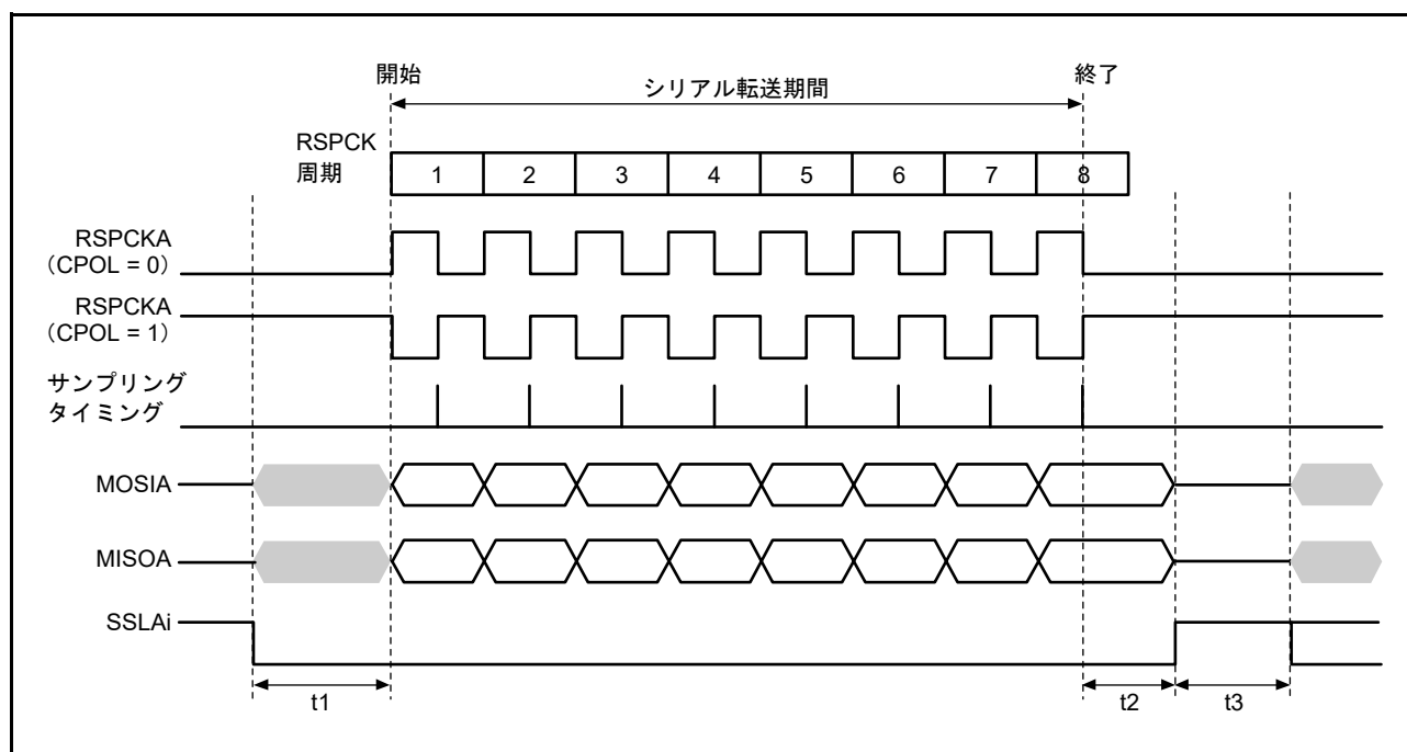
図 29.23 RSPI 転送フォーマット (CPHA ビット = 1)
