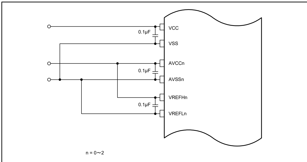
図 31.37 各電源端子の接続例
