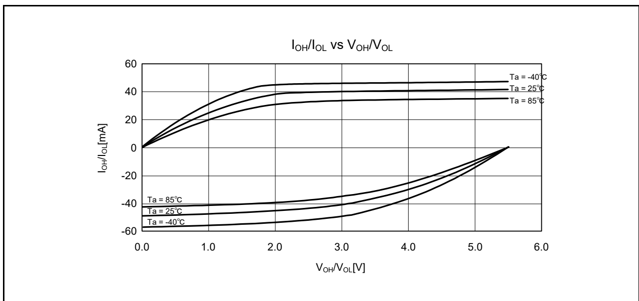
図 37.7 通常出力を選択したときの V_{OH}/V_{OL} 、 I_{OH}/I_{OL} 温度特性 VCC = 5.5V (参考データ)
