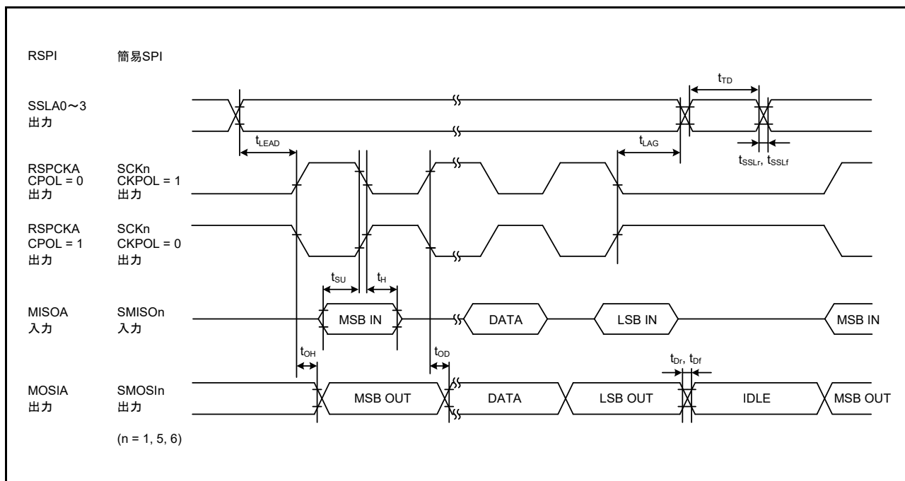
図 37.47 RSPI タイミング (マスタ、CPHA = 1)/ 簡易 SPI タイミング (マスタ、CKPH = 0)
