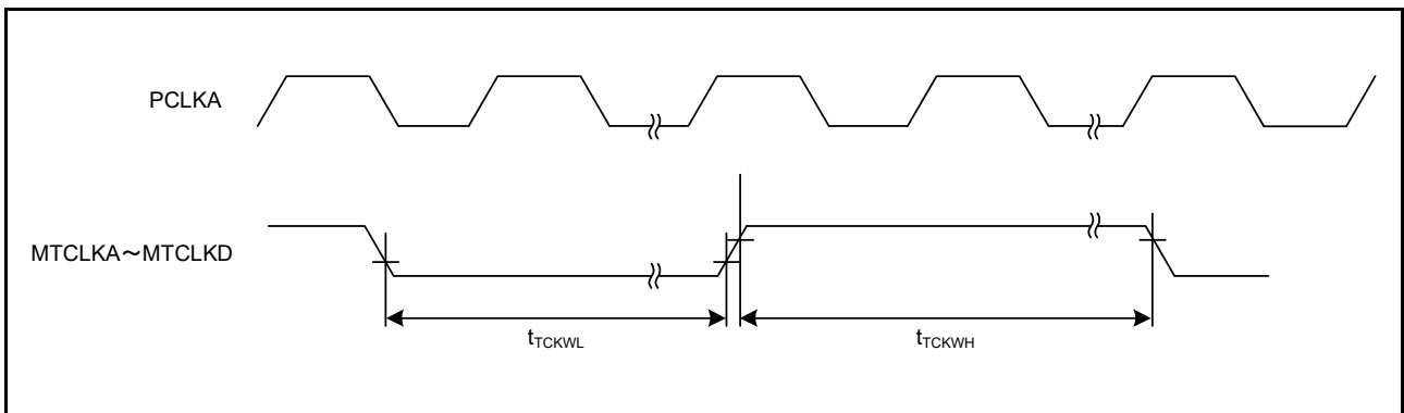
図 37.36 MTU3 クロック入力タイミング
