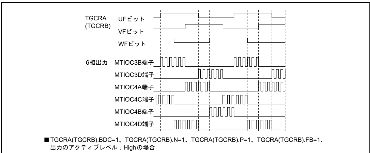
図 20.81 UF、VF、WF ビット設定による出力相の切り替え動作例 (2)
