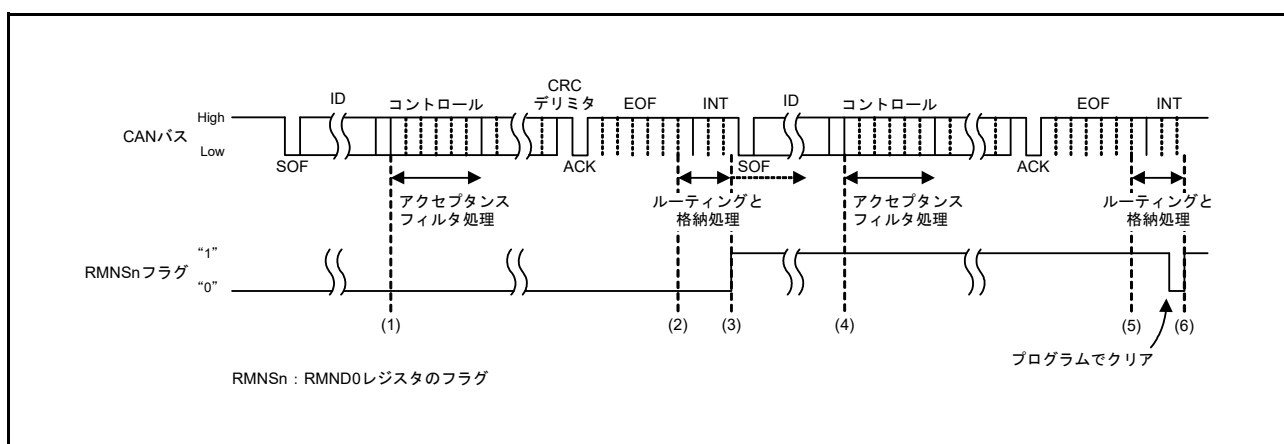
図 28.23 受信バッファの受信タイミング図
