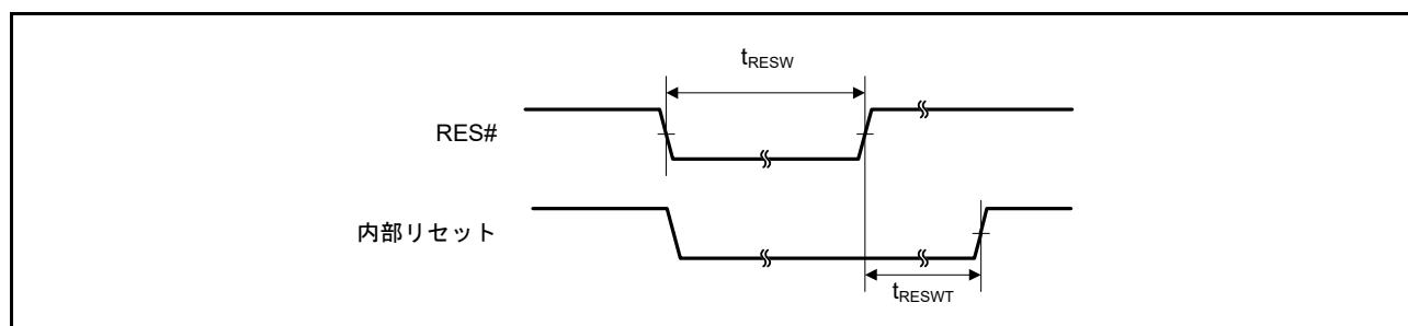
図 37.28 リセット入力タイミング (1)
