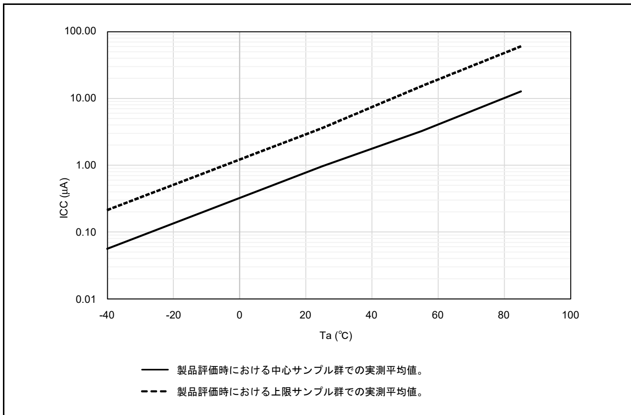
図 37.2 ソフトウェアスタンバイモード時の温度依存性 (参考データ)
