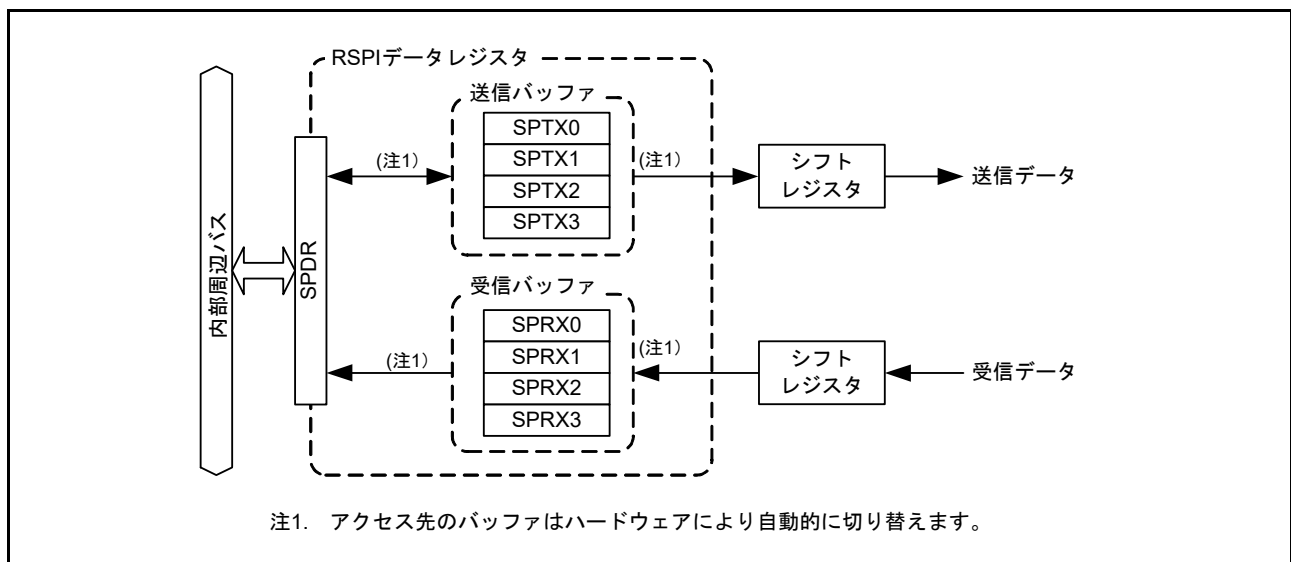
図 29.2 SPDR レジスタの構造図
