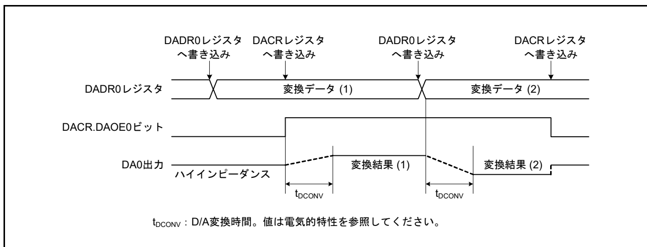
図 32.2 8ビットD/Aコンバータの動作例
