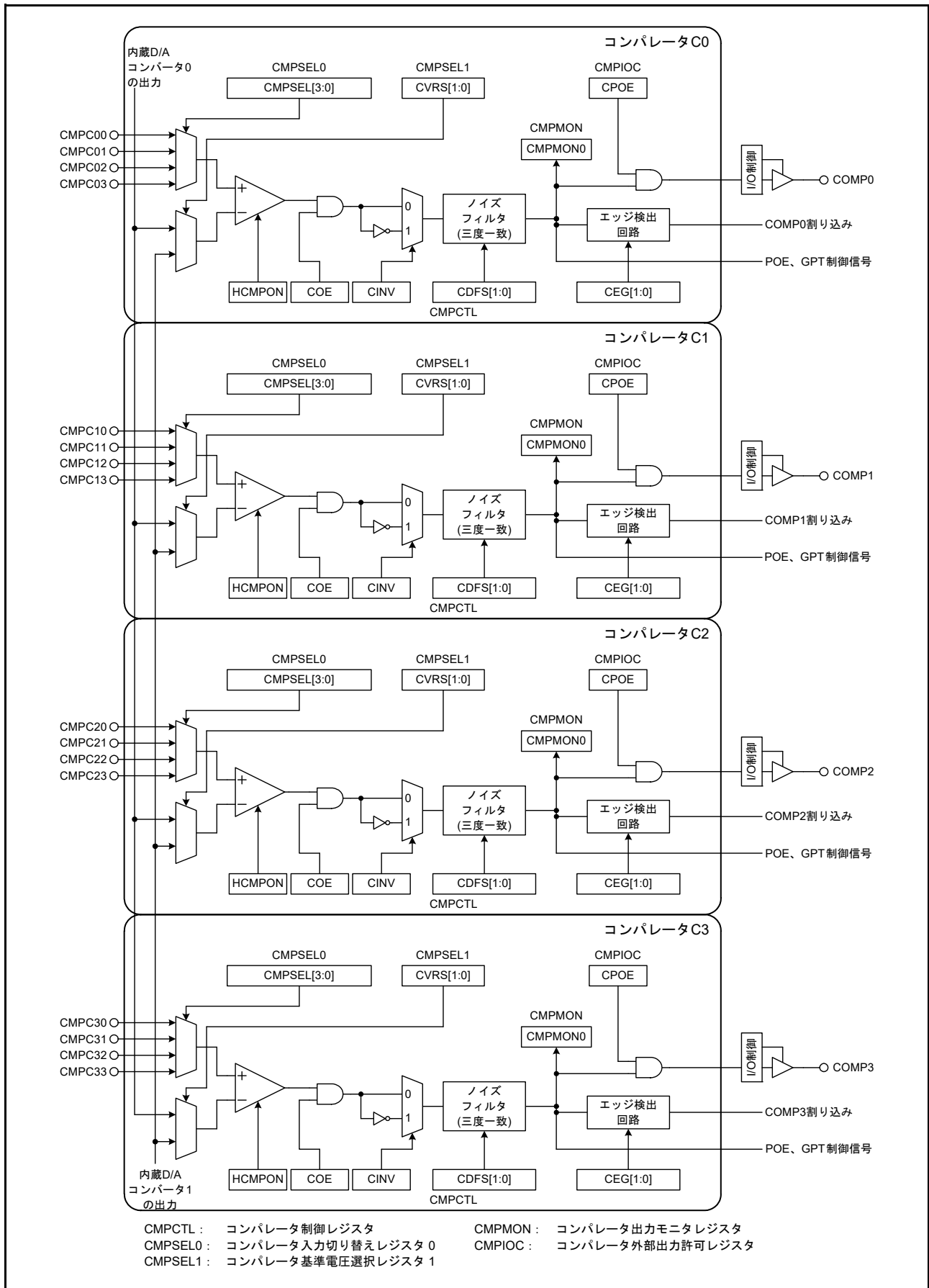
図 33.1 コンパレータ C のブロック図
