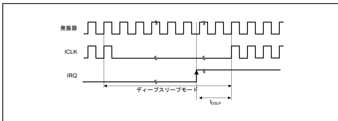
図 37.31 ディープスリープモード解除タイミング
