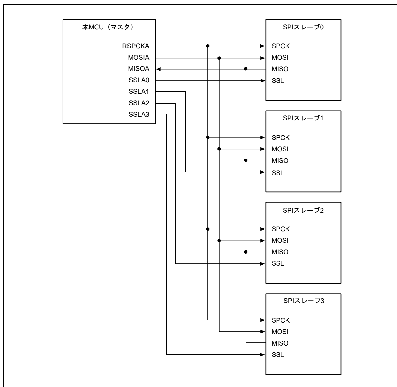
図 29.8 シングルマスタ / マルチスレーブの構成例 (本 MCU = マスタ)
