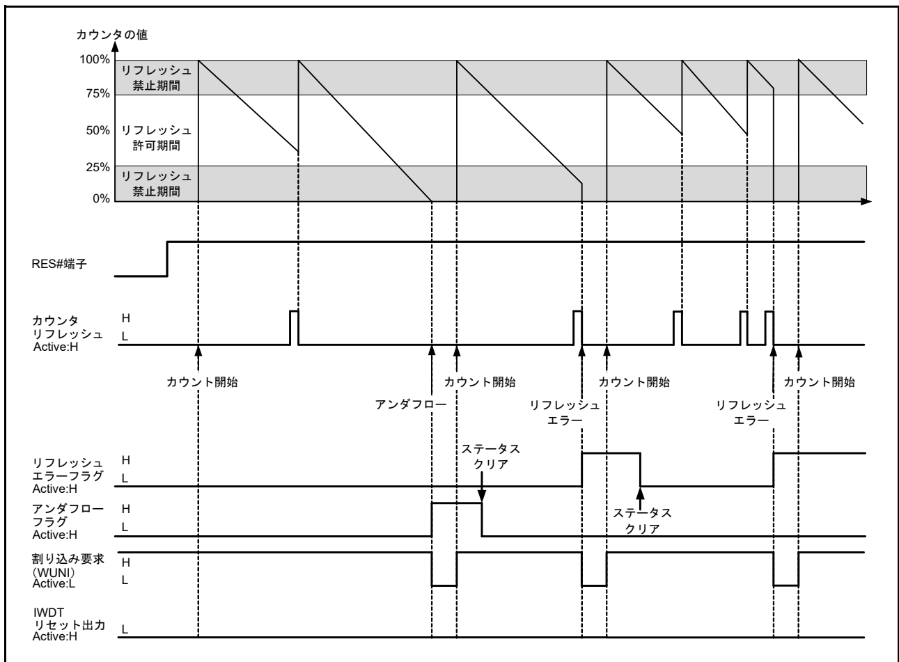
図 25.4 オートスタートモード動作例
