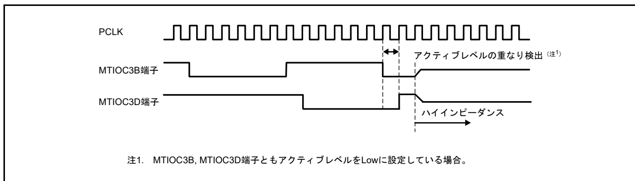
図 21.9 出力レベル検出動作
