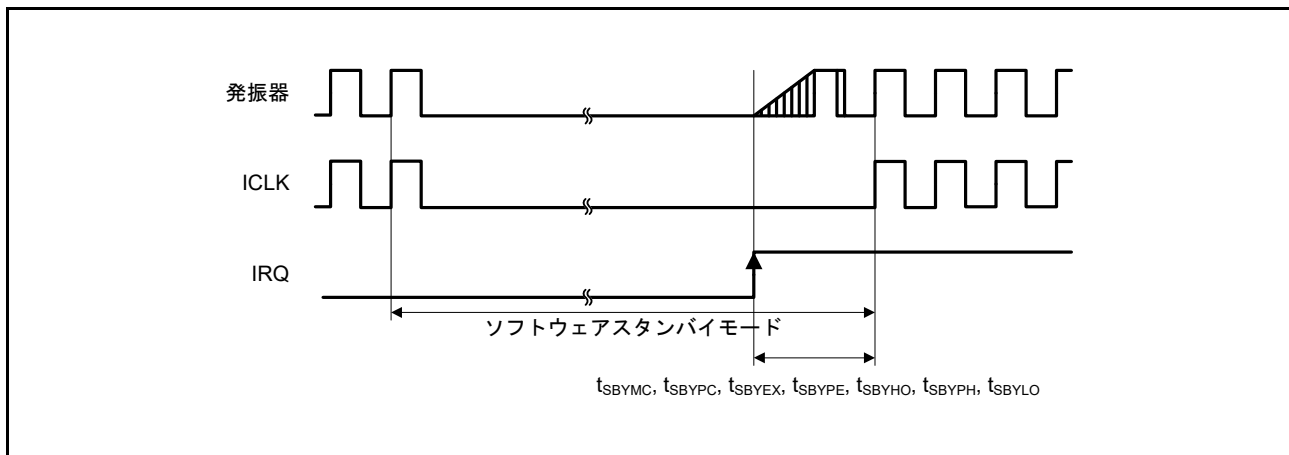
図 37.30 ソフトウェアスタンバイモード復帰タイミング
