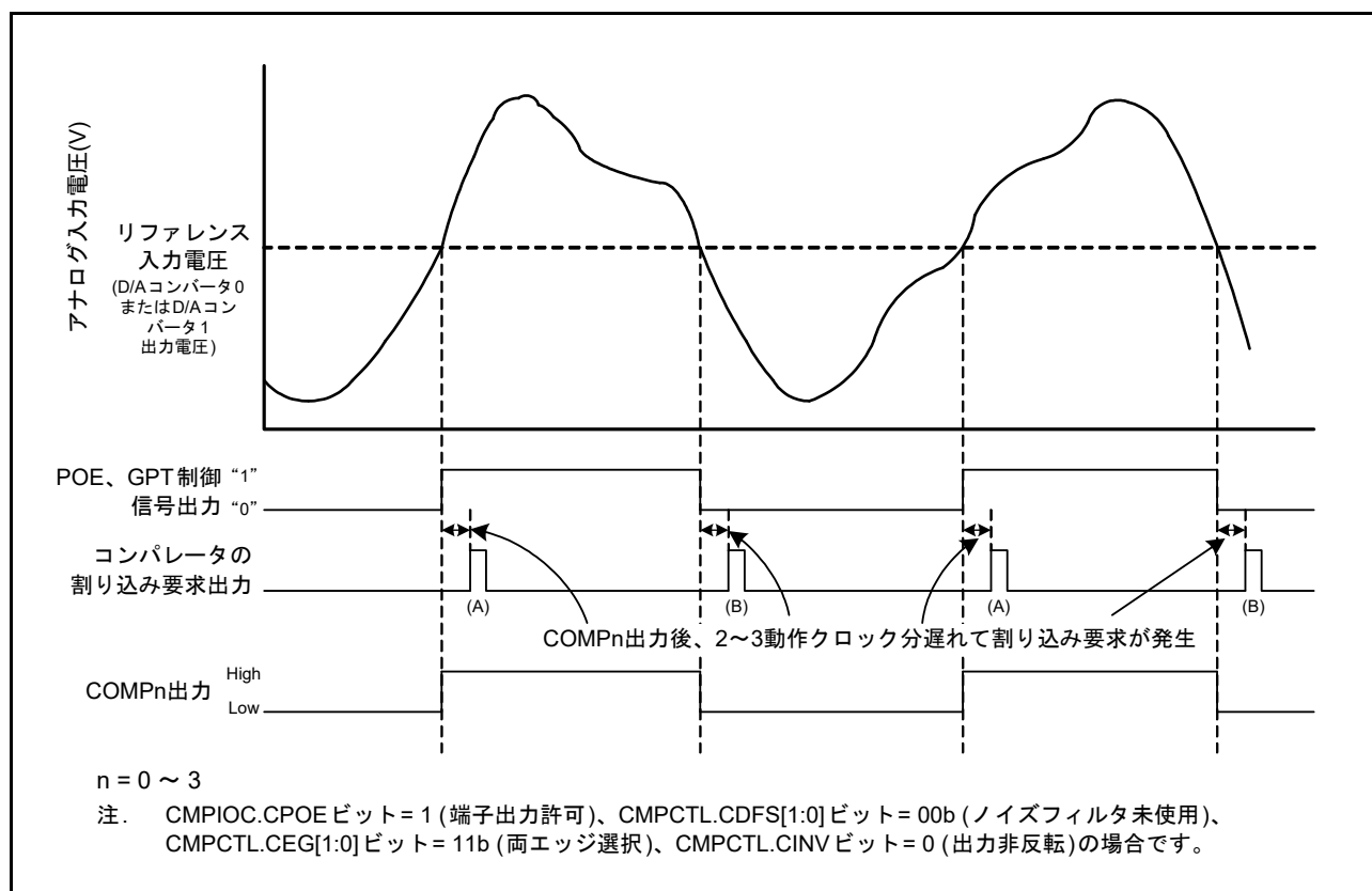
図 33.2 コンパレータの動作例
