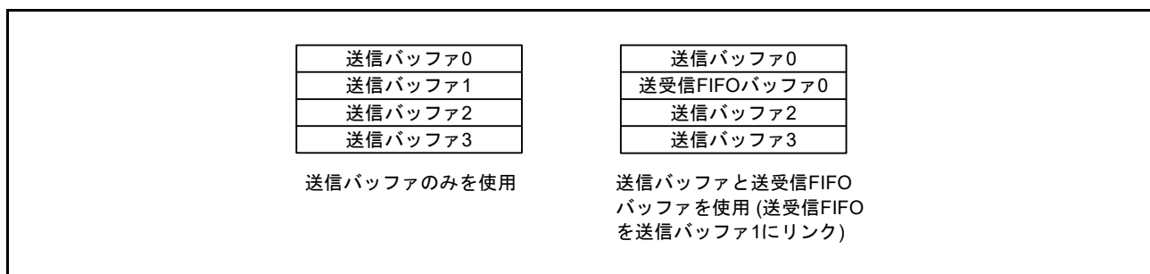
図 28.7 送受信 FIFO バッファのリンク
