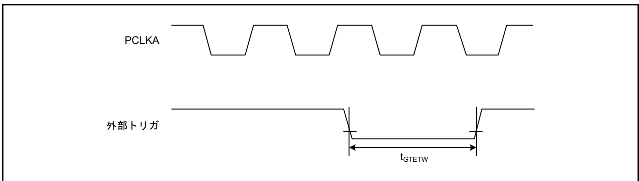
図 37.39 GPT 外部トリガ入力タイミング
