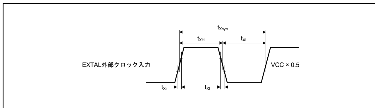
図 37.20 EXTAL 外部クロック入力タイミング
