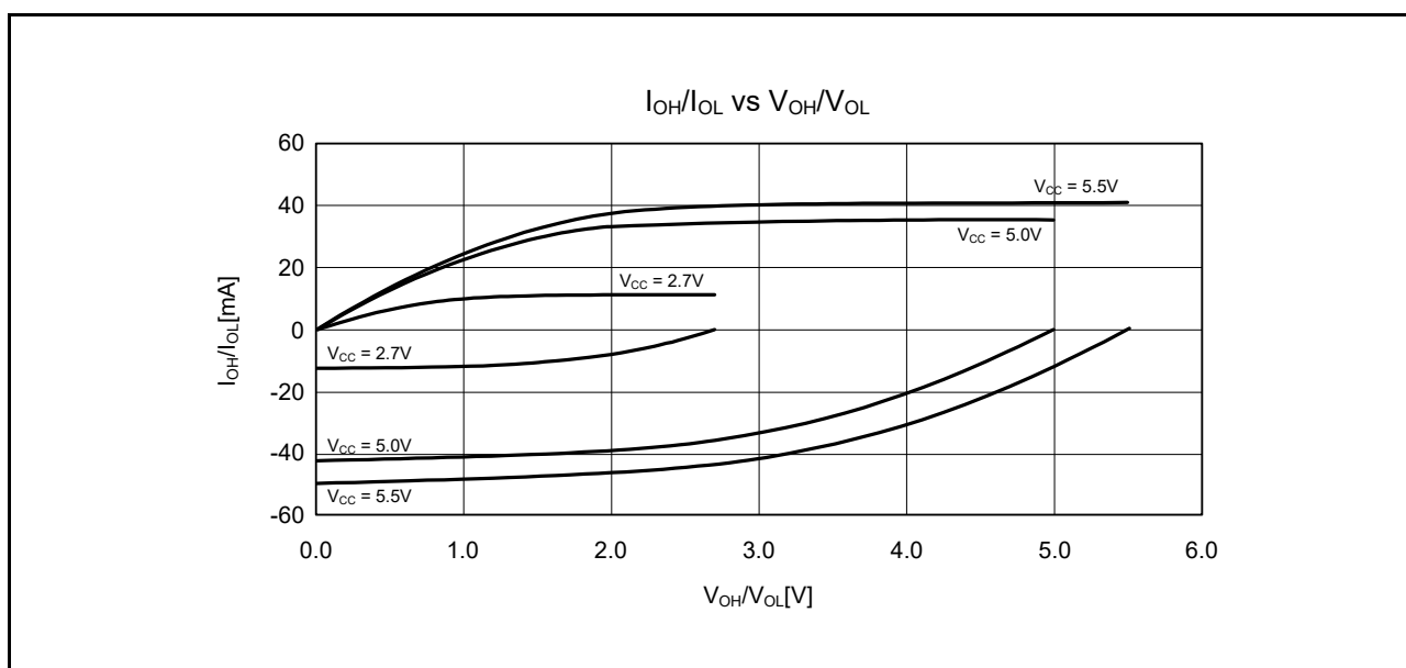
図 37.4 通常出力を選択したときの V OH /V OL 、I OH /I OL 電圧特性 T a = 25°C (参考データ)
