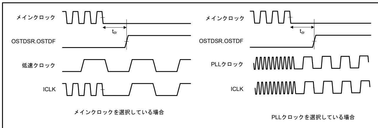
図 37.58 発振停止検出タイミング
