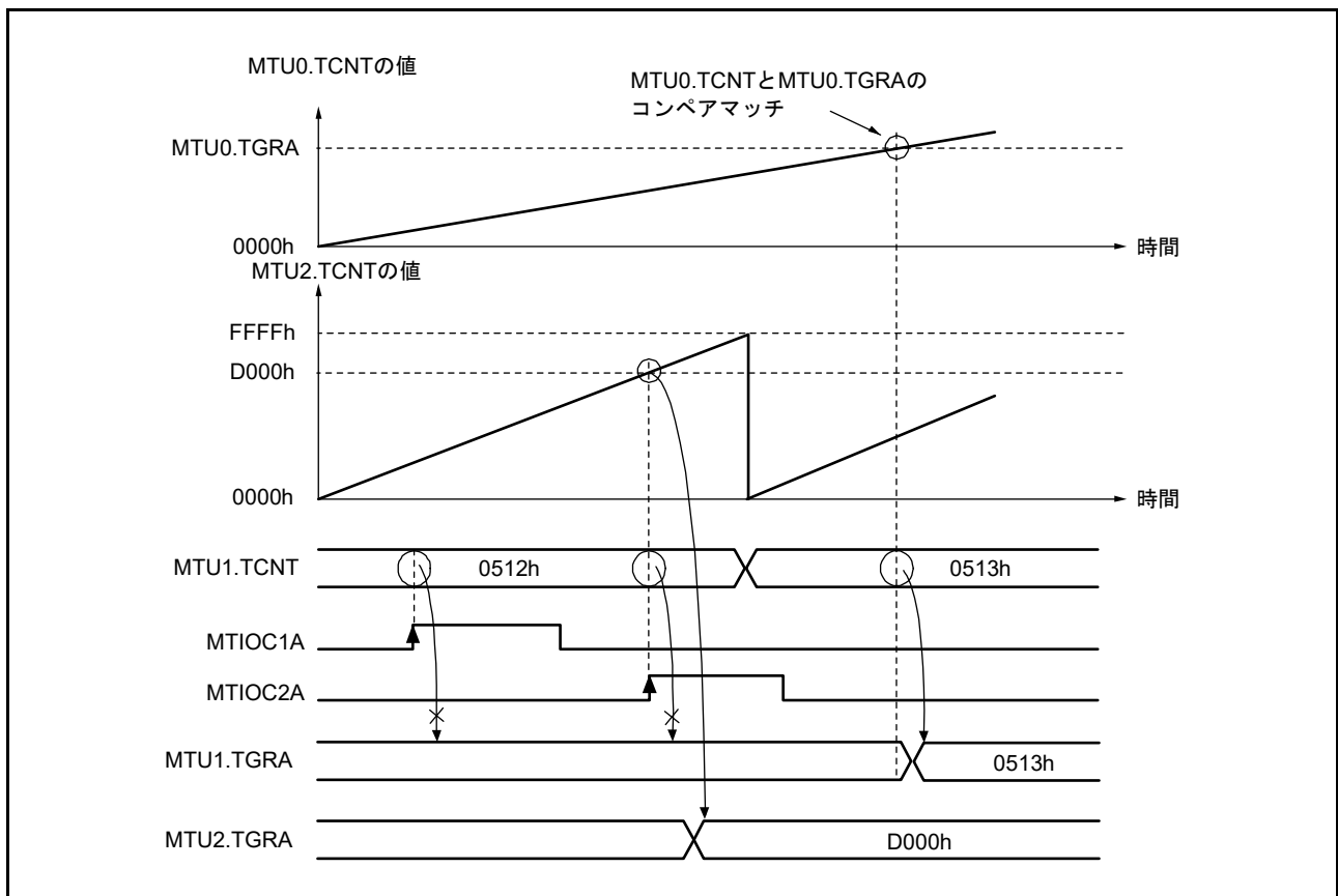
図 20.25 カスケード接続動作例 (d)
