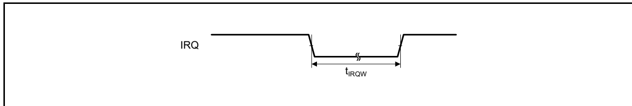
図 37.33 IRQ 割り込み入カタイミング
