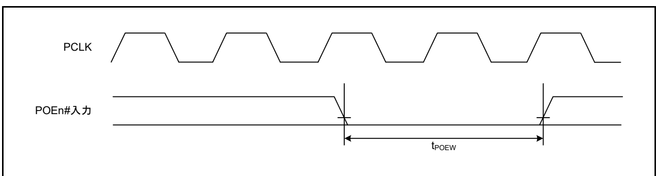
図 37.37 POE# 入力タイミング
