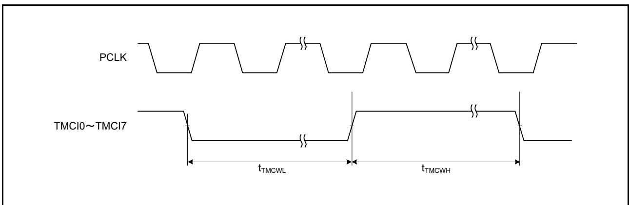
図 37.41 TMR クロック入力タイミング
