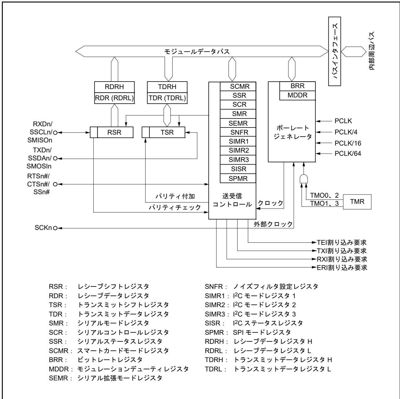
図 26.2 SClg (SCI5, SCI6) のブロック図
