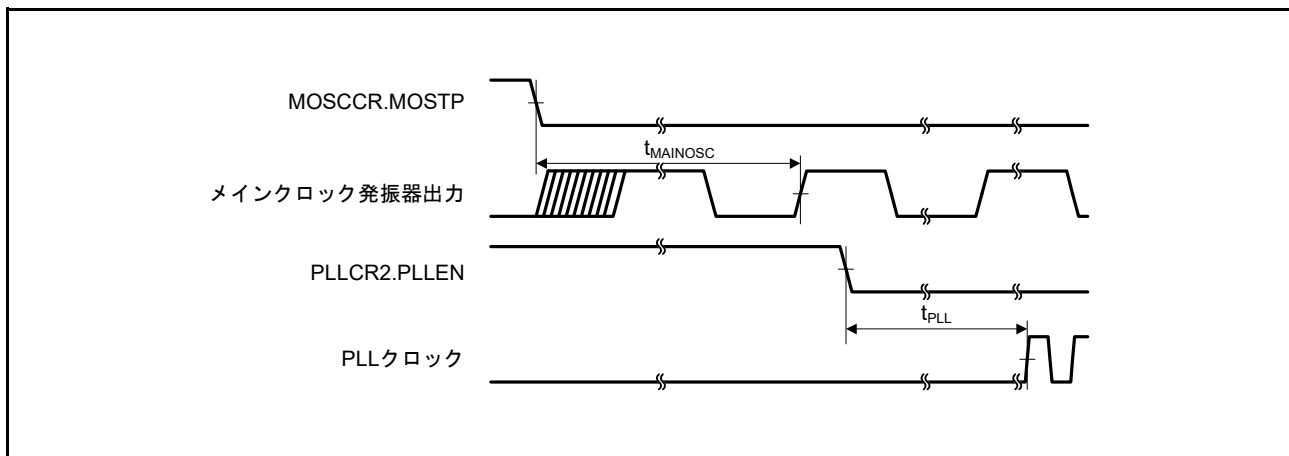
図 37.26 PLL クロック発振開始タイミング (メインクロック発振安定後に PLL を動作させたとき)
