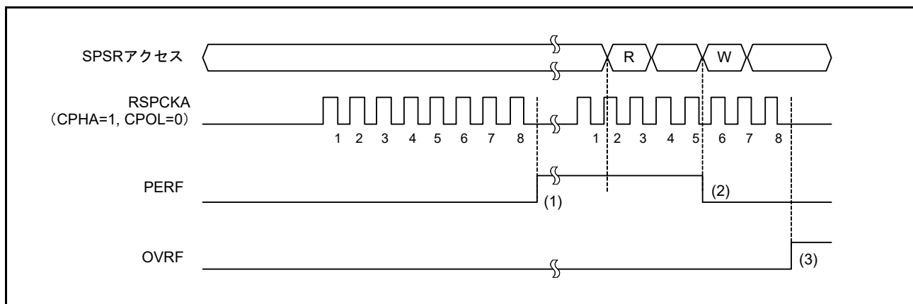
図 29.30 PERF フラグの動作例
