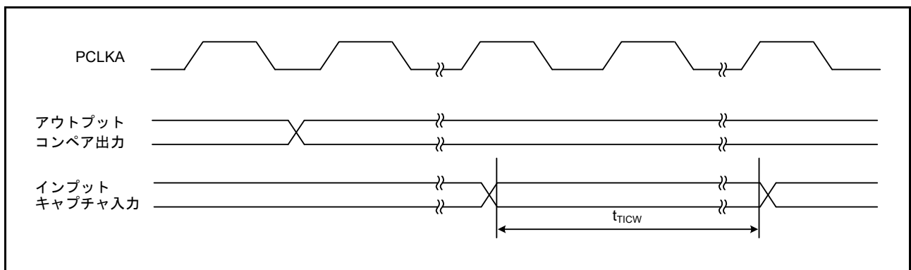
図 37.35 MTU3入出力タイミング
