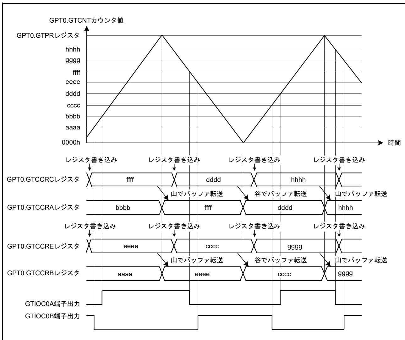
図 22.35 三角波 PWM モード 2 動作例
