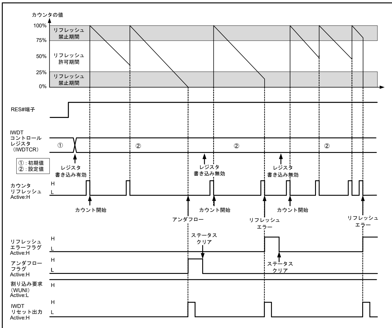
図 25.3 レジスタスタートモード動作例
