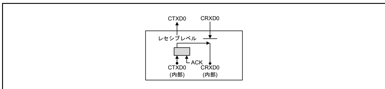
図 28.12 セルフテストモード1 選択時の接続
