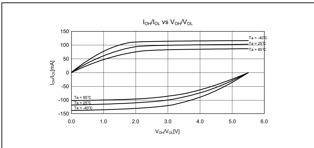
図 37.11 通常出力を選択したときの V_{OH}/V_{OL} 、 I_{OH}/I_{OL} 温度特性 V_{CC} = 5.5V (参考データ)
