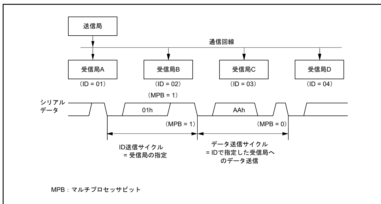
図 26.16 マルチプロセッサフォーマットを使用した通信例（受信局 A へのデータ“AAh”の送信の例）
