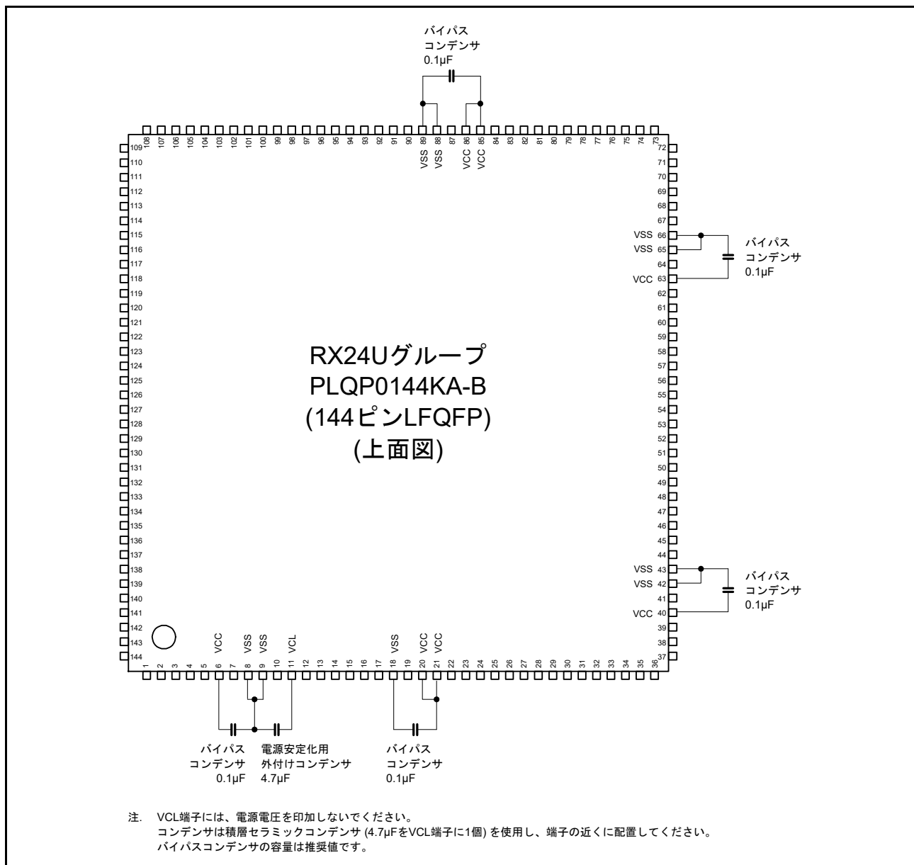
図 37.59 コンデンサ接続方法 (144 ピン)
