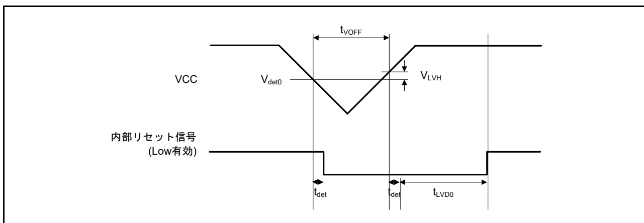
図 37.55 電圧検出回路タイミング (V det0 )
