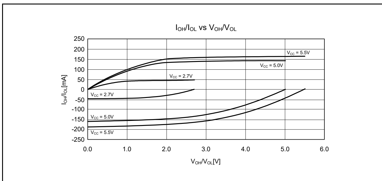
図 37.12 大電流端子の V_{OH}/V_{OL} 、 I_{OH}/I_{OL} 電圧特性 T_a = 25^\circ\text{C} (参考データ)
