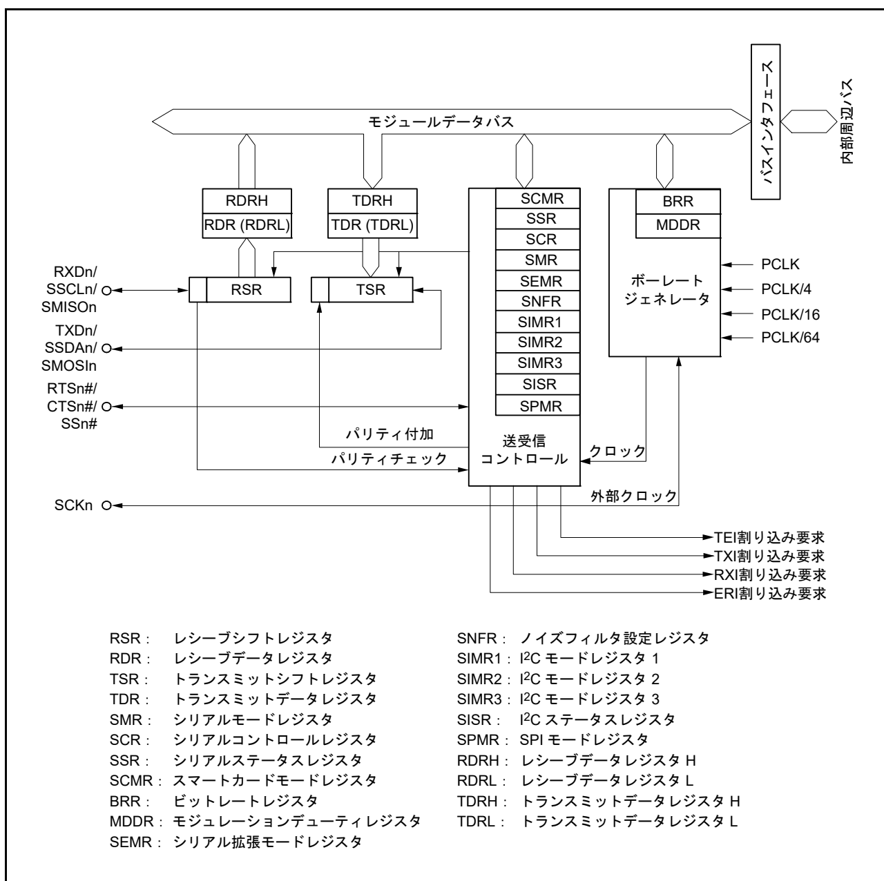
図 26.1 SCl g (SCI1, SCI8, SCI9, SCI11) のブロック図
