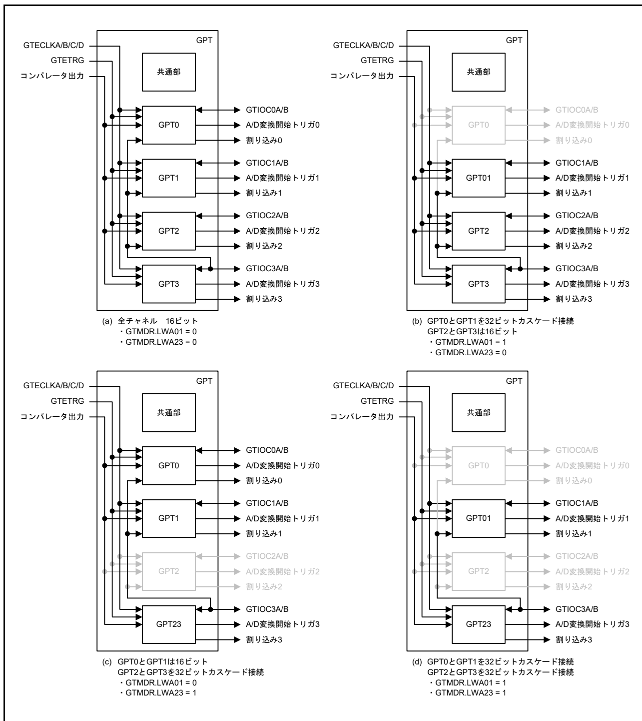
図 22.2 チャネル構成バリエーション
