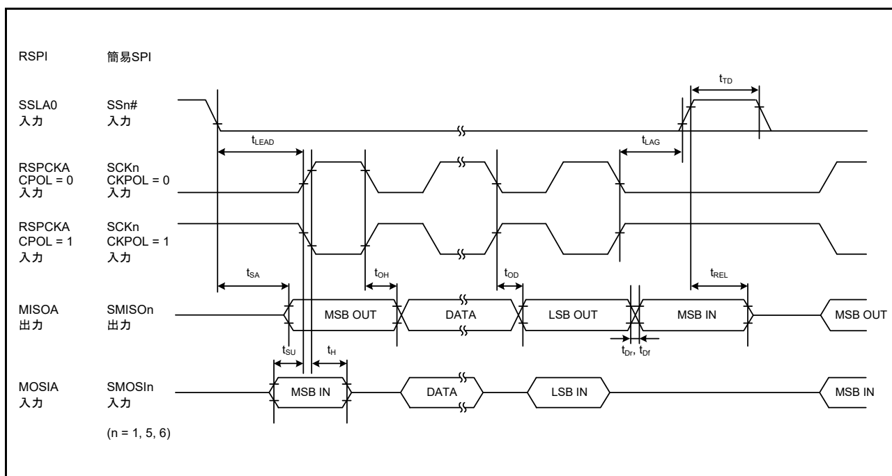
図 37.48 RSPI タイミング (スレーブ、CPHA = 0)/ 簡易 SPI タイミング (スレーブ、CKPH = 1)
