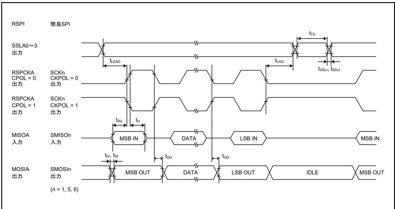
図 37.46 RSPi タイミング ( マスタ、CPHA = 0) / 簡易 SPI タイミング ( マスタ、CKPH = 1)
