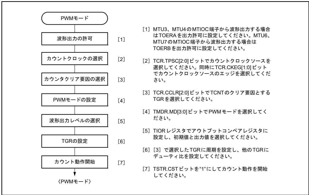
図 20.26 PWM モードの設定手順例
