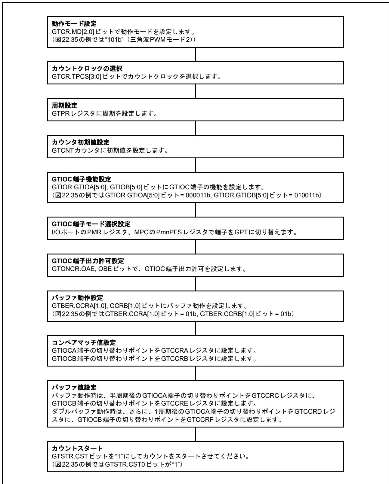
図 22.36 三角波 PWM モード 2 設定例
