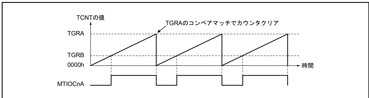
図 20.27 PWM モード1 の動作例 (n = 0 ~ 4, 6, 7, 9)
