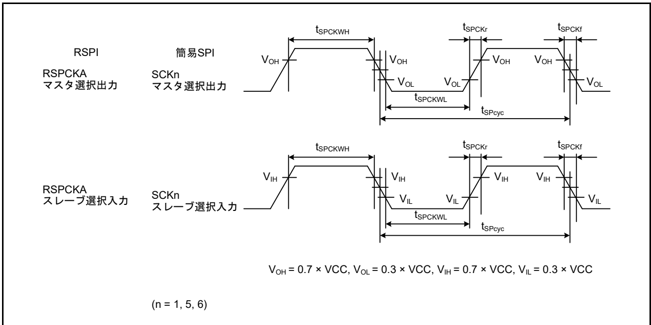
図 37.45 RSPi クロックタイミング / 簡易 SPI クロックタイミング
