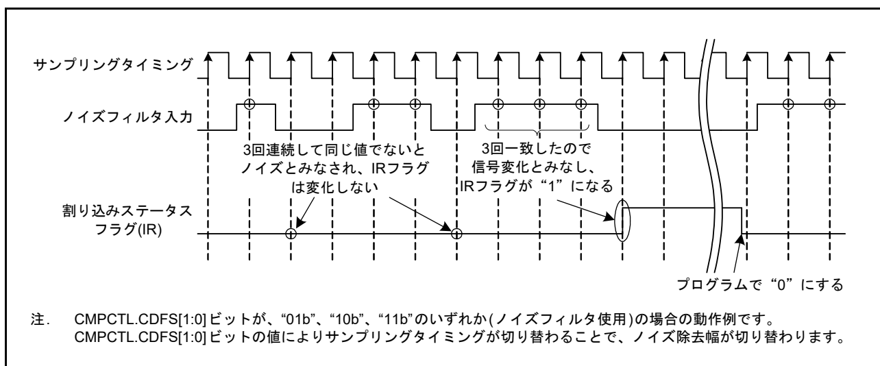
図 33.4 コンパレータノイズフィルタと割り込み動作例
