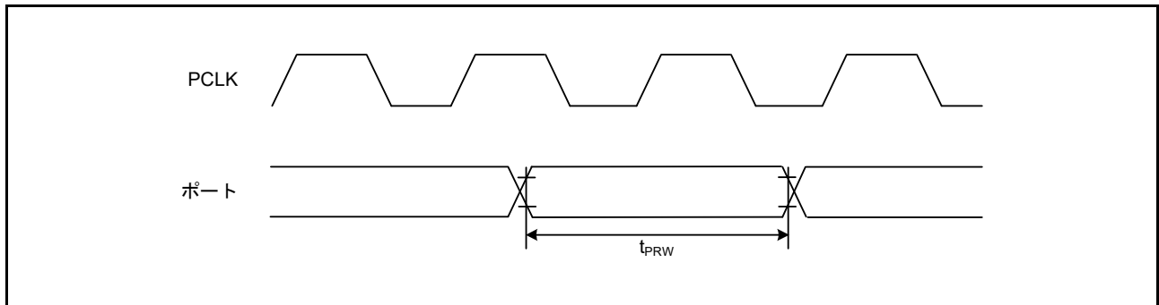
図 37.34 I/Oポート入力タイミング
