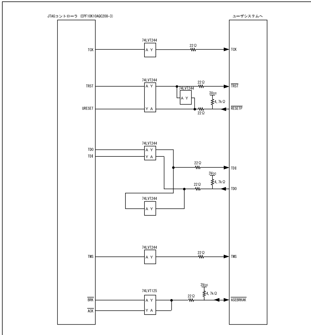
図 6.8 Hitachi-UDI 端子部分のユーザシステムインタフェース回路 (HS7705KCI02H) ( Model 名 : HS0005KCI04H )
