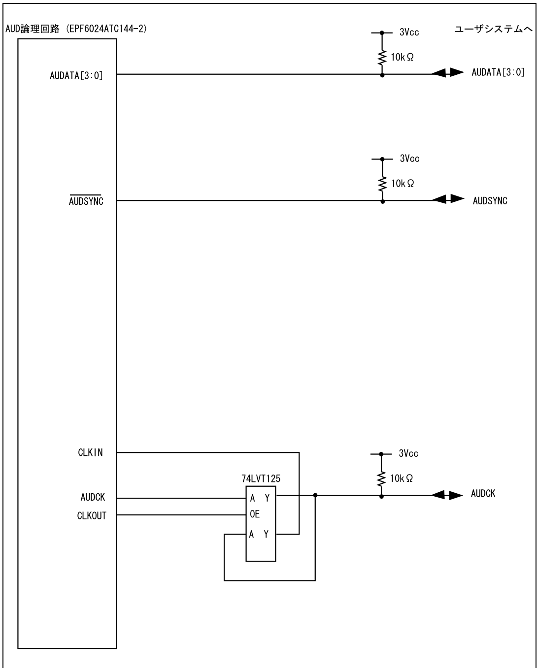
図 6.6 AUD 端子部分のユーザシステムインタフェース回路 (HS7705KCM02H) ( Model 名 : HS0005KCM04H )
