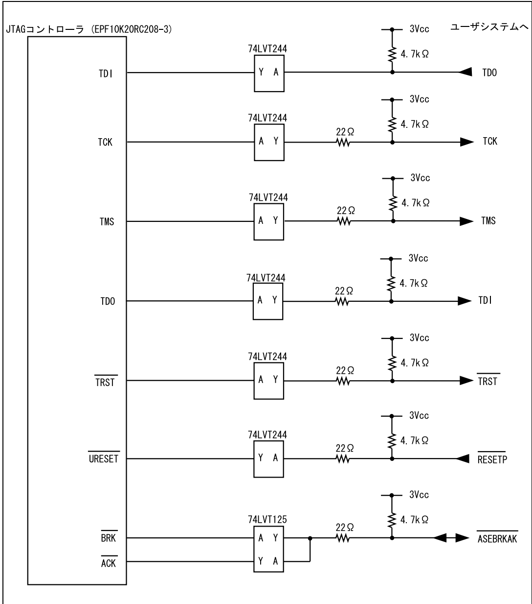
図 6.7 ユーザシステムインタフェース回路 (HS7705KCI01H) (Model 名 : HS0005KCI03H)
