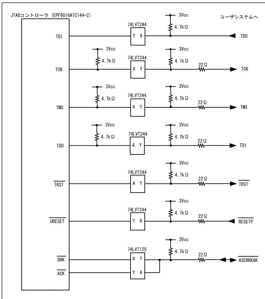
図 6.4 ユーザシステムインタフェース回路 (HS7705KCM01H) (Model名: HS0005KCM03H)
