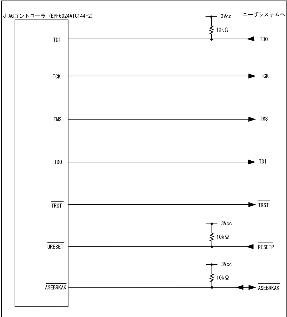
図 6.5 Hitachi-UDI 端子部分のユーザシステムインタフェース回路 (HS7705KCM02H) (Model 名 : HS0005KCM04H)
