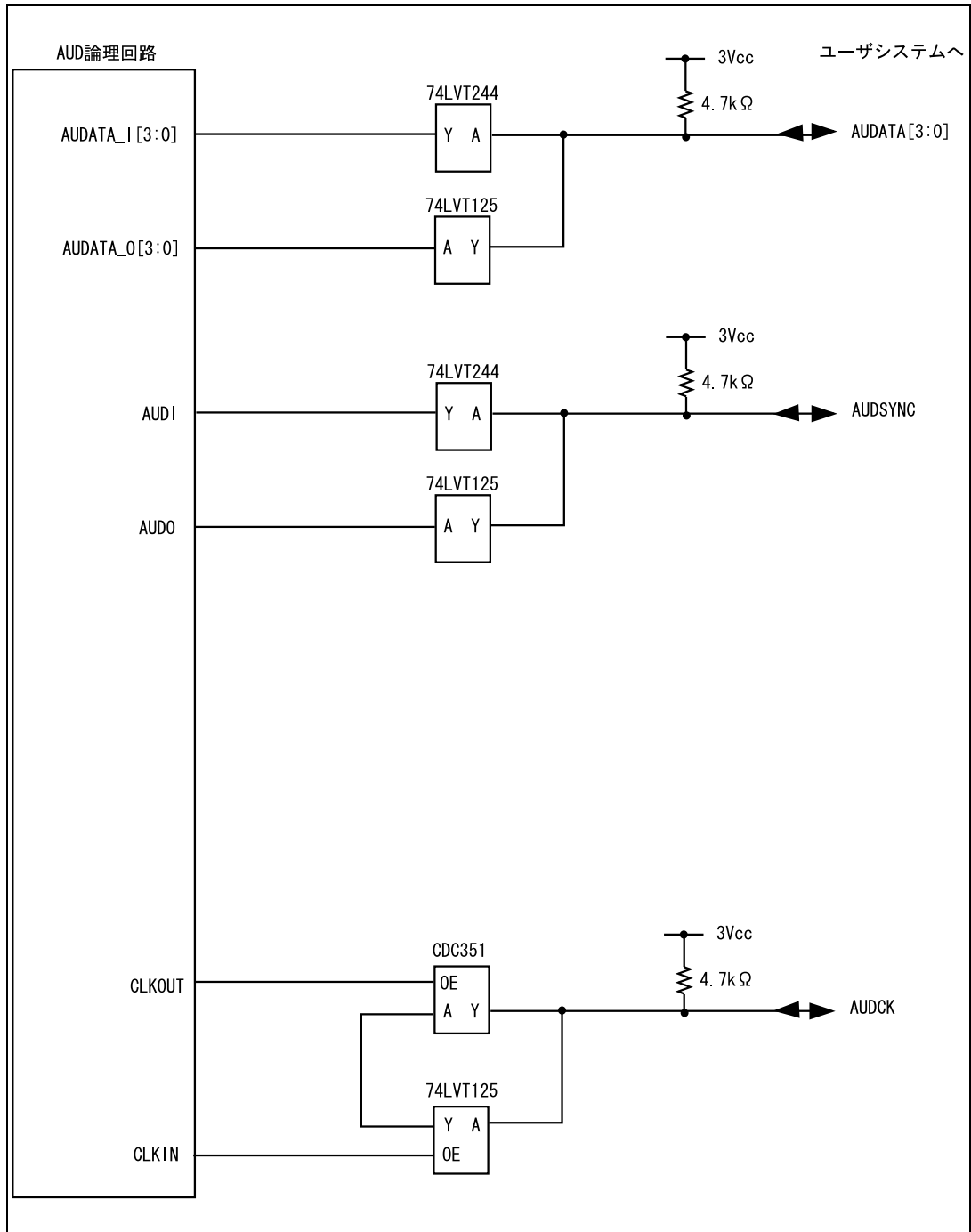
図 6.9 AUD 端子部分のユーザシステムインタフェース回路 (HS7705KC102H) ( Model 名 : HS0005KC104H )
