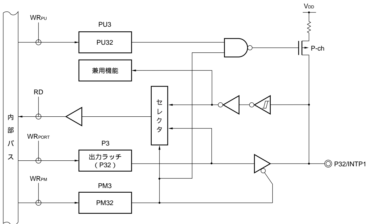
図4 - 8 P32のブロック図
