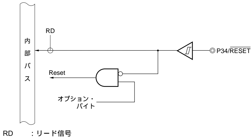
図4 - 9 P34のブロック図 ( \mu PD78F920x)
