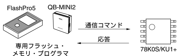
図16-7 通信コマンド
