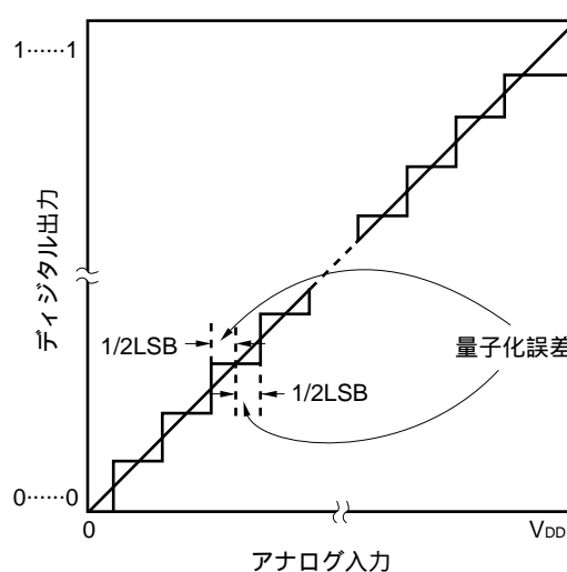
図9 - 14 量子化誤差
