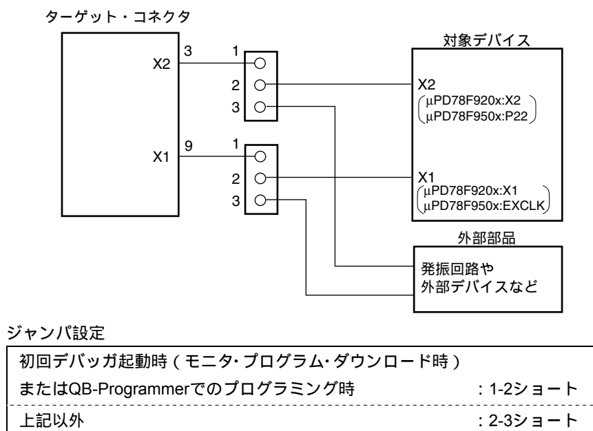
図17 - 5 X1, X2端子を使用する場合
