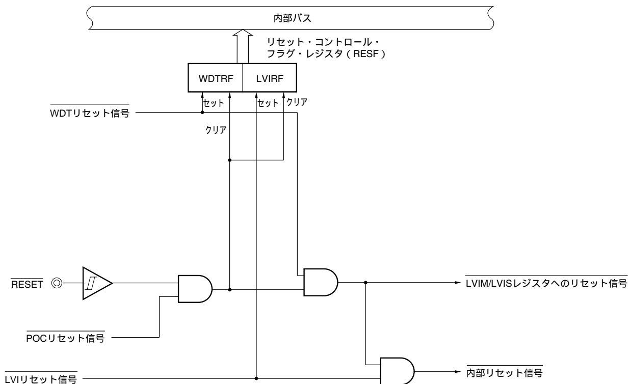
図12-1 リセット機能のブロック図
