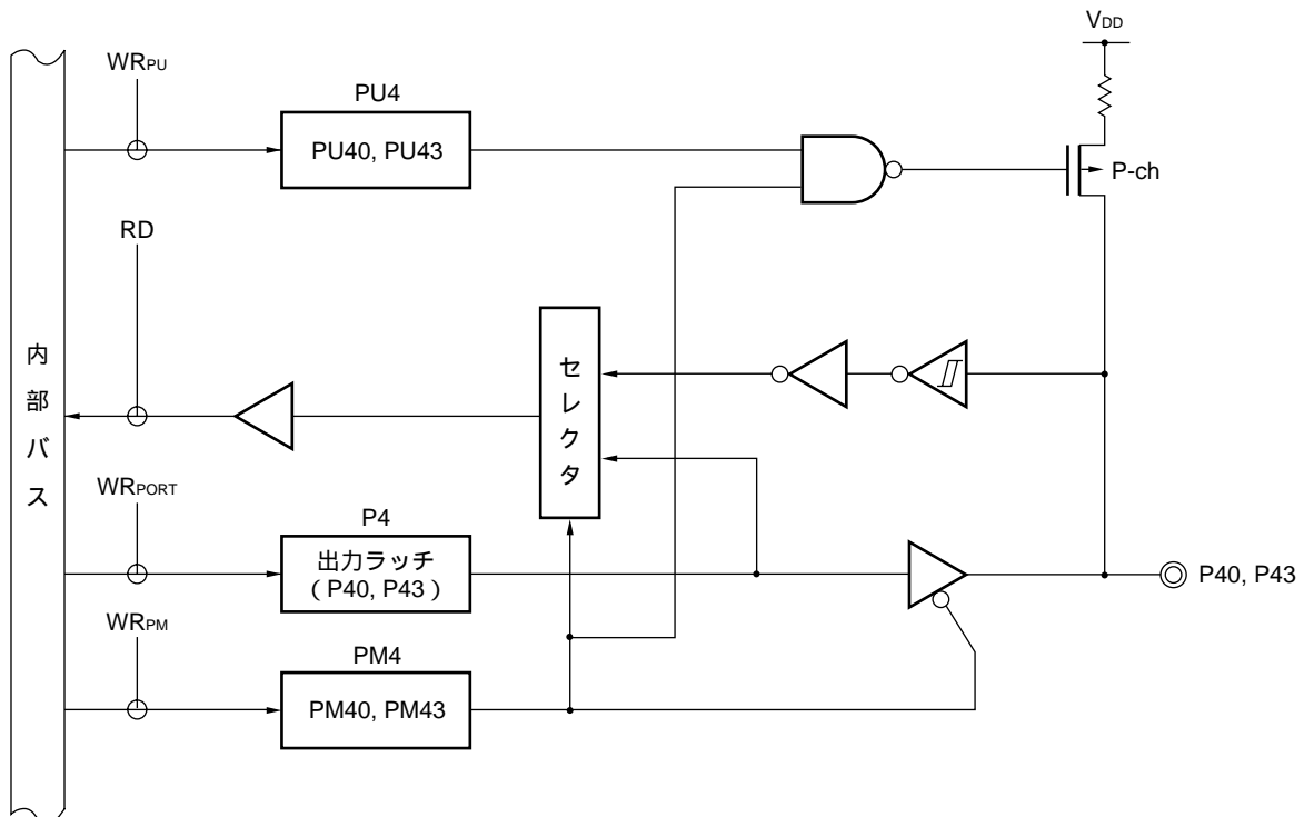
図4 - 11 P40, P43のブロック図
