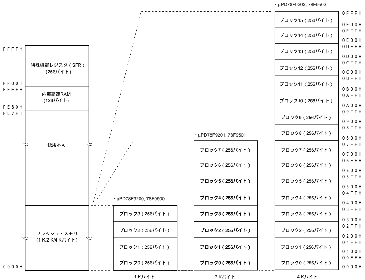
図16 - 1 フラッシュ・メモリ・マッピング
