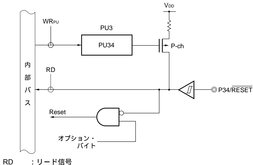
図4 - 10 P34のブロック図 ( \mu PD78F950x)
