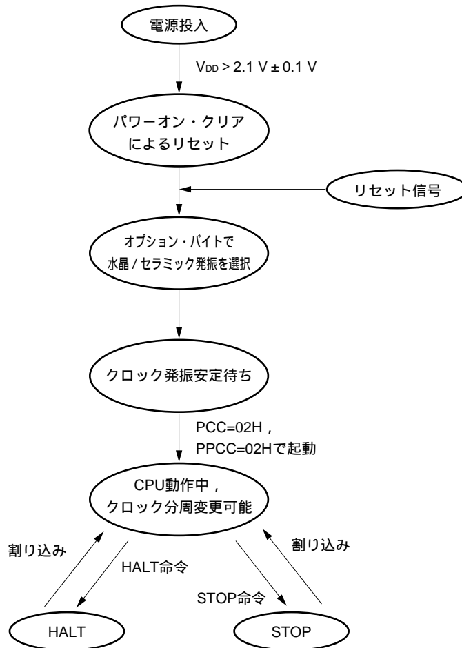
図5 - 11 水晶/セラミック発振によるデフォルト・スタートの状態遷移図 ( \mu PD78F920xのみ)
