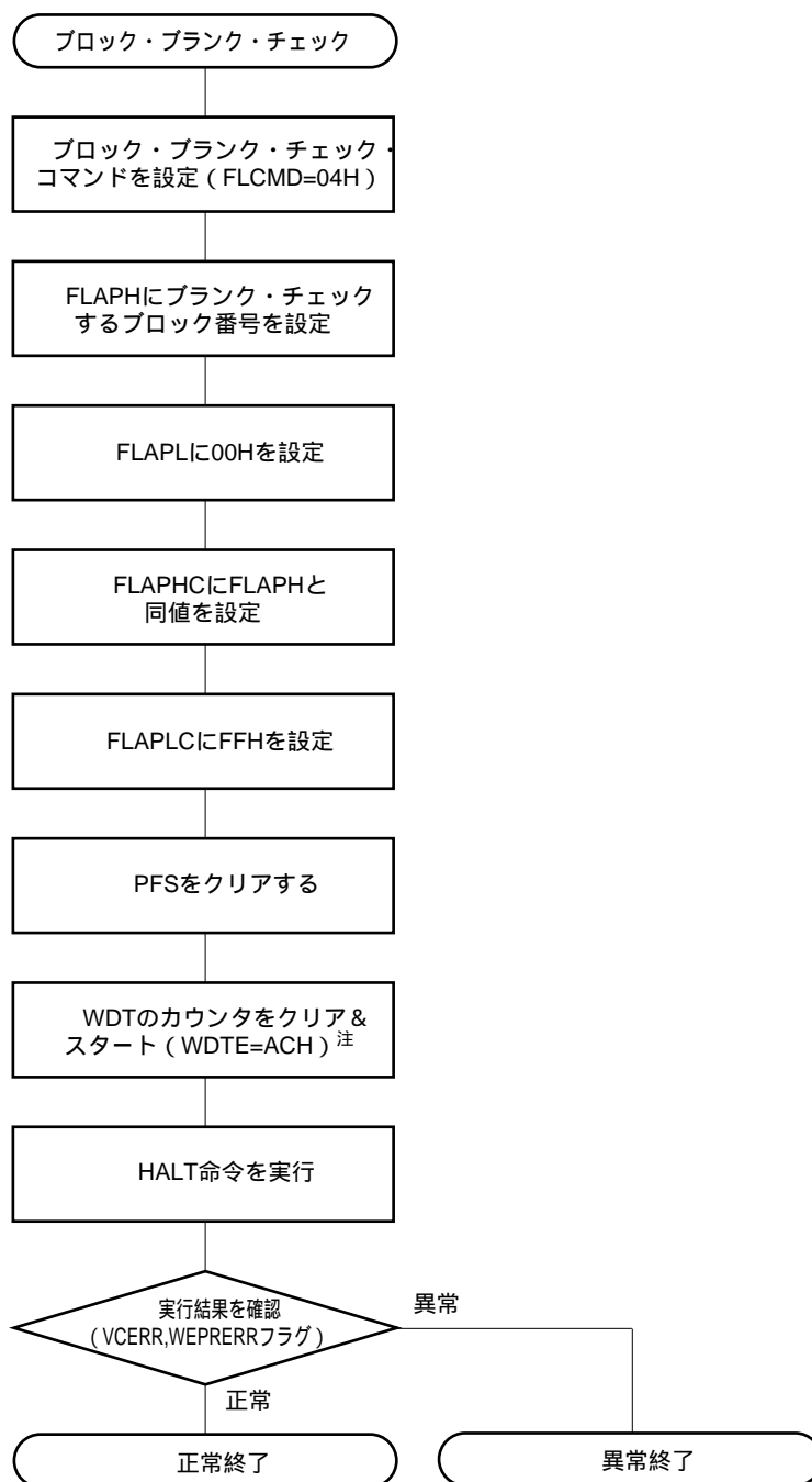
図16 - 21 セルフ・プログラミング・モードのブロック・ブランク・チェック動作例
