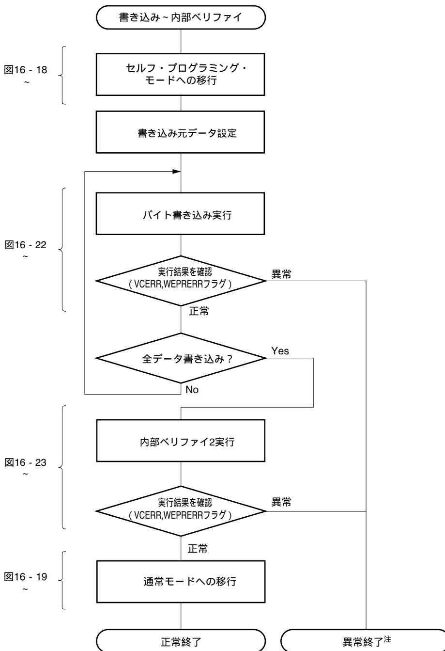
図16 - 26 コマンド実行時間を最小にしたい場合の動作例 (書き込み～内部ペリファイ)
