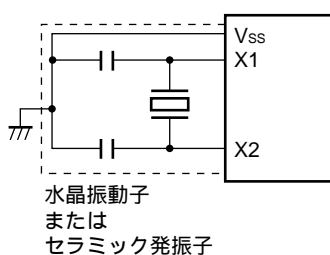
図5 - 6 水晶 / セラミック発振回路の外付け回路 ( \mu PD78F920xのみ)
