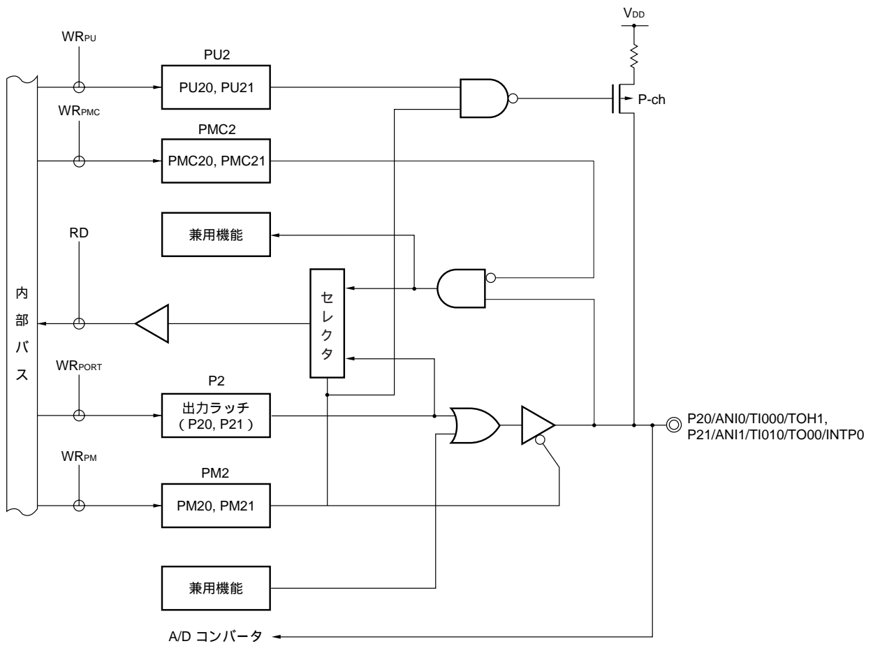
図4 - 2 P20, P21のブロック図 (μ PD78F920x)
