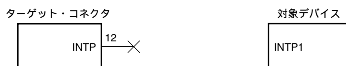
図17 - 3 QB-MINI2をプログラミング用にのみ使用する場合
