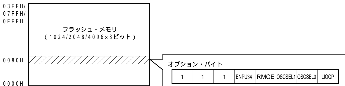
図15 - 2 オプション・バイトの位置 ( \mu PD78F950x)
