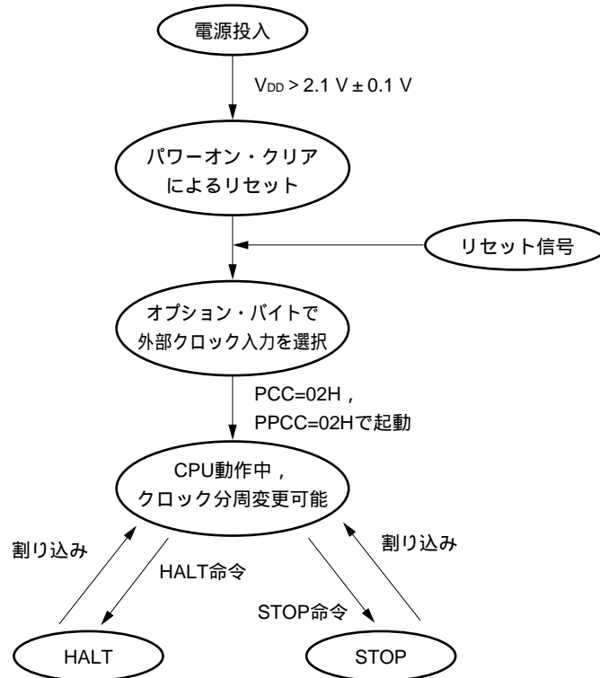
図5 - 13 外部クロック入力によるデフォルト・スタートの状態遷移図
