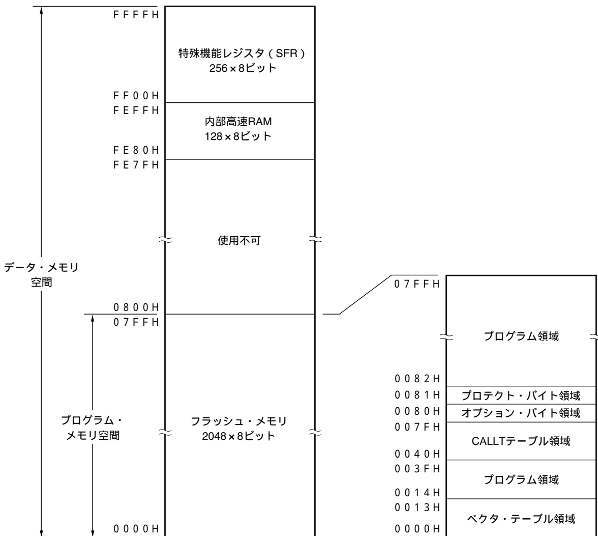
図3 - 2 メモリ・マップ (μ PD78F9201, 78F9501)
