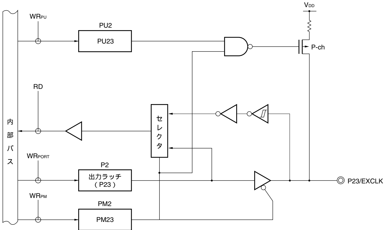
図4 - 7 P23のブロック図 (μ PD78F950x)
