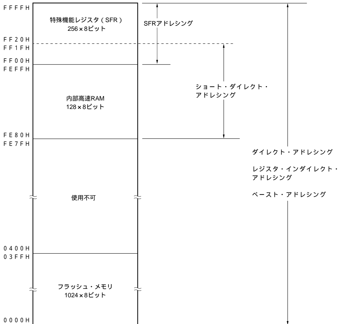
図3 - 4 データ・メモリのアドレッシング (μ PD78F9200, 78F9500)
