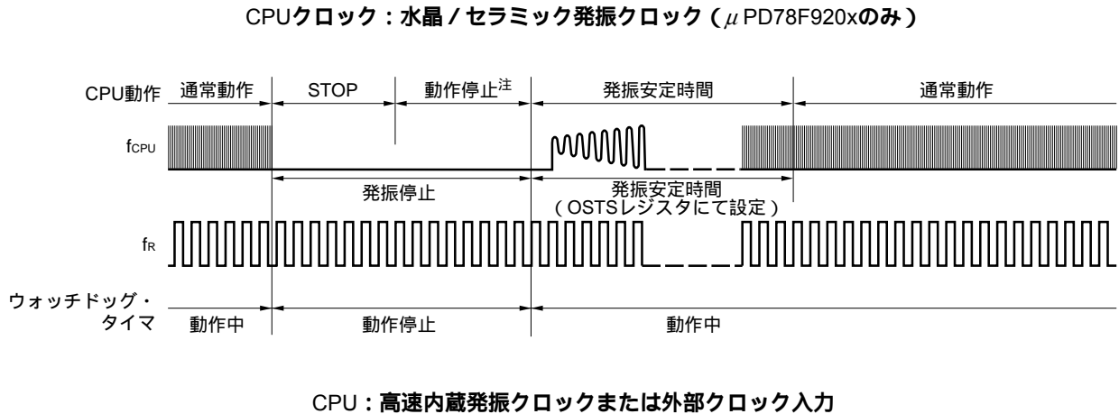
図8 - 7 STOPモード時の動作 (WDT動作クロック：低速内蔵発振クロック)
