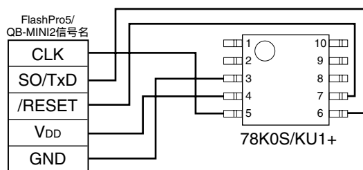
図16 - 3 FlashPro5/QB-MINI2との配線図
