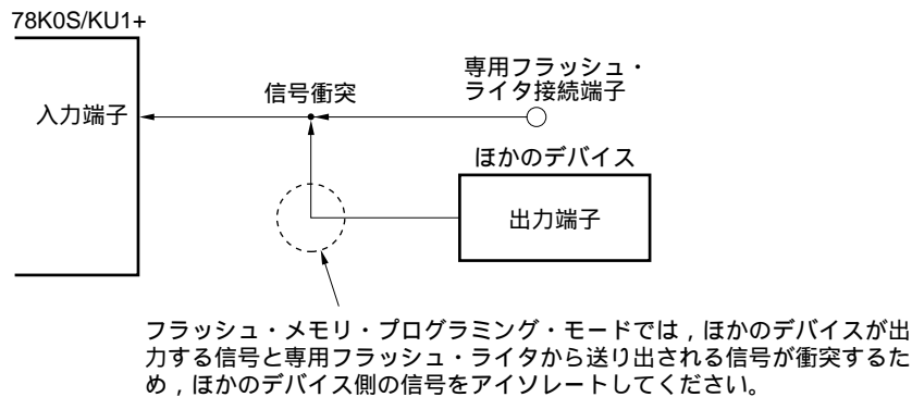
図16-6 信号の衝突 (RESET端子)
