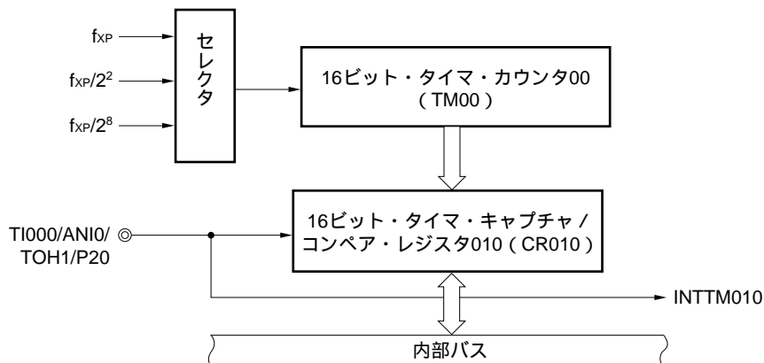
図6 - 20 フリー・ランニング・カウンタによるパルス幅測定の構成図
