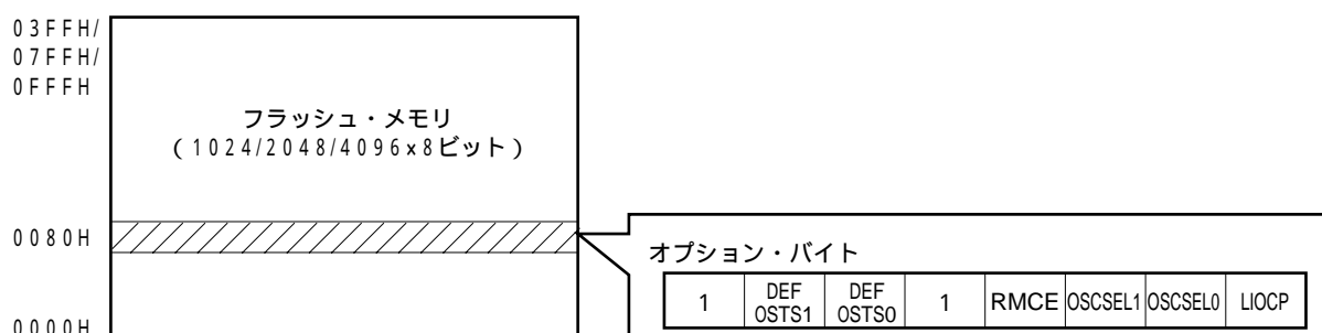
図15-1 オプション・バイトの位置 ( \mu PD78F920x)
