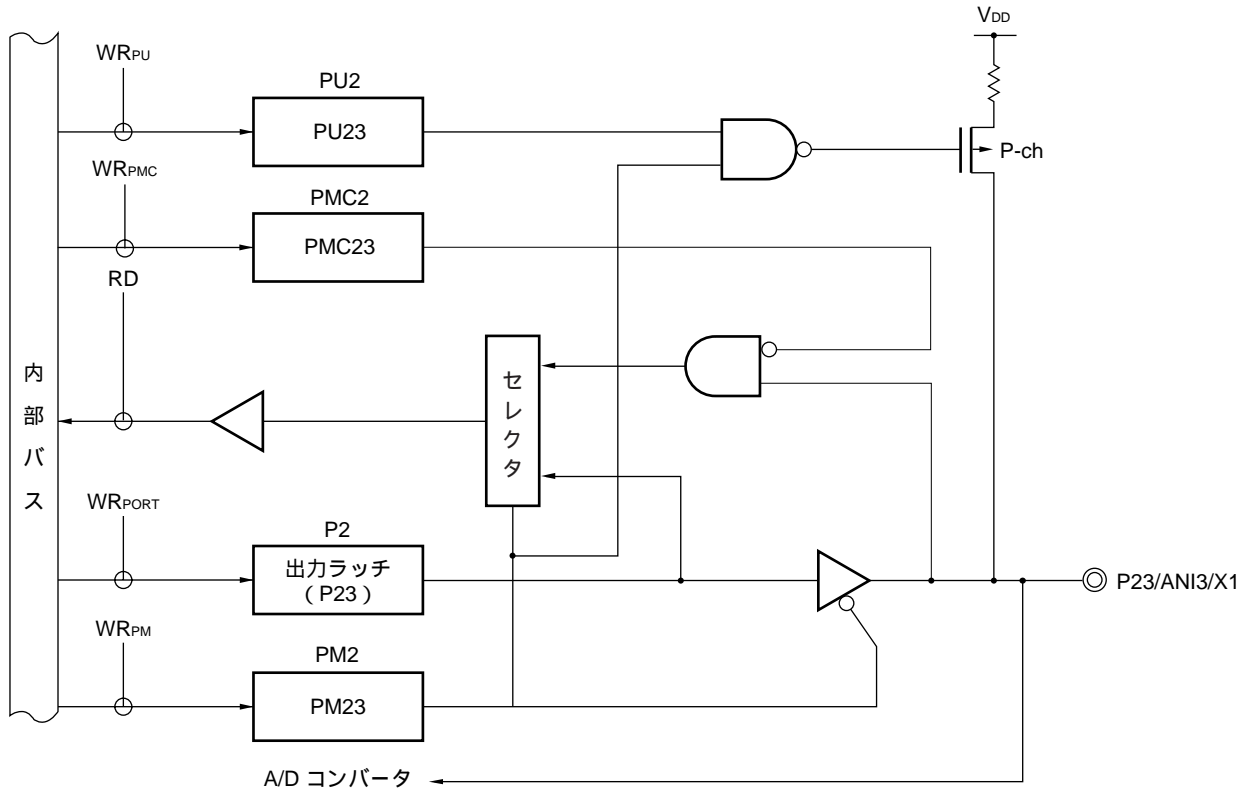
図4 - 4 P23のブロック図 (μ PD78F920x)
