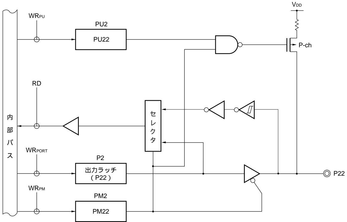
図4 - 6 P22のブロック図 ( \mu PD78F950x)
