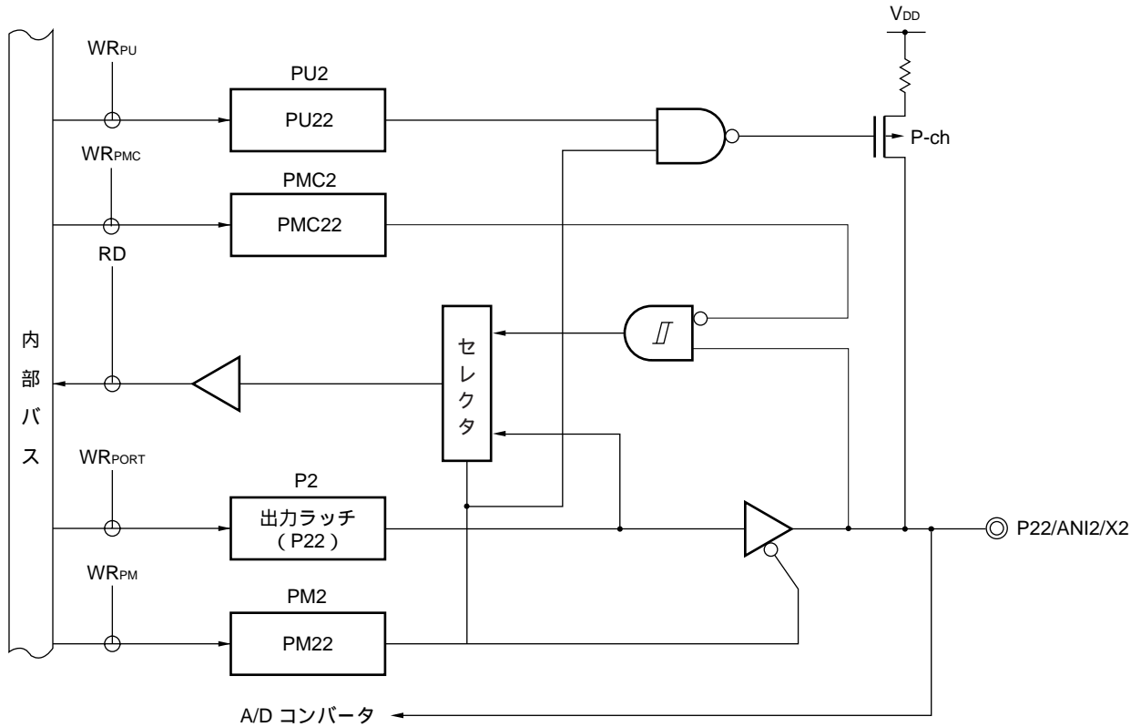
図4 - 3 P22のブロック図 (μ PD78F920x)
