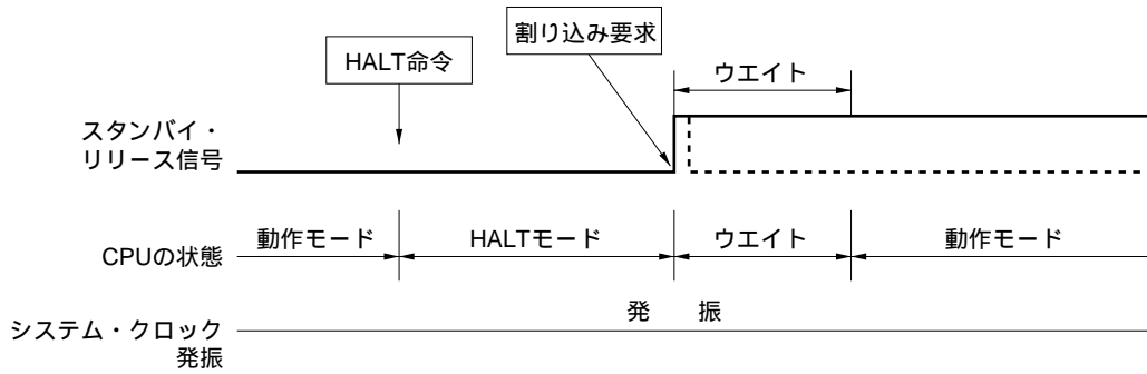
図11-2 HALTモードの割り込み要求発生による解除
