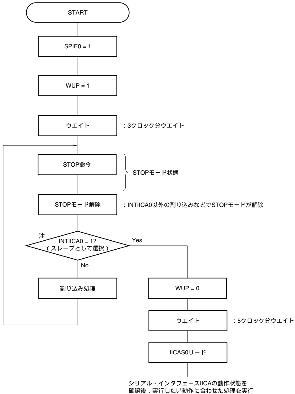
図16 - 24 INTIICA0以外でSTOPモードが解除後にスレーブとして動作させる場合 (マスタとして動作させる必要がない場合)
