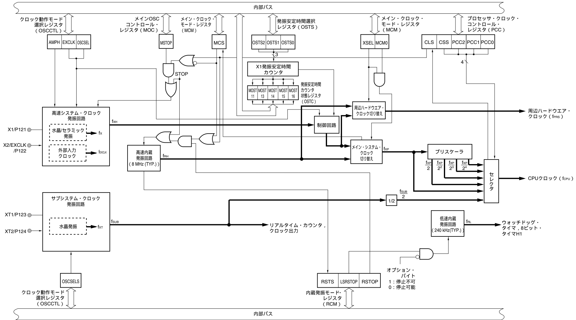
図5-2 クロック発生回路のブロック図 (78K0/KC2-A (48ピン))
