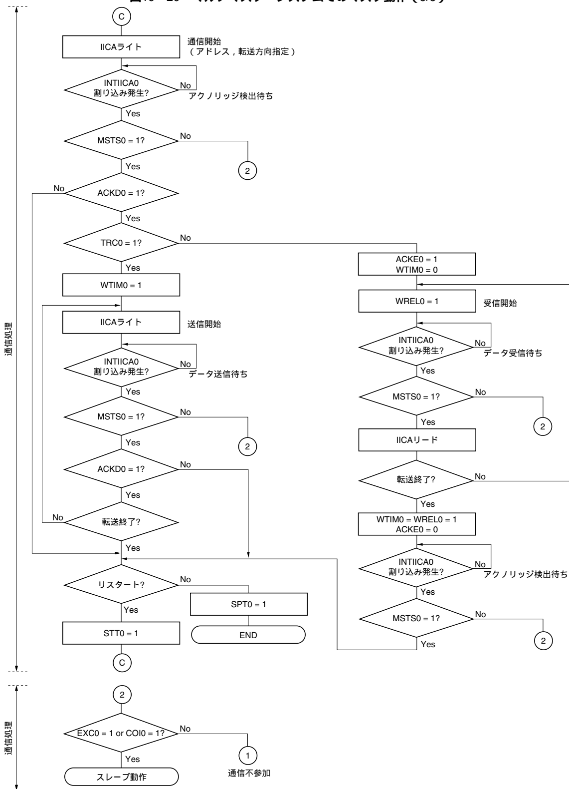
図16 - 29 マルチマスタ・システムでのマスタ動作 (3/3)
