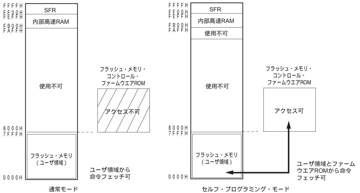
図25 - 12 セルフ・プログラミングの動作モードとメモリ・マップ ( \mu PD78F0593の場合)
