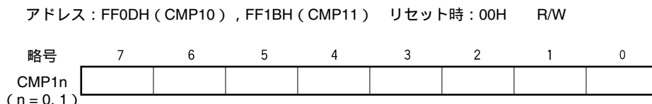
図8-4 8ビット・タイマHコンペア・レジスタ1n (CMP1n) のフォーマット
