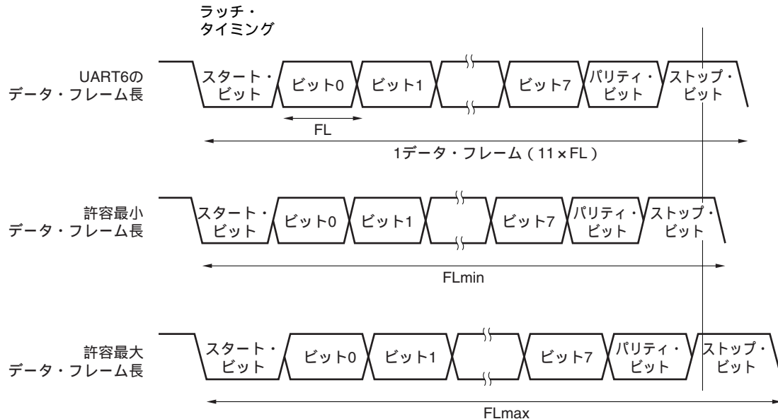
図14 - 25 受信時の許容ボー・レート範囲
