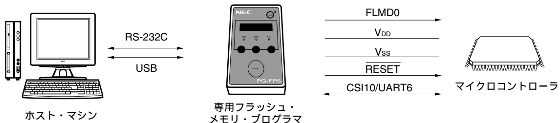
図25-2 フラッシュ・メモリにプログラムを書き込むための環境
