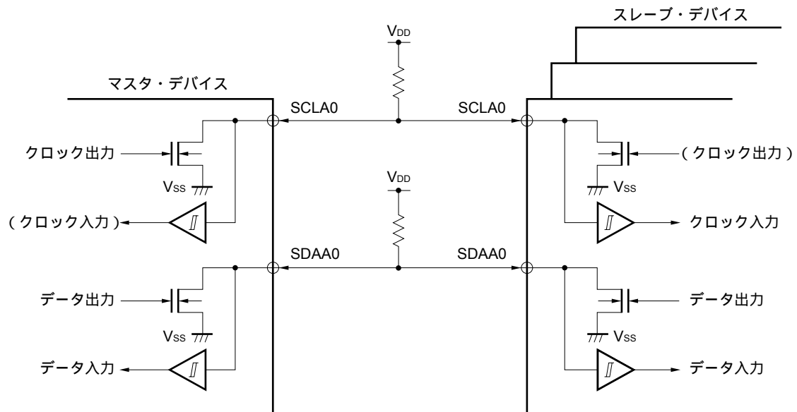
図16 - 12 端子構成図
