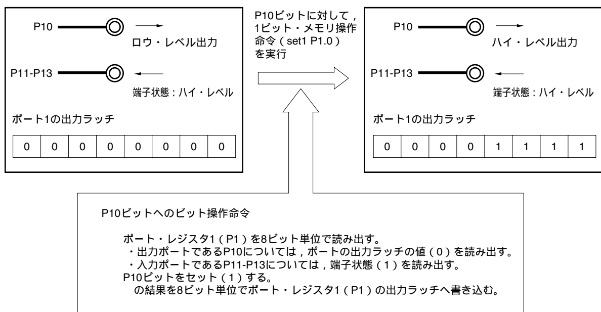
図4 - 29 ビット・メモリ操作命令（P10の場合）
