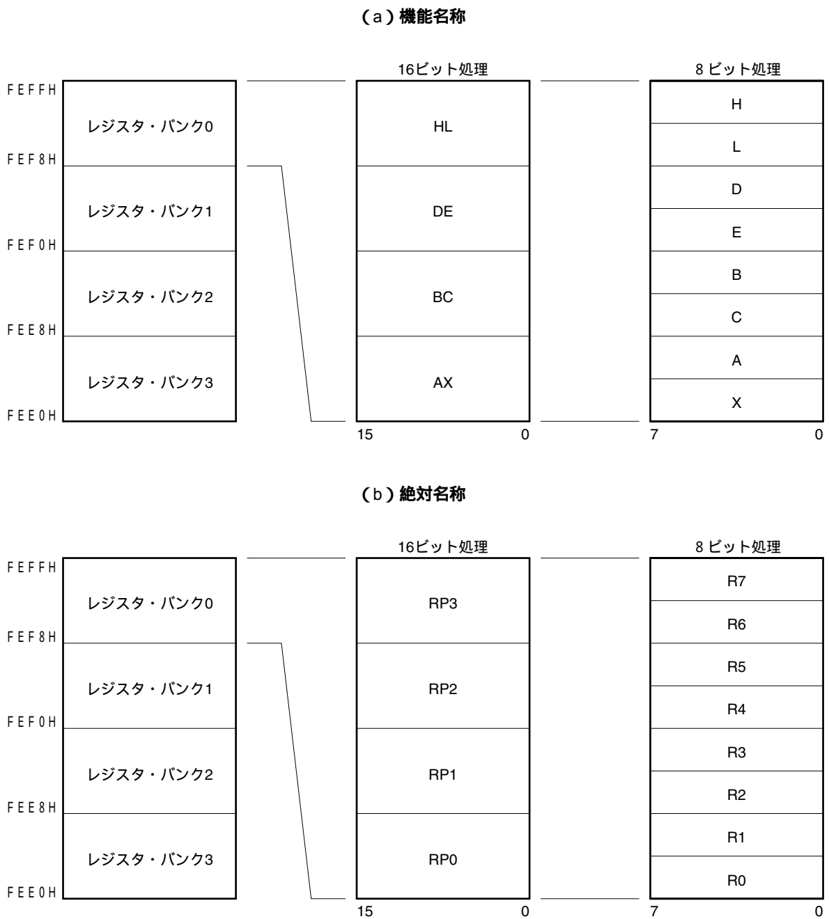
図3 - 10 汎用レジスタの構成
