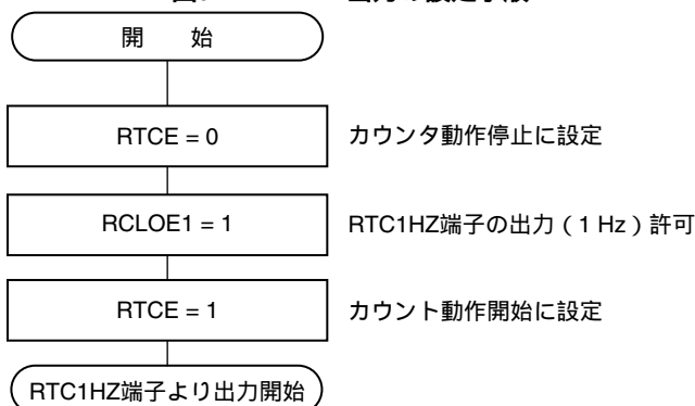
図9 - 22 1 Hz出力の設定手順
