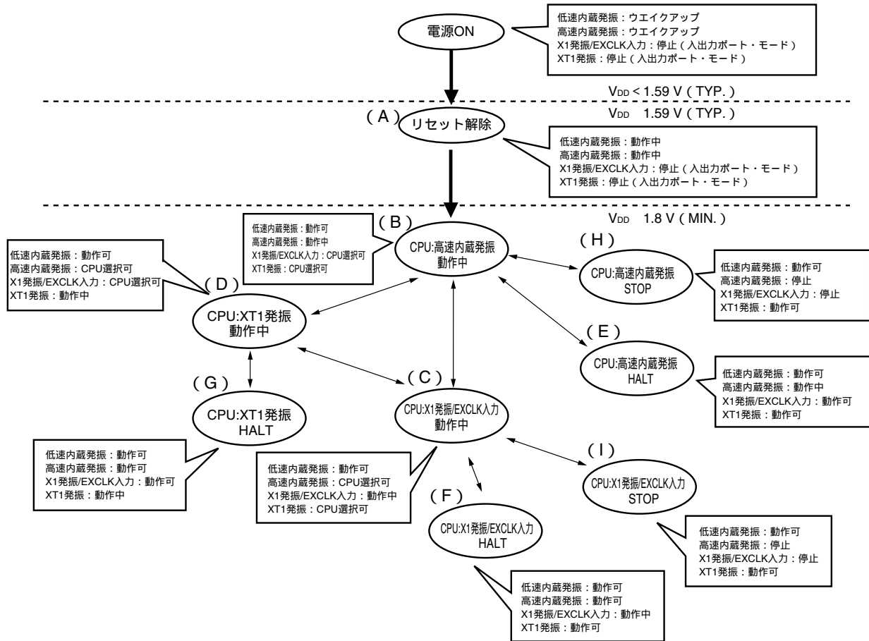
図5-16 CPUクロック状態移行図 (1.59 V POCモード設定時 (オプション・バイト: POCMODE = 0)) (78K0/KC2-A (48ピン))
