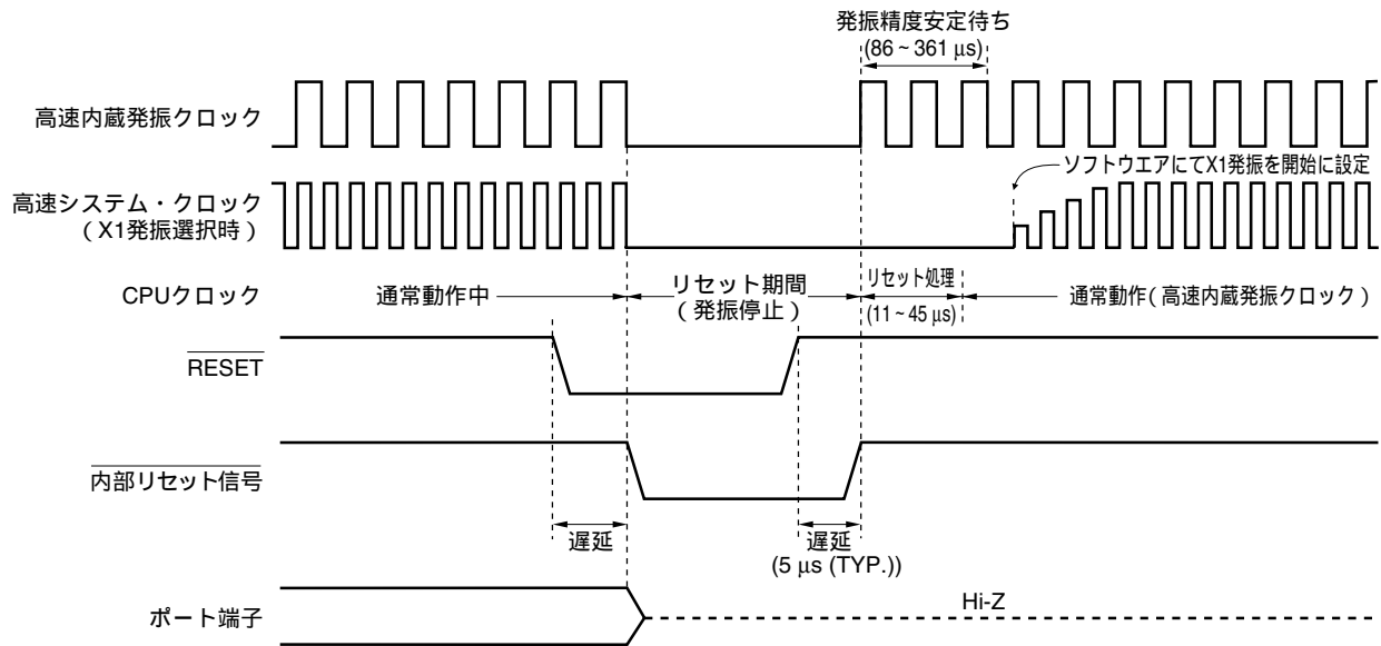
図21 - 2 \overline{\text{RESET}} 入力によるリセット・タイミング
