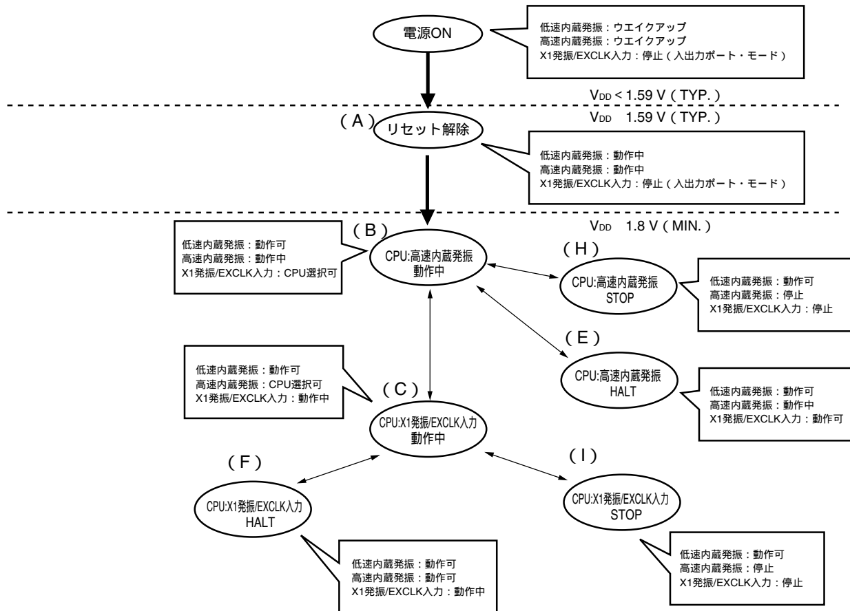
図5 - 15 CPUクロック状態移行図 (1.59 V POCモード設定時 (オプション・バイト : POCMODE = 0) ) (78K0/KB2-A, 78K0/KC2-A (36ピン) )
