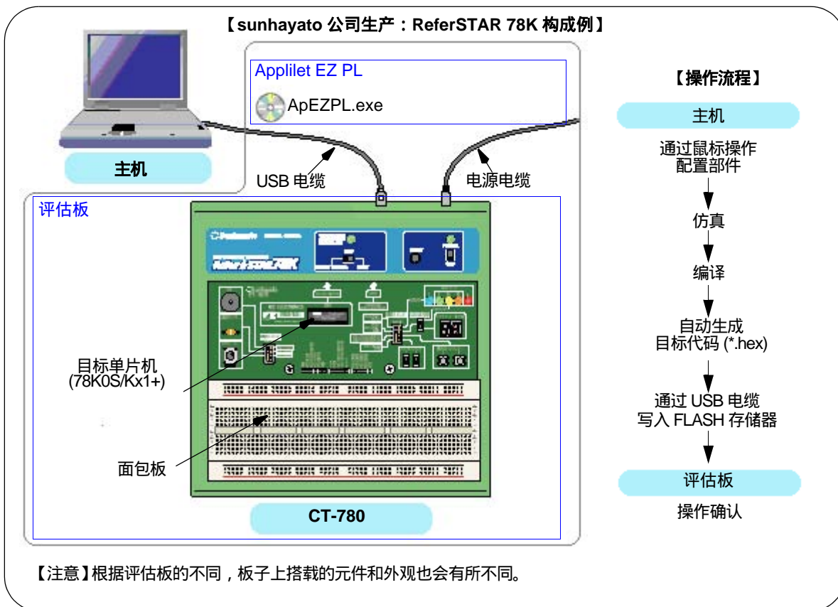
图 1-2 系统构成
