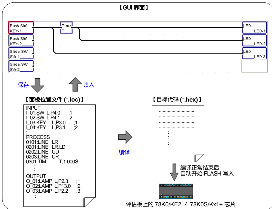
图 5-5 目标代码的自动生成 / FLASH 写入的操作
