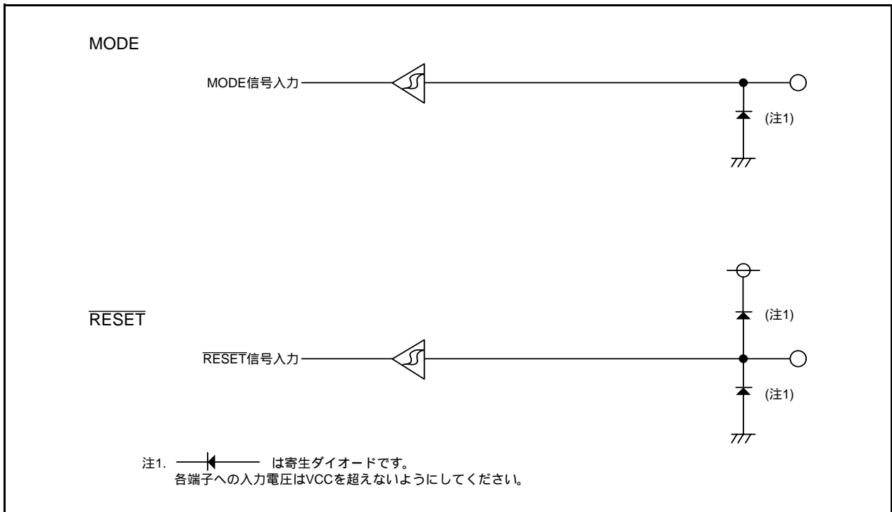
図7.13 端子の構成
