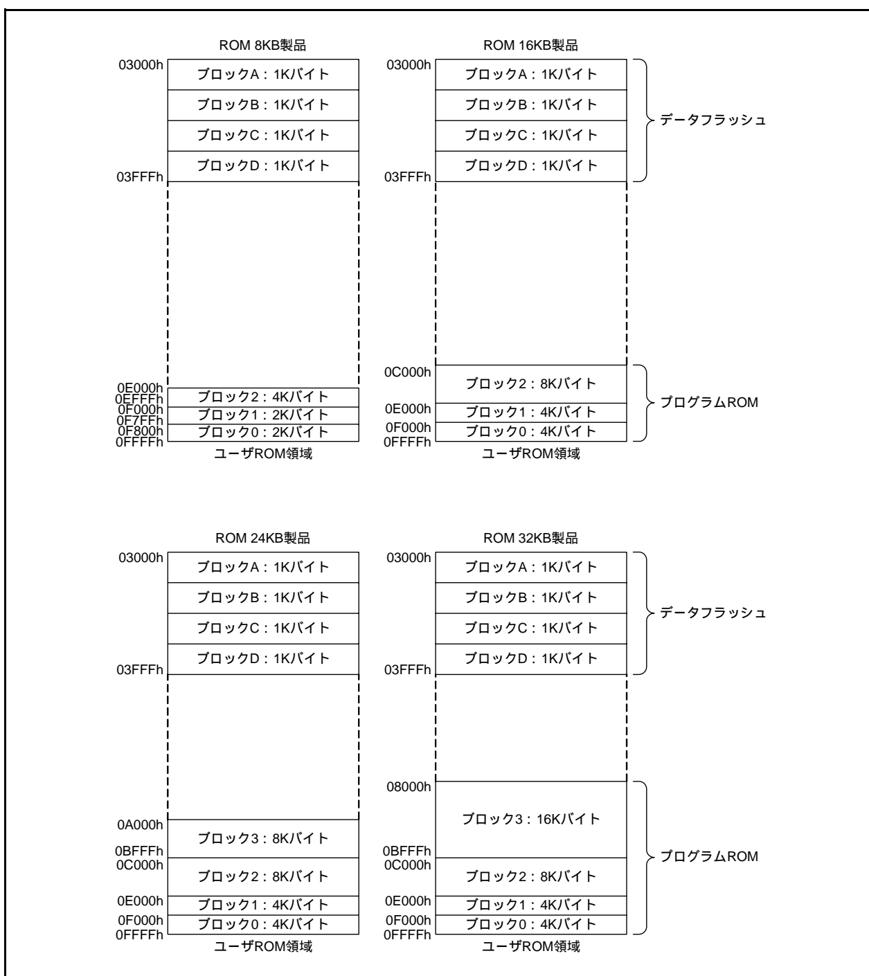
図 31.1 R8C/3JCグループのフラッシュメモリのブロック図
