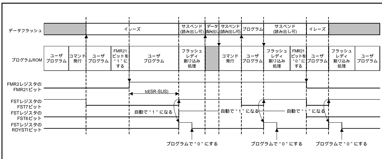
図 31.3 サスペンド動作に関するタイミング
