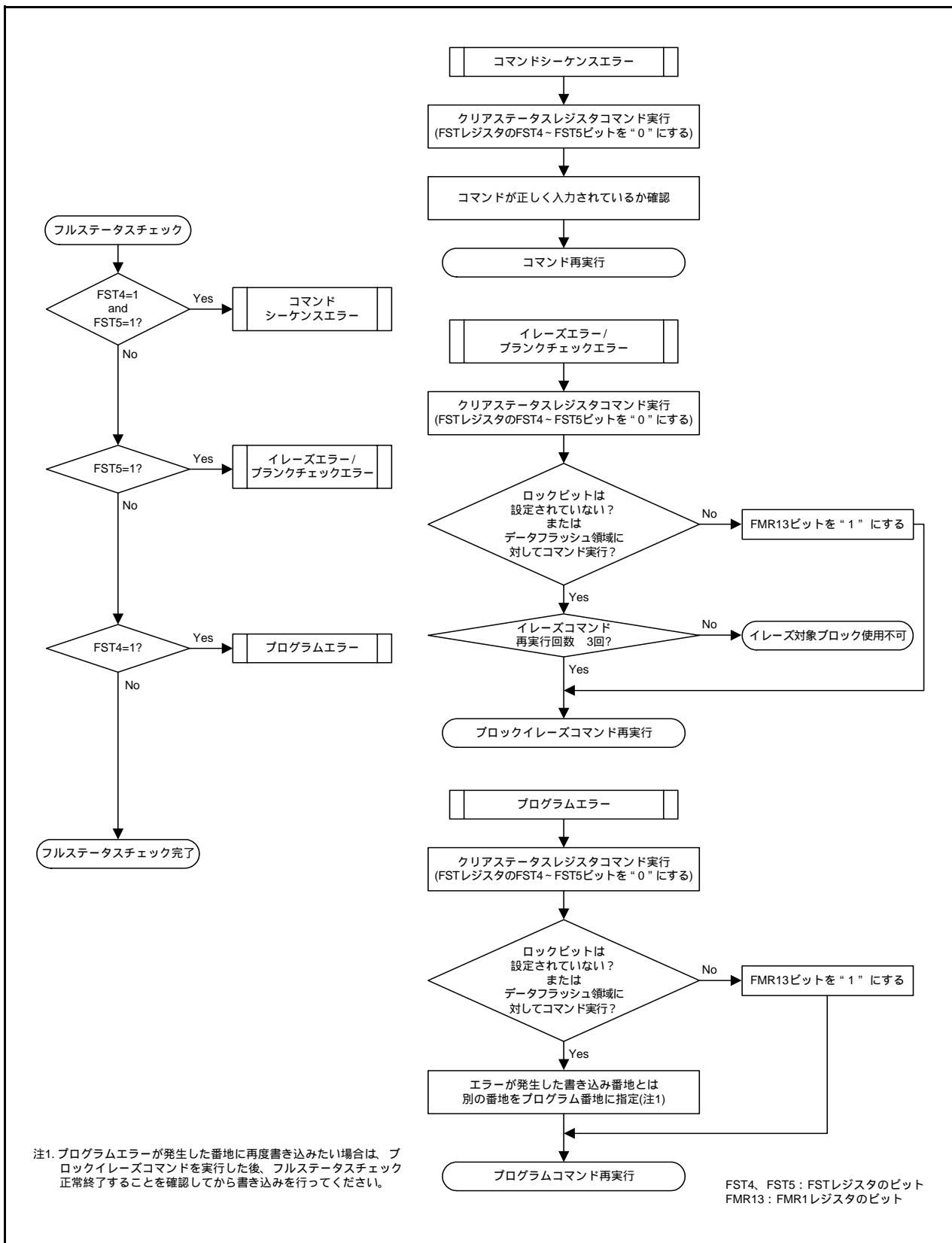
図 31.16 フルステータスチェックフローチャート、各エラー発生時の対処方法
