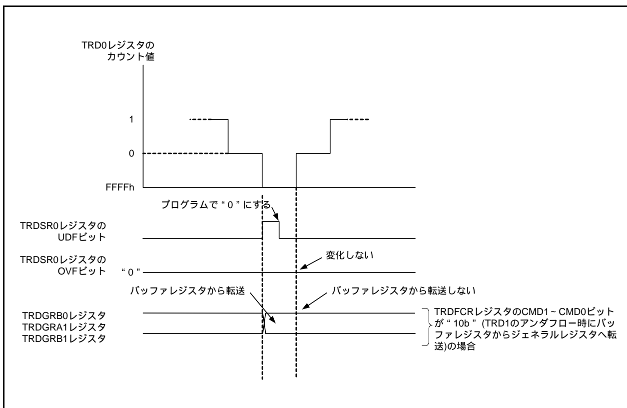
図 34.3 相補PWMモード TRD1がアンダフローしたときの動作
