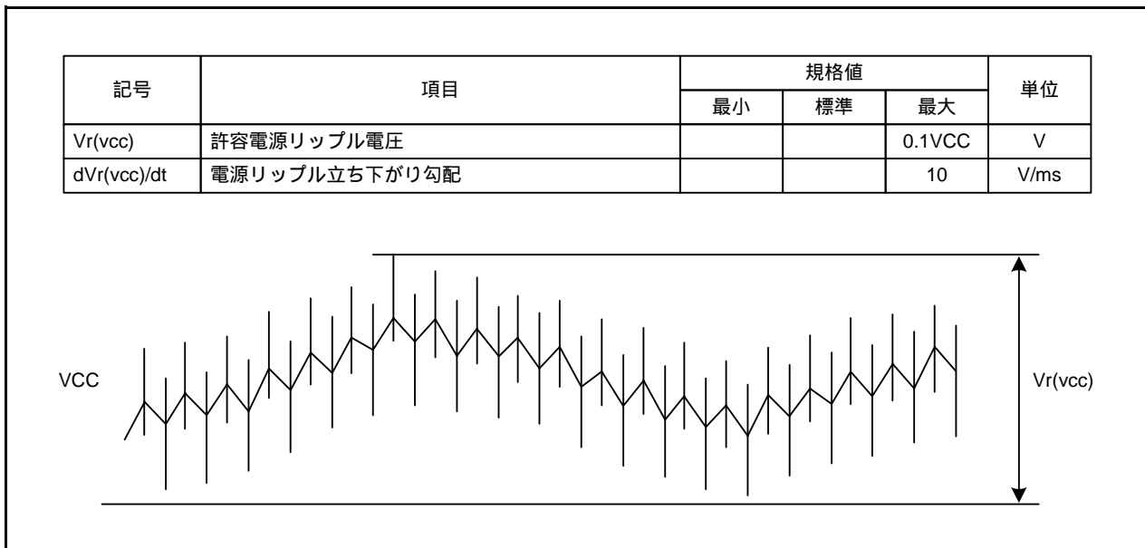
図34.7 電源リップルの定義
