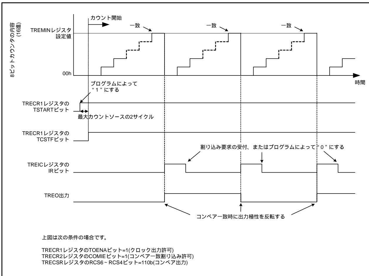
図 21.5 アウトプットコンペアーモードの動作例
