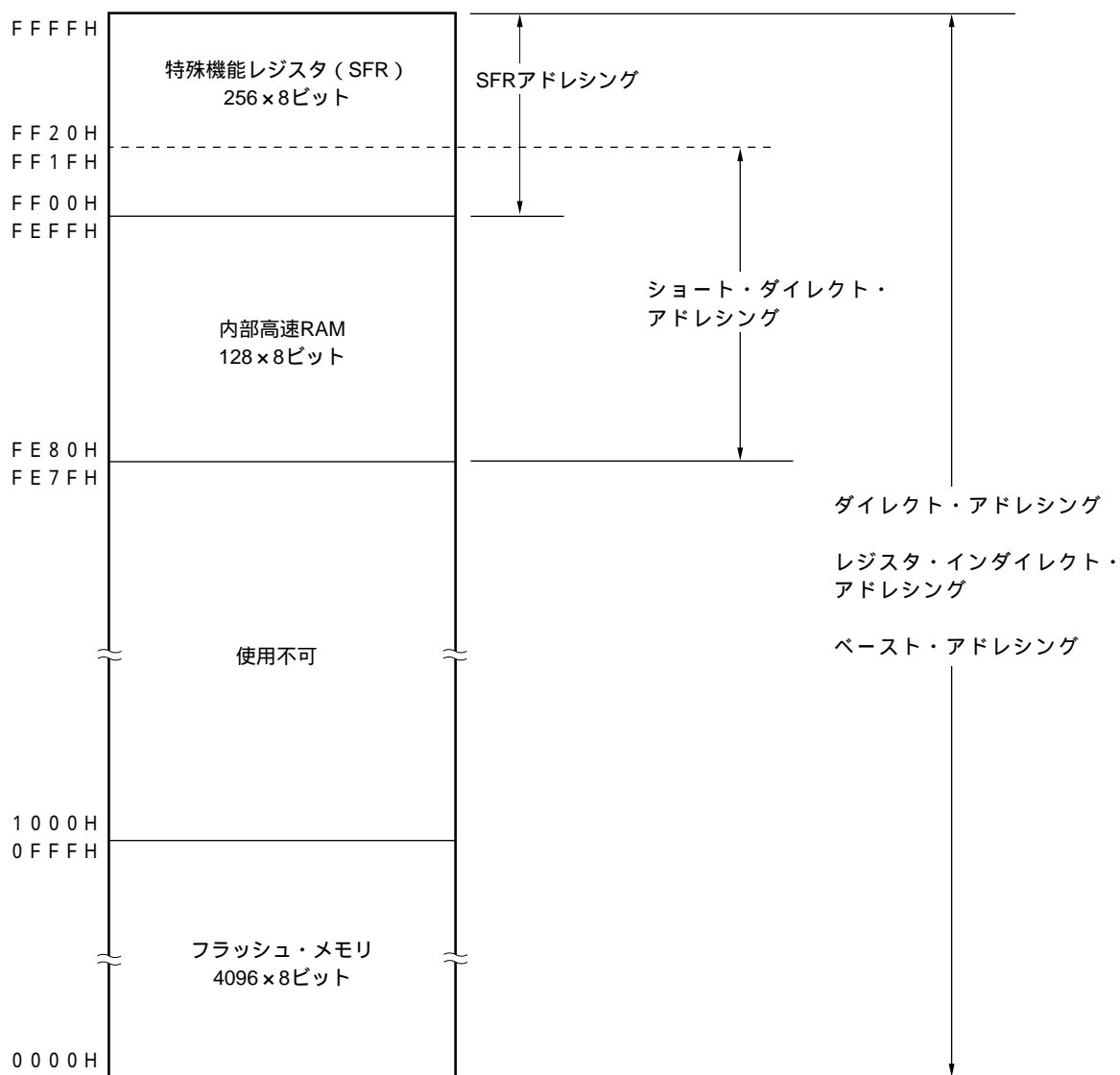
図3-6 データ・メモリのアドレッシング ( \mu PD78F9512)
