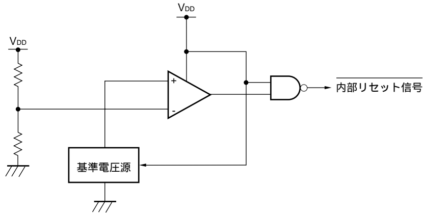
図12 - 1 パワーオン・クリア回路のブロック図
