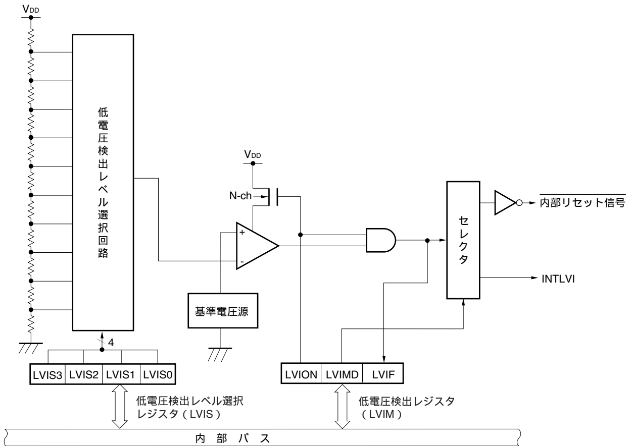
図13 - 1 低電圧検出回路のブロック図
