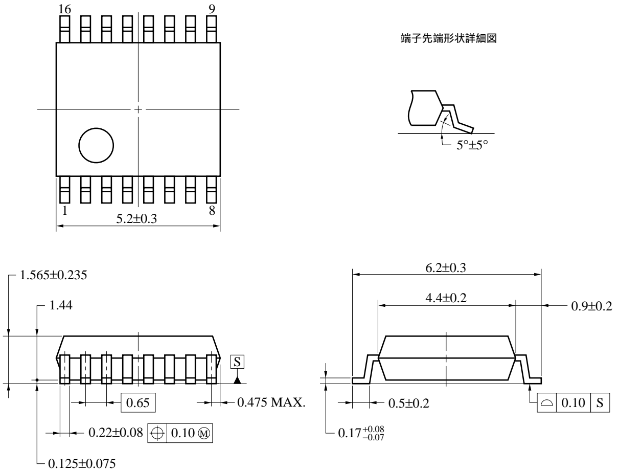
16ピン・プラスチック・SSOP (5.72 mm (225)) 外形図 (単位: mm)
