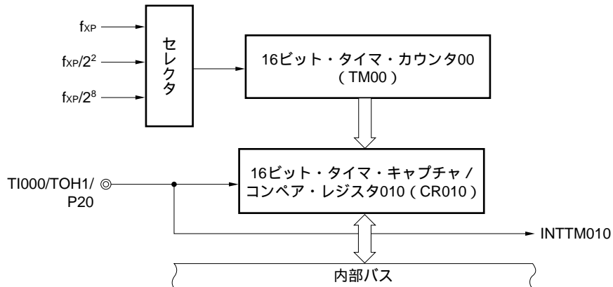
図6 - 19 フリー・ランニング・カウンタによるパルス幅測定の構成図
