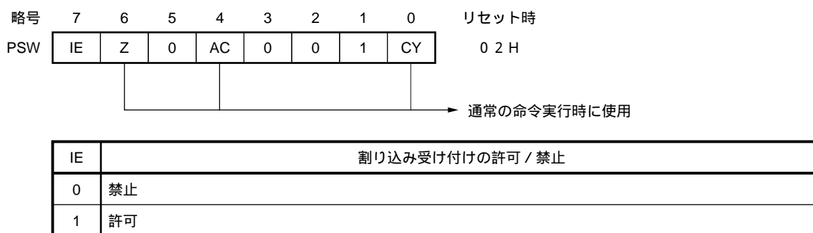
図9-5 プログラム・ステータス・ワード (PSW) の構成
