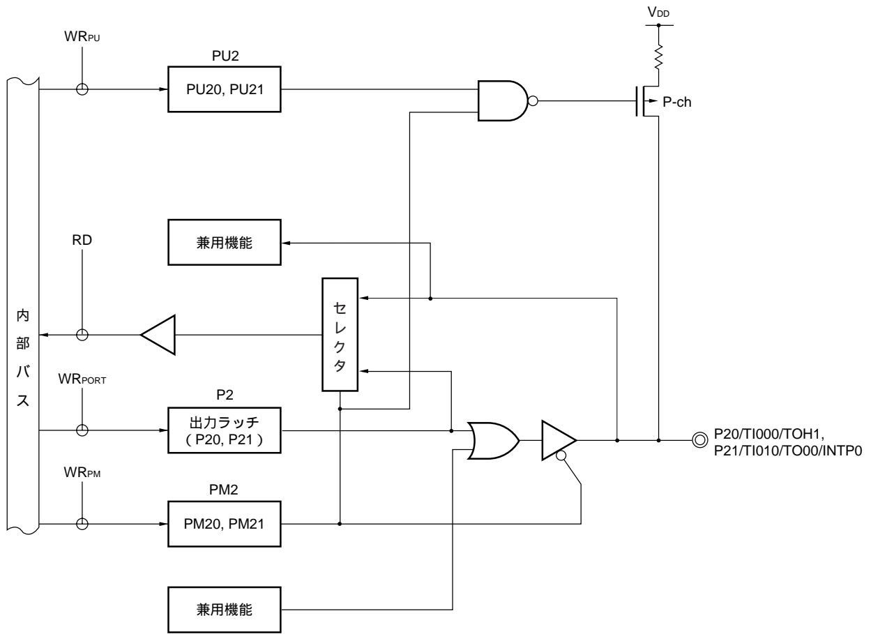
図4 - 2 P20, P21のブロック図
