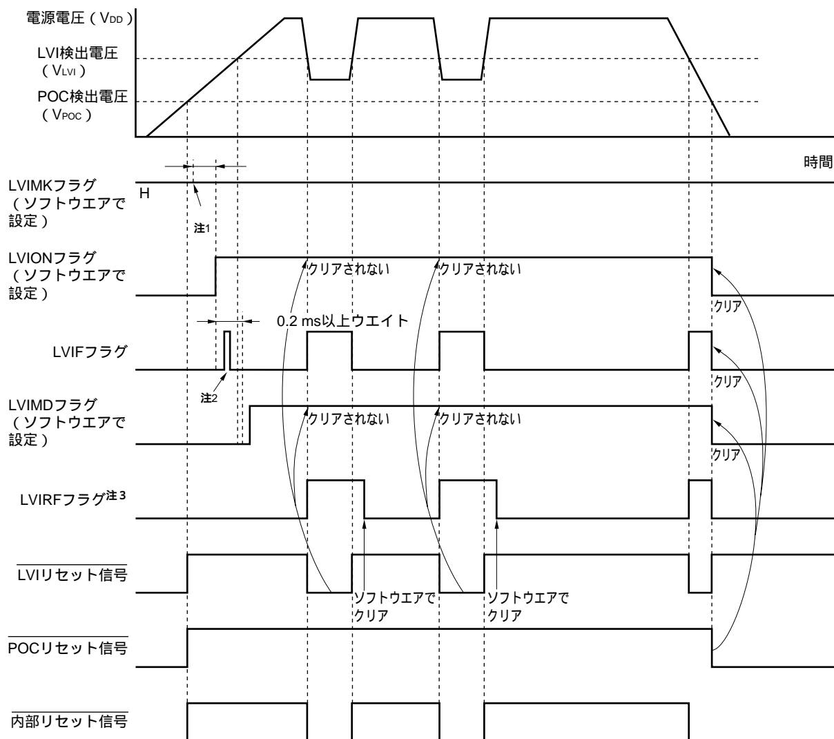
図13-4 低電圧検出回路の内部リセット信号発生タイミング
