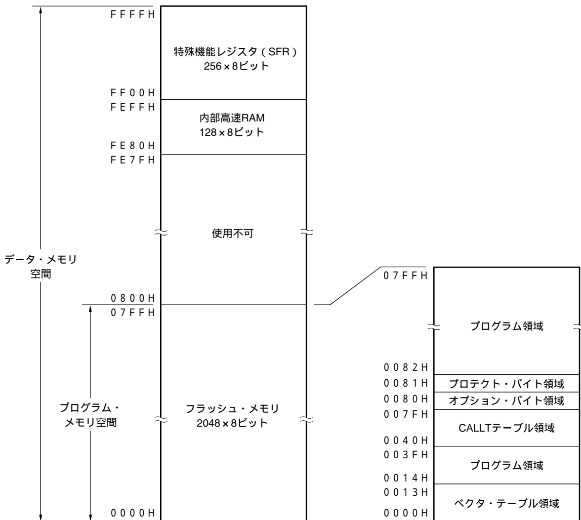
図3-2 メモリ・マップ (μ PD78F9511)
