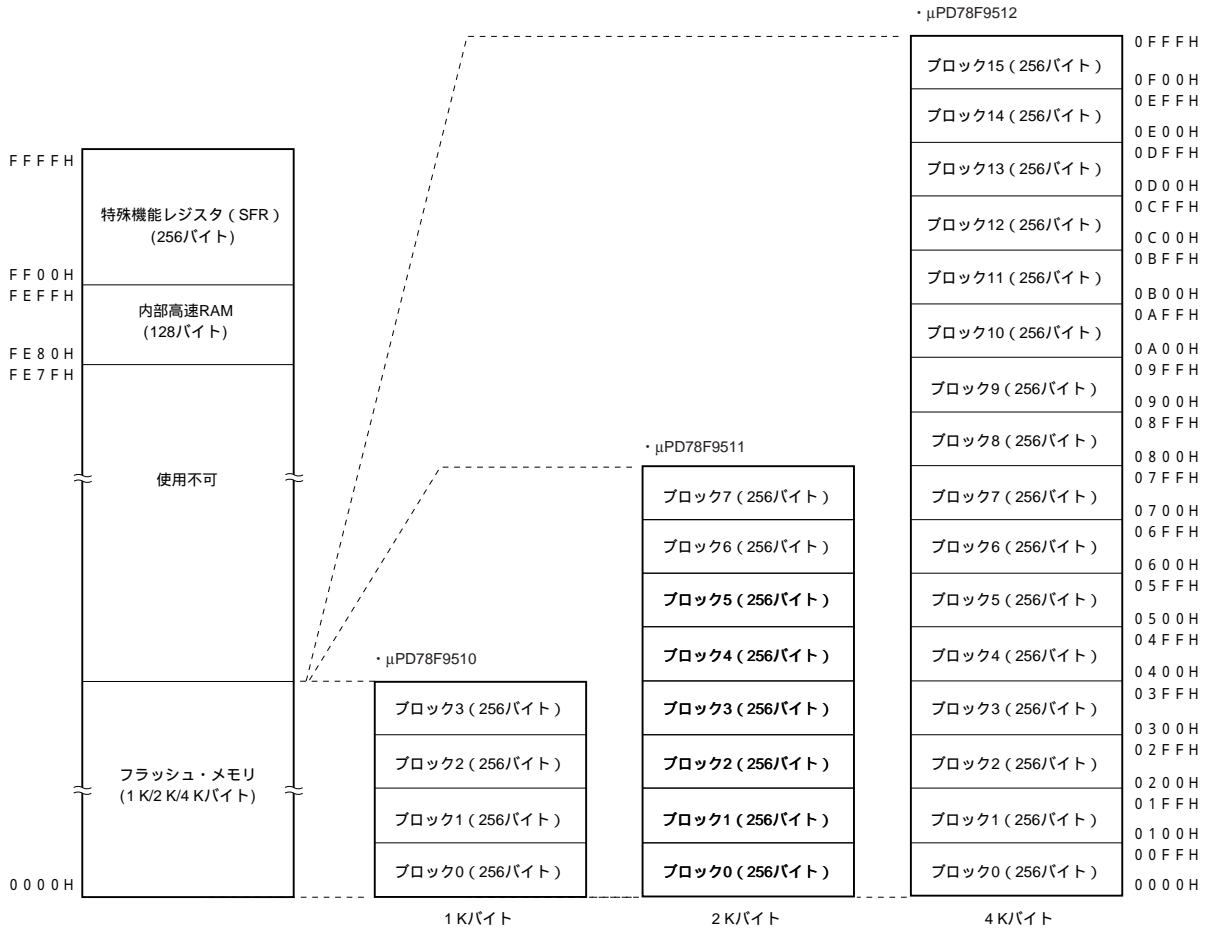
図15-1 フラッシュ・メモリ・マッピング
