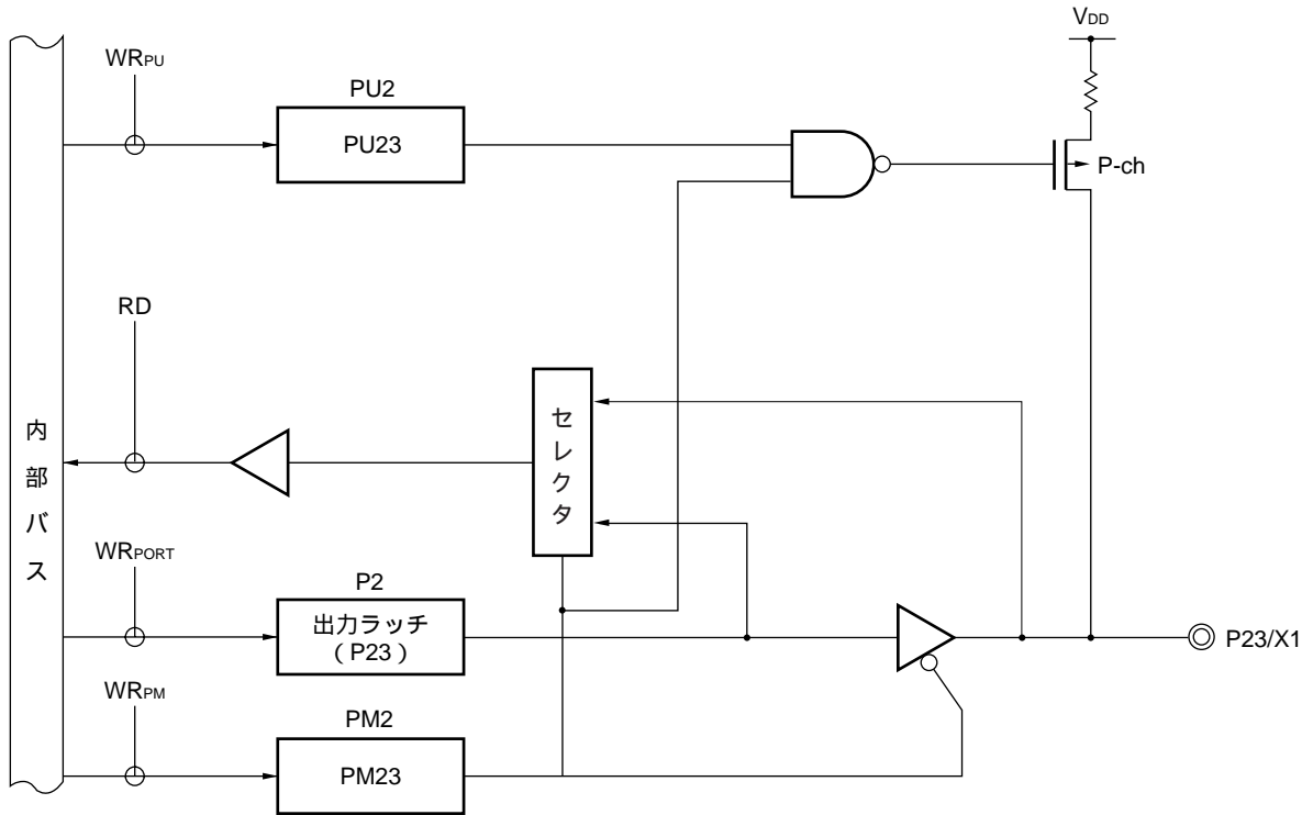
図4 - 4 P23のブロック図
