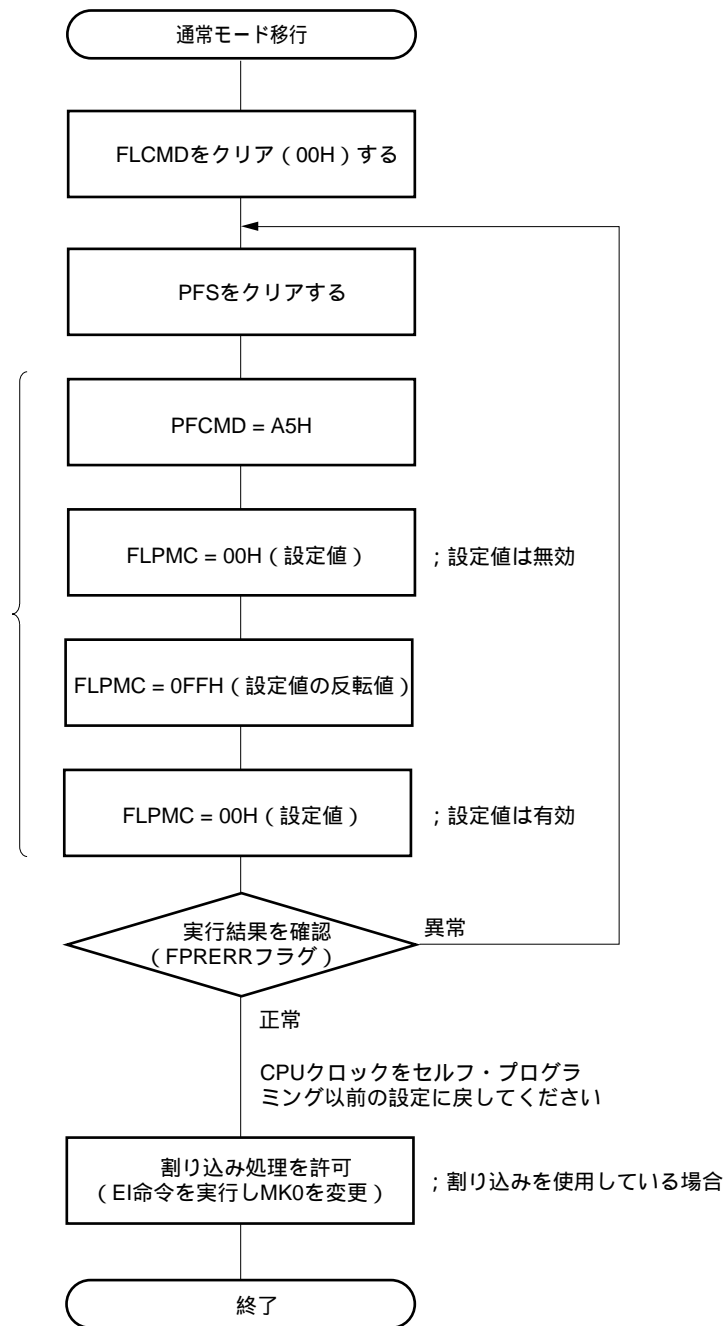
図15 - 21 通常モードへの移行例
