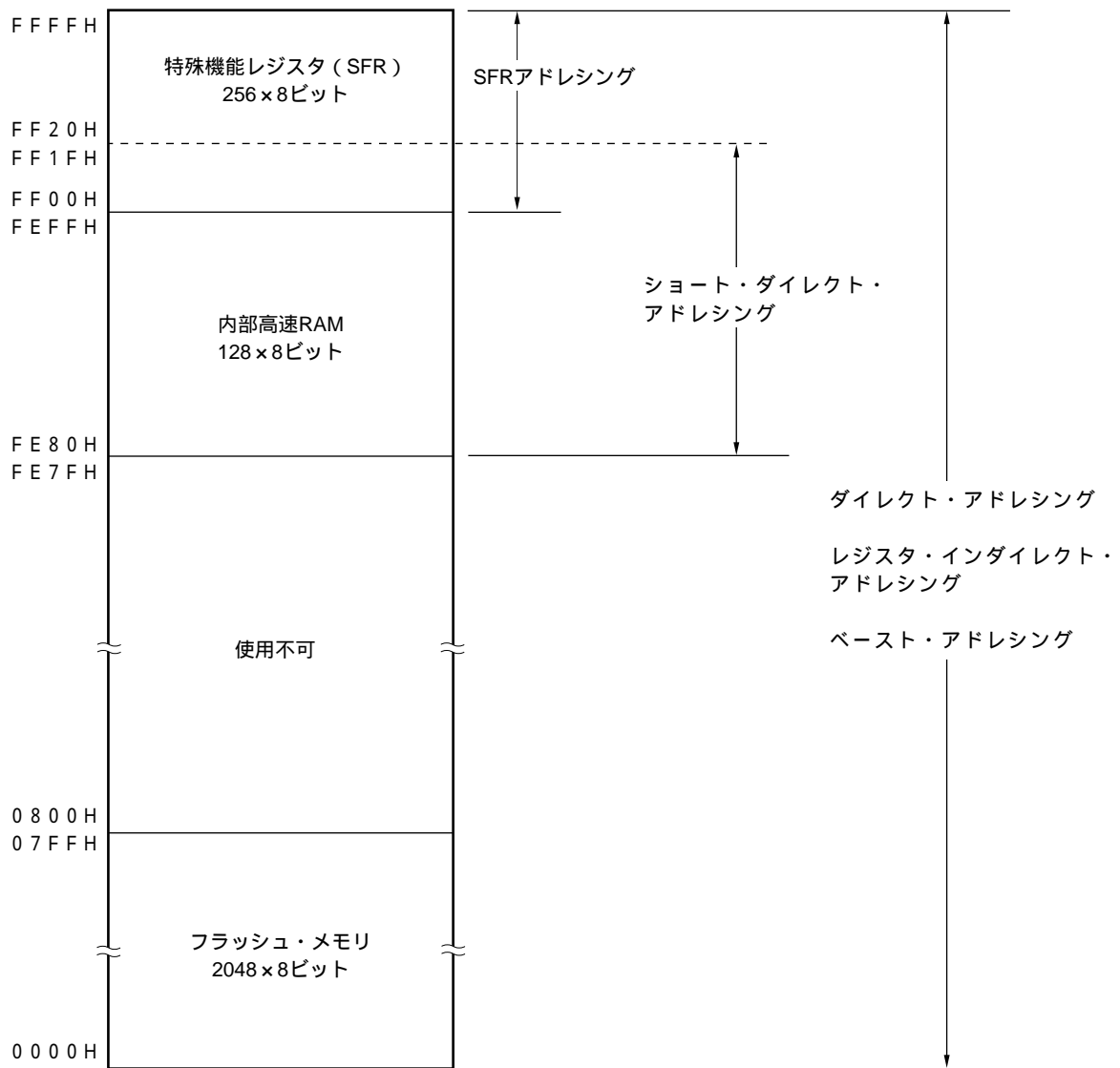
図3-5 データ・メモリのアドレッシング ( \mu PD78F9511)
