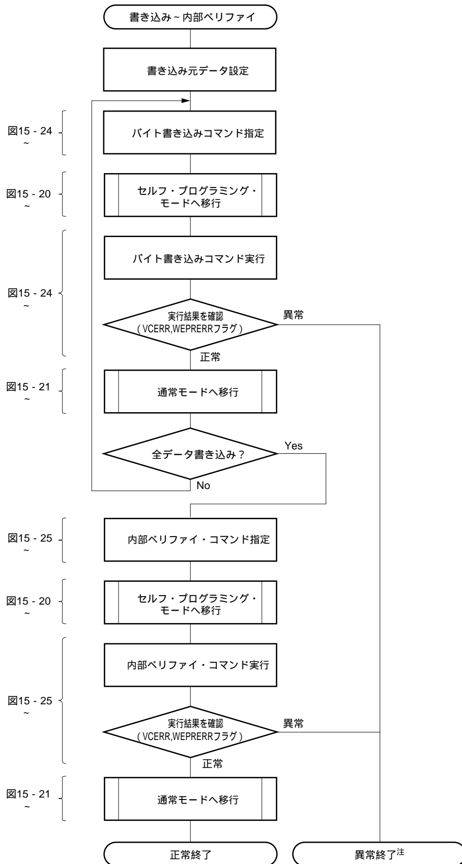
図15 - 30 割り込み禁止時間を最小にしたい場合の動作例（書き込み～内部ベリファイ）
