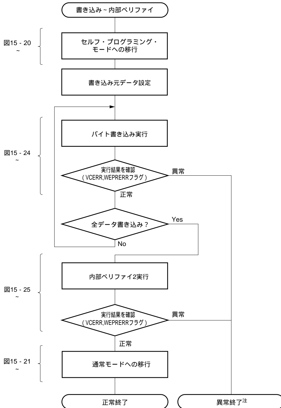
図15 - 28 コマンド実行時間を最小にしたい場合の動作例 (書き込み～内部ペリファイ)
