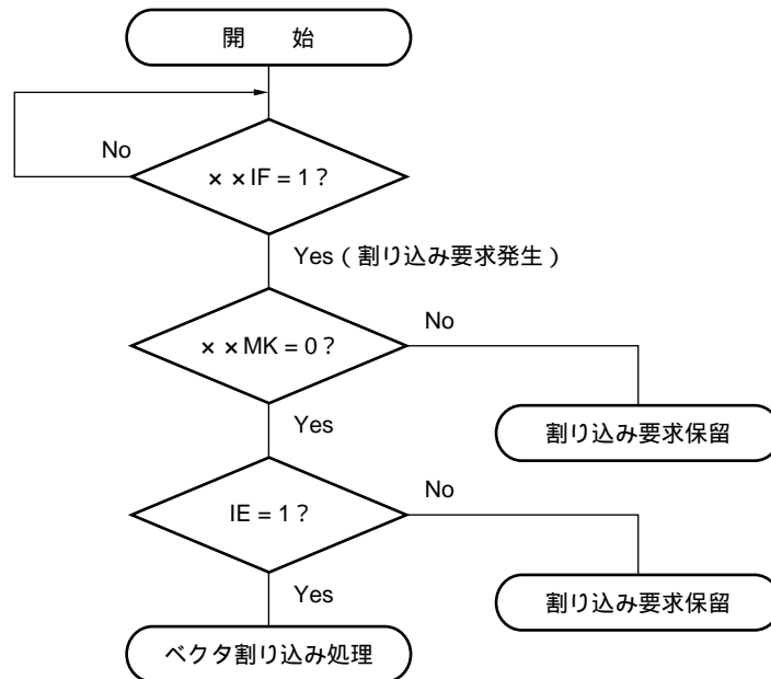
図9 - 6 割り込み要求受け付け処理アルゴリズム
