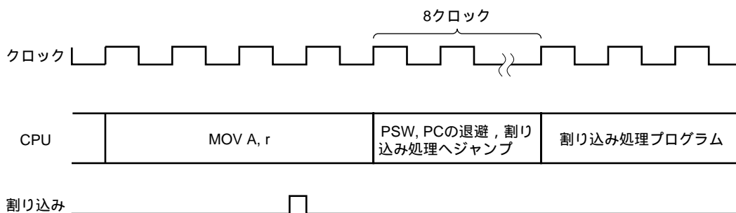
図9 - 7 割り込み要求の受け付けタイミング (MOV A, rの例)
