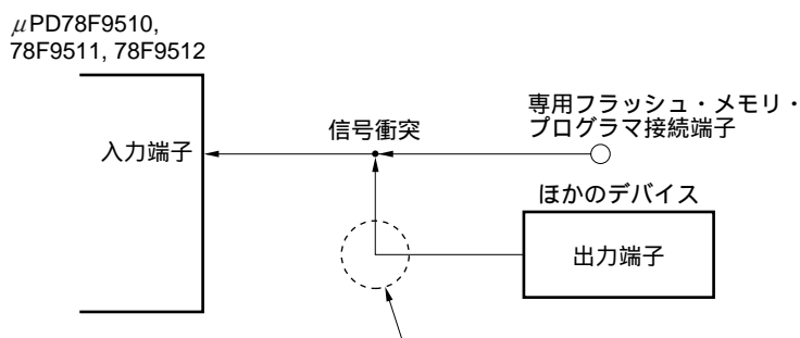
図15 - 8 信号の衝突 (RESET端子)
