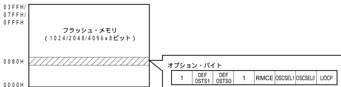
図14 - 1 オプション・バイトの位置
