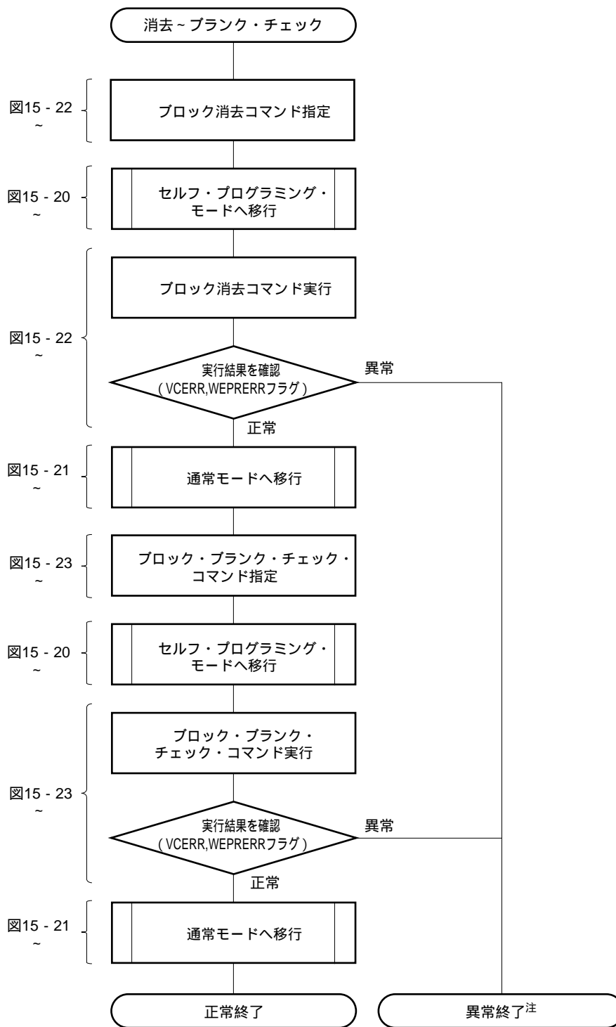
図15 - 29 割り込み禁止時間を最小にしたい場合の動作例（消去～ブランク・チェック）
