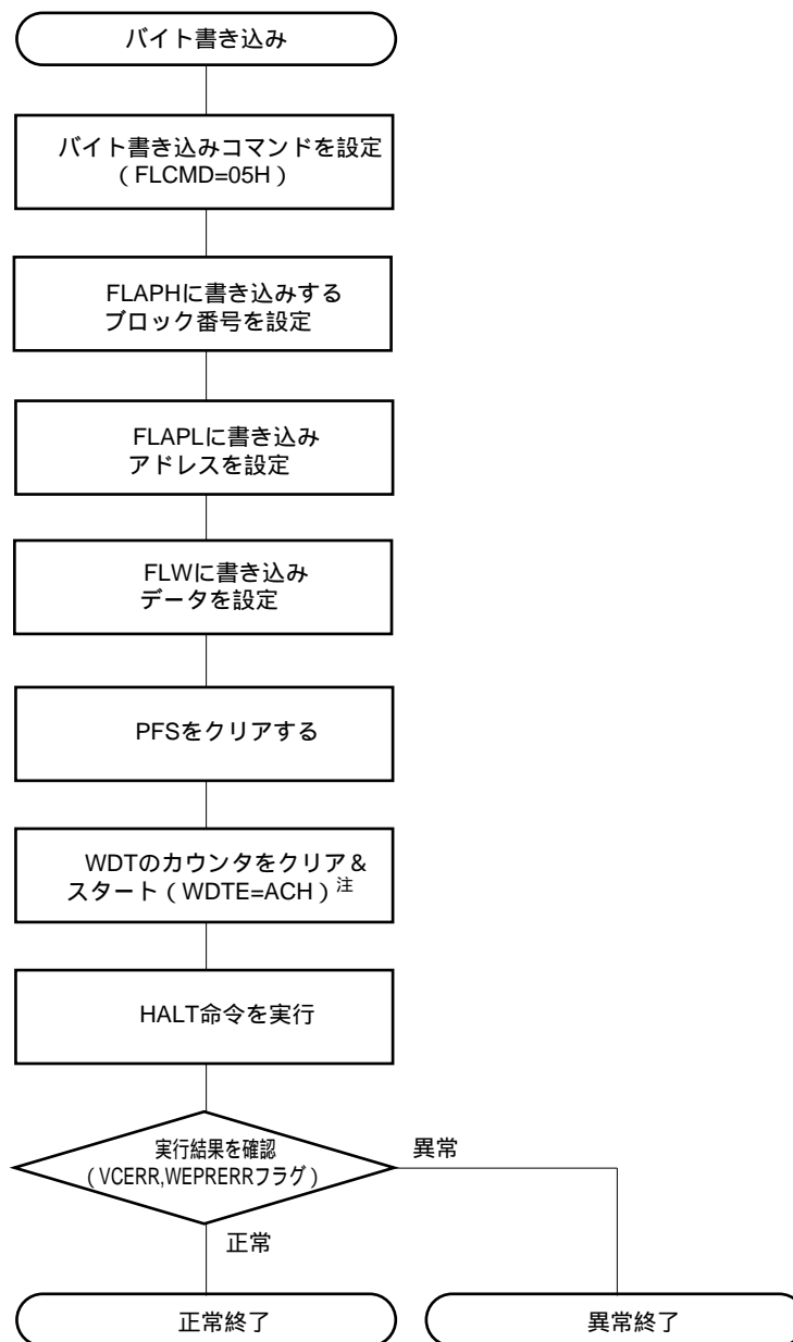
図15 - 24 セルフ・プログラミング・モードのバイト書き込み動作例
