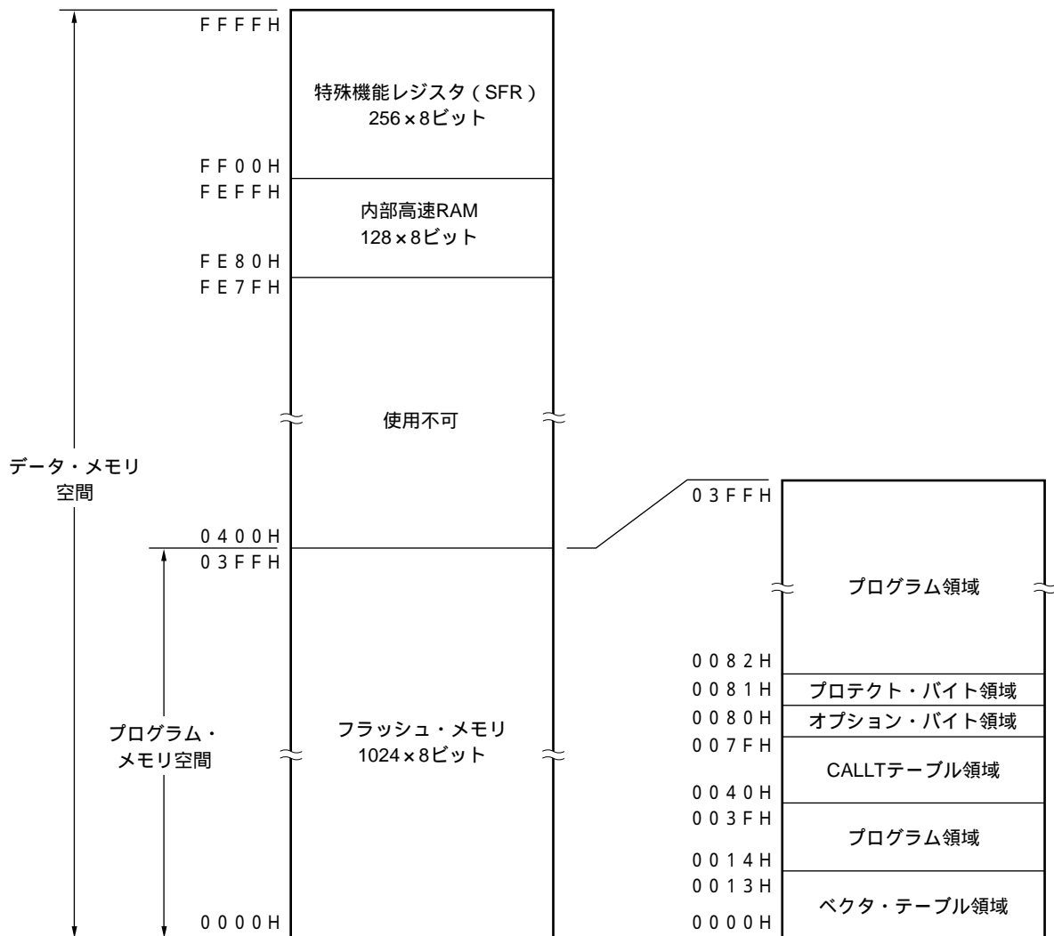
図3 - 1 メモリ・マップ (μPD78F9510)
