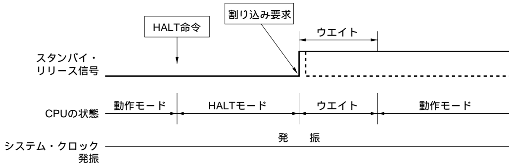
図10 - 2 HALTモードの割り込み要求発生による解除
