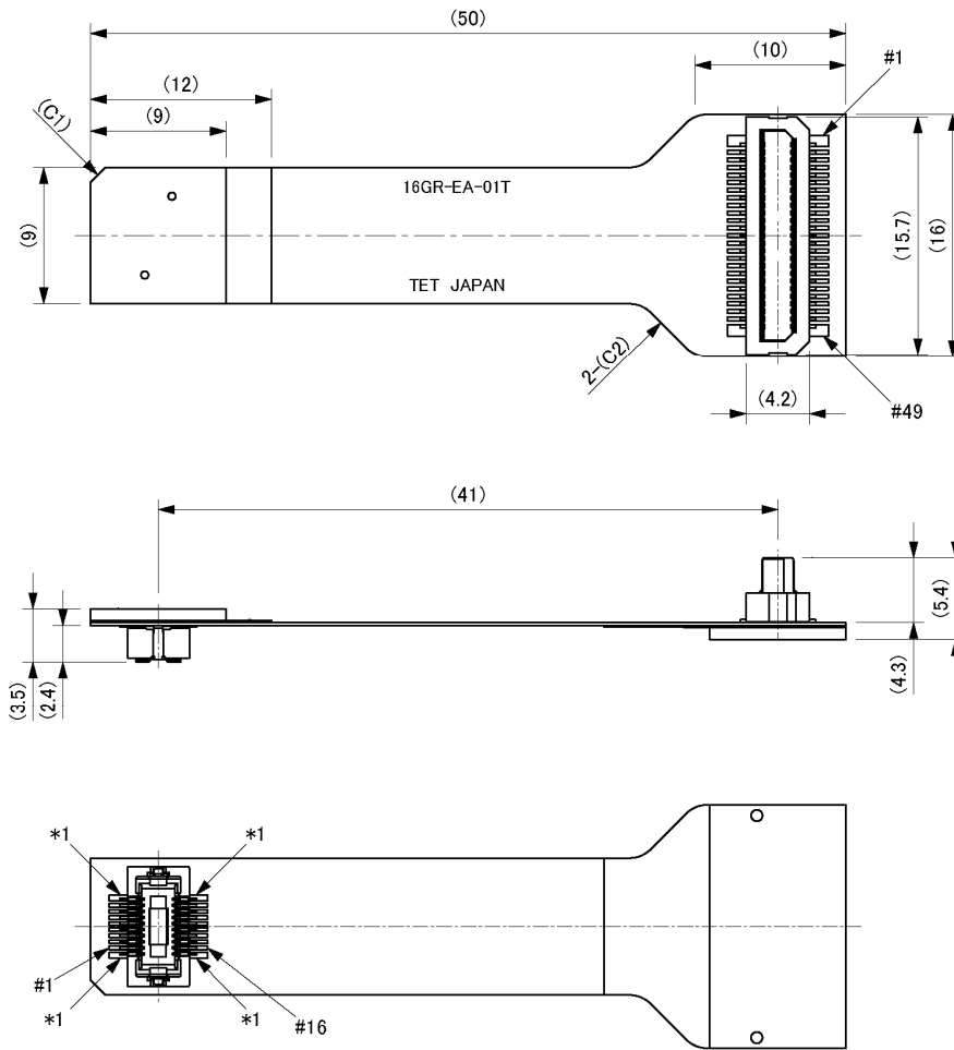
図B-2 エクステンション・アダプタ (QB-16GR-EA-01T)
