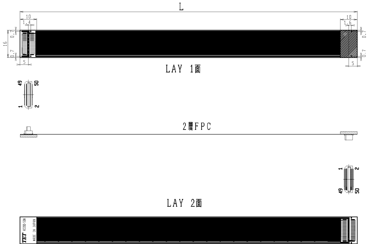
図B-3 エミュレーション・プローブ(QB-50-EP-01T)
