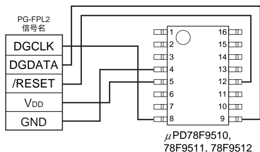
図15 - 5 PG-FPL2との配線図
