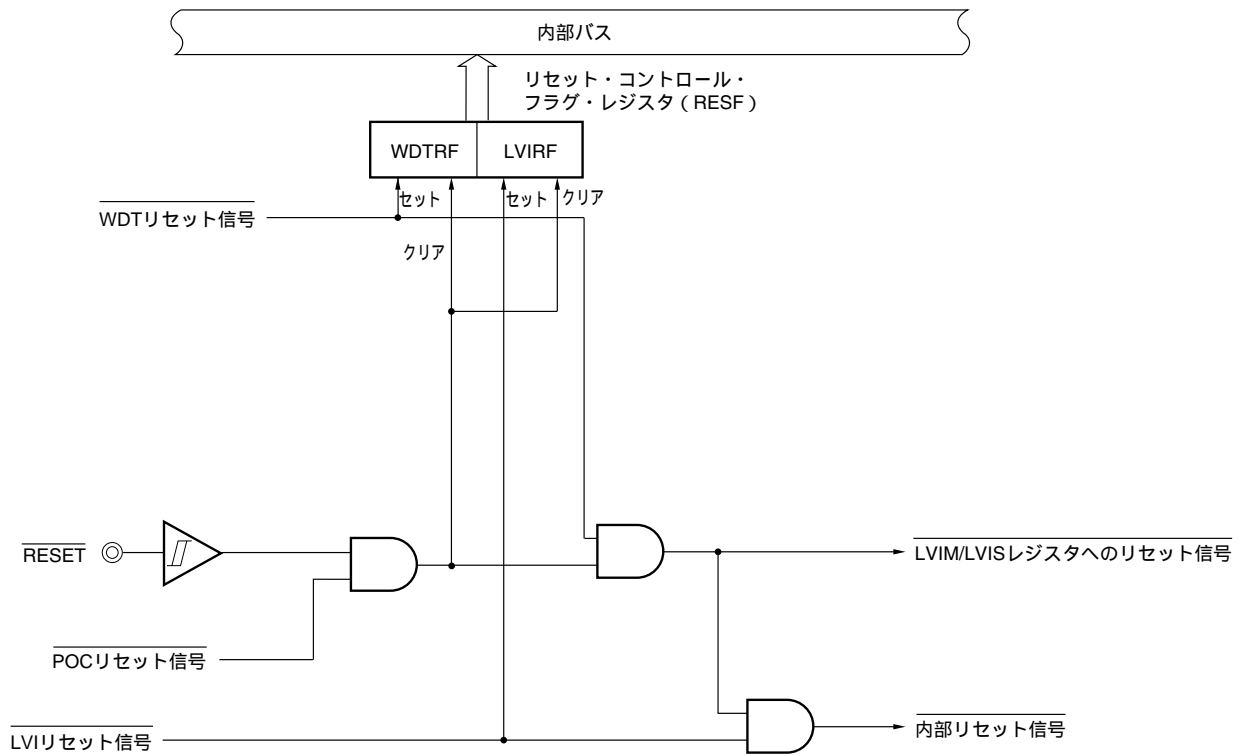
図11-1 リセット機能のブロック図
