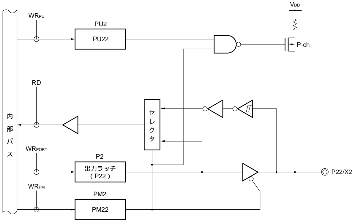
図4 - 3 P22のブロック図
