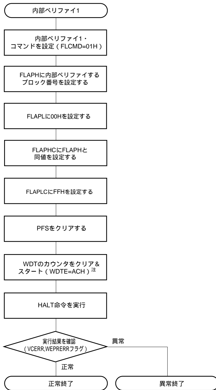
図15 - 25 セルフ・プログラミング・モードの内部ベリファイ1動作例
