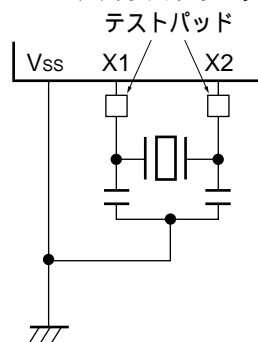
図15-6 テストパッドの実装例
