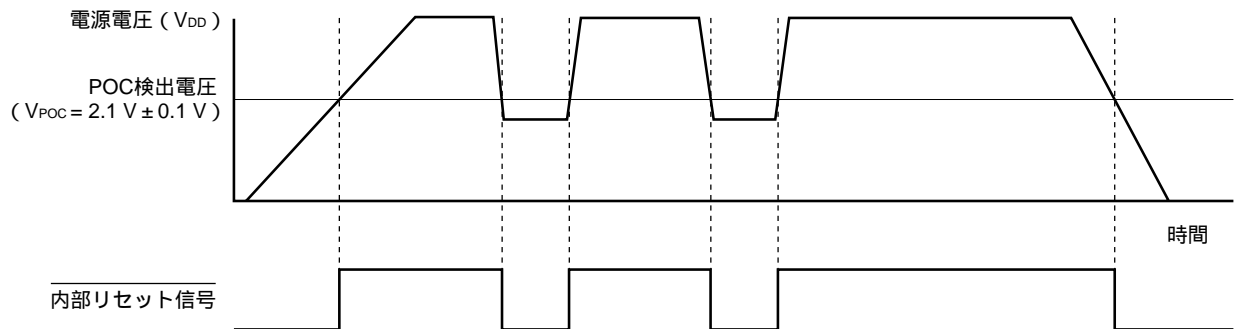
図12 - 2 パワーオン・クリア回路の内部リセット信号発生のタイミング
