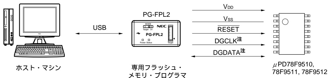
図15-3 フラッシュ・メモリにプログラムを書き込むための環境 (PG-FPL2)
