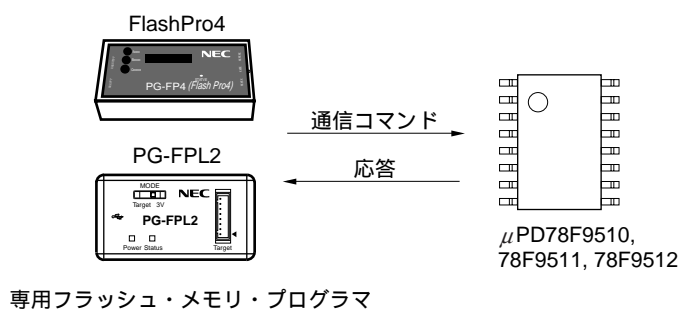
図15-9 通信コマンド
