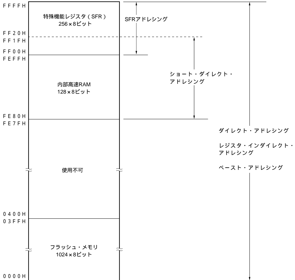
図3 - 4 データ・メモリのアドレッシング (μ PD78F9510)
