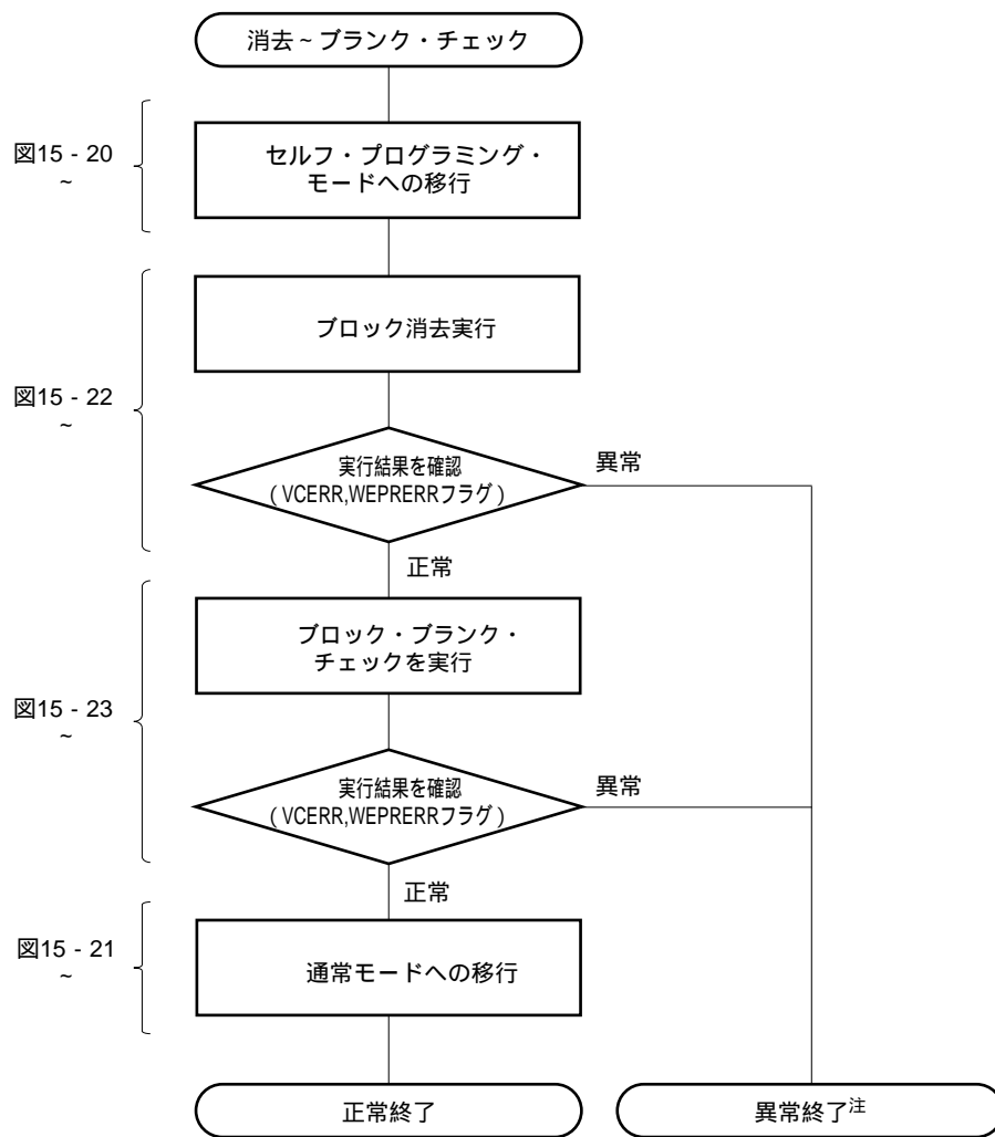
図15 - 27 コマンド実行時間を最小にしたい場合の動作例 (消去～ブランク・チェック)
