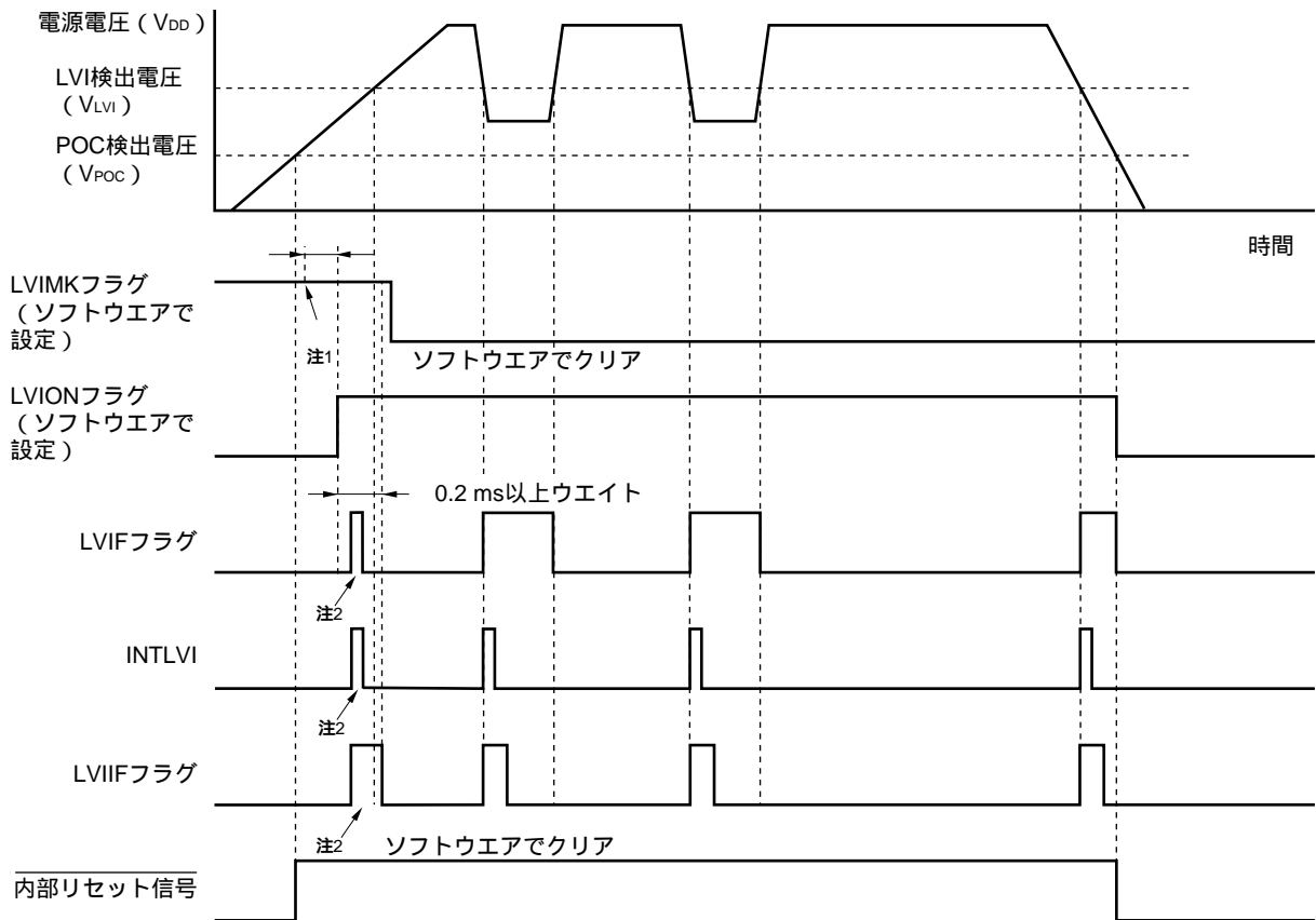
図13 - 5 低電圧検出回路の割り込み信号発生時のタイミング
