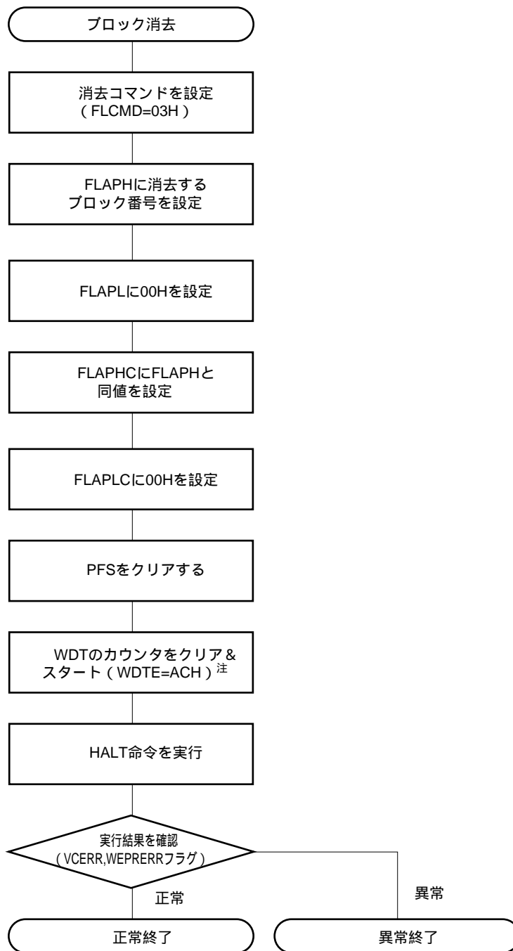
図15 - 22 セルフ・プログラミング・モードのブロック消去動作例
