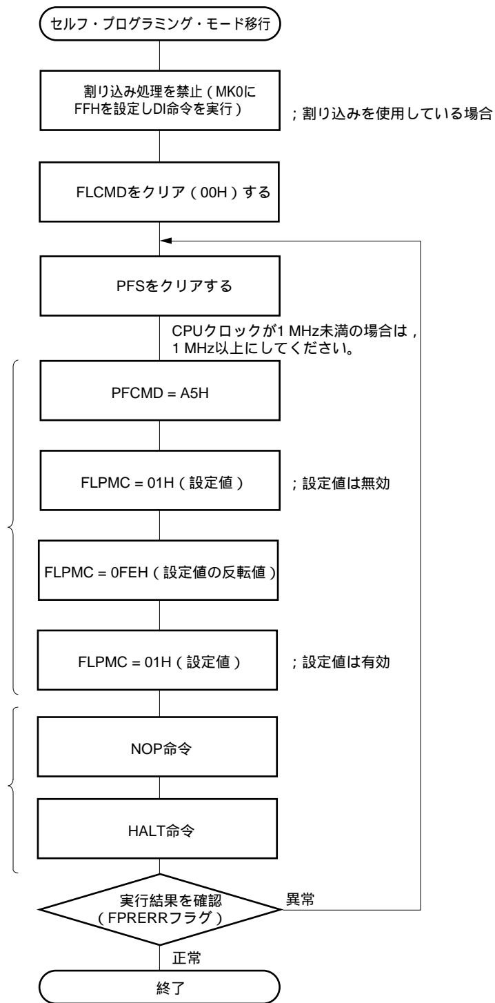
図15 - 20 セルフ・プログラミング・モードへの移行例
