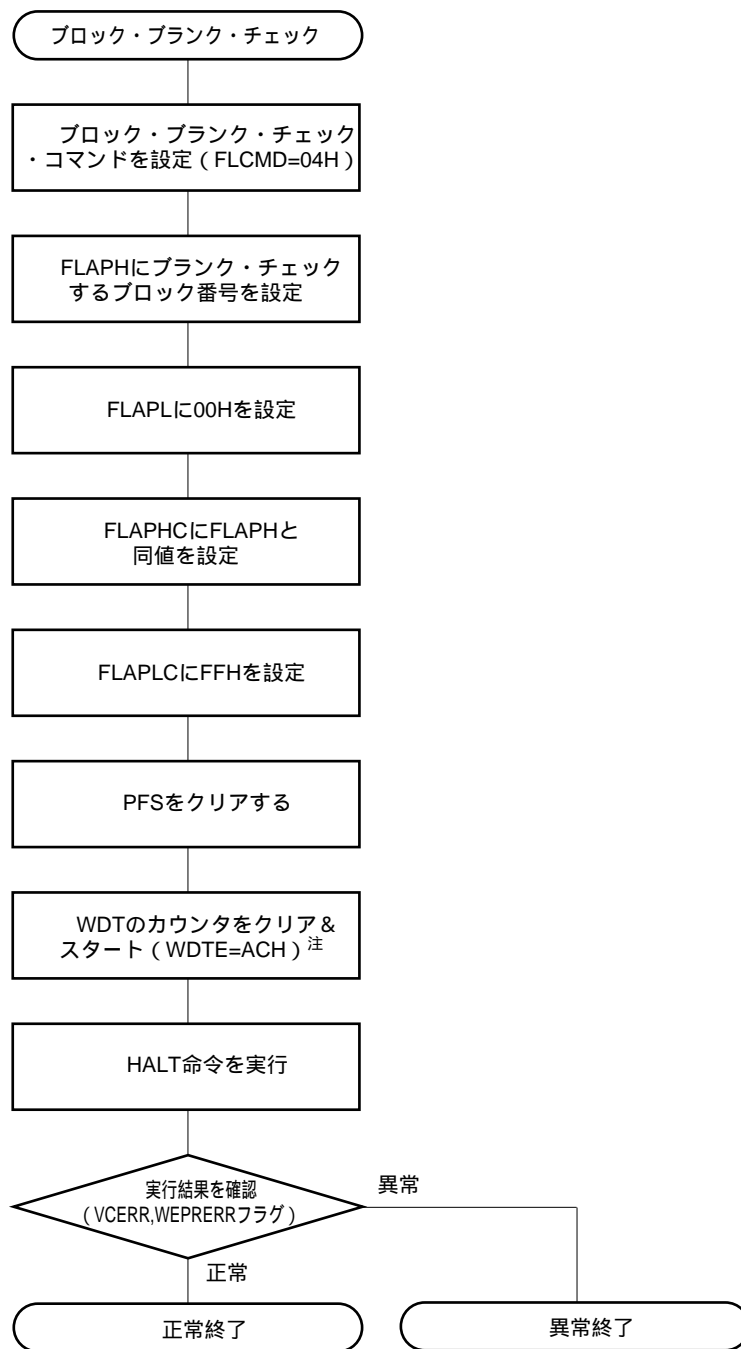
図15 - 23 セルフ・プログラミング・モードのブロック・ブランク・チェック動作例
