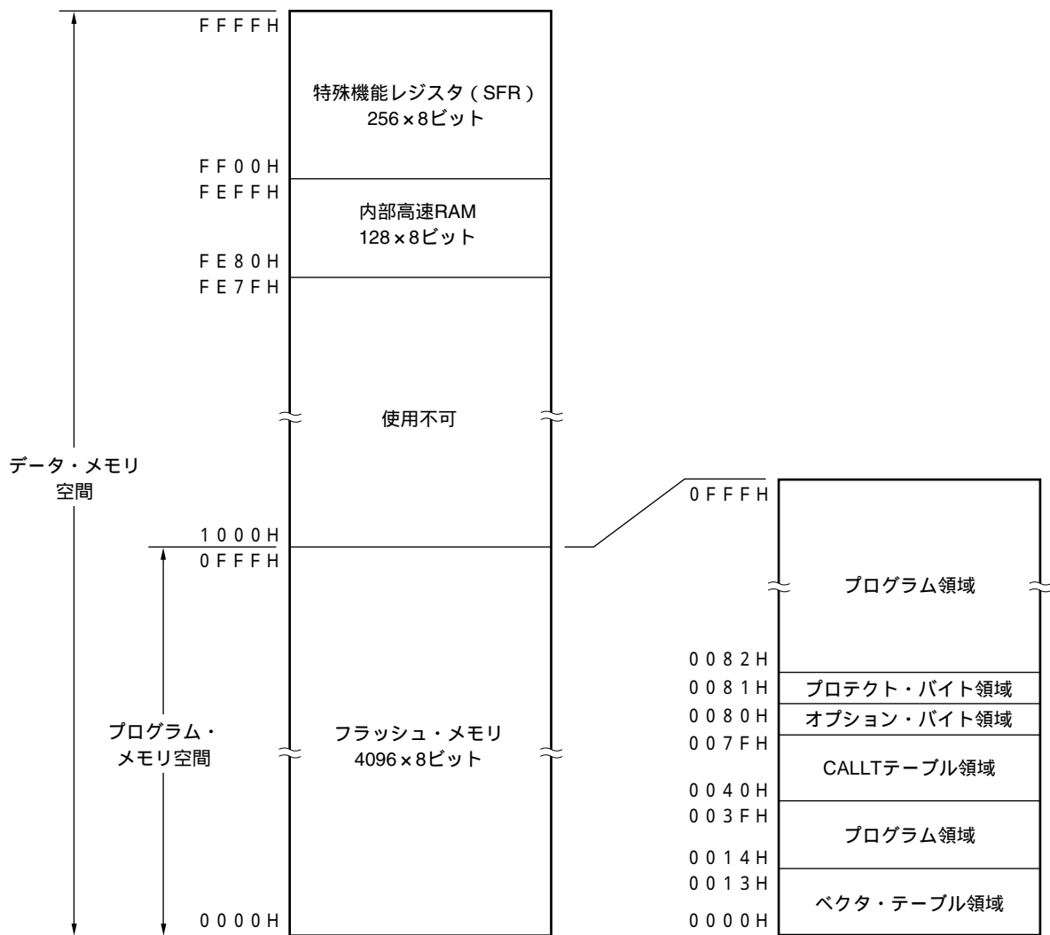
図3-3 メモリ・マップ (μ PD78F9512)
