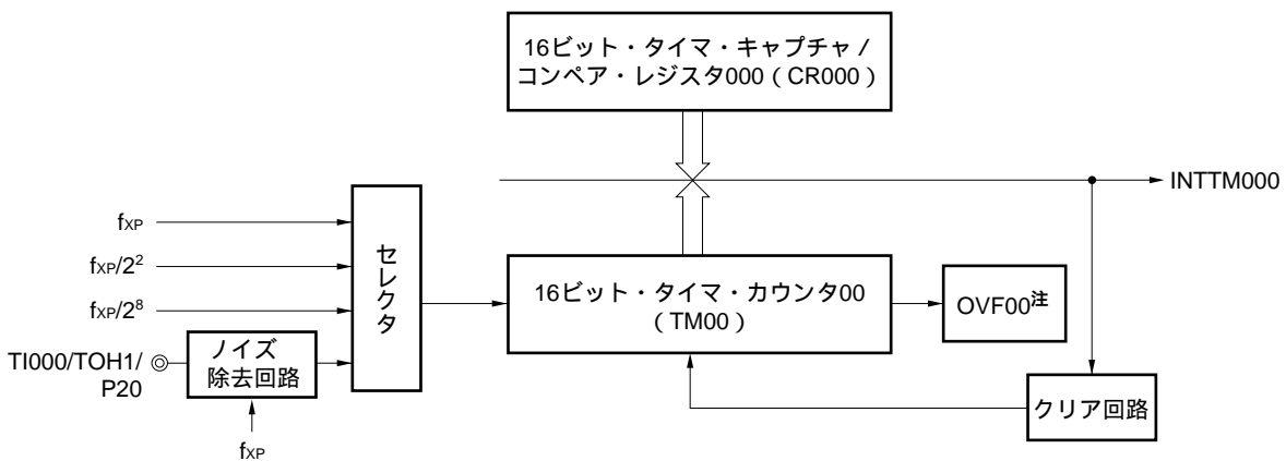
図6 - 11 インターバル・タイマの構成図
