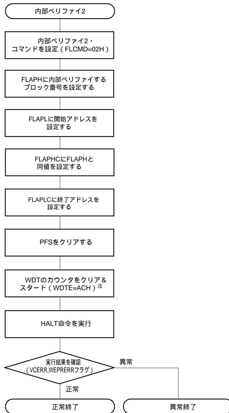
図15 - 26 セルフ・プログラミング・モードの内部ベリファイ2動作例
