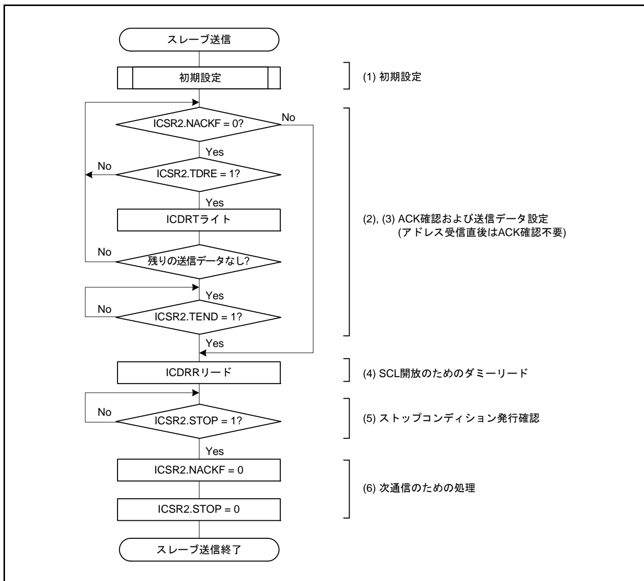
図 42.14 スレーブ送信のフローチャート例
