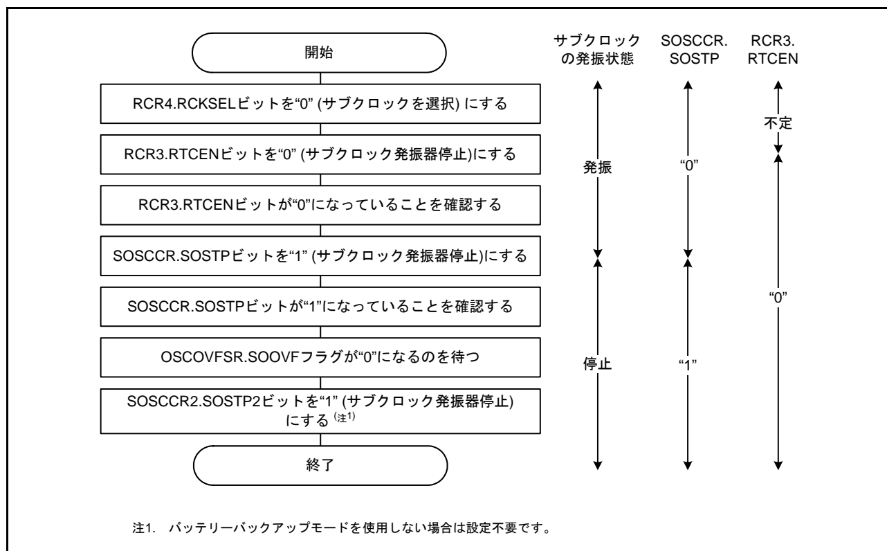
図 9.13 サブクロックを使用しない場合のフローチャート例
