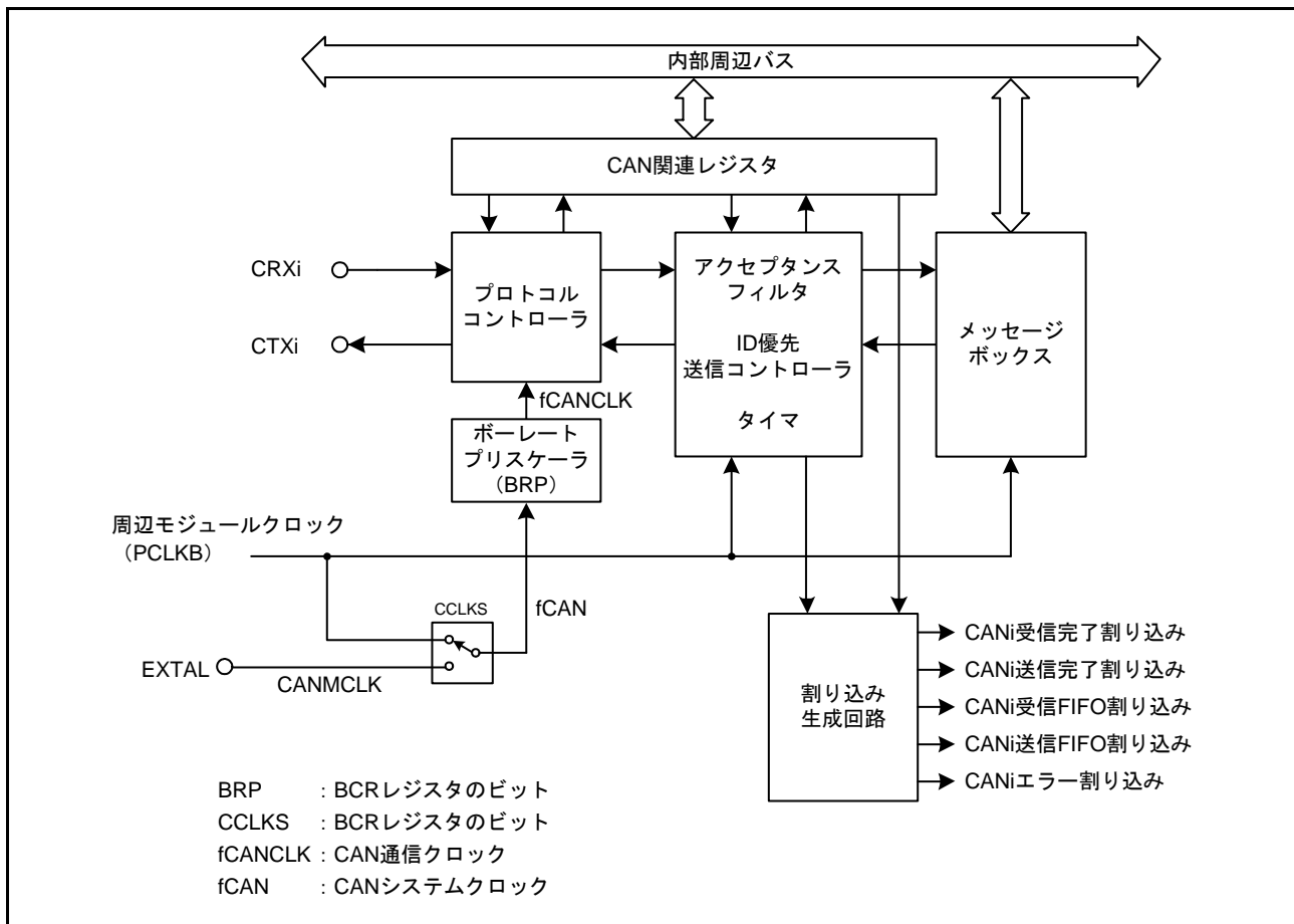
図 43.1 CAN モジュールブロック図 (i = 0 ~ 2)
