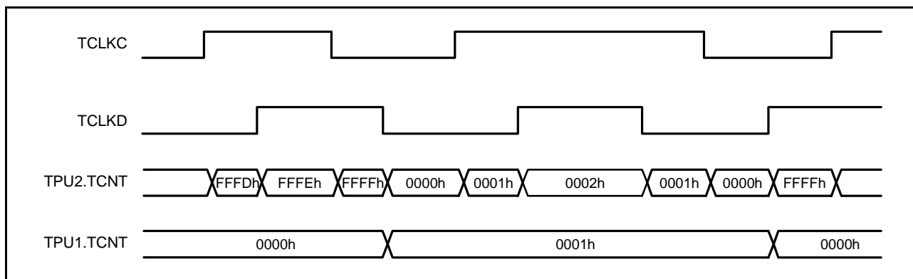
図 27.19 カスケード接続動作例 (2)
