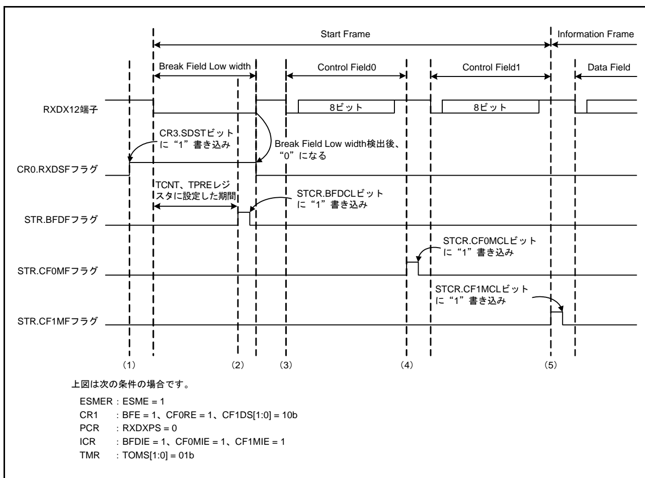
図 40.64 Start Frame 受信時の動作例
