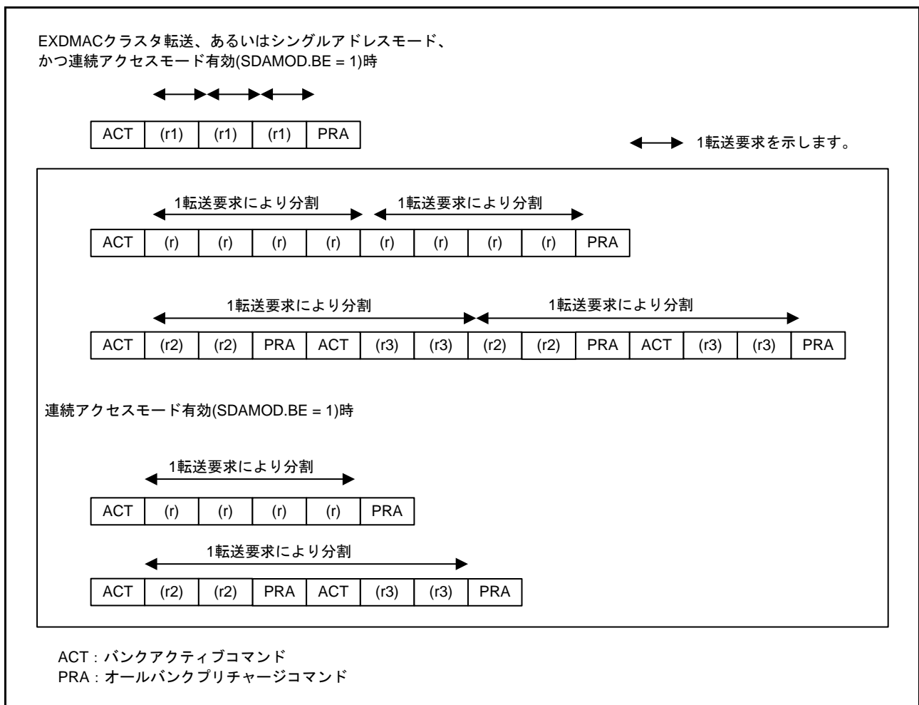
図 16.18 連続アクセスの動作例
