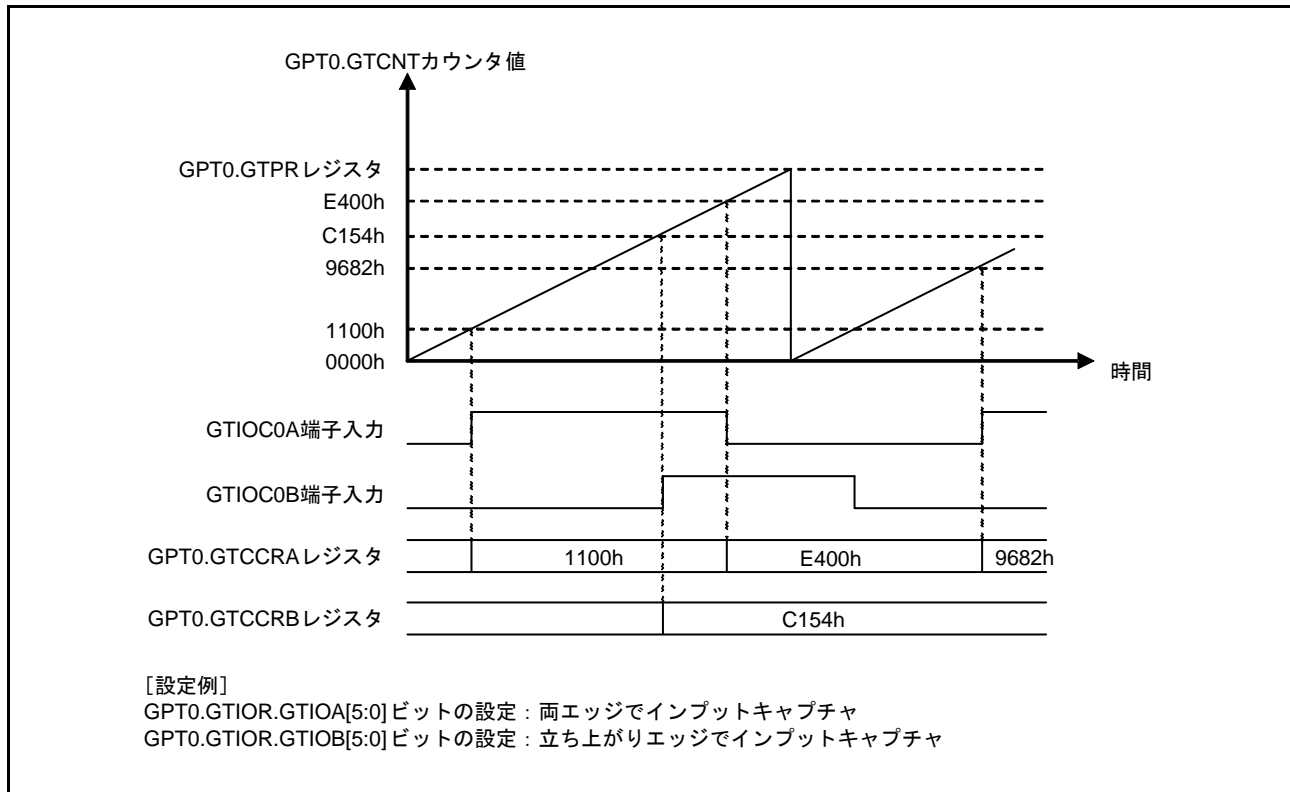
図 26.11 インพุットキャプチャ動作例
