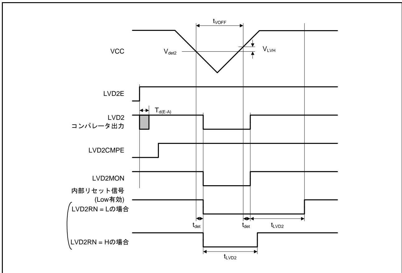
図 64.93 電圧検出回路タイミング ( V_{det2} )
