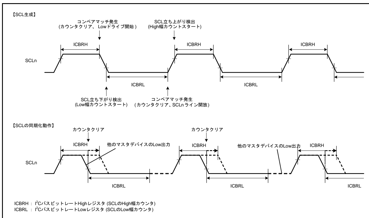
図 42.20 RIIC の SCL 生成および SCL 同期化動作
