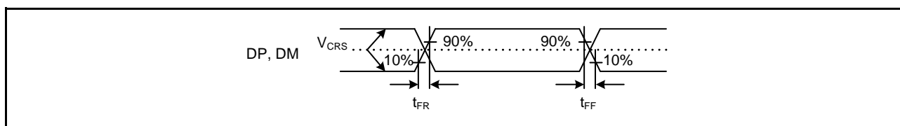
図 64.88 DP、DM 出カタイミング (フルスピード時)
