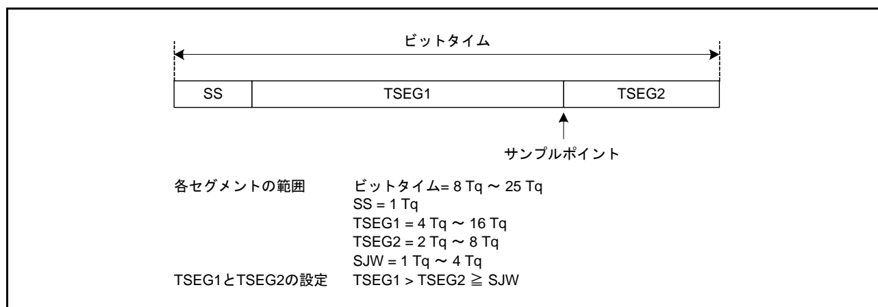
図 43.12 ビットタイミング図
