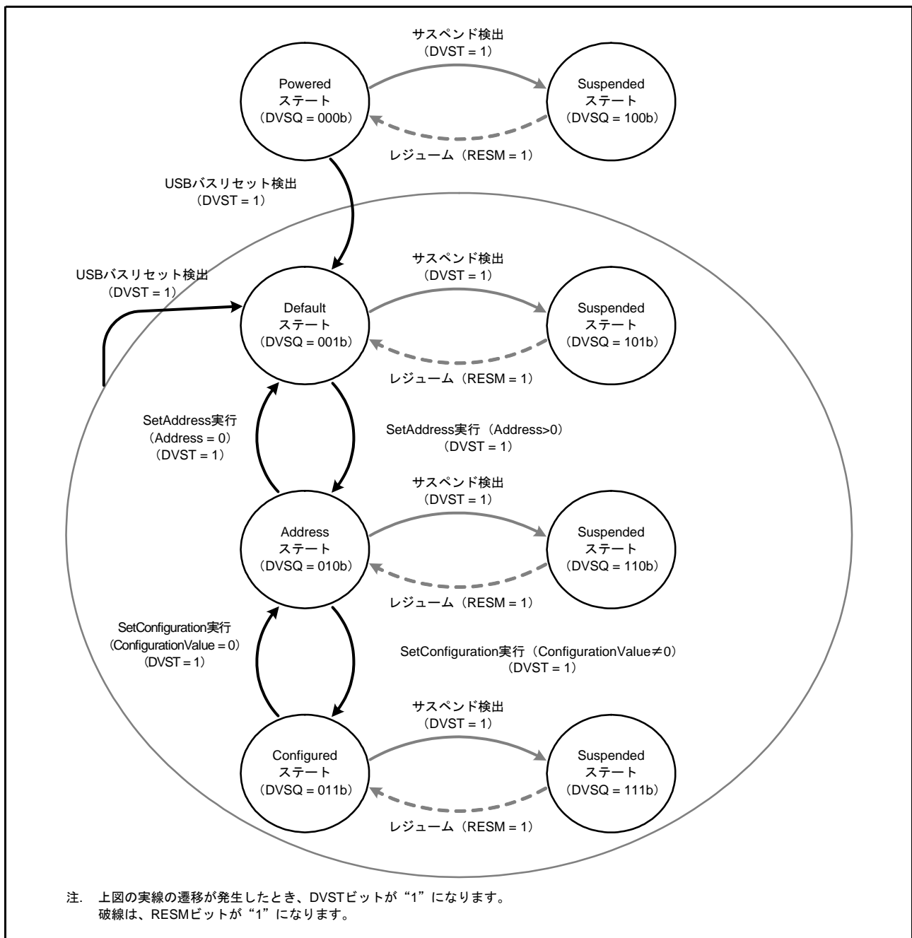
図 38.14 デバイスステート遷移図
