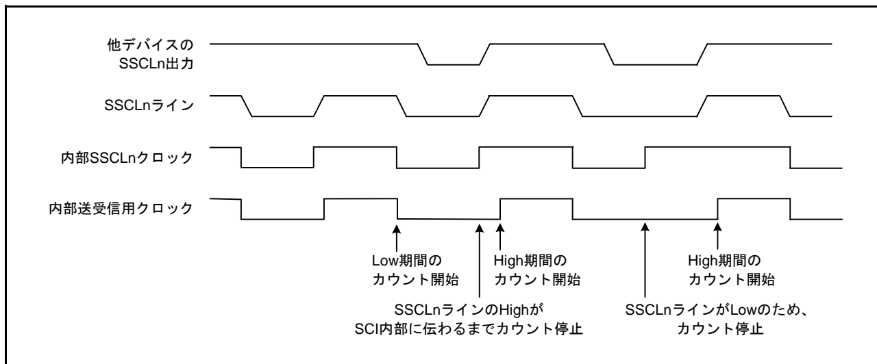
図 40.49 クロック同期化の動作例
