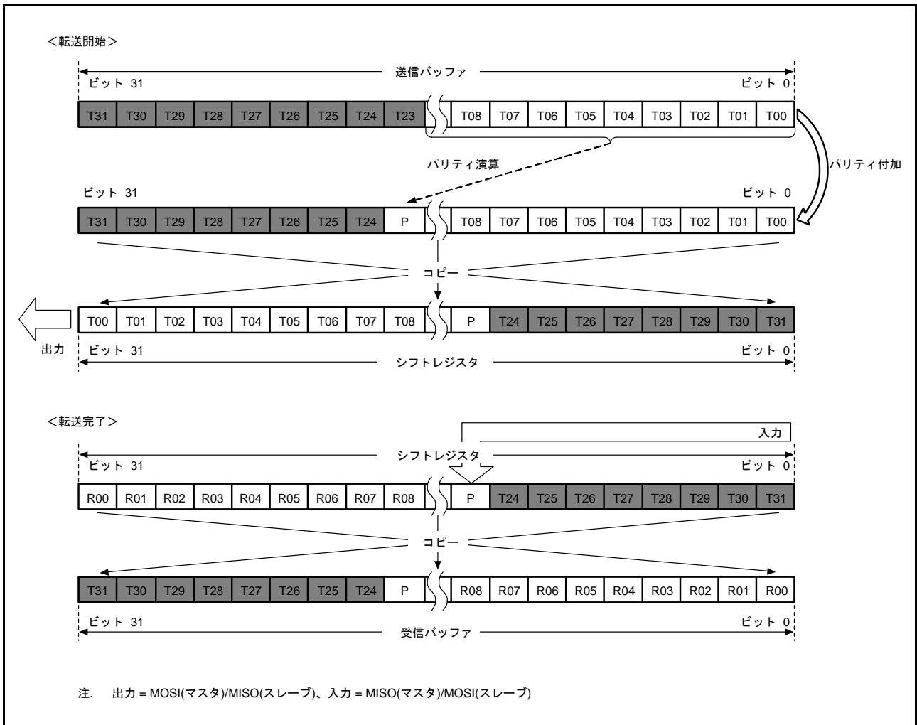
図 44.21 LSB ファースト (24 ビットデータ / パリティ機能有効)
