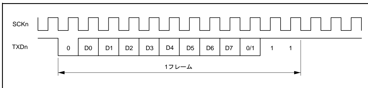
図 40.7 出カクロックと送信データの位相関係 (調歩同期式モード: SMR.CHR = 0、PE = 1、MP = 0、STOP = 1)
