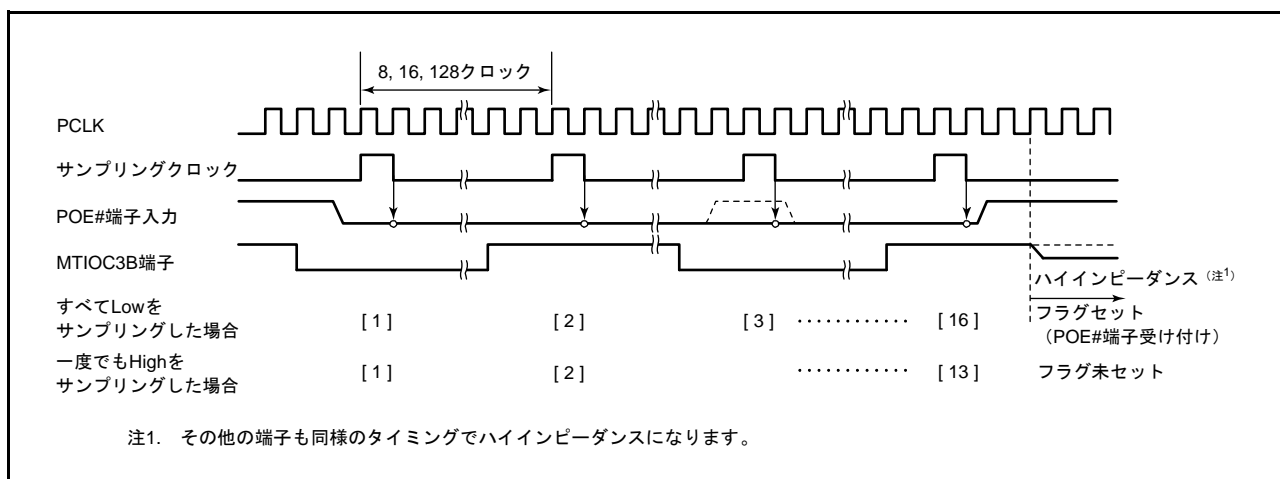
図 25.4 Low 検出を選択した場合の動作
