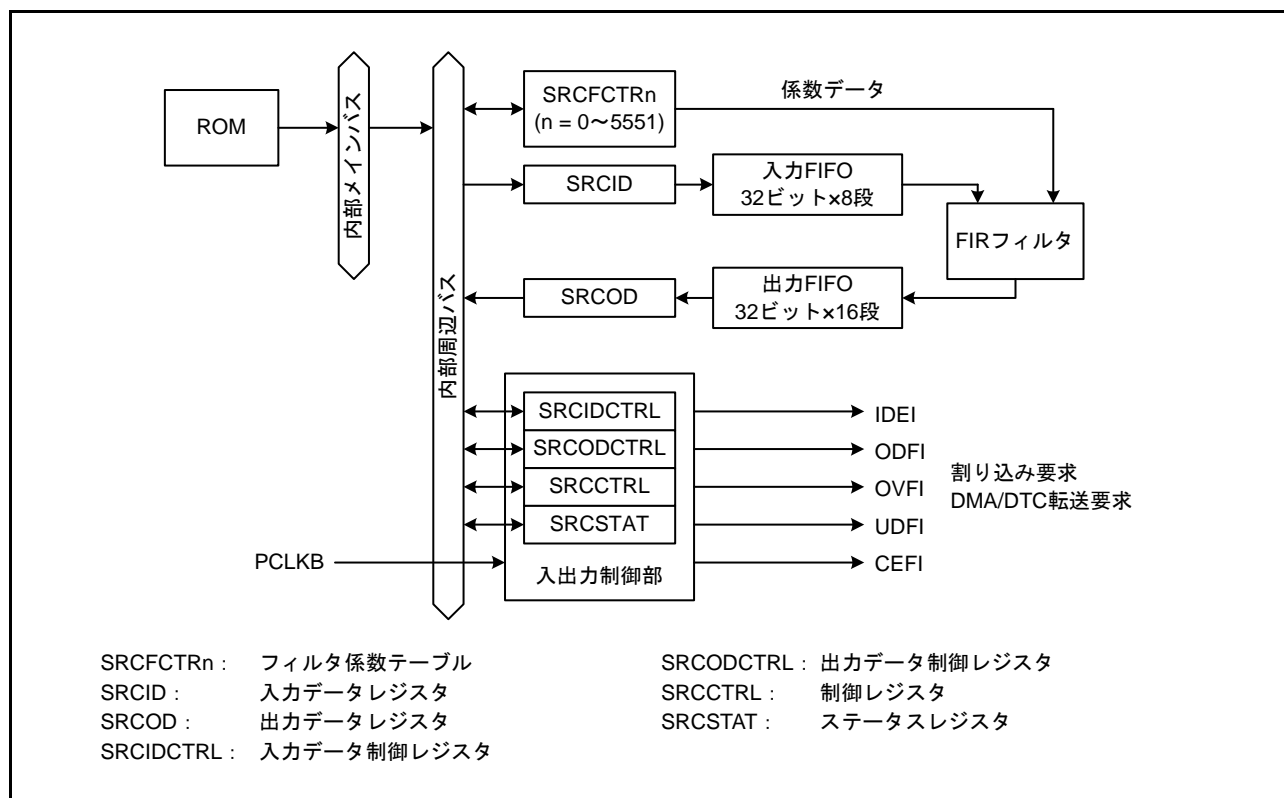
図 48.1 サンプリングレートコンバータのブロック図
