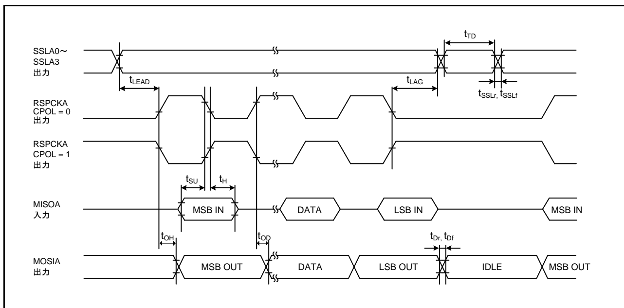
図 64.59 RSPCKA タイミング (マスタ、CPHA = 1) (ビットレート : PCLKB を 2 分周以外に設定)
