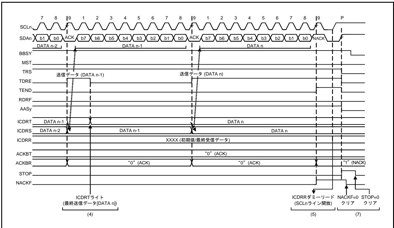
図 42.16 スレーブ送信の動作タイミング (2)
