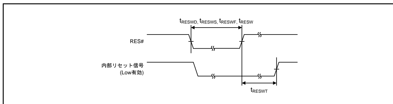
図 64.2 リセット入力タイミング
