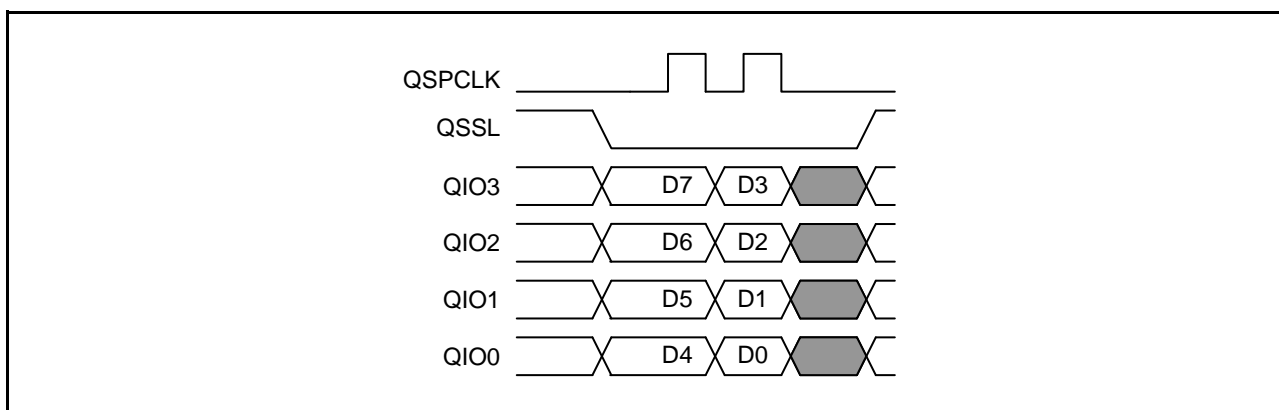
図 45.5 Quad-SPI モード転送フォーマット
