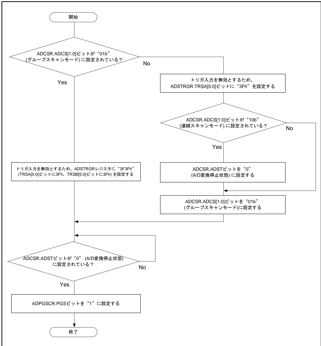
図 57.26 ADPGSCR.PGS ビット設定時のフロー
