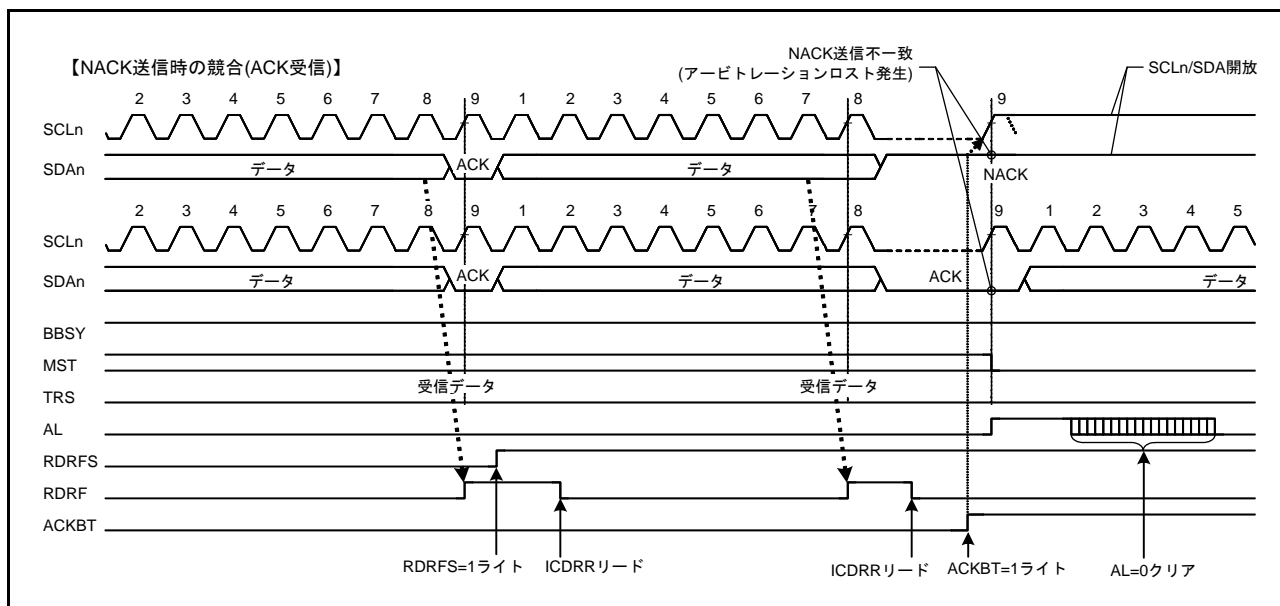
図 42.34 NACK 送信アービトレーションロス検出動作例 (NALE ビット = 1 のとき)
