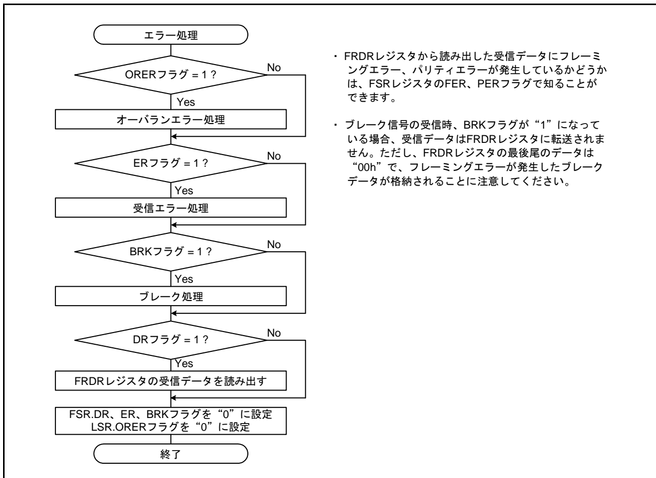
図 41.11 シリアル受信フローの例 (2)
