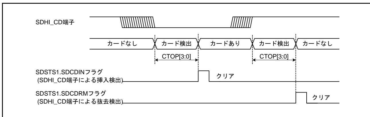
図 49.6 SDHI_CD 端子によるカード検出例
