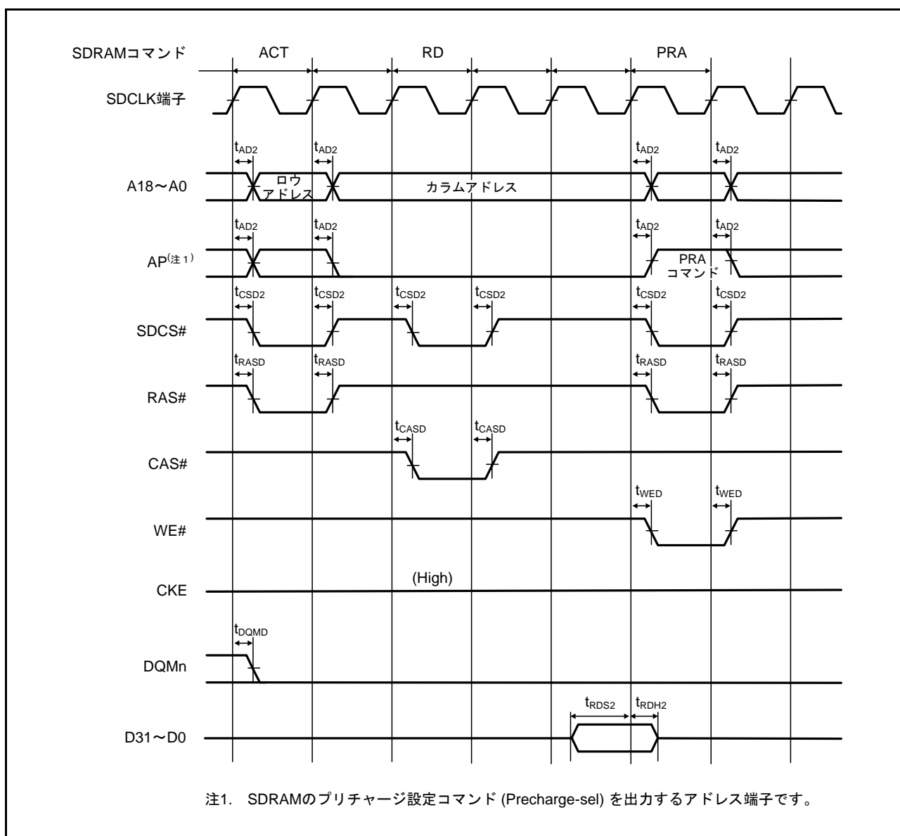
図 64.23 SDRAM 空間シングルリードバスタイミング
