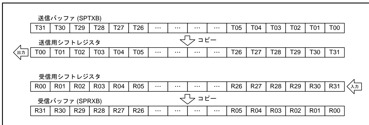
図 45.9 LSB ファースト転送 (32 ビットデータ)
