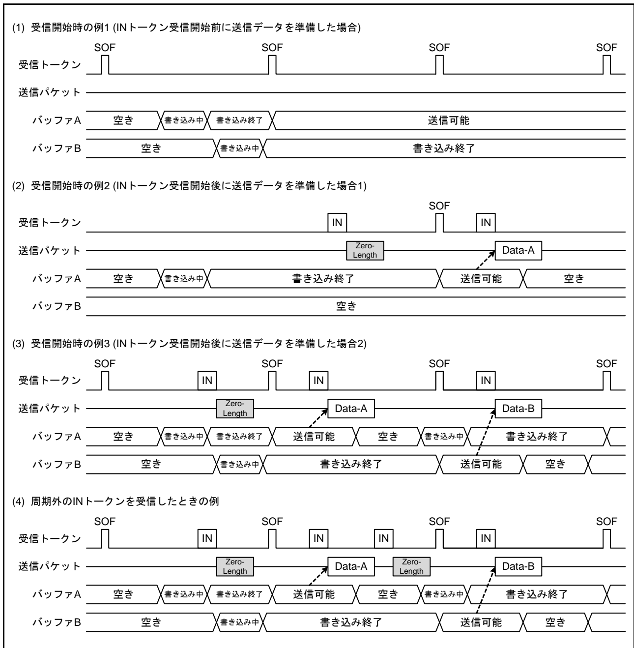
図 39.17 データセットアップ機能動作例
