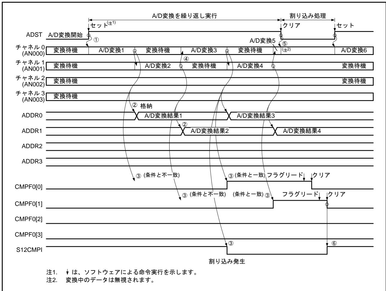
図 57.34 コンペア機能の動作例 (AN000, AN001, AN002, AN003 コンペア対象)
