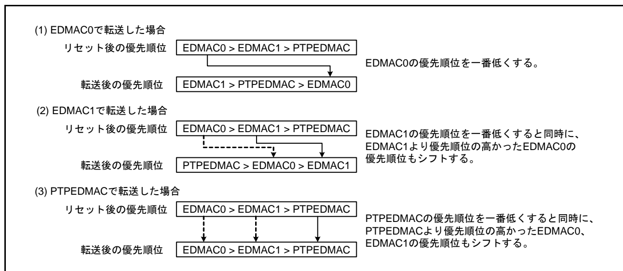
図 37.9 ラウンドロビン方式の動作
