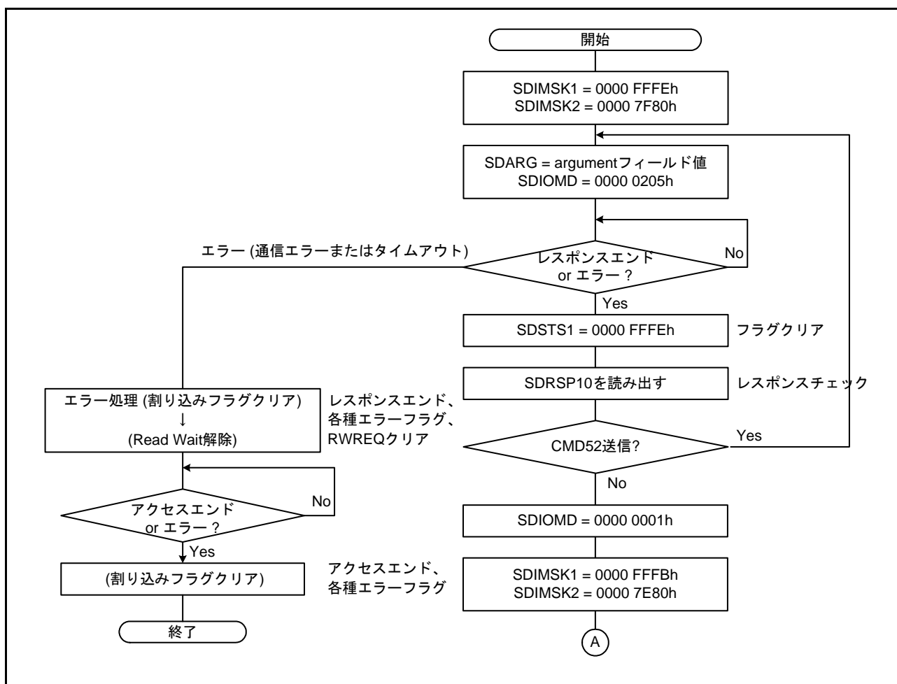
図 49.17 IO_RW_EXTENDED コマンド (CMD53/ マルチブロックリード) のシーケンス中に Read Wait 状態にした後、SDIO none abort コマンド (CMD52) を送信する例
