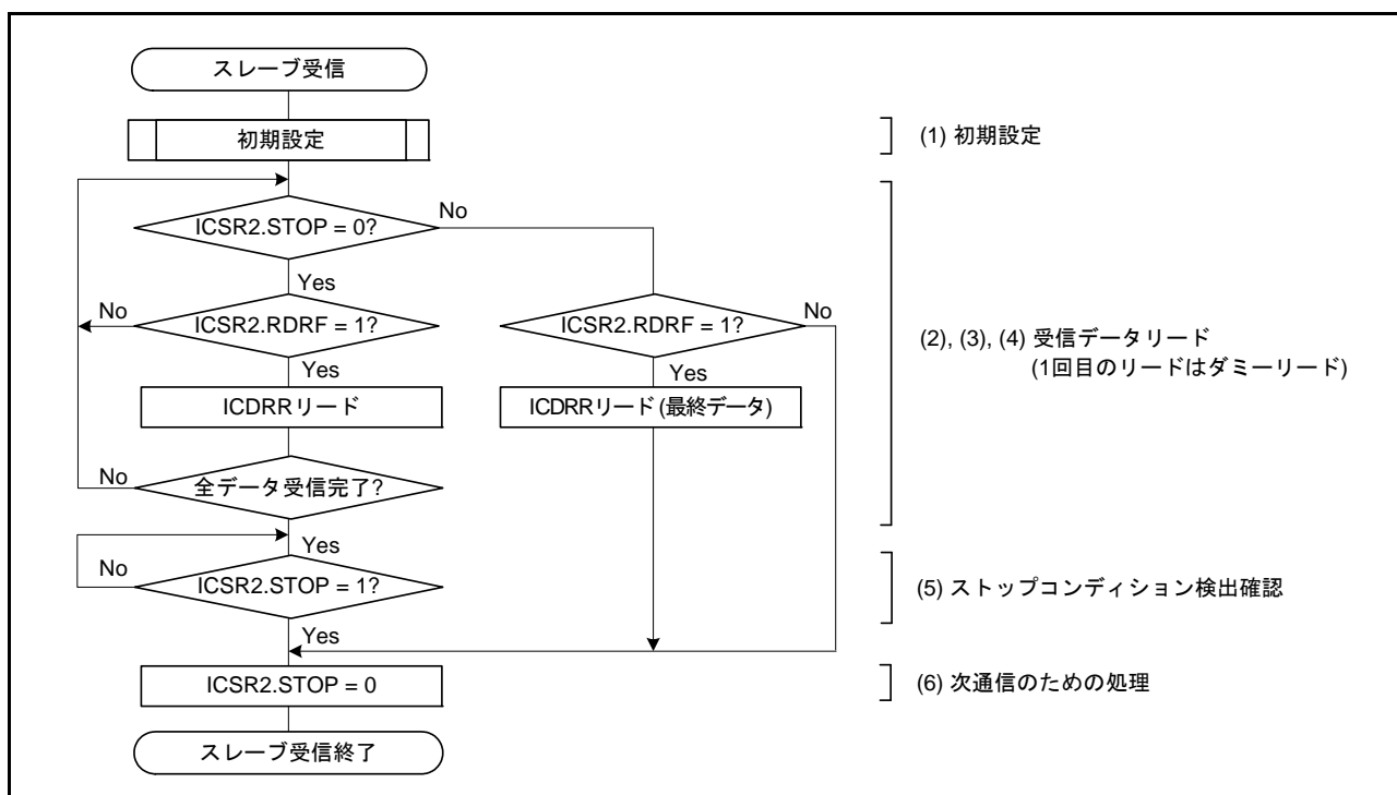
図 42.17 スレーブ受信のフローチャート例
