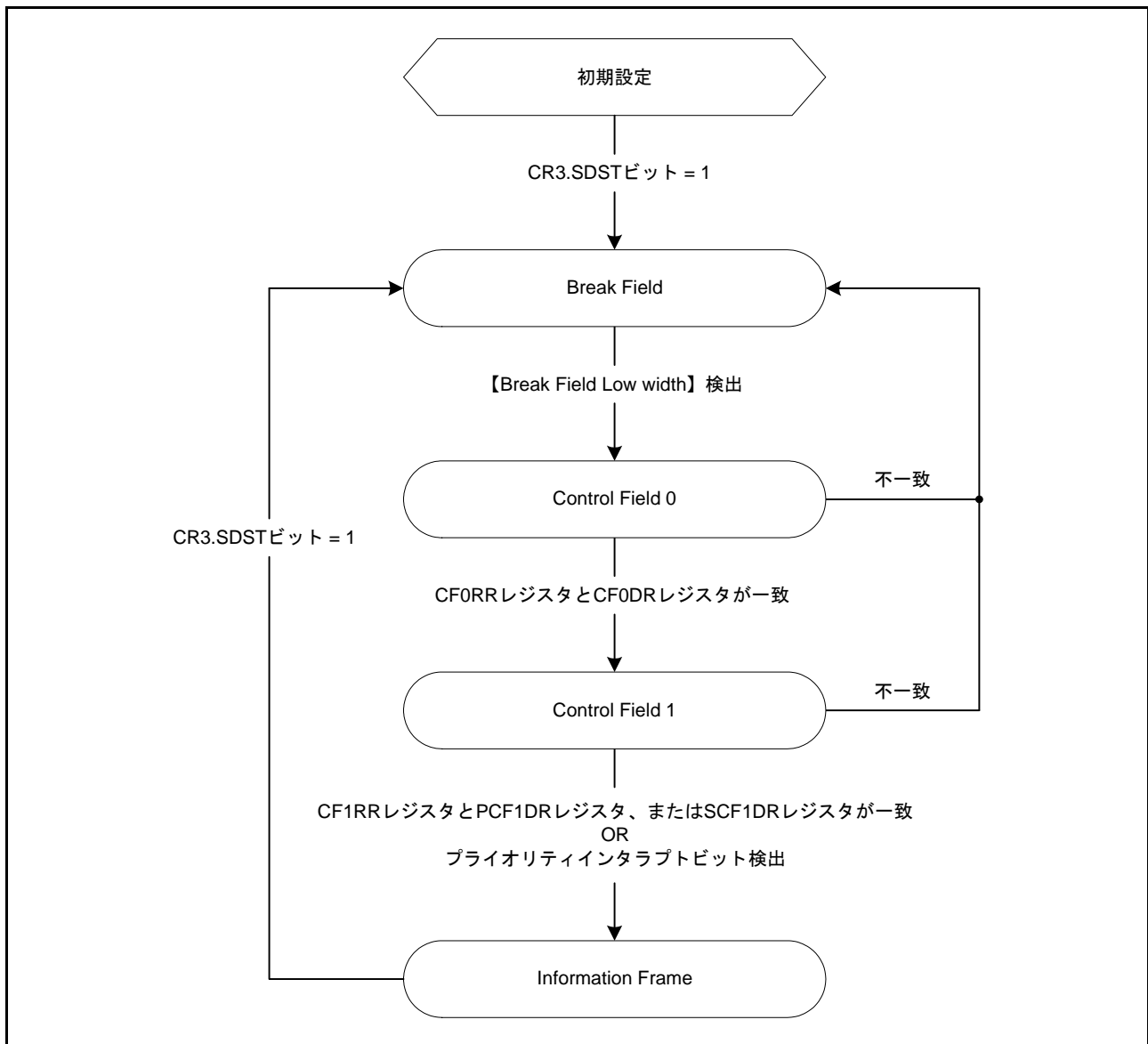
図 40.67 Start Frame 受信時の状態遷移図
