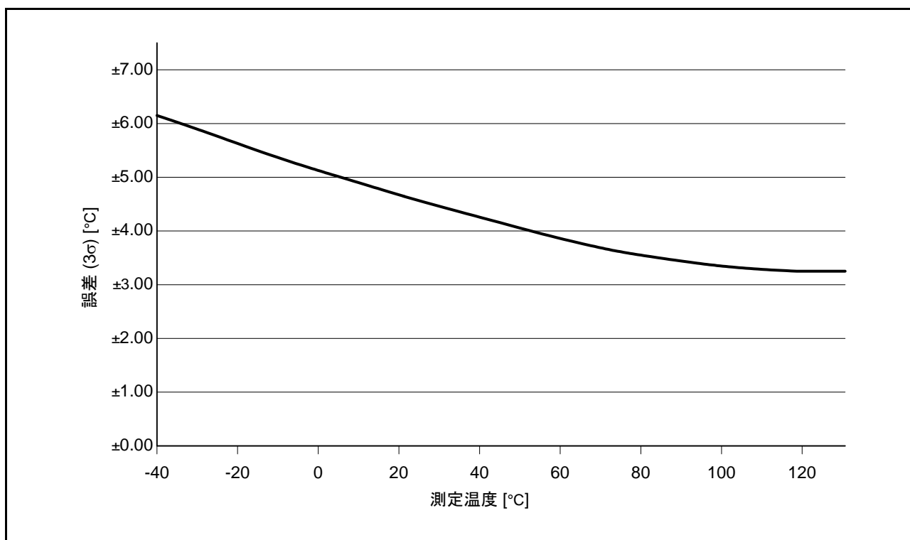
図 59.2 製品の測定温度誤差
