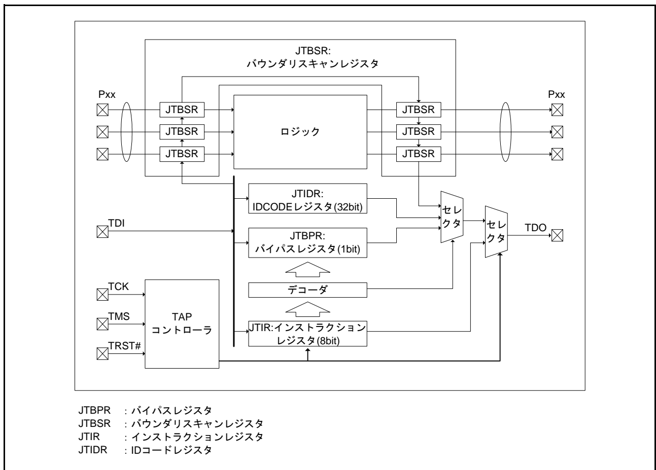
図 52.1 JTAG ブロック図
