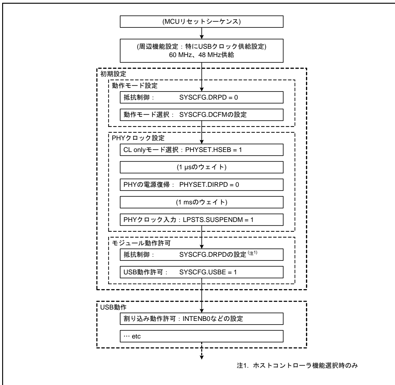
図 39.2 PHY クロック設定方法 (CL only モードの時)
