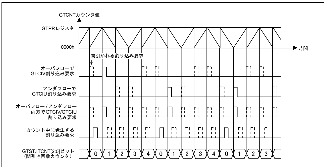
図 26.75 割り込み間引き機能の動作例 (のこぎり波でカウント方向を切替えながら動作、オーバーフロー/アンダフロー両方をカウントして間引き、間引き回数 4 の場合)
