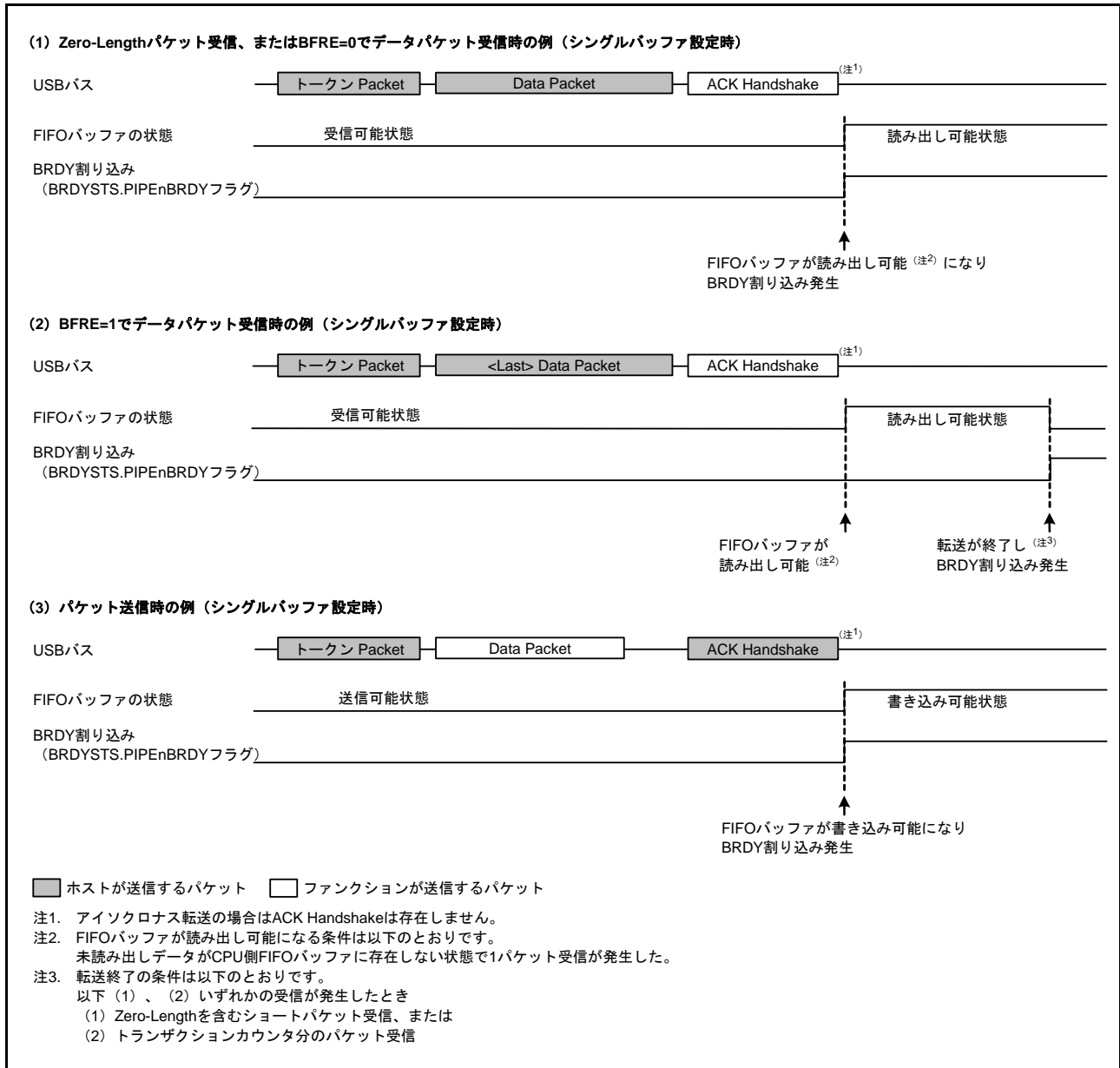
図 38.11 BRDY 割り込み発生タイミング図
