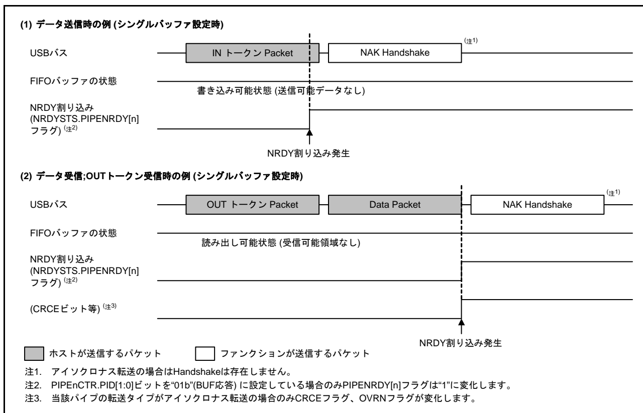
図 39.7 NRDY 割り込み発生タイミング図 (ファンクションコントローラ機能選択時)
