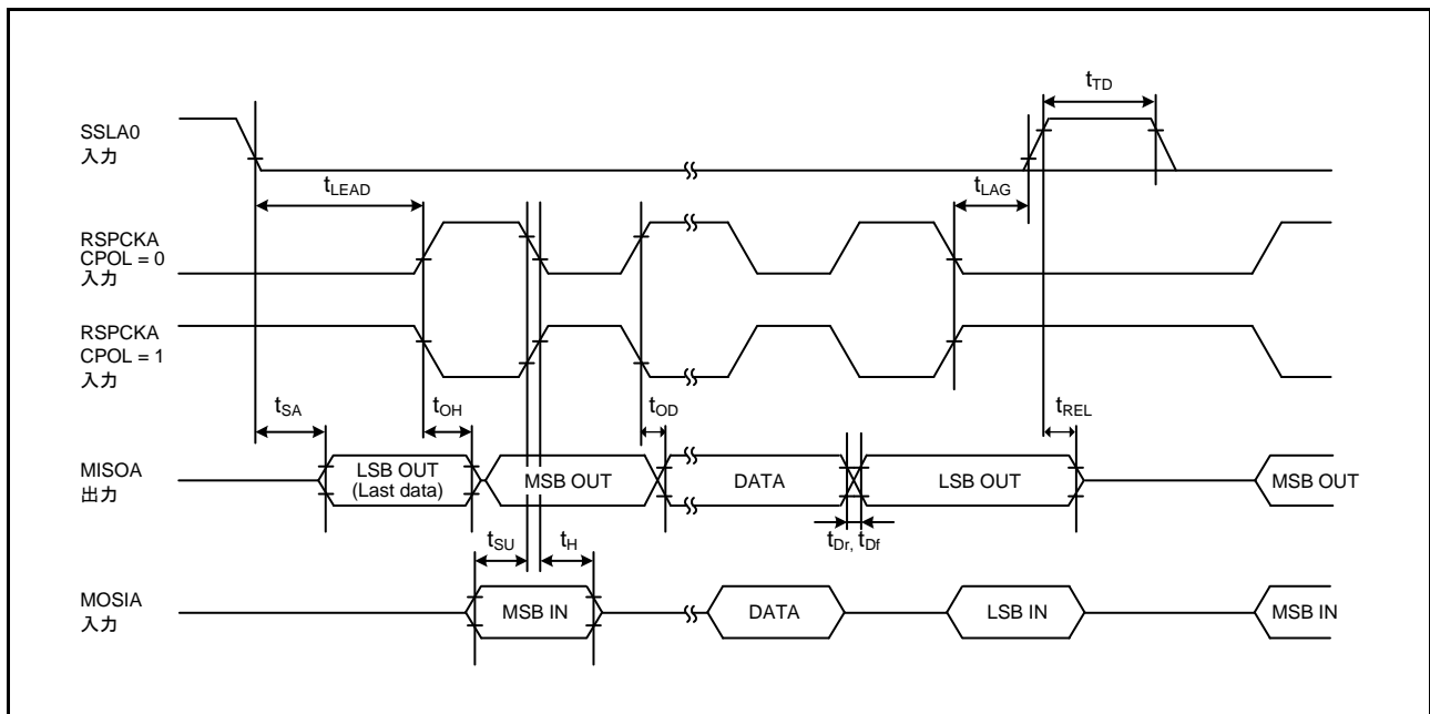
図 64.62 RSPi タイミング (スレーブ、CPHA = 1)
