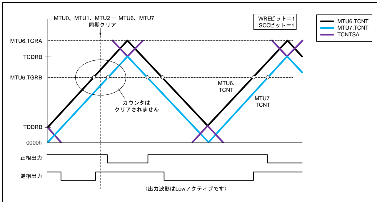
図 24.74 アップカウント中のデッドタイム時に同期クリアが発生した場合 (図 24.66 のタイミング③、MTU6、MTU7 の TWCRB レジスタの WRE ビット = 1、SCC ビット = 1)
