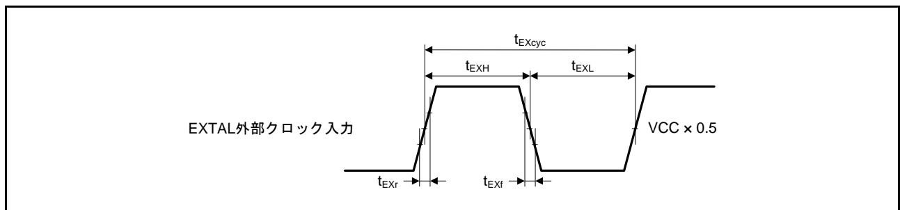
図 64.4 EXTAL 外部クロック入力タイミング
