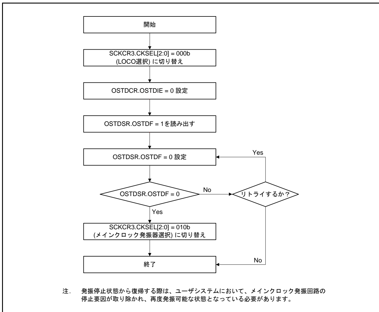
図 9.9 発振停止検出からの復帰のフローチャート例
