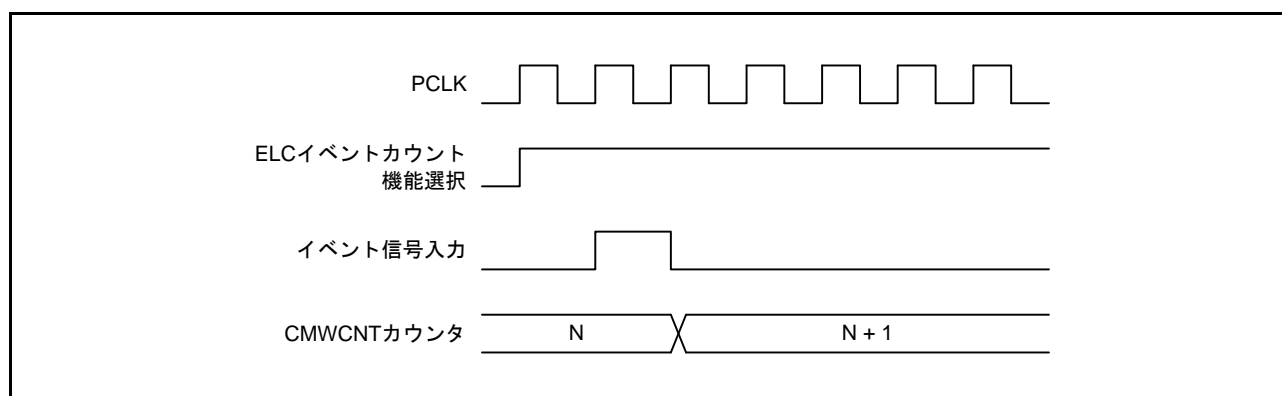
図 31.18 イベント受け付けによるイベントカウント動作
