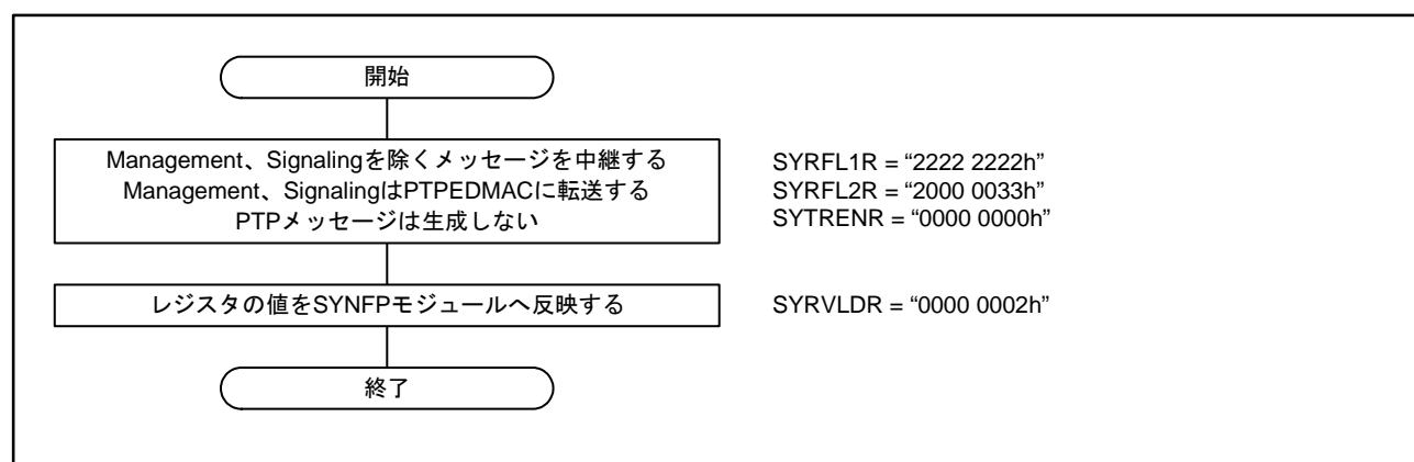
図36.22 E2E TC動作の開始手順
