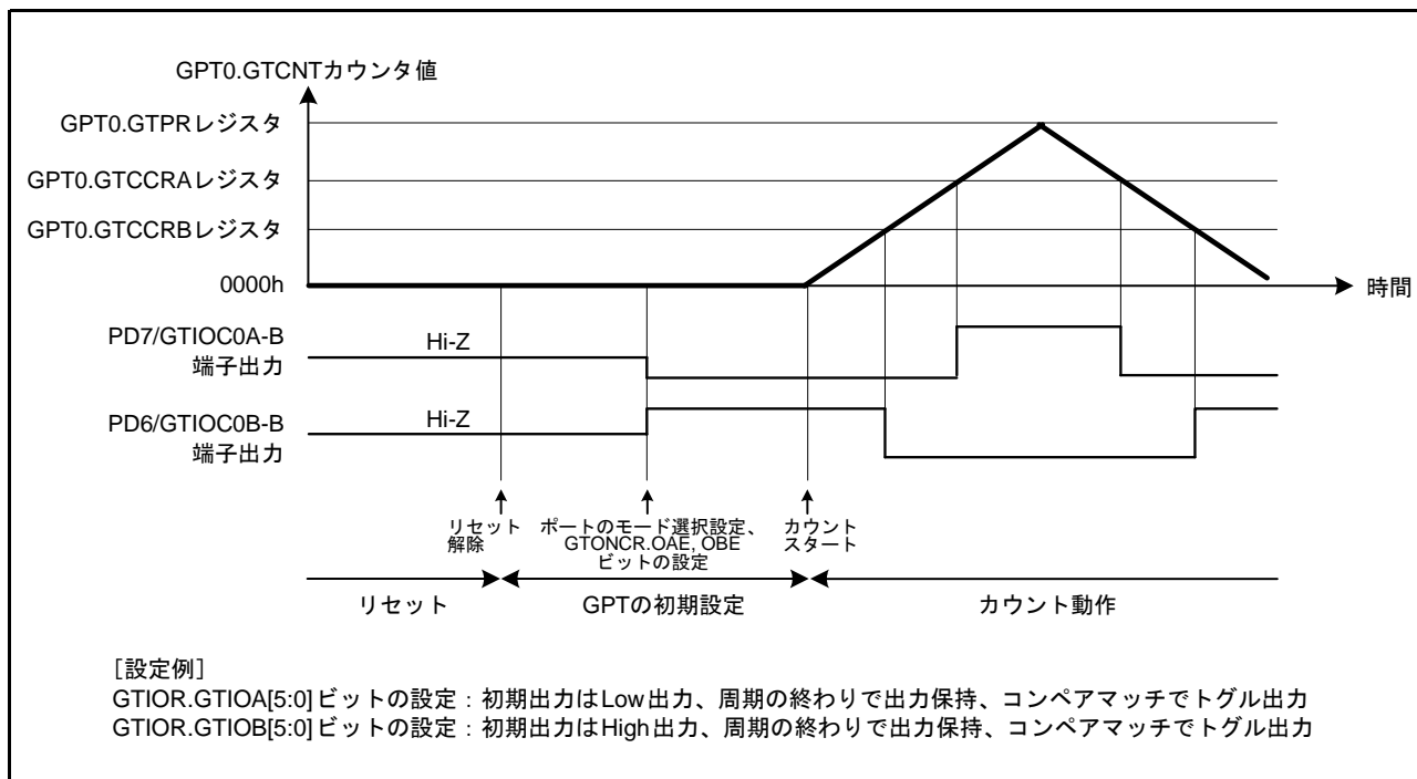
図 26.90 リセット後の端子設定例
