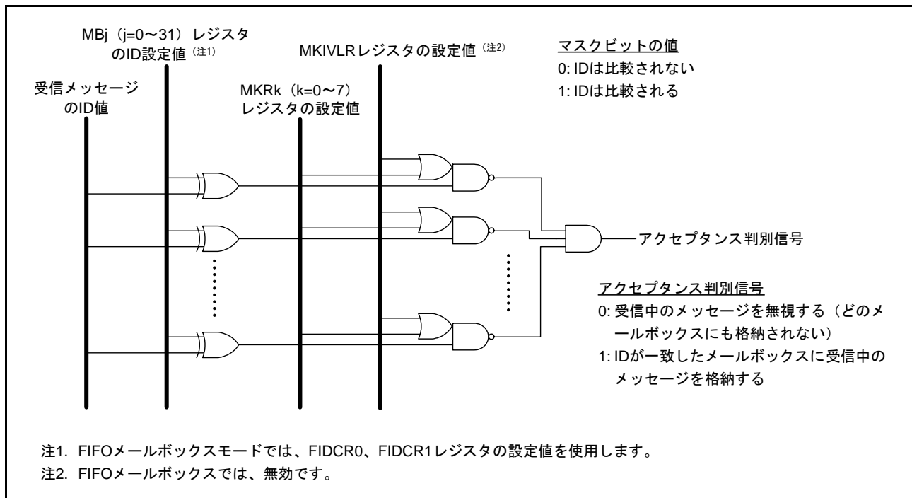
図 43.17 アクセプタンスフィルタ処理
