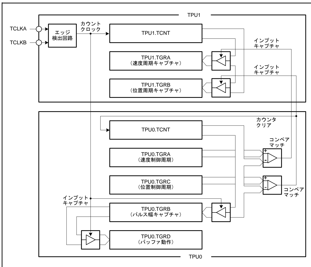
図 27.29 位相計数モードの応用例
