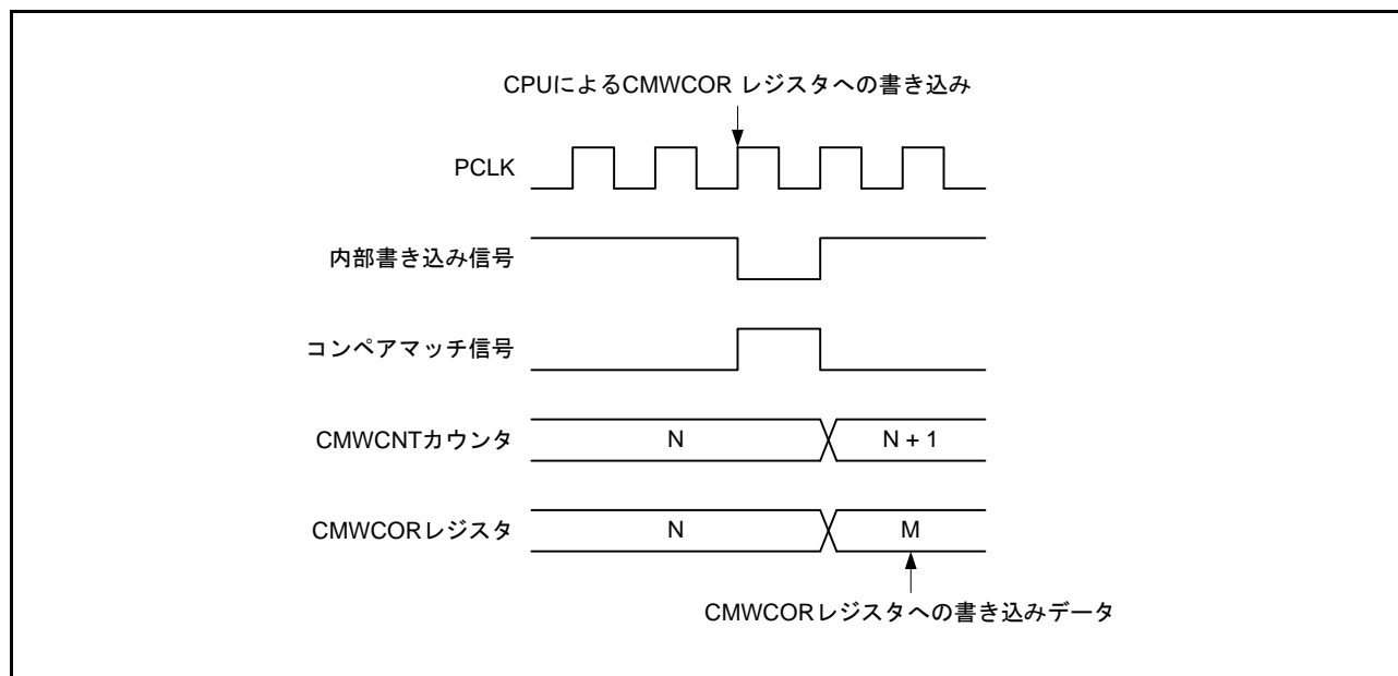
図 31.25 CMWCOR レジスタへの書き込みとコンペアマッチの競合
