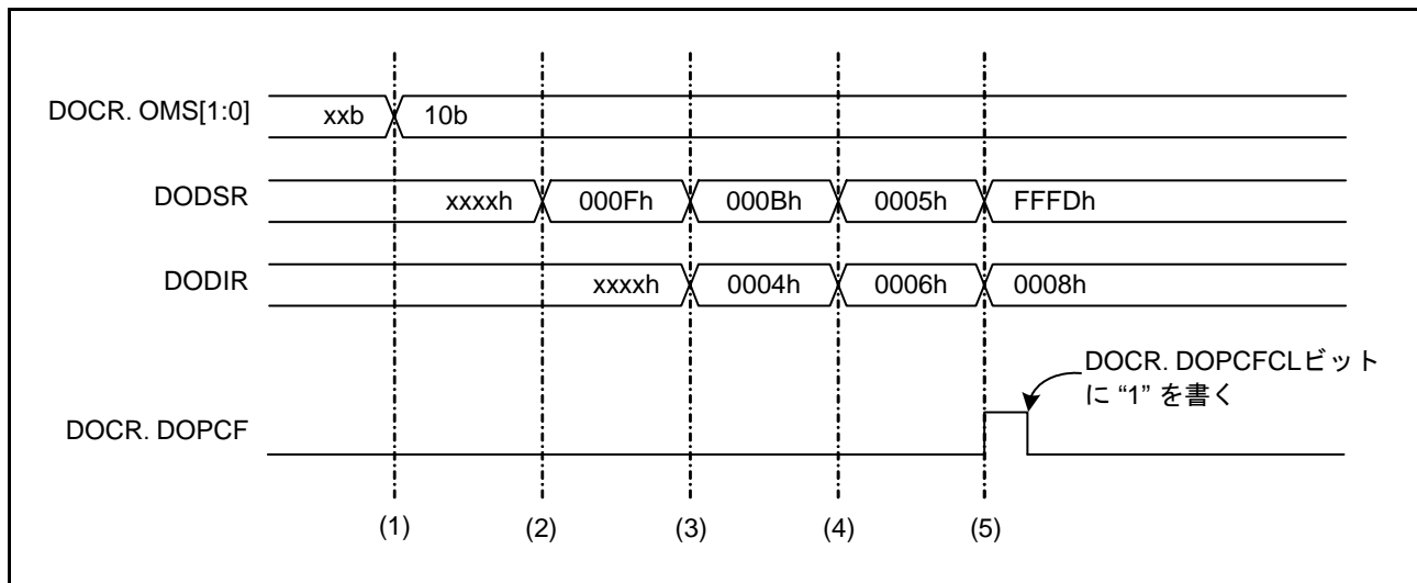
図 60.4 データ減算モードの動作例
