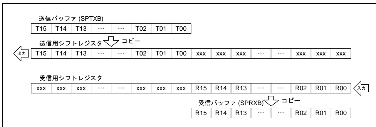
図 45.7 MSB ファースト転送 (16 ビットデータ)
