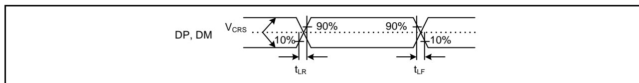
図 64.86 DP、DM 出カタイミング (ロースピード時)
