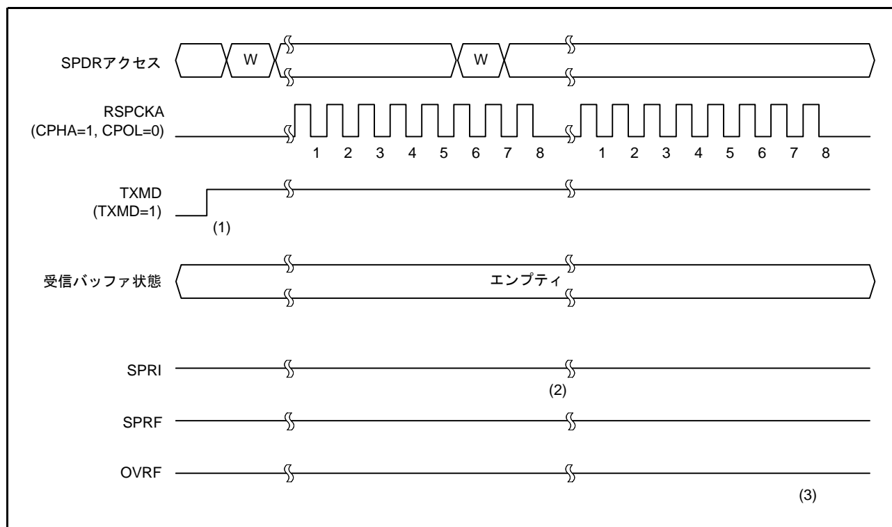
図 44.25 SPCR.TXMD = 1 の動作例
