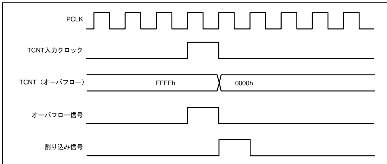
図 27.41 TCImV 割り込みのセットタイミング
