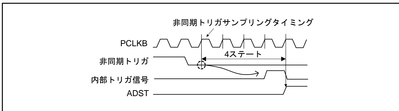
図 57.40 非同期トリガ入力タイミング
