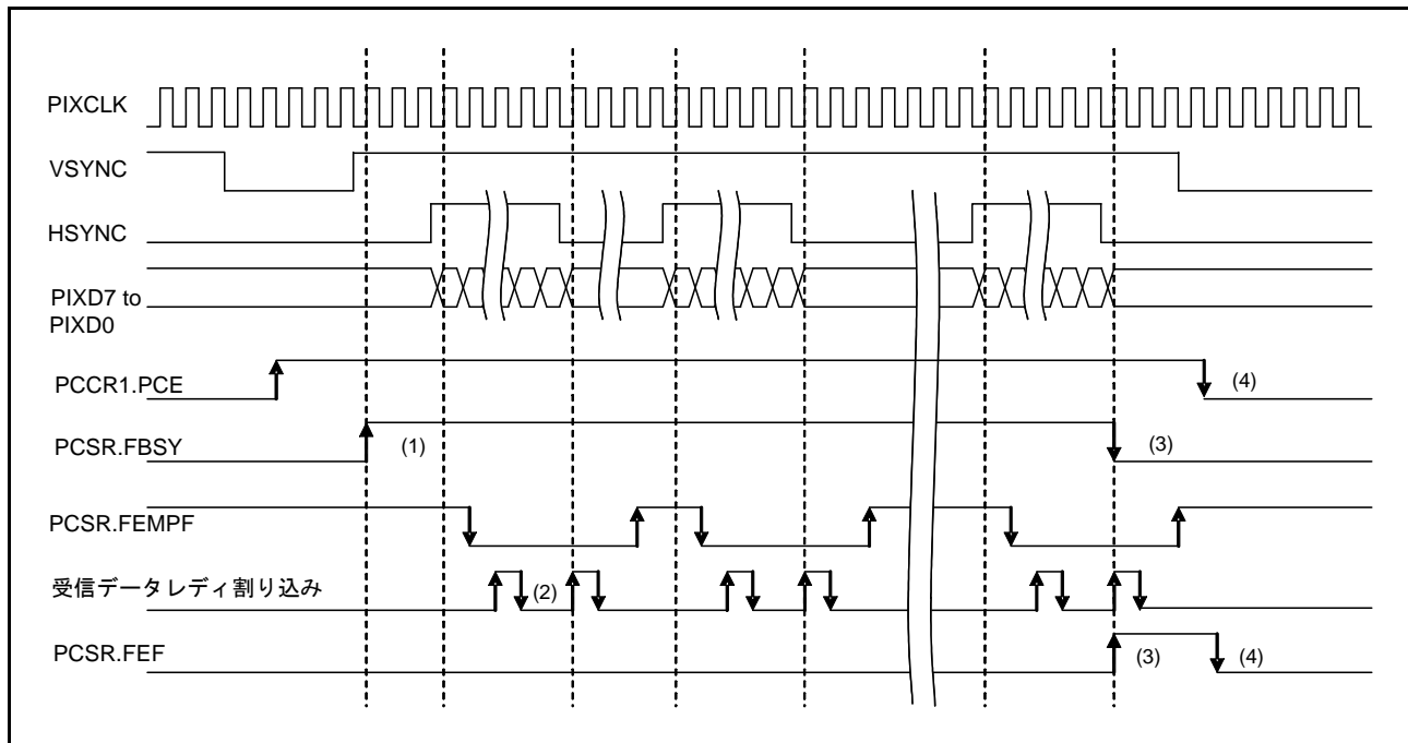
図 51.11 受信動作例
