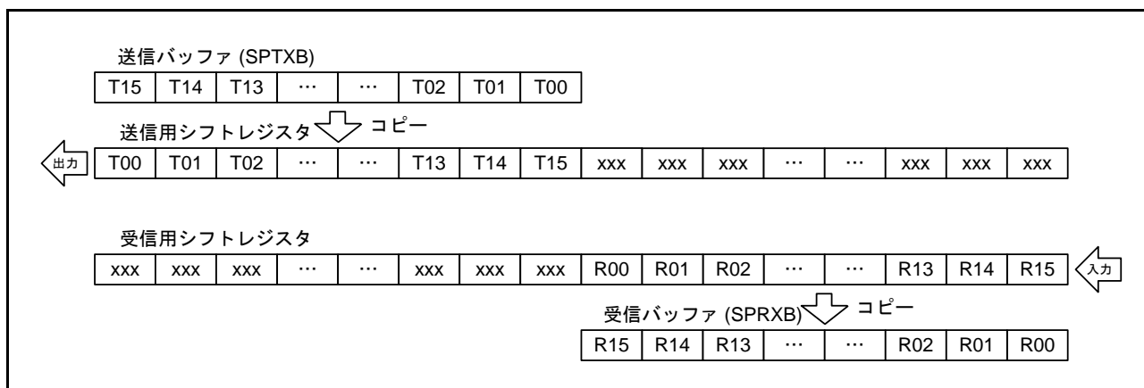
図 45.10 LSB ファースト転送 (16 ビットデータ)
