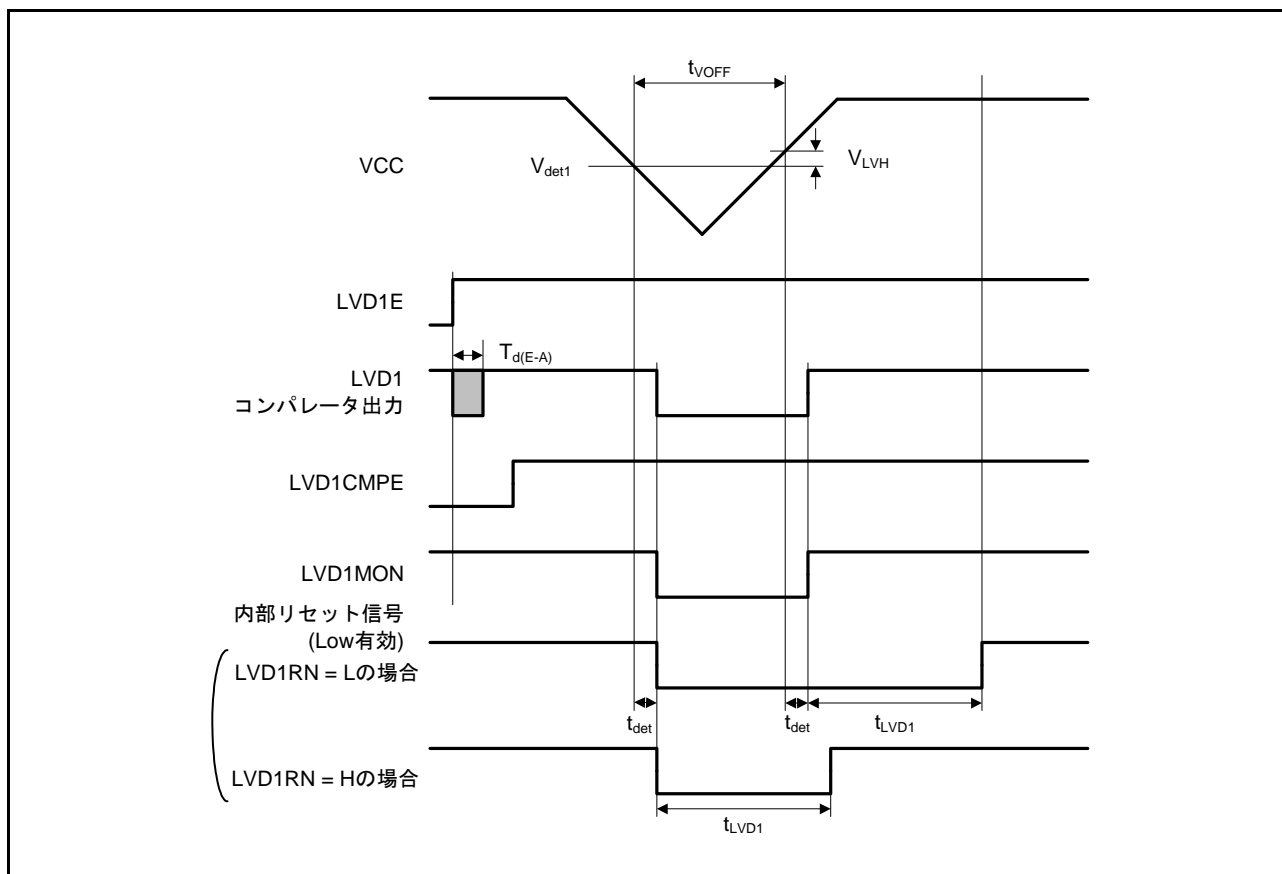
図 64.92 電圧検出回路タイミング ( V_{det1} )
