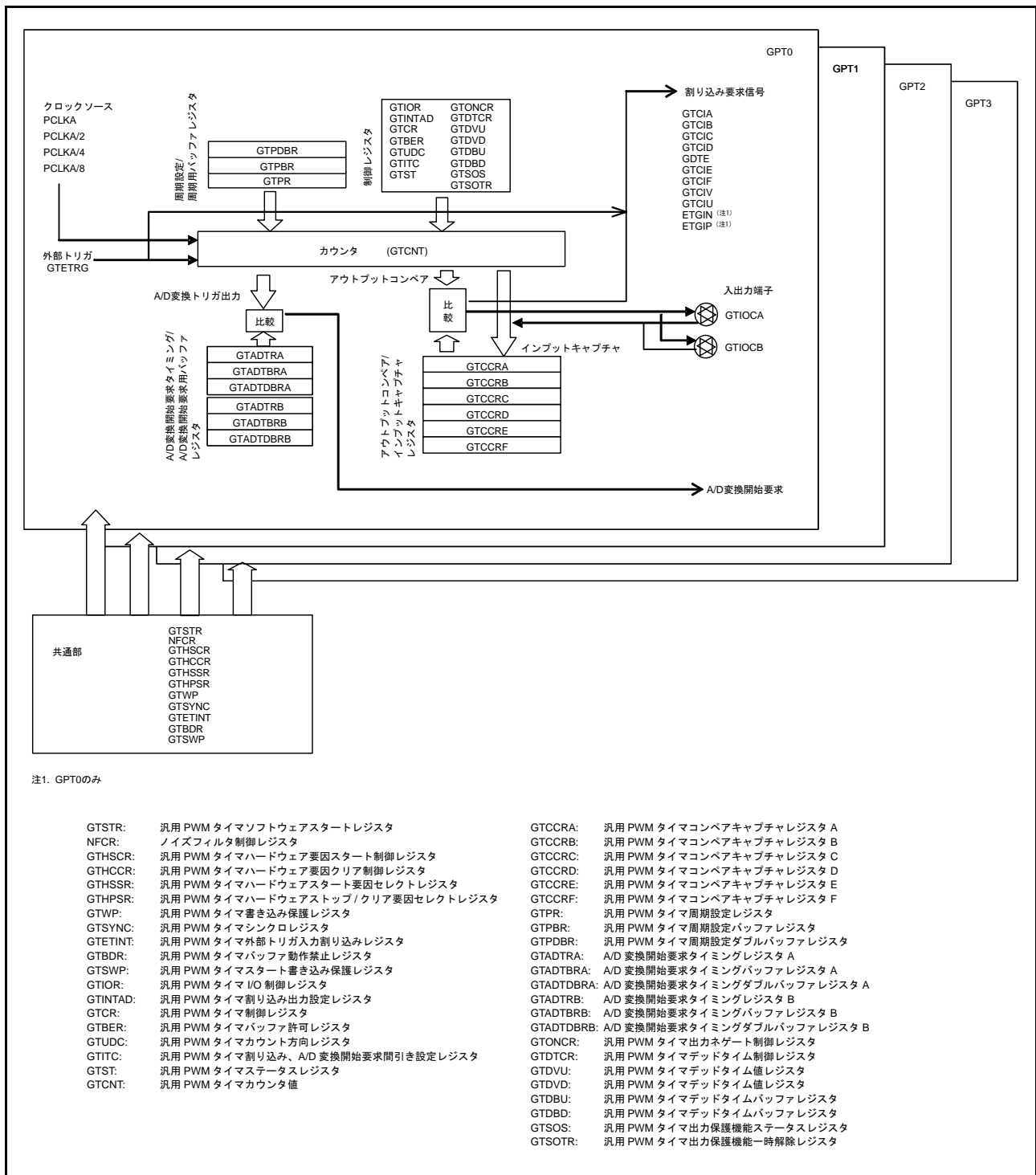
図 26.1 GPT のブロック図
