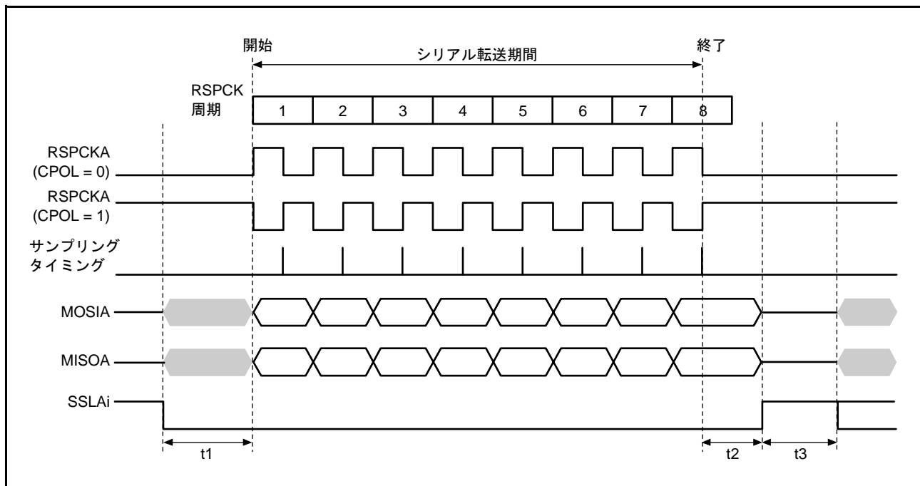
図 44.23 RSPI 転送フォーマット (CPHA ビット = 1)
