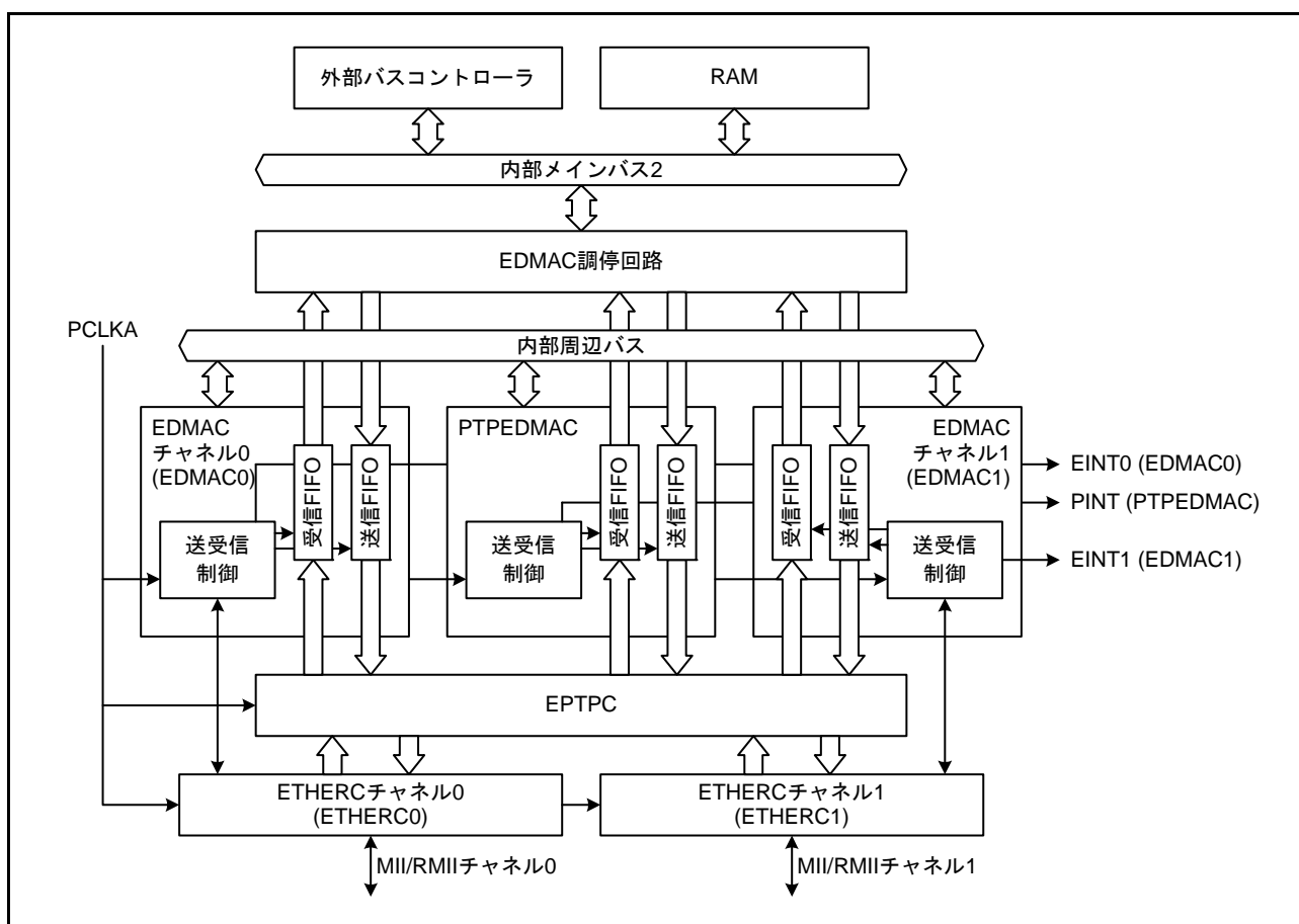
図 37.1 EDMAC の構成
