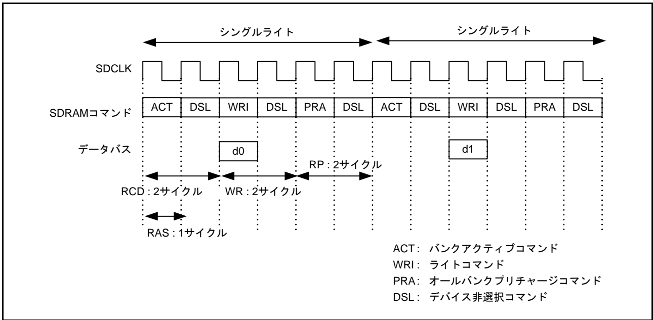
図 16.75 シングルライトタイミング例 (3)
