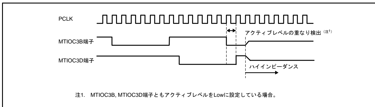
図 25.5 出力レベル検出動作
