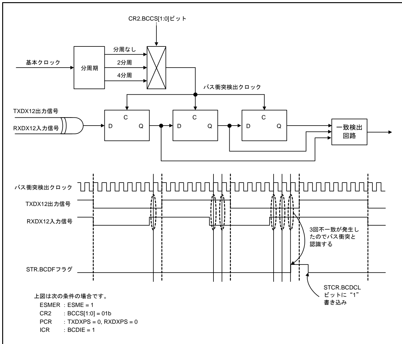
図 40.69 バス衝突検出機能の動作例
