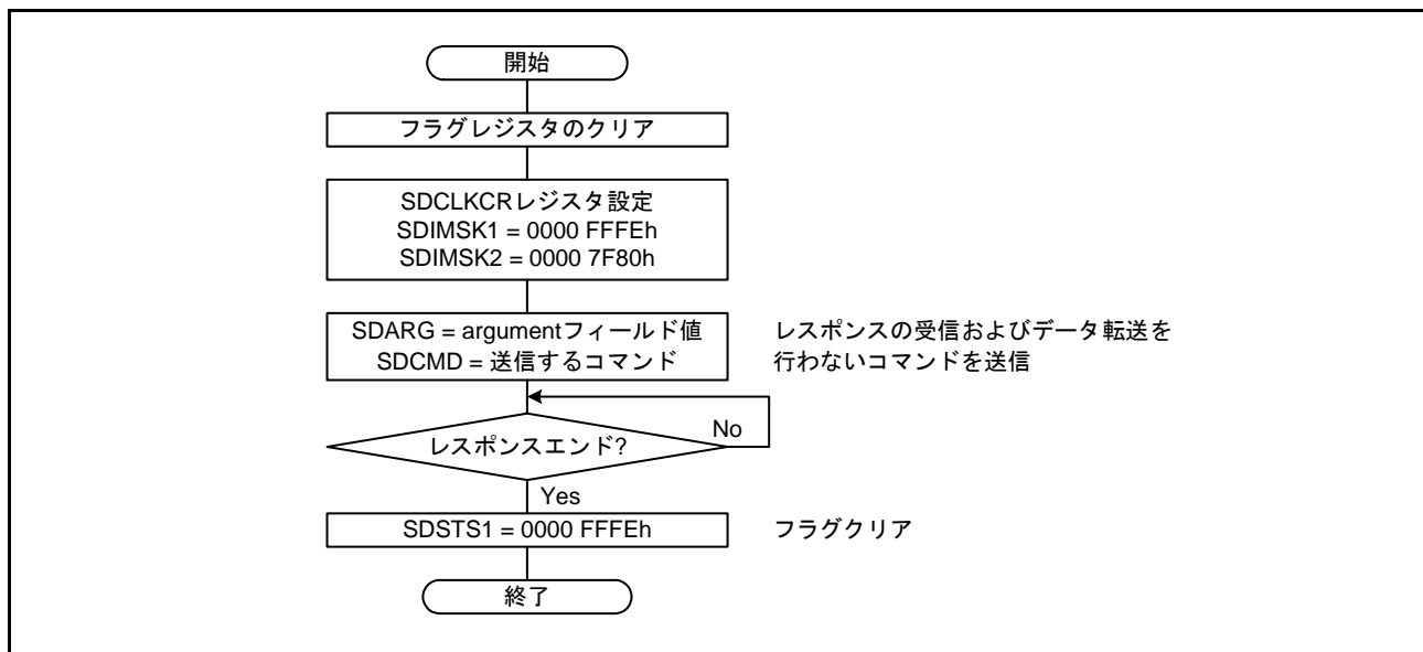
図 49.8 レスポンスの受信とデータ転送のないコマンドの送信例
