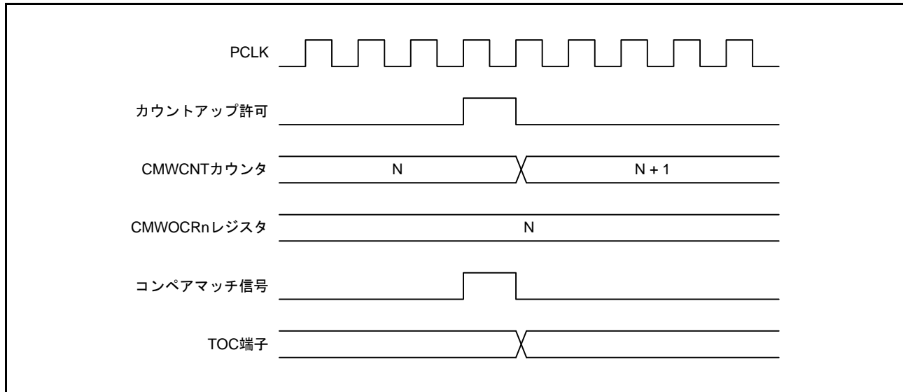
図 31.11 アウトプットコンペア出力タイミング
