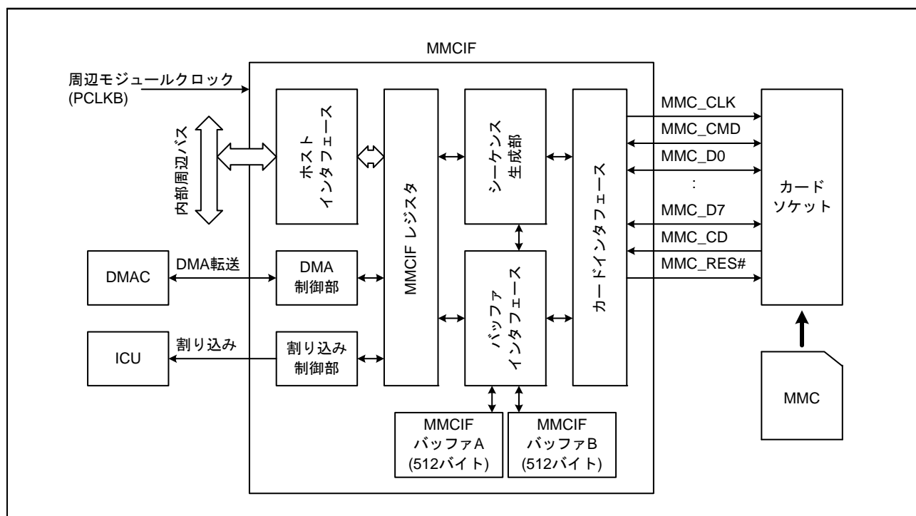
図 50.1 MMCIF のブロック図
