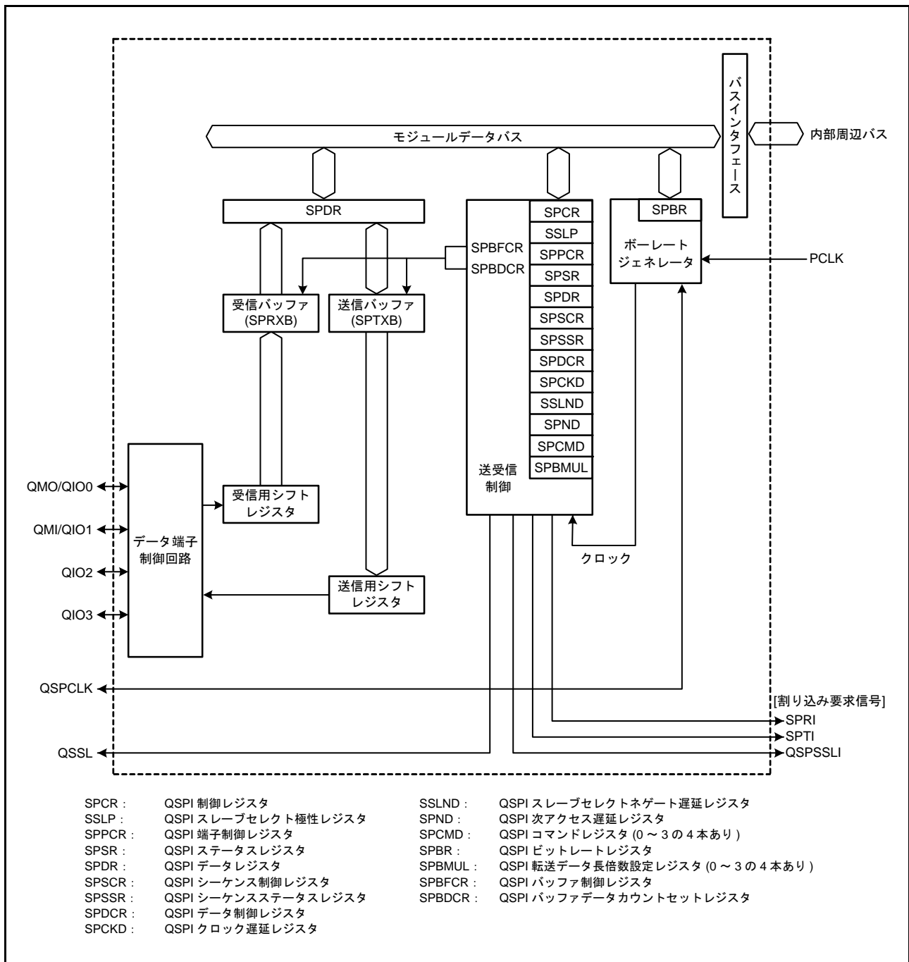
図 45.1 QSPI のブロック図
