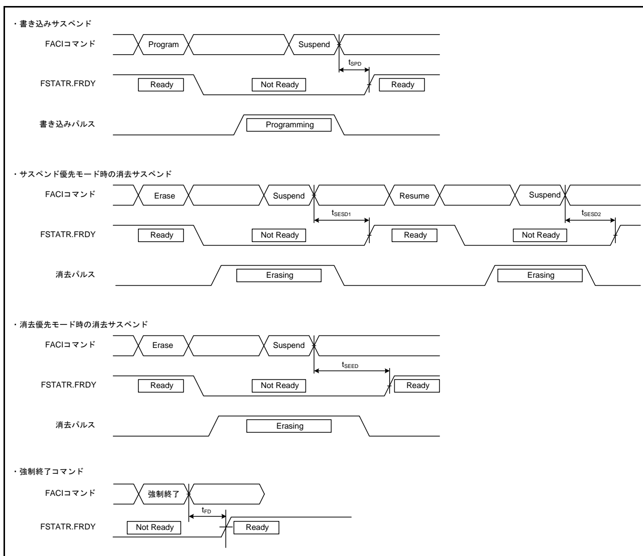
図 64.96 フラッシュメモリプログラム/イレーズサスペンドタイミング
