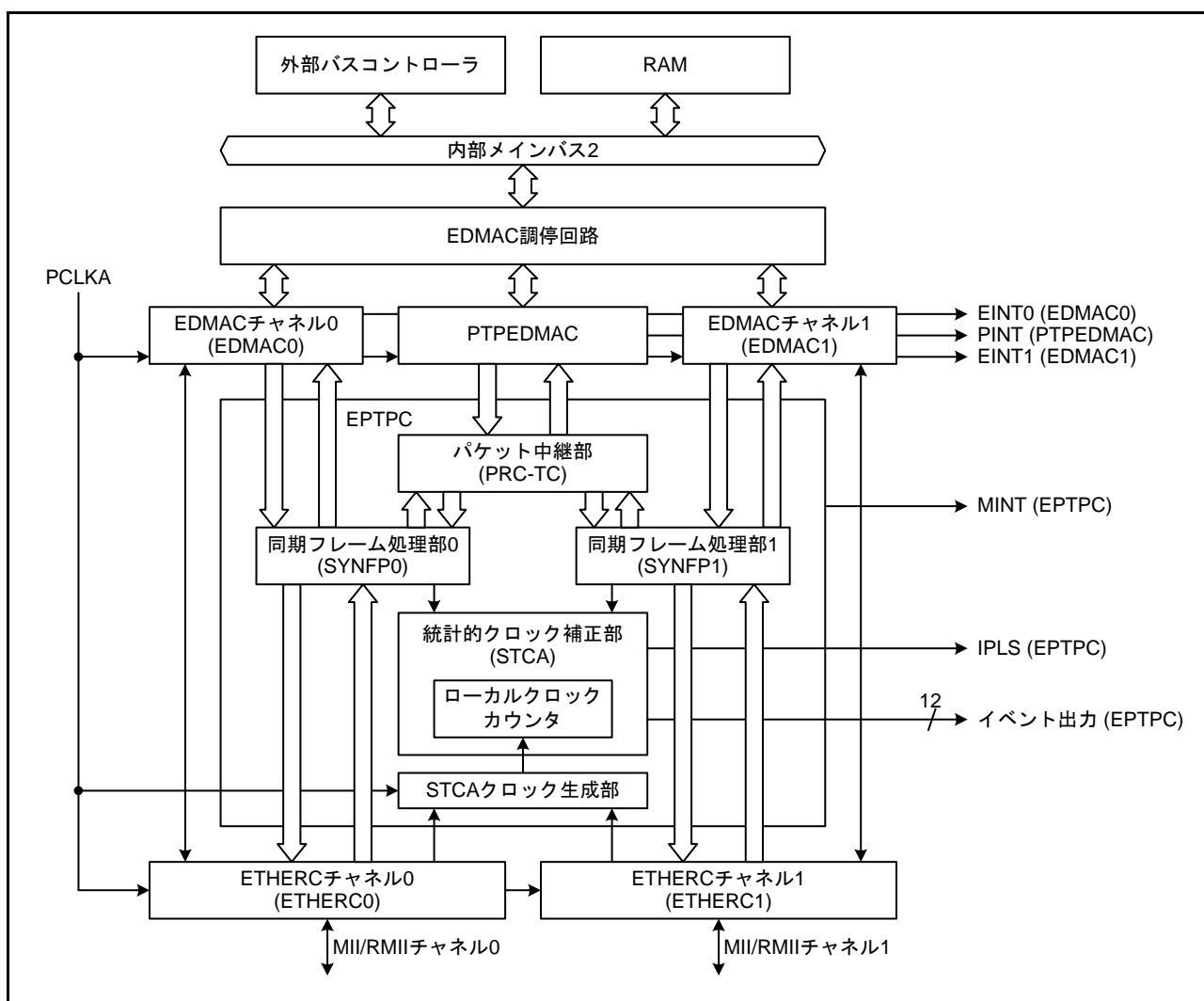
図36.1 EPTPCの構成
