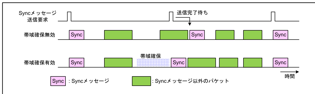
図36.35 Syncメッセージ送信帯域確保機能
