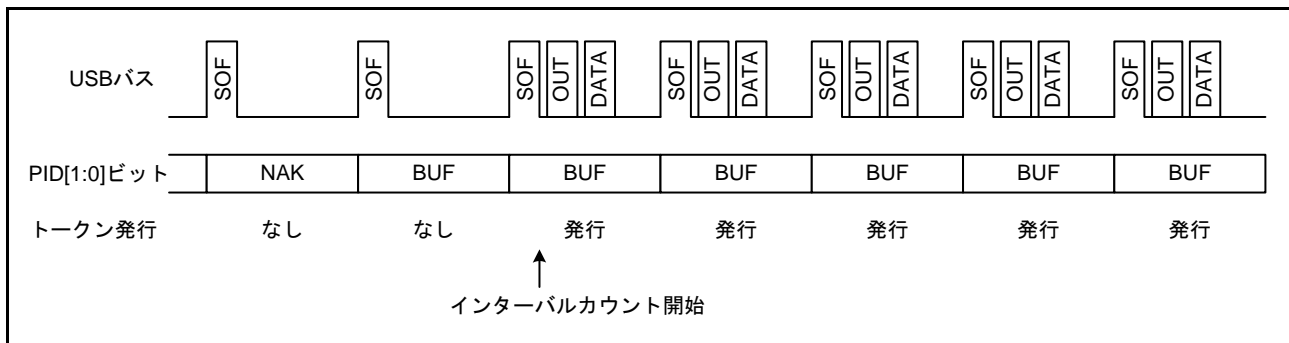
図 39.13 IITV[2:0] ビットが“000b”の場合のトークン発行有無
