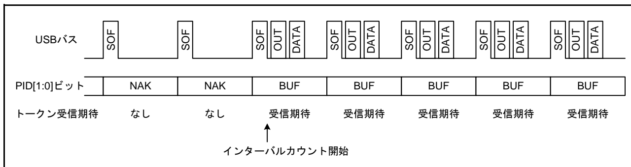
図 39.15 IITV[2:0] ビットが “000b” の場合のフレームとトークン受信期待有無の関係
