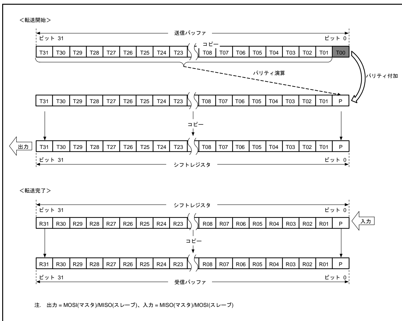
図 44.18 MSB ファースト転送 (32 ビットデータ / パリティ機能有効)
