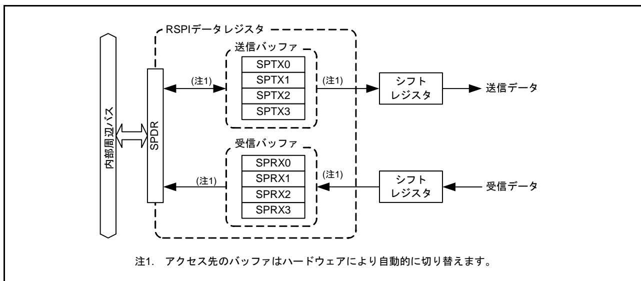
図 44.2 SPDR レジスタの構造図
