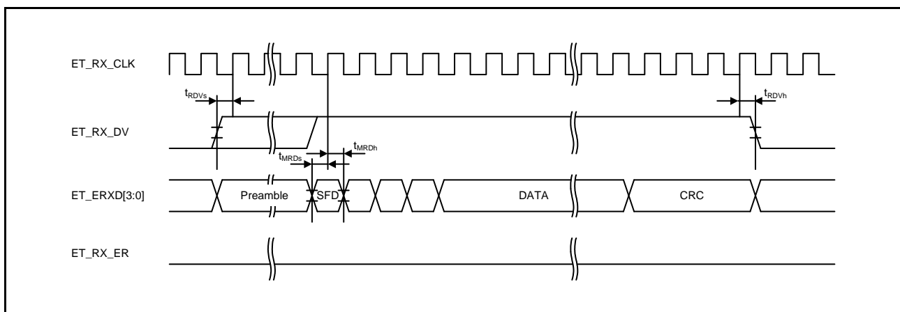
図 64.79 MII 受信タイミング (正常動作時)
