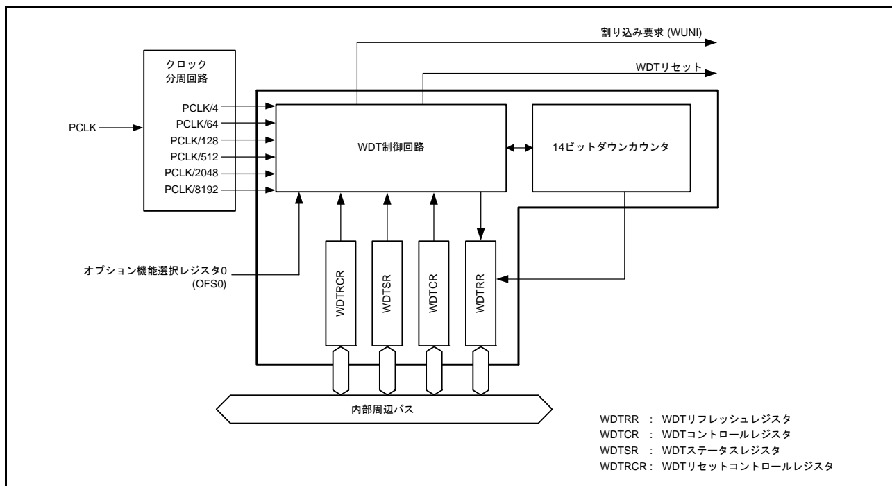
図 33.1 WDT のブロック図
