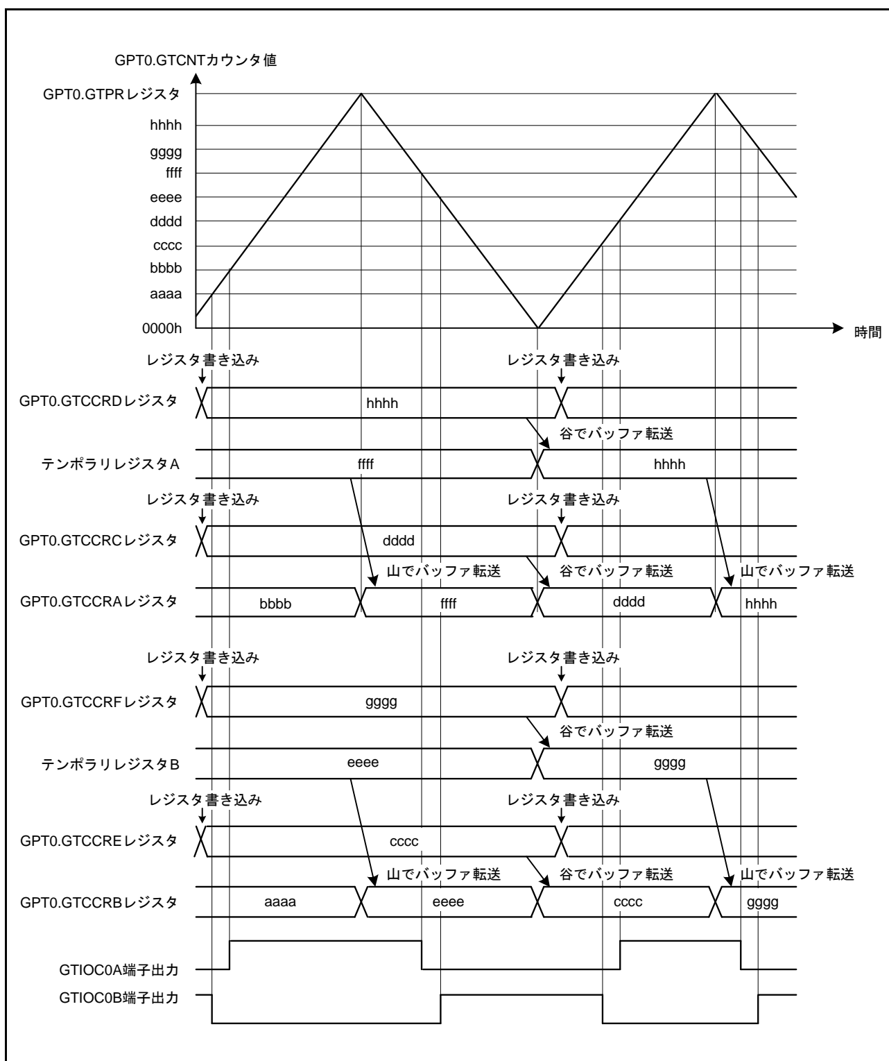
図 26.35 三角波 PWM モード 3 動作例 (初期出力で GTIOC0A 端子 = Low 出力 / GTIOC0B 端子 = High 出力、GTCCRA/GTCCRB レジスタのコンペアマッチでトグル出力、周期の終わりで出力保持の場合)
