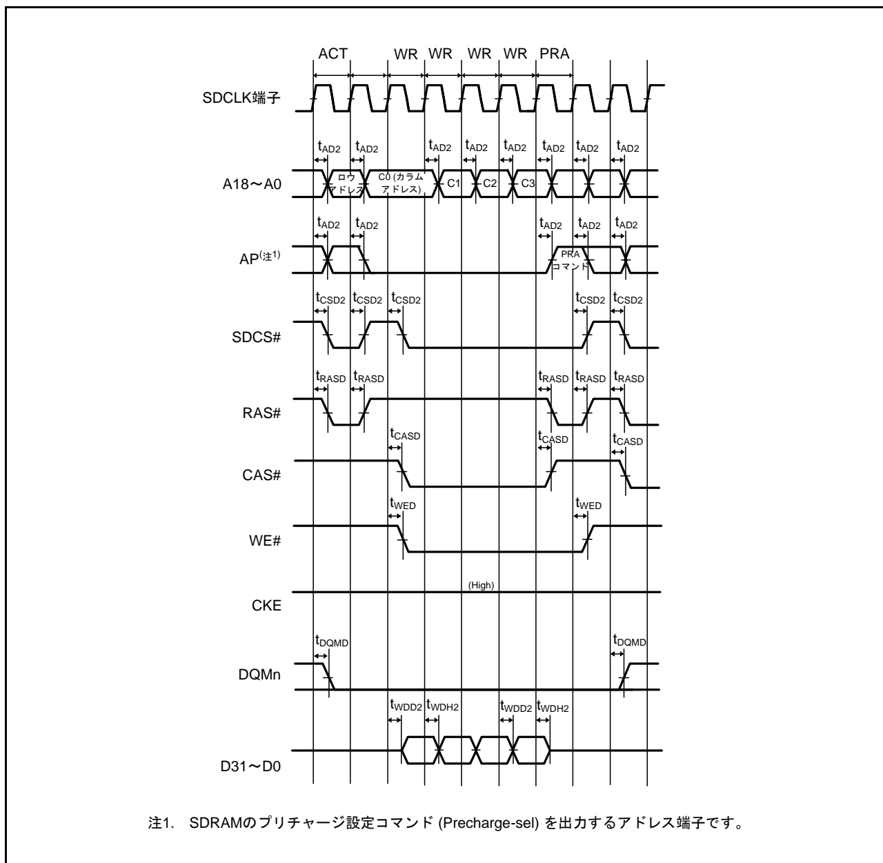
図 64.26 SDRAM 空間複数ライトバスタイミング
