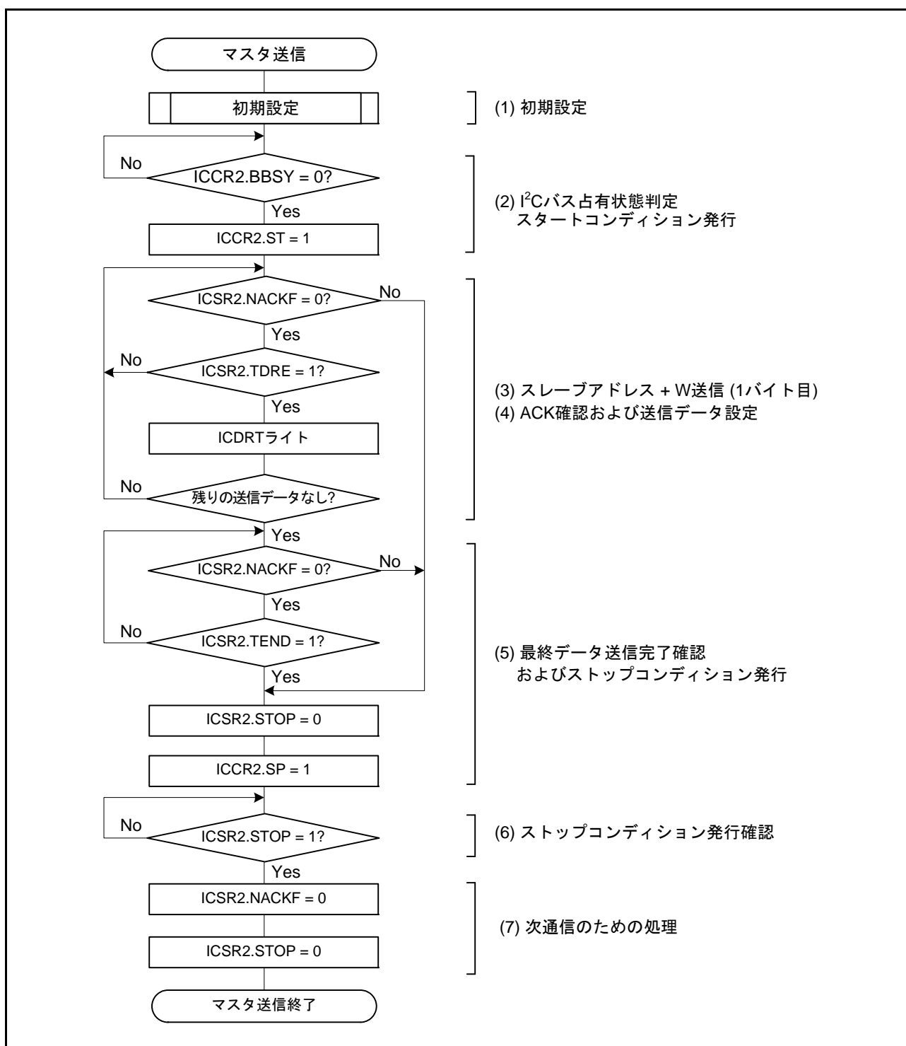
図 42.5 マスタ送信のフローチャート例
