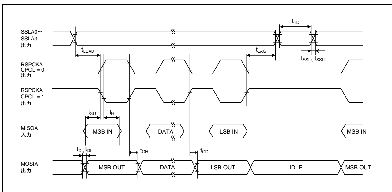
図 64.57 RSPCKA タイミング (マスタ、CPHA = 0) (ビットレート : PCLKB を 2 分周以外に設定)
