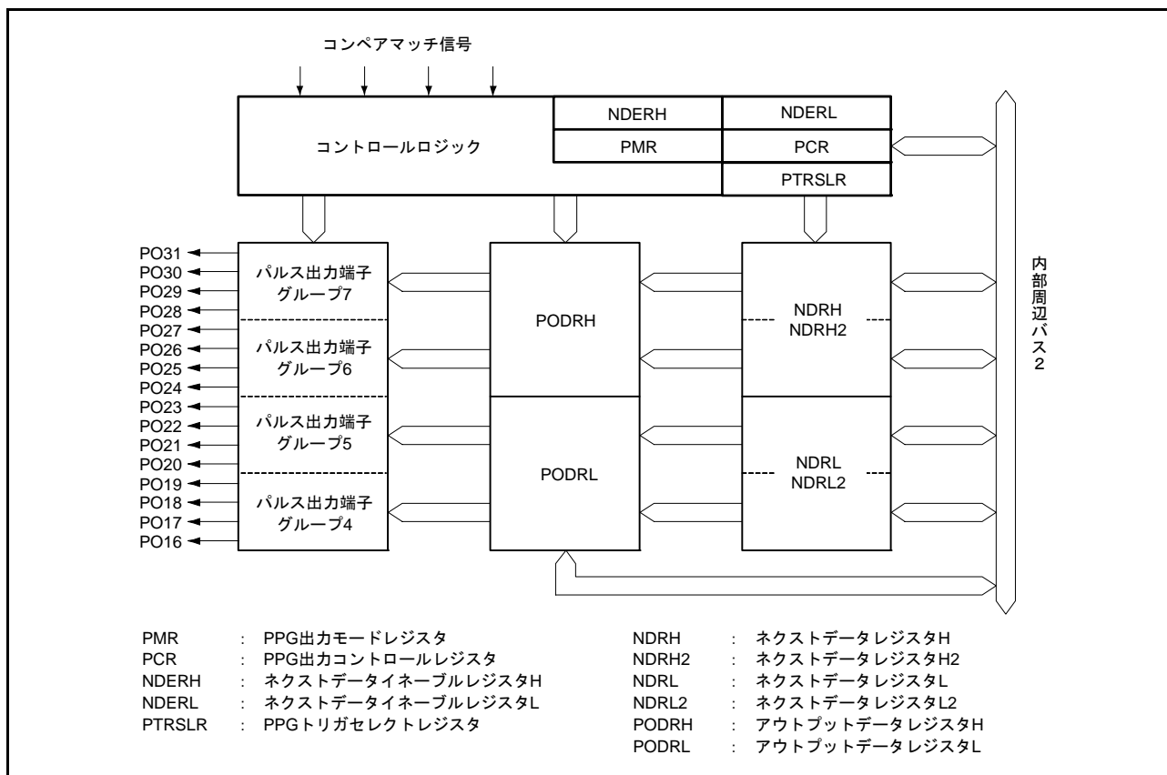
図 28.2 PPG1 のブロック図
