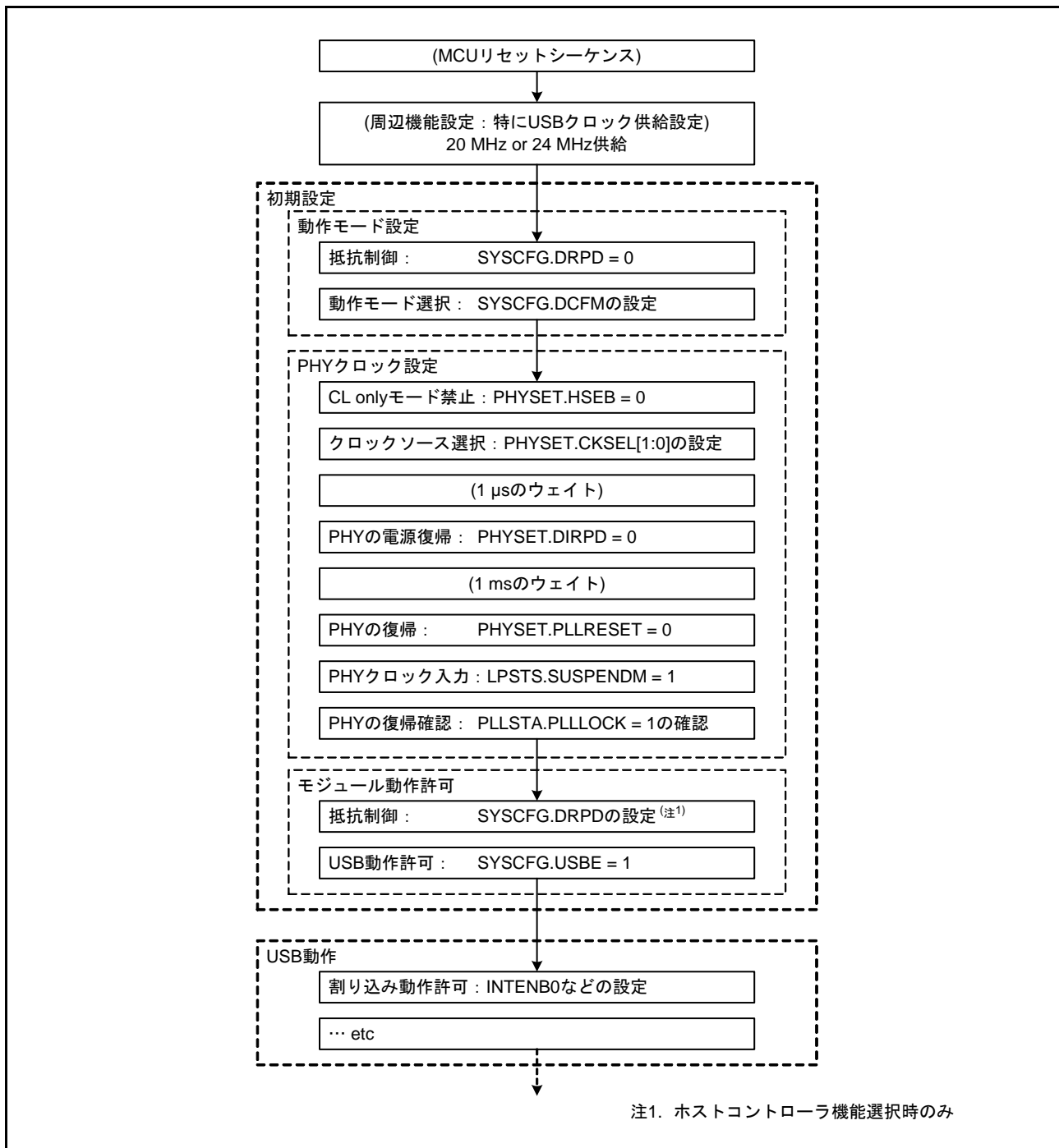
図 39.3 PHY クロック設定方法 (CL only モードでない時)
