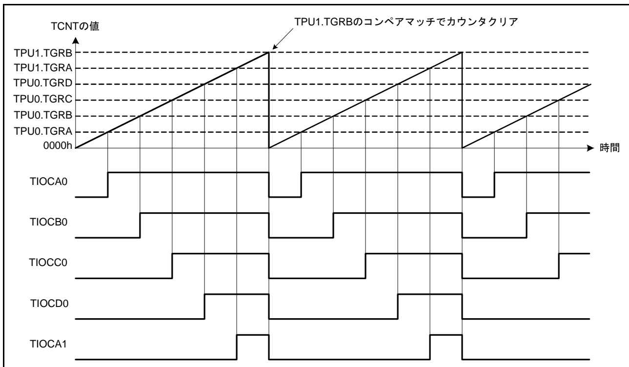
図 27.22 PWM モードの動作例 (2)
