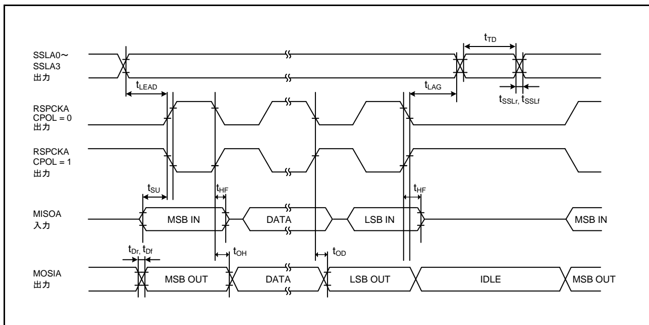
図 64.58 RSPCKA タイミング (マスタ、CPHA = 0) (ビットレート : PCLKB を 2 分周に設定)
