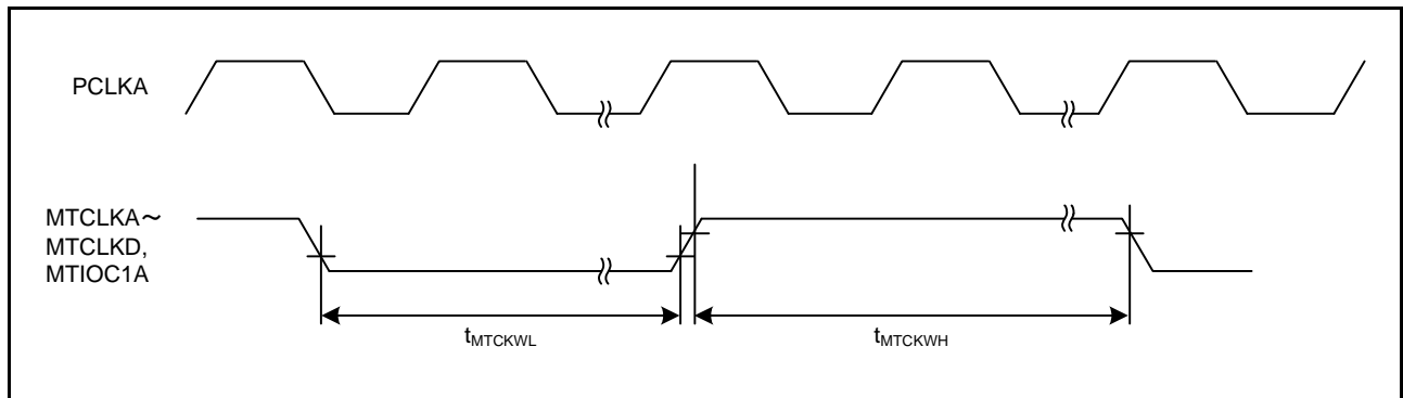
図 64.39 MTU3 クロック入力タイミング
