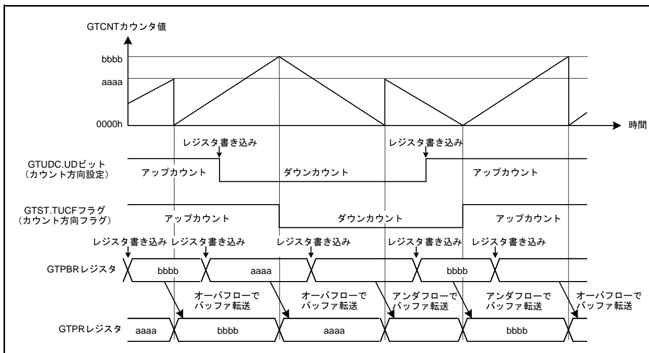
図 26.43 カウンタ方向切り替え機能の動作例（バッファ動作時）
