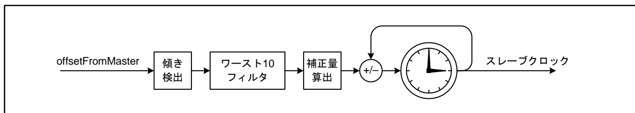
図36.24 時刻補正回路の構成
