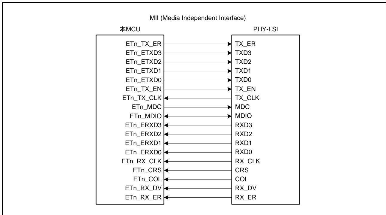
図 35.2 PHY-LSI との接続例 (MII)
