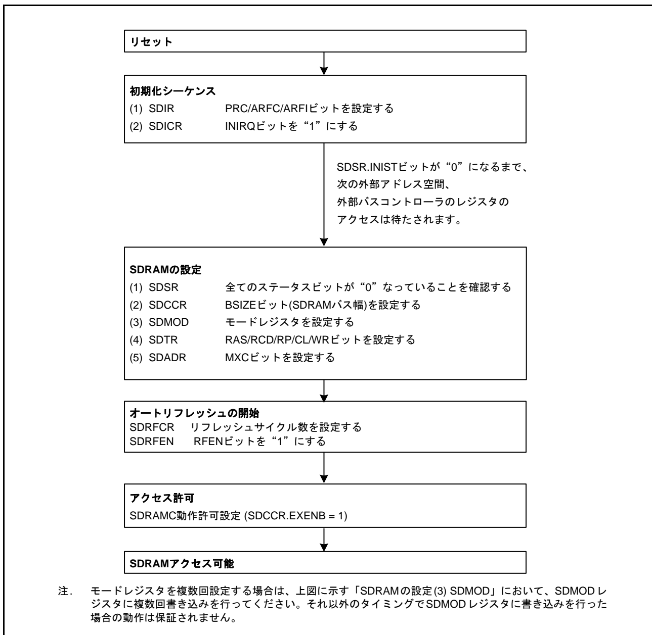
図 16.65 SDRAMC の設定手順
