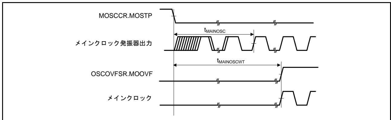
図 64.5 メインクロック発振開始タイミング
