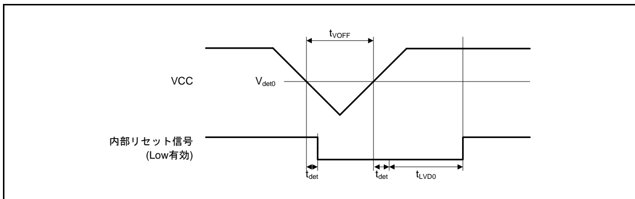
図 64.91 電圧検出回路タイミング ( V_{det0} )
