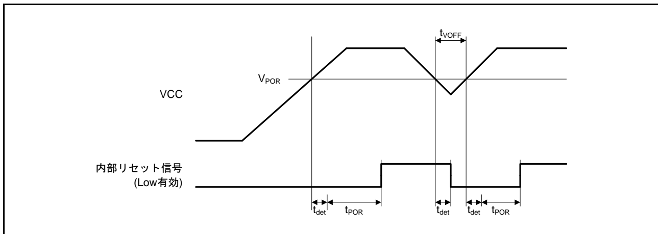
図 64.90 パワーオンリセットタイミング
