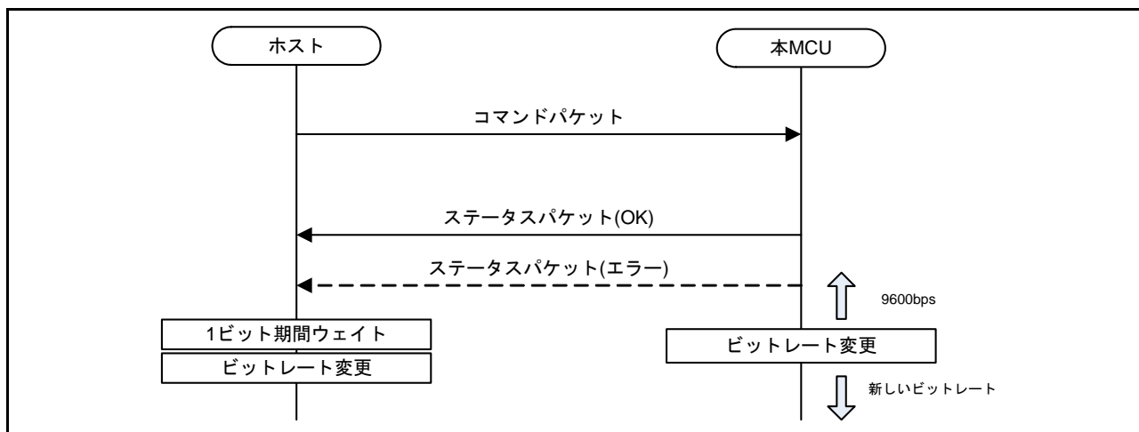
図 63.13 ビットレート設定コマンドの通信シーケンス
