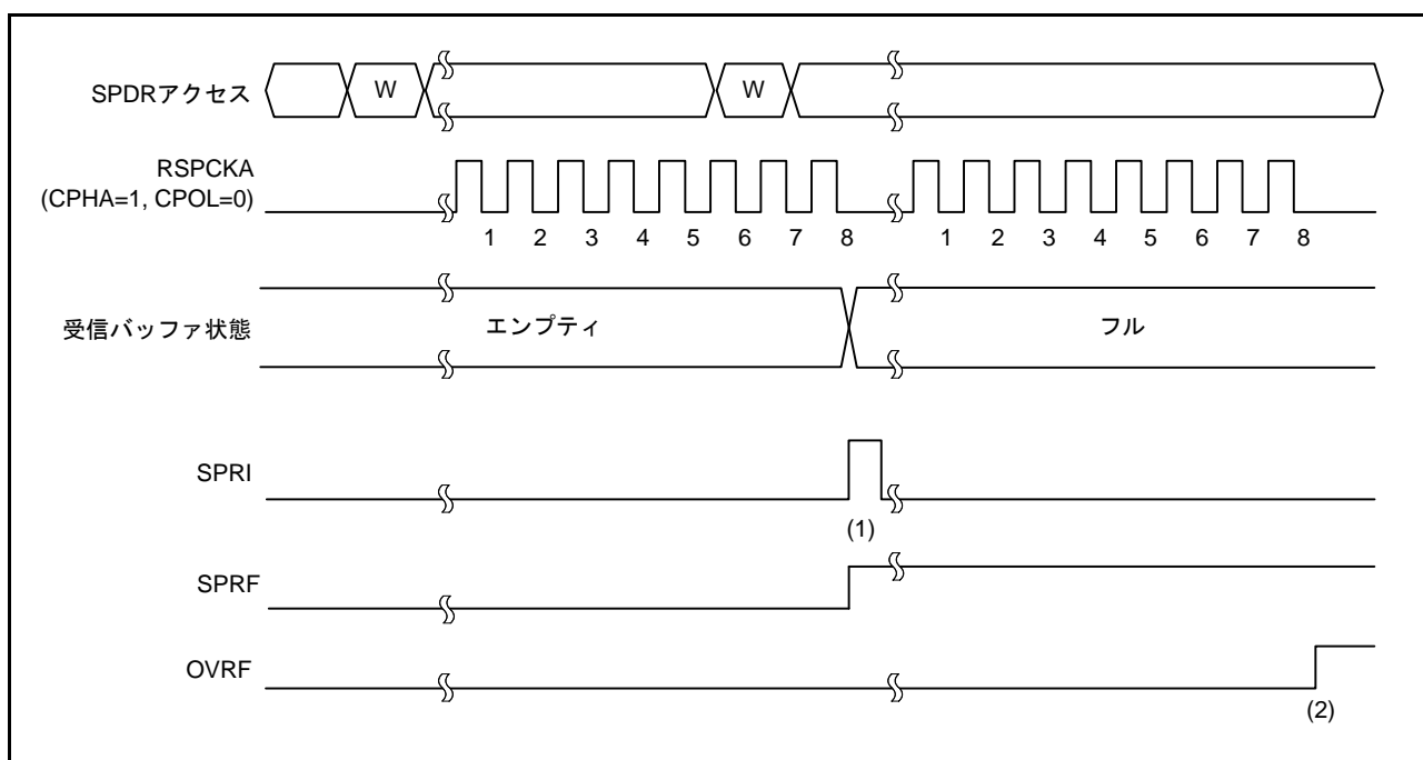
図 44.24 SPCR.TXMD = 0 の動作例
