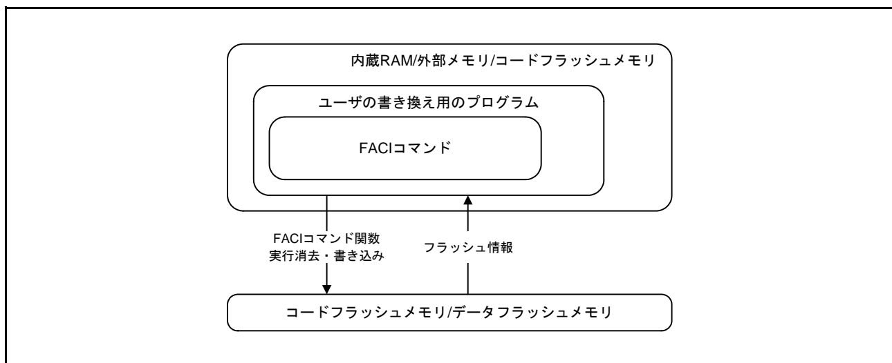
図 63.21 セルフプログラミングの概念
