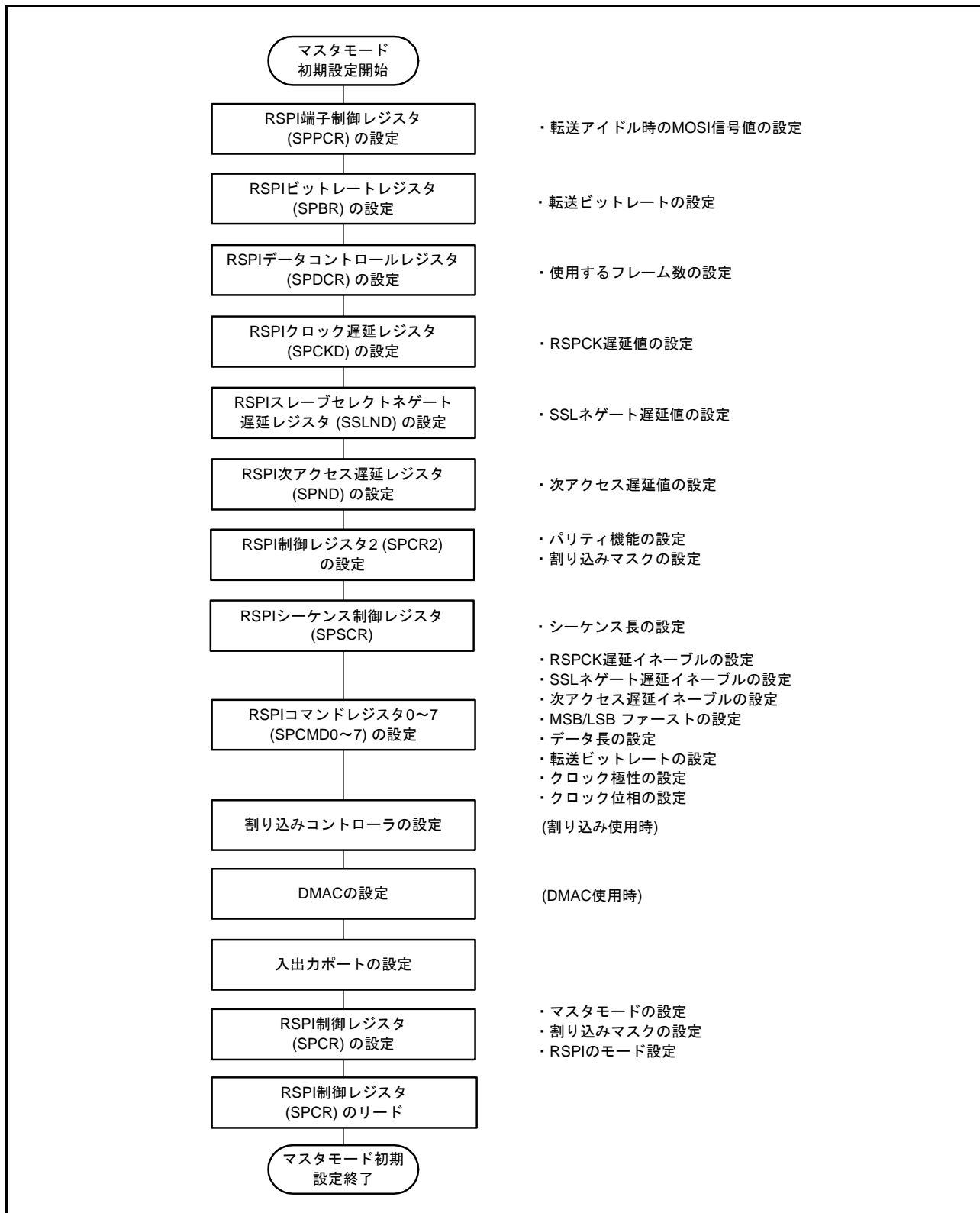
図 44.46 マスタモード時の初期化フロー例 (クロック同期式動作)
