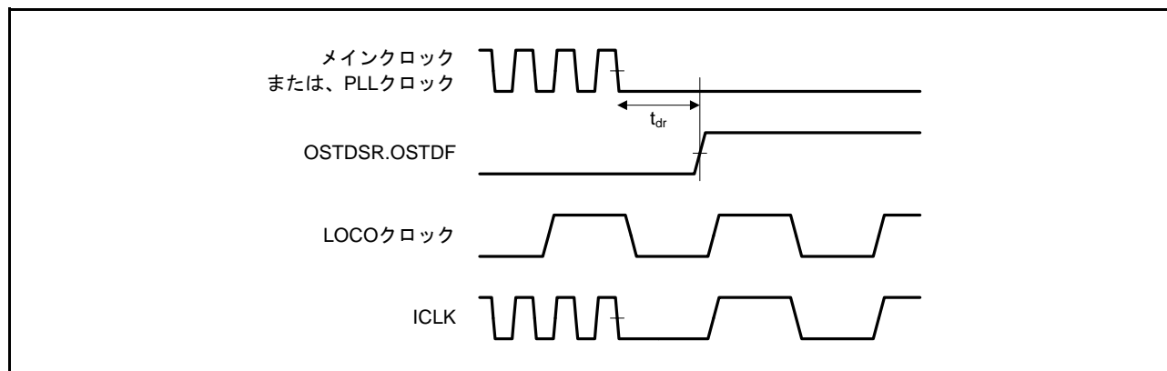
図 64.94 発振停止検出タイミング
