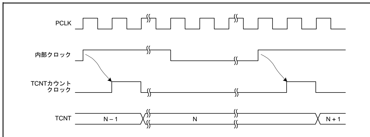
図 29.5 内部クロック動作時のカウンタタイミング
