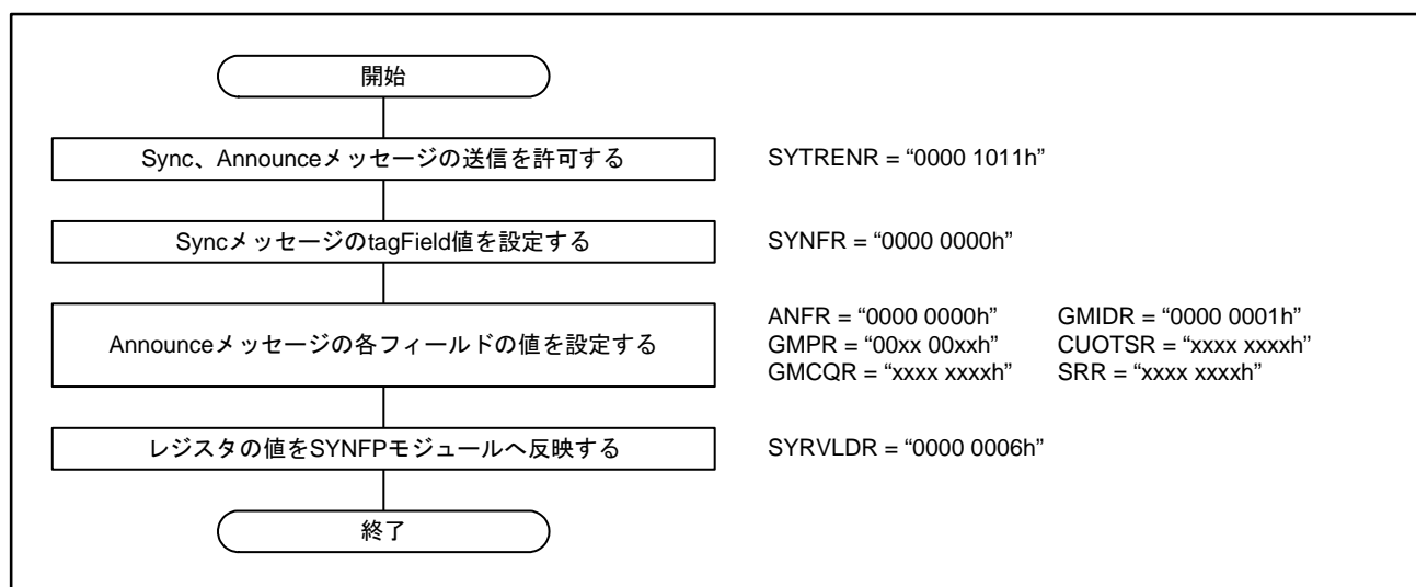
図36.18 P2Pマスタ動作の開始手順
