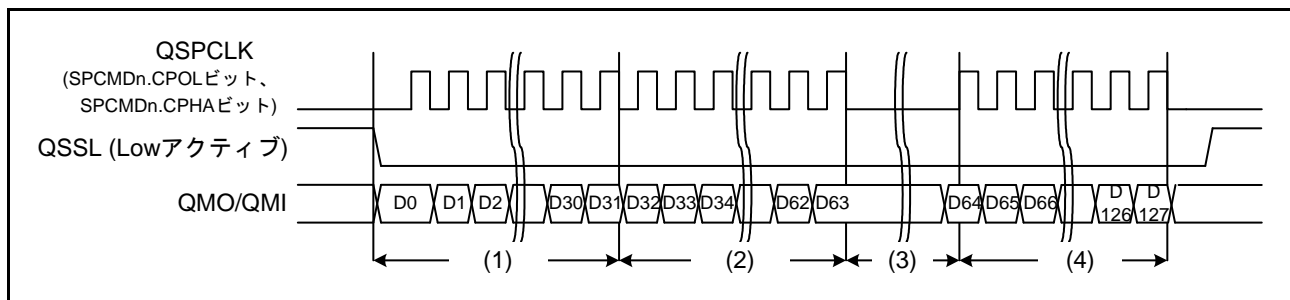
図 45.13 転送データ長を 128 ビットに設定したバースト転送の例 (Single-SPI モード) ( n = 0 \sim 3 )
