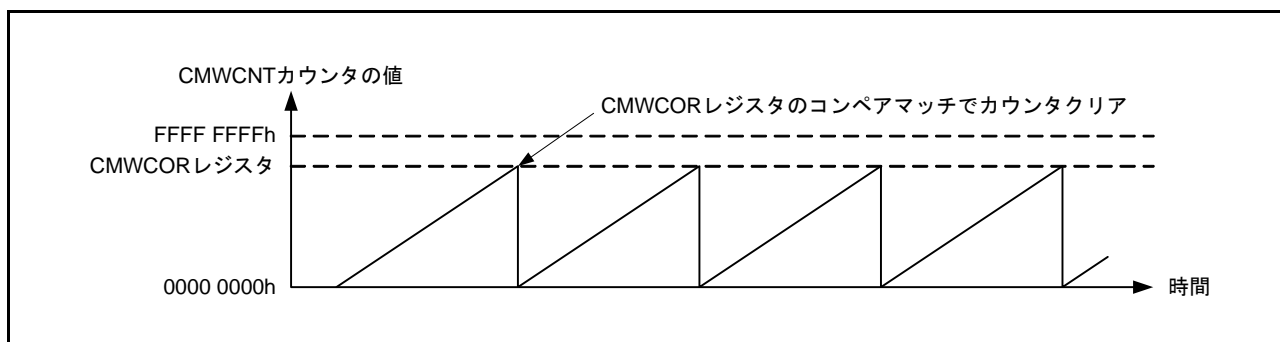
図 31.4 コンペアマッチ動作例
