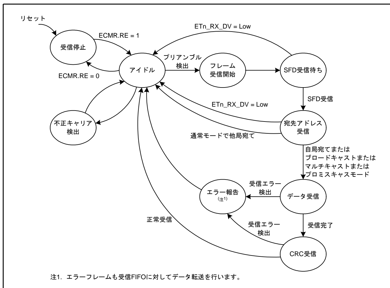
図 35.5 ETHERC 受信部状態遷移図
