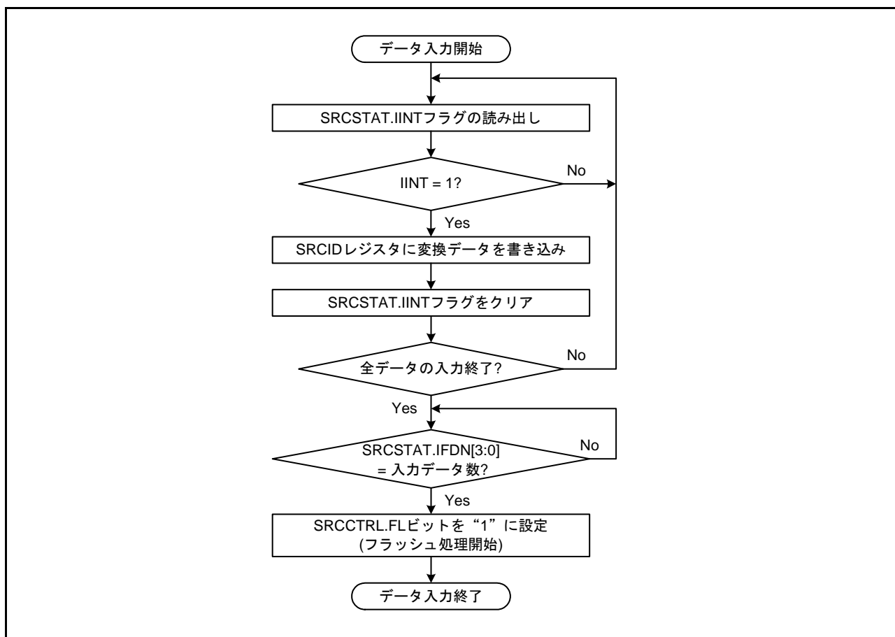
図 48.3 データ入力手順
