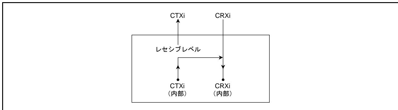
図 43.6 リッスンオンリモード選択時の接続 (i = 0 ~ 2)
