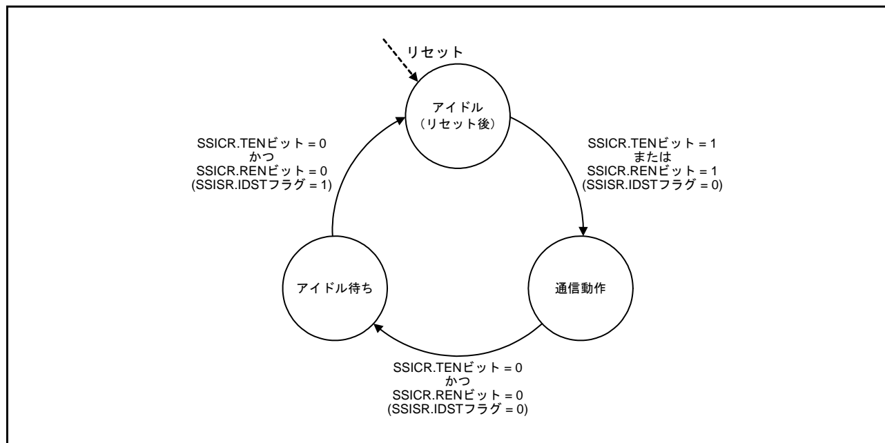
図 47.18 動作状態遷移図
