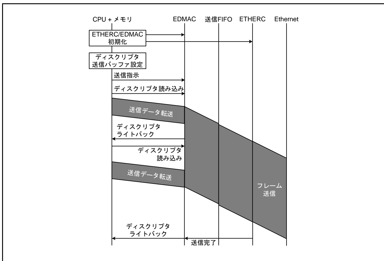
図 37.5 送信フローの例
