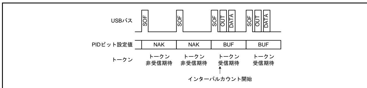
図 38.18 IITV[2:0] = 000b の場合のフレームとトークン受信期待有無の関係
