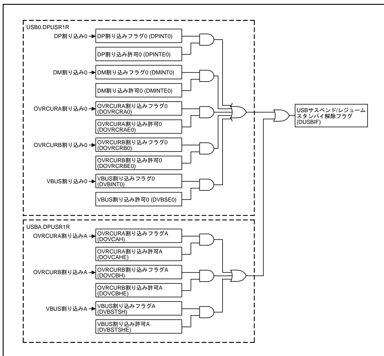
図 11.2 USB サスペンド/レジャーームディープスタンバイ解除フラグ (DUSBIF) の構成
