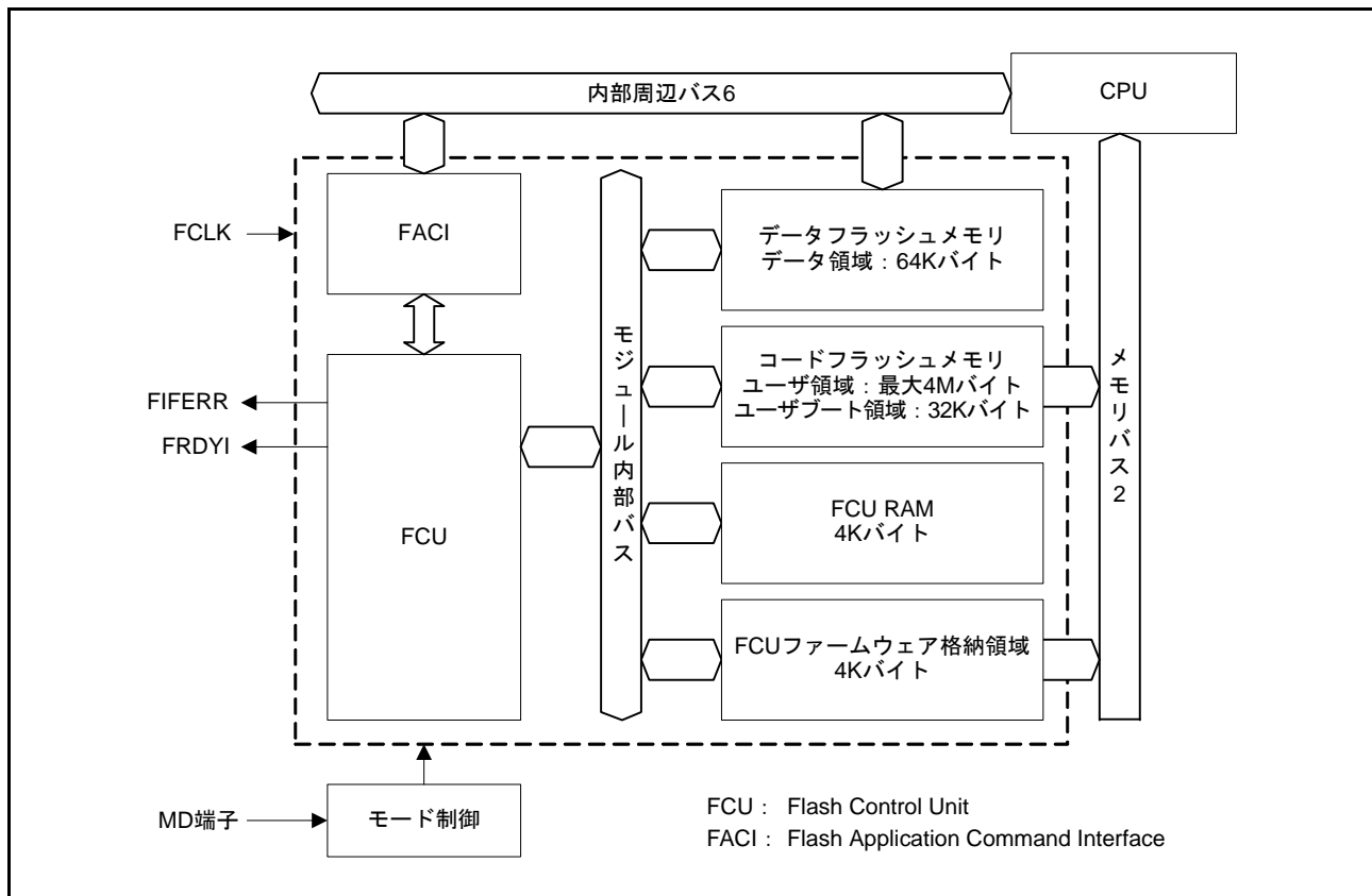
図 63.1 フラッシュメモリ関連のブロック図
