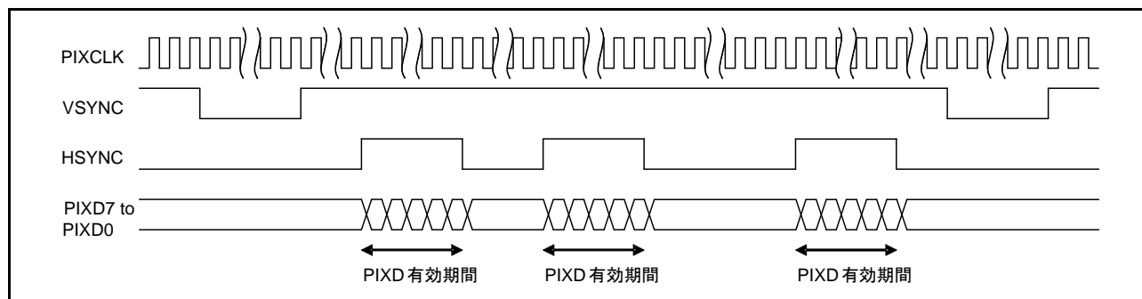
図 51.4 PDC 通信フォーマット (VPS = 0, HPS = 0)
