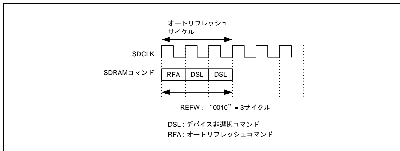
図 16.54 オートリフレッシュサイクルタイミング例 (1)
