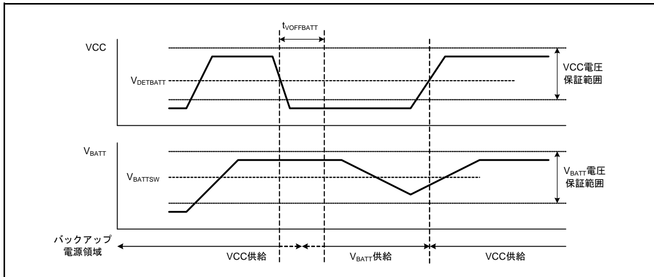
図 64.95 バッテリバックアップ機能特性
