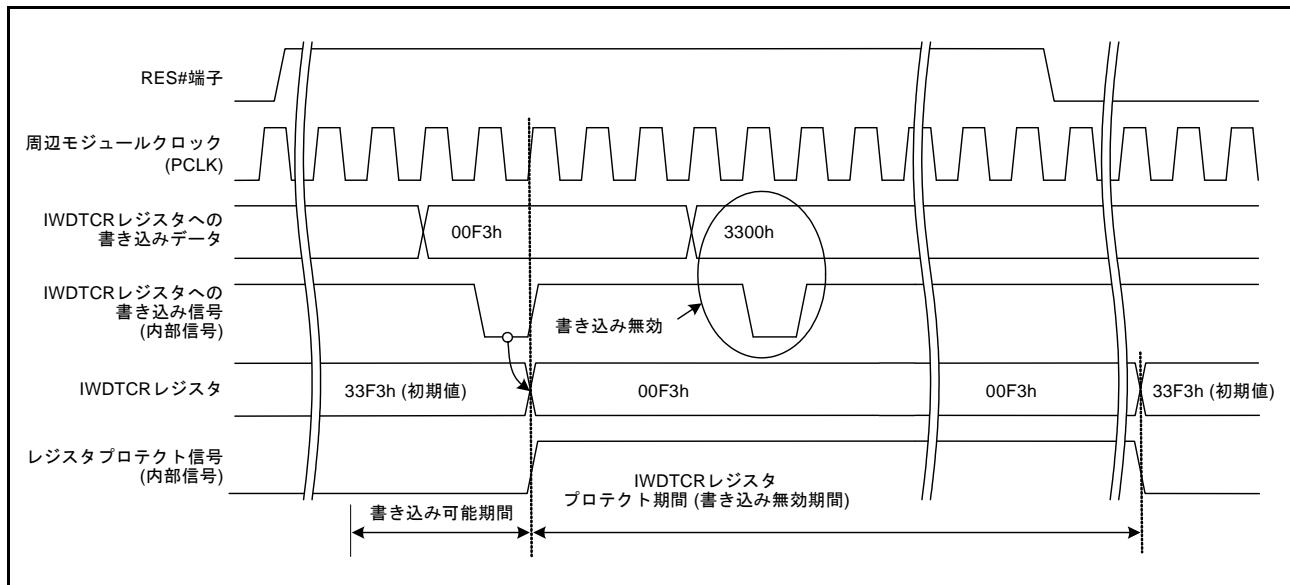
図 34.5 IWDTCR レジスタ書き込み制御波形
