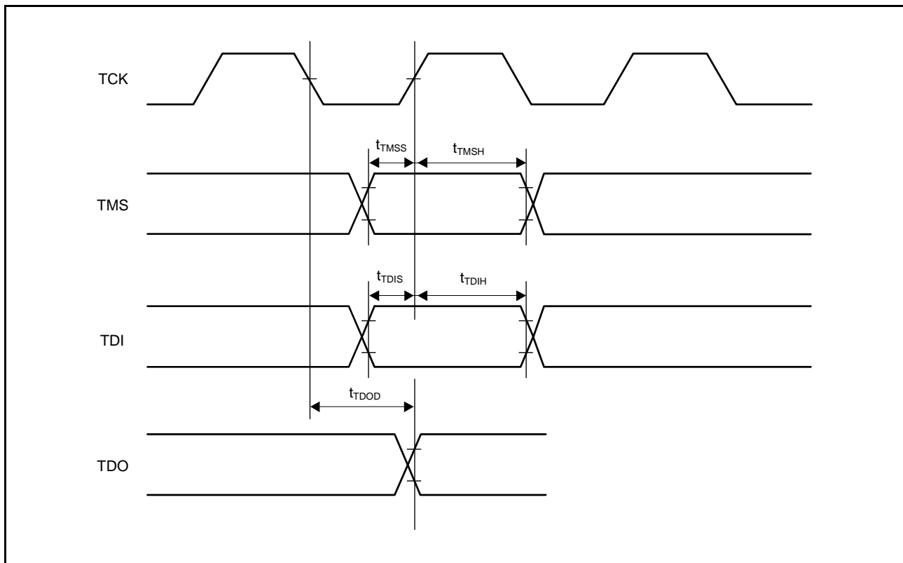
図 64.99 バウンダリスキャン入出力タイミング
