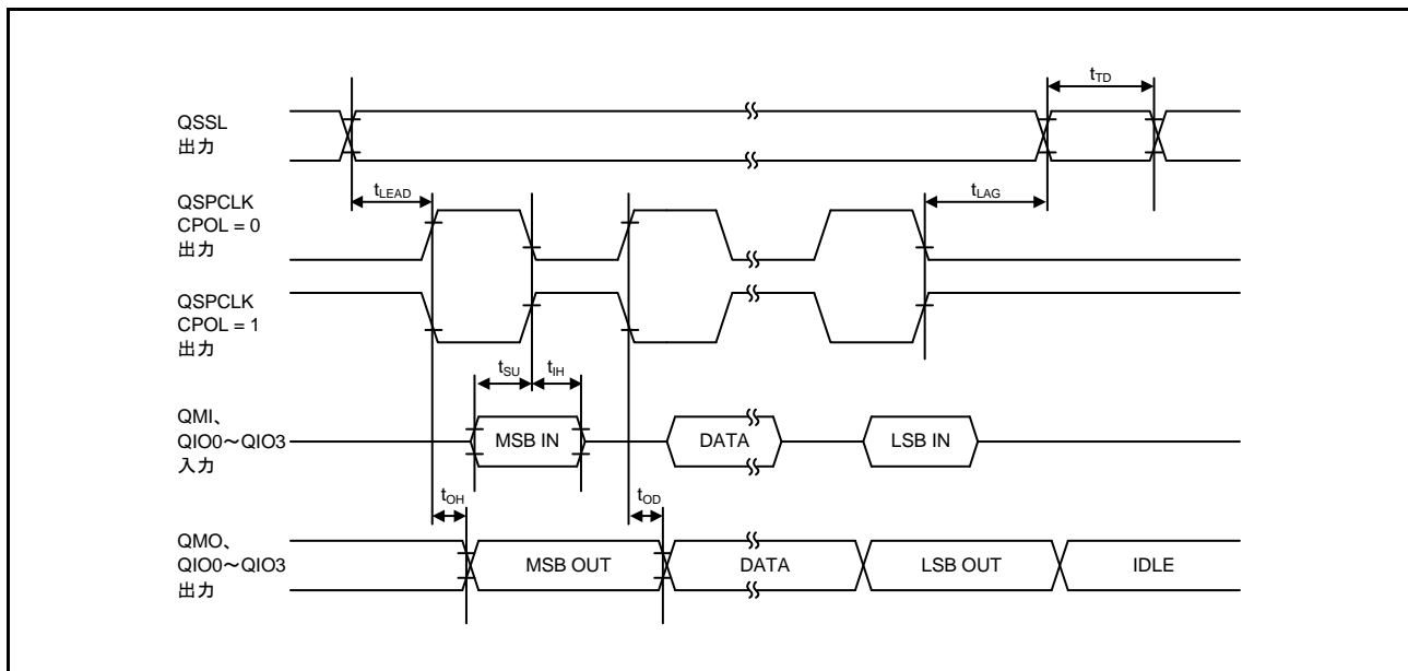
図 64.65 送受信タイミング (CPHA = 1)
