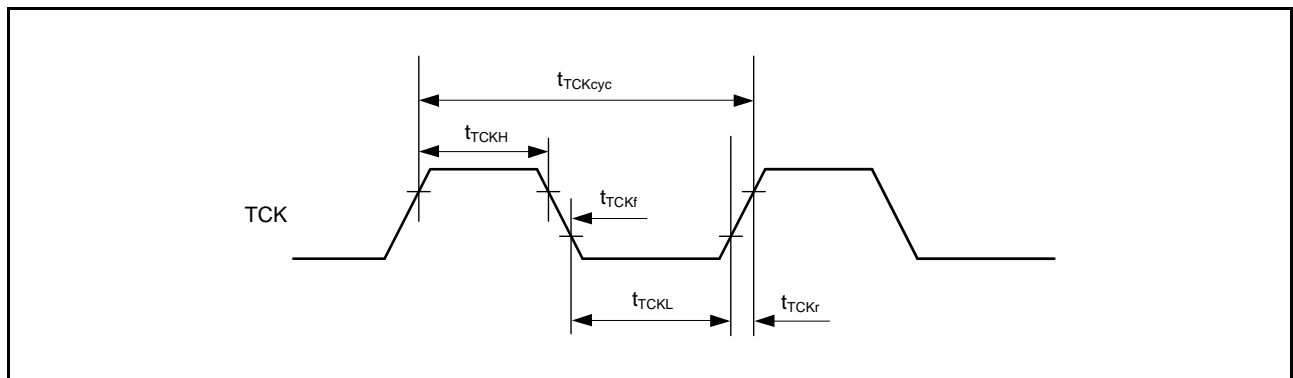
図 64.97 バウンダリスキャン TCK タイミング
