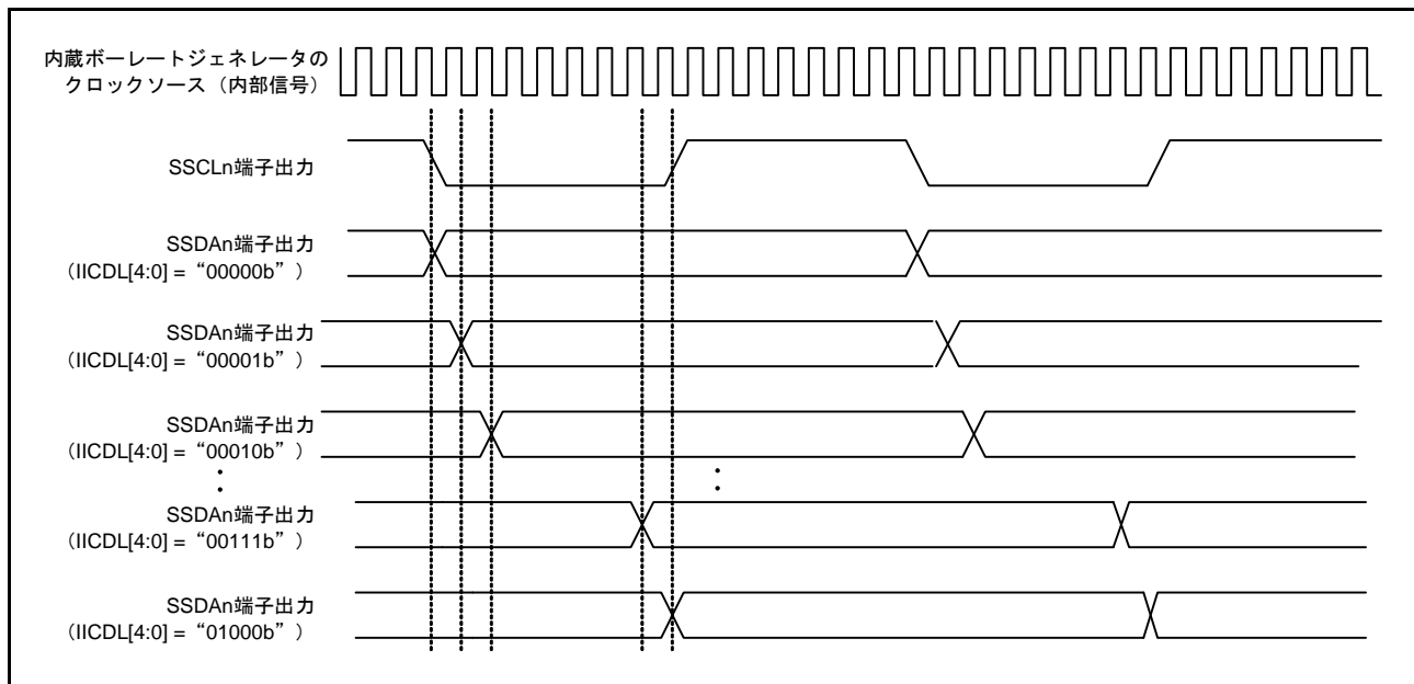
図 40.50 SSDA 出力遅延のタイミング
