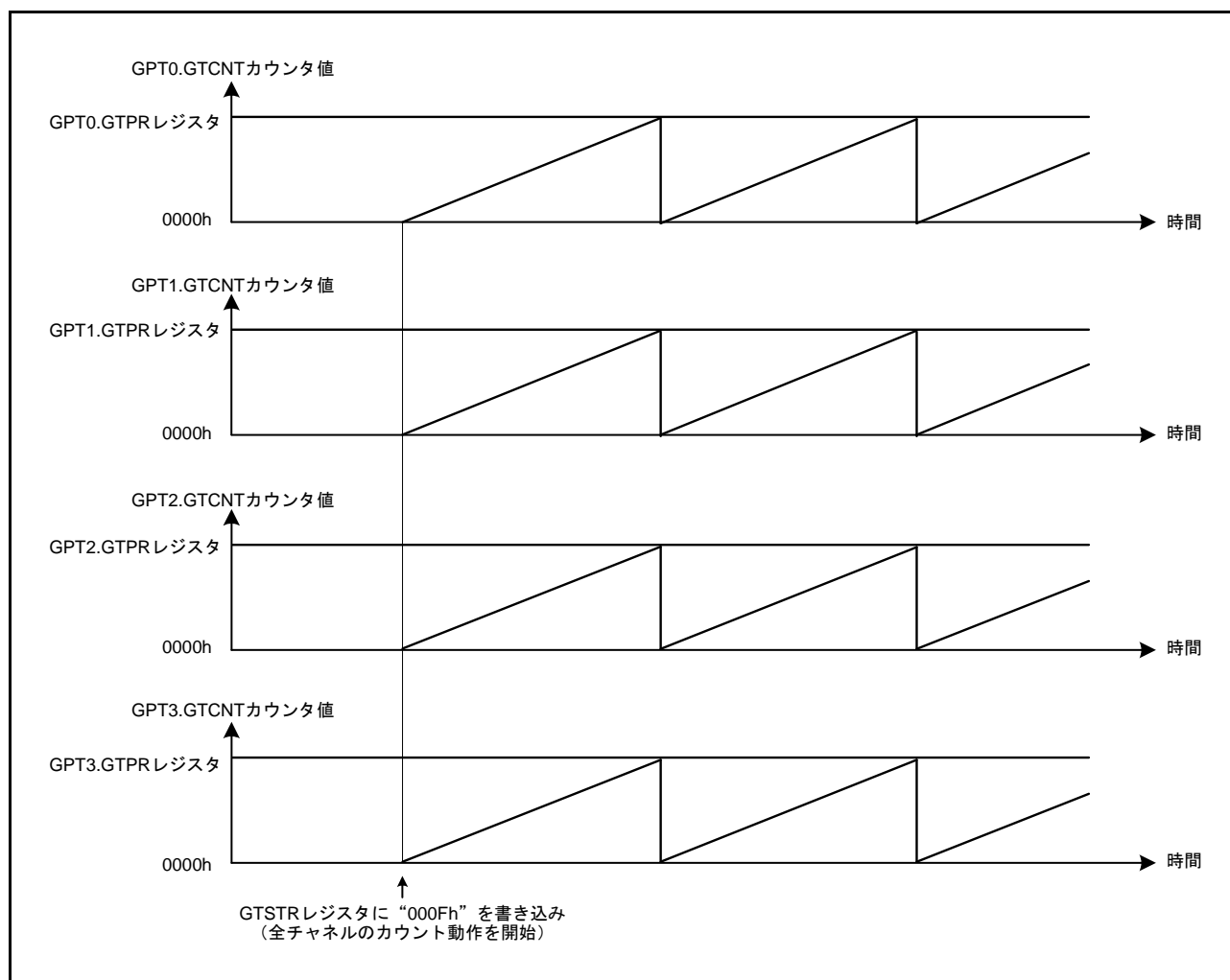
図 26.57 ソフトウェアによる同時スタート動作例 (カウンタ周期 (GTPR レジスタ値) が同一のとき)
