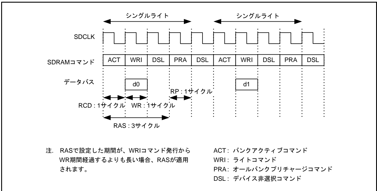
図 16.76 シングルライトタイミング例 (4)
