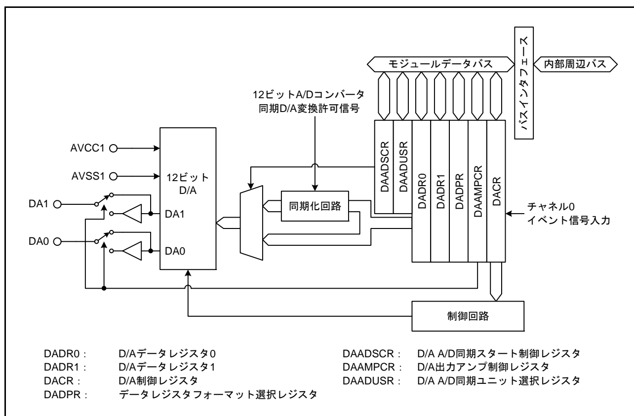
図58.1 12ビットD/Aコンバータのブロック図
