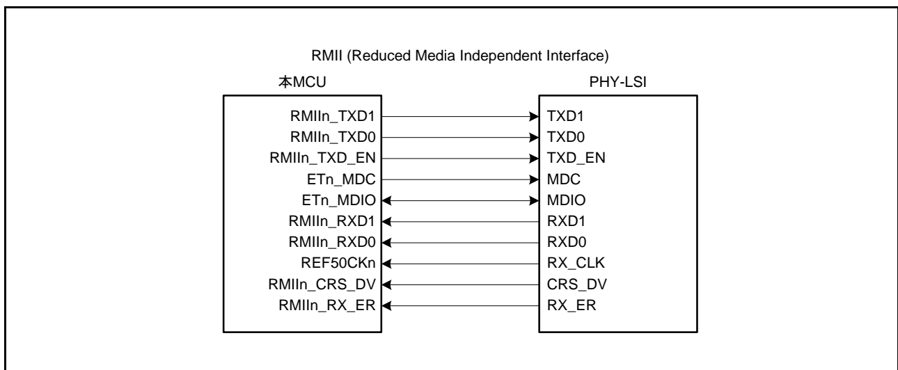
図 35.3 PHY-LSI との接続例 (RMII)
