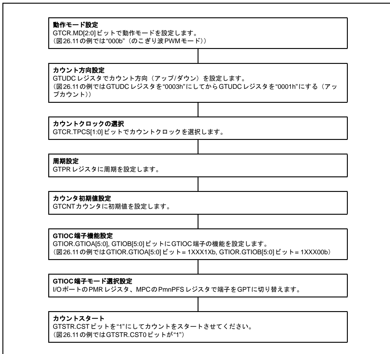
図 26.12 インプットキャプチャ動作設定例
