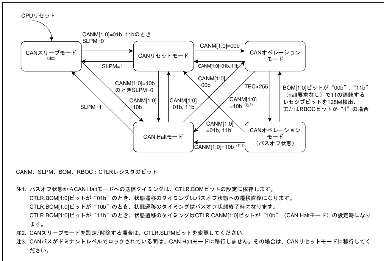
図 43.9 CAN 動作モード間の移行
