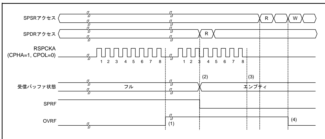
図 44.27 SPRF フラグと OVRF フラグの動作例
