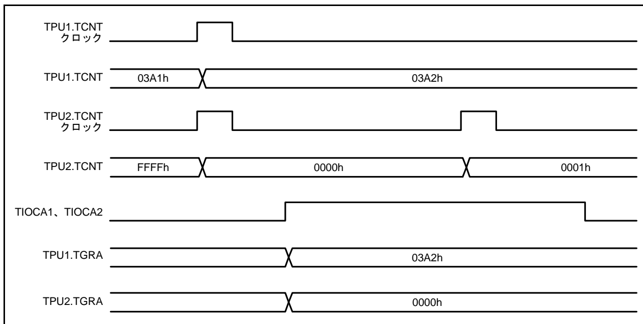
図 27.18 カスケード接続動作例 (1)
