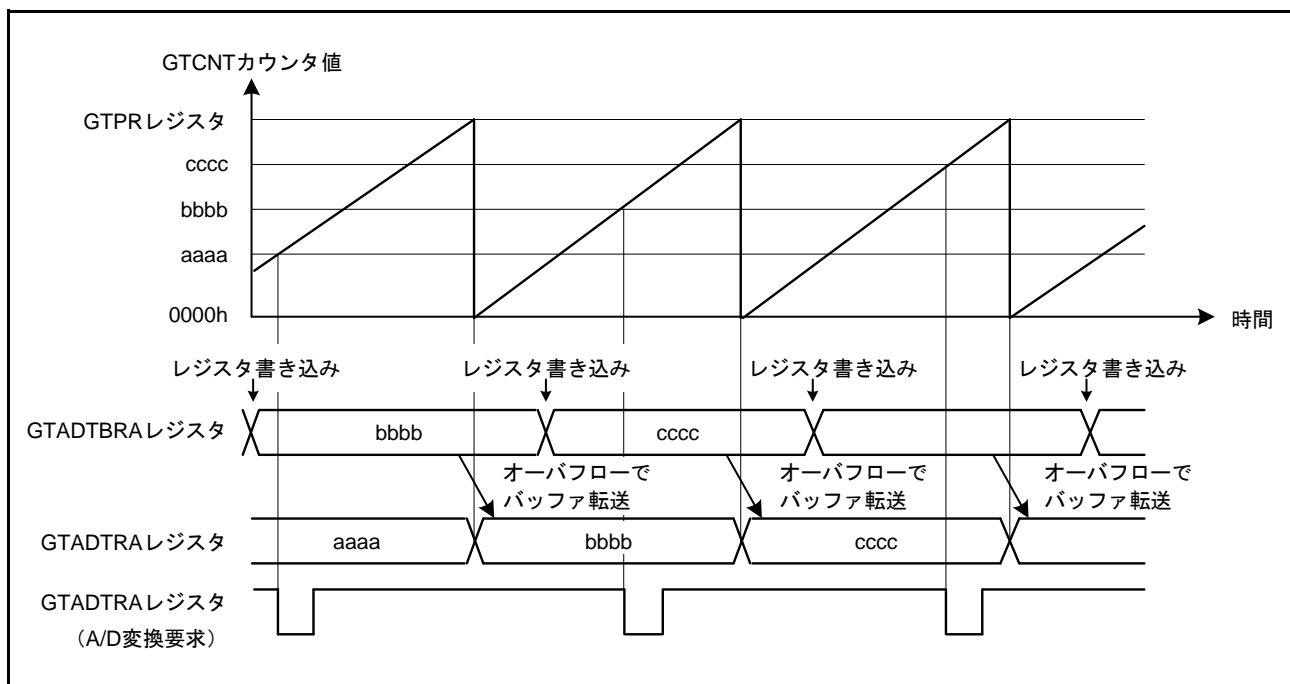
図 26.23 GTADTRA, GTADTRB レジスタのバッファ動作例 (のこぎり波でアップカウント、アップカウントで A/D 変換要求発生の場合)
