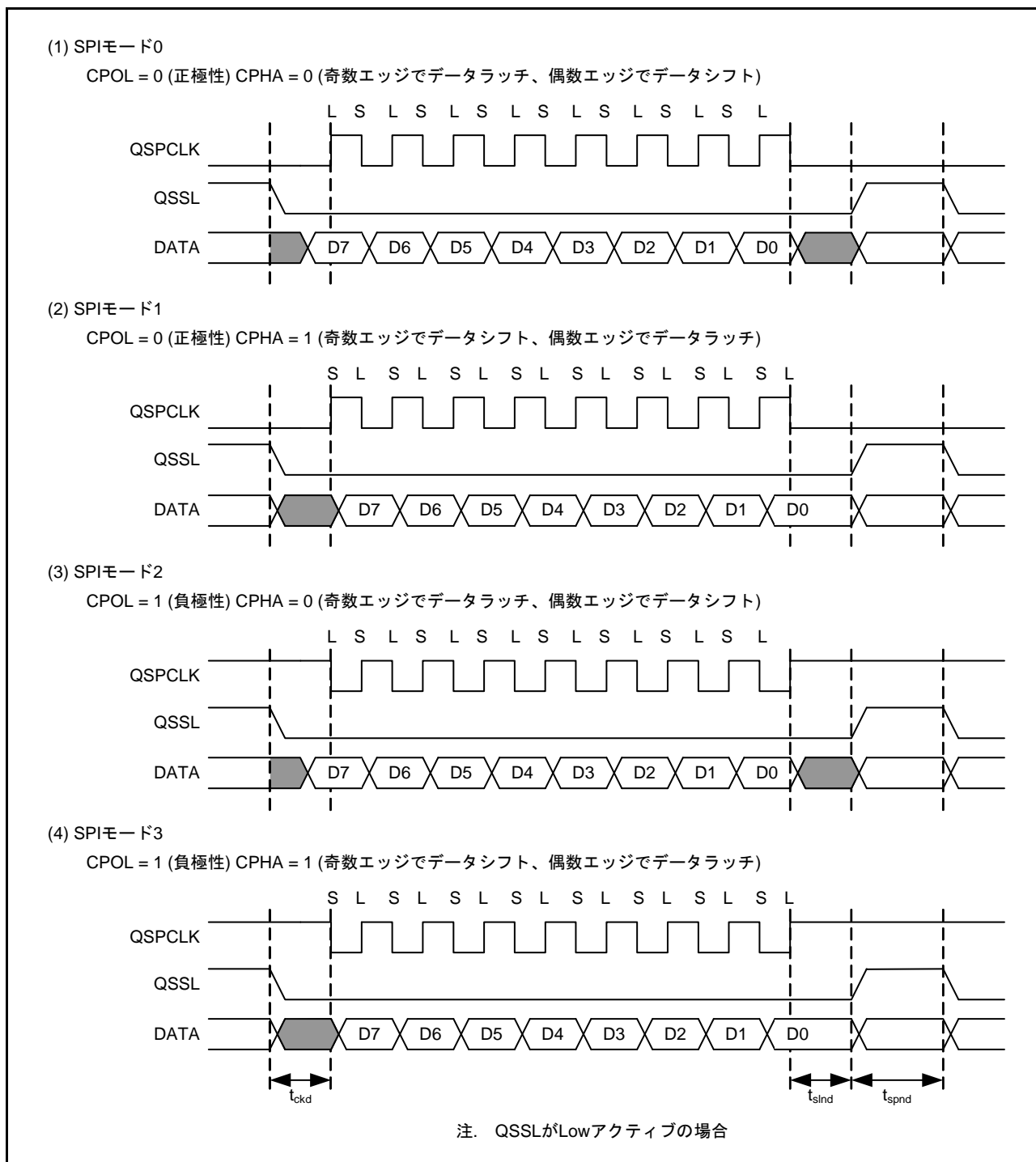
図45.2 クロック設定と転送タイミング
