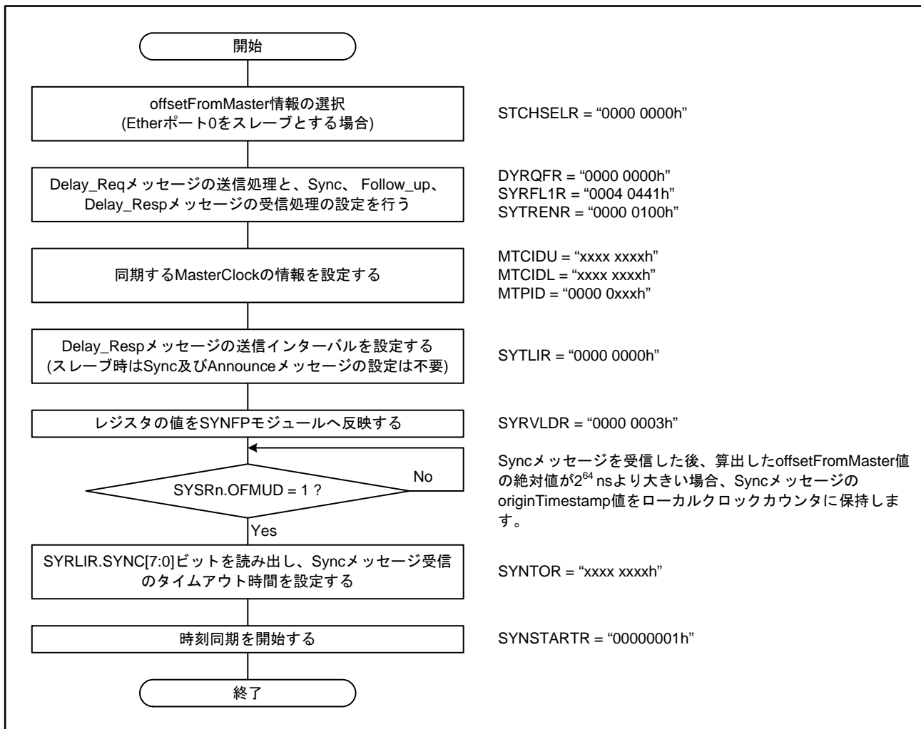
図36.13 E2Eスレーブ動作の開始手順
