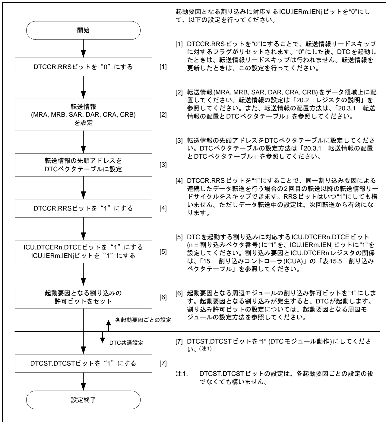
図 20.14 DTC の設定手順
