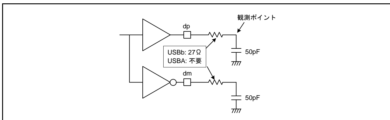
図 64.89 測定回路 (フルスピード時)
