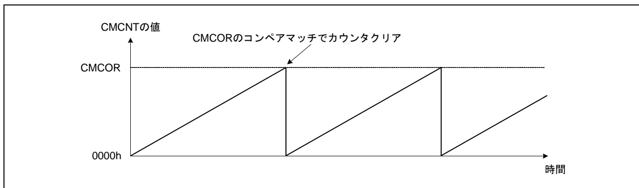
図 30.2 CMCNT カウンタの動作
