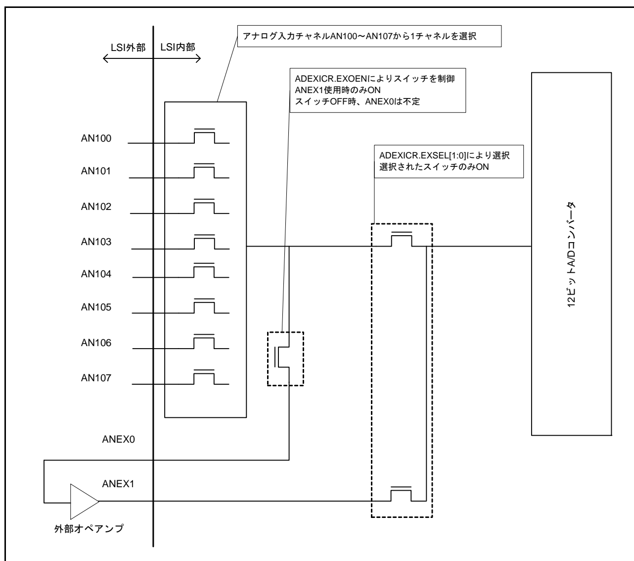
図 57.32 ANEX1 使用時の拡張アナログ入力構成例
