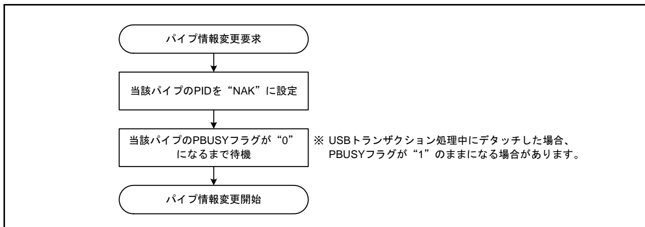
図 39.11 USB 通信許可 (PID[1:0] ビットが “01b” (BUF 応答)) 状態からのパイプ情報変更手順
