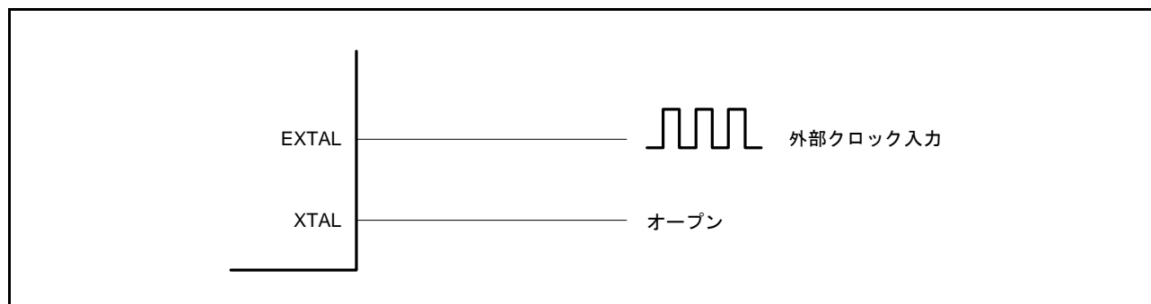
図 9.4 外部クロックの接続例
