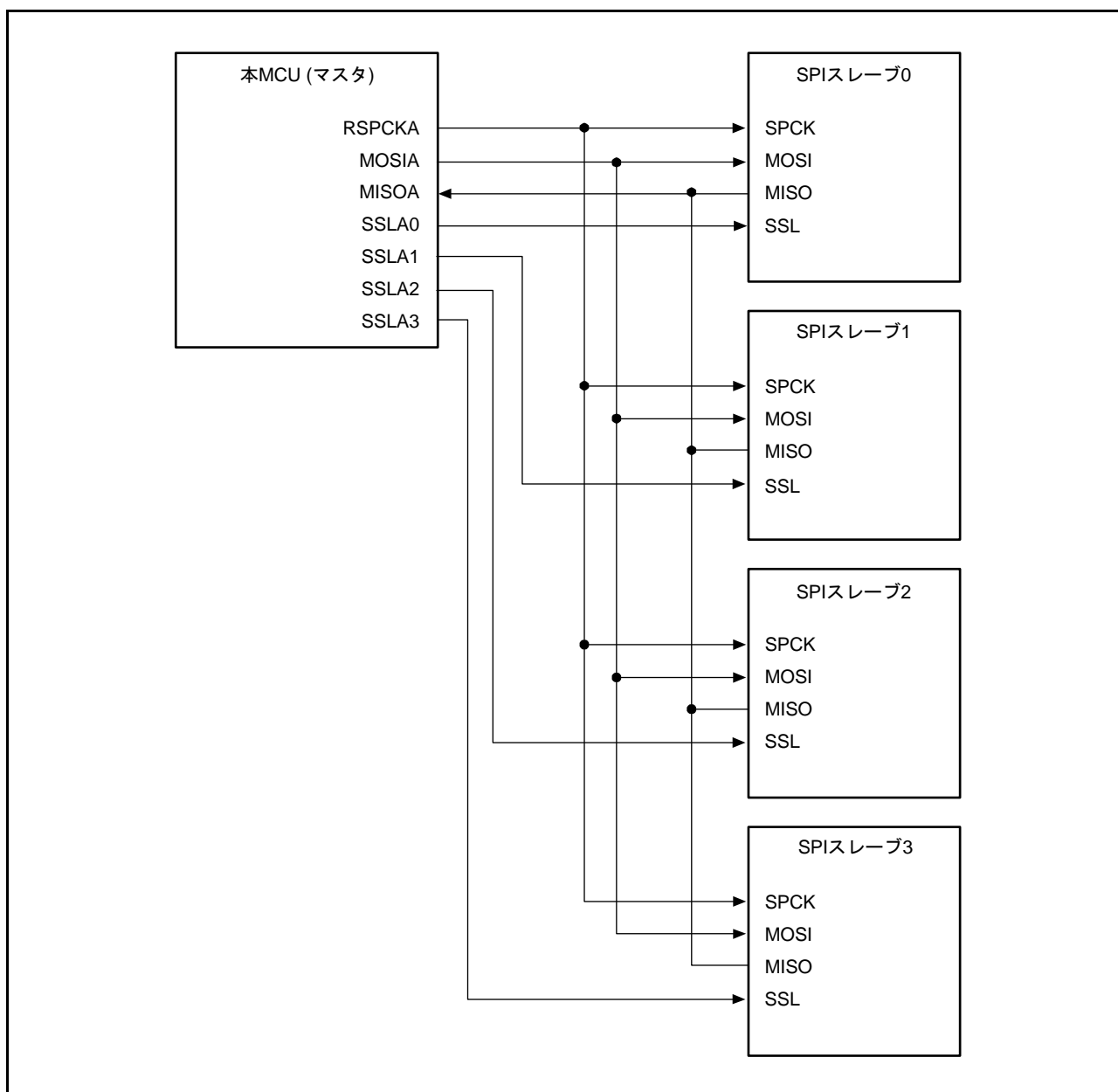
図 44.8 シングルマスタ / マルチスレーブの構成例 (本 MCU = マスタ)
