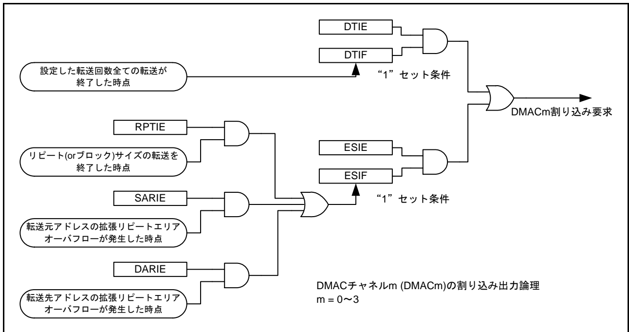
図 18.13 割り込み出力の概略論理図 (DMAC0～DMAC3)
