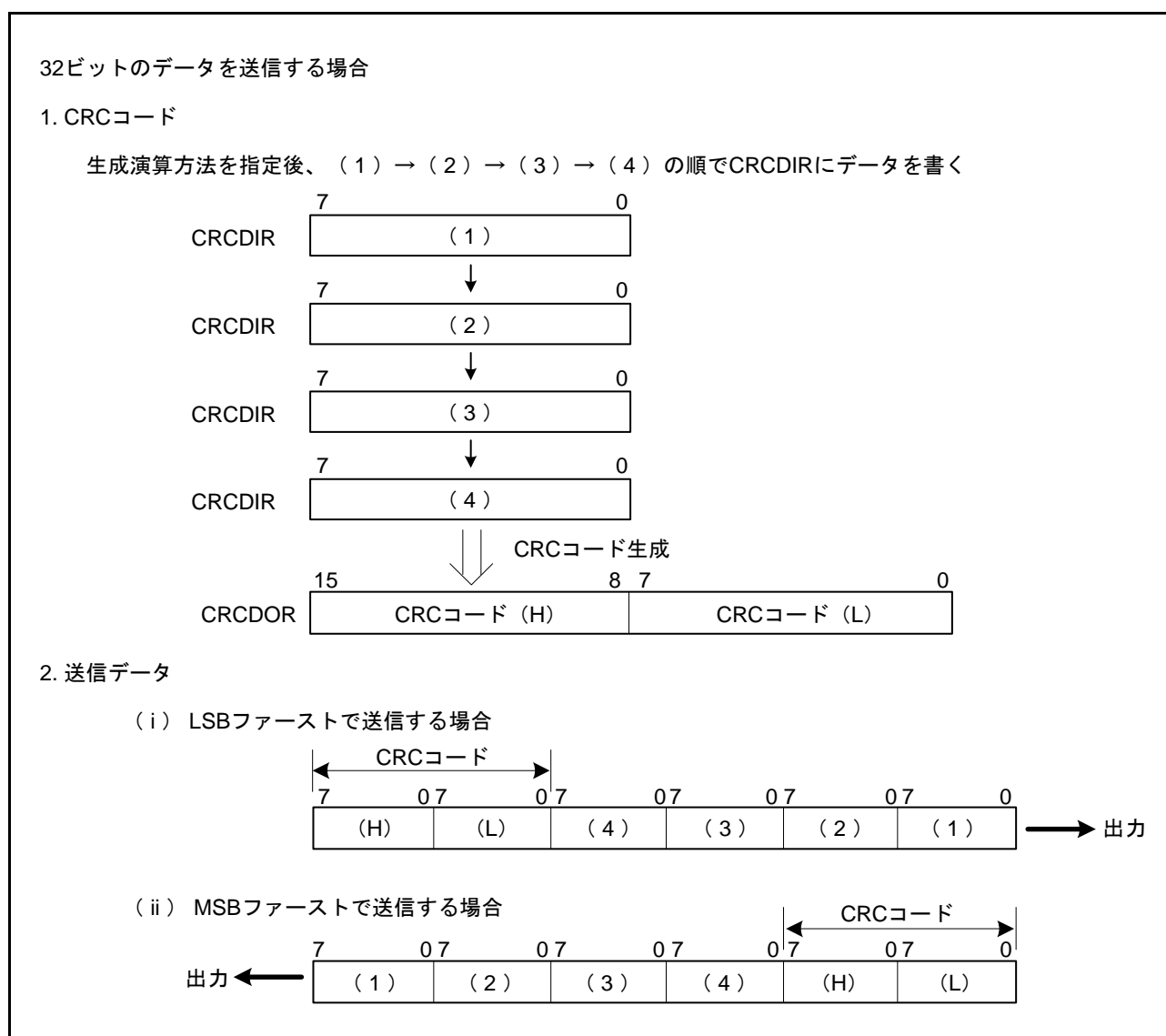
図 46.6 LSB ファーストと MSB ファーストの送信データ
