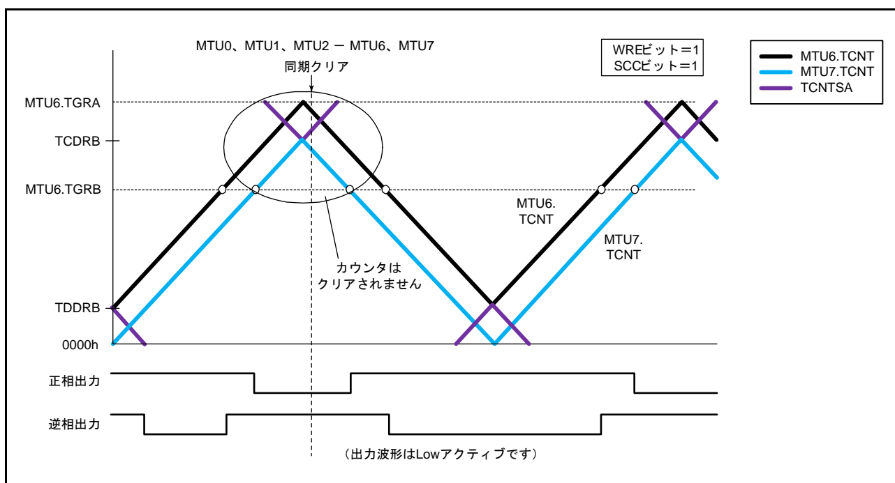
図 24.75 Tb1 区間で同期クリアが発生した場合 (図 24.66 のタイミング⑥、MTU6、MTU7 の TWCRB レジスタの WRE ビット = 1、SCC ビット = 1)
