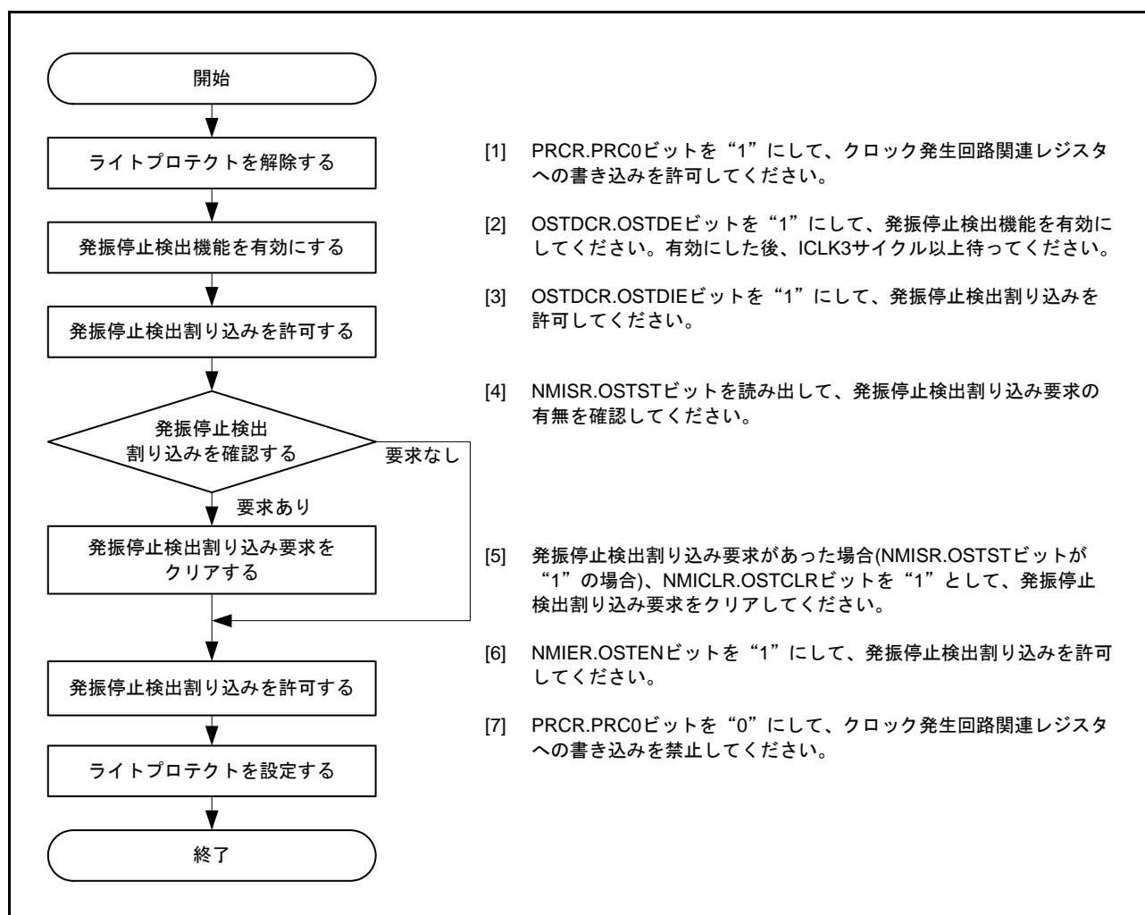
図 9.8 発振停止検出機能の初期化手順のフローチャート例
