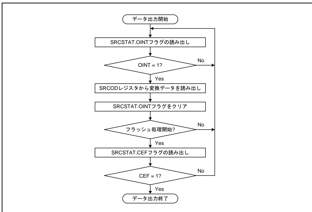
図 48.4 データ出力手順
