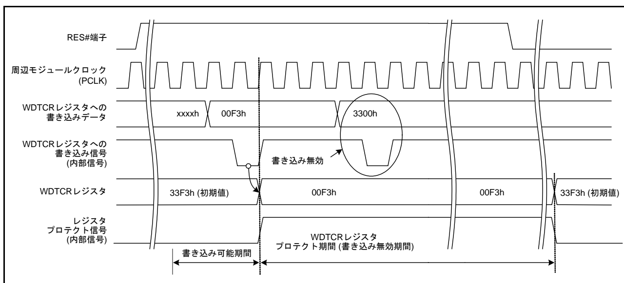
図 33.5 WDTCR レジスタ書き込み制御波形
