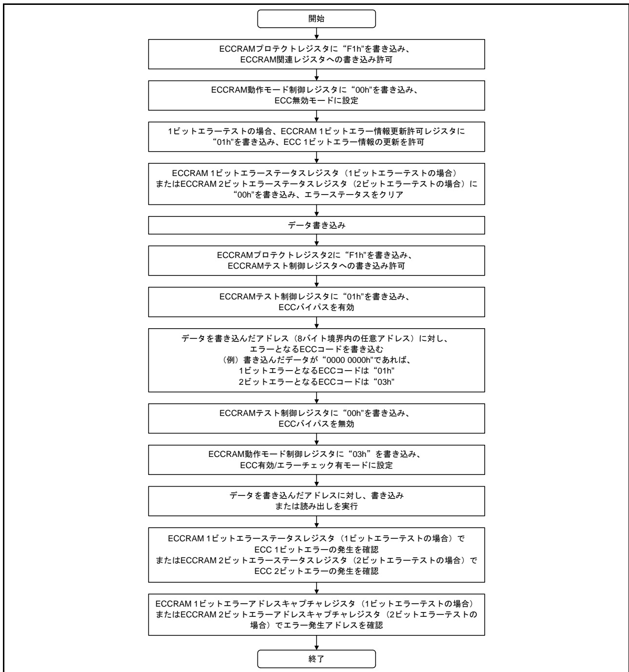
図 61.1 ECC コード制御回路テストフロー
