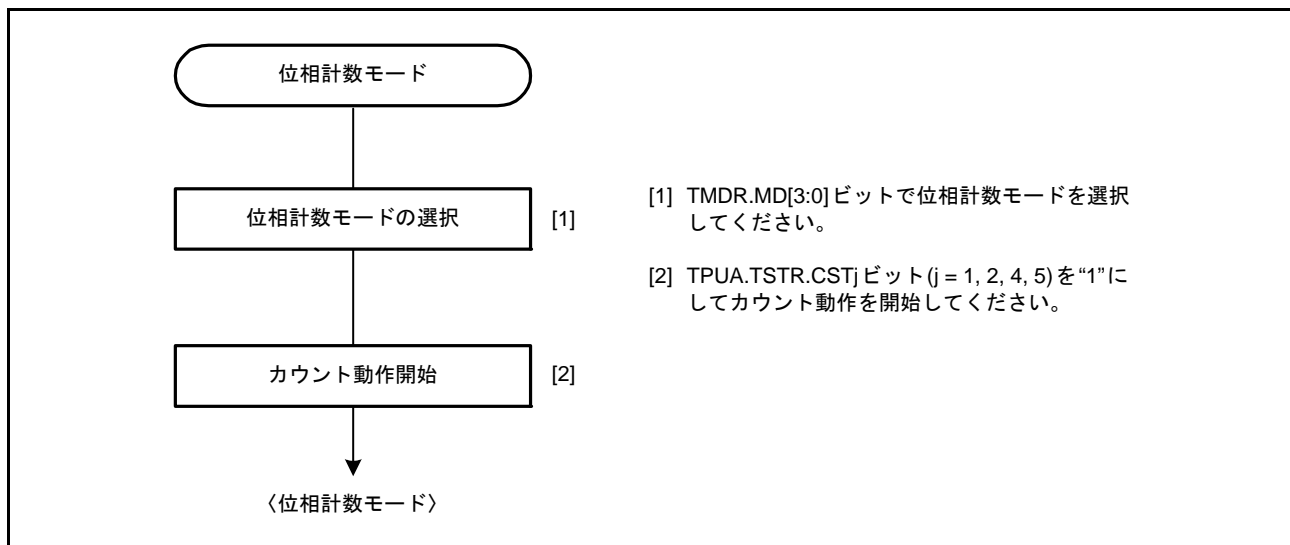
図27.24 位相計数モードの設定手順例
