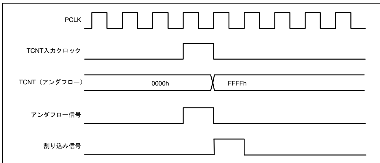
図 27.42 TCImU 割り込みのセットタイミング
