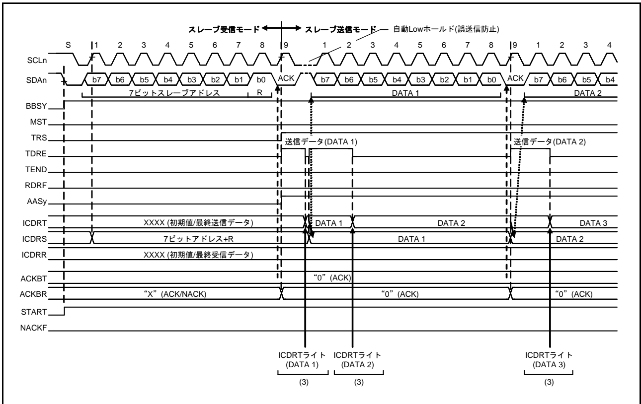
図 42.15 スレーブ送信の動作タイミング (1) (7 ビットアドレスフォーマットの時)
