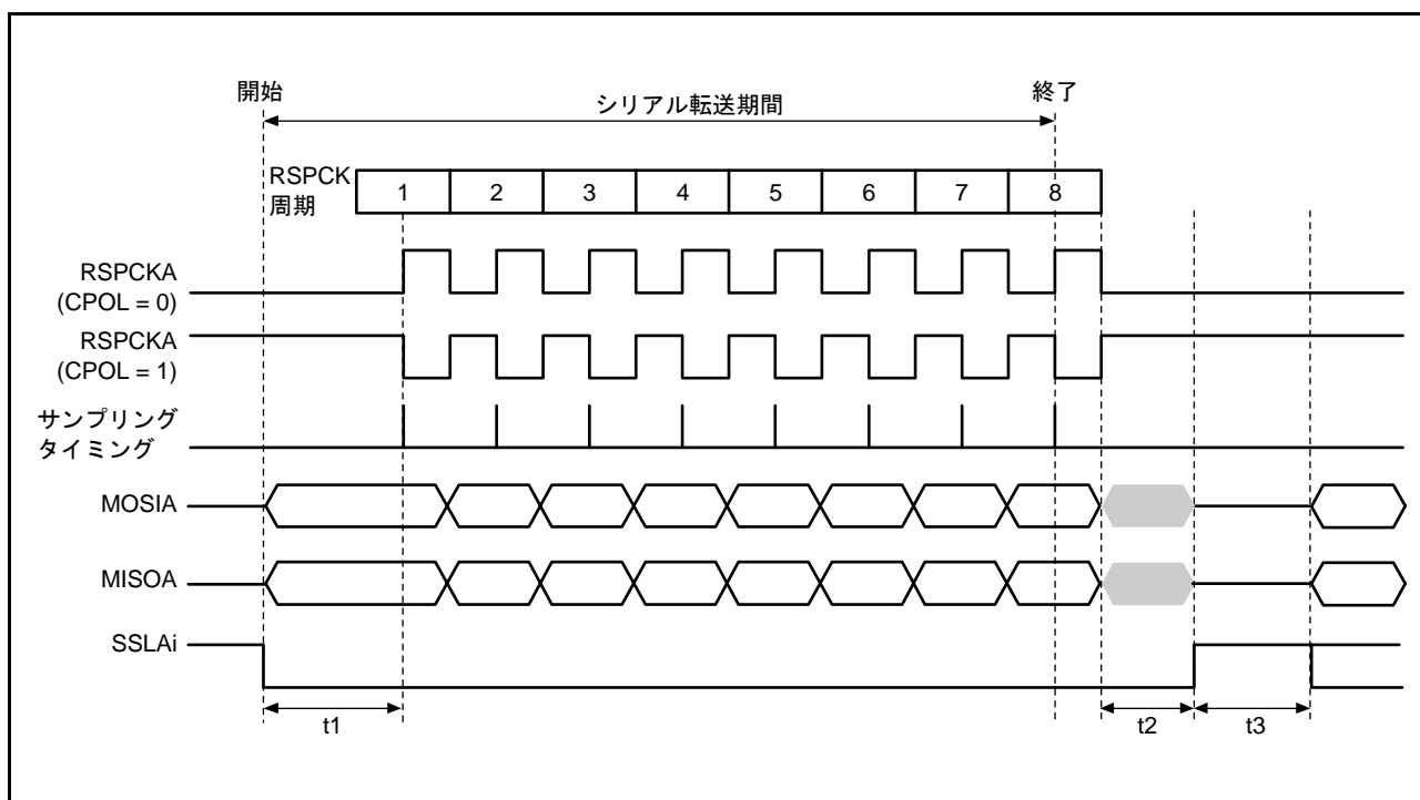
図 44.22 RSPI 転送フォーマット (CPHA ビット = 0)
