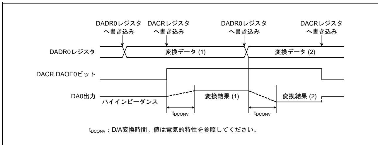
図 58.2 12ビットD/Aコンバータの動作例
