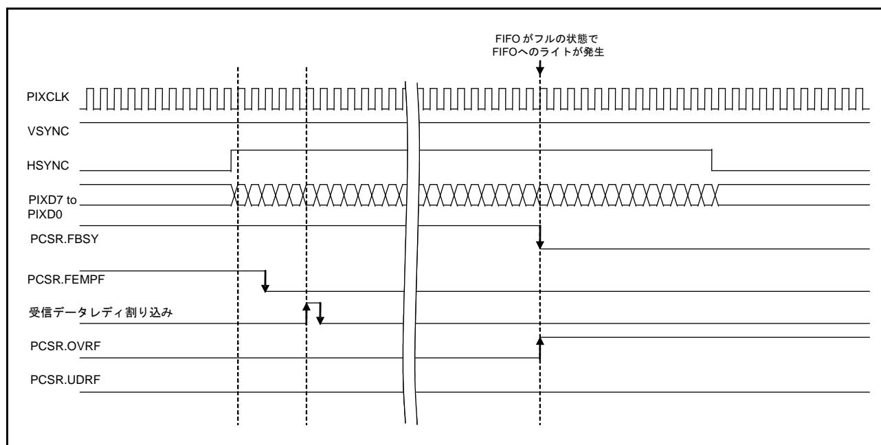
図 51.14 オーバラン
