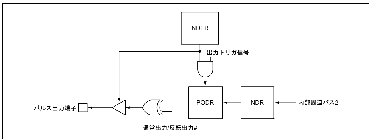
図 28.4 PPG 概要図
