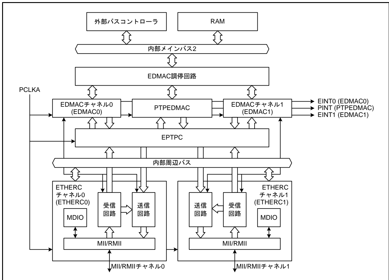
図 35.1 ETHERC の構成
