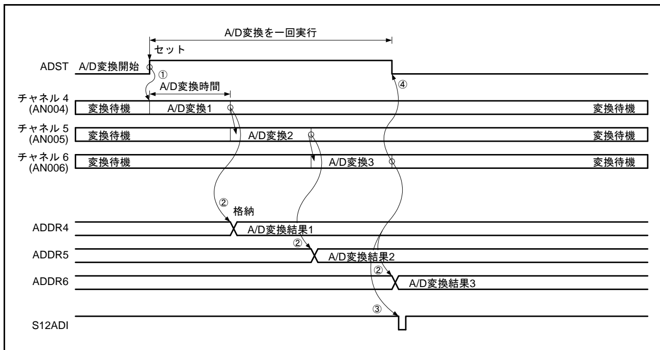
図 57.4 シングルスキャンモードの動作例 (基本動作 : AN004 ~ AN006 選択)
