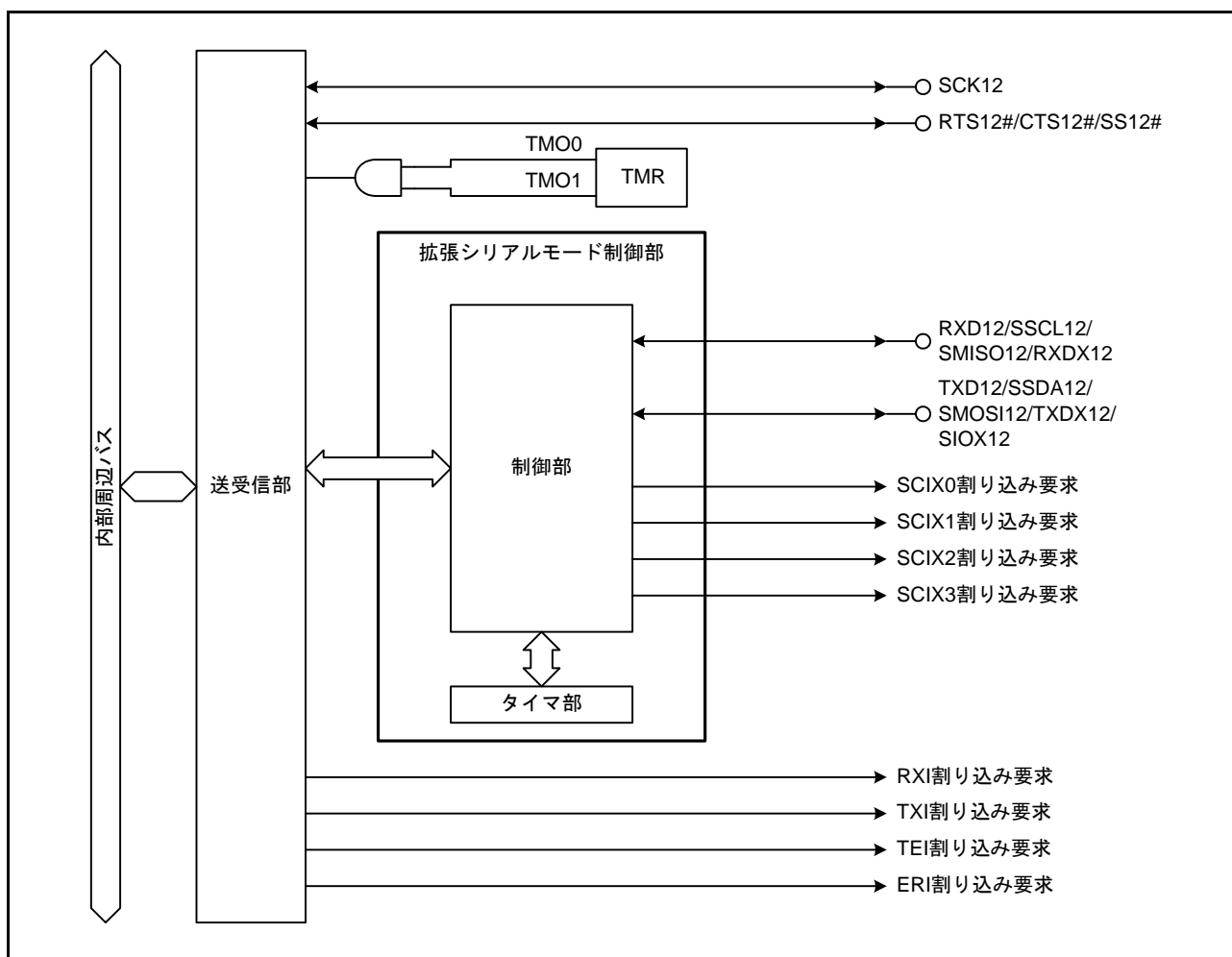
図 40.3 SCIh (SCI12) のブロック図
