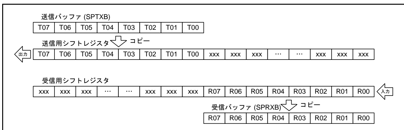
図 45.8 MSB ファースト転送 (8 ビットデータ)
