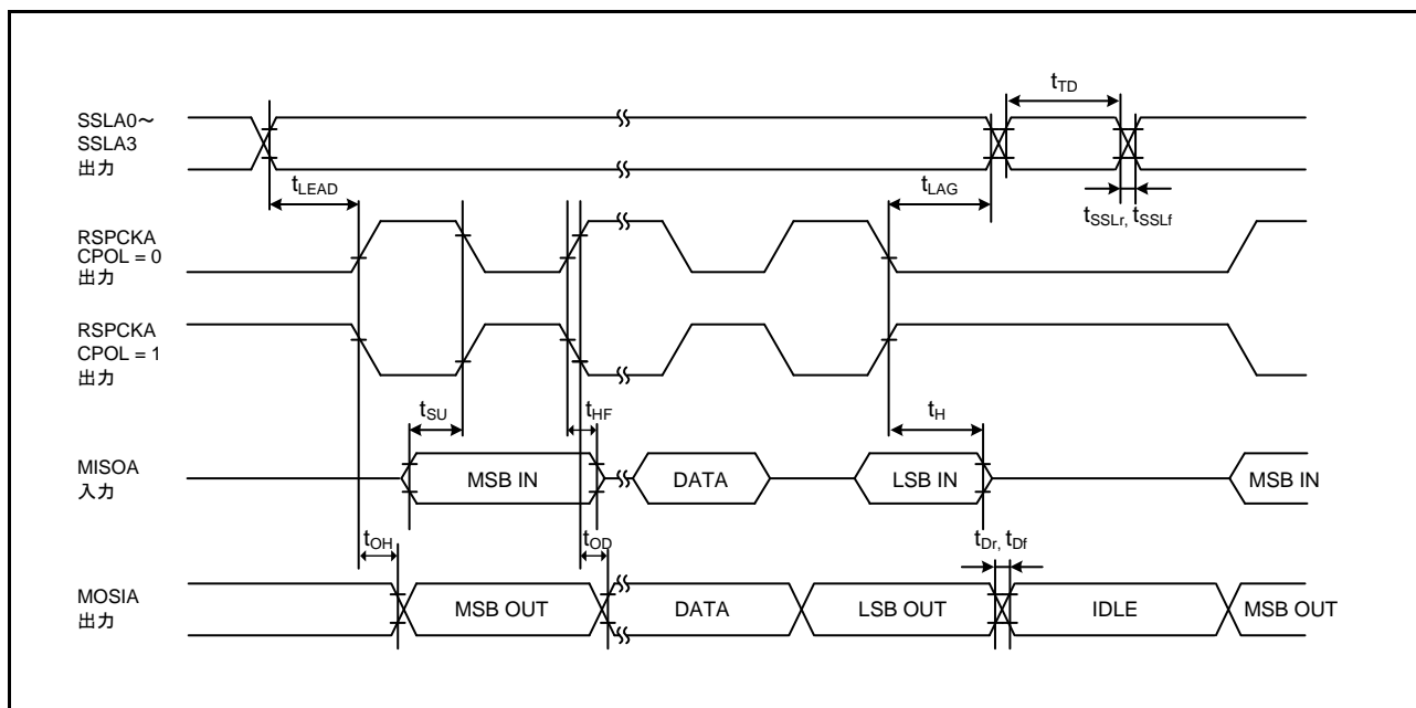
図 64.60 RSPI タイミング (マスタ、CPHA = 1) (ビットレート : PCLKB を 2 分周に設定)
