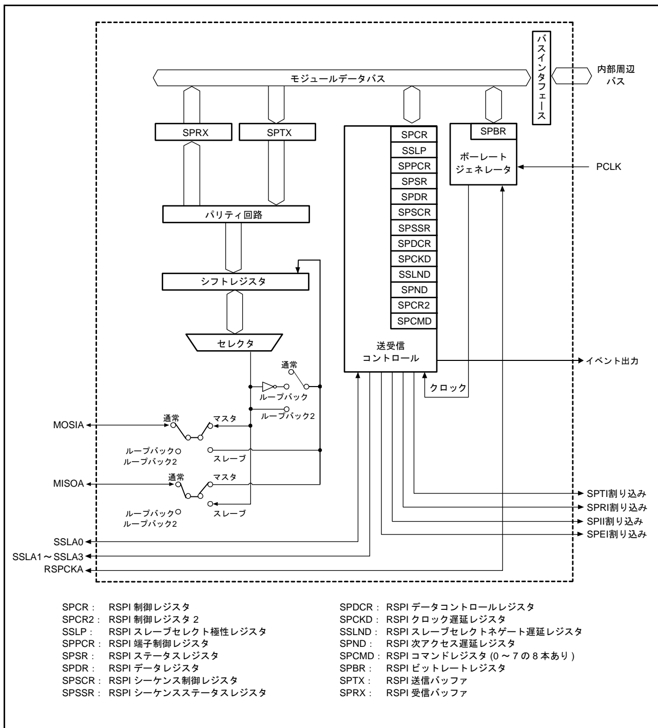
図 44.1 RSPI のブロック図
