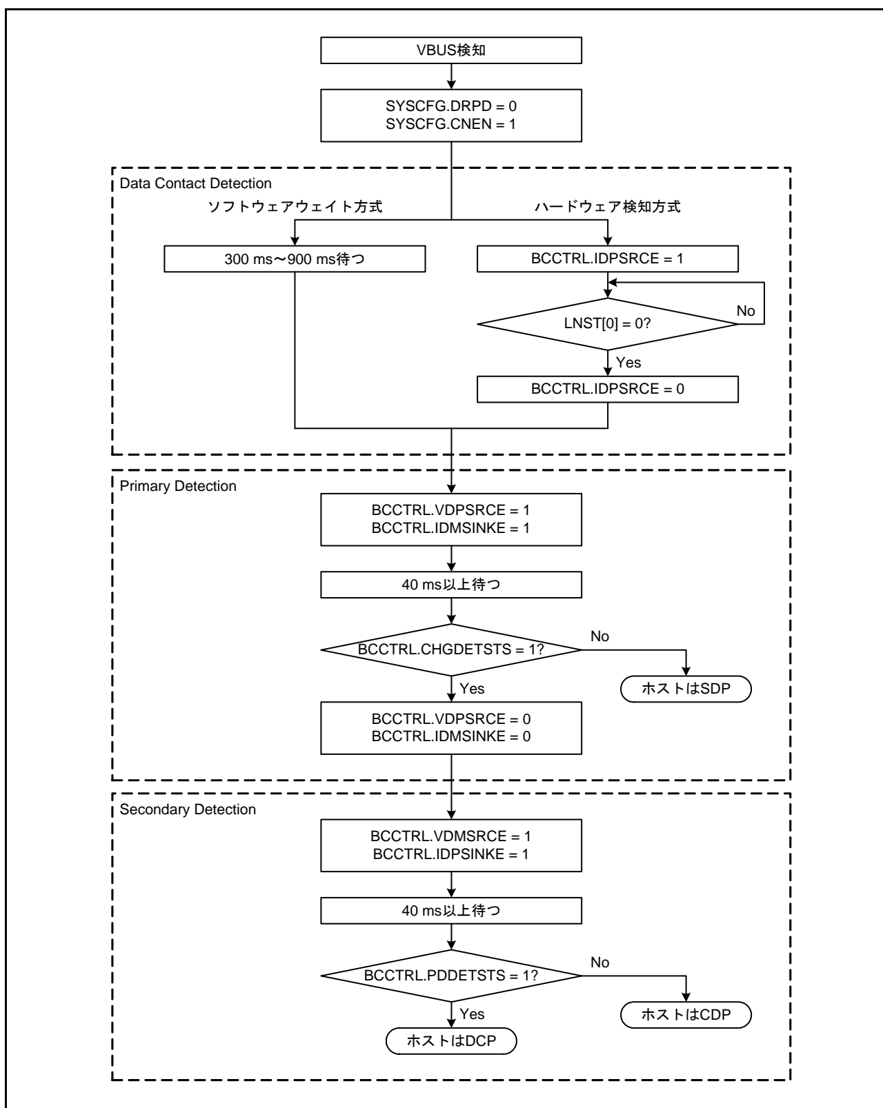
図 39.20 Portable Device としての処理フロー
