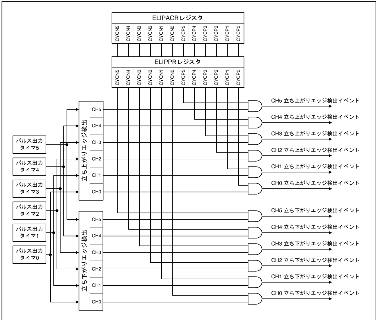
図36.38 パルス出力タイマとELCの関係
