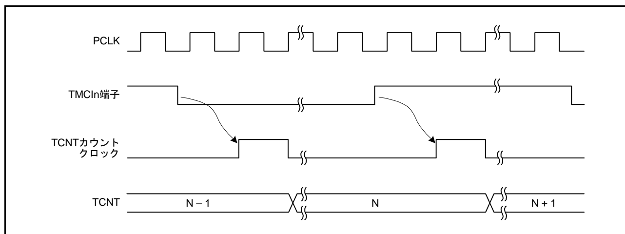
図 29.6 外部クロック動作時のカウンタタイミング (両エッジの場合)
