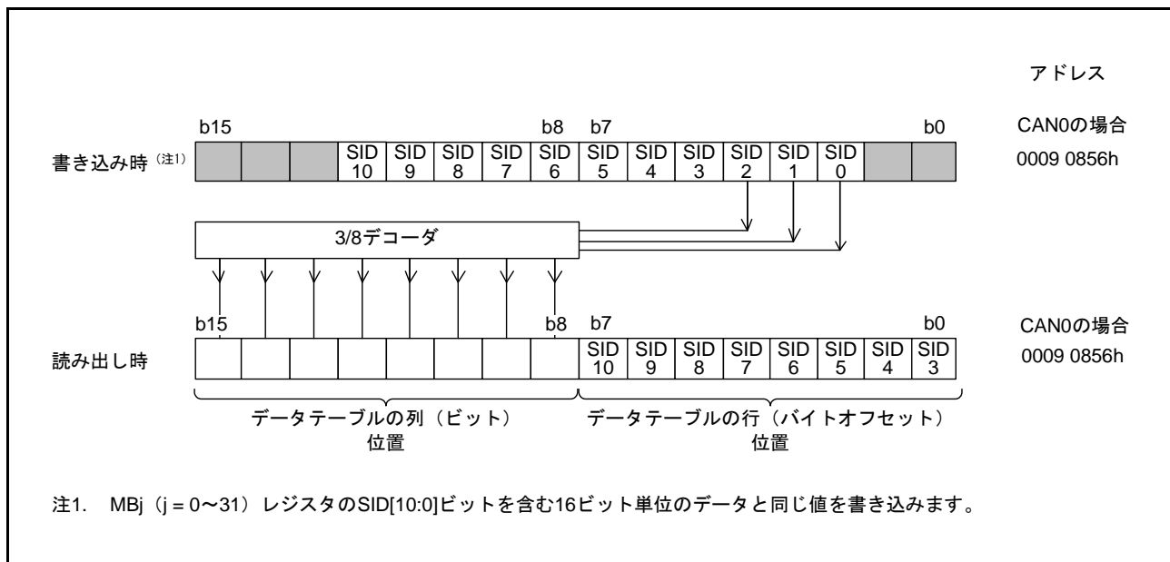
図 43.5 AFSR レジスタの書き込み、読み出し
