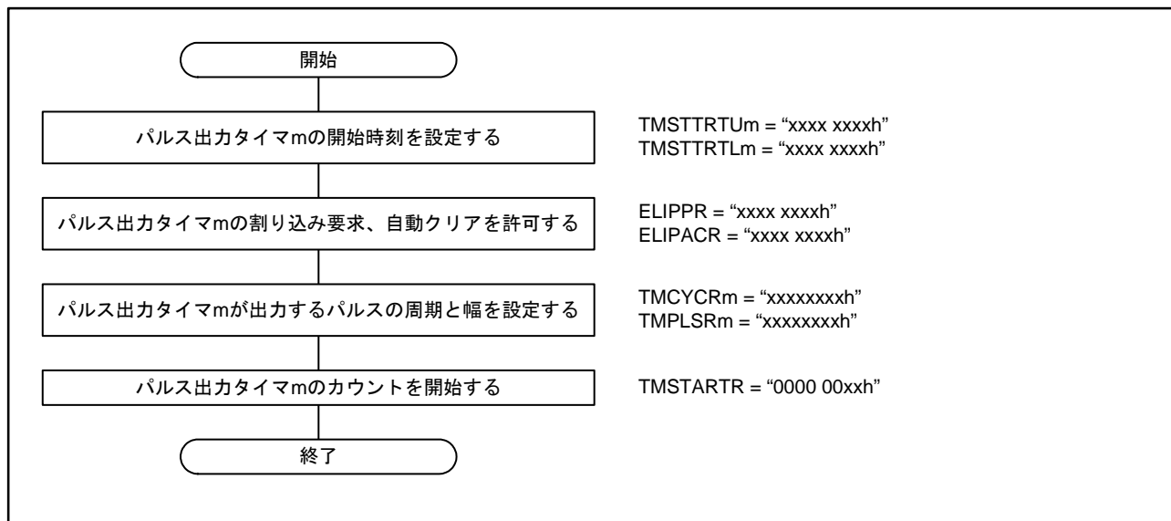
図36.33 パルス出カタイマ設定手順
