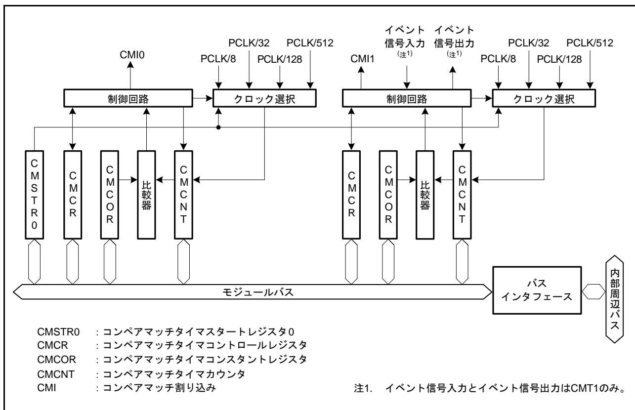
図 30.1 CMT (ユニット 0) のブロック図
