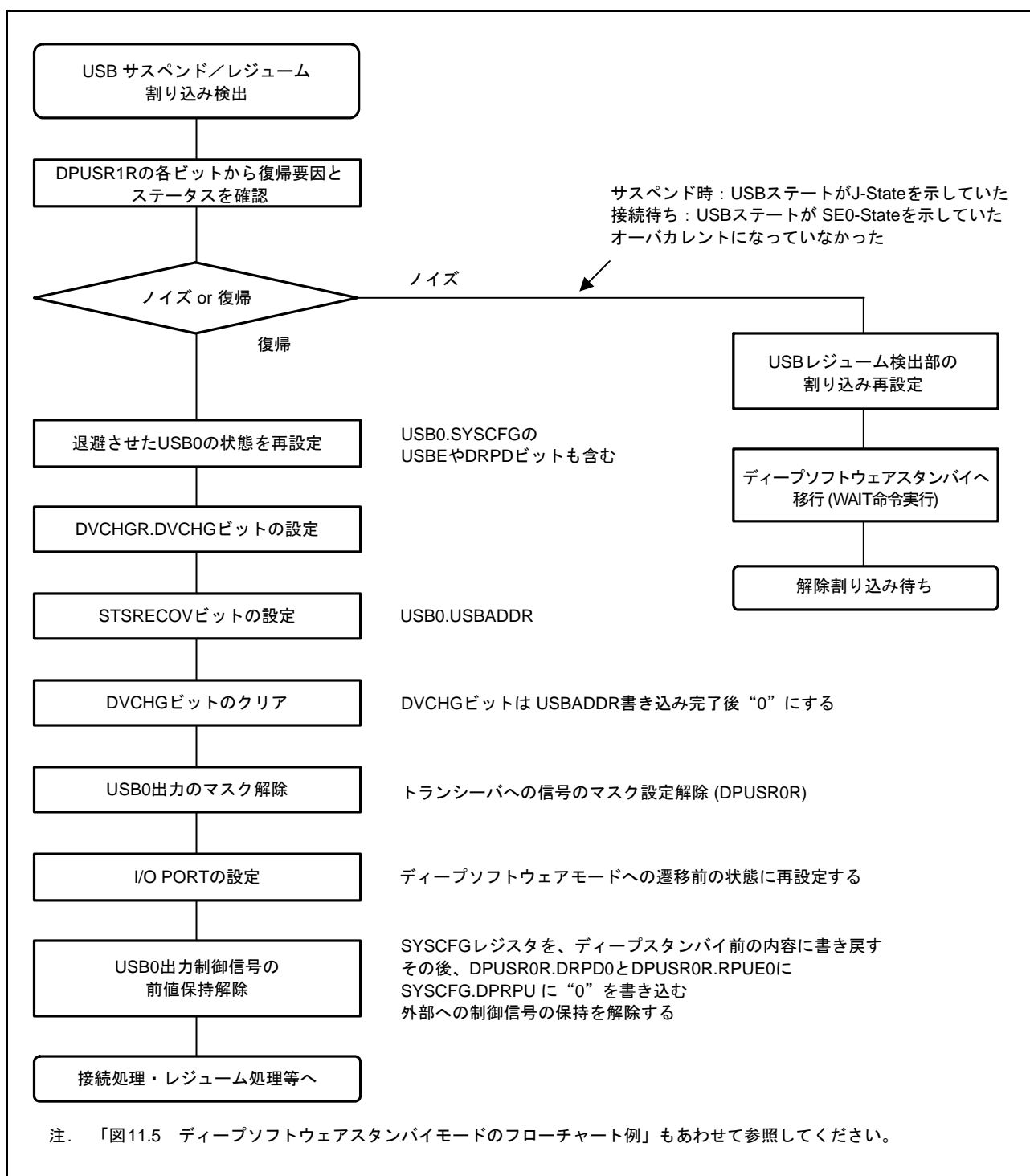
図 38.8 ホスト時のディープソフトウェアスタンバイ解除時の USB 設定フロー
