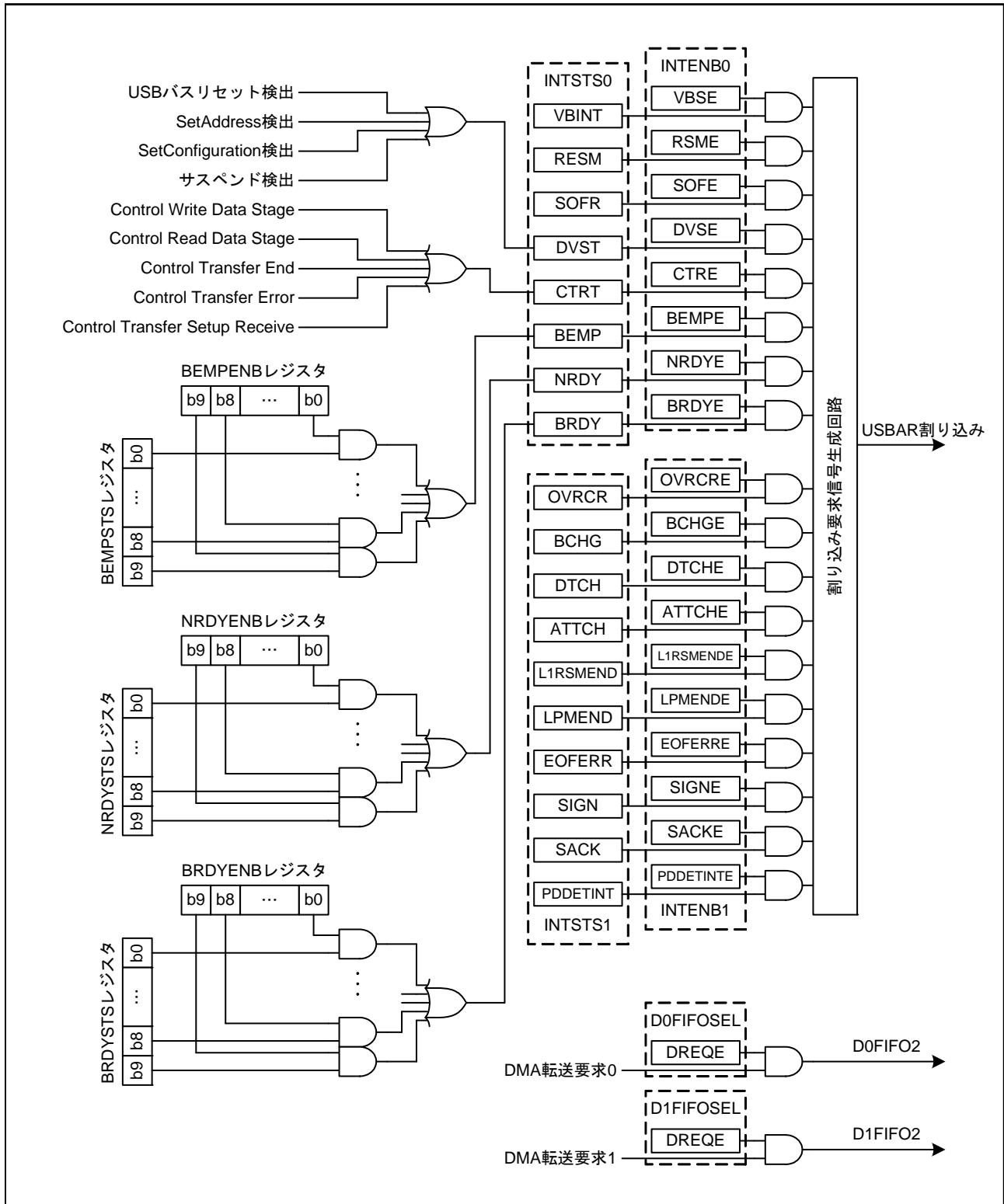
図 39.5 割り込み関連図
