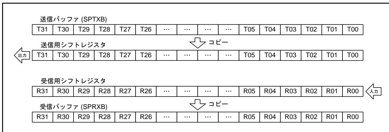
図 45.6 MSB ファースト転送 (32 ビットデータ)
