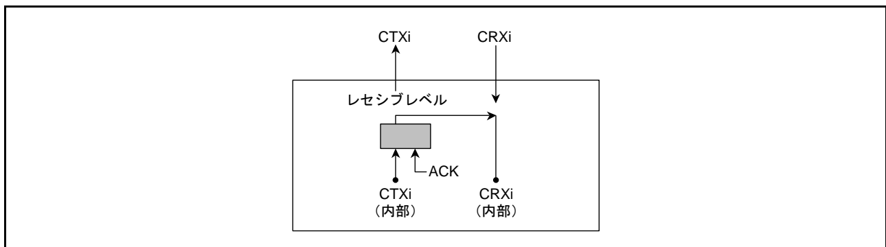
図43.8 セルフテストモード1選択時の接続 (i=0~2)
