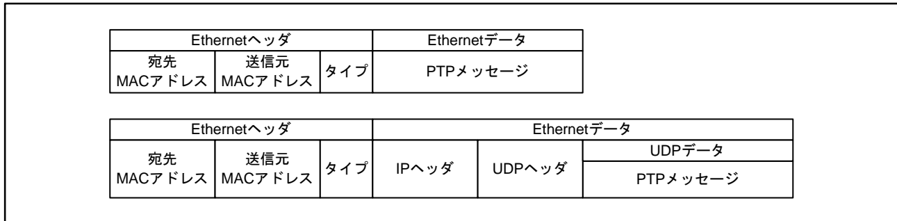
図36.2 PTPメッセージのフレームフォーマット
