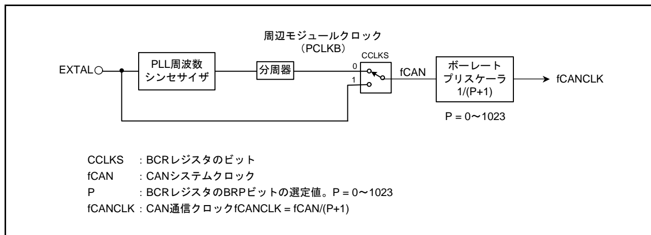
図 43.11 CAN クロック発生回路のブロック図
