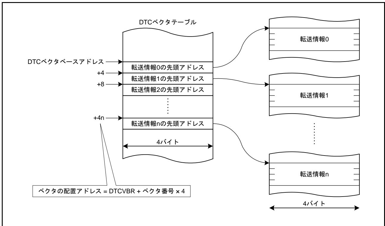
図 20.2 DTC ベクタテーブルと転送情報の対応
