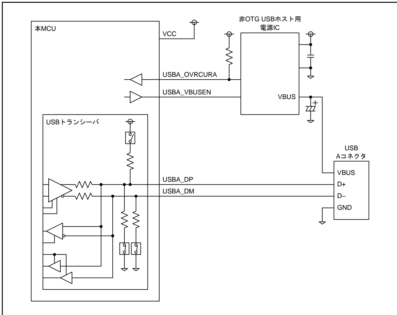
図 39.26 USB コネクタのホスト接続例
