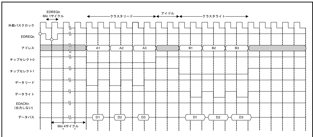
図 19.17 クラスタ転送デュアルアドレスモードでのバスサイクル例
