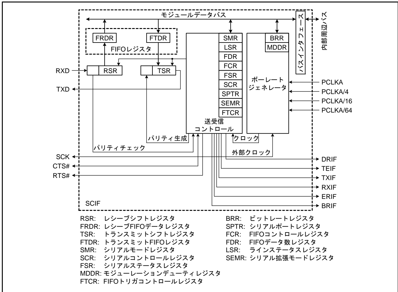
図 41.1 SCIFA のブロック図
