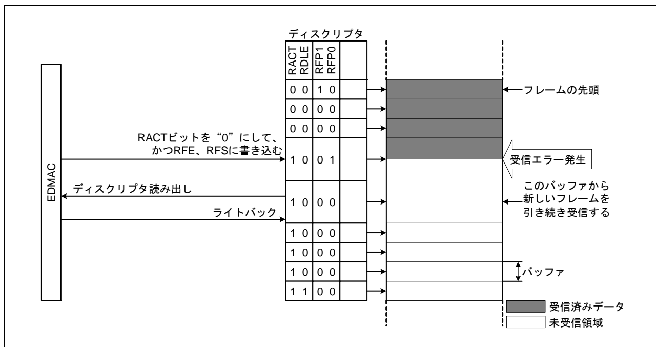
図 37.8 受信エラー発生後の EDMAc 動作
