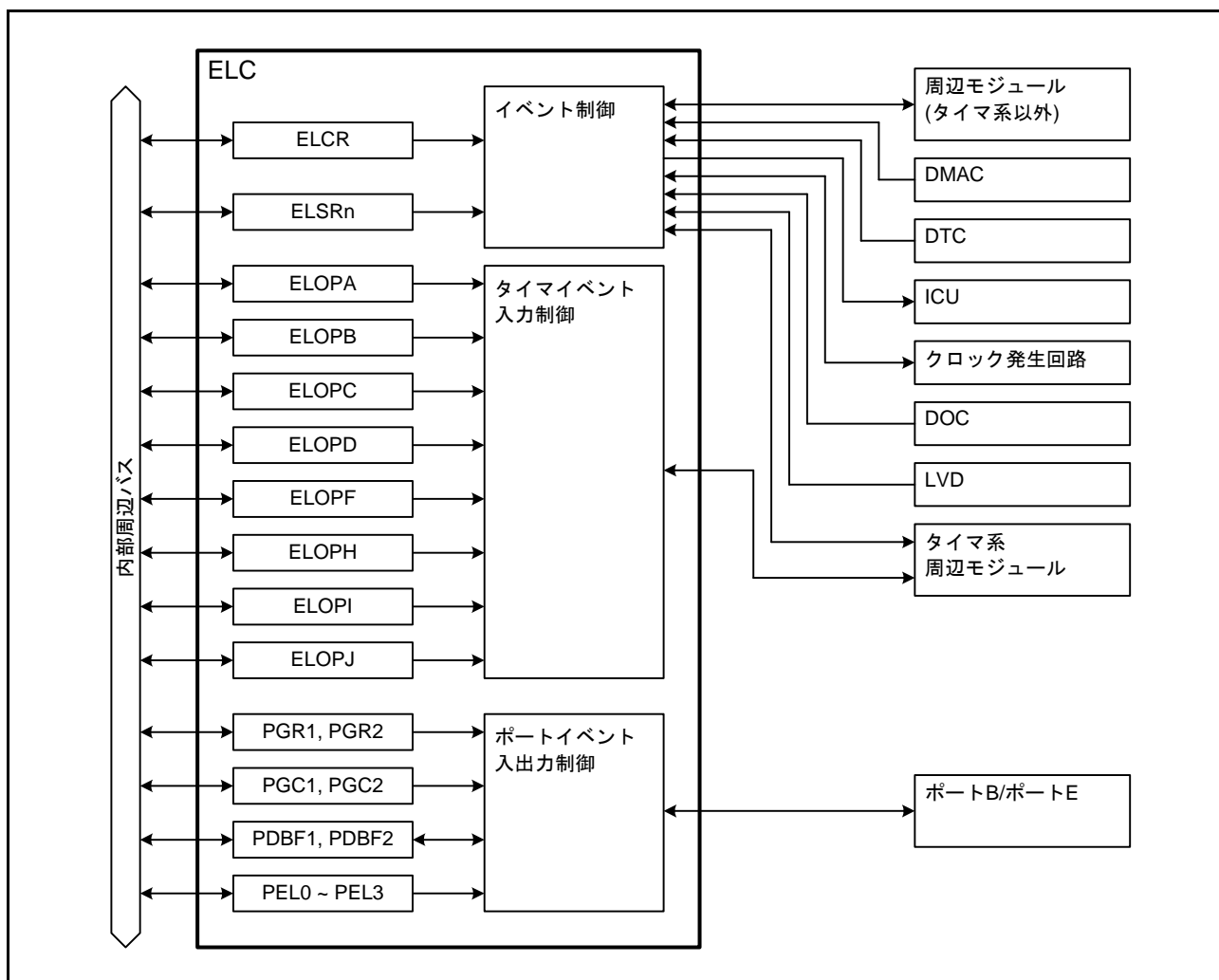
図 21.1 ELC のブロック図 (n = 0, 3, 4, 7, 10 ~ 13, 15, 16, 18 ~ 28, 33, 35 ~ 38, 41 ~ 45)
