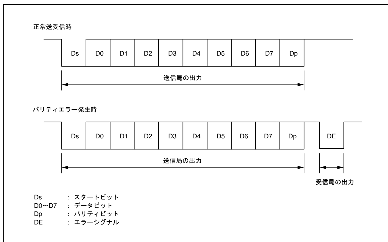
図 40.34 スマートカードインタフェースモードのデータフォーマット
