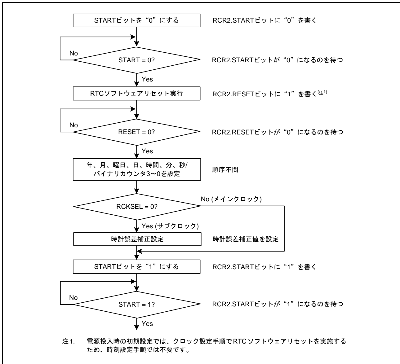
図 32.4 時刻設定手順
