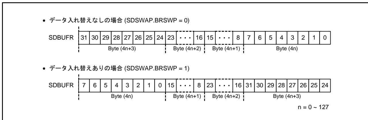
図 49.5 SDBUFRレジスタ読み出し時のデータ配置
