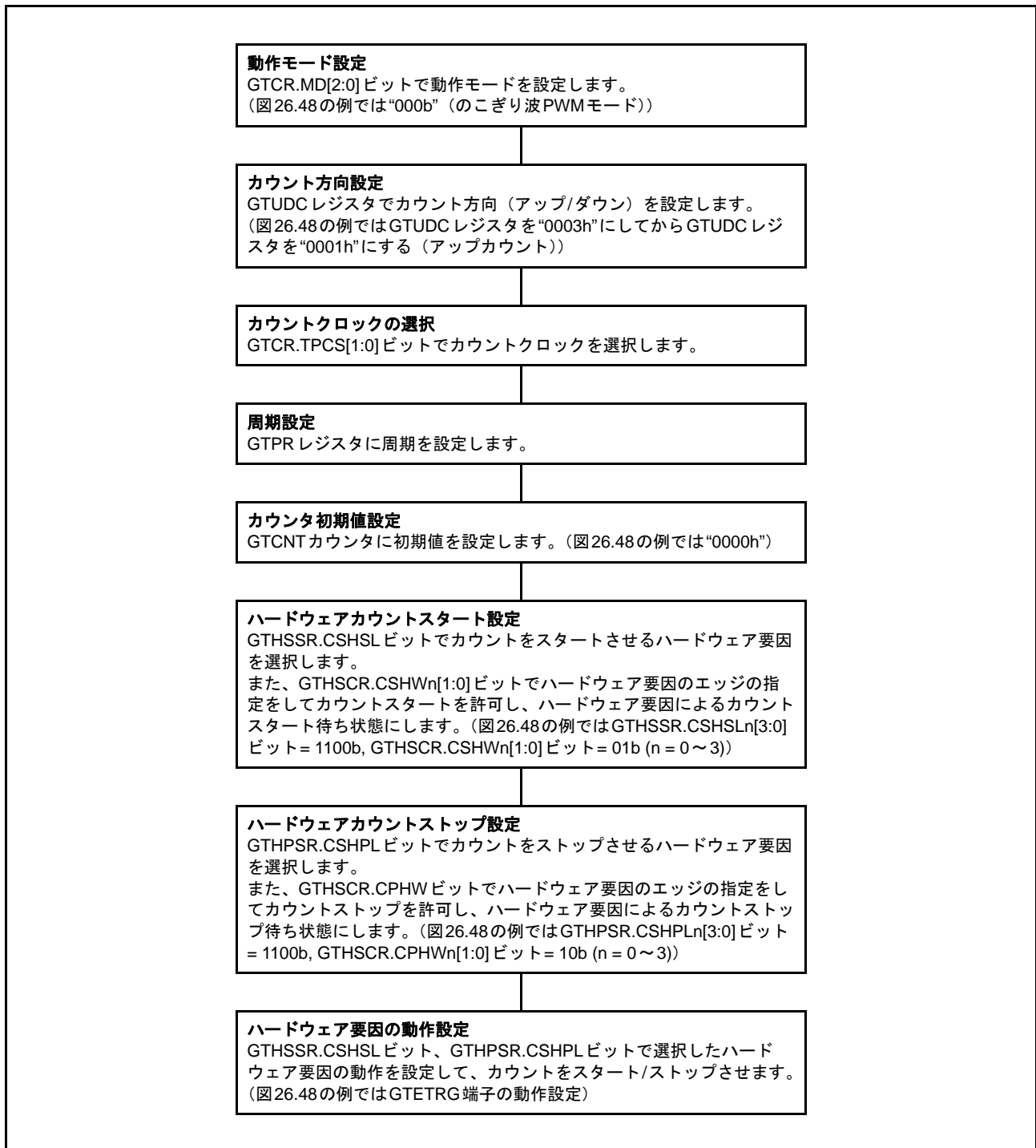
図 26.49 ハードウェア要因によるカウントスタート/ストップ動作設定例
