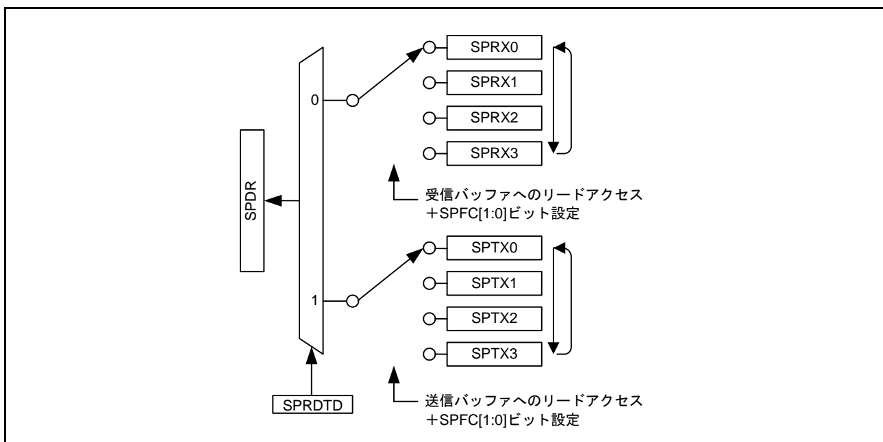
図 44.4 SPDR レジスタの構成図 (リード時)
