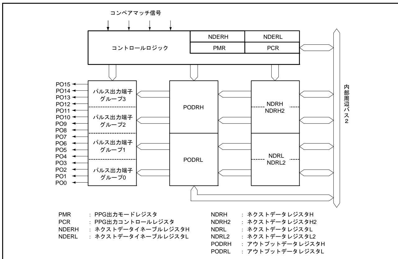
図 28.1 PPG0 のブロック図
