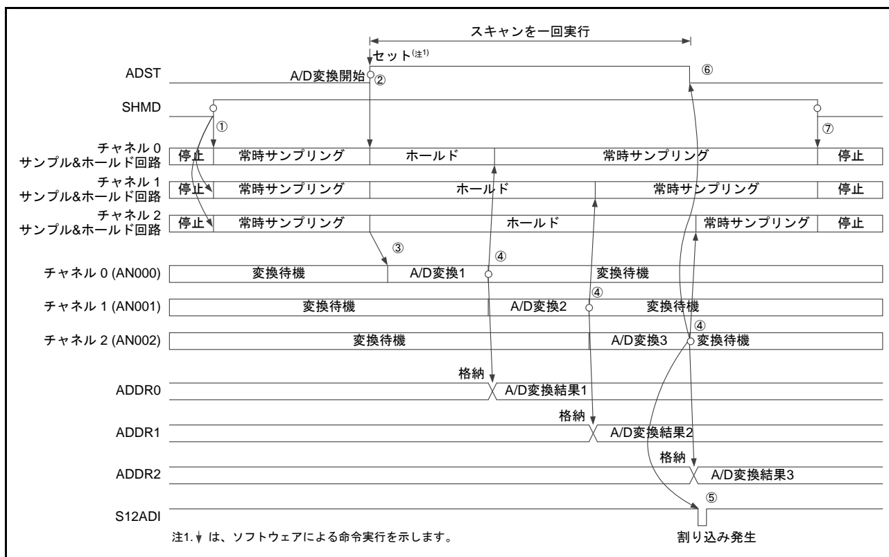
図 57.6 シングルスキャンモードの動作例 (チャンネル専用サンプル&ホールド回路使用 : AN000 ~ AN002 選択、常時サンプリング有効)
