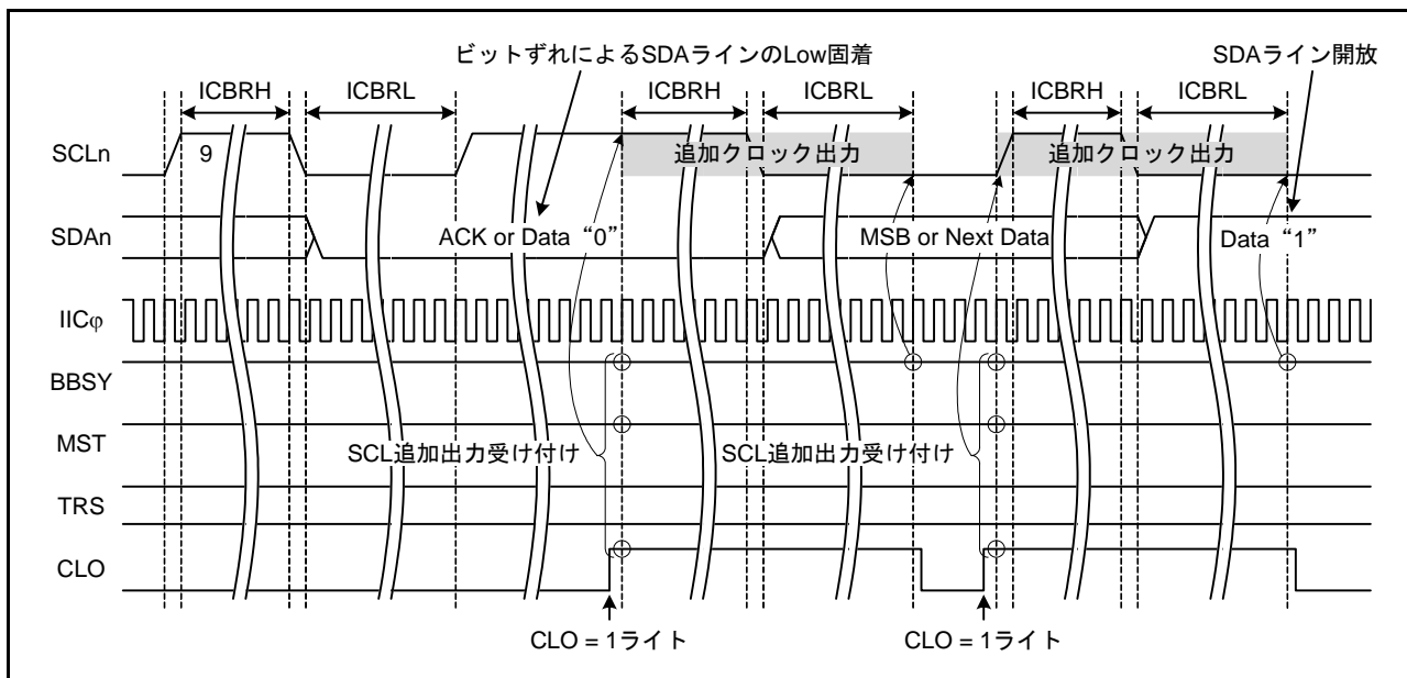
図 42.39 SCL 追加出力機能 (CLO ビット)
