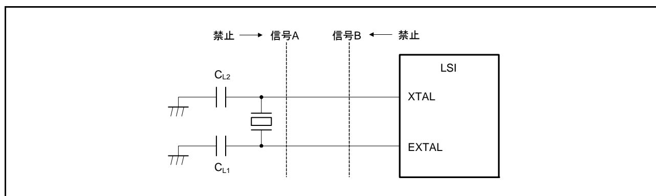
図 9.10 発振回路部のボード設計に関する注意事項（メインクロック発振器の場合、サブクロック発振器も同様）
