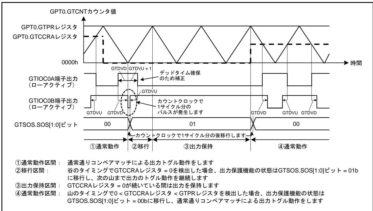
図 26.84 山のバッファ転送で GTCRA レジスタが“0000h”である場合の出力保護機能の動作例 (山のバッファ転送で 0 < \text{GTCRA レジスタ} < \text{GTPR レジスタ} に復帰、アクティブレベルは Low の場合)
