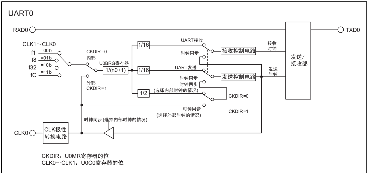
图 20.1 UART0 的框图
