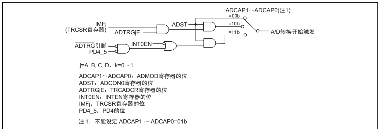
图 22.4 A/D 转换开始控制部的框图
