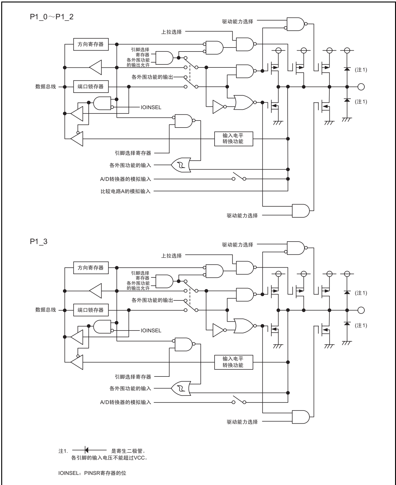
图 7.2 I/O 端口的结构 (2)
