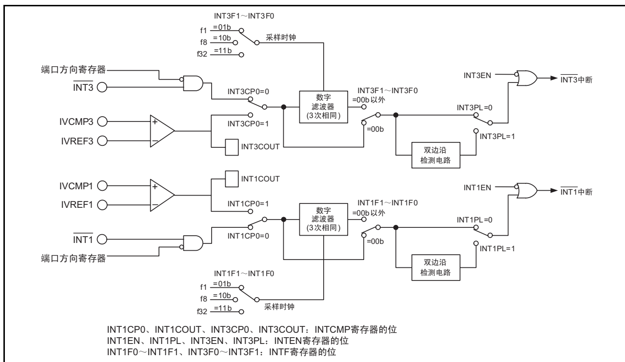
图 24.1 比较电路 B 的框图
