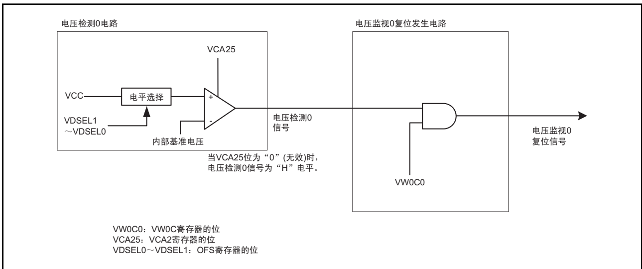
图 6.2 电压监视 0 复位发生电路的框图
