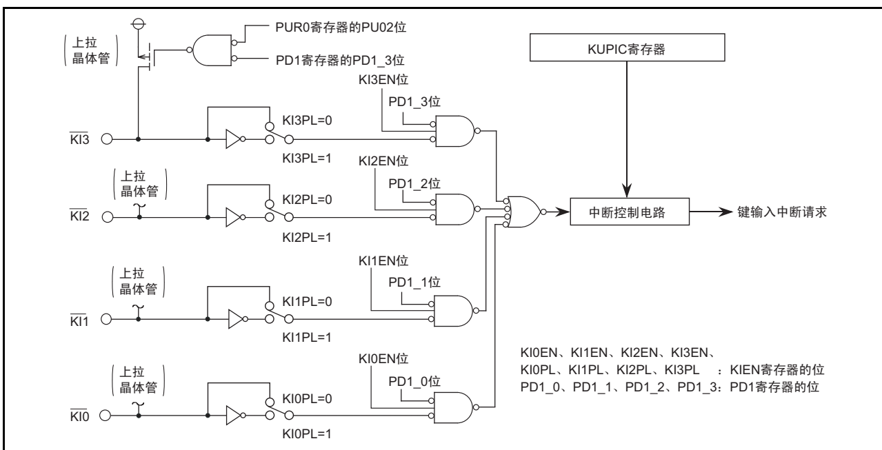
图 11.11 键输入中断的框图
