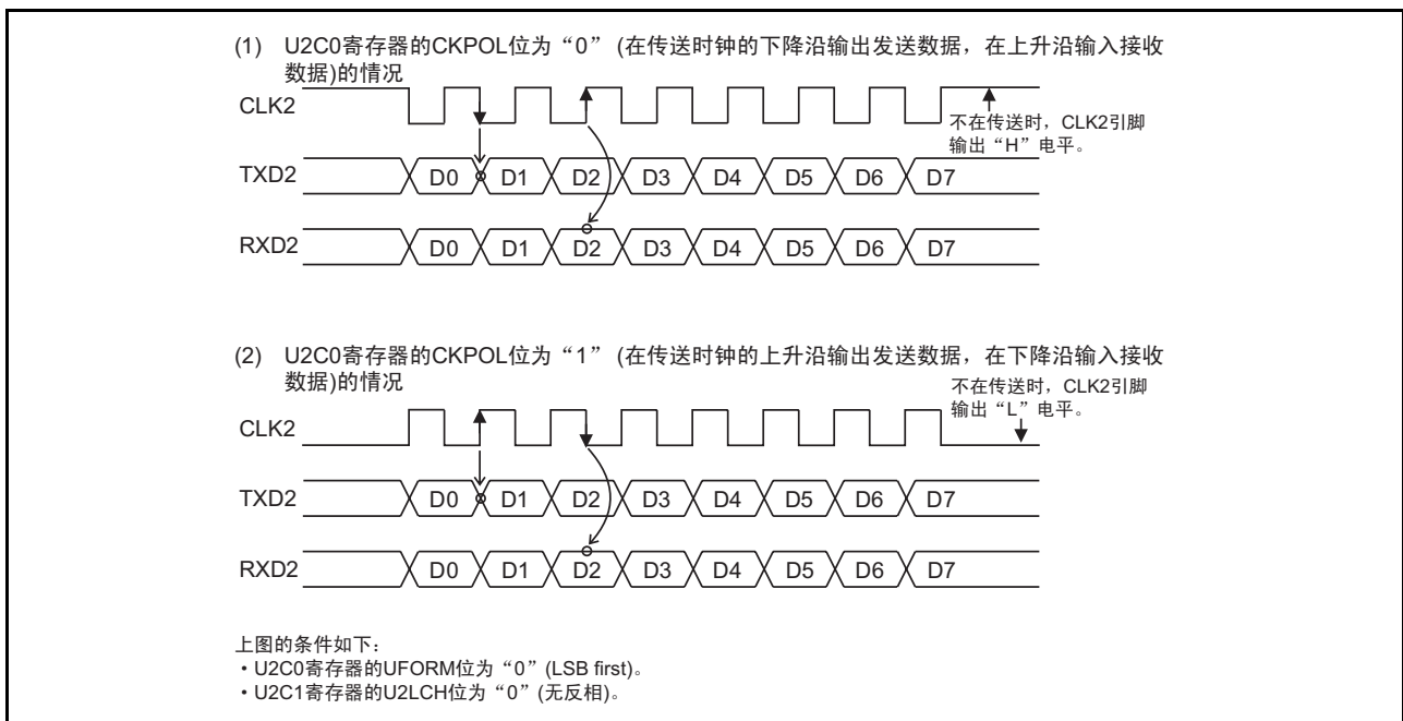
图 21.4 传送时钟的极性
