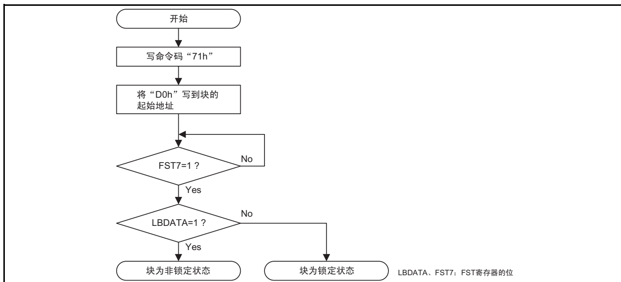
图 25.12 读锁定位状态的流程图
