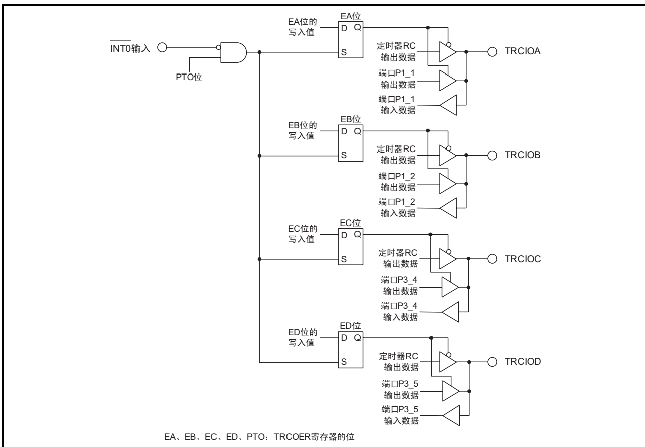
图 18.6 脉冲输出的强制截止
