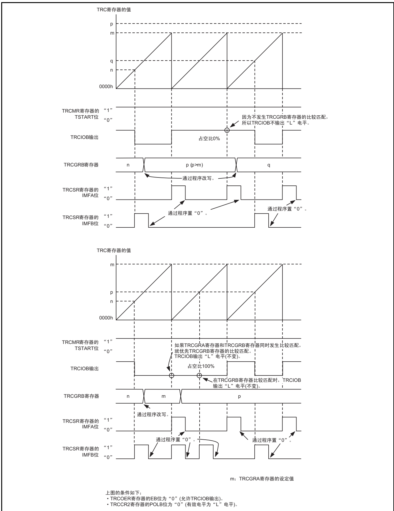
图 18.15 PWM 模式的运行例子 (占空比为 0% 和 100%)
