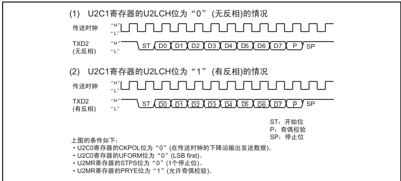
图 21.10 串行数据的逻辑
