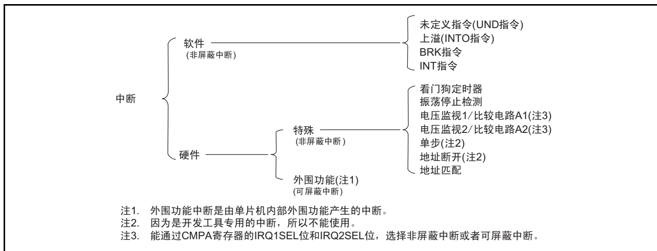
图 11.1 中断的分类
