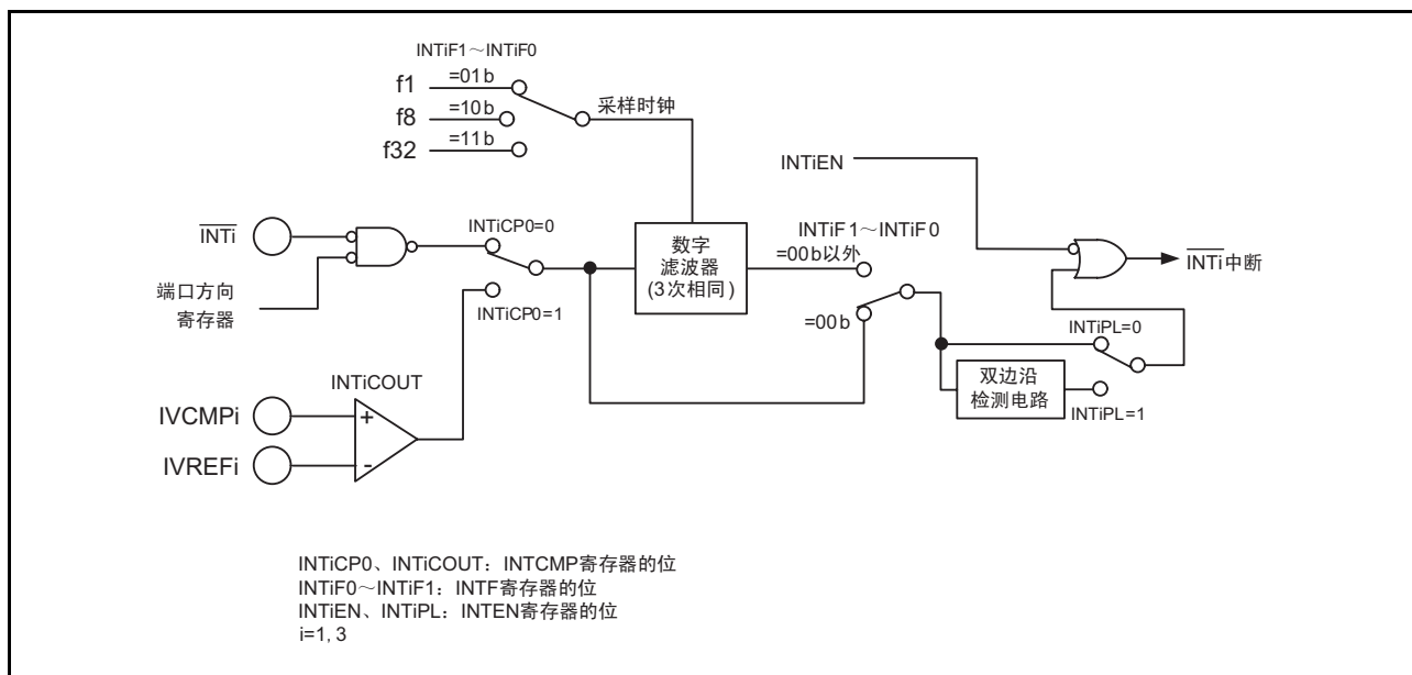
图 24.3 比较电路 Bi 数字滤波器的结构
