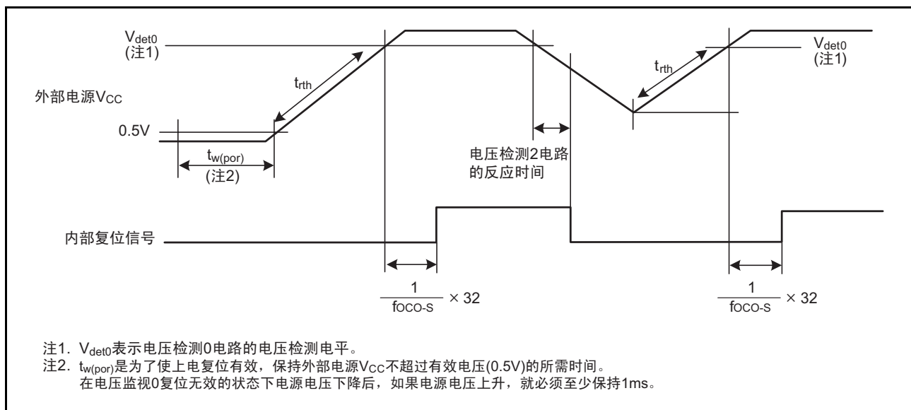
图 27.3 上电复位电路的电特性
