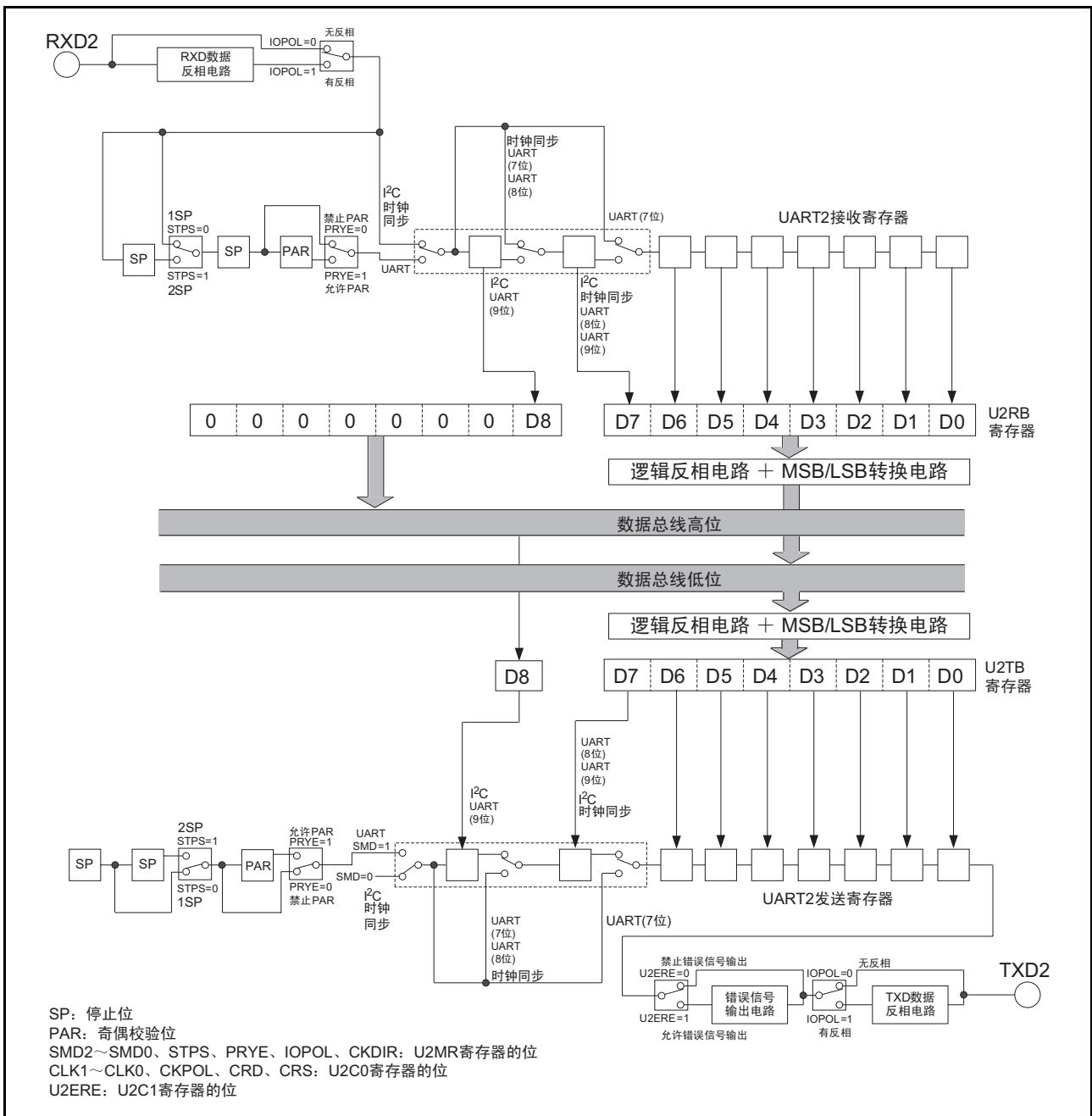
图 21.2 UART2 发送 / 接收部的框图
