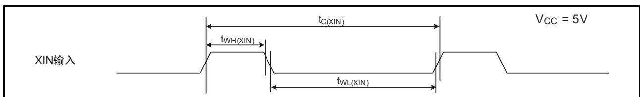
图 27.4 V CC =5V 时的 XIN 和 XCIN 的输入时序
