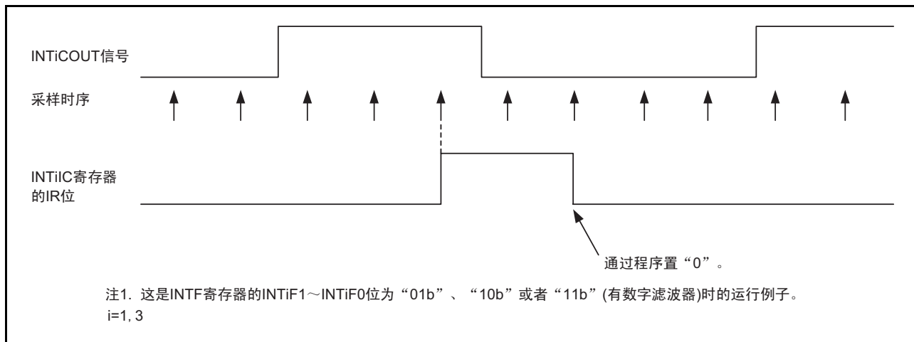
图 24.4 比较电路 Bi 数字滤波器的运行例子
