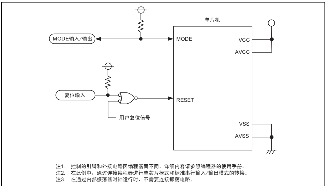
图 25.16 使用标准串行输入 / 输出模式 3 时的引脚处理例子
