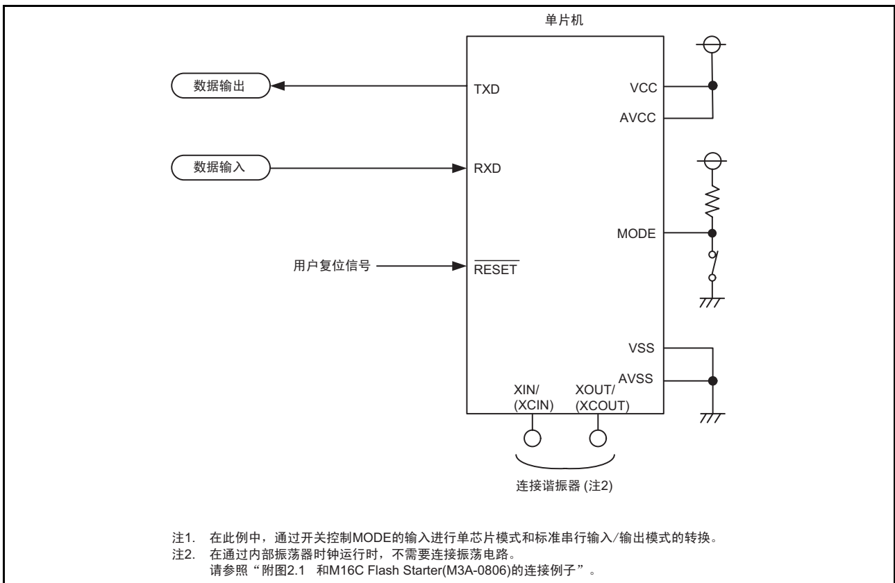
图 25.15 使用标准串行输入 / 输出模式 2 时的引脚处理例子
