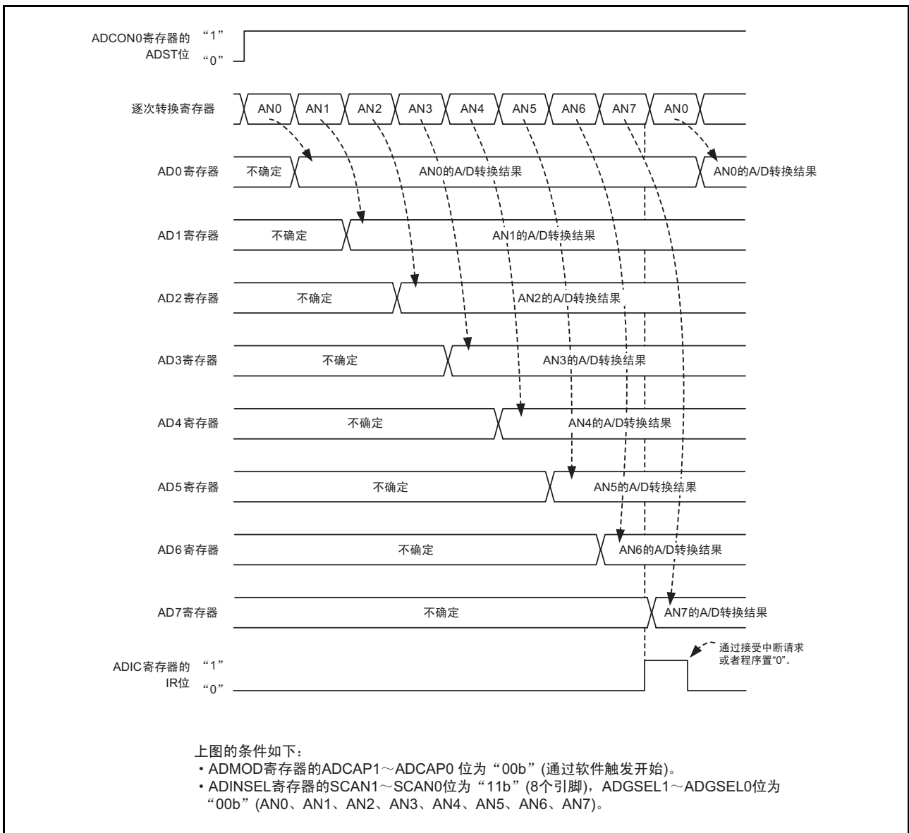
图 22.9 重复扫描模式的运行例子
