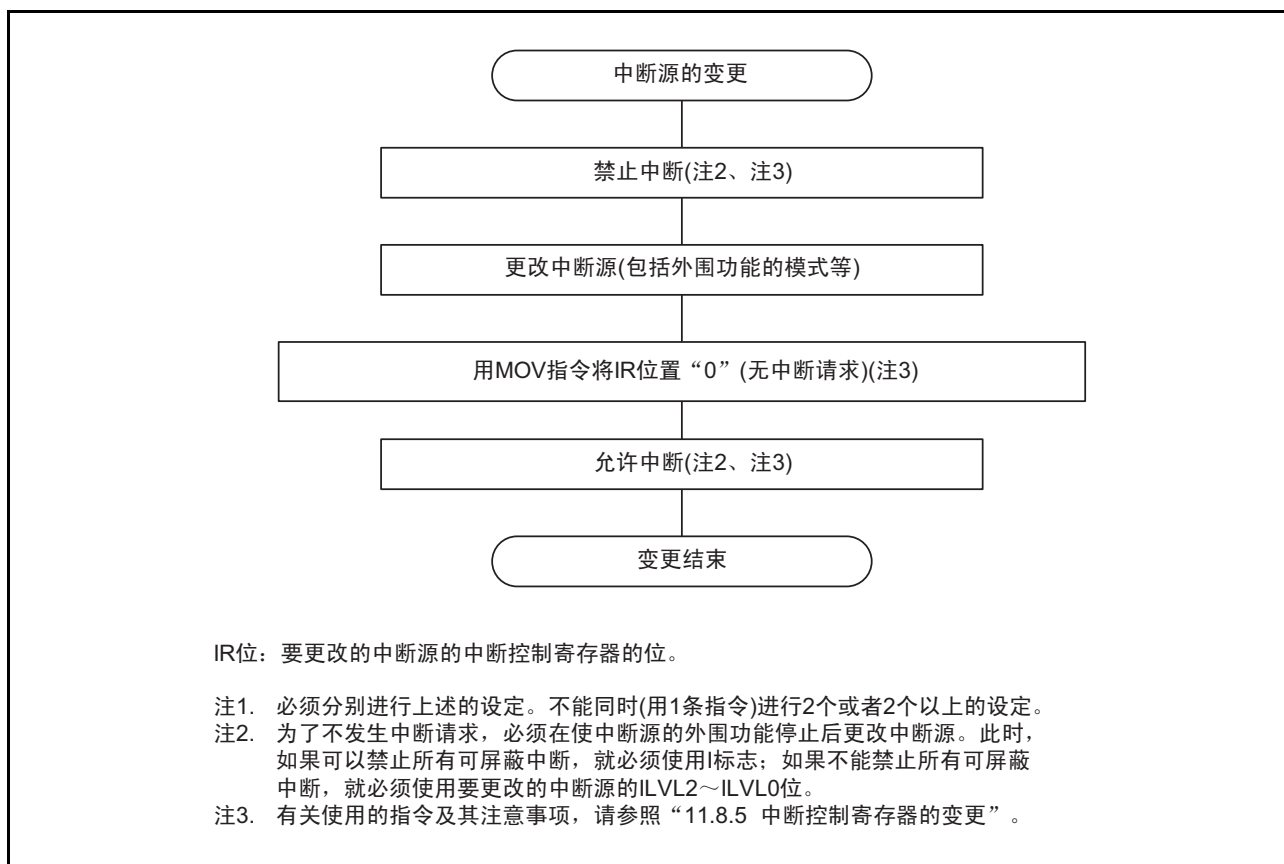
图 28.1 中断源的变更步骤例子
