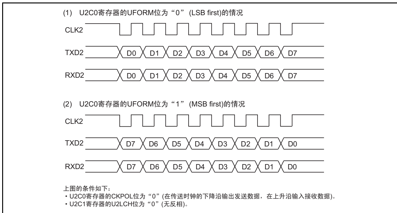
图 21.5 传送格式
