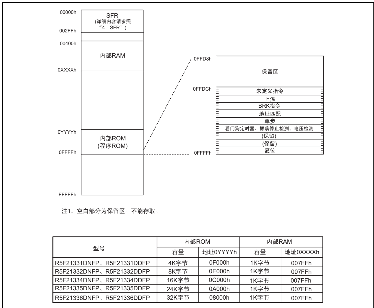
图 3.1 R8C/33D 群的存储器分配图
