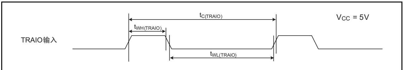
图 27.5 V_{CC}=5V 时的 TRAIO 输入时序
