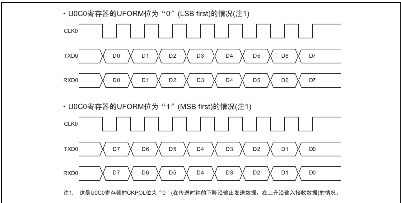
图 20.5 传送格式
