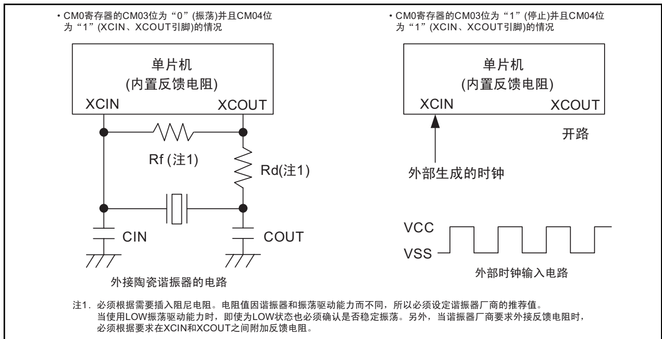
图 9.5 XCIN 时钟的连接电路例子
