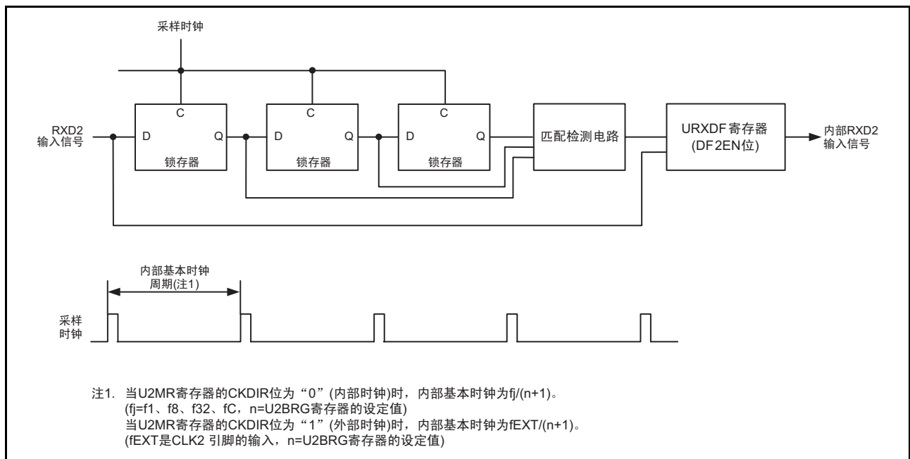
图 21.22 RXD2 数字滤波器电路的框图
