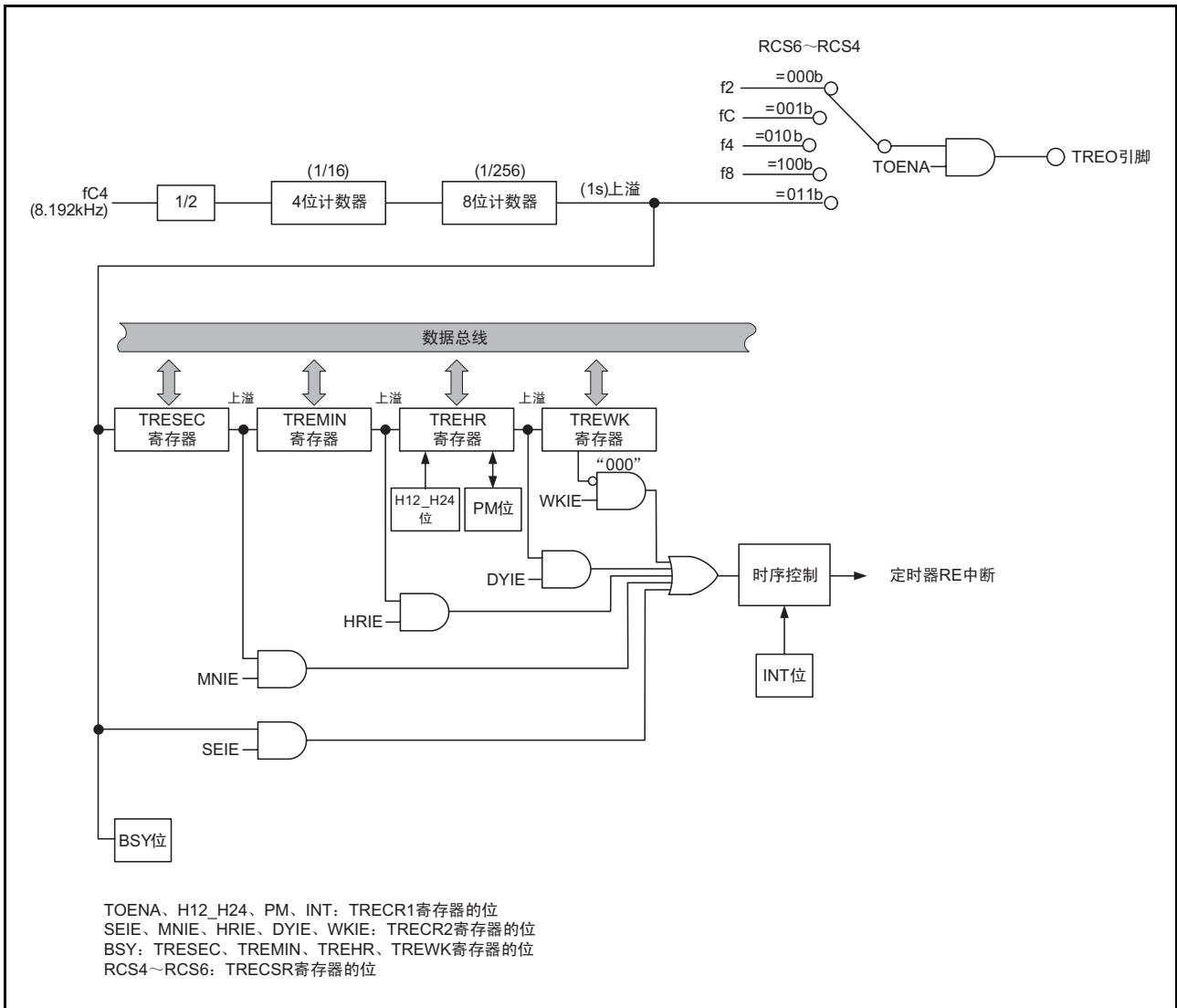
图 19.1 实时时钟模式的框图
