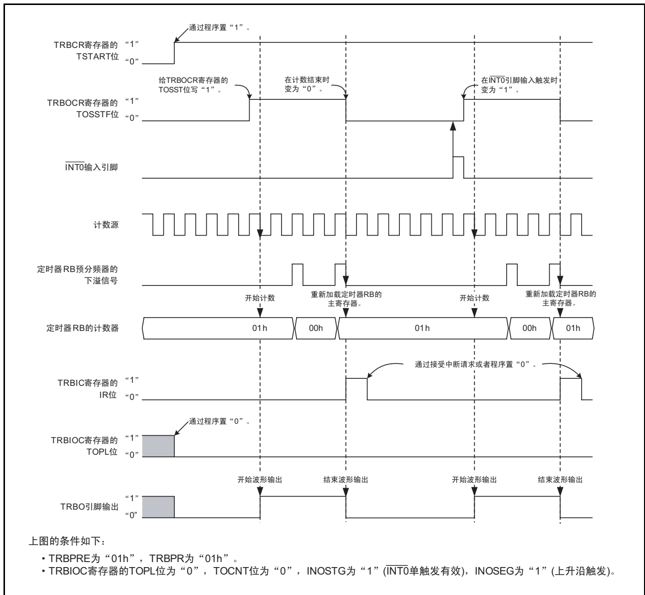
图 17.4 可编程单触发发生模式的运行例子
