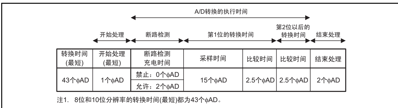
图 22.3 A/D 转换周期数 ( \phi_{AD}=f_{AD} )
