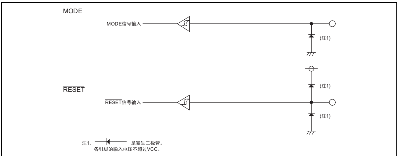
图 7.11 引脚的结构
