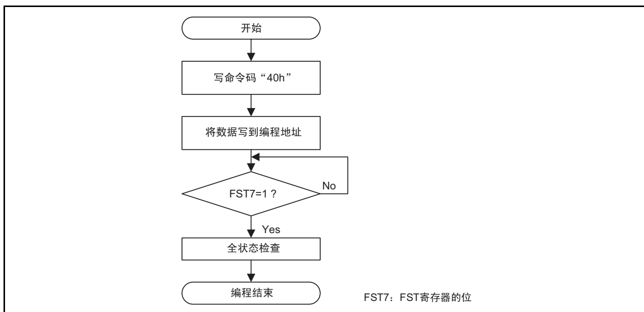
图 25.6 编程的流程图（禁止闪存就绪状态的中断）
