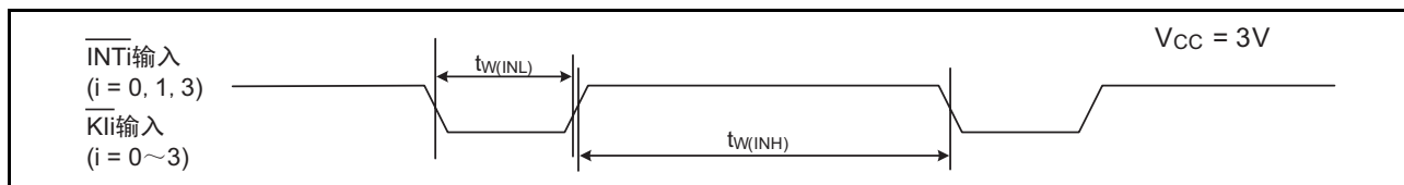
图 27.11 V_{CC}=3V 时的外部中断 \overline{INTi} 和键输入中断 \overline{Kli} 的输入时序
