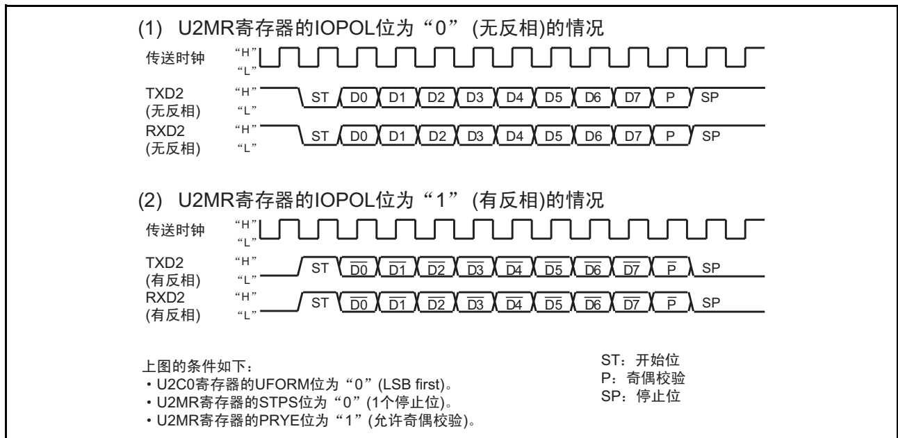
图 21.11 TXD 和 RXD 输入 / 输出极性的转换
