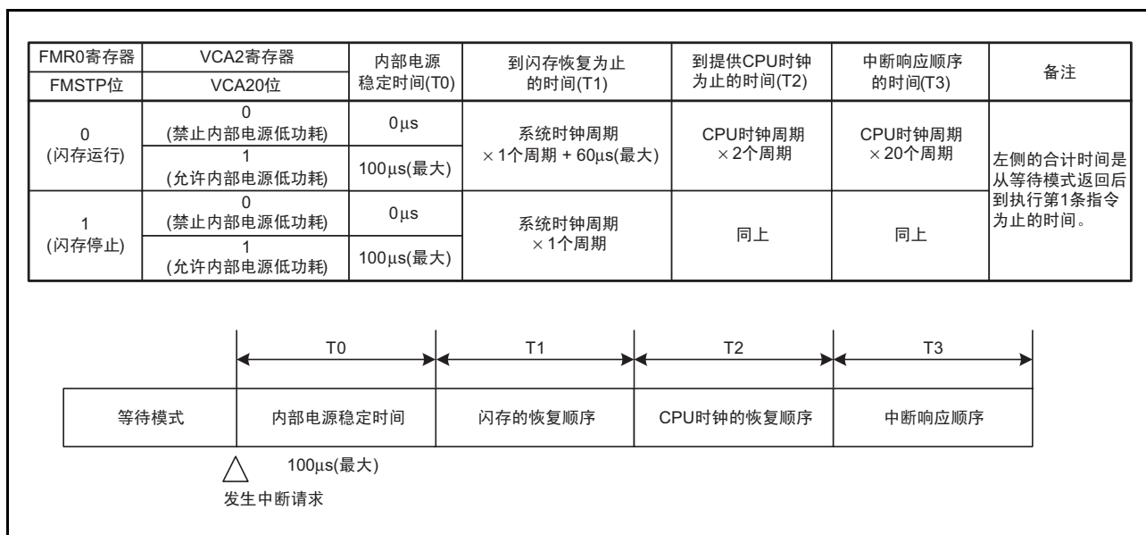
图 9.7 从执行 WAIT 指令后的等待模式到执行中断程序的时间
