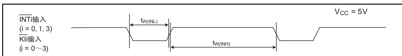
图 27.7 V_{CC}=5V 时的外部中断 \overline{\text{INTi}} 和键输入中断 \overline{\text{Kli}} 的输入时序
