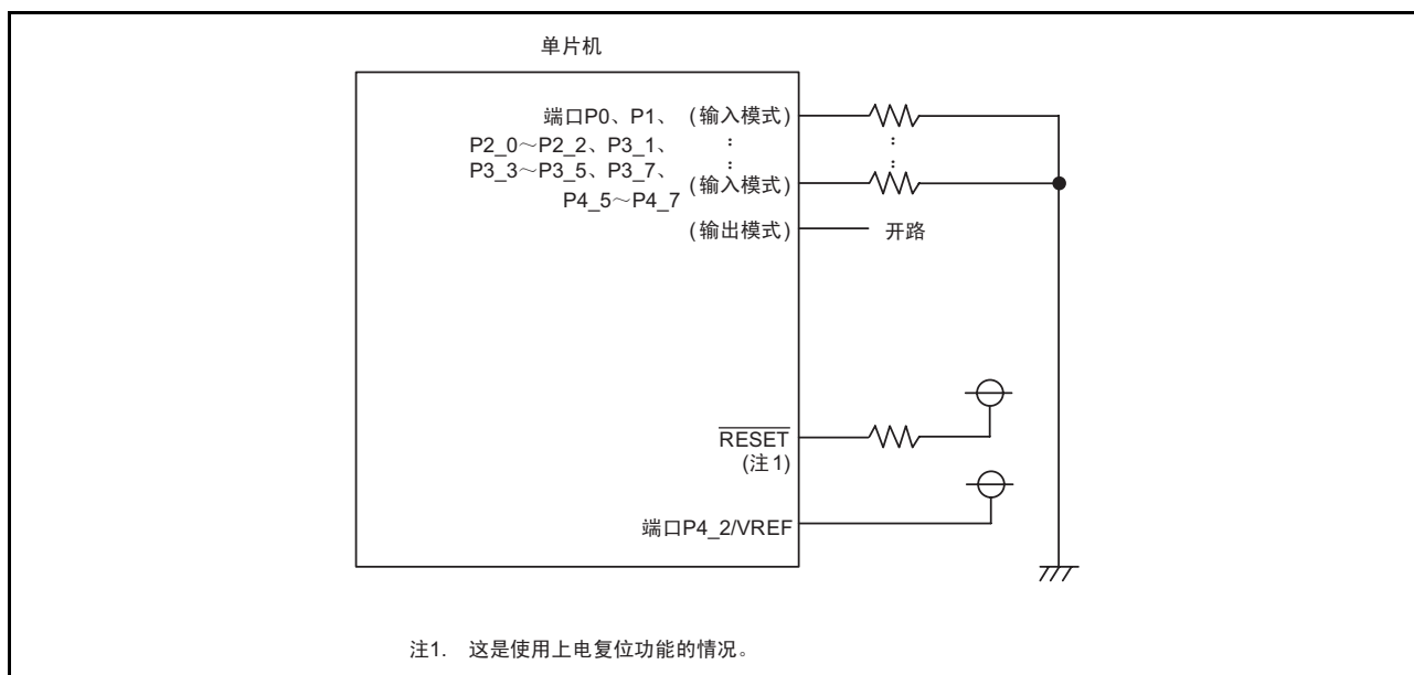
图 7.12 未使用引脚的处理例子
