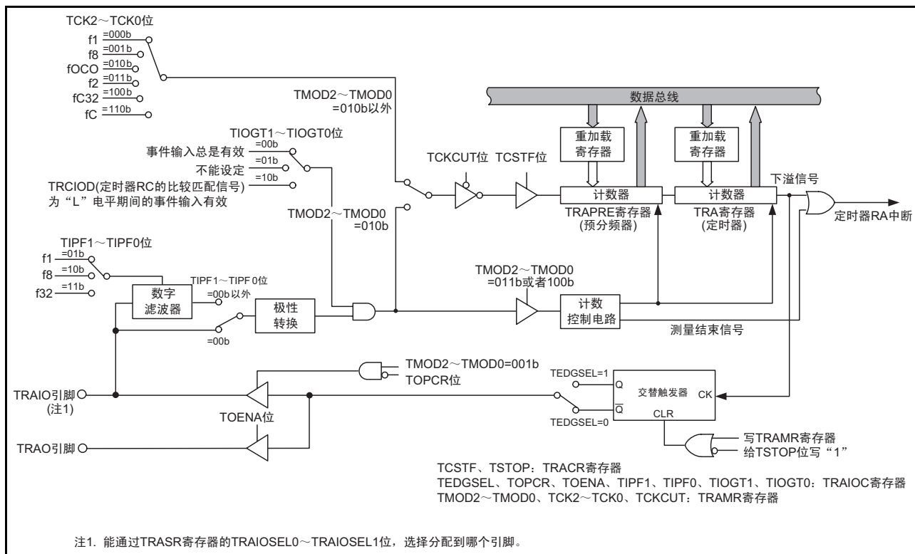
图 16.1 定时器 RA 的框图
