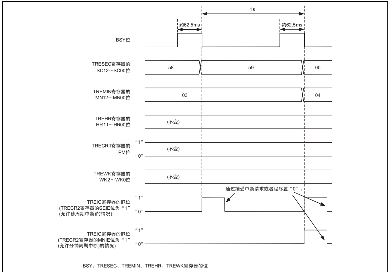
图 19.3 实时时钟模式的运行例子
