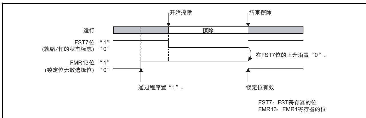
图 25.5 FMR13 位操作的相关时序
