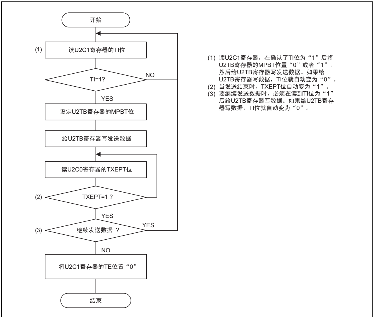
图 21.19 多处理器数据发送的流程图例子
