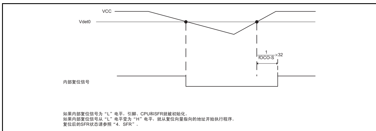
图 6.5 电压监视 0 复位的运行例子
