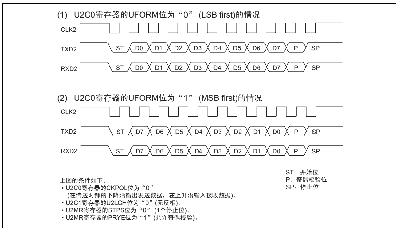
图 21.9 传送格式
