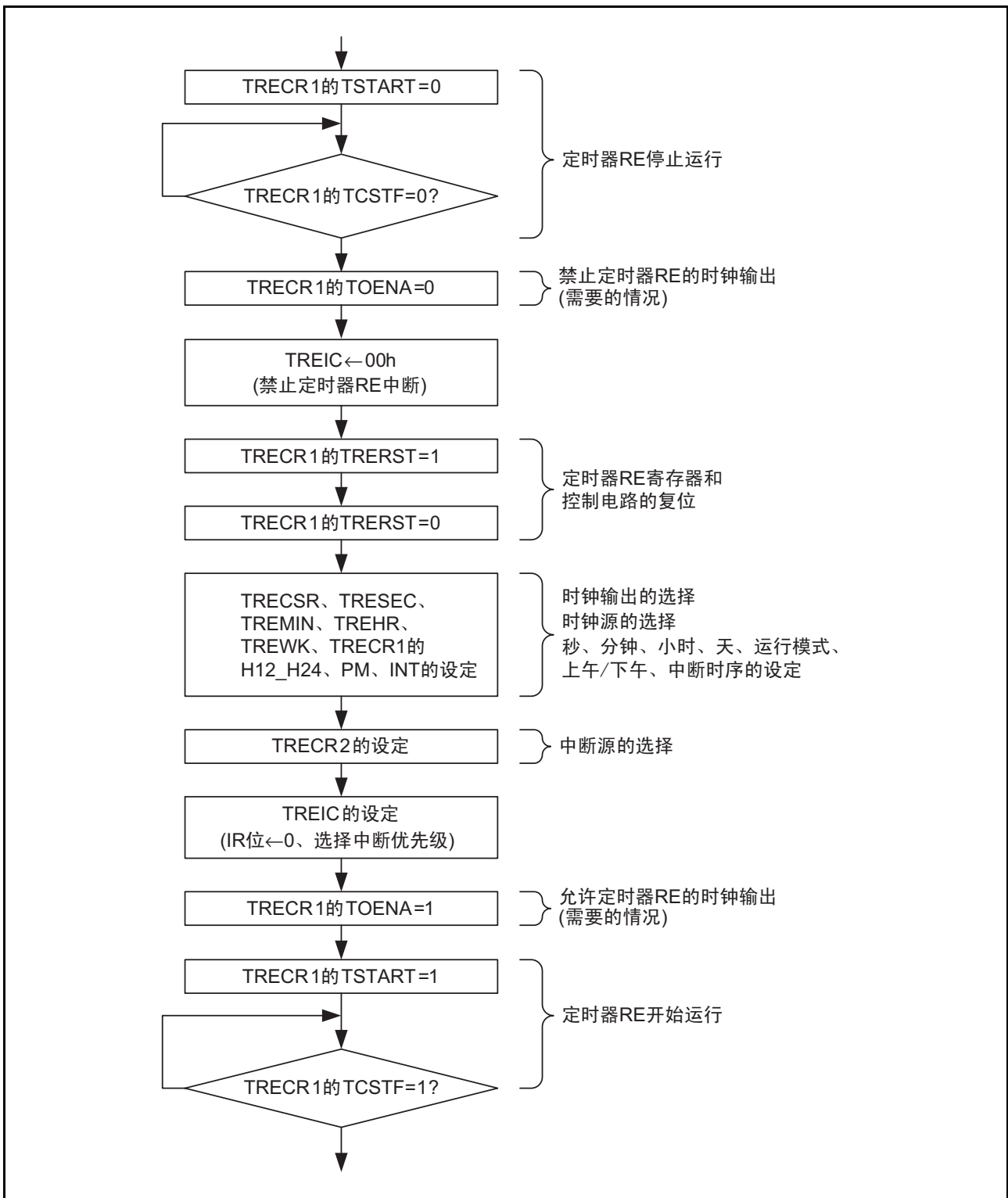
图 19.6 实时时钟模式的设定例子
