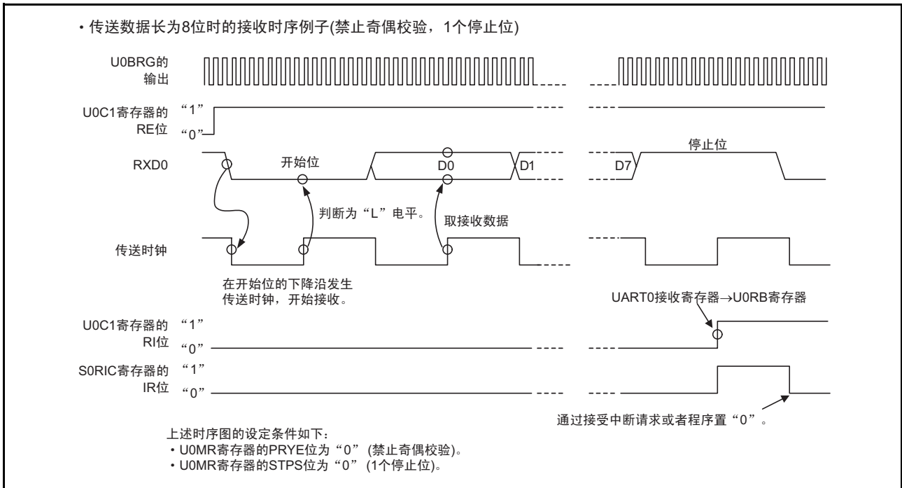
图 20.7 UART 模式的接收时序例子
