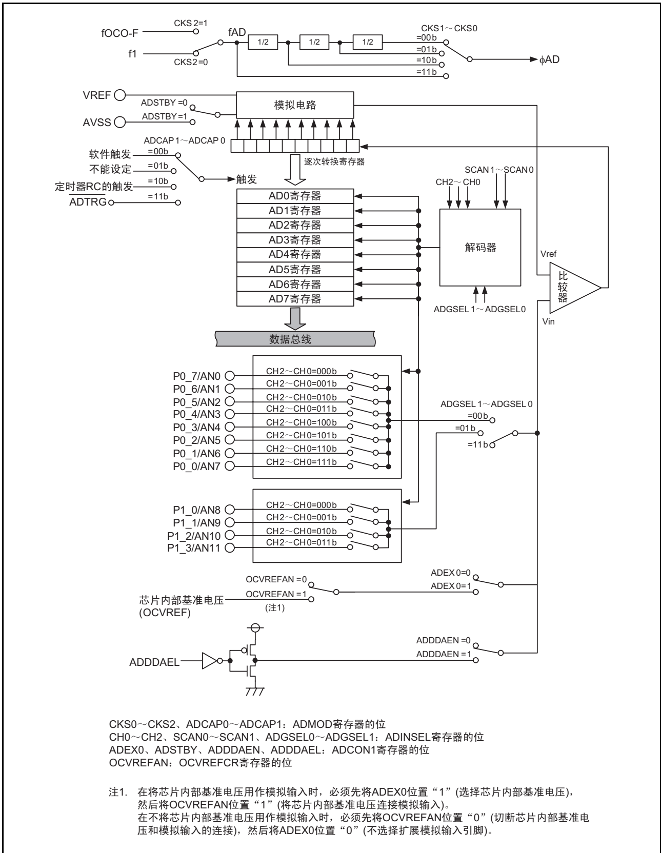
图 22.1 A/D 转换器的框图
