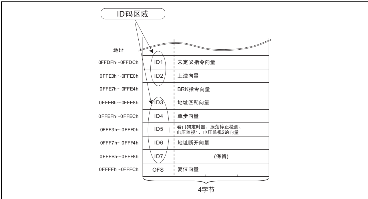
图 12.1 ID 码区域
