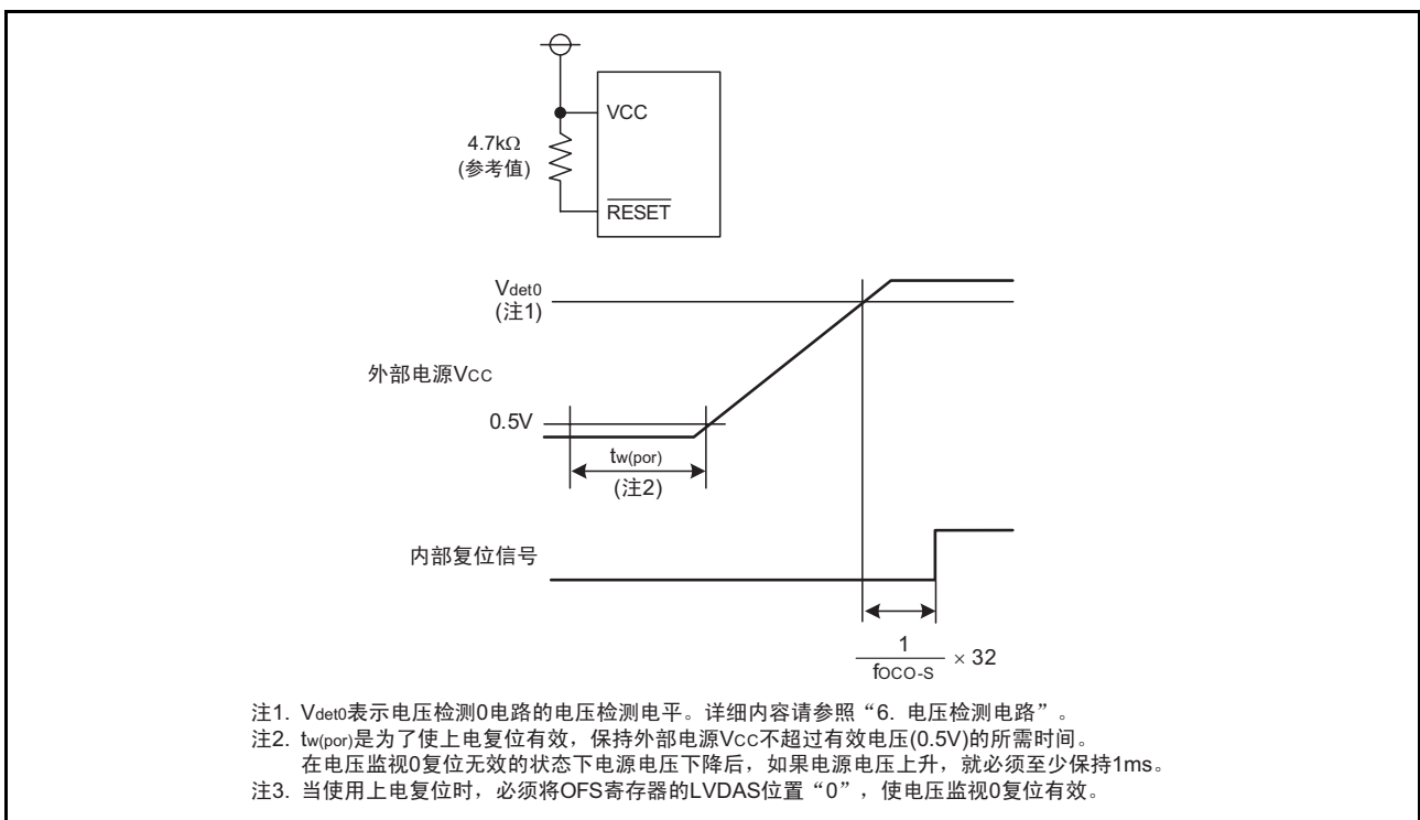
图 5.6 上电复位的电路例子和运行
