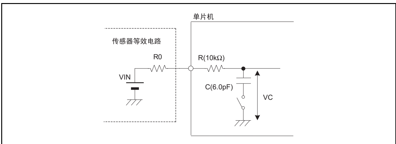
图 22.10 模拟输入引脚和外部传感器的等效电路例子
