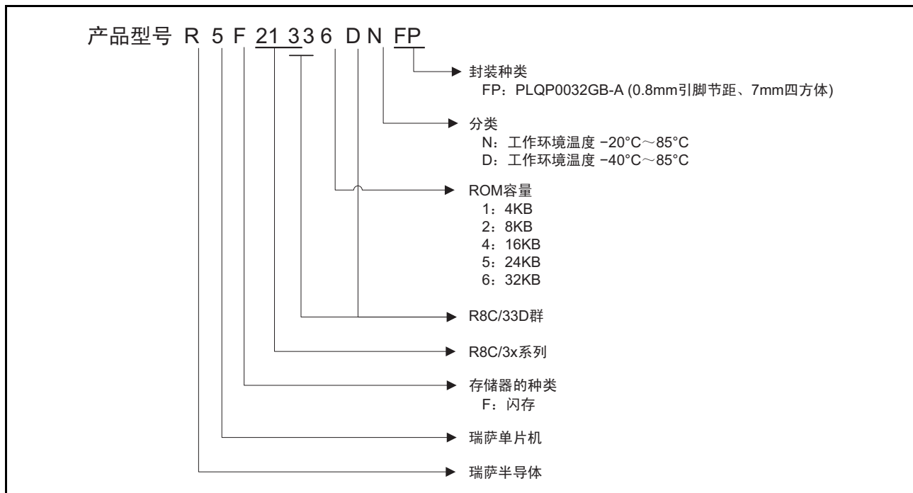
图 1.1 R8C/33D 群的产品型号、存储器容量和封装
