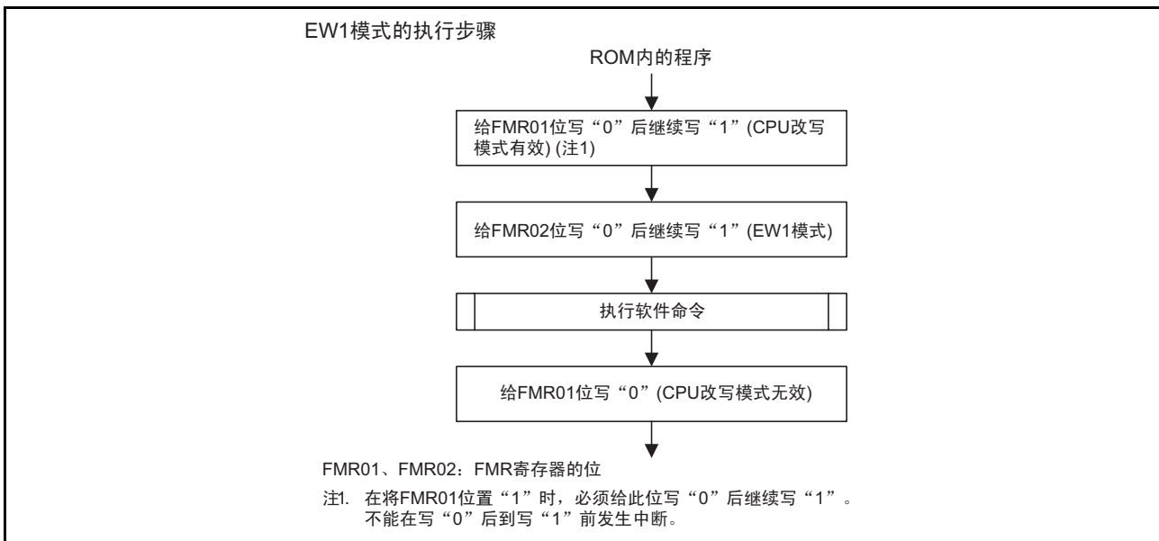
图 25.4 EW1 模式的设定和解除方法
