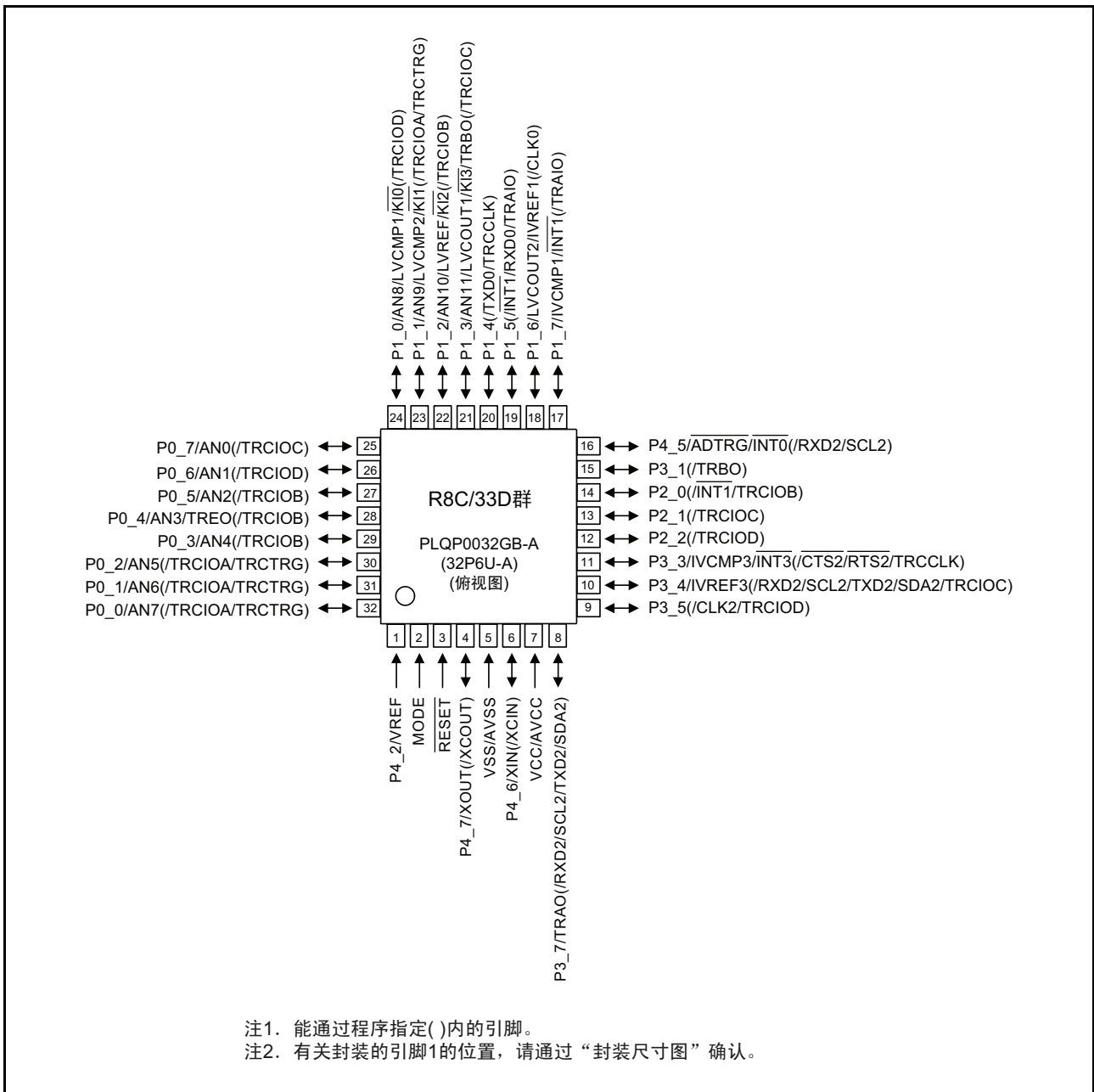
图 1.3 引脚排列图（俯视图）
