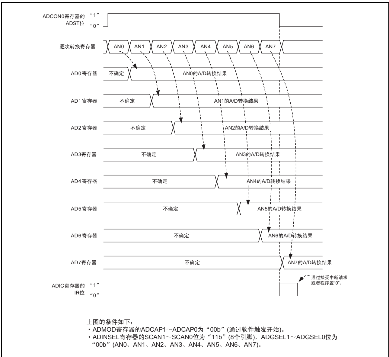
图 22.8 单次扫描模式的运行例子
