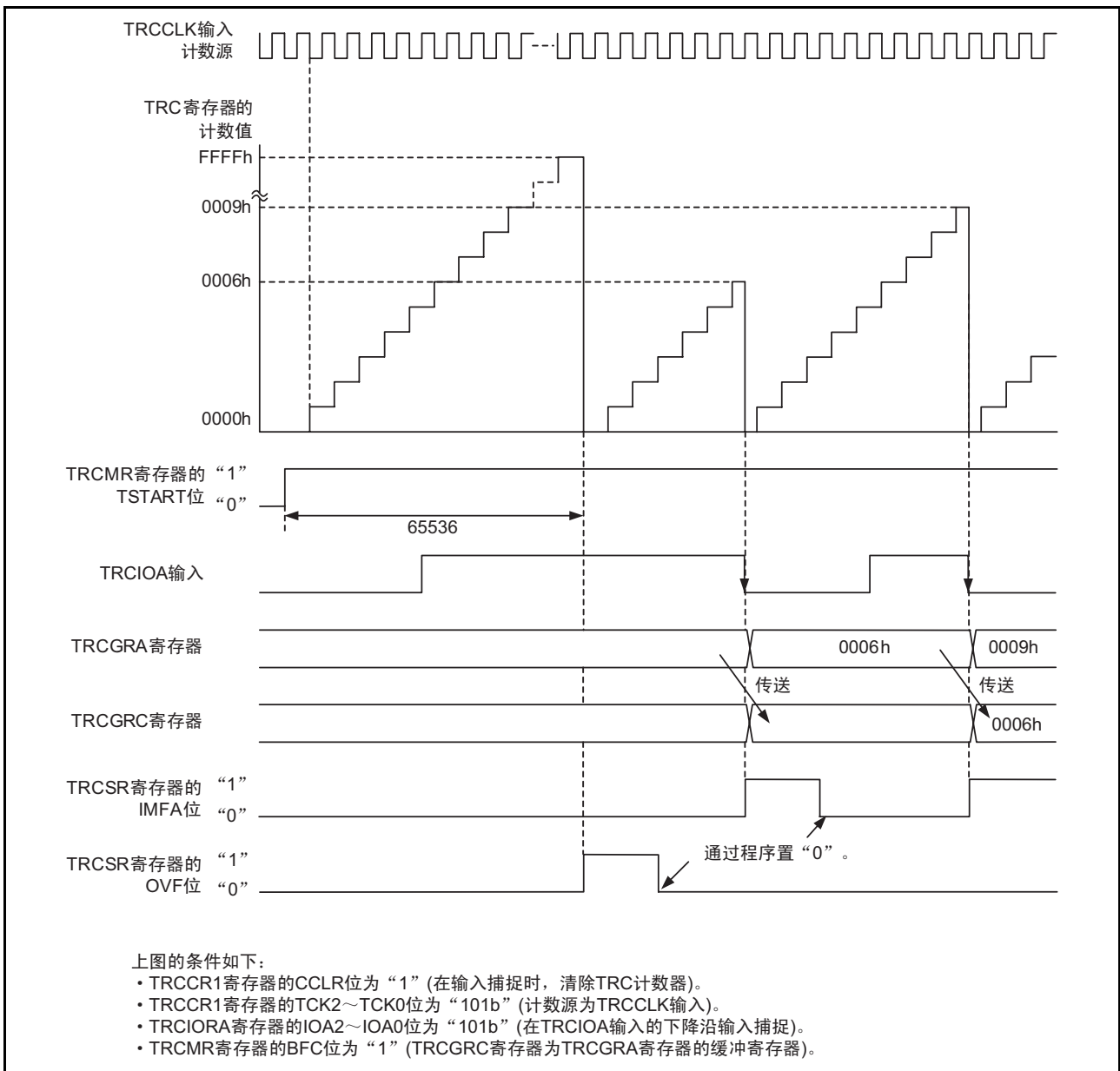
图 18.8 输入捕捉功能的运行例子
