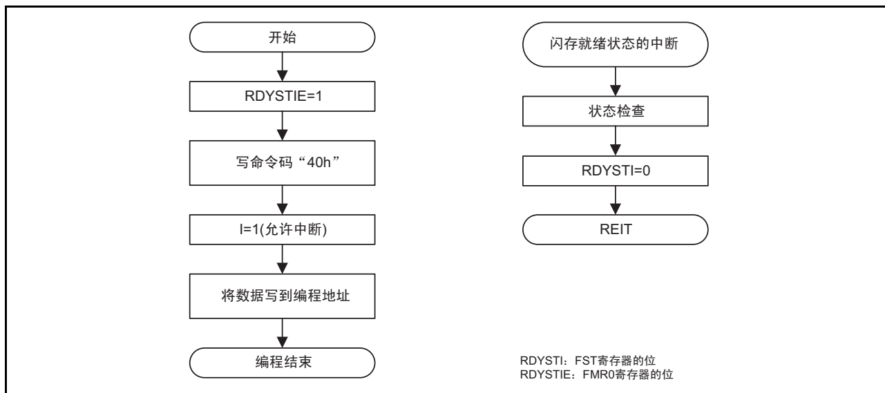
图 25.7 编程的流程图（允许闪存就绪状态的中断）
