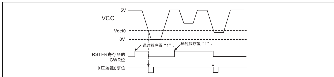
图 5.8 冷启动 / 热启动的判断功能的运行例子
