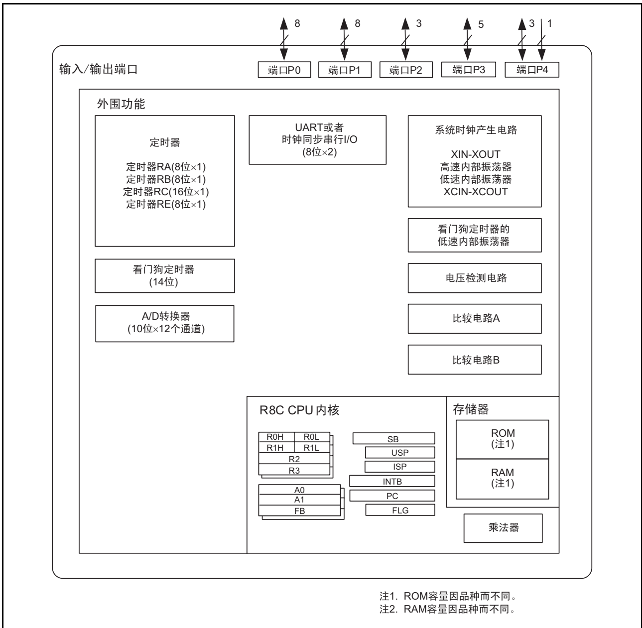
图 1.2 框图
