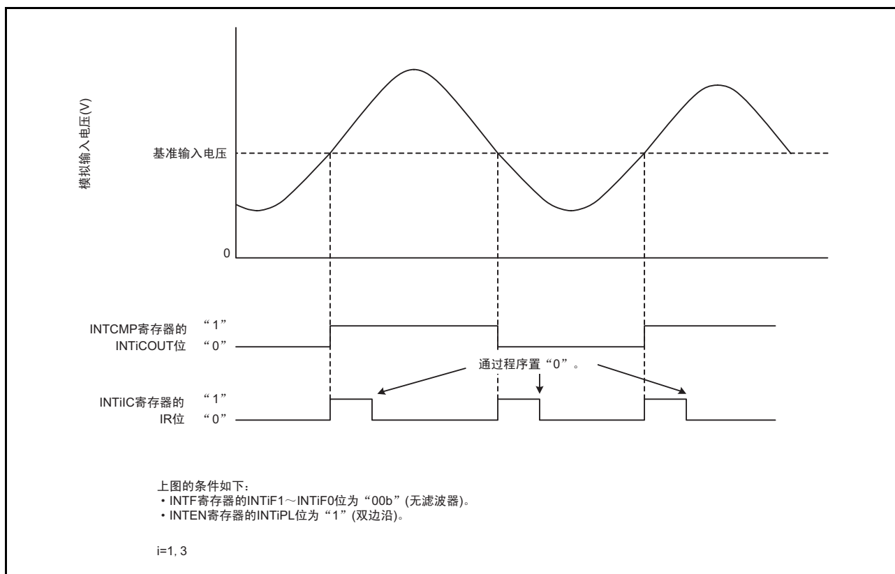
图 24.2 比较电路 Bi (i=1,3) 的运行例子
