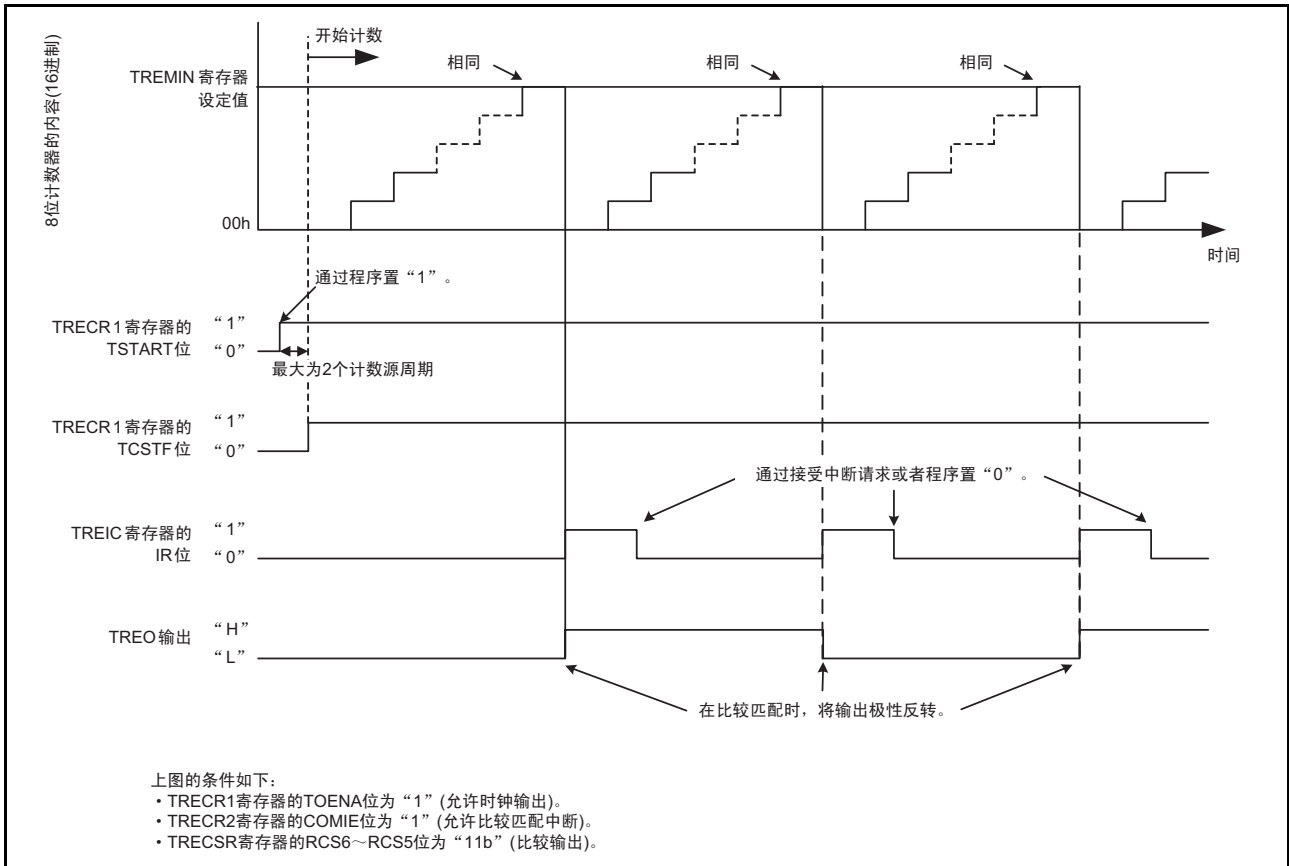
图 19.5 输出比较模式的运行例子
