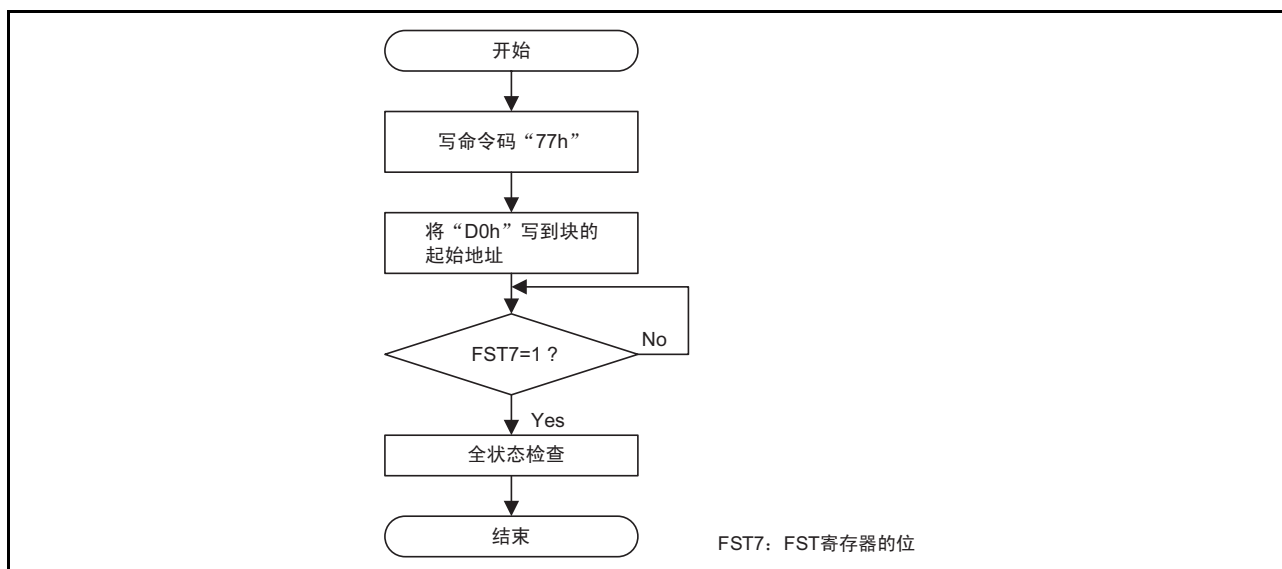
图 25.11 锁定位编程的流程图
