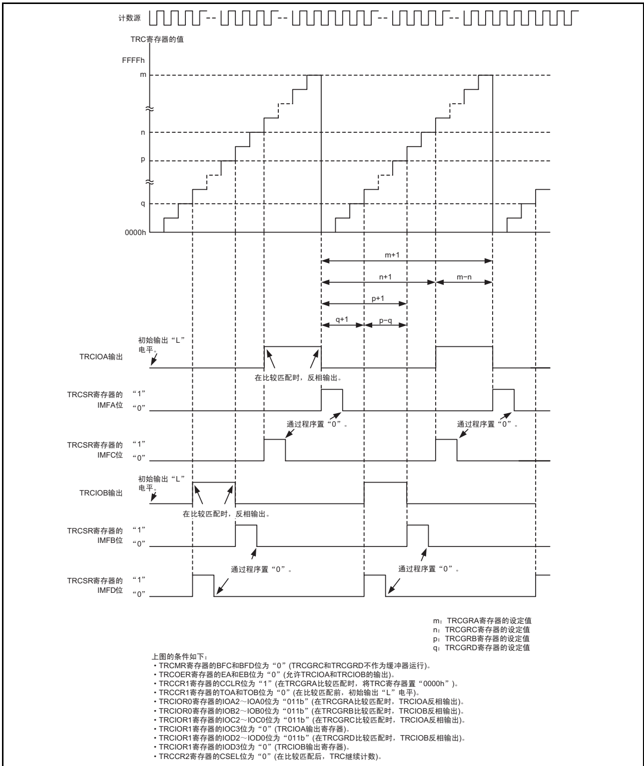
图 18.12 将 TRCGRC 和 TRCGRD 分别用于 TRCIOA 引脚和 TRCIOB 引脚的输出控制时的运行例子
