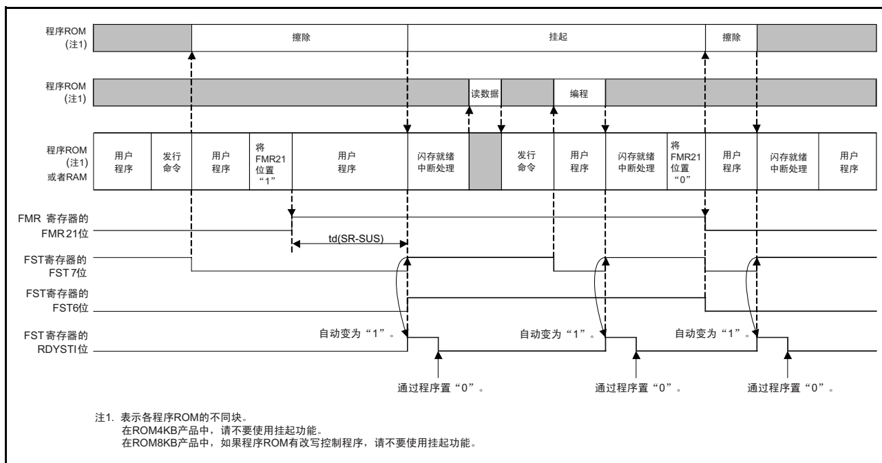
图 25.2 挂起的相关时序
