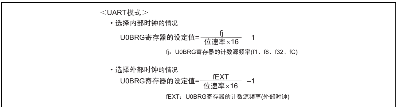
图 20.8 U0BRG 寄存器的设定值的计算式
