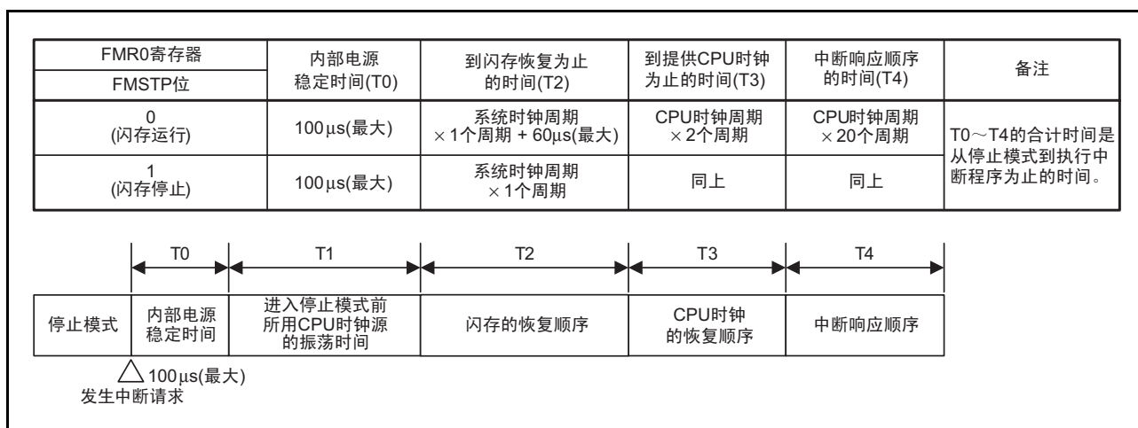
图 9.8 从停止模式到执行中断程序的时间
