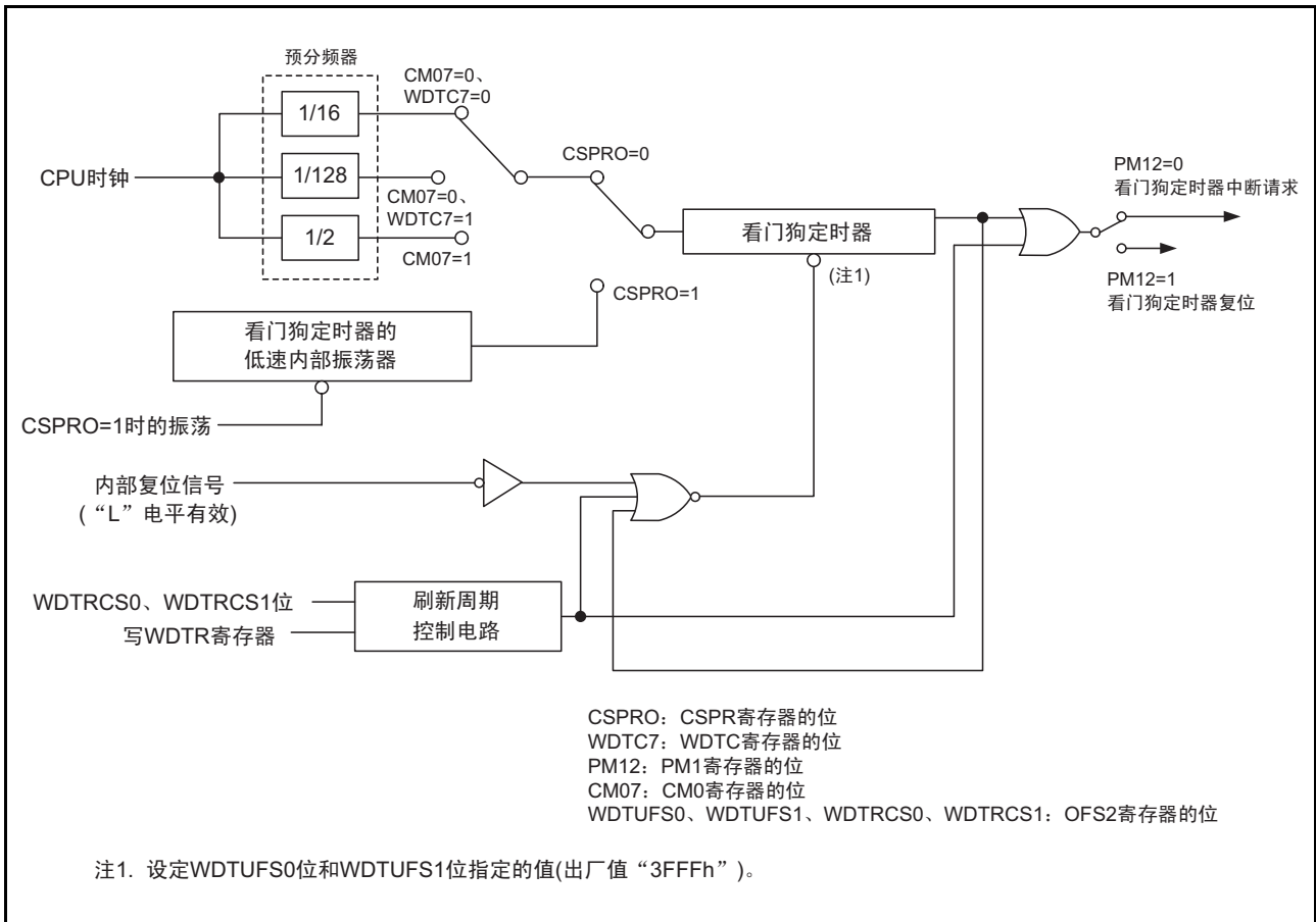
图 14.1 看门狗定时器的框图
