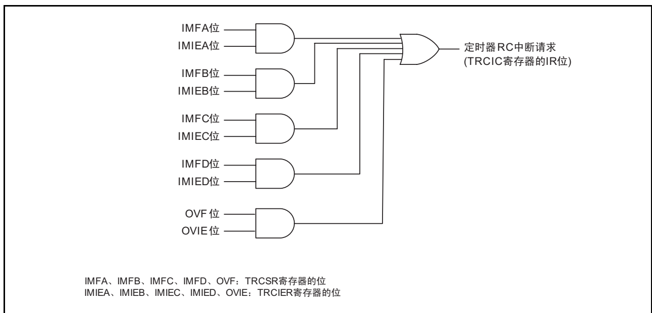
图 18.20 定时器 RC 中断的框图
