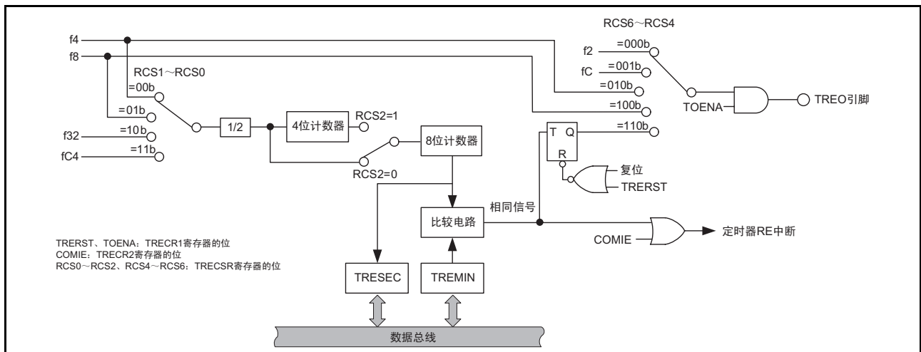
图 19.4 输出比较模式的框图
