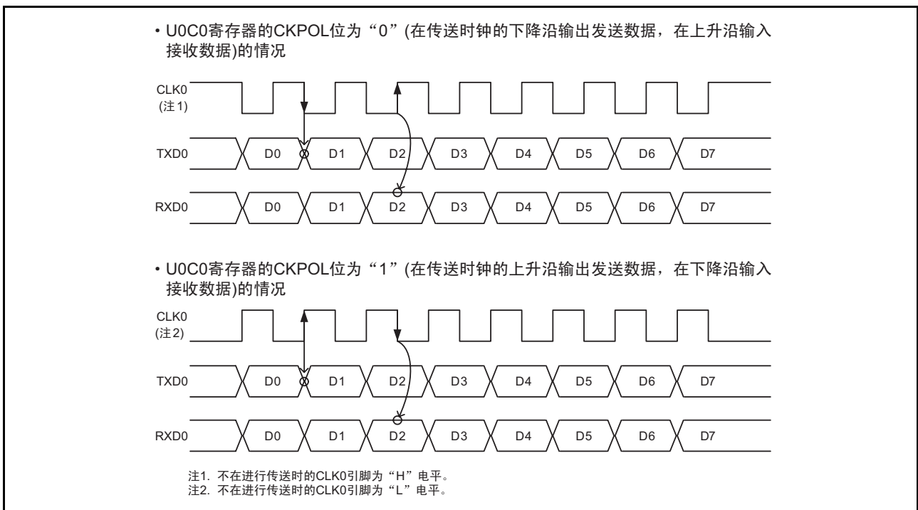
图 20.4 传送时钟的极性
