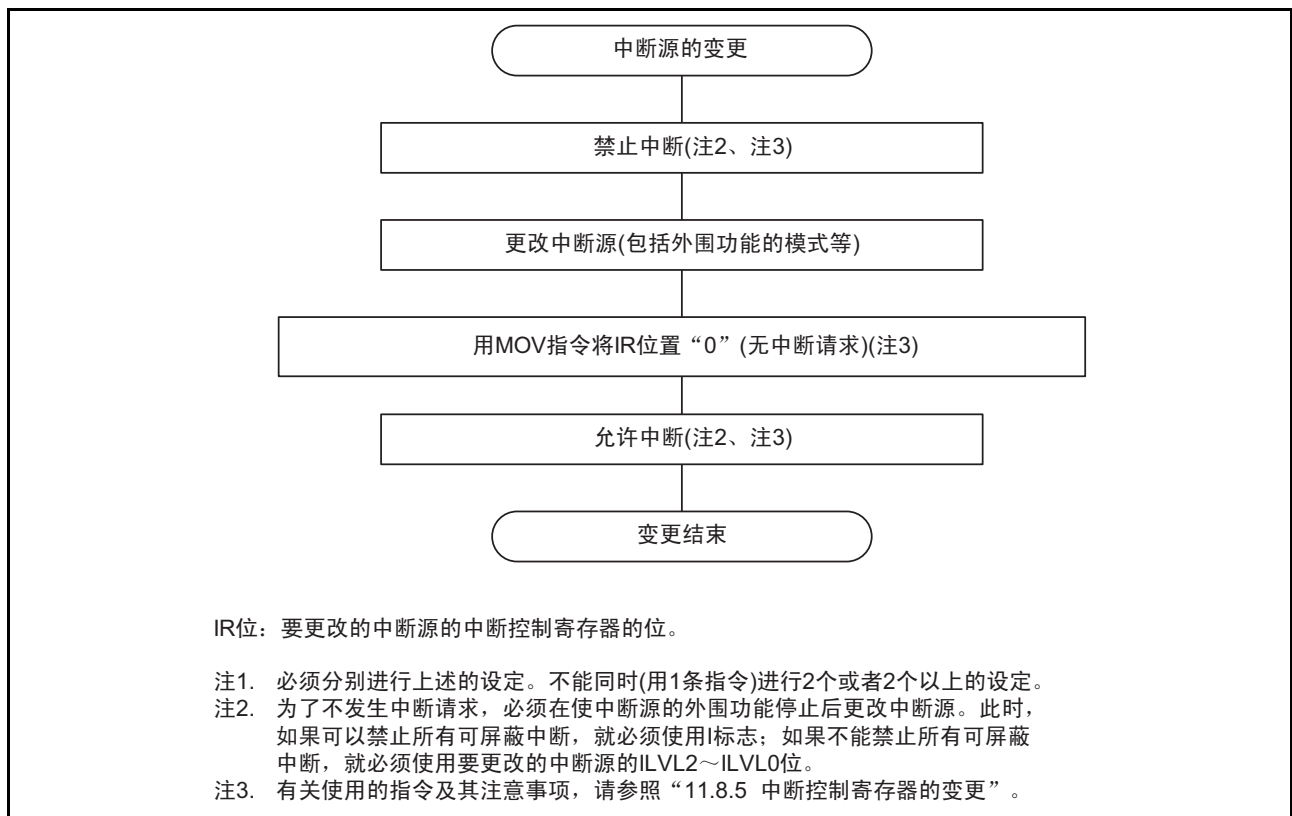
图 11.12 中断源的变更步骤例子
