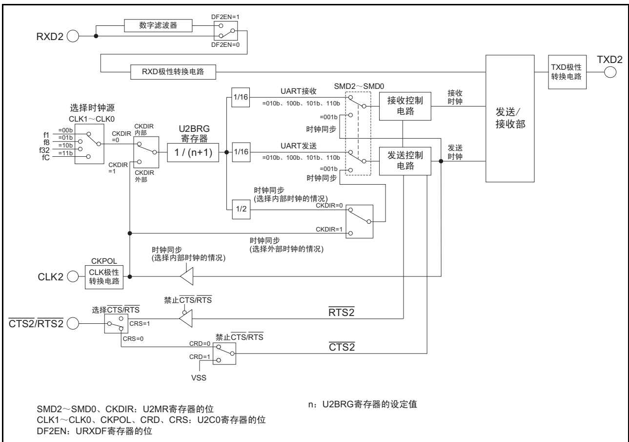
图 21.1 UART2 的框图
