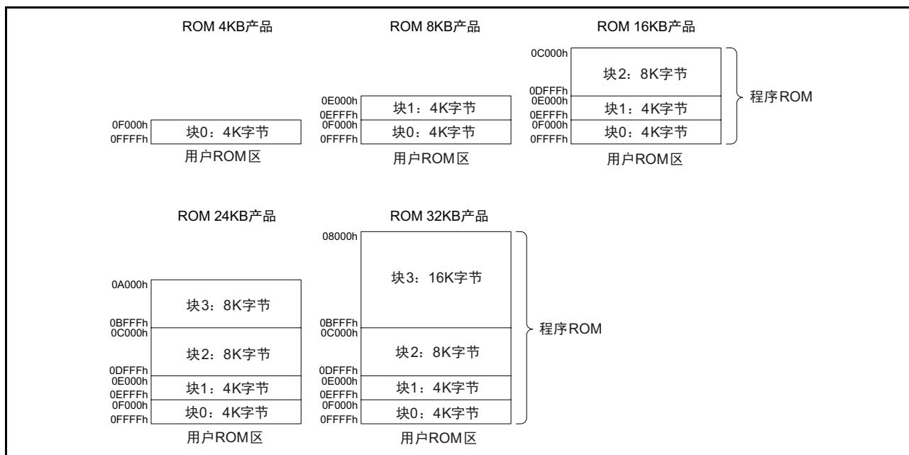
图 25.1 R8C/33D 群的闪存框图
