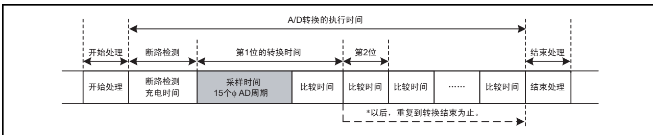
图 22.2 A/D 转换时序图
