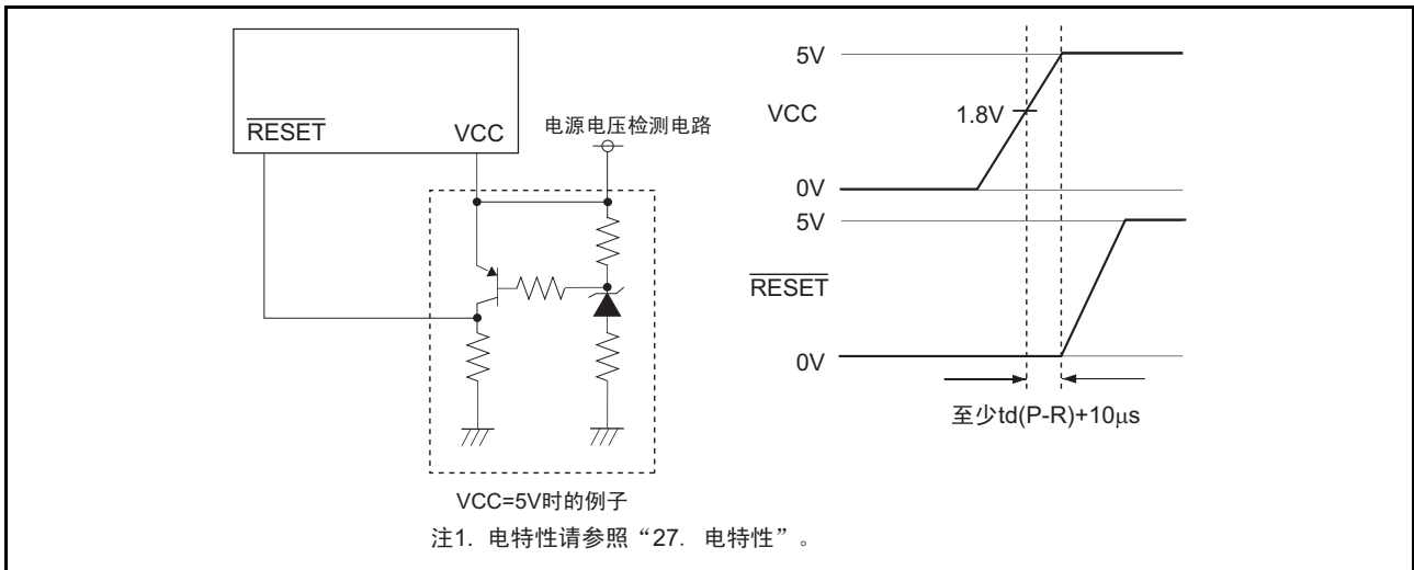
图 5.5 硬件复位的电路例子（外接电源电压检测电路的使用例子）和运行
