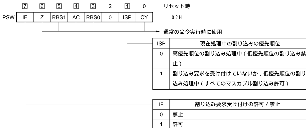
図18 - 13 プログラム・ステータス・ワードの構成
