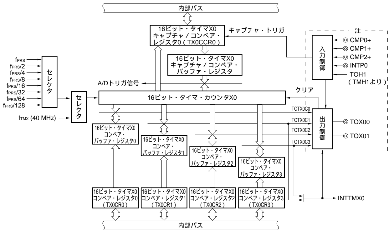
図6 - 1 16ビット・タイマX0のブロック図
