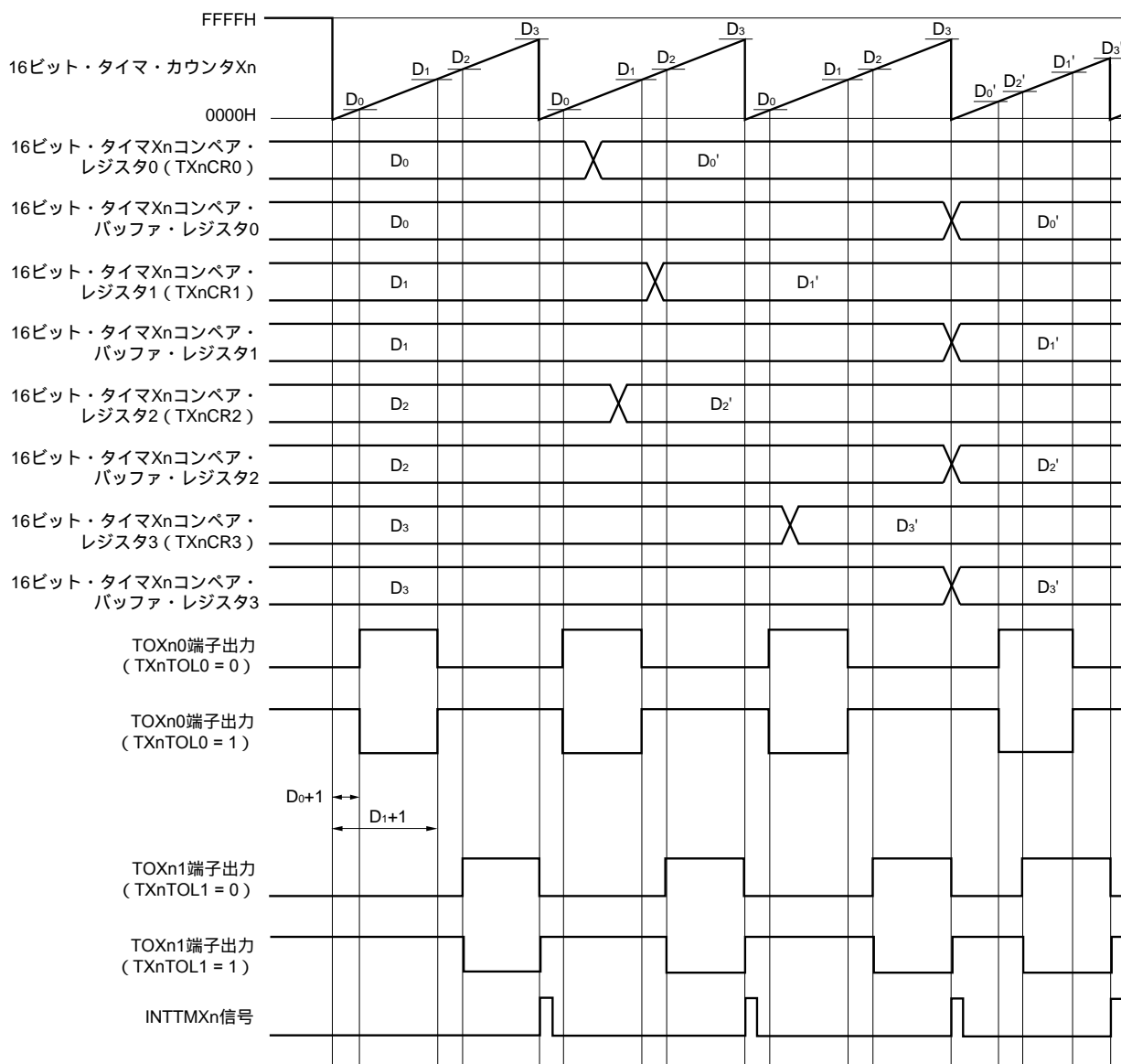
図6 - 30 PWM出力タイミング (TMXn単体動作, PWM出力: TOXn0, TOXn1端子)
