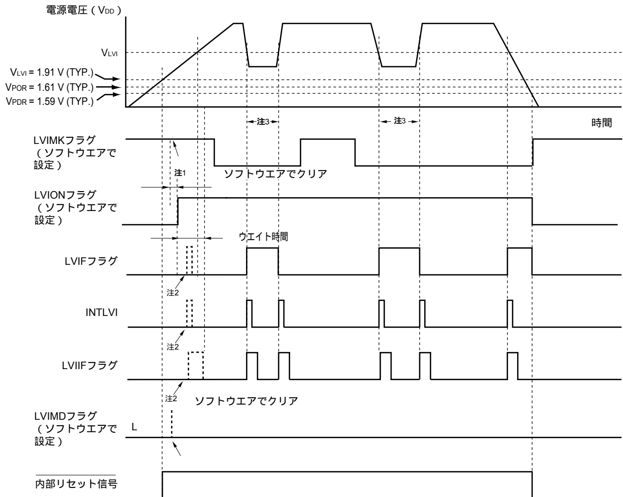
図22 - 7 割り込み信号発生タイミング (LVISTART = 1)
