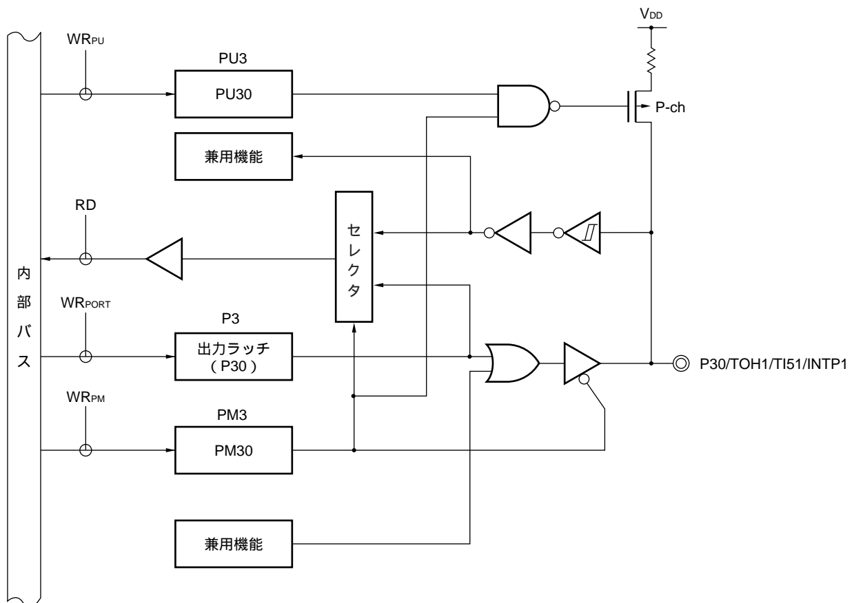
図4 - 12 P30のブロック図
