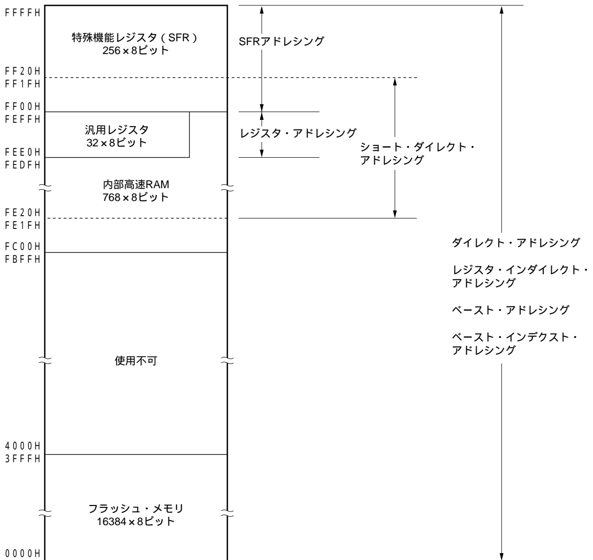
図3-6 データ・メモリとアドレッシングの対応 (μ PD78F0742, 78F0744, 78F0746, 78F0752, 78F0754, 78F0756)
