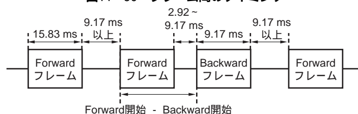
図14 - 30 フレーム間のタイミング
