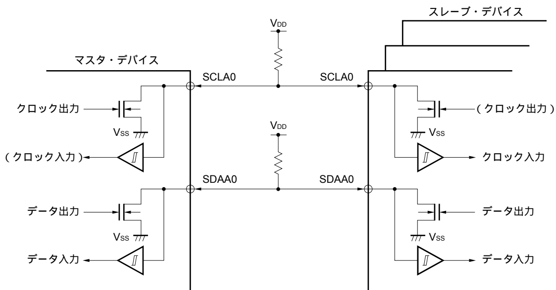
図15 - 14 端子構成図
