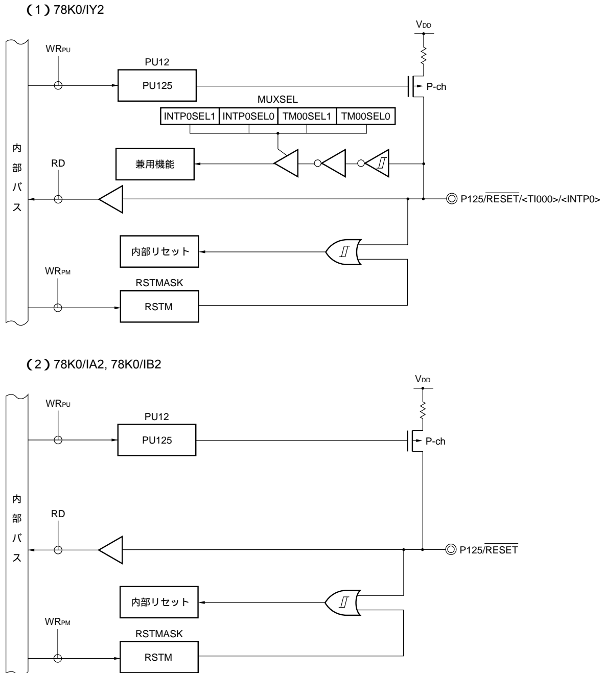
図4 - 24 P125のブロック図
