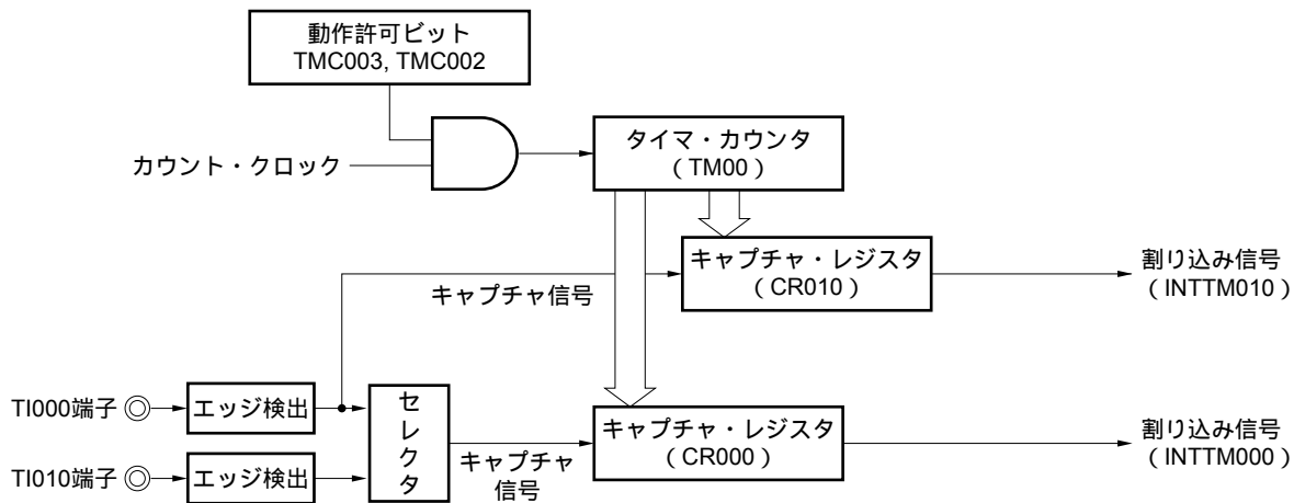
図7 - 37 フリー・ランニング・タイマ・モードのブロック図 (CR000 : キャプチャ・レジスタ / CR010 : キャプチャ・レジスタ)
