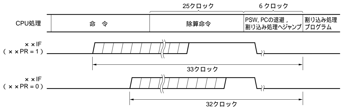
図18 - 16 割り込み要求の受け付けタイミング (最大時間)
