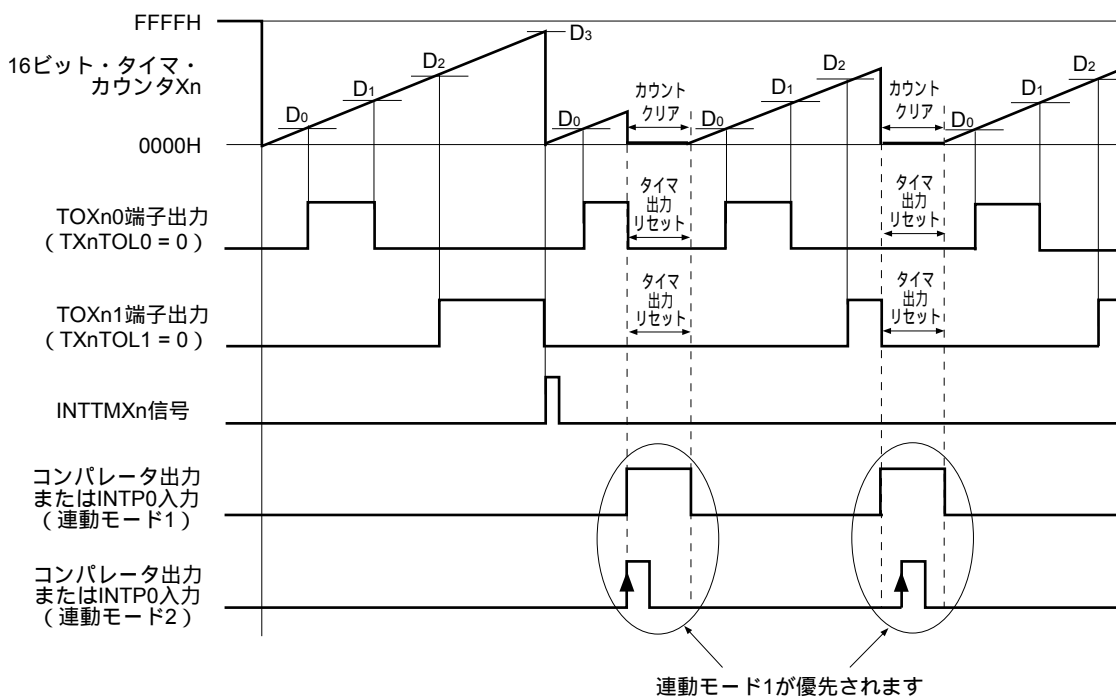
図6-52 連動モード1と連動モード2競合時のタイミング
