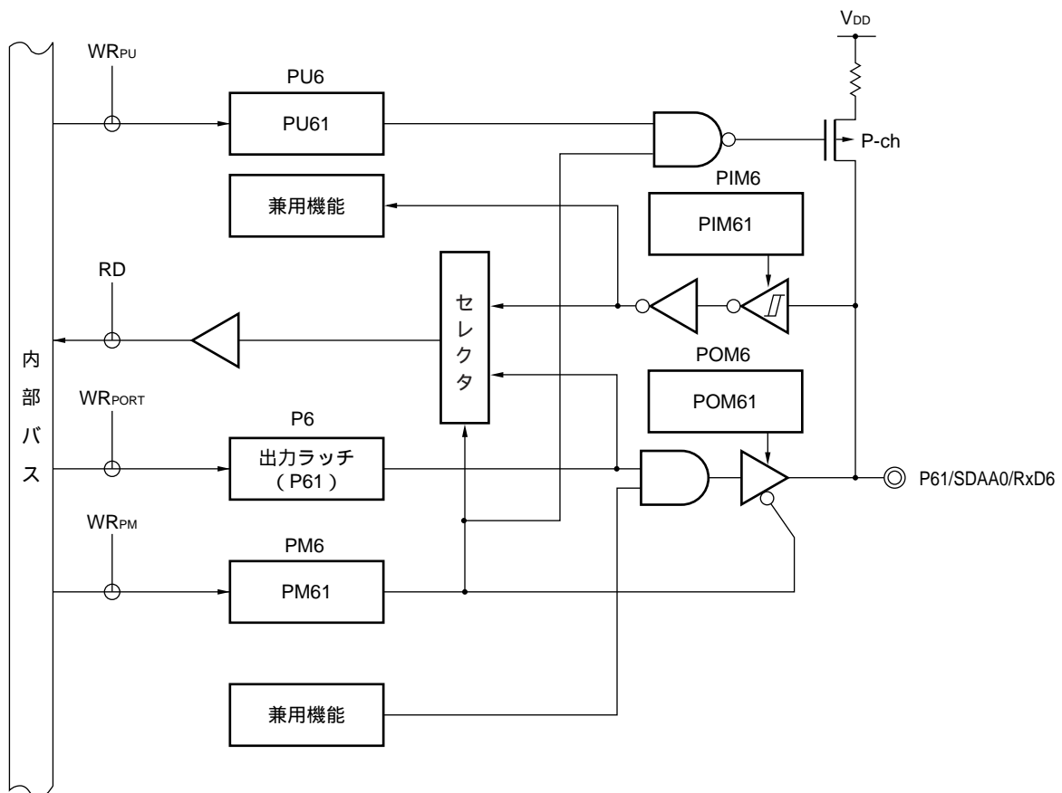
図4-21 P61のブロック図
