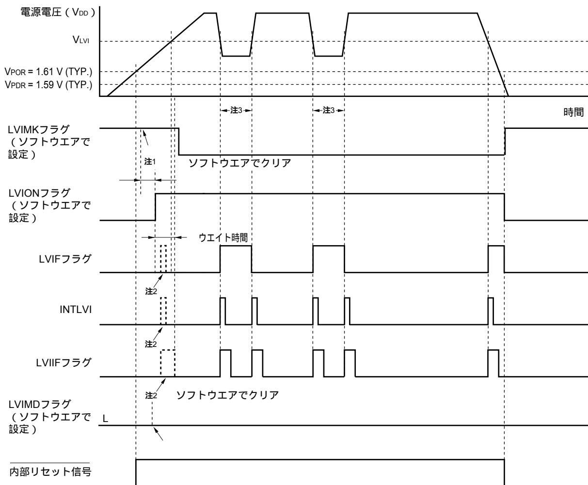
図22 - 6 割り込み信号発生タイミング (LVISTART = 0)
