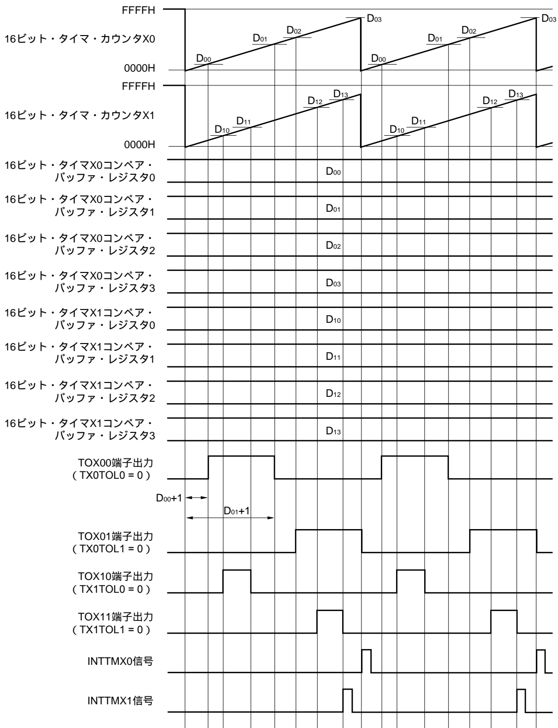
図6 - 34 PWM出力タイミング (同期スタート/クリア・モード, TMX0デュアル出力, TMX1デュアル出力)
