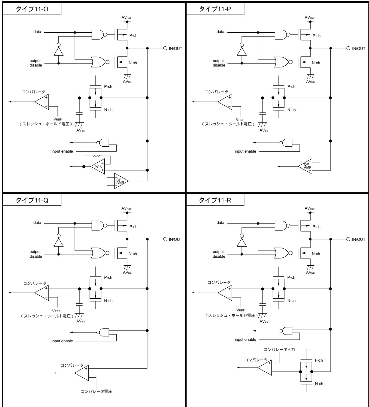
図2 - 1 端子の入出力回路一覧 (2/3)
