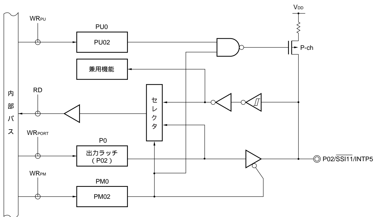
図4 - 3 P02のブロック図
