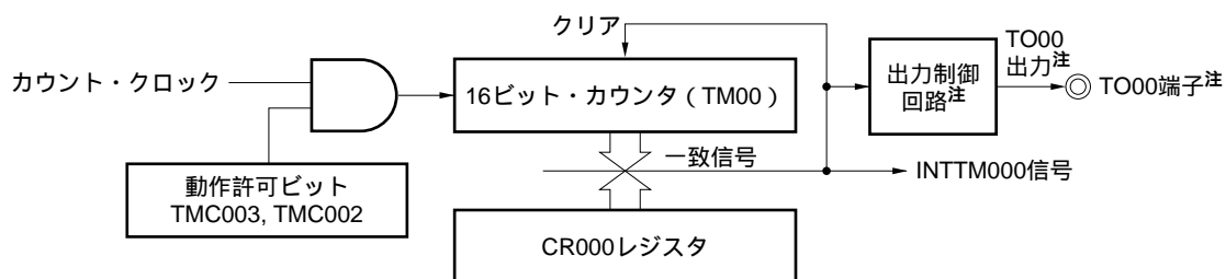
図7-16 方形波出力動作のブロック図
