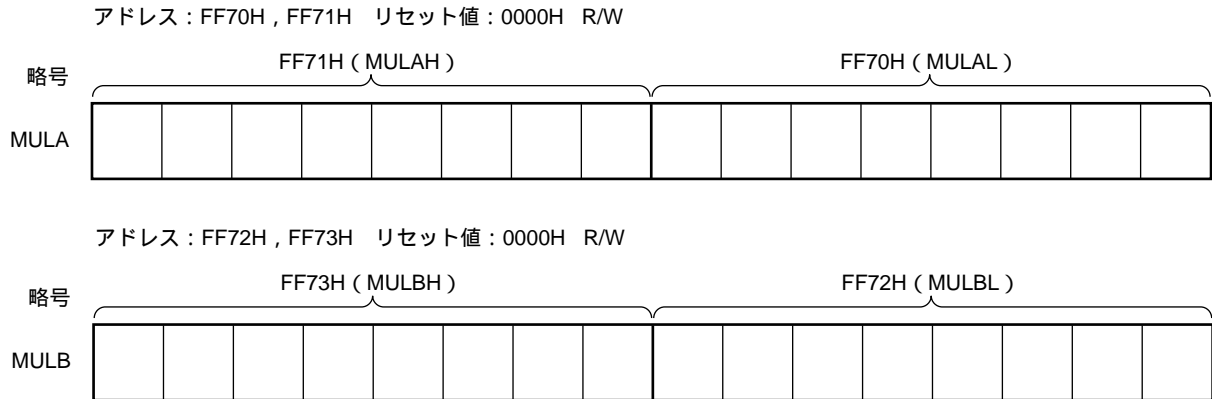
図17-3 乗算入力データ・レジスタA, B (MULA, MULB) のフォーマット
