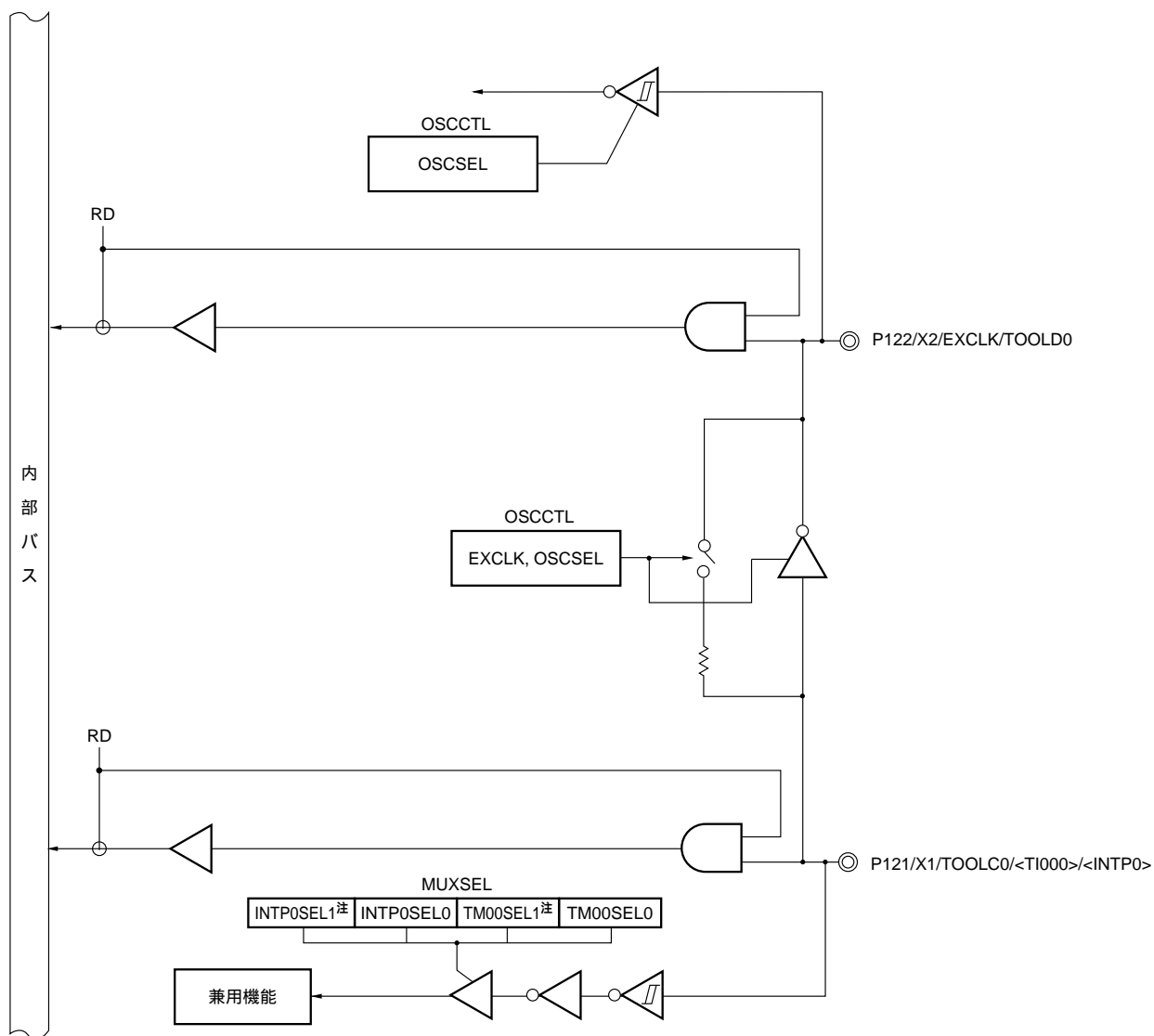
図4 - 23 P121, P122のブロック図
