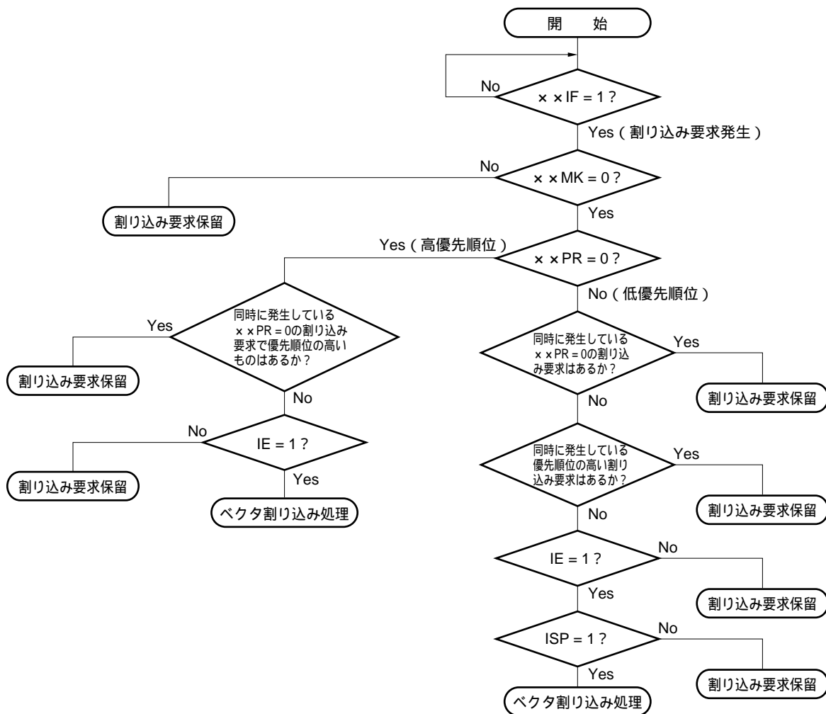
図18 - 14 割り込み要求受け付け処理アルゴリズム
