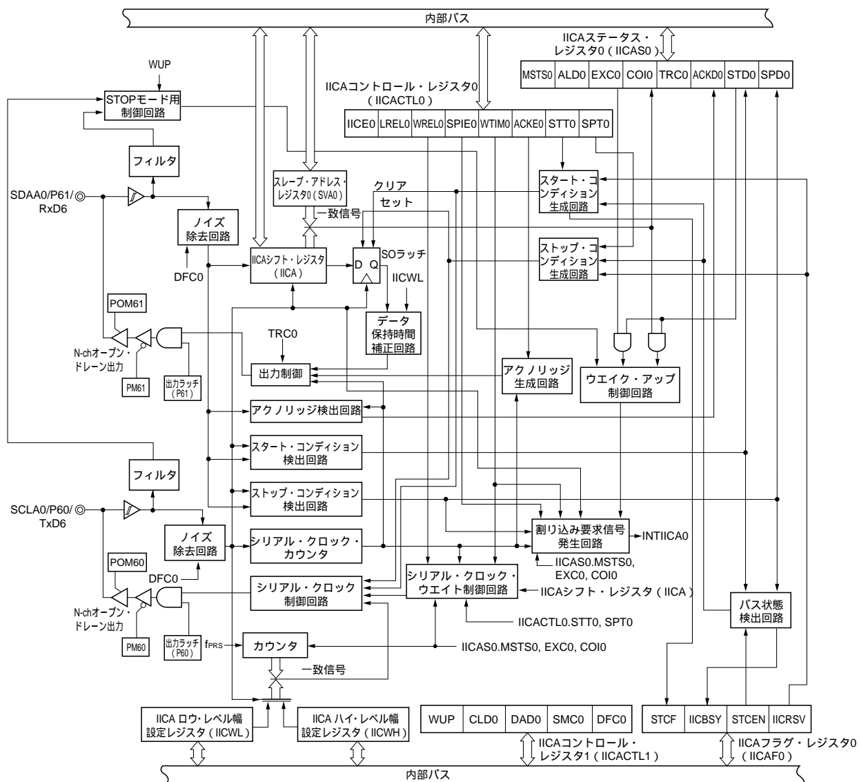
図15 - 1 シリアル・インタフェースIICAのブロック図
