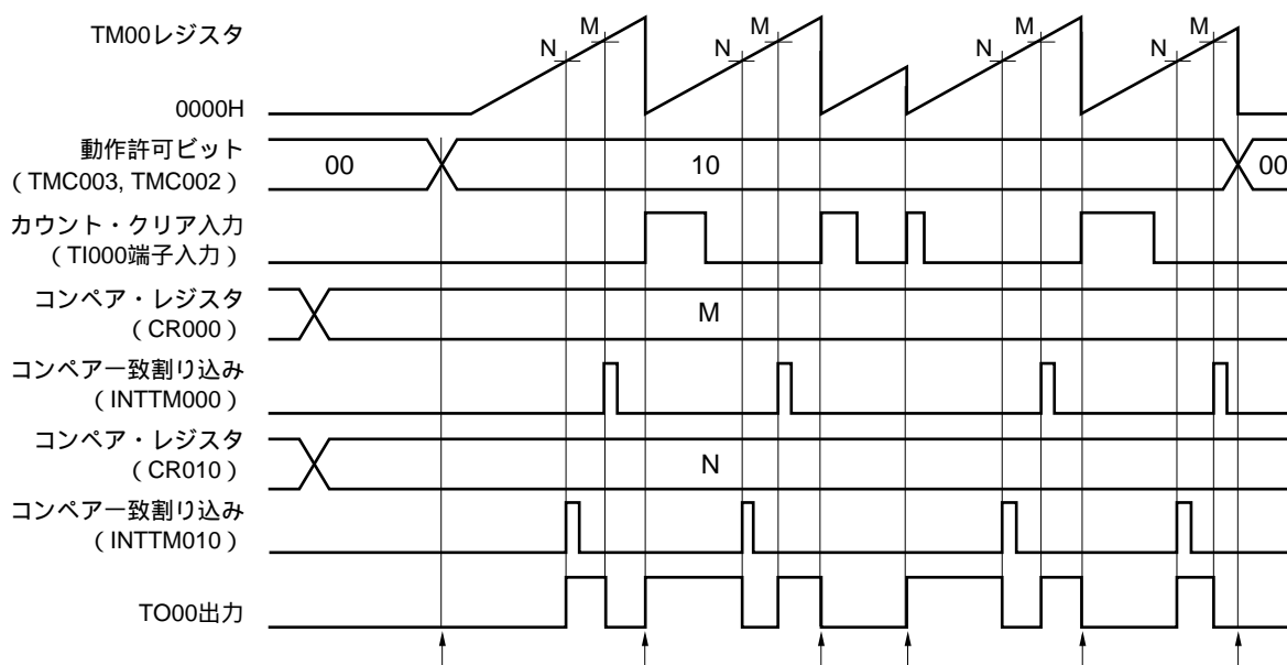
図7-32 TI000端子の有効エッジ入力によるクリア&スタート・モード動作時のソフトウェア処理例
