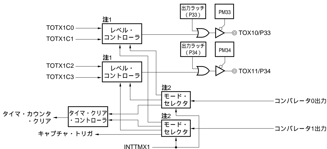
図6 - 45 16ビット・タイマX0とX1の出力構成のブロック図
