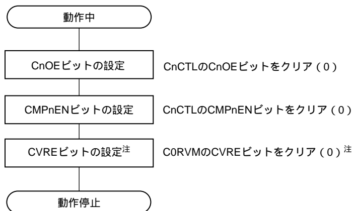
図13 - 14 コンパレータ動作停止の手順例
