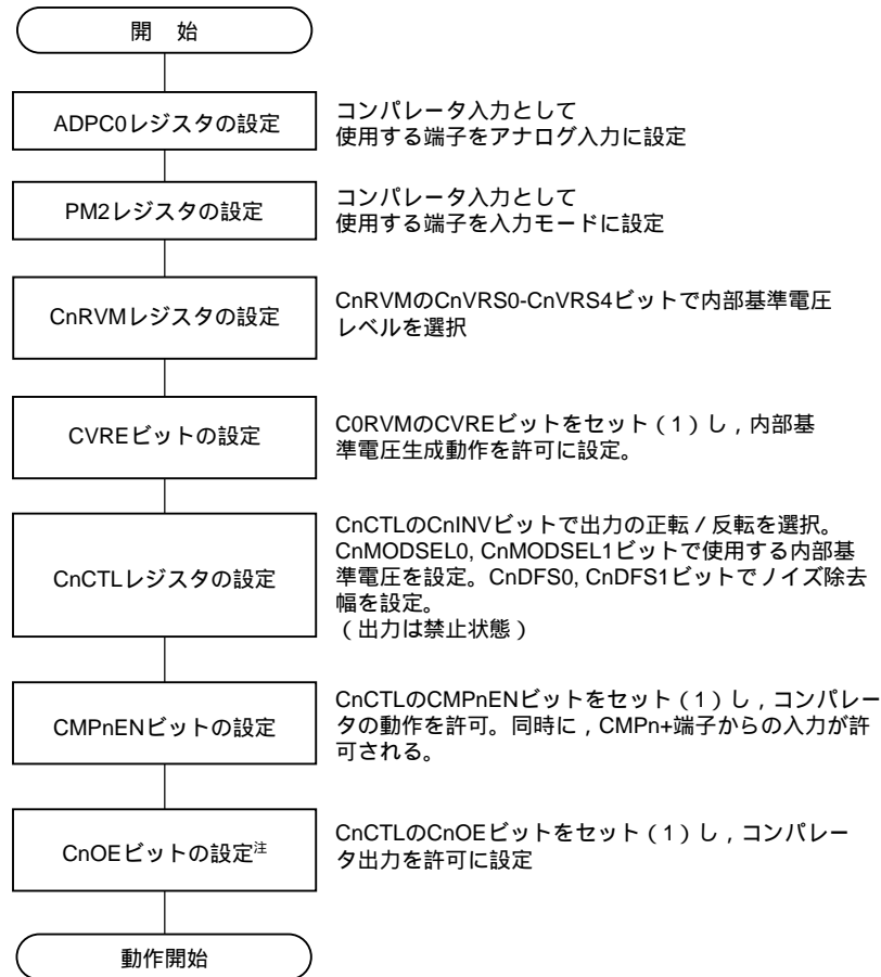
図13 - 11 コンパレータ動作開始の手順例（基準電圧に内部基準電圧を使用する場合）
