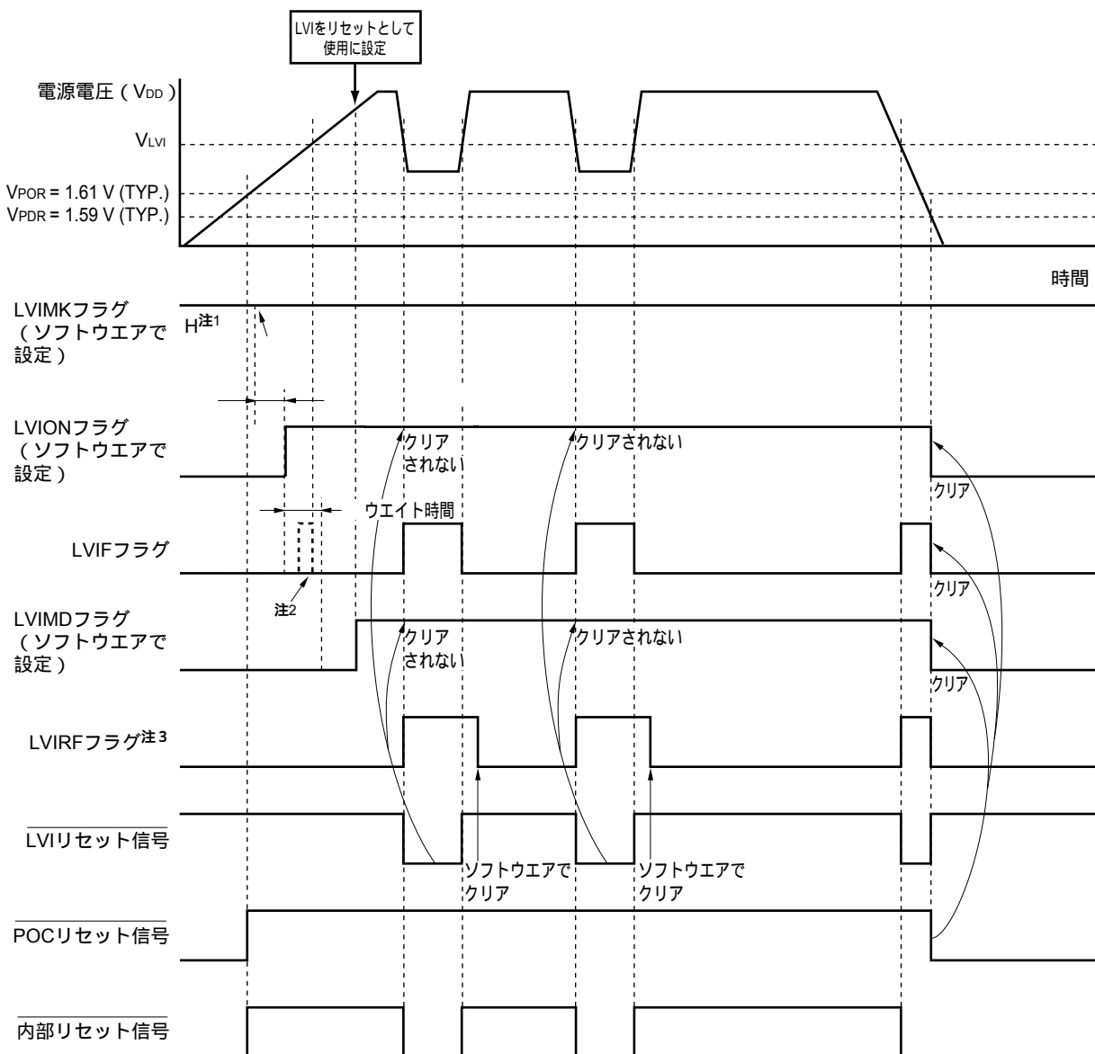
図22 - 4 内部リセット信号発生タイミング (LVISTART = 0)
