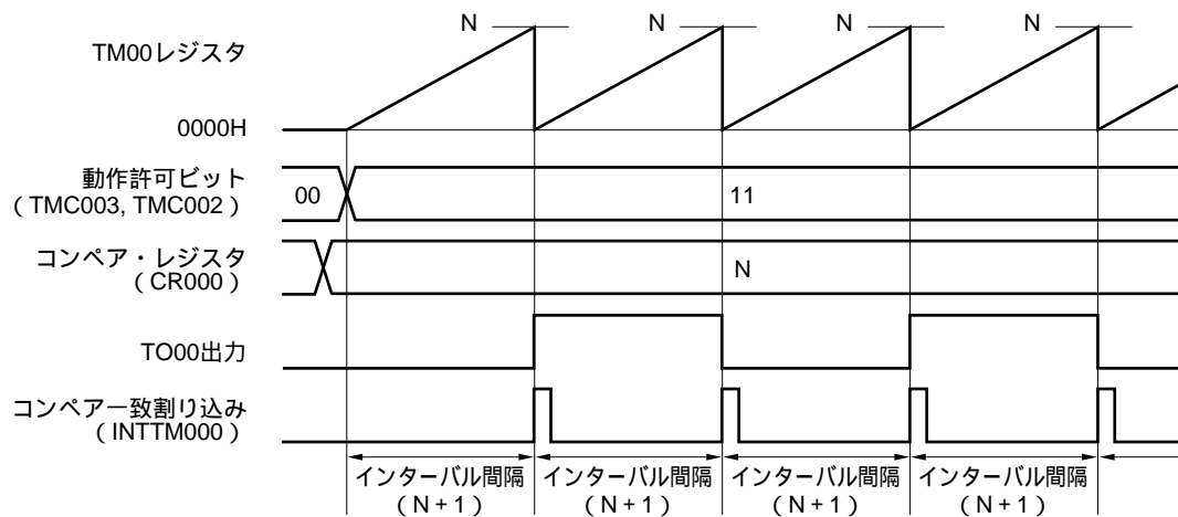
図7-17 方形波出力動作の基本タイミング例
