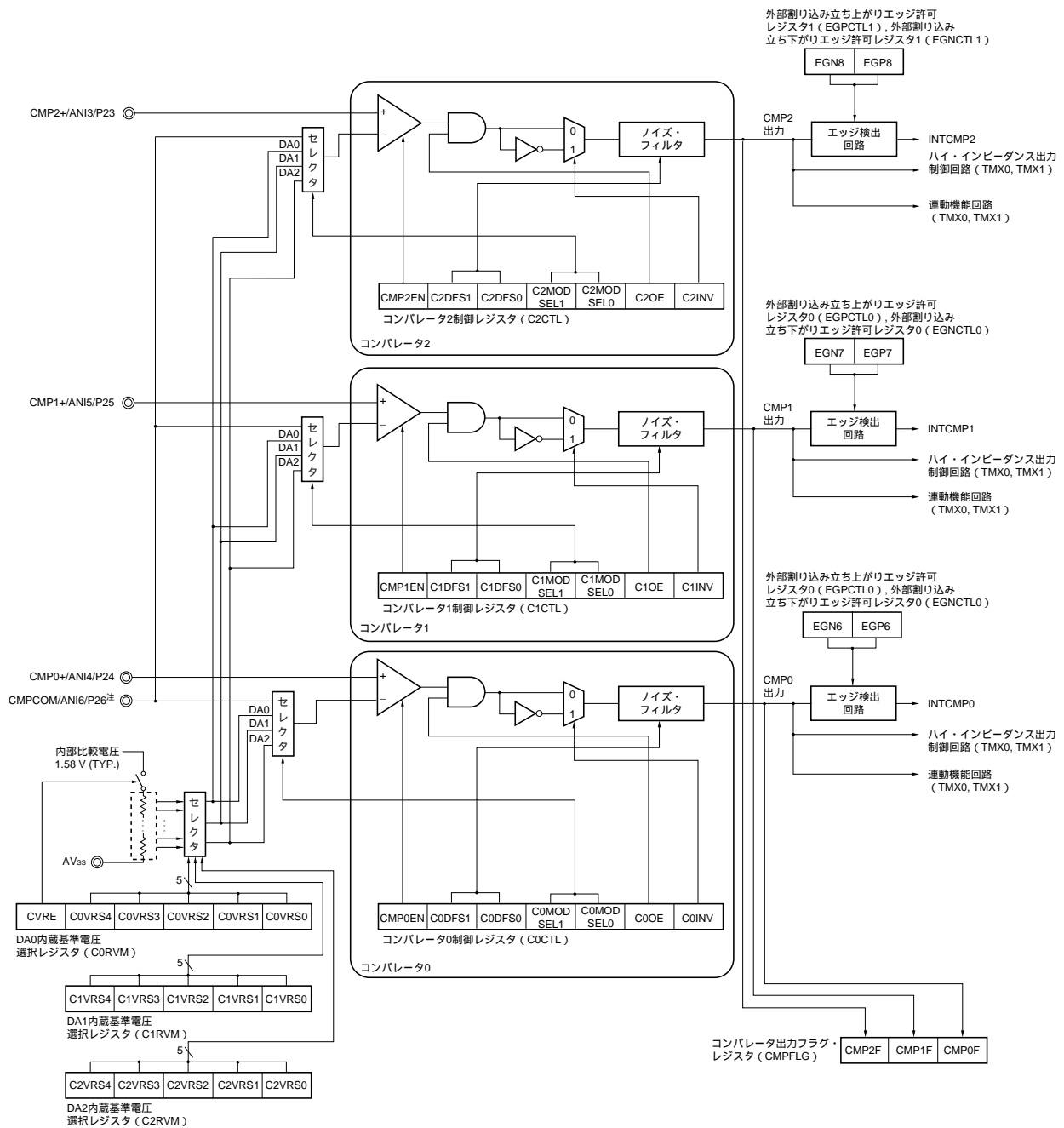
図13 - 1 コンパレータのブロック図
