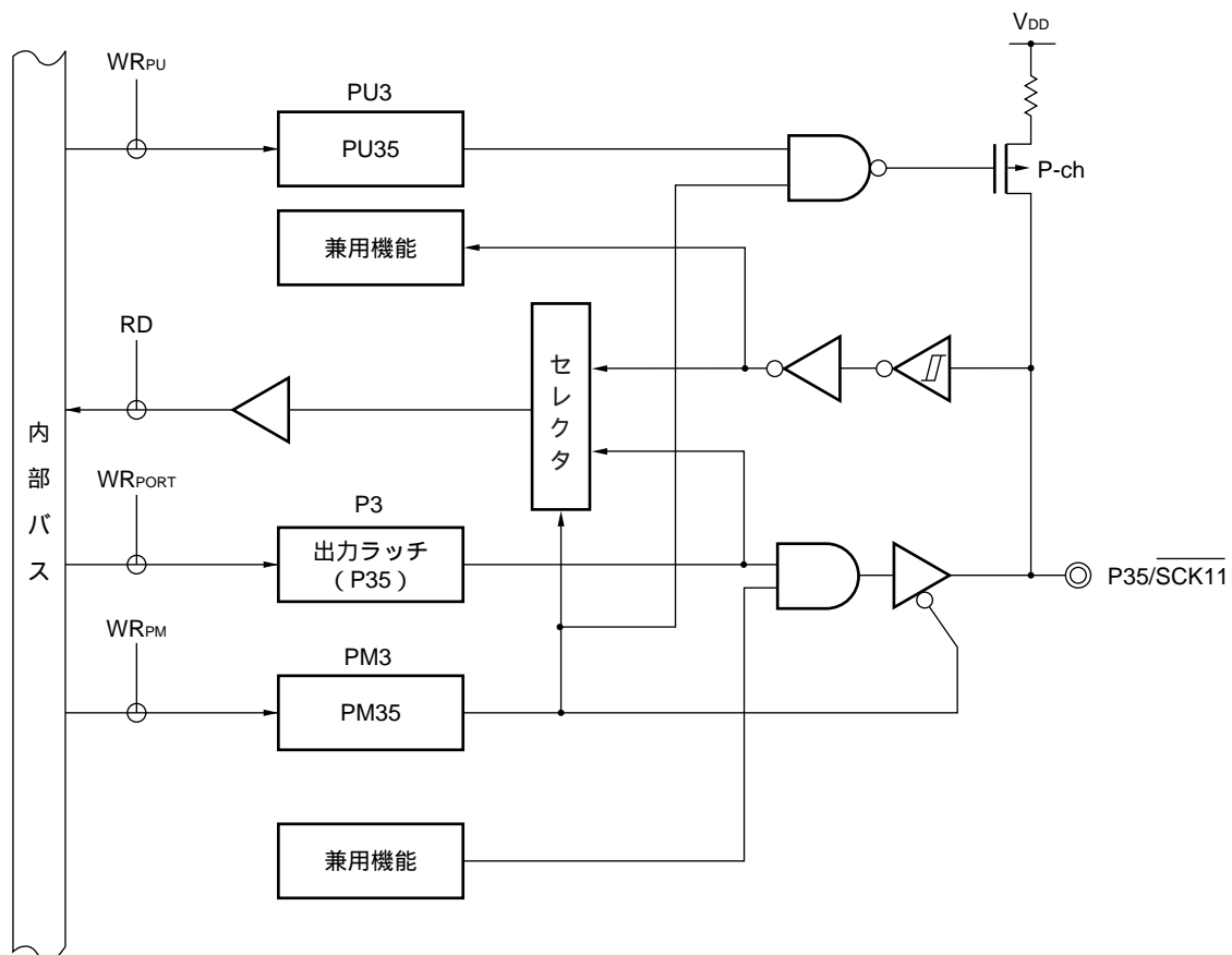
図4 - 17 P35のブロック図
