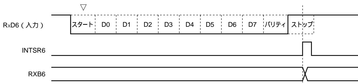
図14 - 21 受信完了割り込み要求タイミング
