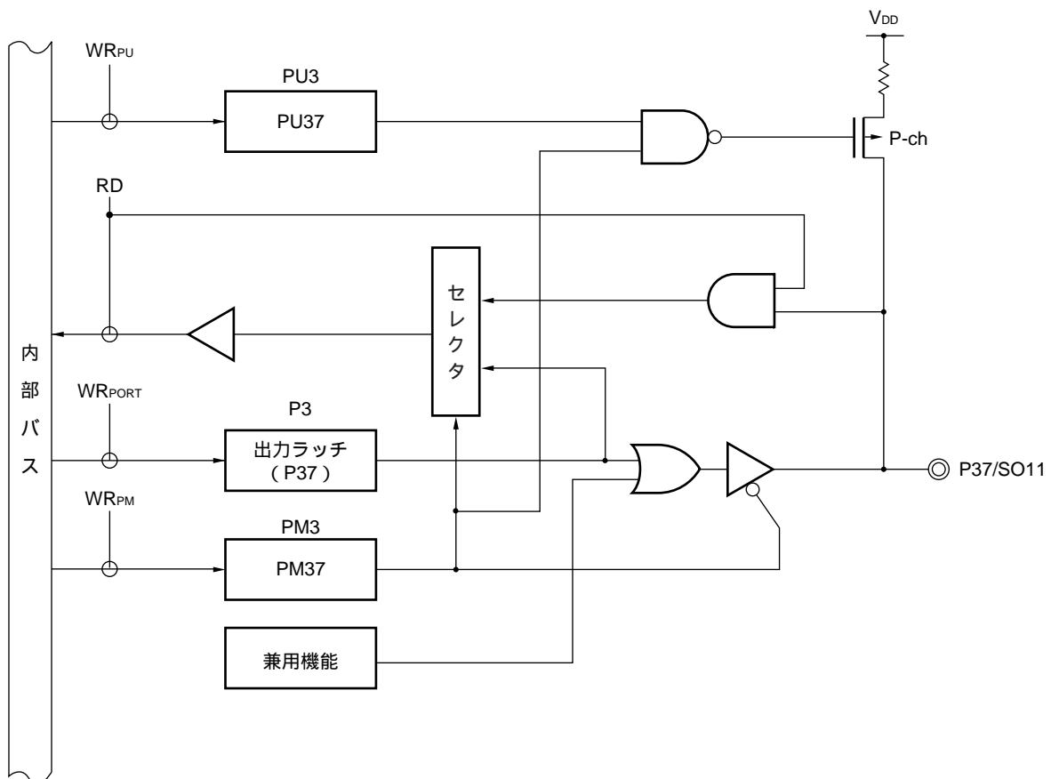
図4-19 P37のブロック図
