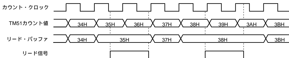
図8 - 12 8ビット・タイマ・カウンタ51 (TM51) のリード・タイミング
