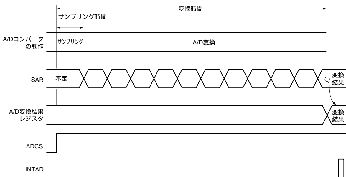
図11 - 15 A/Dコンバータの基本動作 (ソフトウェア・トリガ・モード)
