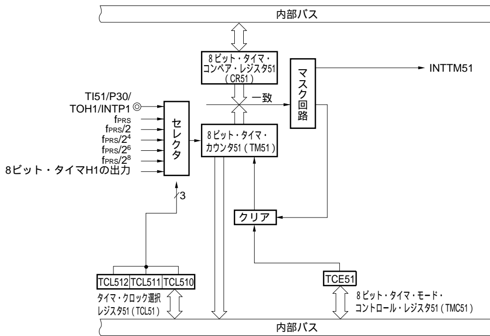
図8-1 8ビット・タイマ／イベント・カウンタ51のブロック図
