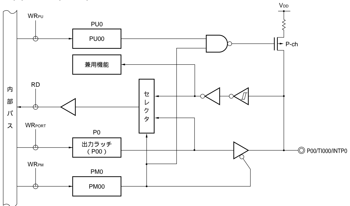
図4-1 P00のブロック図(2/2)
