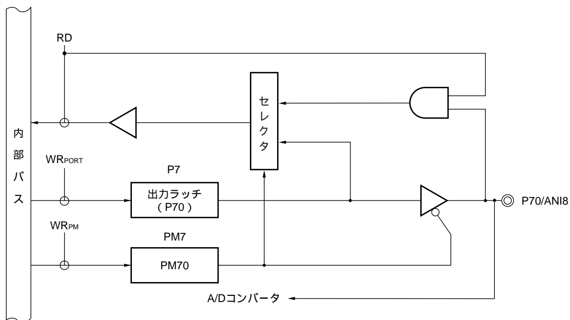
図4 - 22 P70のブロック図
