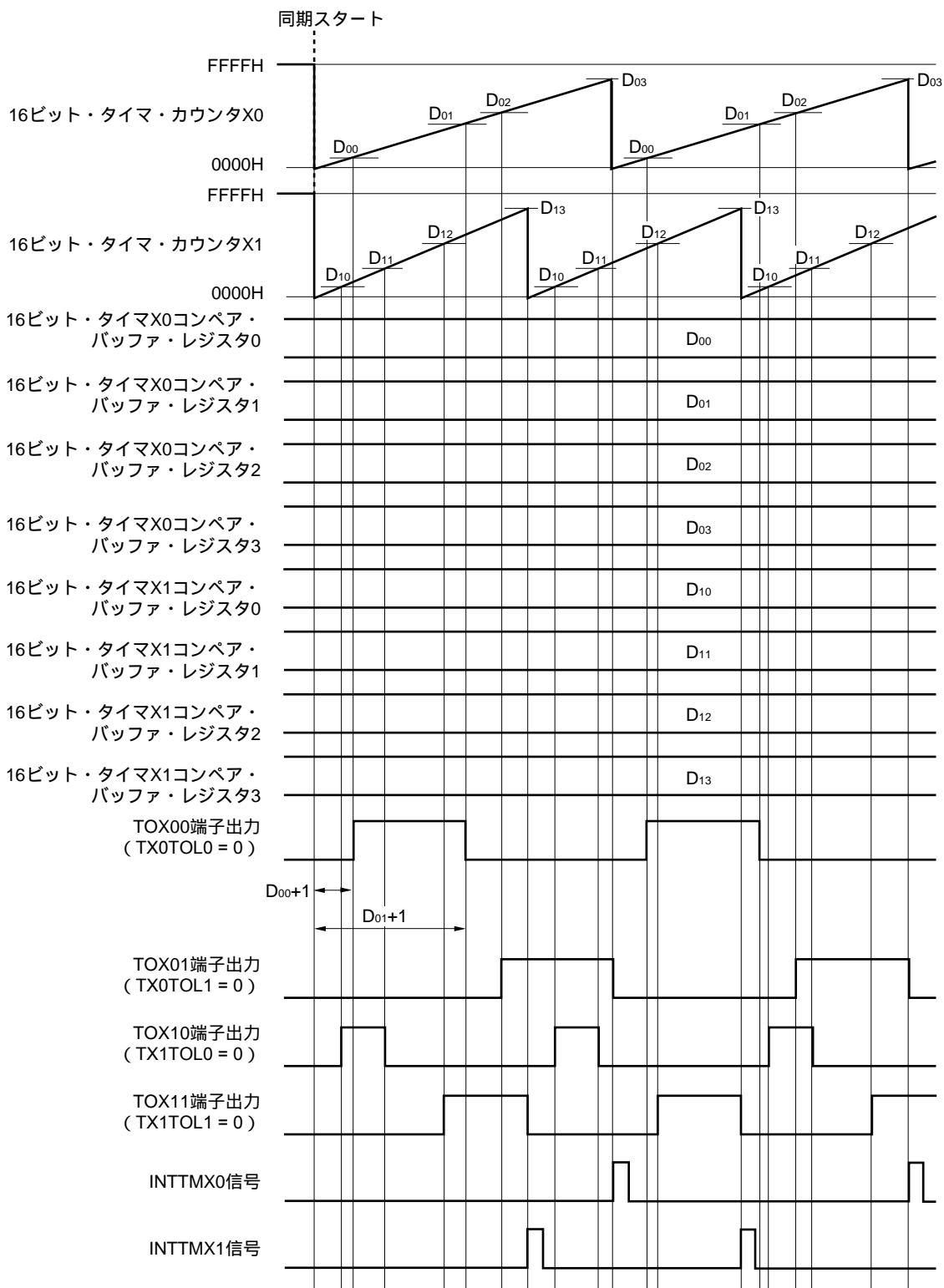
図6 - 32 PWM出力タイミング (同期スタート・モード, TMX0デュアル出力, TMX1デュアル出力)
