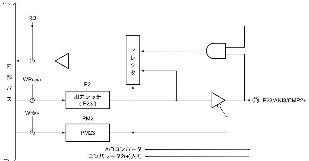
図4 - 7 P23のブロック図
