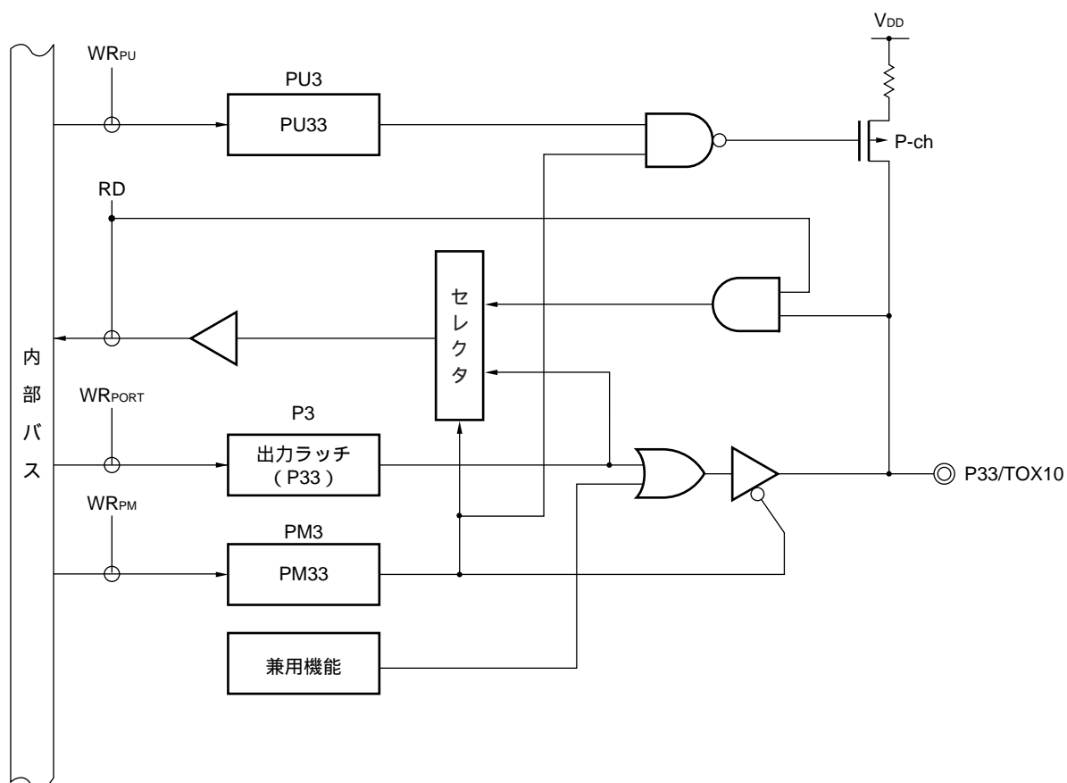
図4 - 15 P33のブロック図
