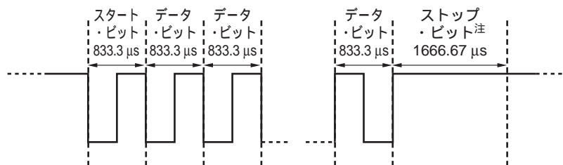
図14 - 29 フレーム内のタイミング
