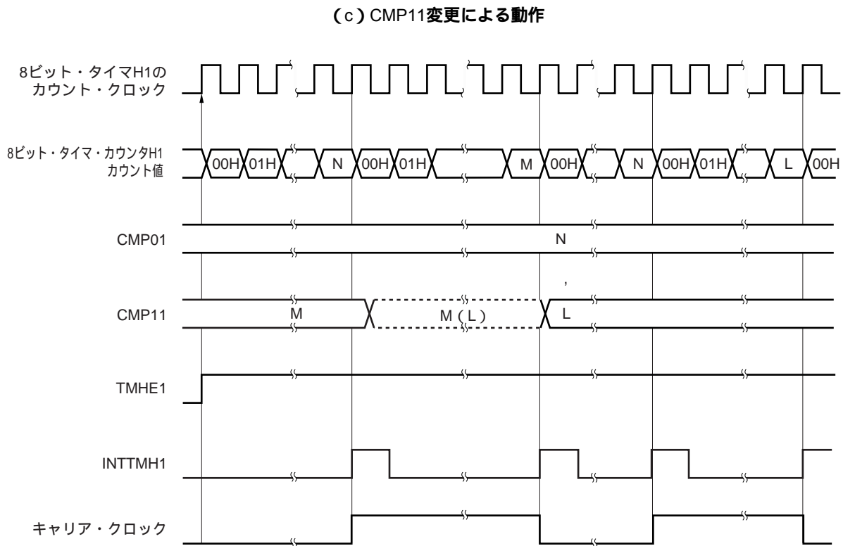
図9-15 キャリア・ジェネレータ・モード動作のタイミング (3/3)
