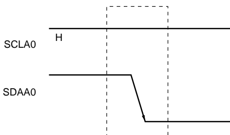
図15 - 16 スタート・コンディション
