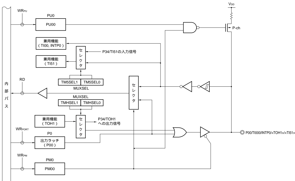
図4-1 P00のブロック図 (1/2)
