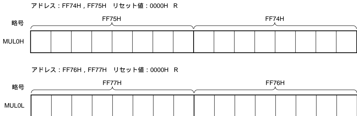
図17 - 2 16ビット上位乗算結果格納レジスタ, 16ビット下位乗算結果格納レジスタ (MUL0H, MUL0L) のフォーマット
