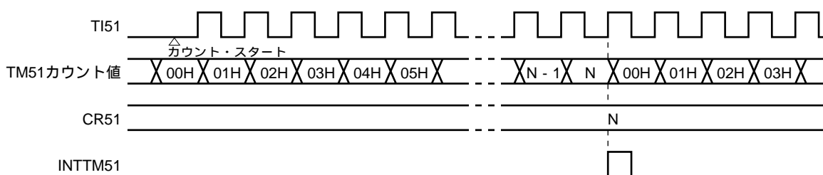
図8 - 10 外部イベント・カウンタ動作のタイミング (立ち上がりエッジ指定時)
