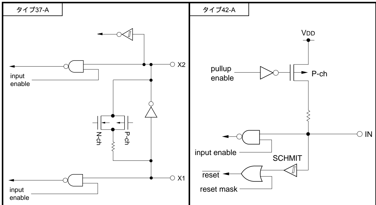
図2 - 1 端子の入出力回路一覧 (3/3)
