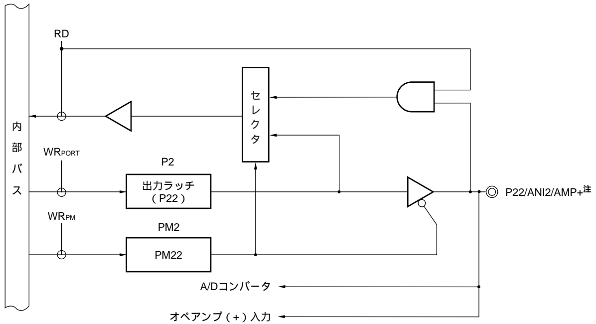
図4 - 6 P22のブロック図
