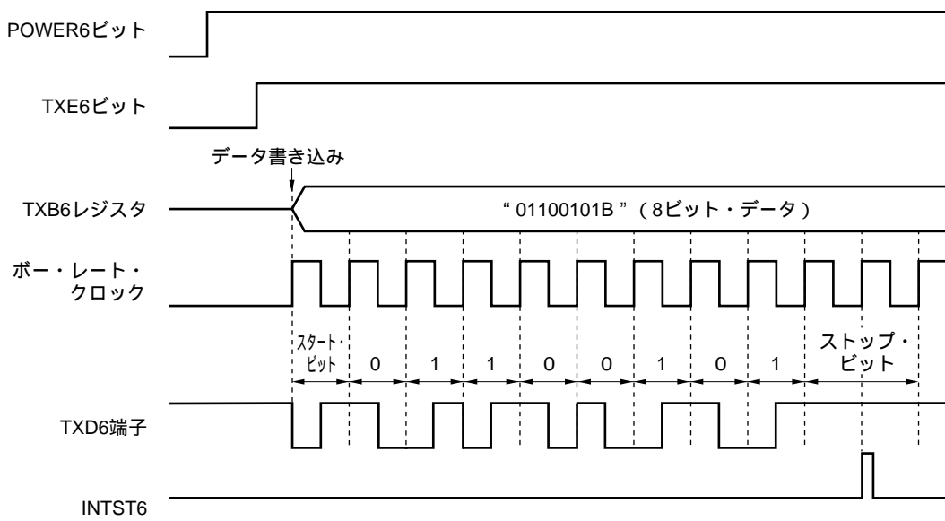
図14 - 32 DALI通信 (スレーブ送信) のタイミング例
