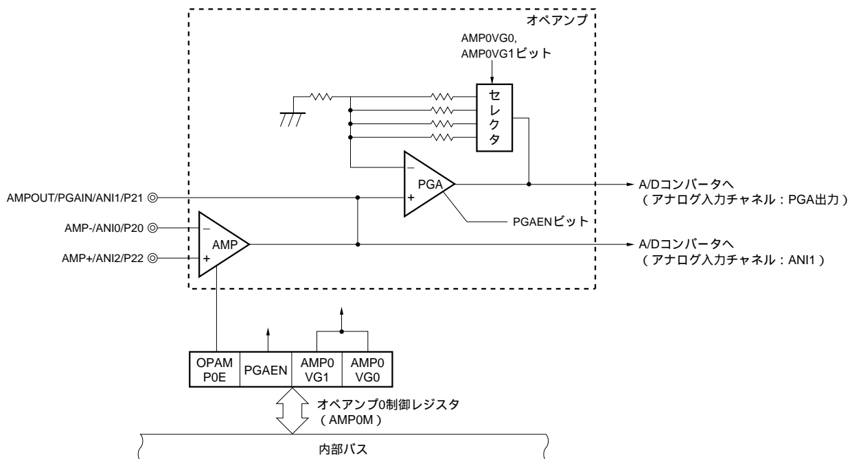
図12-1 オペアンプのブロック図
