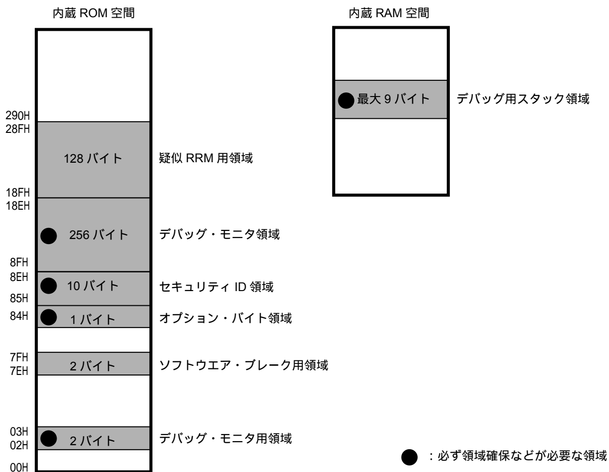
図26 - 2 QB-MINI2が使用する予約領域
