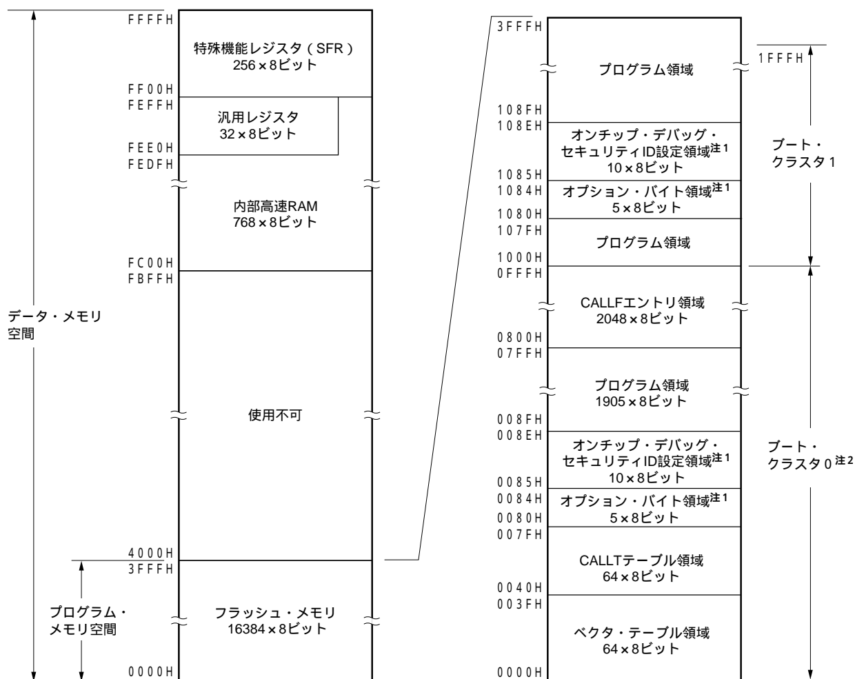
図3-3 メモリ・マップ (μ PD78F0742, 78F0744, 78F0746, 78F0752, 78F0754, 78F0756)
