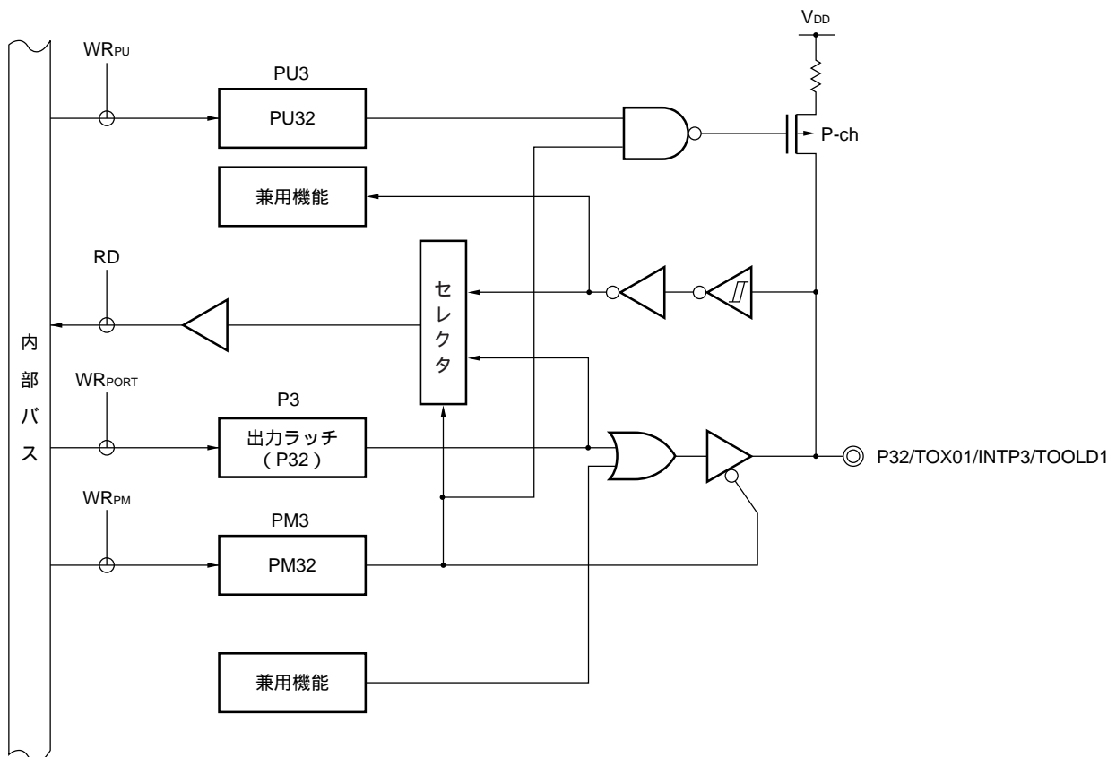
図4 - 14 P32のブロック図
