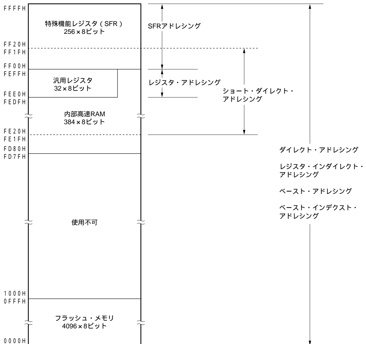
図3-4 データ・メモリとアドレッシングの対応 ( \mu PD78F0740, 78F0750)
