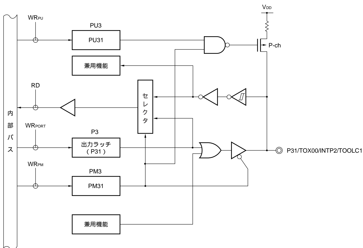
図4 - 13 P31のブロック図
