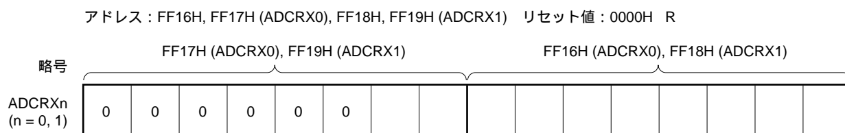
図11 - 8 TMXn同期用10ビットA/D変換結果レジスタ (ADCRXn) のフォーマット
