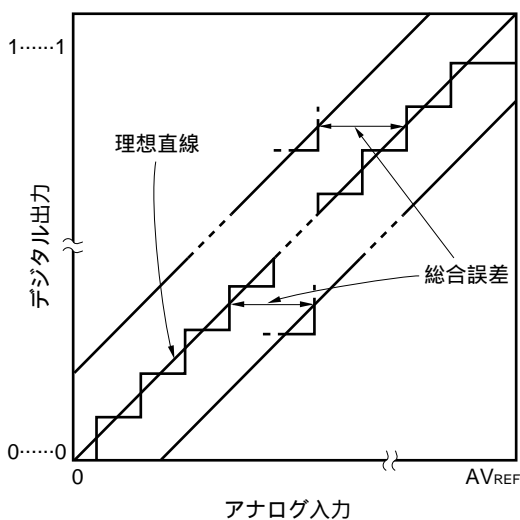
図11 - 19 総合誤差
