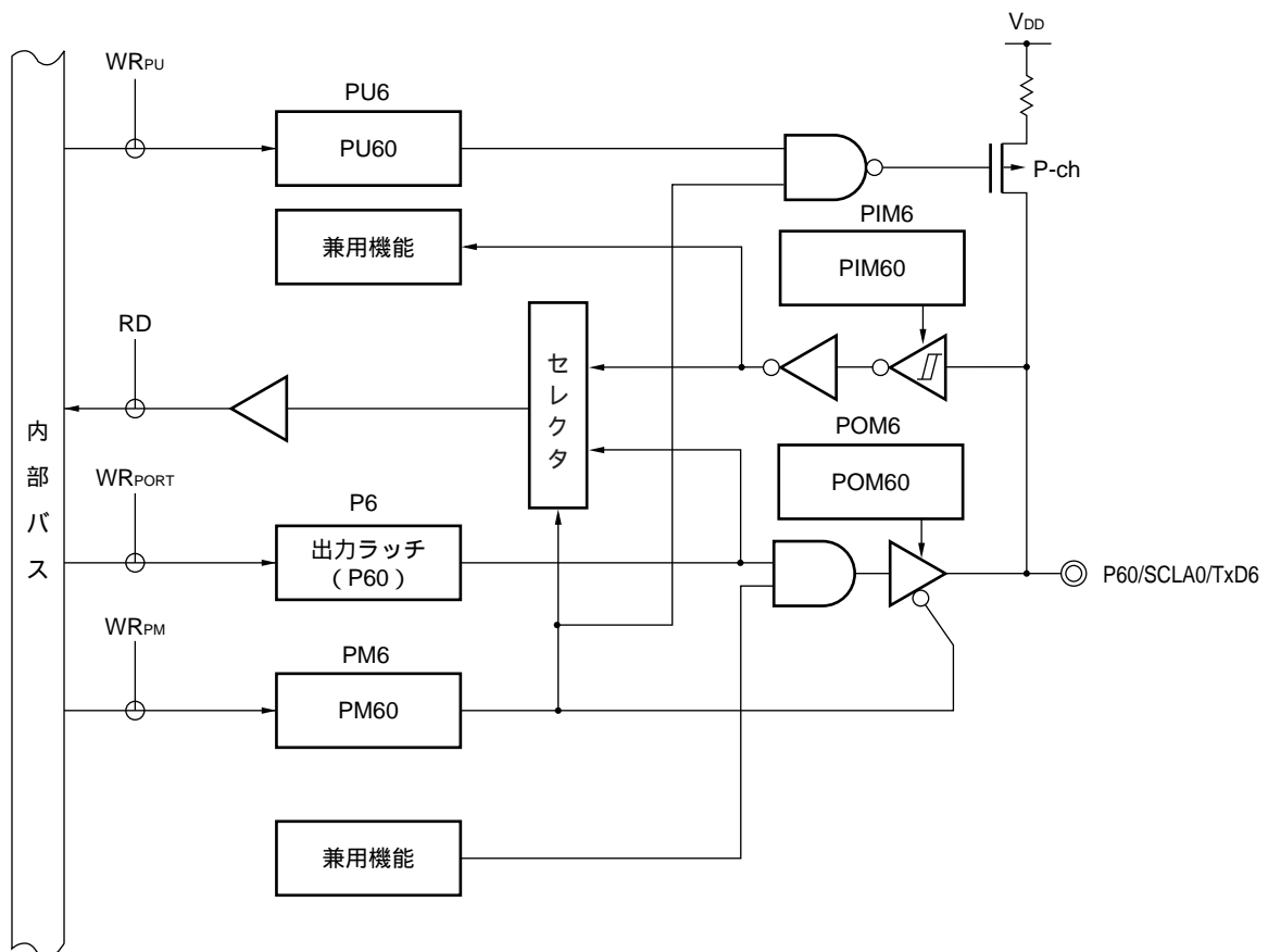
図4 - 20 P60のブロック図
