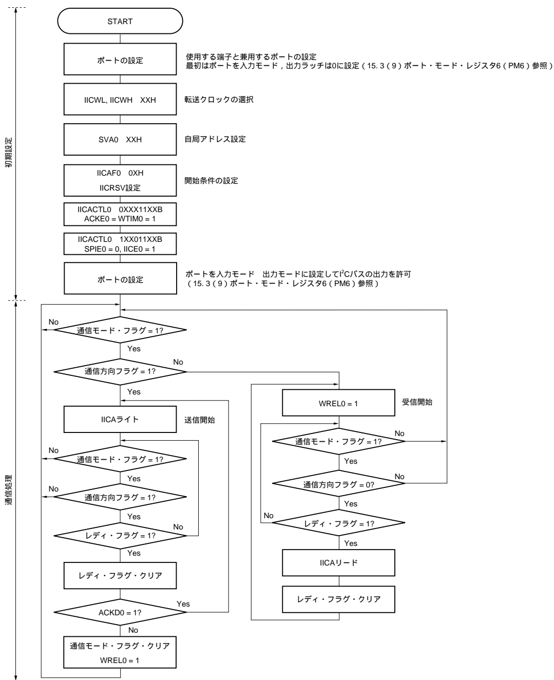
図15 - 31 スレーブ動作手順（1）
