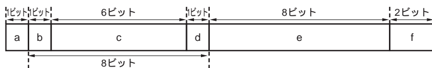
図14 - 27 Forwardフレームの構造
