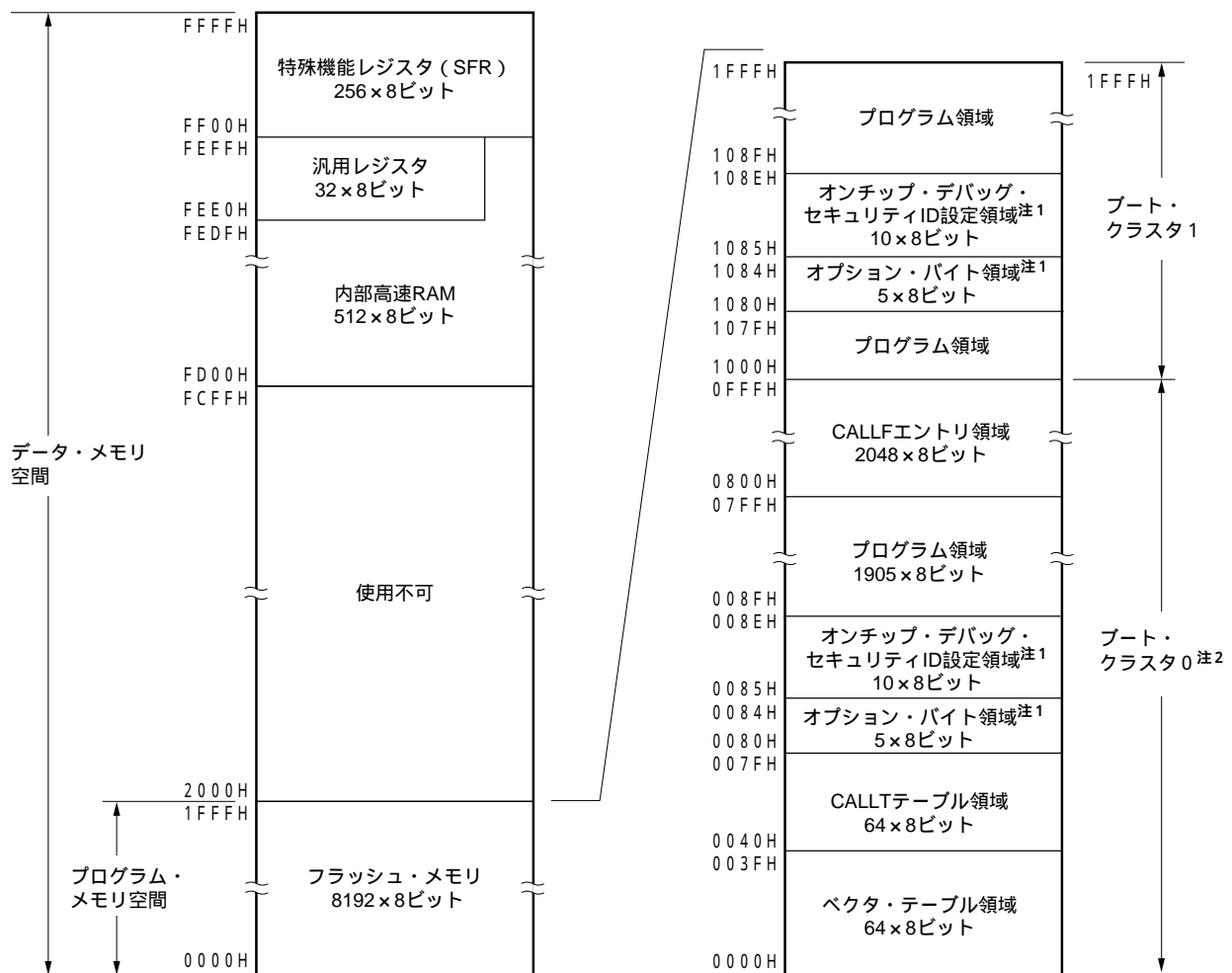
図3-2 メモリ・マップ (μ PD78F0741, 78F0743, 78F0745, 78F0751, 78F0753, 78F0755)
