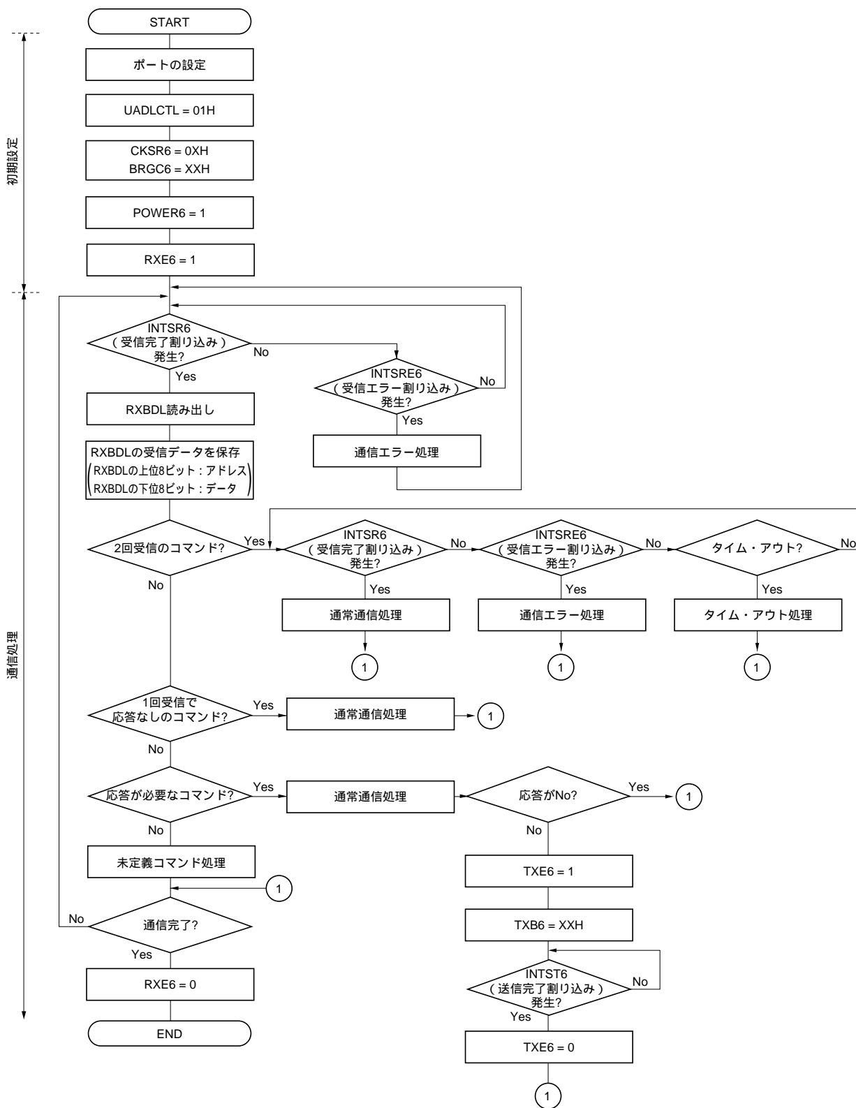
図14 - 31 DALI通信 (スレーブ送受信) のフロー・チャート例
