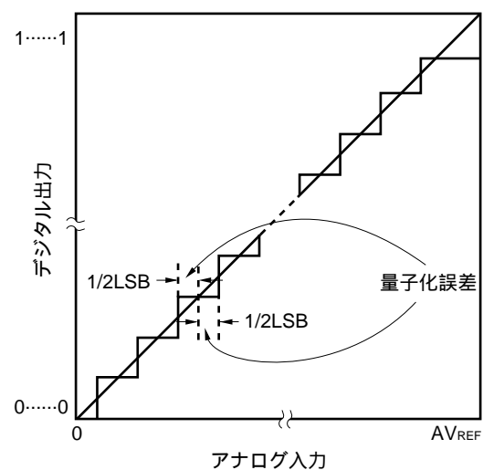
図11 - 20 量子化誤差
