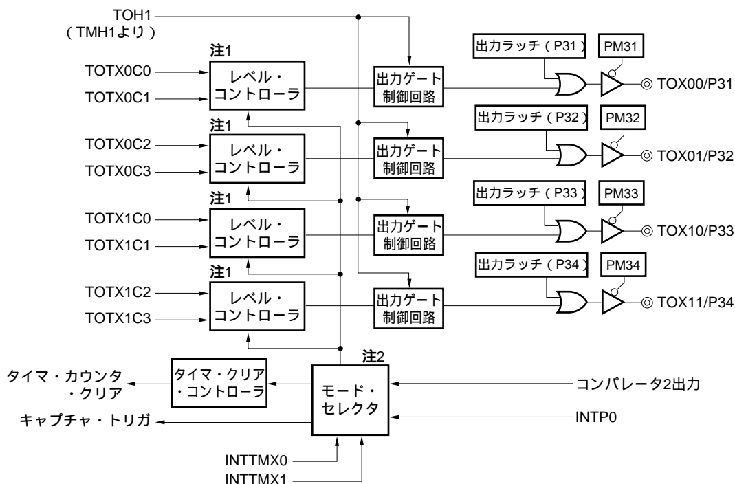
図6 - 45 16ビット・タイマX0とX1の出力構成のブロック図
