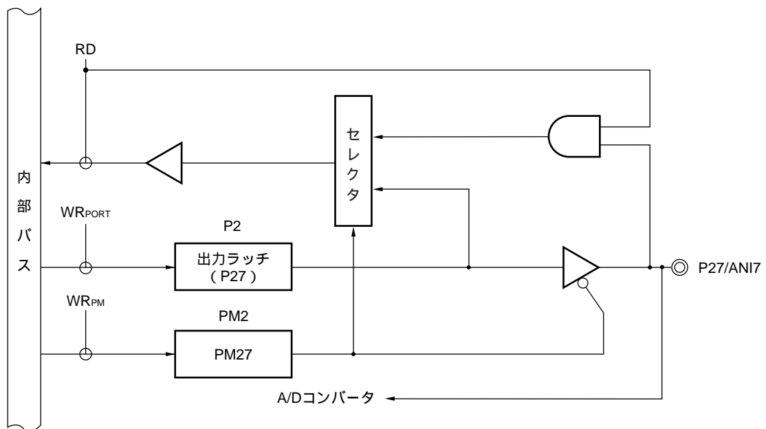
図4 - 11 P27のブロック図
