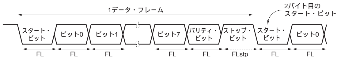
図14 - 36 連続送信時のデータ・フレーム長
