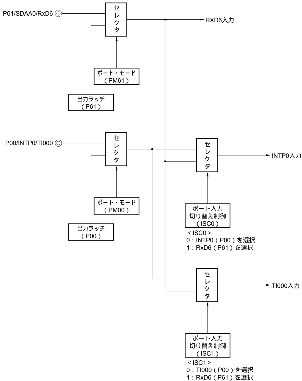
図14 - 3 LINの受信操作のポート構成図
