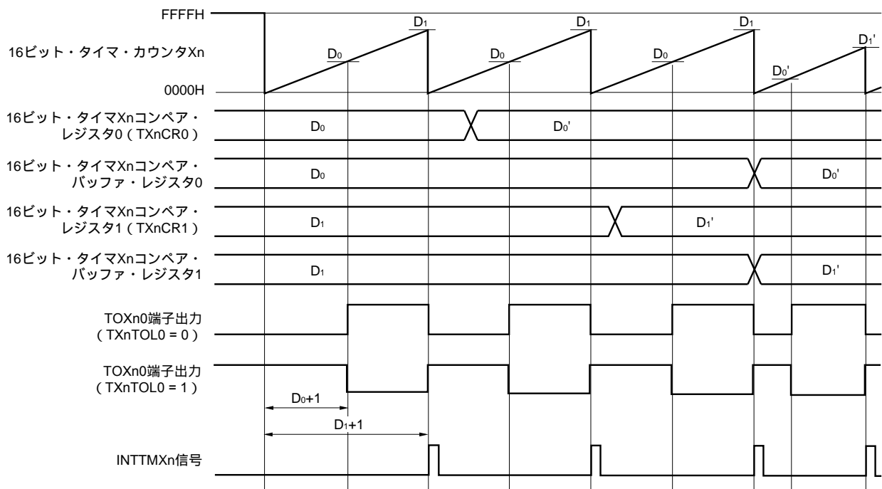
図6 - 28 PWM出力タイミング (TMXn単体動作, PWM出力: TOXn0端子)
