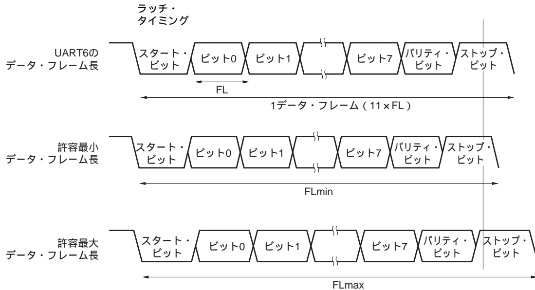
図14 - 35 受信時の許容ボー・レート範囲
