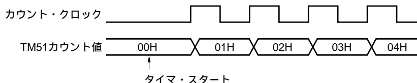
図8 - 11 8ビット・タイマ・カウンタ51 (TM51) のスタート・タイミング
