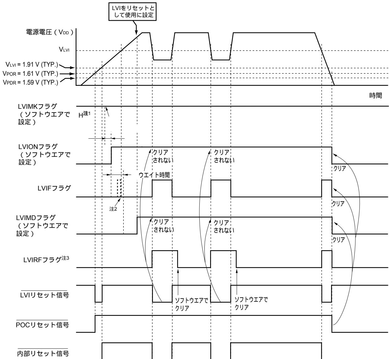
図22 - 5 内部リセット信号発生タイミング (LVISTART = 1)
