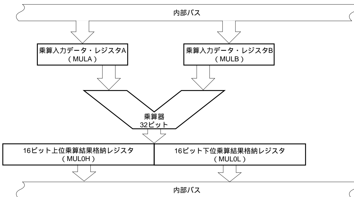
図17 - 1 乗算器のブロック図
