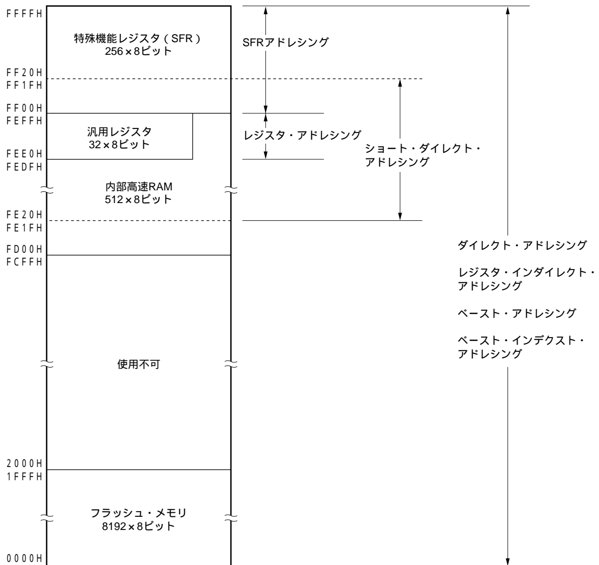
図3-5 データ・メモリとアドレッシングの対応 ( \mu PD78F0741, 78F0743, 78F0745, 78F0751, 78F0753, 78F0755)
