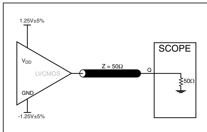
2.5V LVCMOS Output Load Test Circuit
