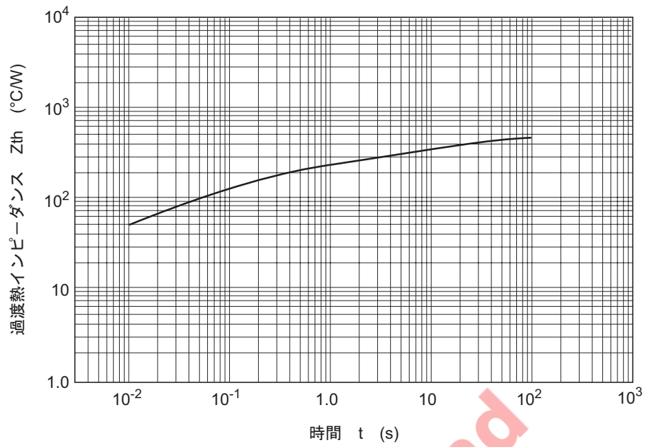
図4. 過渡熱インピーダンス特性
