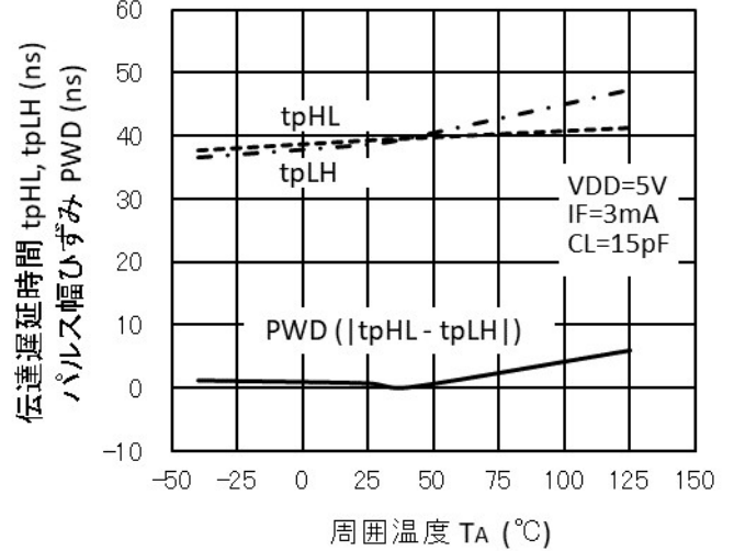
伝達遅延時間、パルス幅ひずみ vs. 周囲温度
