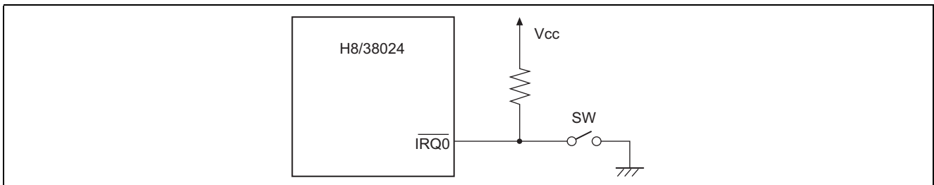
図 1 スリープ(高速)モードへの遷移におけるスイッチ接続例
