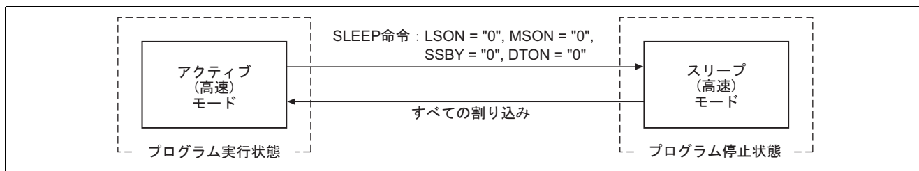
図 2 スリープ(高速)モードへのモード遷移図
