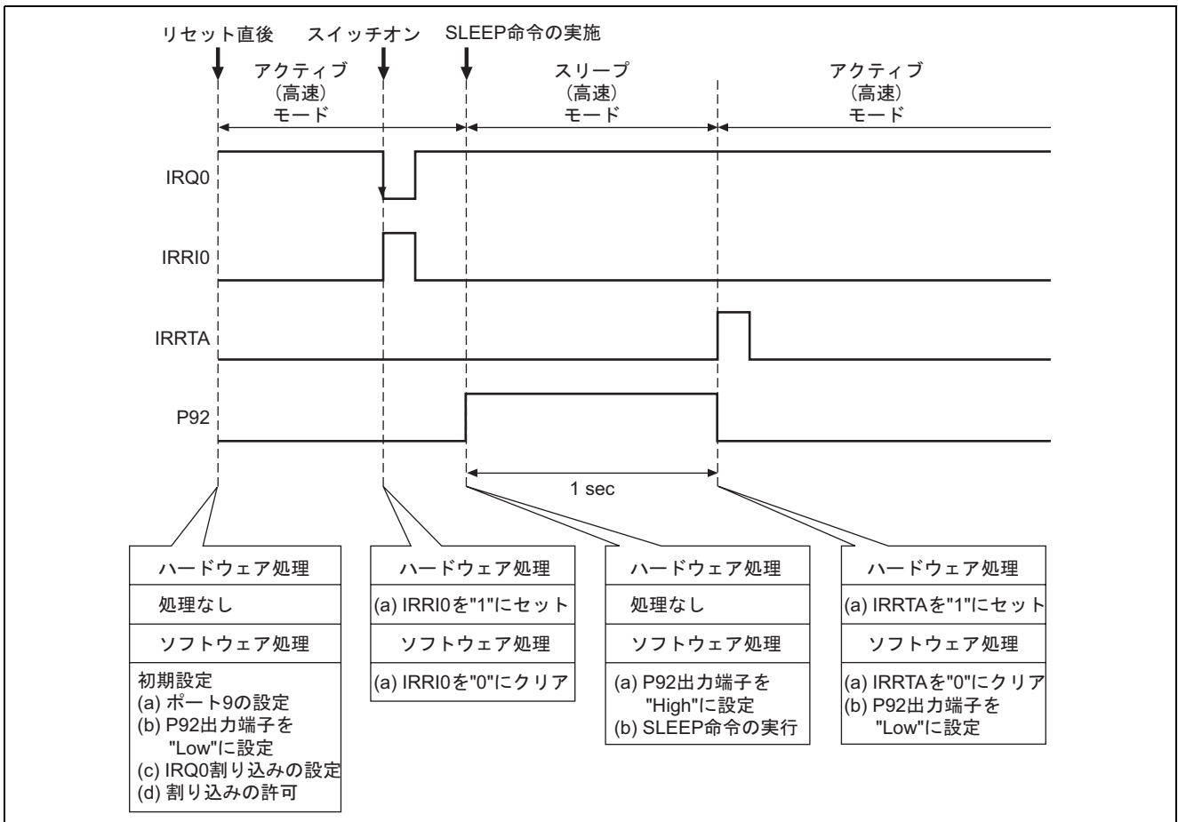
図3 スリープ(高速)モードへの遷移の動作説明
