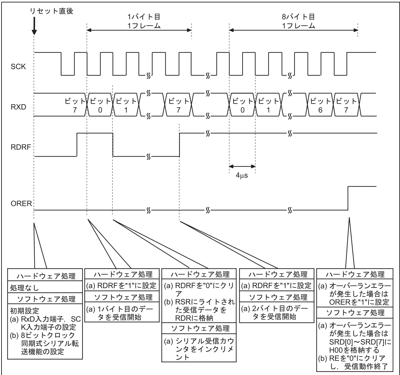
図3 クロック同期式シリアルデータ受信時の動作
