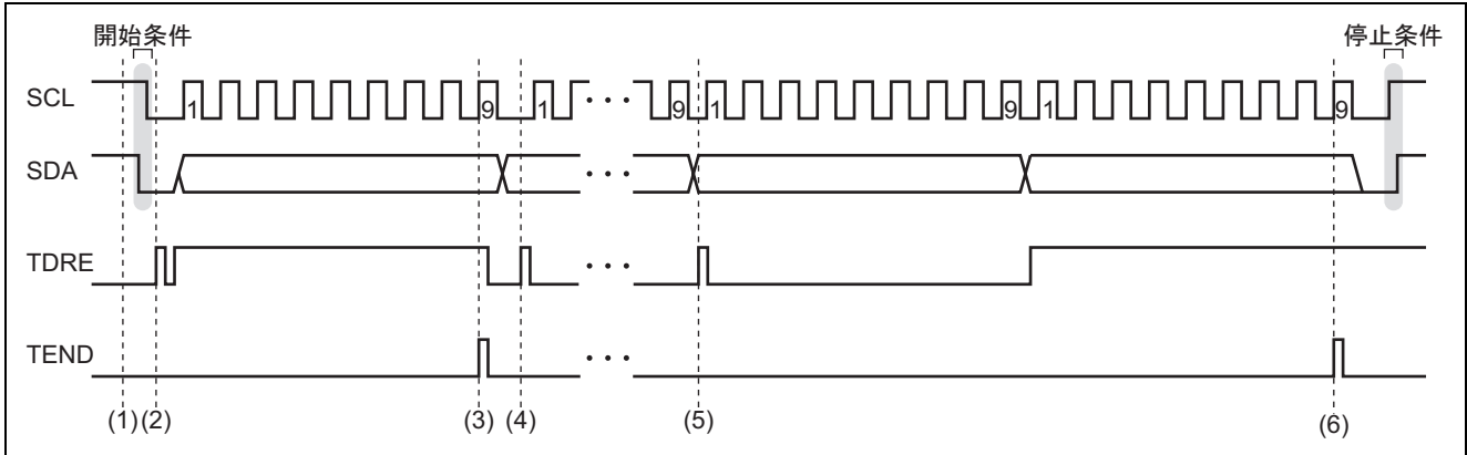
図 2 マスタ送信モード動作タイミング
