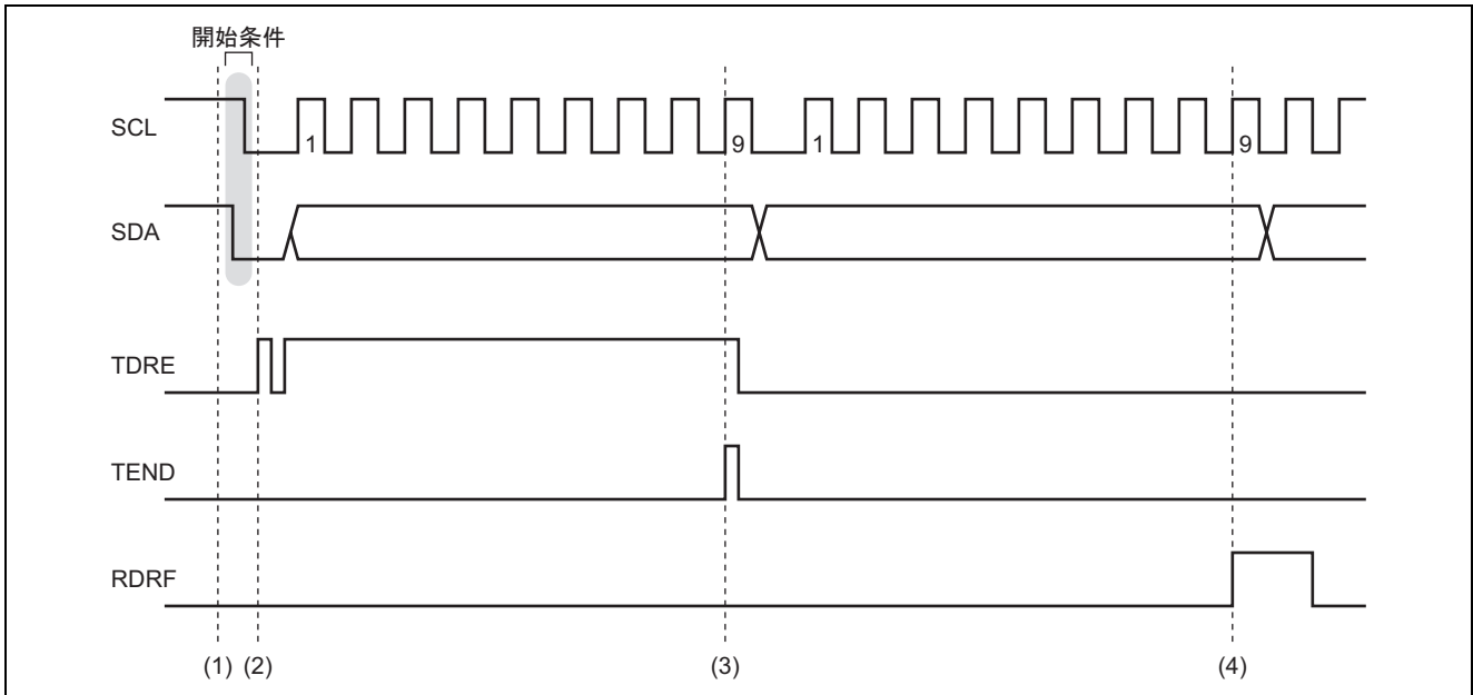
図 3 マスタ受信モード動作タイミング 1
