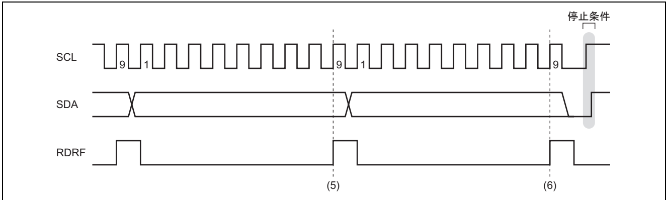
図 4 マスタ受信モード動作タイミング 2
