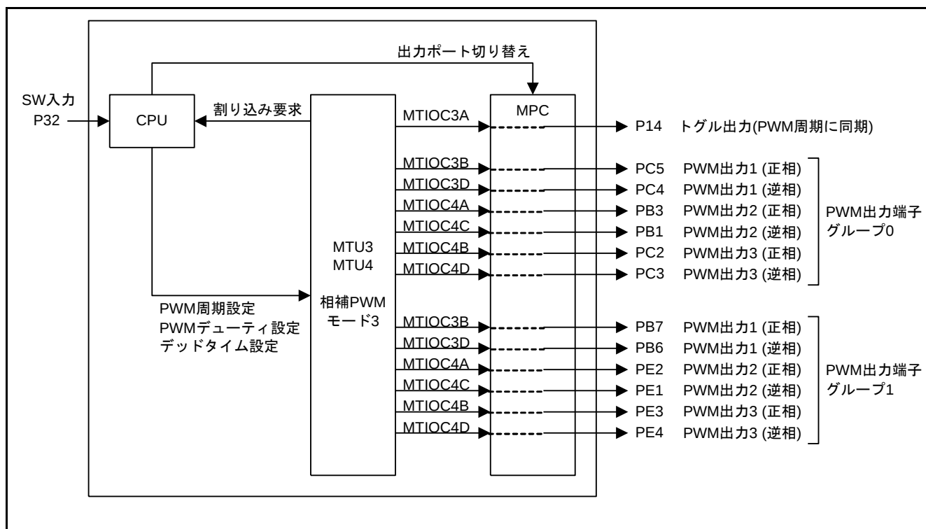
図1.1 ブロック図
