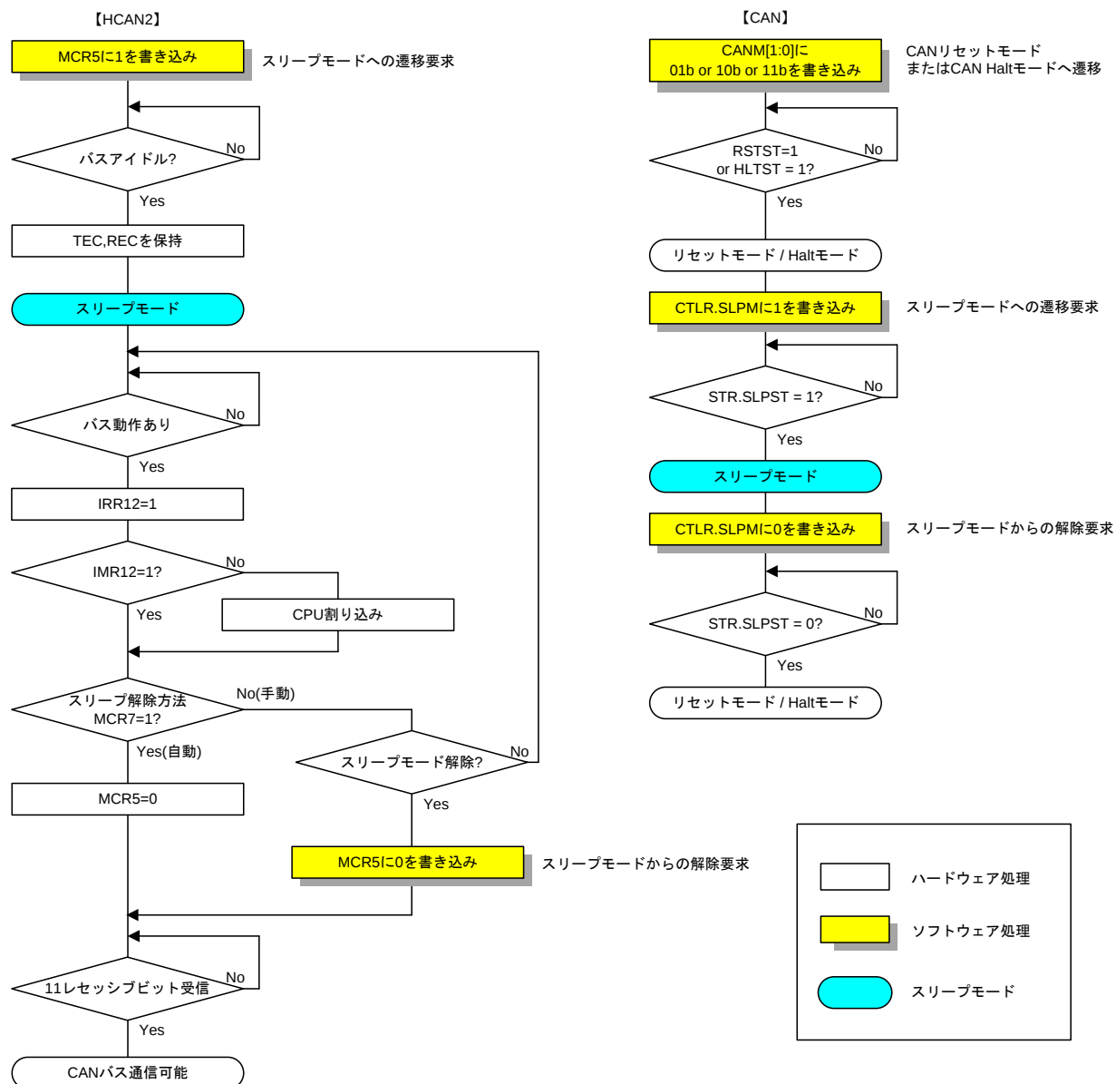
図 1 SH7047 (HCAN2) と RX65N (CAN) のスリープモードへの設定手順
