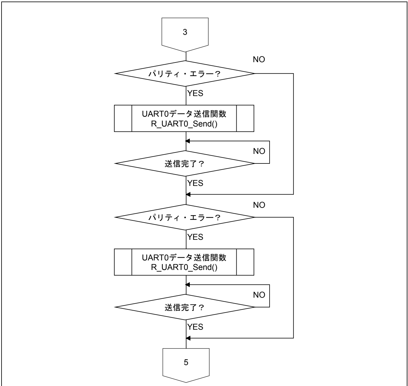
図 5.11 メイン関数 (2/3)
