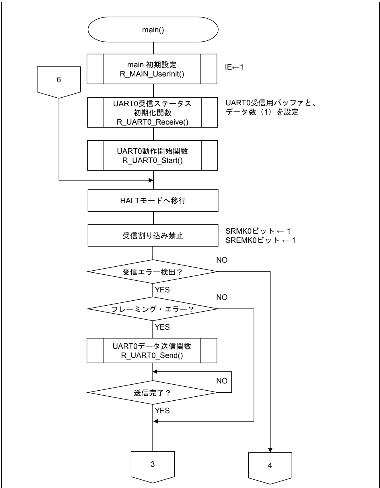
図 5.10 メイン関数 (1/3)
