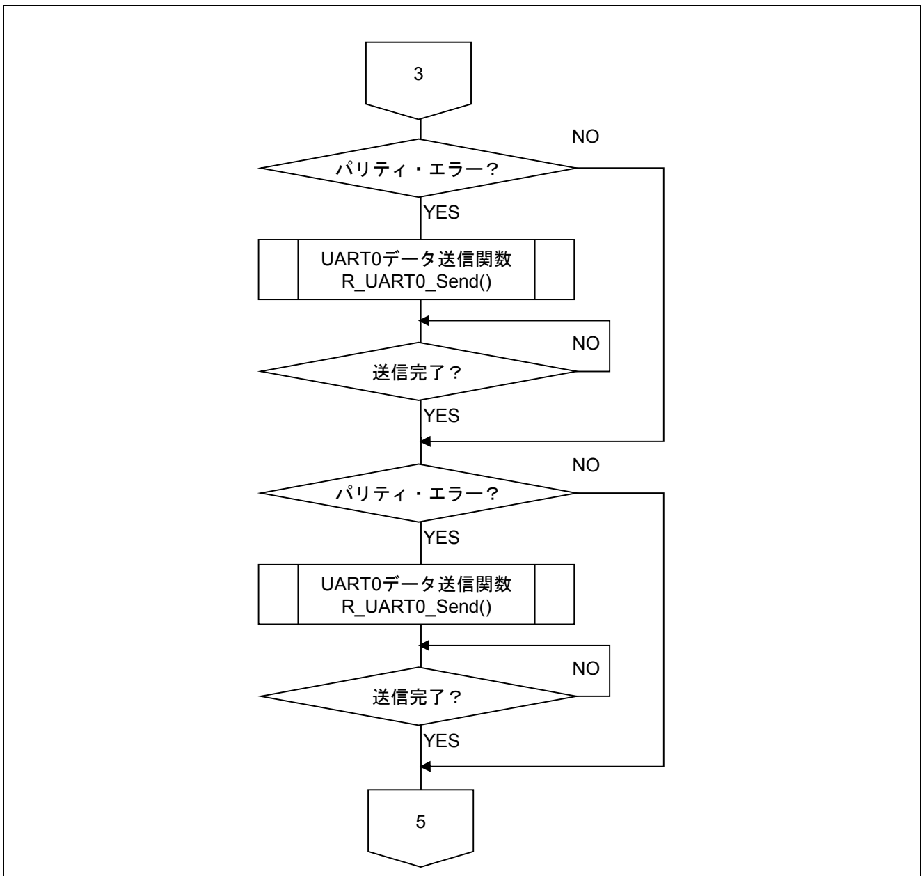
図 5.11 メイン関数 (2/3)
