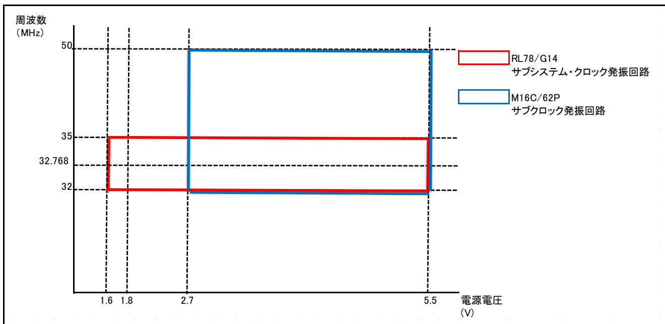
図 1.3 サブクロック発振回路の動作周波数比較
