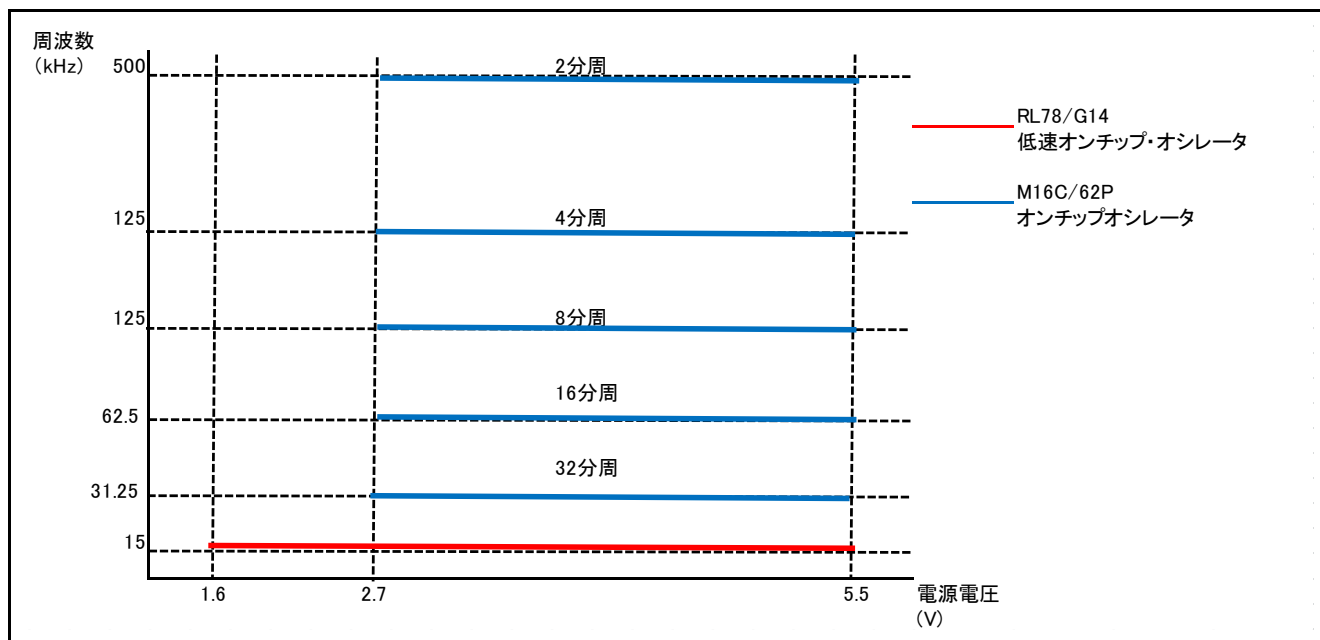
図1.4 低速オンチップオシレータの動作周波数比較
