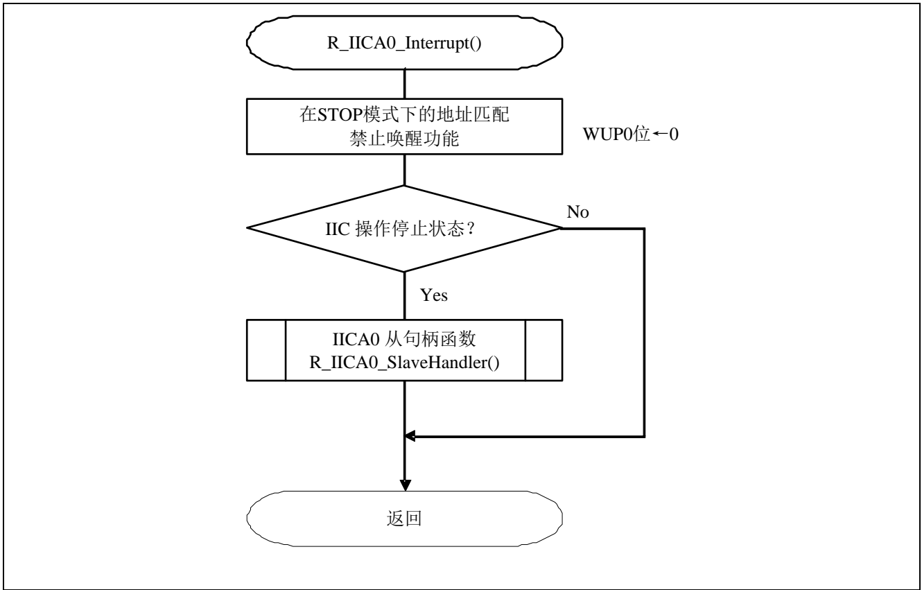
图 5.10 IICA0 中断程序
