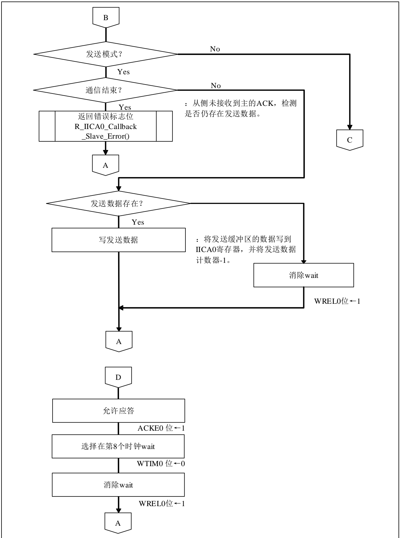
图 5.12 IICA0 从句柄函数 (2/3)
