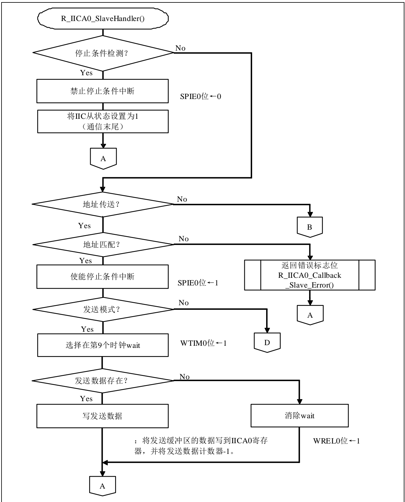
图 5.11 IICA0 从句柄函数 (1/3)
