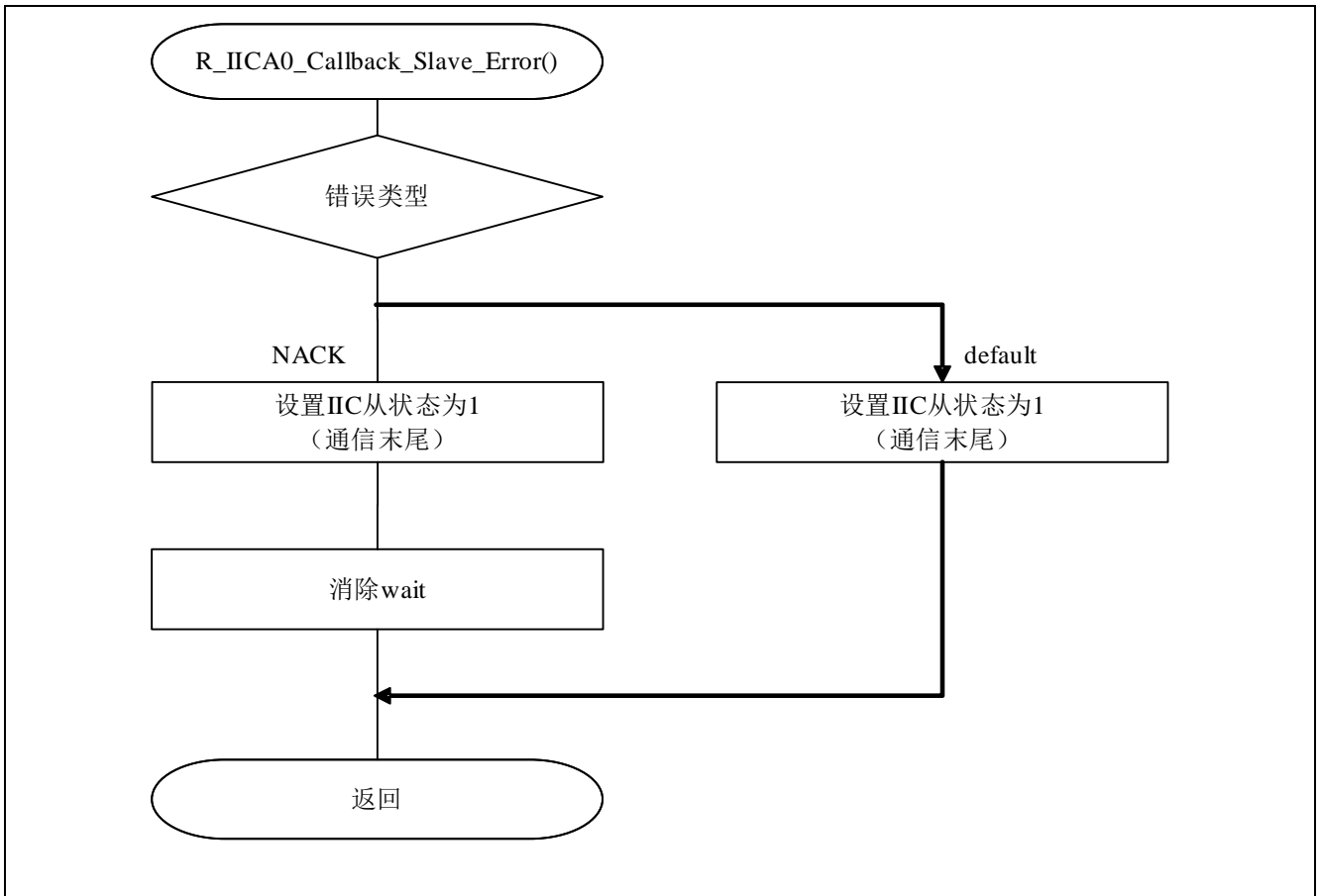
图 5.14 错误标志位返回程序
