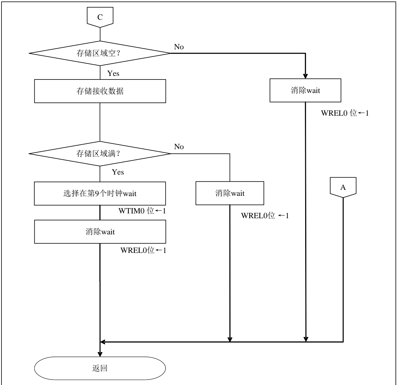
图 5.13 IICA0 从句柄函数 (3/3)
