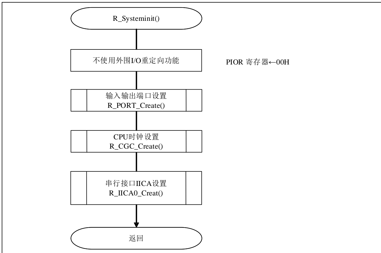
图 5.3 系统函数
