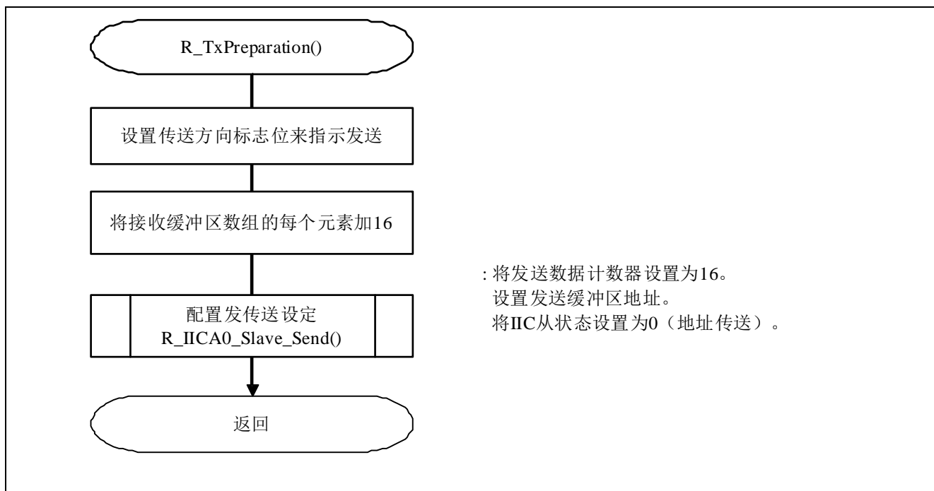
图 5.9 IICA0 发送准备函数
