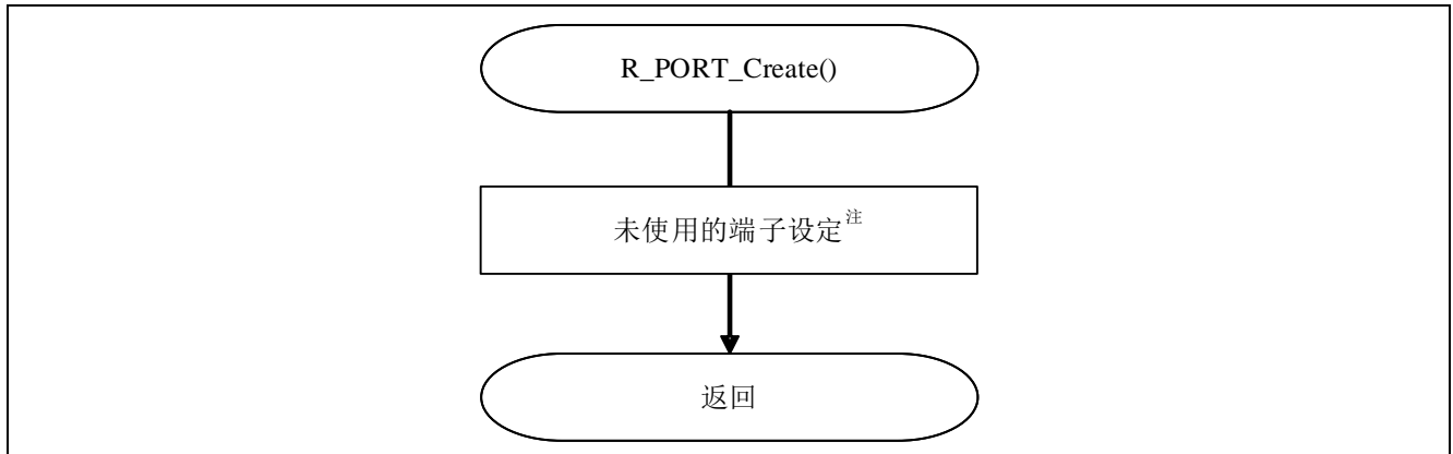
图 5.4 I/O 端口设置流程
