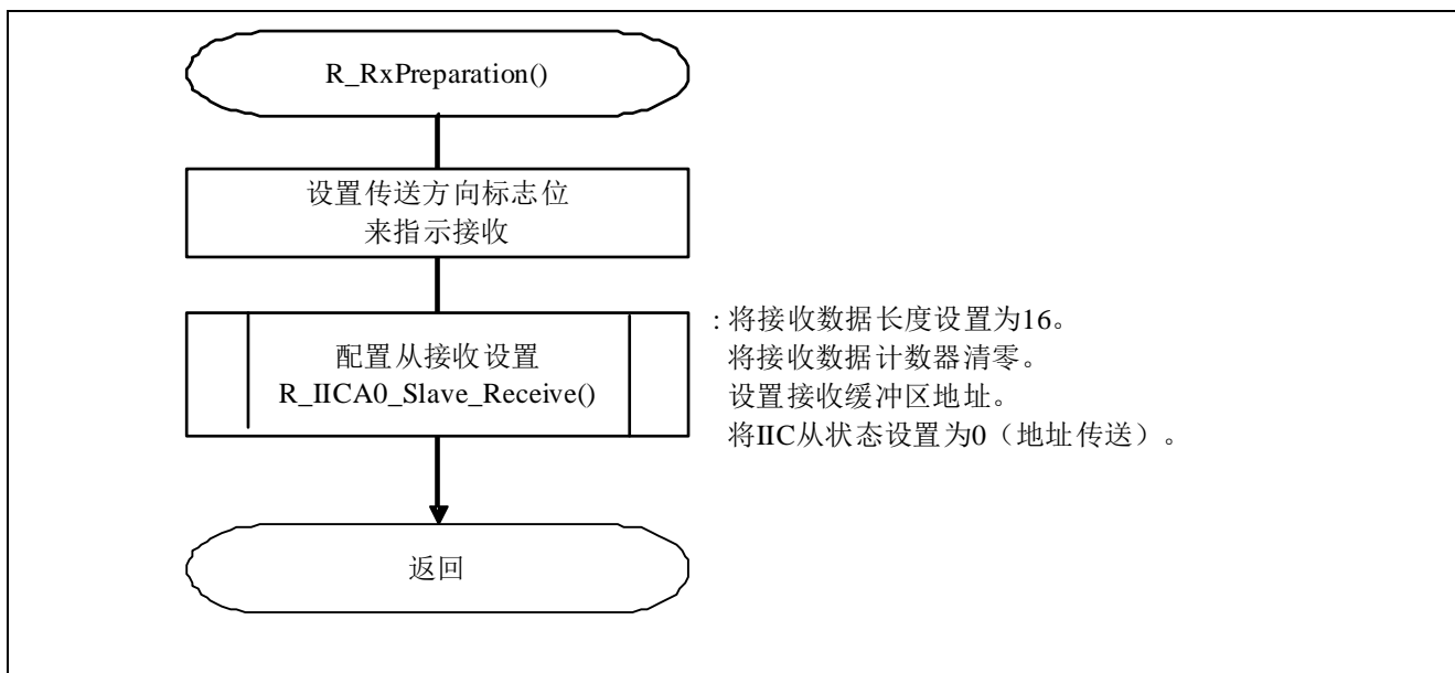
图 5.8 IICA0 接收准备函数
