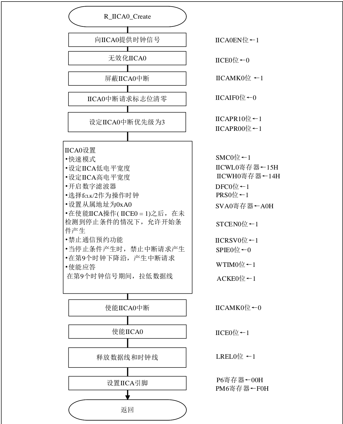
图 5.6 串行接口 IICA 设置
