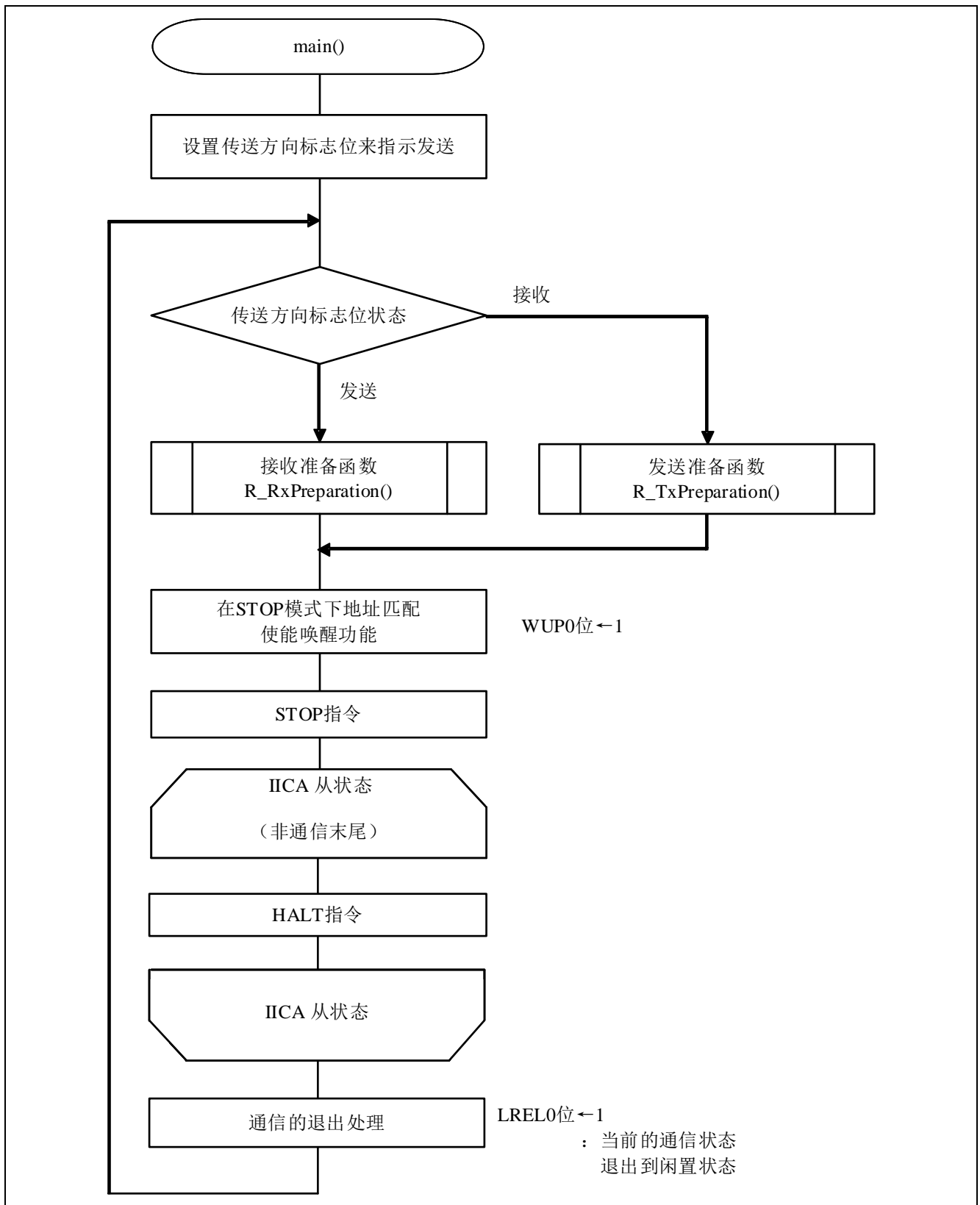
图 5.7 主程序
