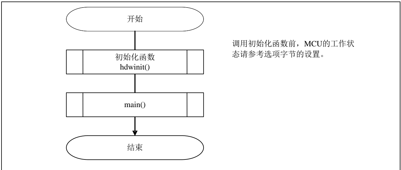
图 5.1 整体流程
