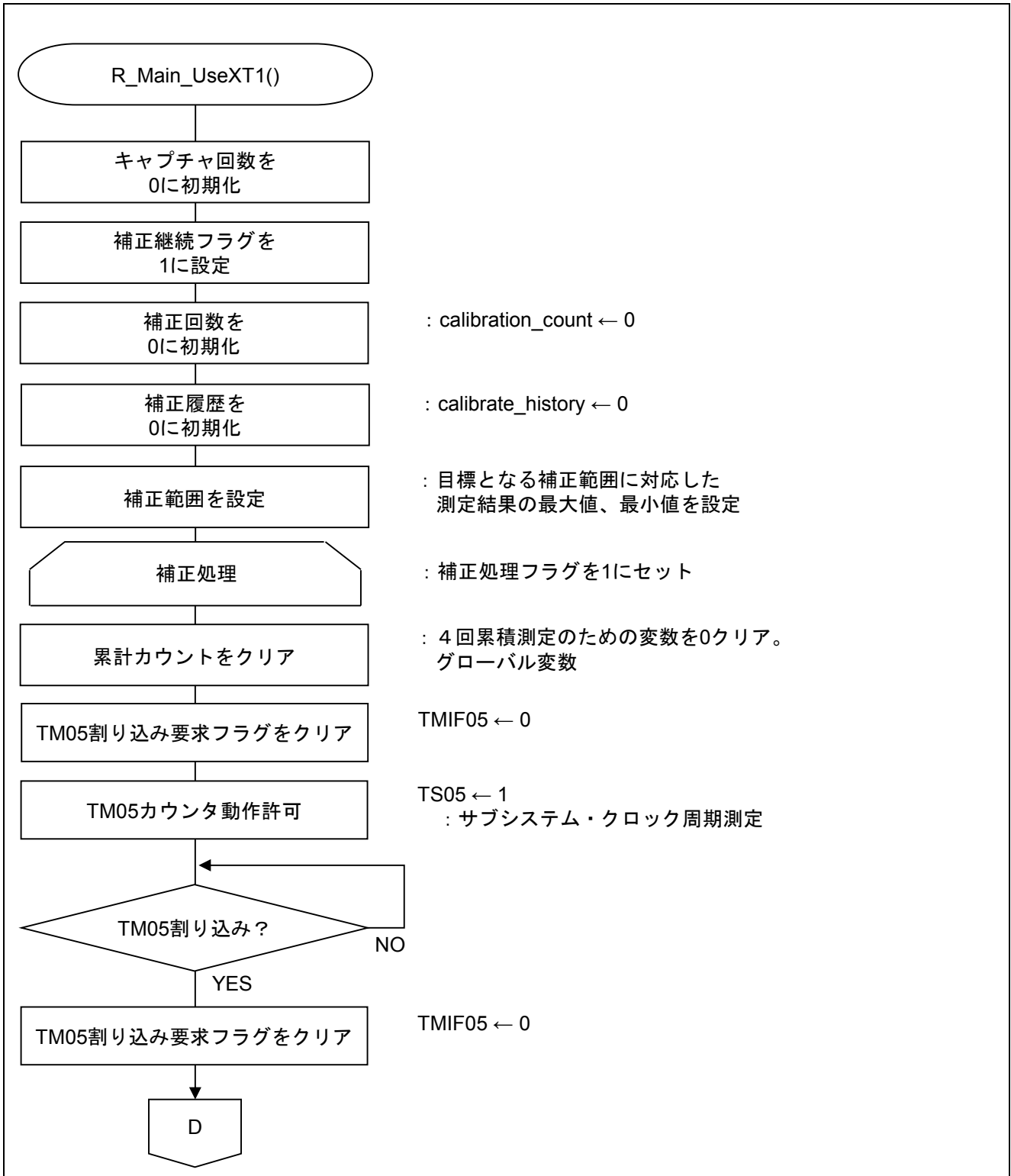
図 5.12 XT1 発振使用のキャリブレーション処理 (1/2)
