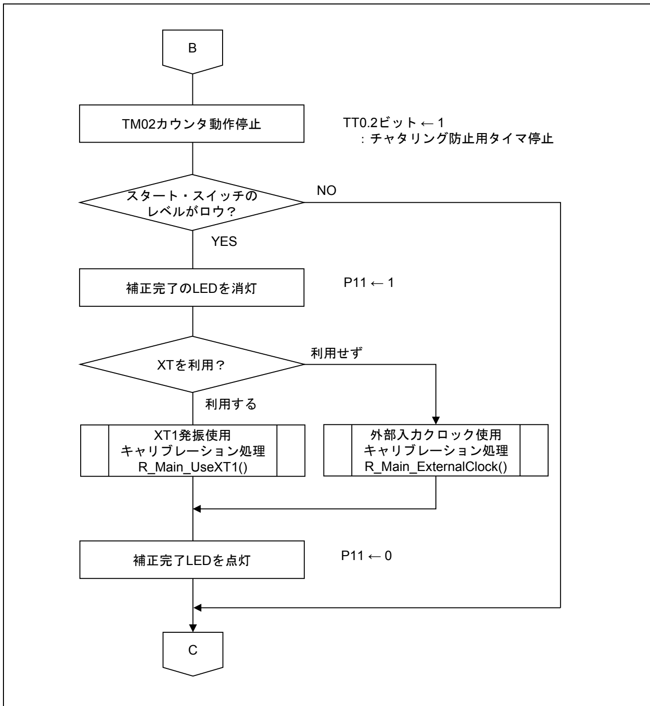
図 5.11 メイン処理 (2/2)
