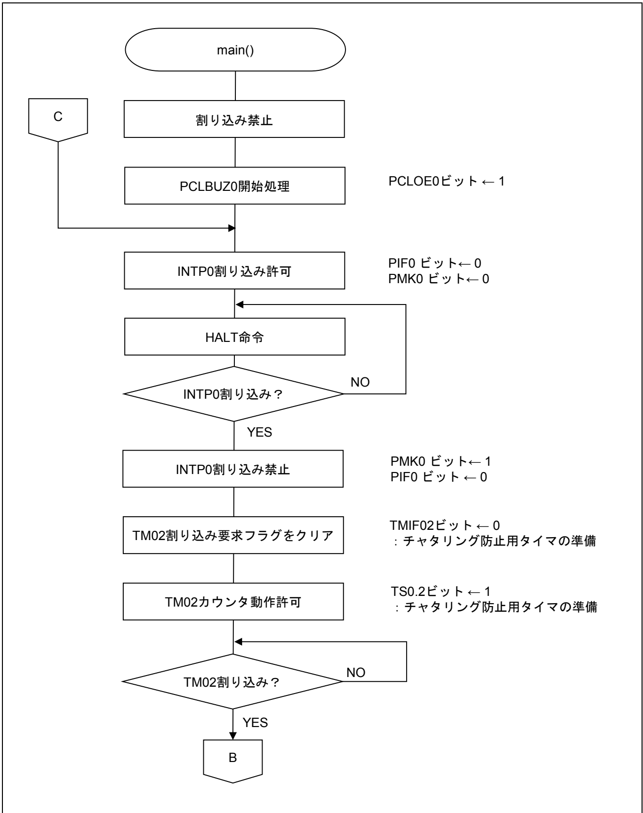
図 5.10 メイン処理 (1/2)
