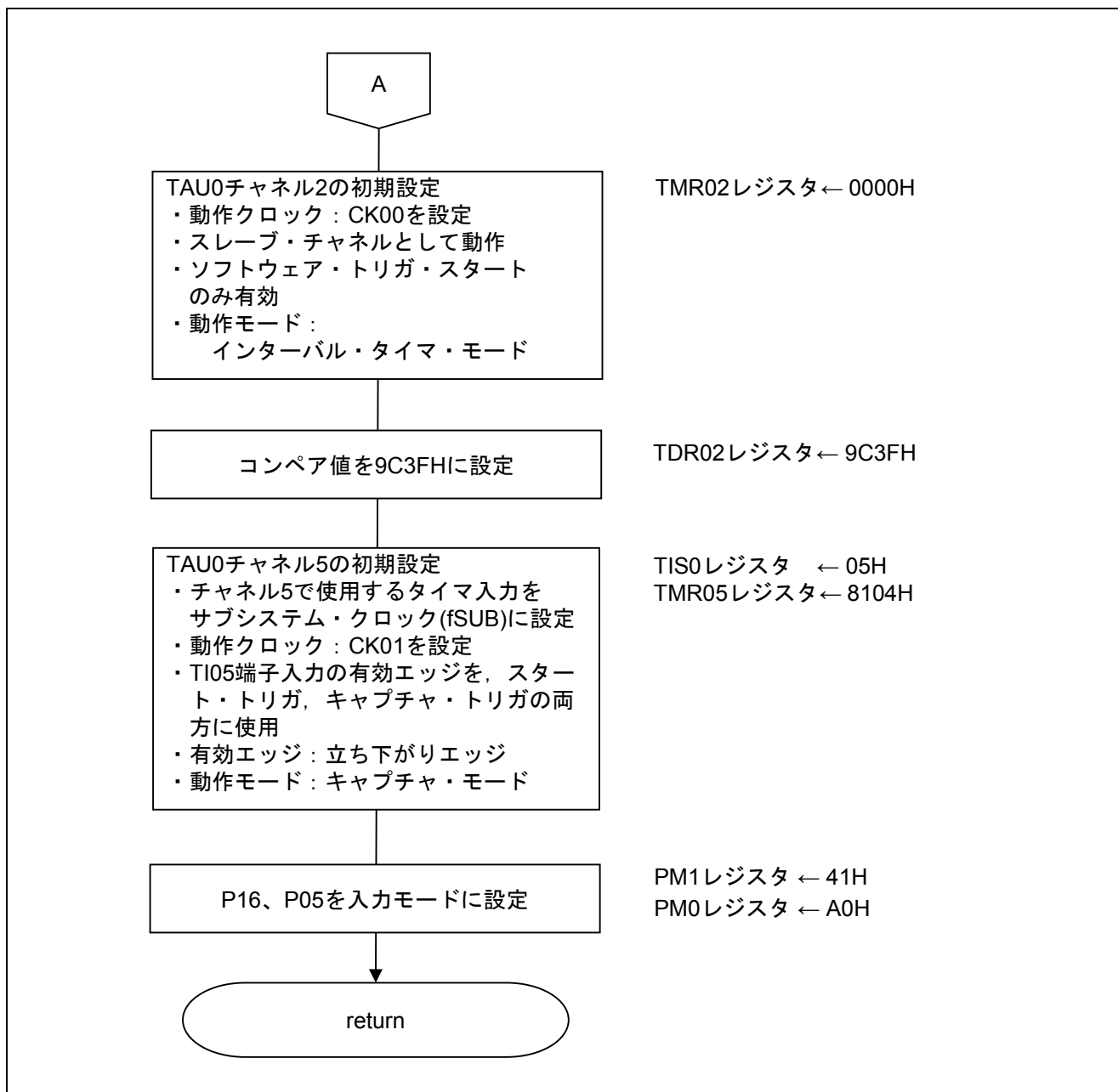
図 5.7 TAU0 の設定 (2/2)
