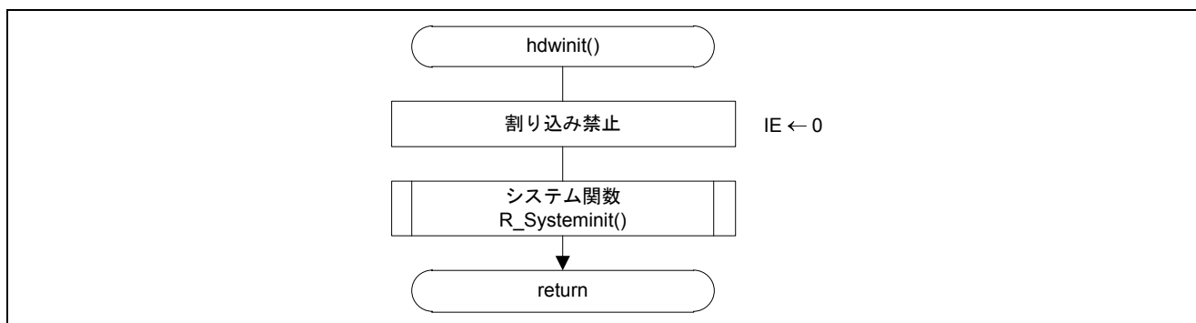
図 5.2 初期設定関数
