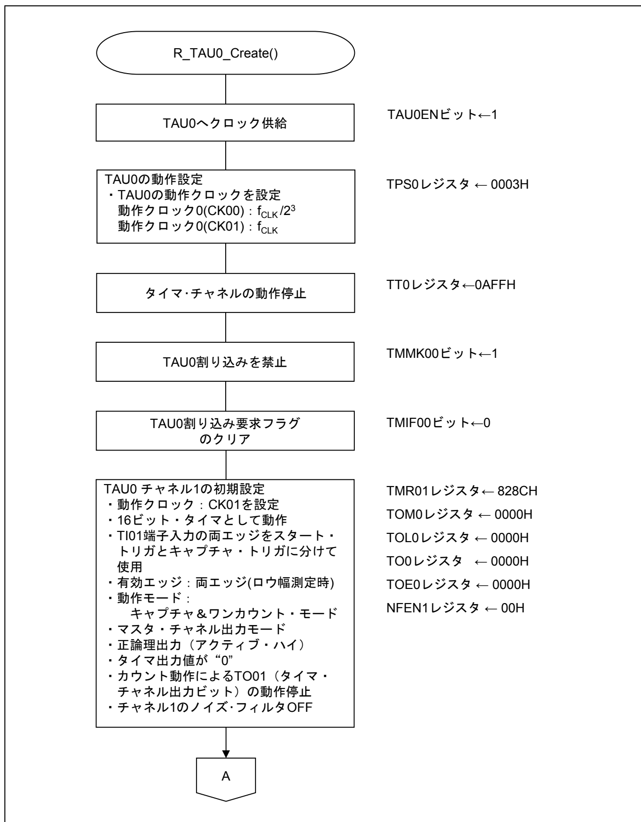
図 5.6 TAU0 の設定 (1/2)
