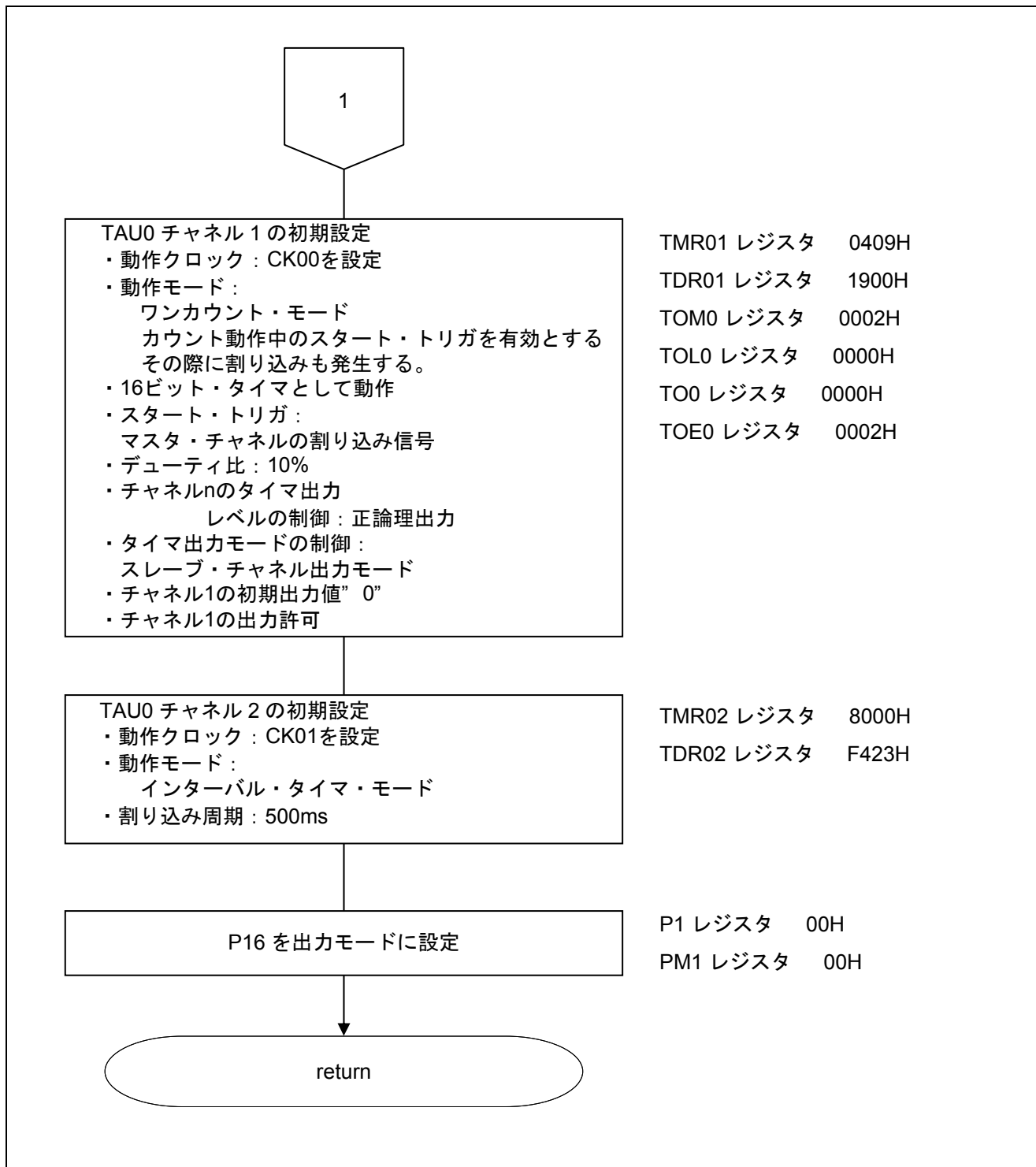
図 5.7 TAU0 の設定 (2/2)
