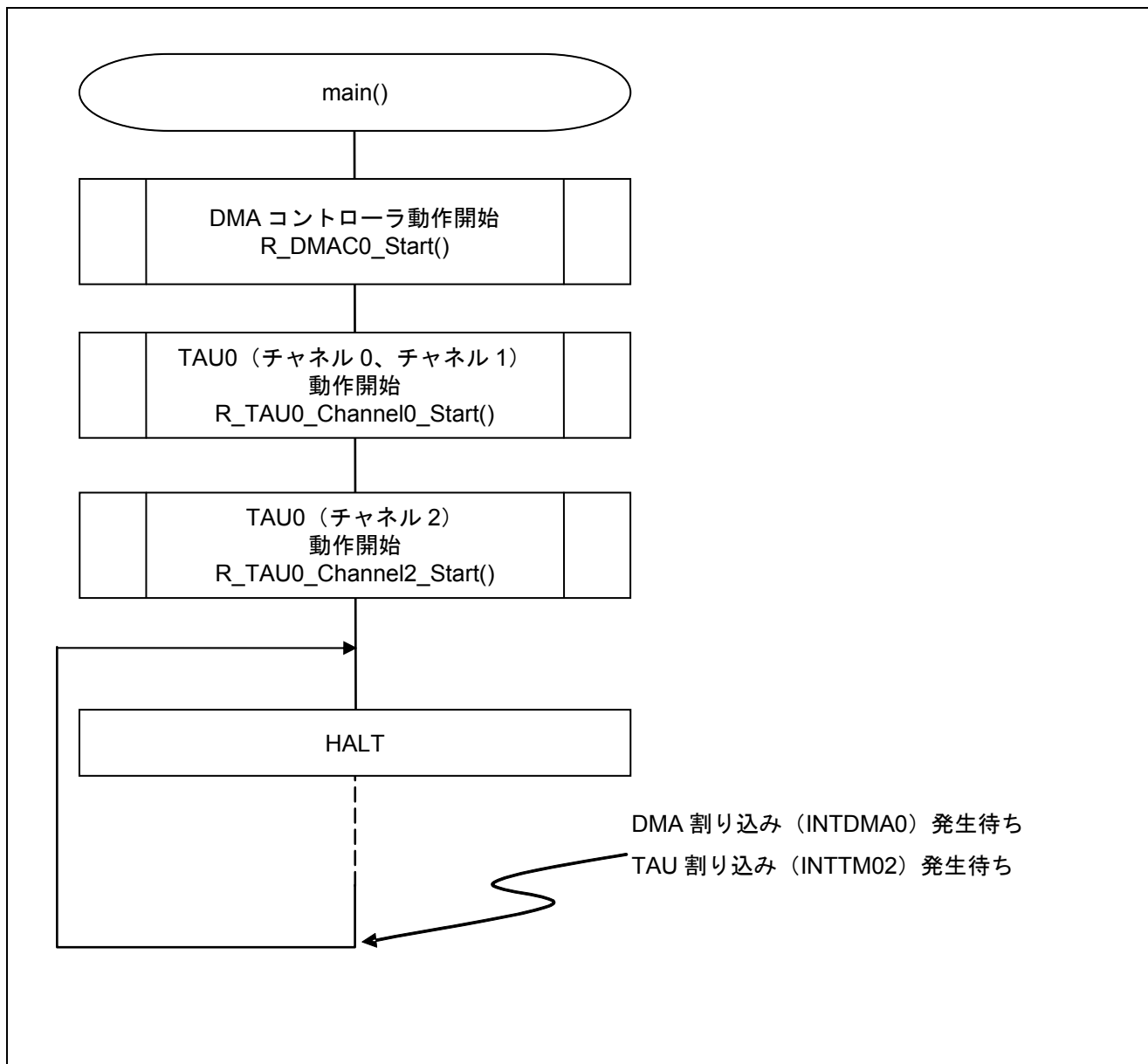
図 5.9 メイン処理
