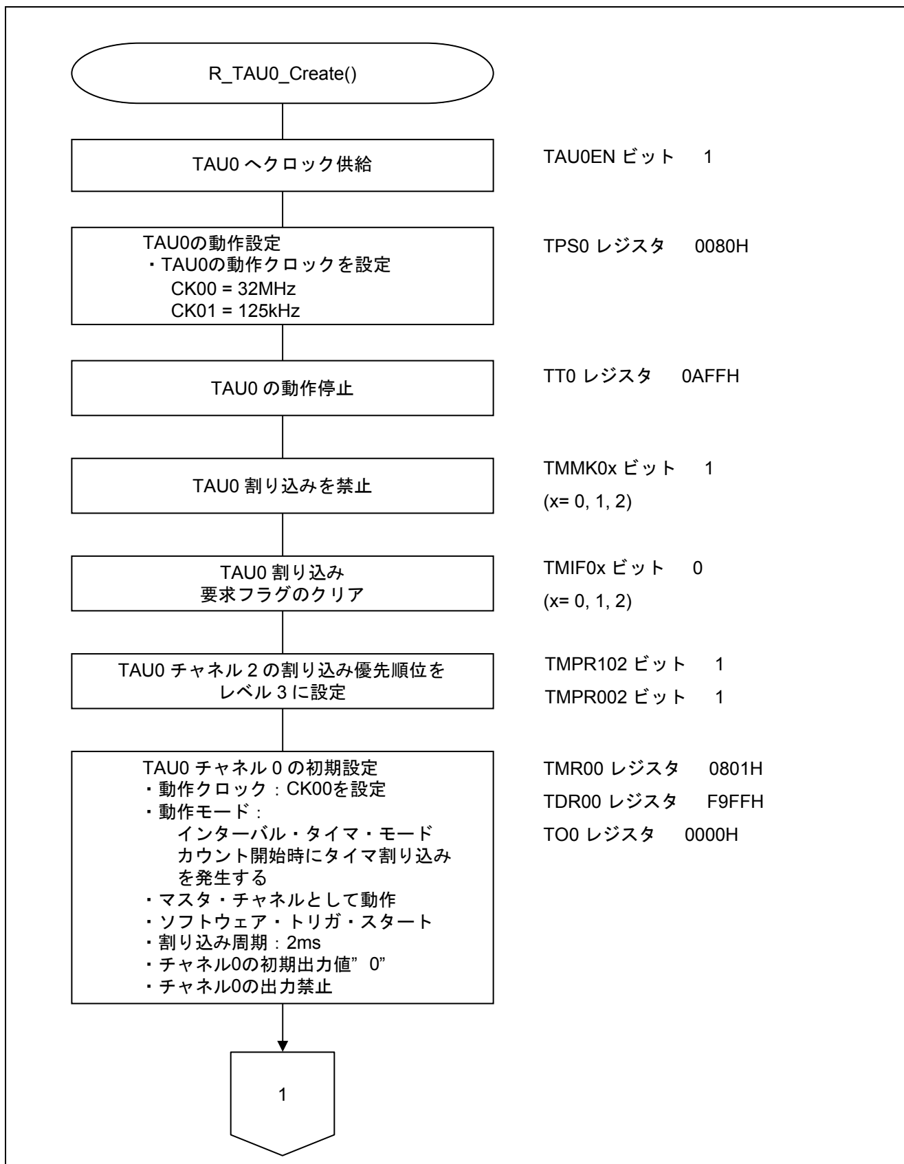
図 5.6 TAU0 の設定 (1/2)
