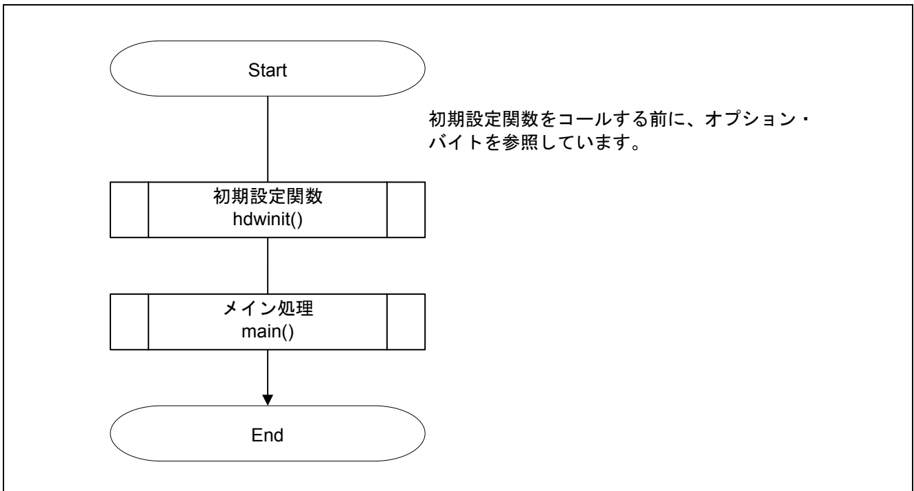
図 5.1 全体フロー
