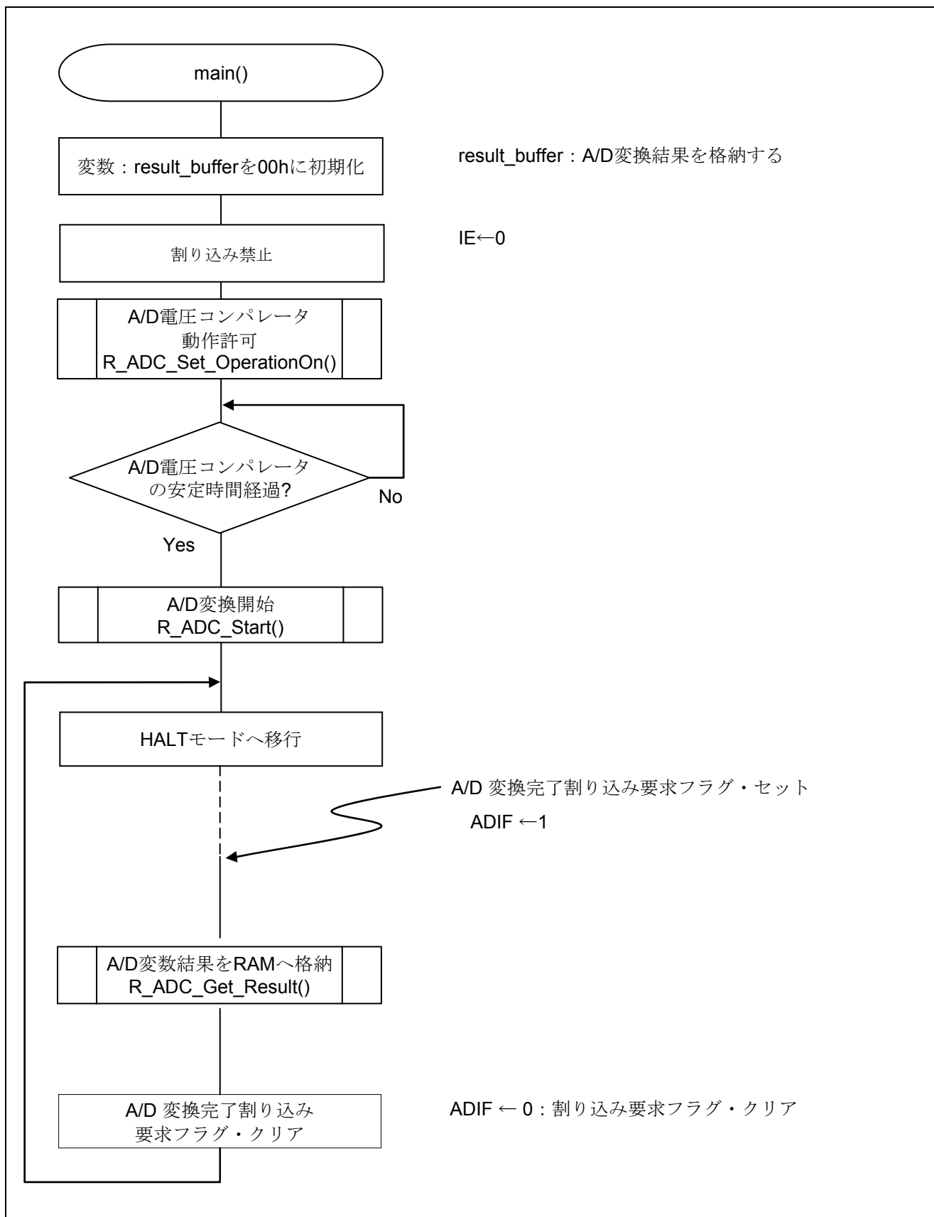
図 5.7 メイン処理
