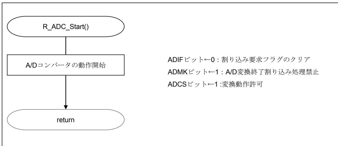
図 5.9 A/D 変換開始
