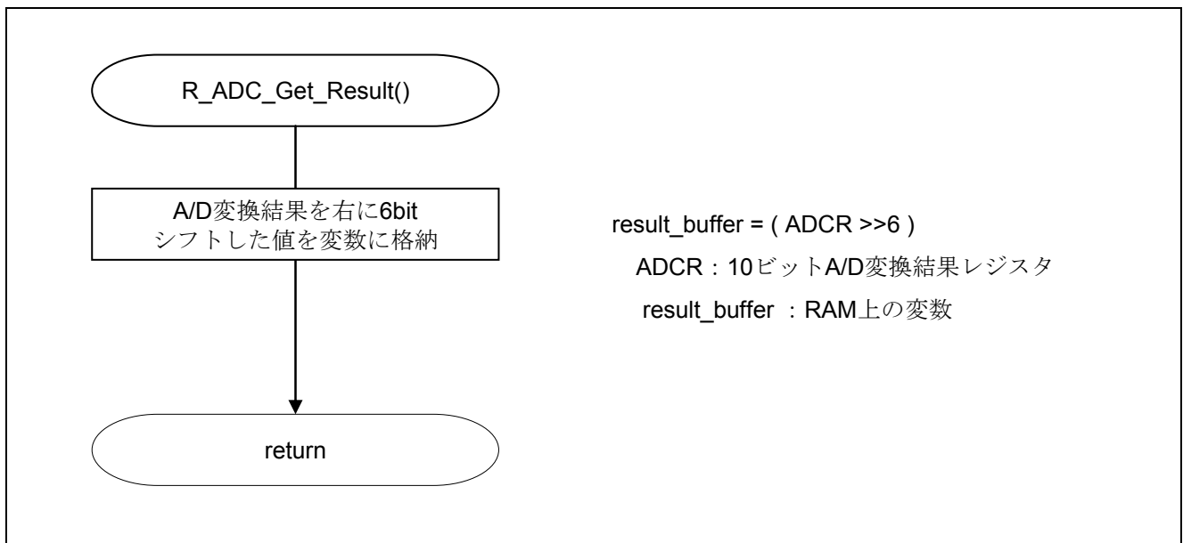
図 5.10 A/D 変換結果を RAM へ格納
