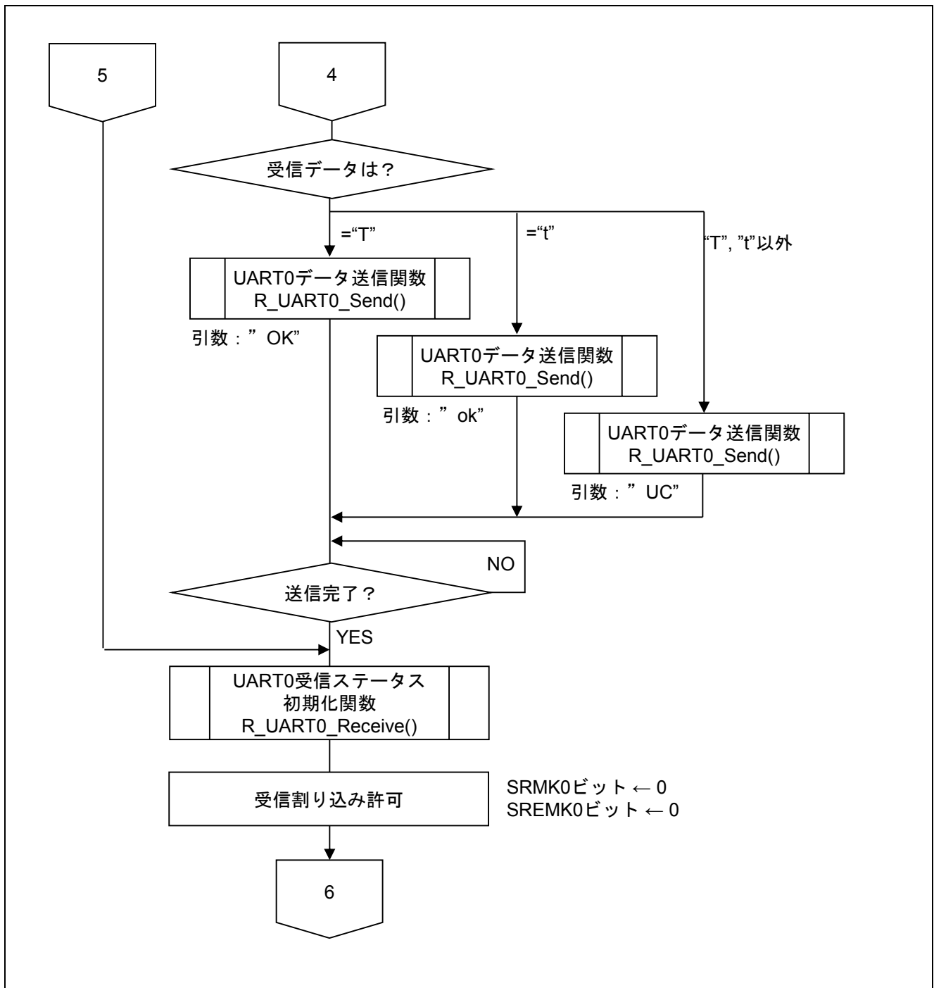
図 5.12 メイン関数 (3/3)
