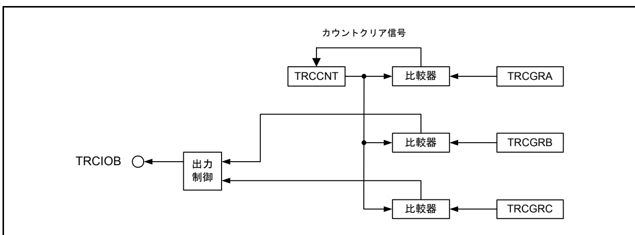
図 3.1 ブロック図
