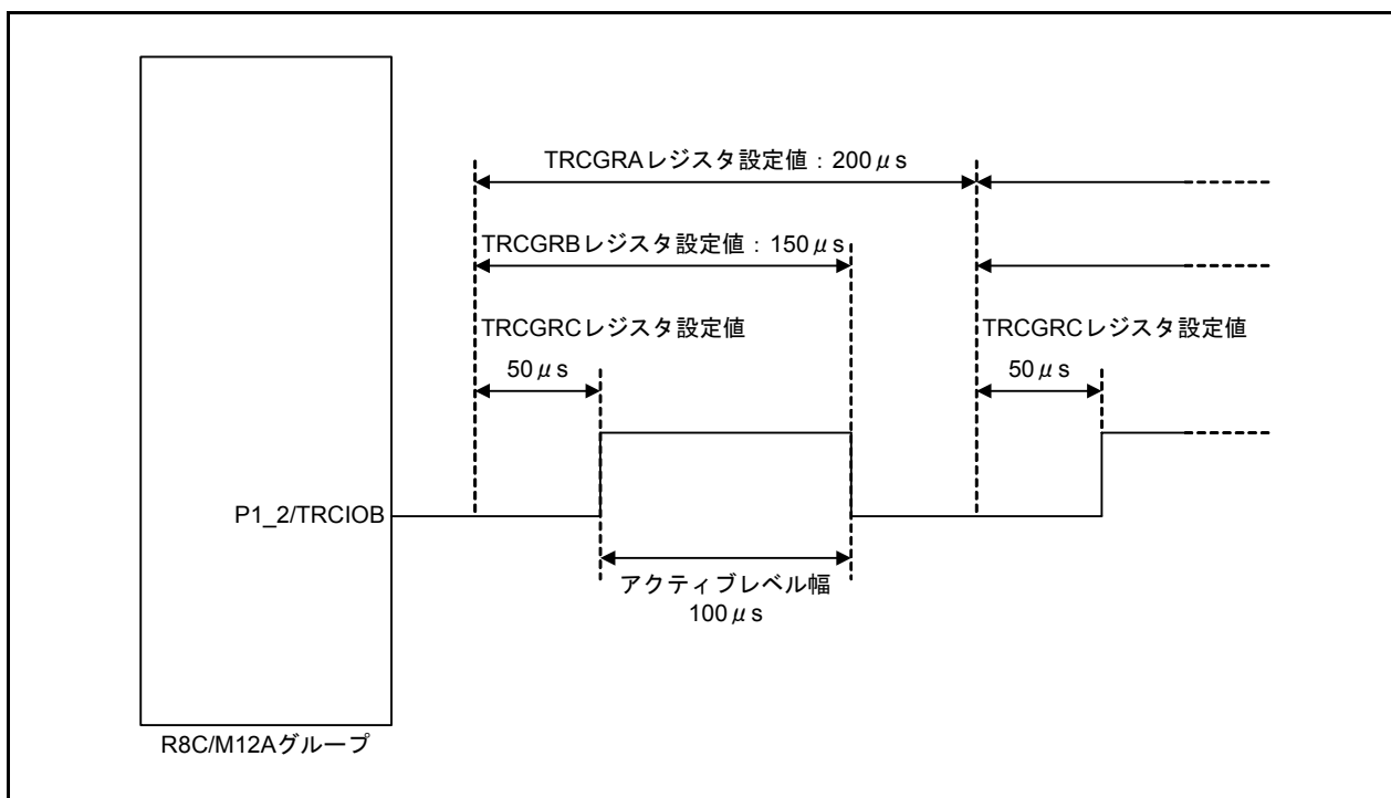
図 3.2 タイミング図
