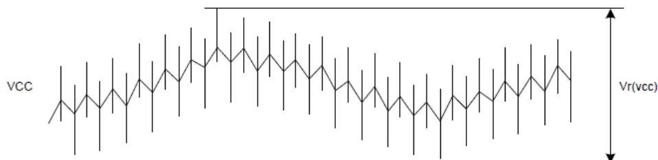
図2 マイコン側の電源電圧変動 (許容リップル電圧) 規格
