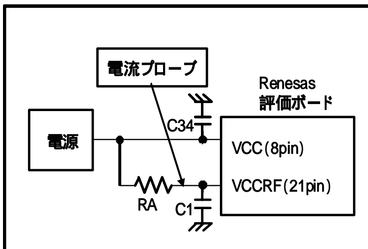
図3 ラッシュ電流評価構成
