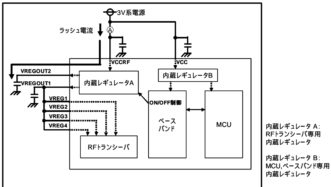
図 1 内蔵レギュレータ構成
