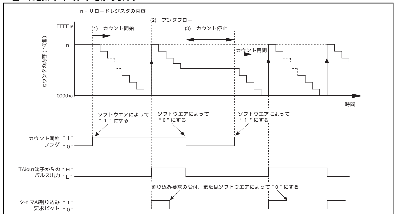
図1 タイマモード、パルス出力機能機能選択時の動作タイミング
