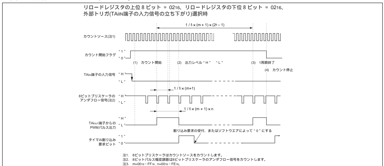
図1 パルス幅変調モード動作、8ビットPWMモード選択時のタイミング
