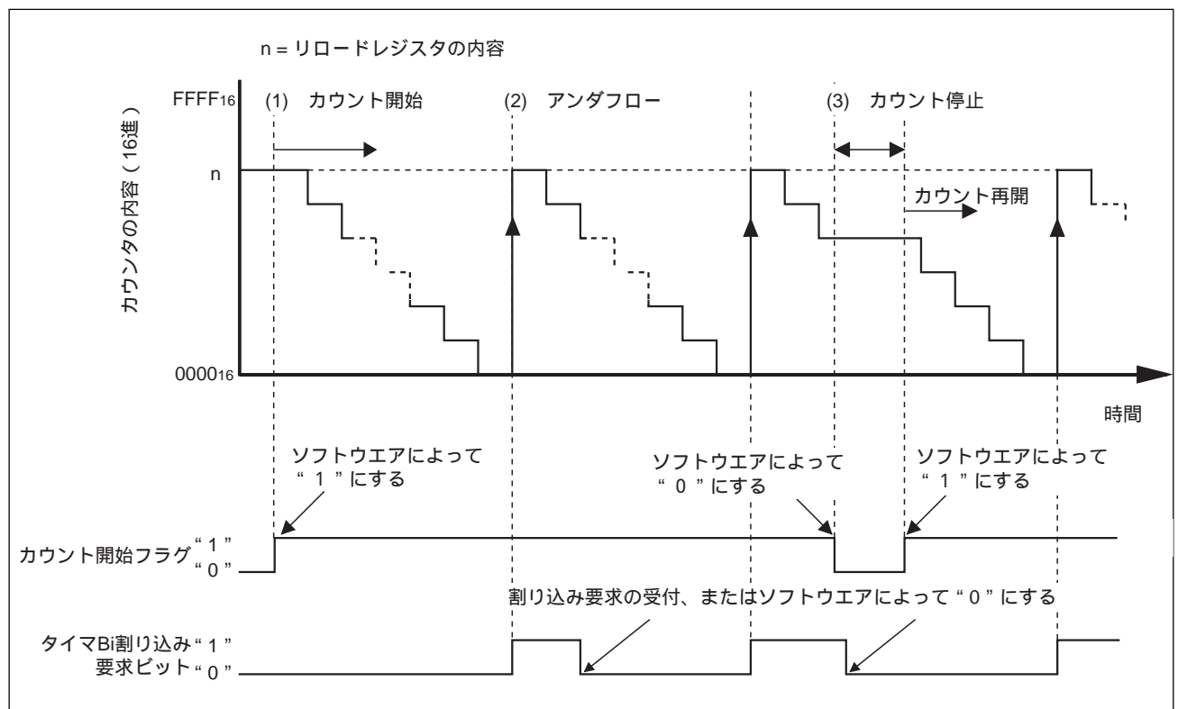
図1 タイマモード動作タイミング
