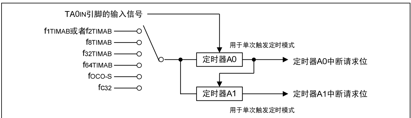
图 2. 延迟单次触发输出的定时器连接示意图
