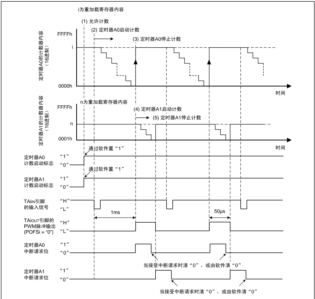
图 1. 延迟单次触发输出的工作时序图
