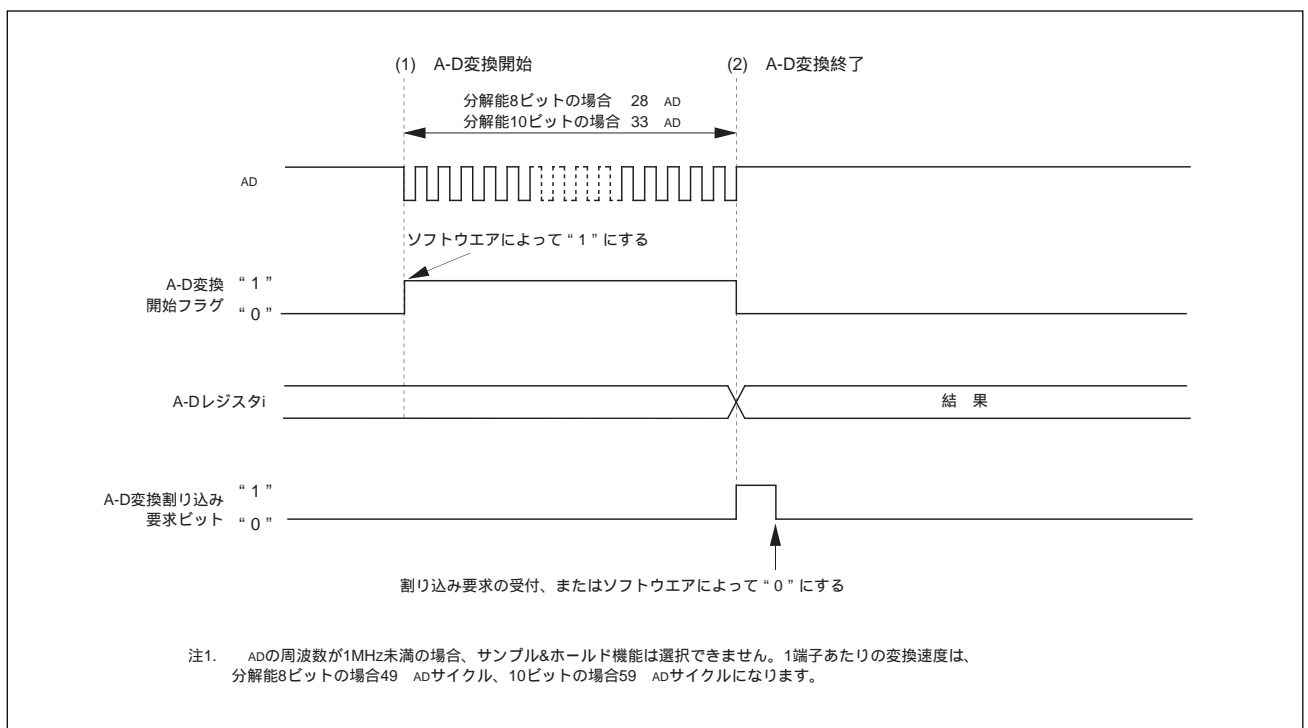
図1 単発モード、拡張アナログ入力選択時の動作タイミング
