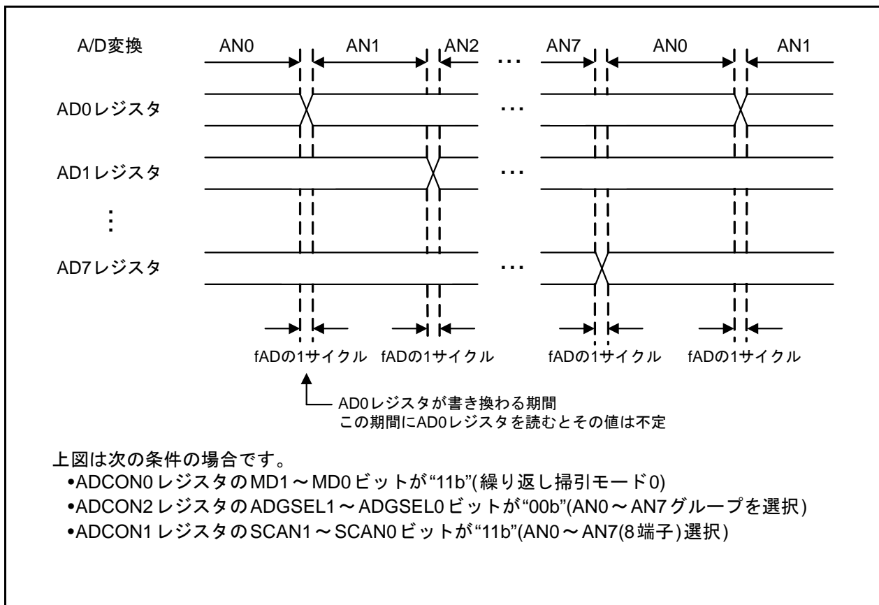
図 4.1 AD ji レジスタの値が書き換わる期間
