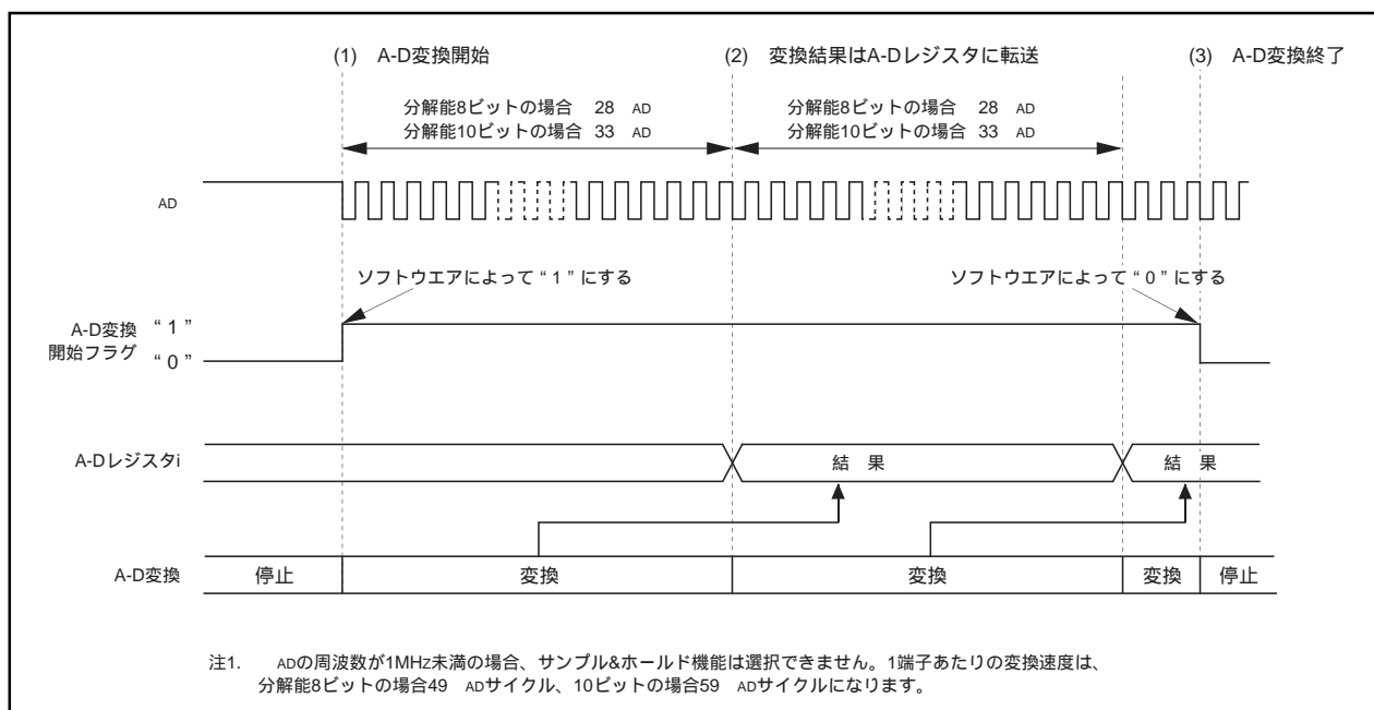
図1 繰り返しモード動作タイミング
