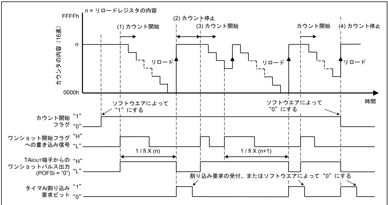
図1 ワンショットタイマモード動作タイミング
