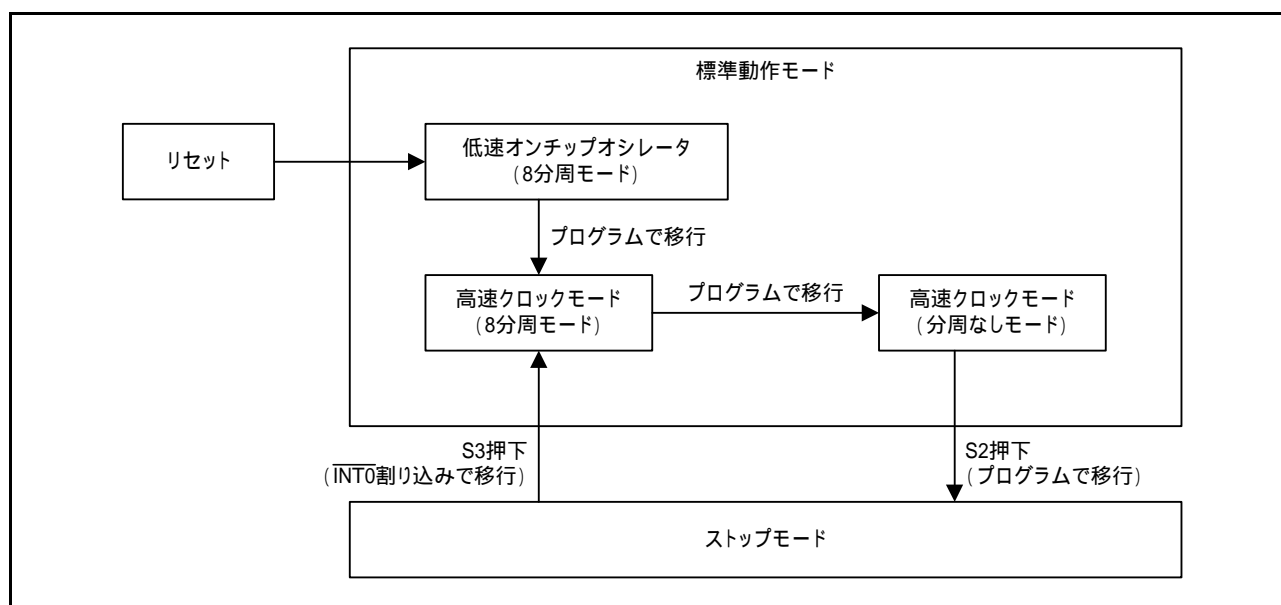
図 3.1 モードの遷移
