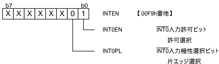
外部入力許可レジスタ
