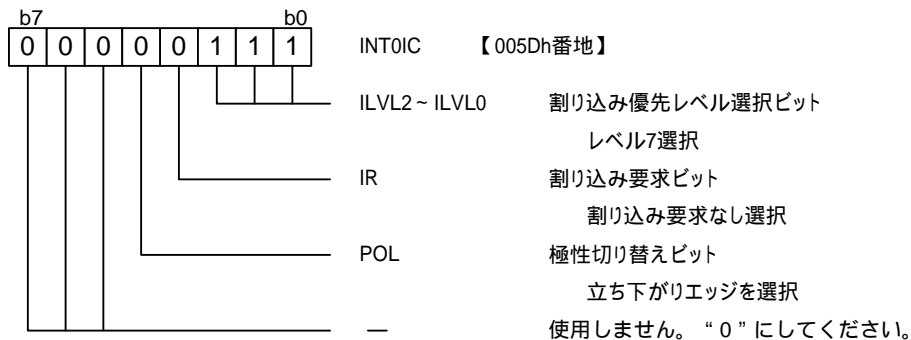
\overline{\text{INT0}} 割り込み制御レジスタ
