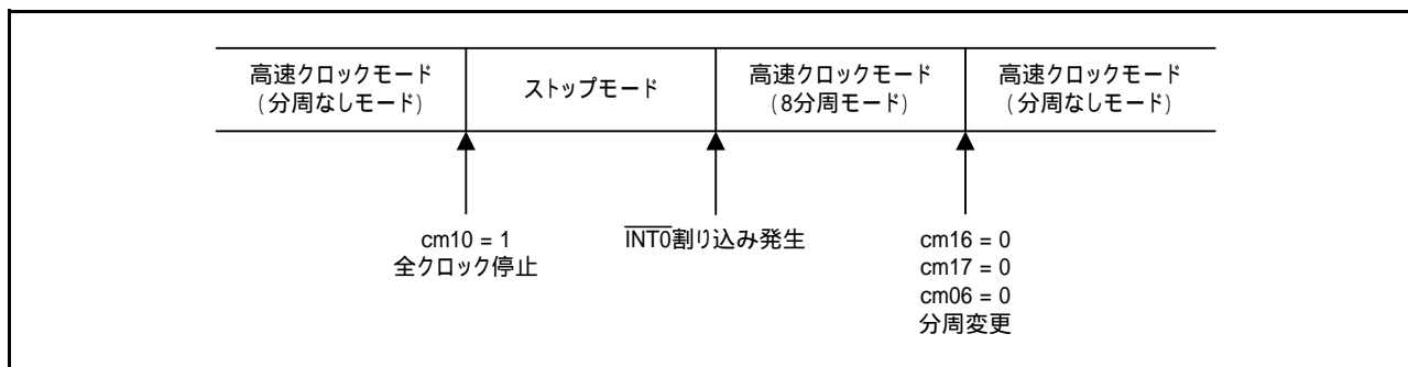
図 4.1 モード移行手順
