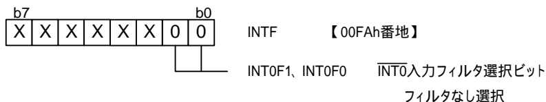
\overline{\text{INT}} 入力フィルタ選択レジスタ
