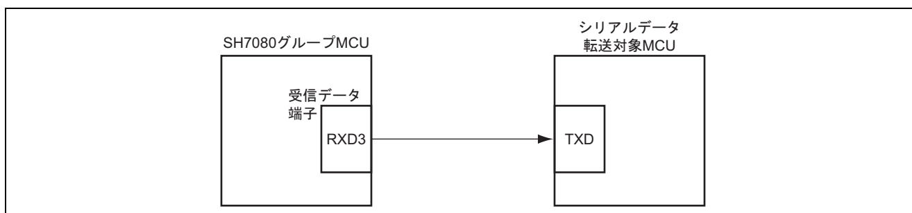
図 1 FIFO 付き調歩同期式シリアルデータ受信動作概要
