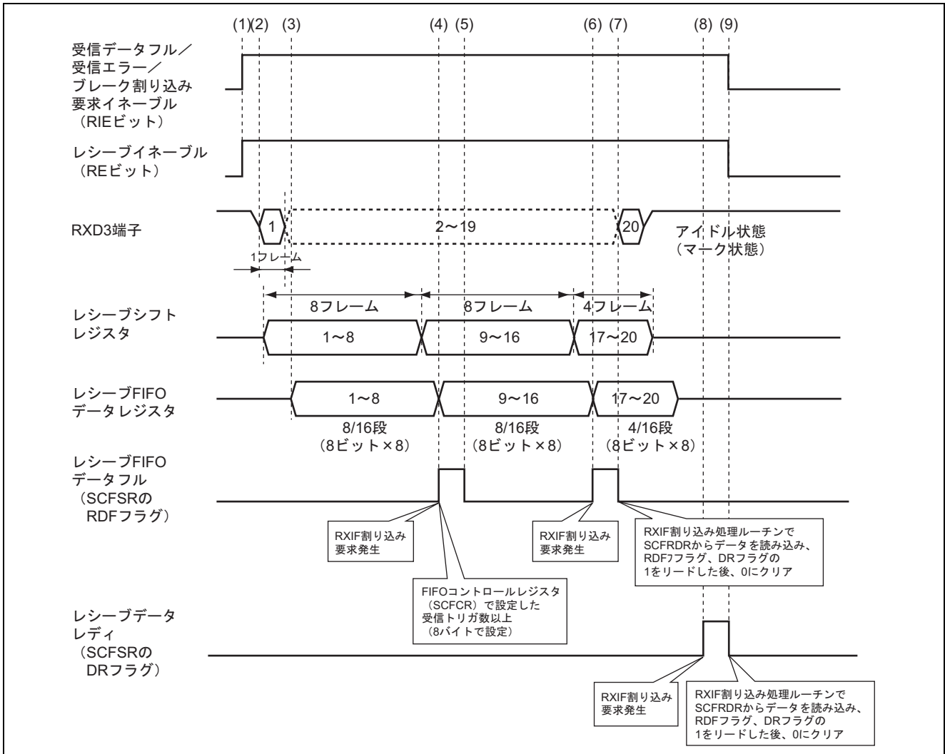
図3 動作説明
