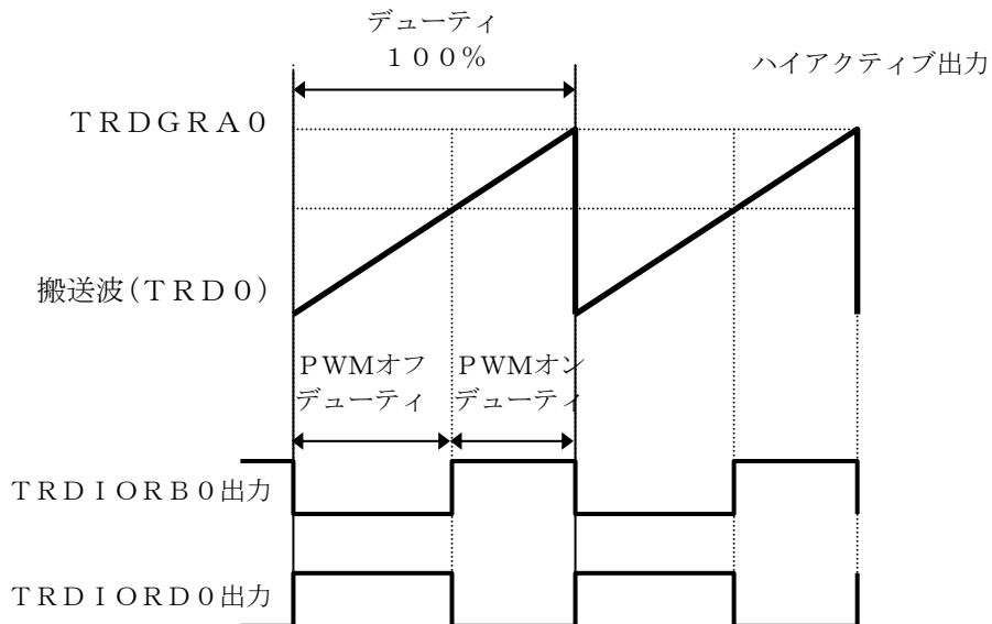
図 3.1.3 PWM出力方法
