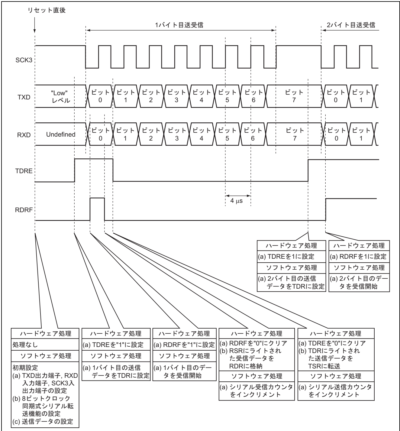
図3 クロック同期式シリアル同時送受信の動作原理
