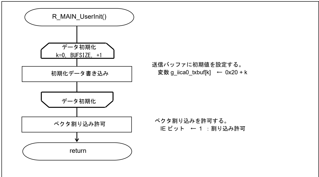
図 5.8 システムの初期化処理関数
