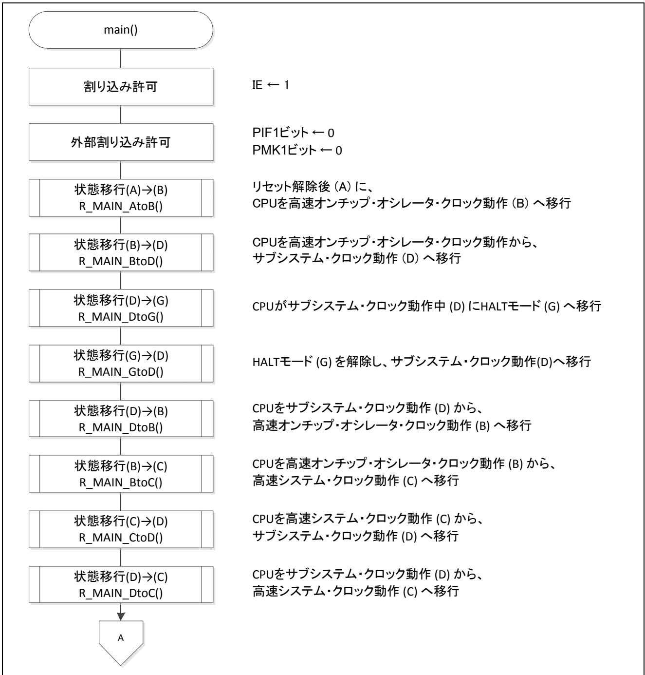
図 5.8 メイン処理(1/2)
