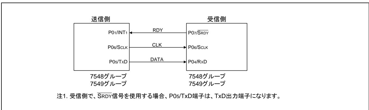
図 3.1 接続図
