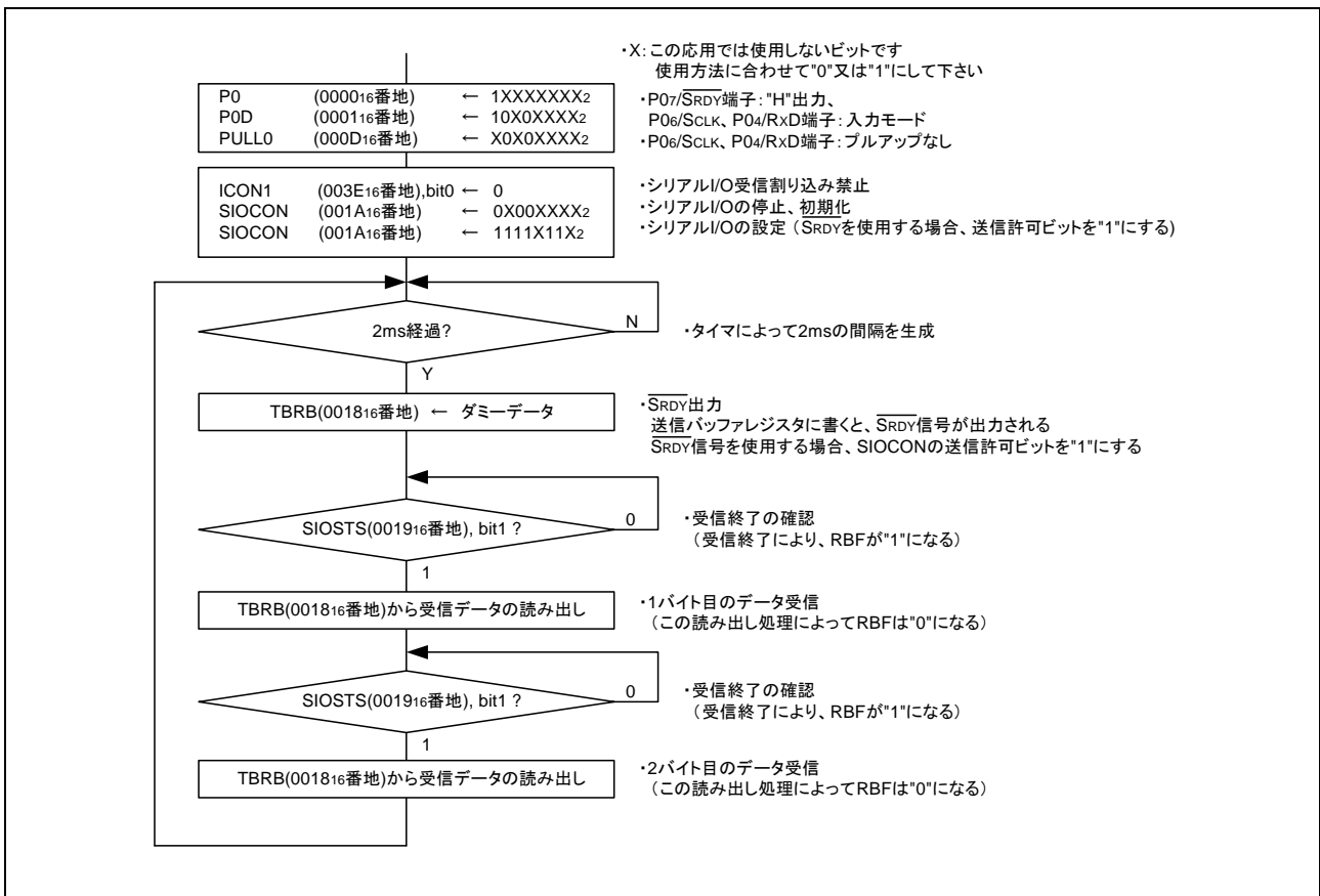
図 3.6 受信側の制御手順
