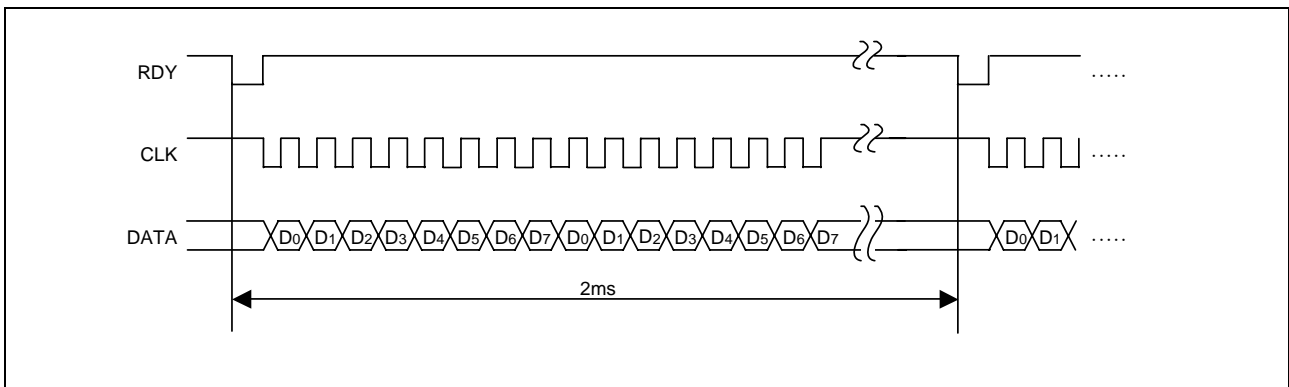
図 3.2 タイミング図
