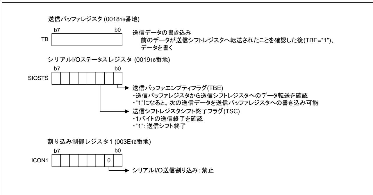
図 3.3 送信側関連レジスタの設定
