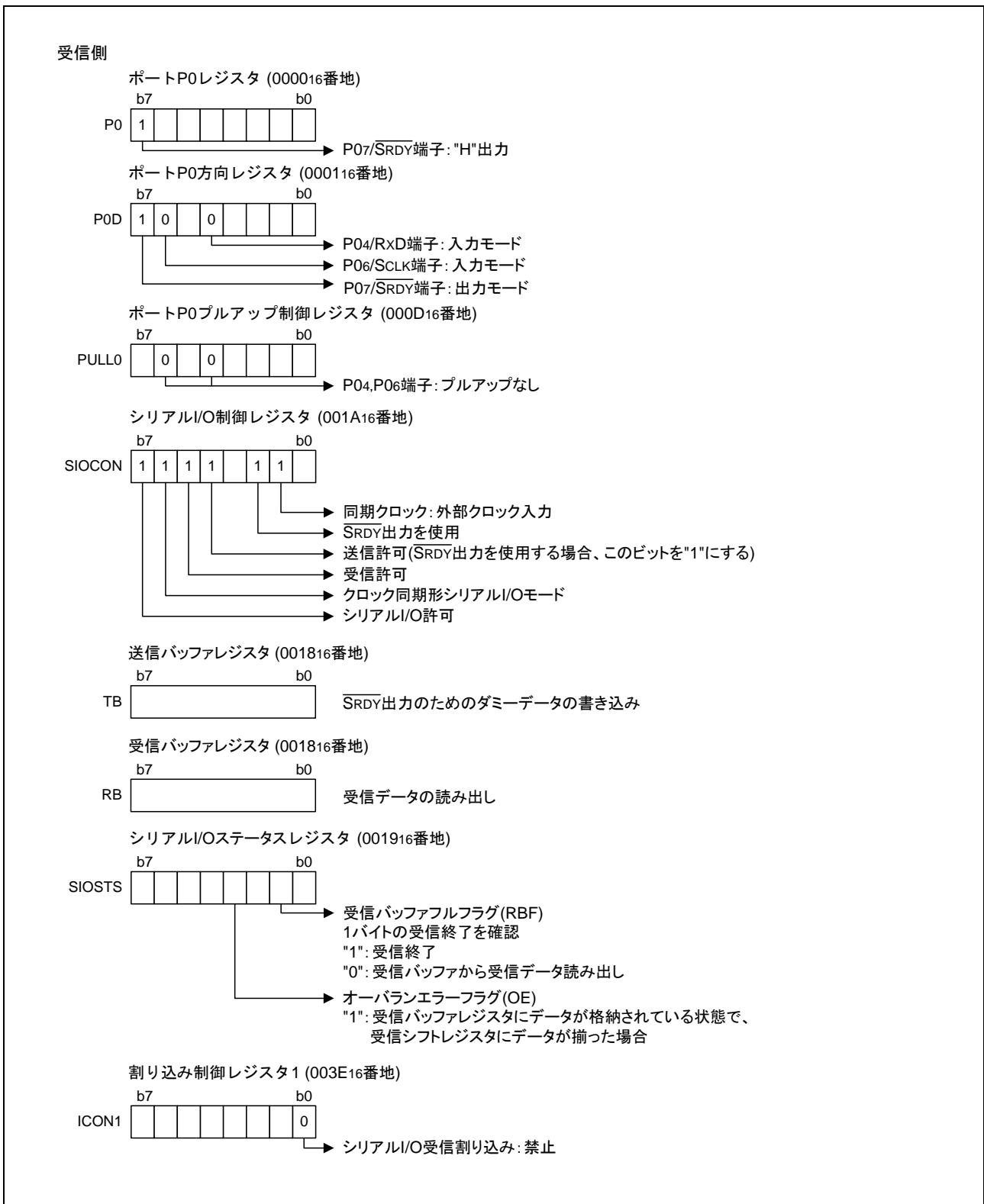
図 3.4 受信側関連レジスタの設定
