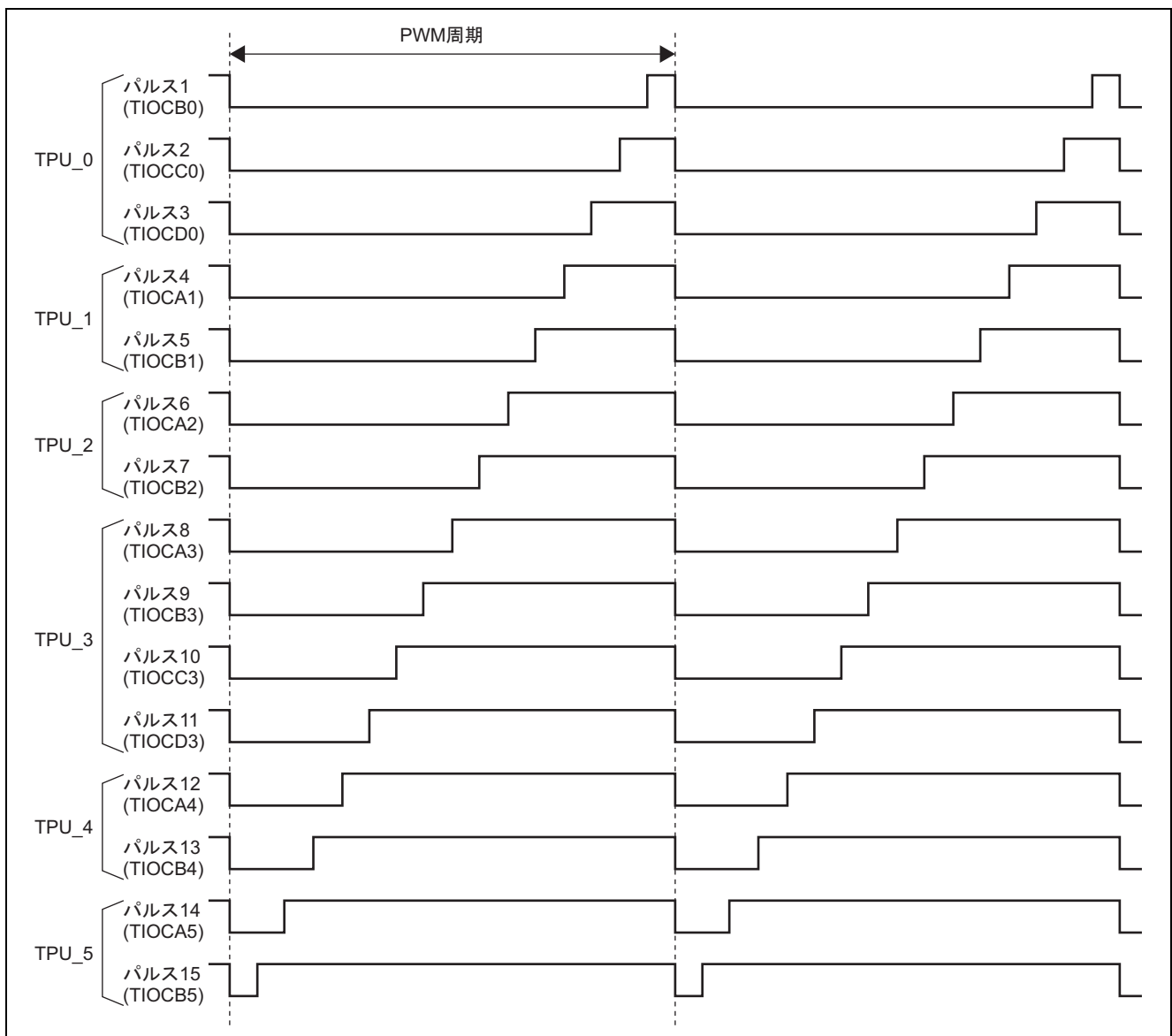
図1 PWM15 相出力例
