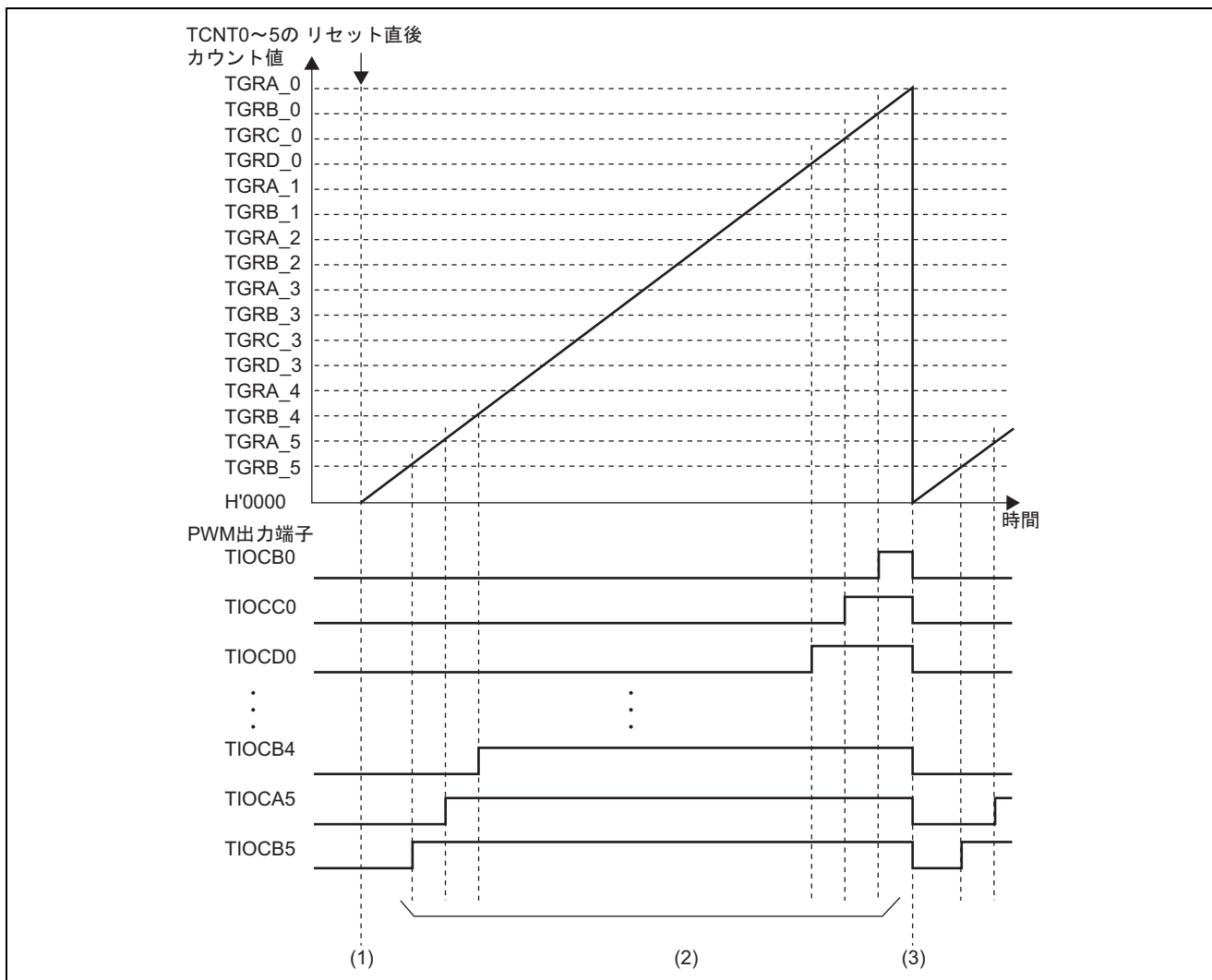
図3 PWM15 相出力動作説明
