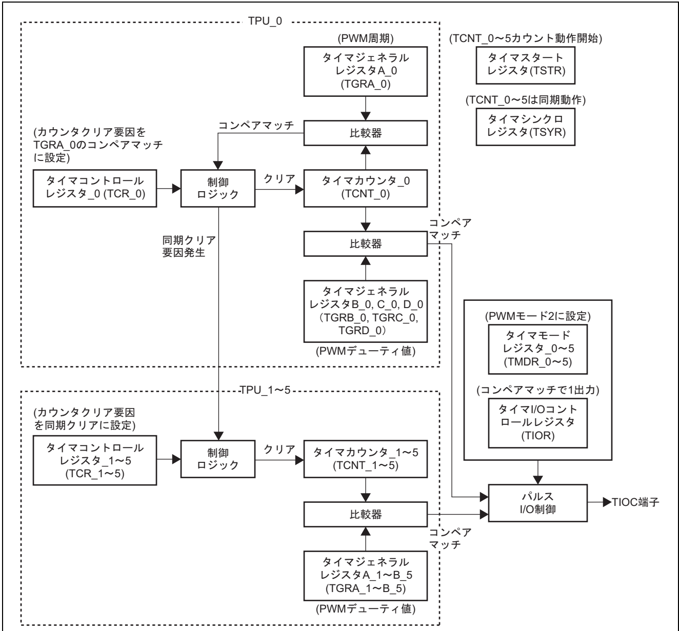
図2 PWM15 相出力ブロック図
