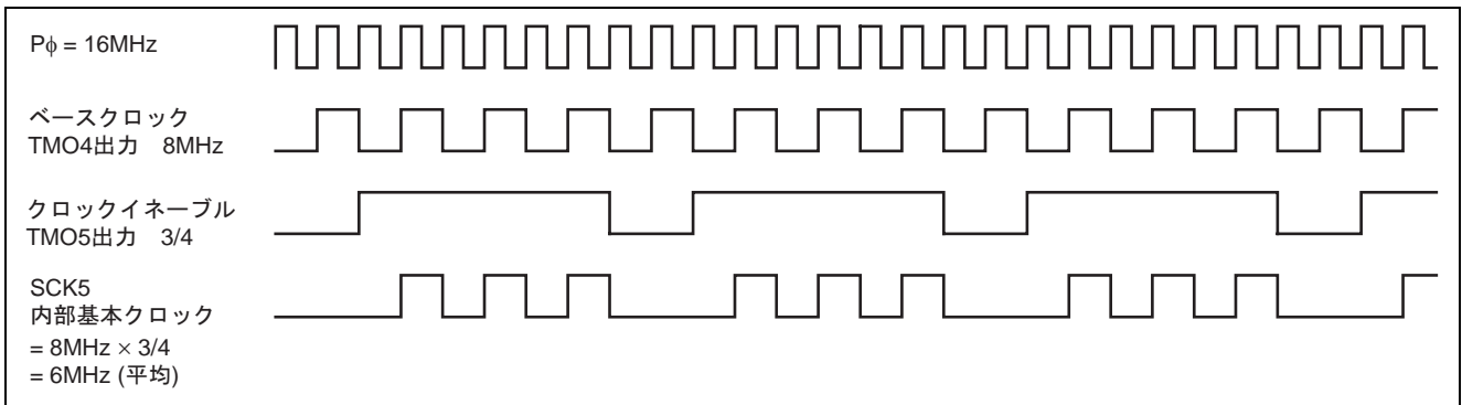
図 7 SCK5 内部基本クロック波形
