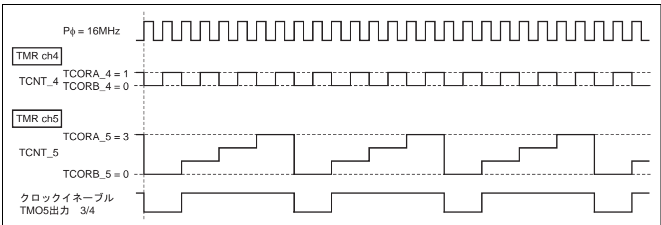
図 6 TMO5 の出力波形
