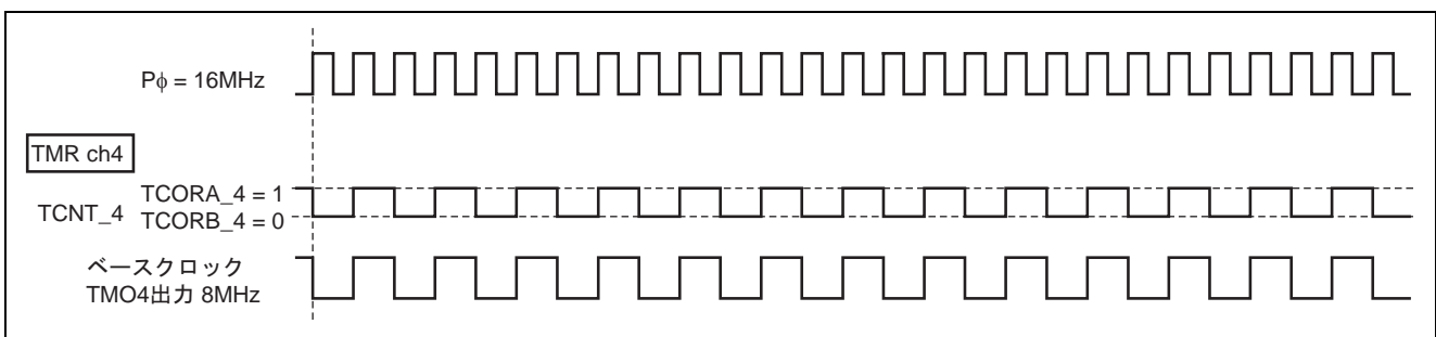
図 5 TMO4 の出力波形
