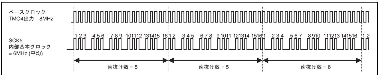
図 8 通信データの 1 ビット期間
