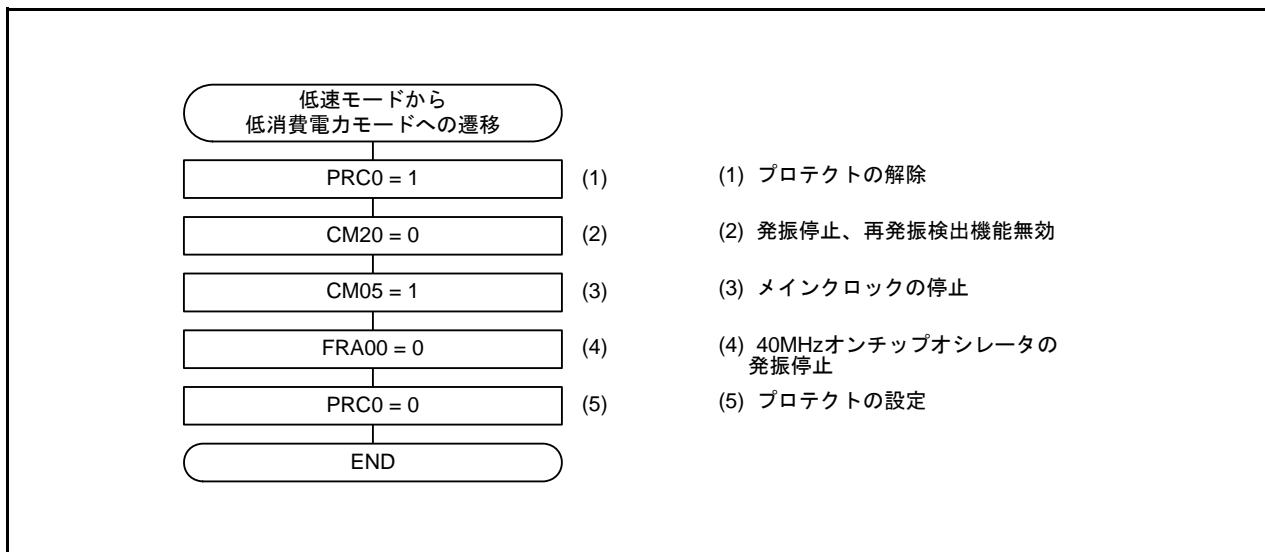
図3.4 低速モードから低消費電力モードに遷移する手順
