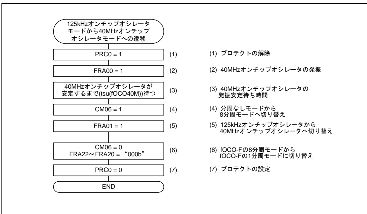
図3.7 125kHzオンチップオシレータモードから40MHzオンチップオシレータモードへの遷移
