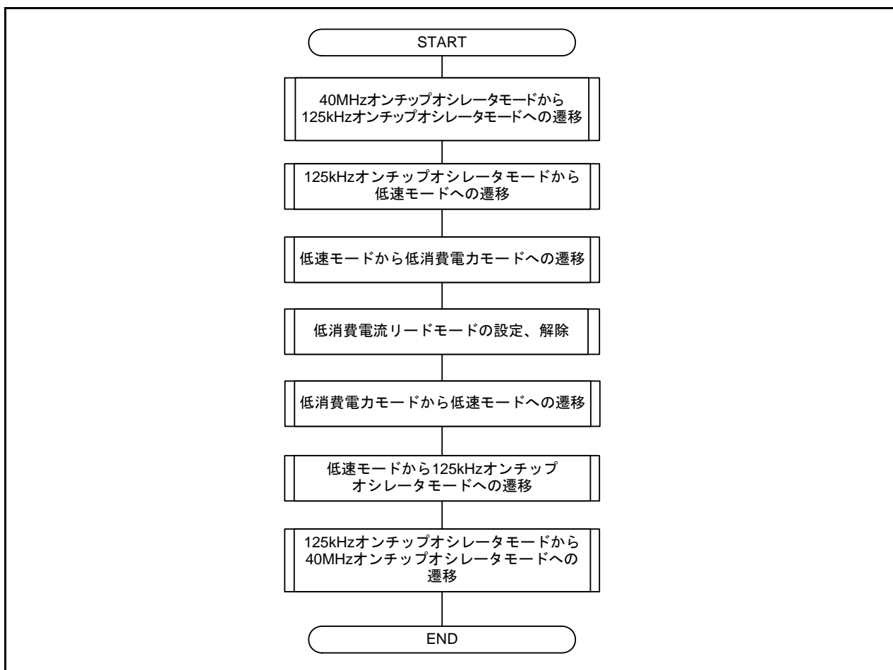
図3.1 40MHzオンチップオシレータモードと低消費電力モード間の遷移手順
