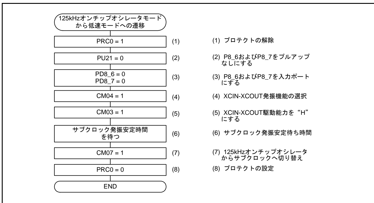
図3.3 125kHzオンチップオシレータモードから低速モードへの遷移
