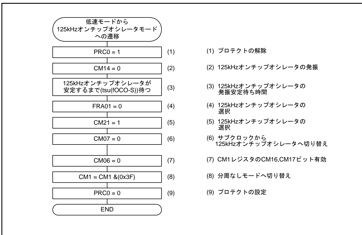
図3.6 低速モードから125kHzオンチップオシレータモードへの遷移
