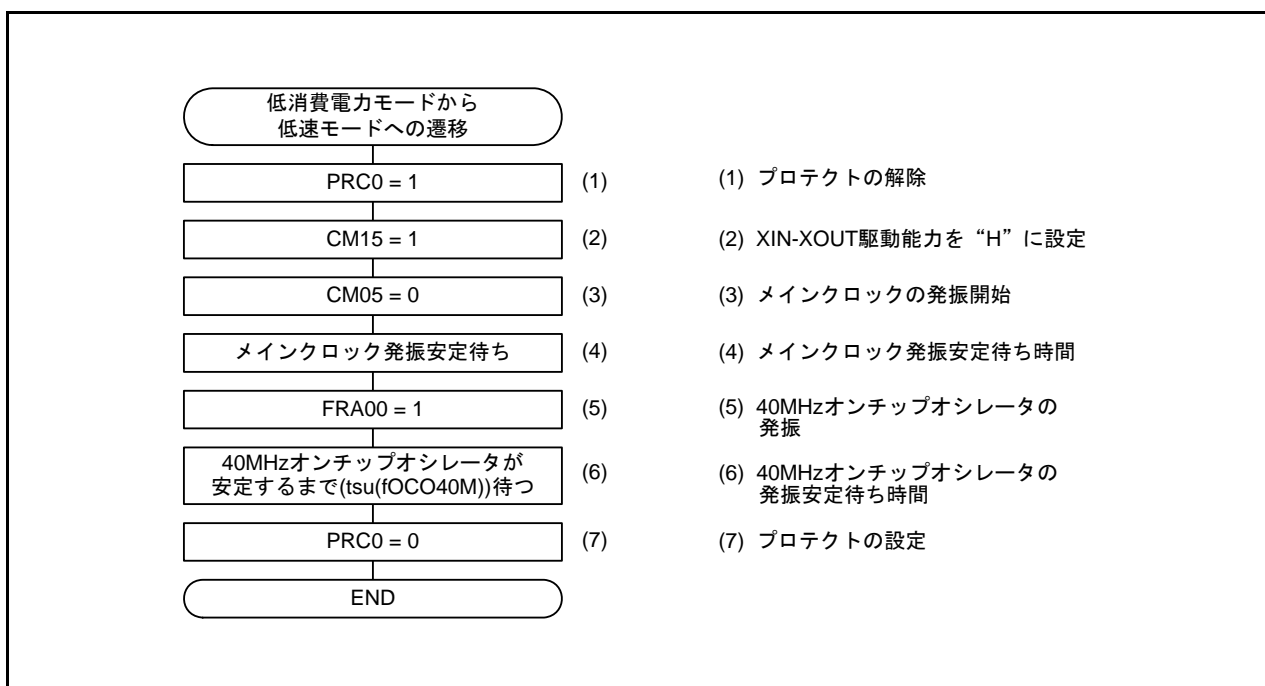
図3.5 低消費電力モードから低速モードに遷移する手順
