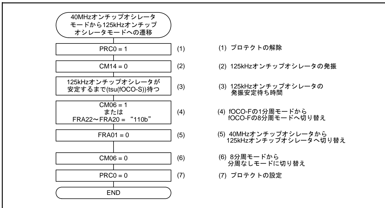
図3.2 40MHzオンチップオシレータモード(fOCO-Fの1分周)から125kHzオンチップオシレータモードへの遷移
