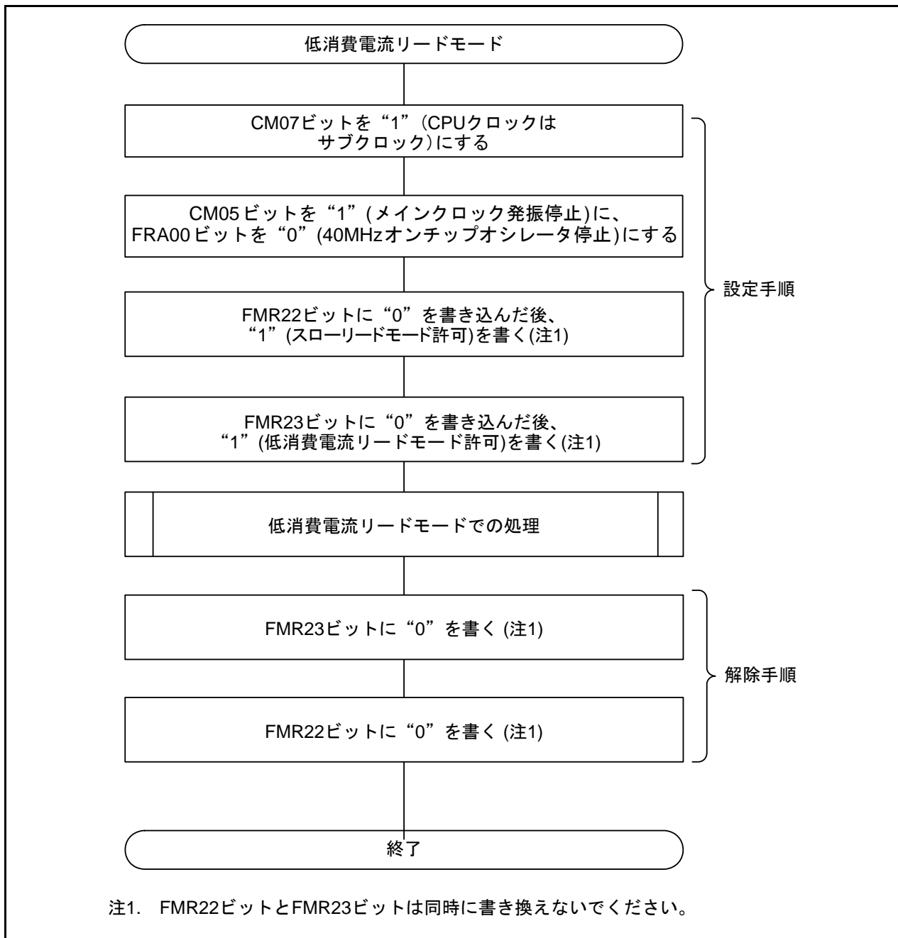
図3.8 低消費電流リードモードの設定、解除
