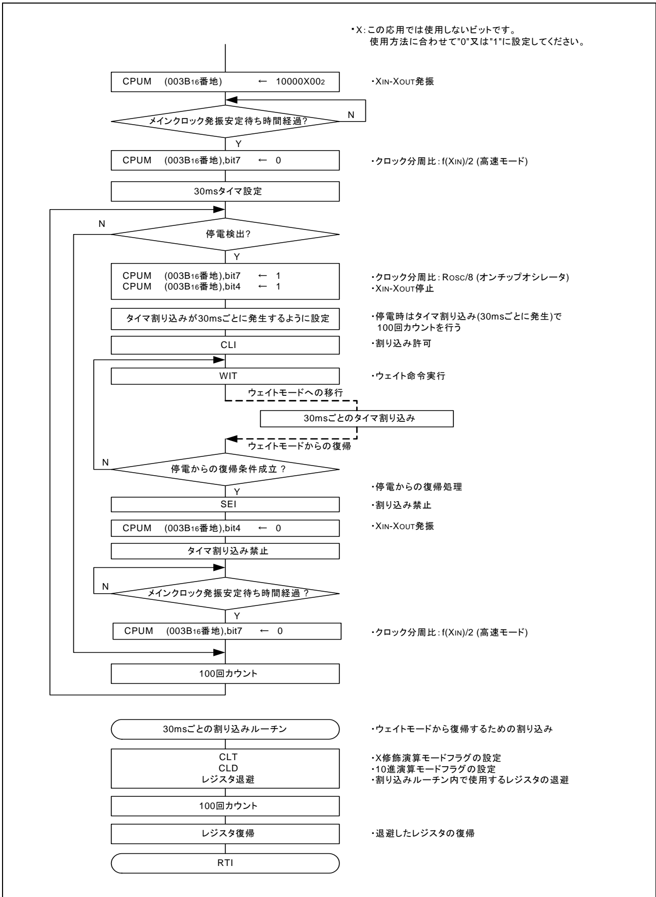
図 3.3 制御手順
