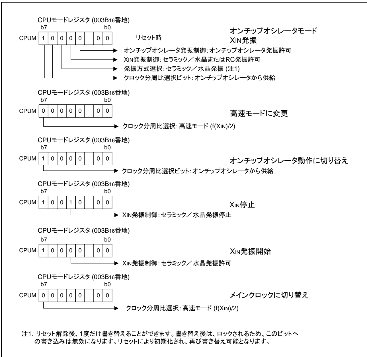
図 3.2 関連レジスタの設定
