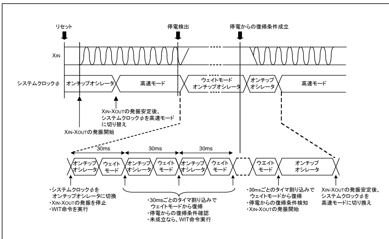
図 3.1 停電時のシステムクロック \phi のモード移行例
