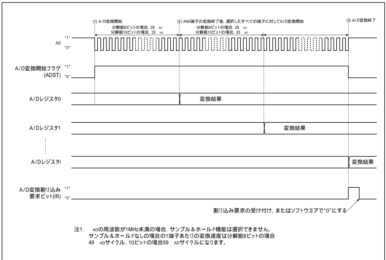
図 2 繰り返し掃引モード1の動作タイミング
